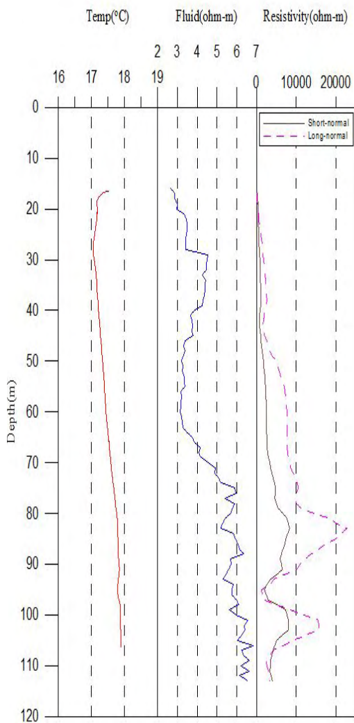
(a) 전기검층
