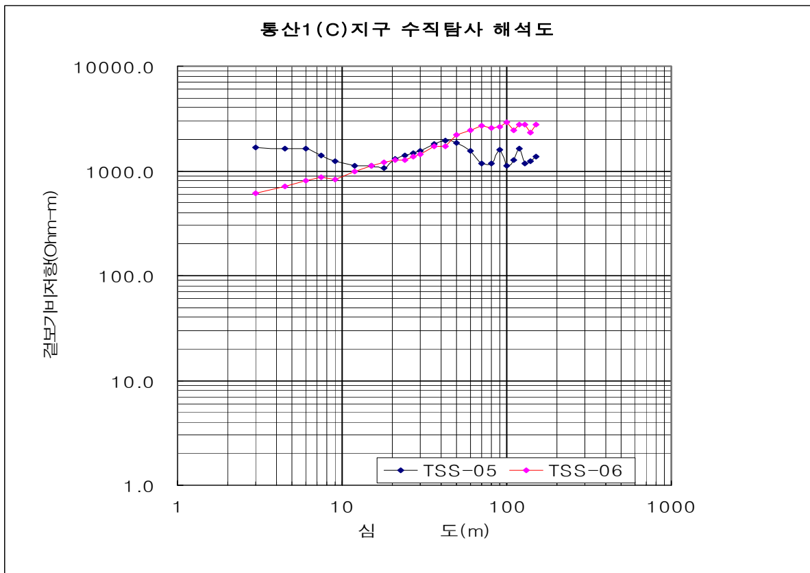
<TSS-05,06해석결과도>
