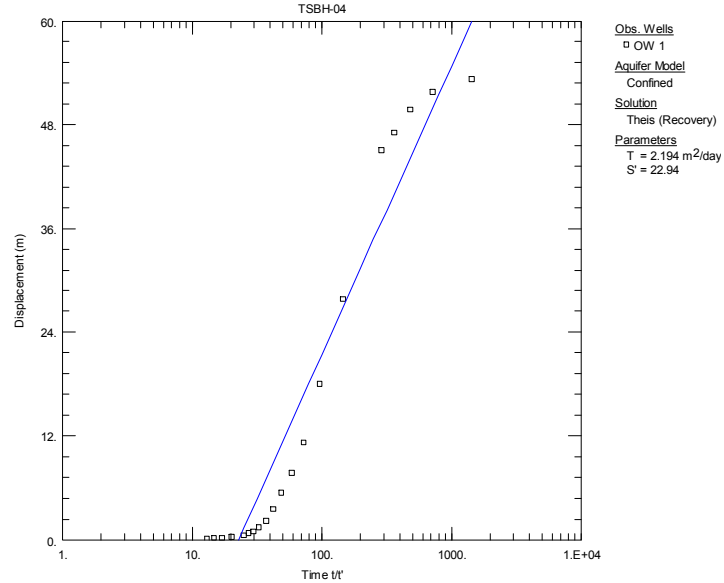
<그림 4-4-5> TSBH-04호공 양수시험 해석 결과도
