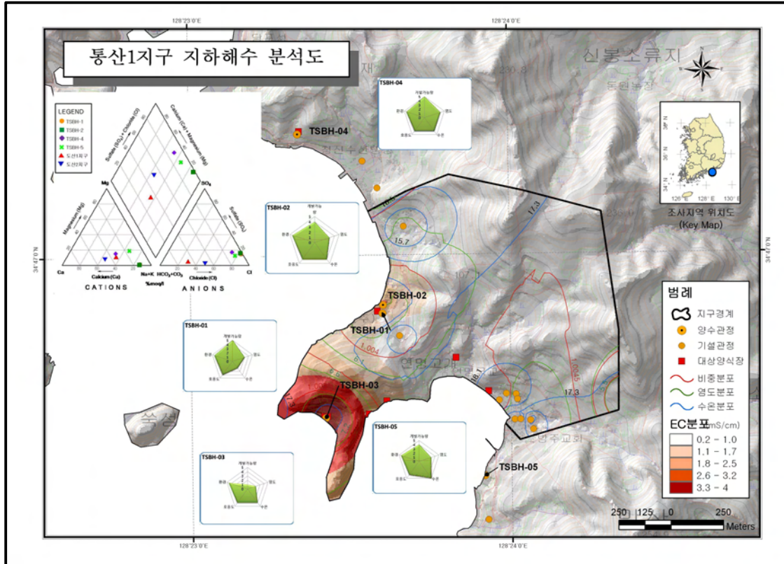
<그림 5-2-9> 통산1지구 지하해수 조사 분석도
