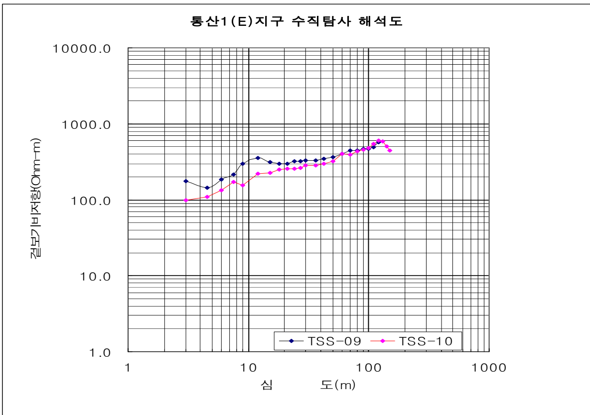
<TSS-09,10해석결과도>
