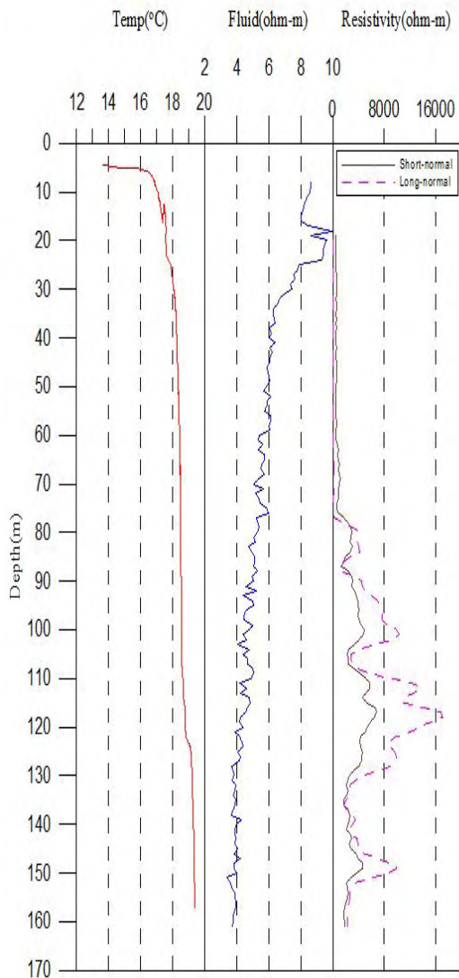
(a) 전기검층
