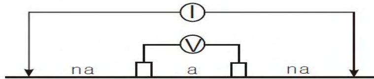
<그림 4-1-1> 슬럼버저배열 전기비저항 수직탐사 측선도
