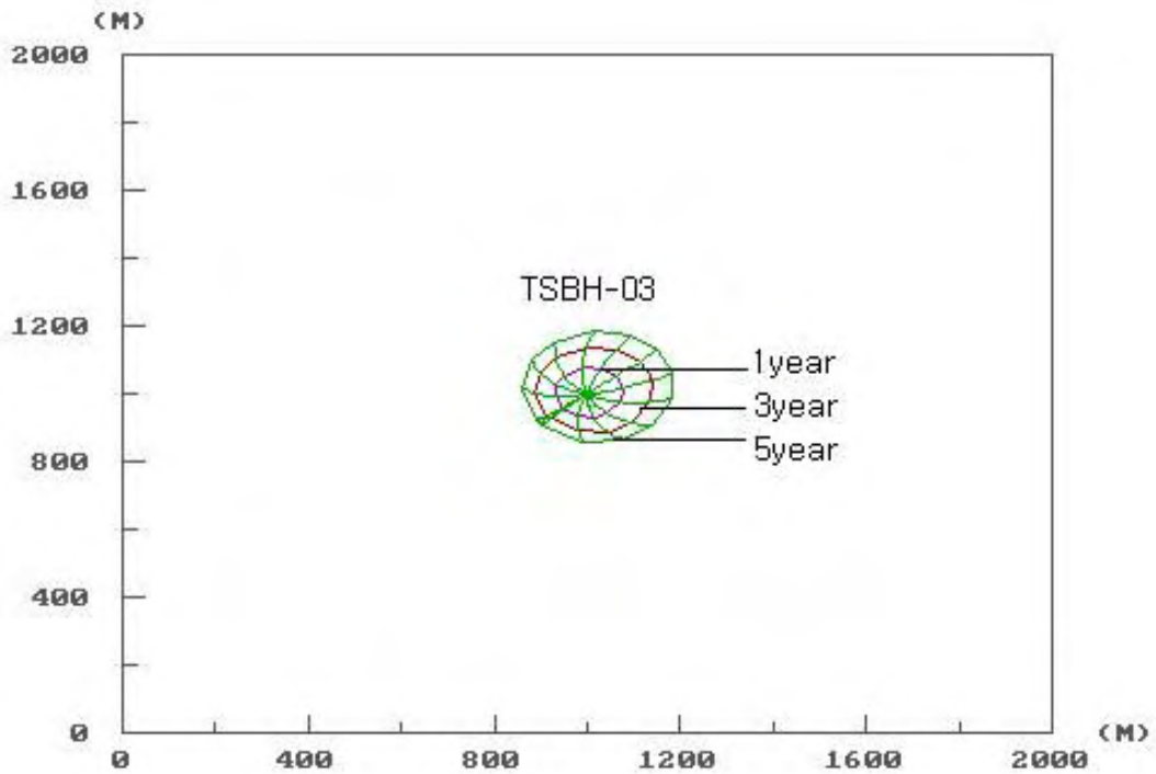
<그림 4-4-9> TSBH-03호공 포획구간
