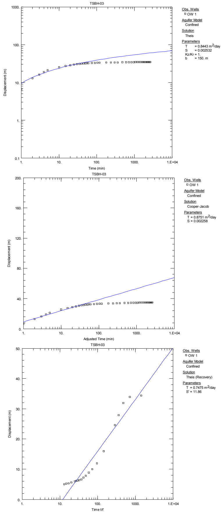
<그림 4-4-4> TSBH-03호공 양수시험 해석 결과도
