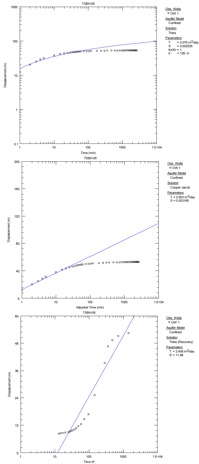
<그림 4-4-6> TSBH-05호공 양수시험 해석 결과도
