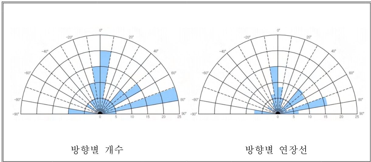
<그림 2-3-3> 통산1지구 선형구조의 방향별 특성
