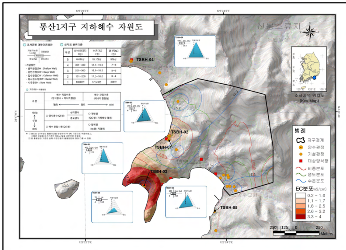
<그림 5-2-10> 통산1지구 지하해수 자원도
