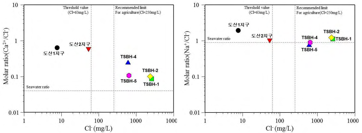
<그림 4-5-5> Ca/Cl, Na/Cl 몰비와 Cl이온 간의 상관관계
