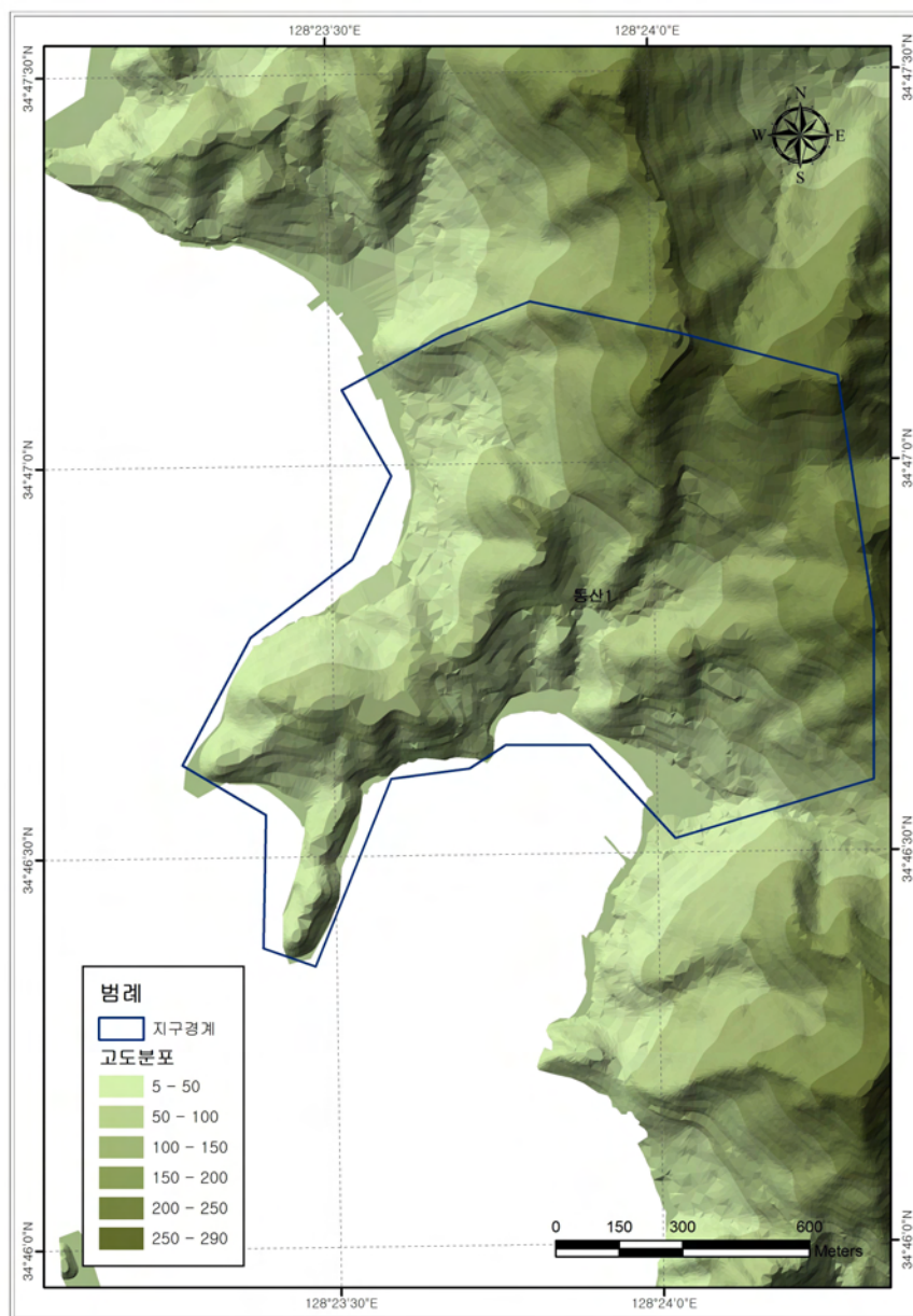
<그림 2-3-1> 통산1지구 지형고도
