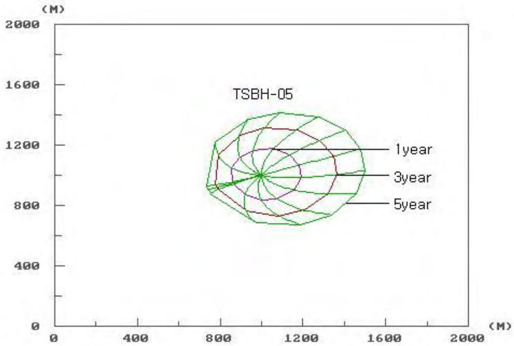
<그림 4-4-11> TSBH-05호공 포획구간
