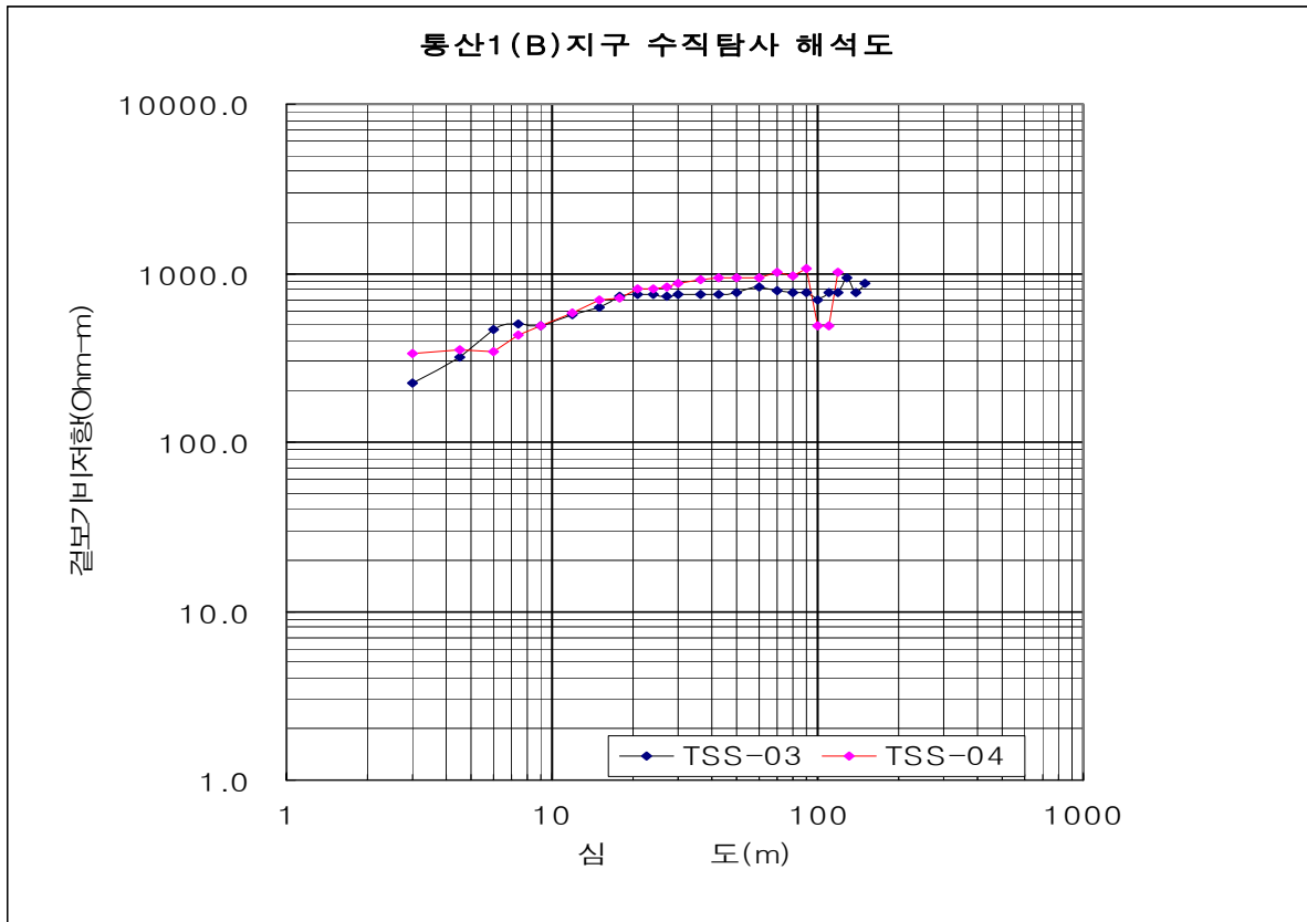
<TSS-03,04해석결과도>
