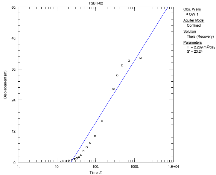
<그림 4-4-3> TSBH-02호공 양수시험 해석 결과도
