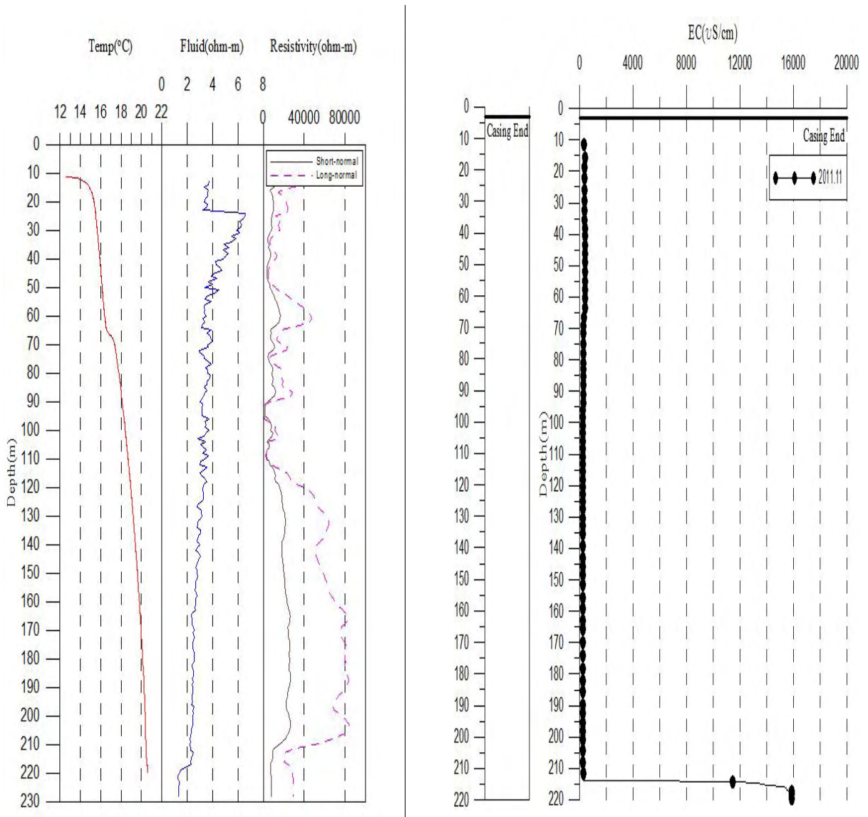
(a) 전기검층
