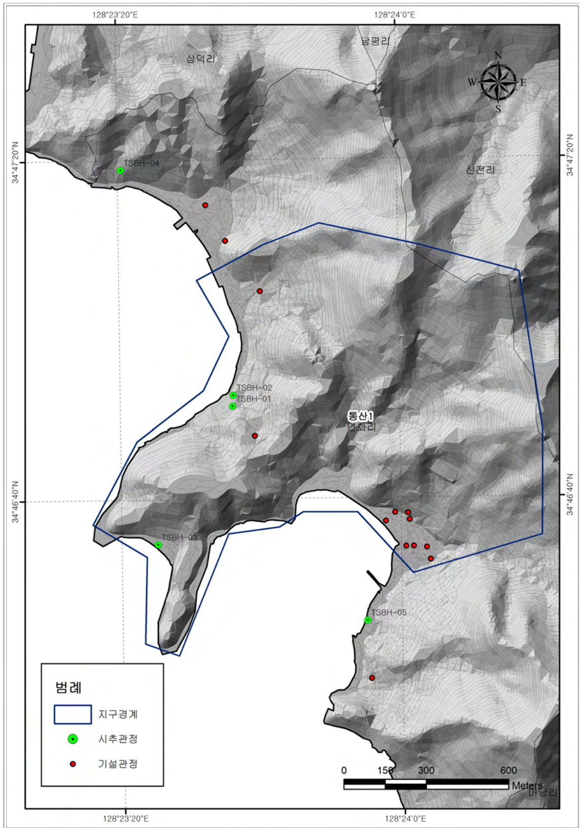
<그림 4-5-2> 통산1지구 기설관정 및 시추조사공 간이수질 측정위치도
