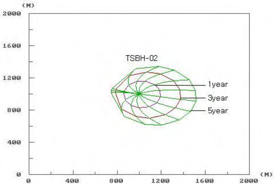
<그림 4-4-8> TSBH-02호공 포획구간
