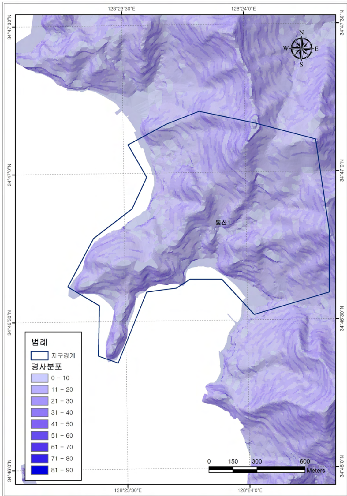
<그림 2-3-2> 통산1지구 지형경사
