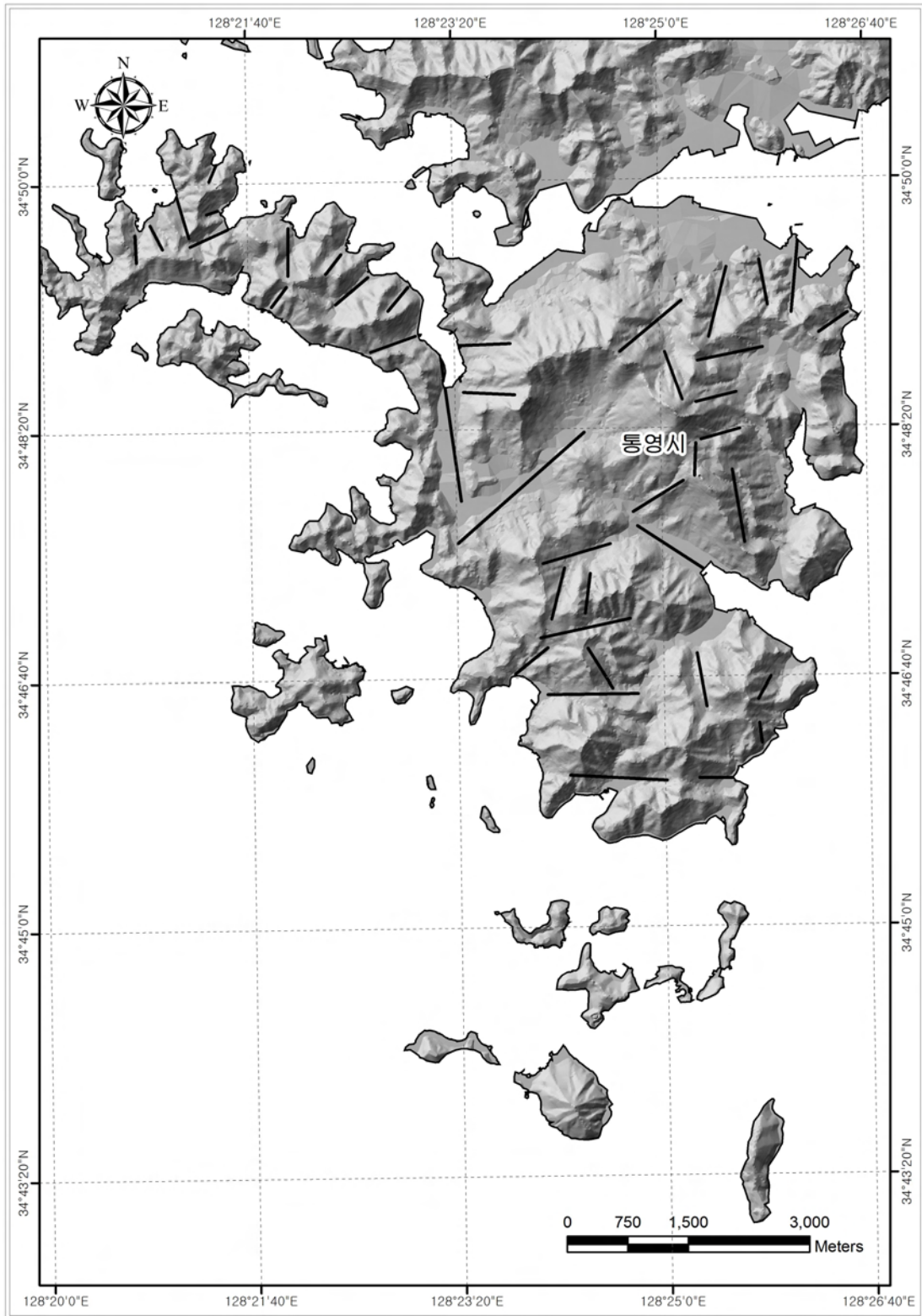
<그림 2-3-4> 통산1지구 선형구조(lineament) 분포도
