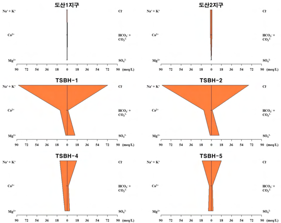
<그림 4-5-4> 통산1지구 지하수의 Stiff diagram
