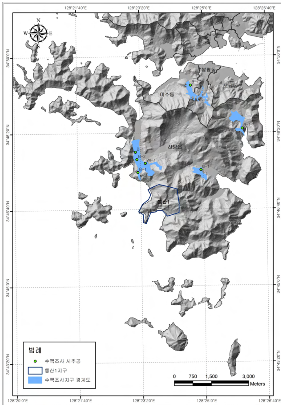
<그림 2-4-1> 통영시 산양읍의 지하수 기초조사 현황도
