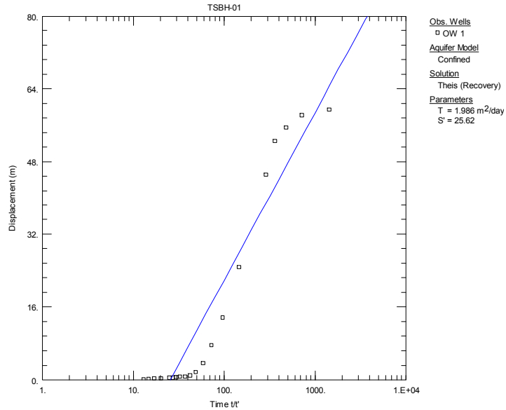
<그림 4-4-2> TSBH-01호공 양수시험 해석 결과도
