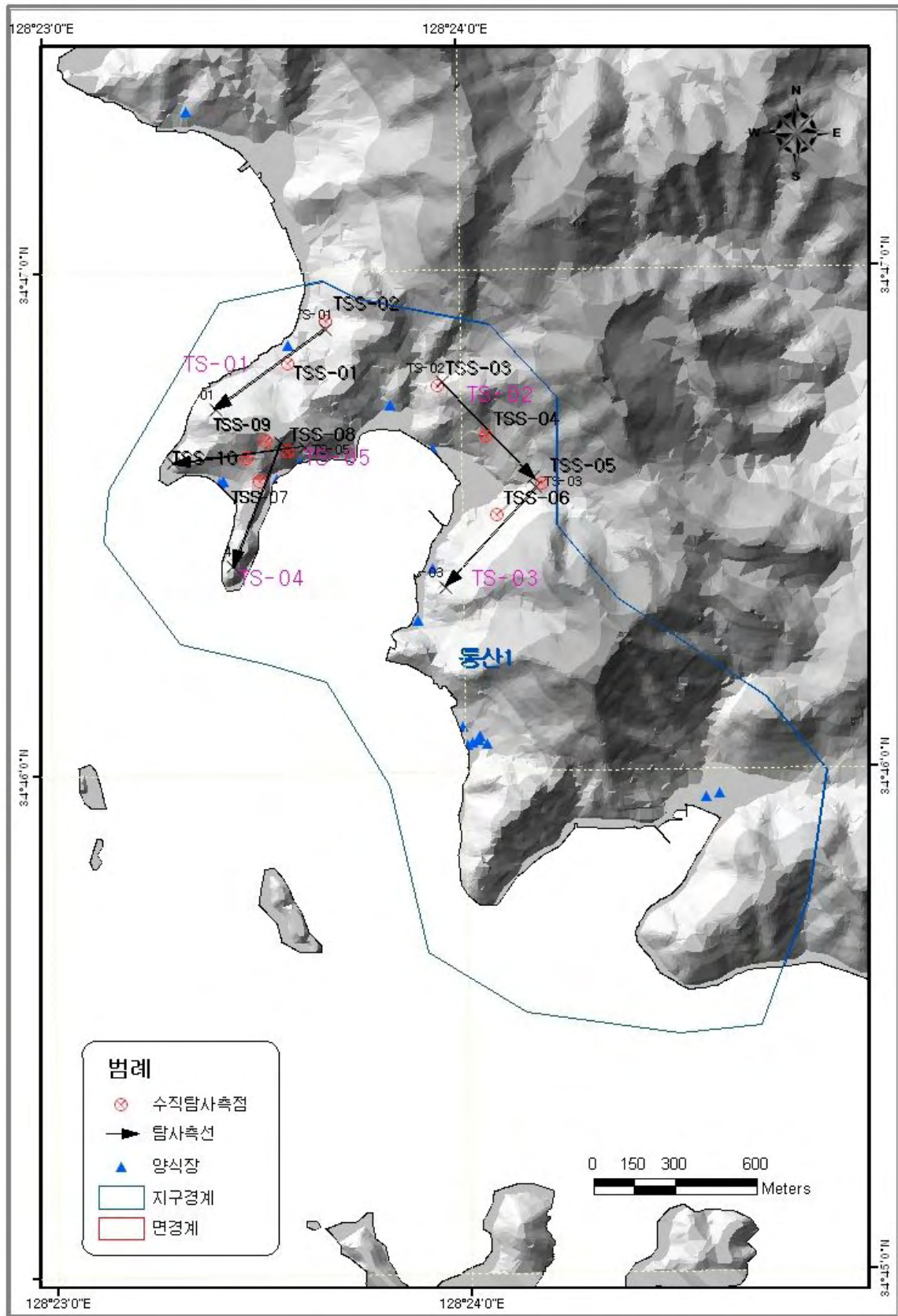
<그림 4-1-2> 통산1지구 물리탐사 측선 위치도
