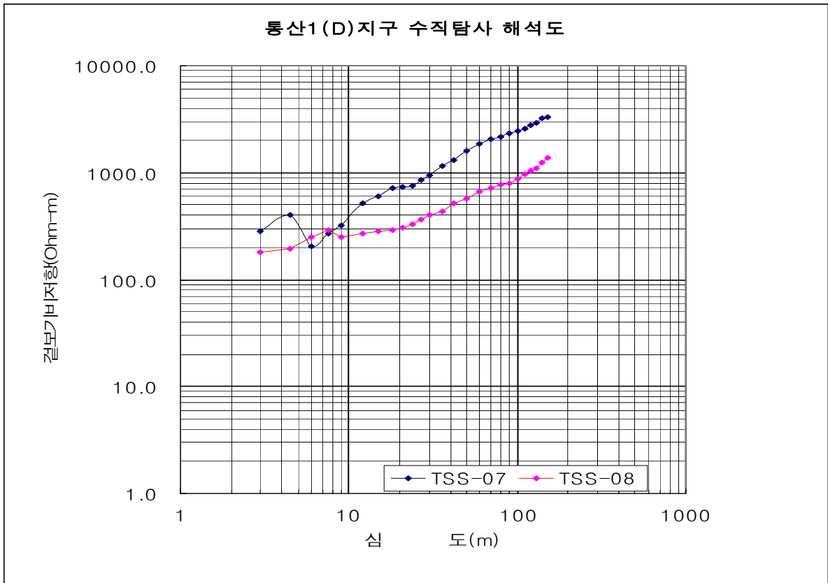
<TSS-07,08해석결과도>
