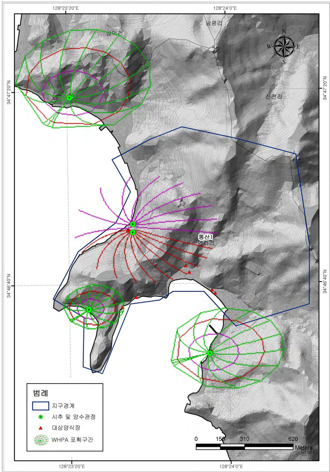
<그림 4-4-13> 조사공별 포획구간 현황도
