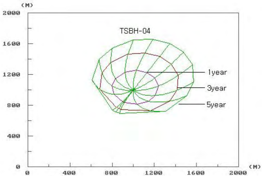
<그림 4-4-10> TSBH-04호공 포획구간
