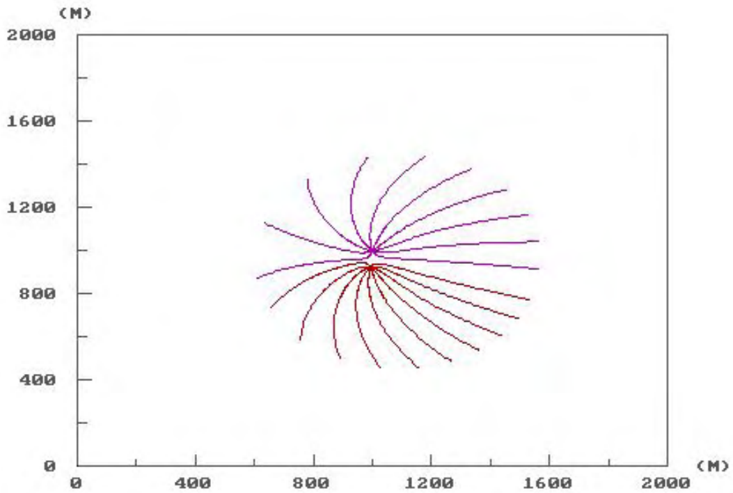
<그림 4-4-12> TSBH-01, 02호공 포획구간(GPTRAC방법)
