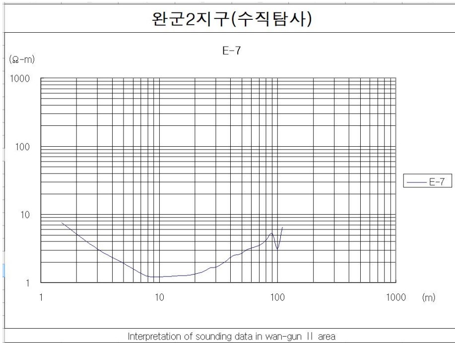
<그림 4-1-19> WG2-07 수직탐사 결과
