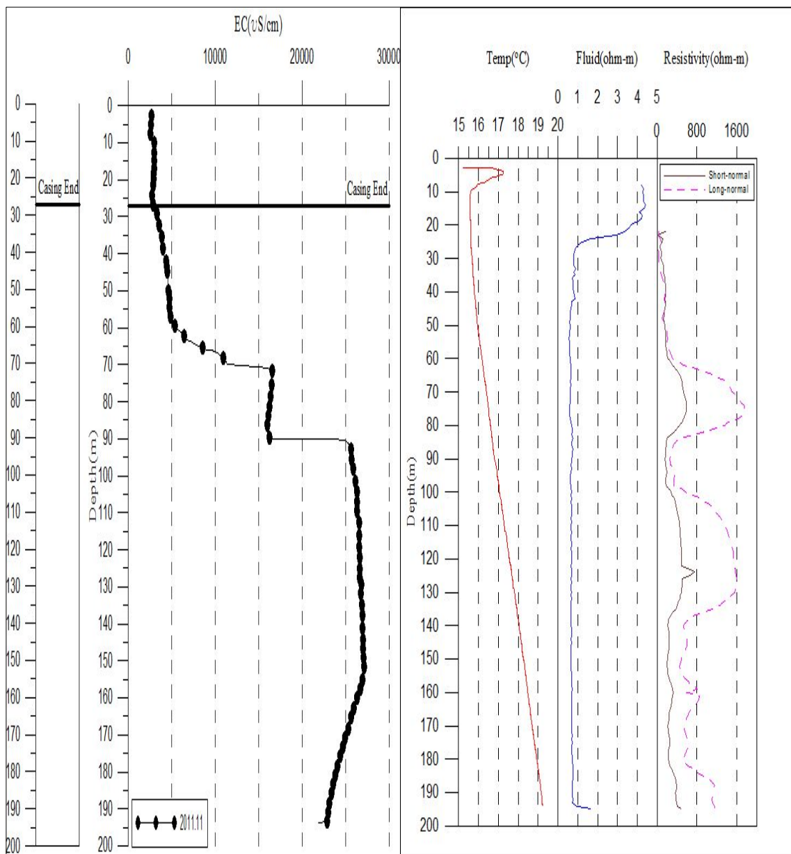
<그림 4-3-2> WG2BH-01호공의 물리검층 결과 그래프
