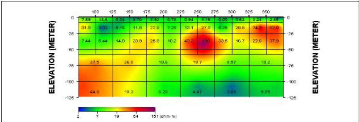
<그림 4-1-11> WG2-07 전기비저항탐사 단면도
