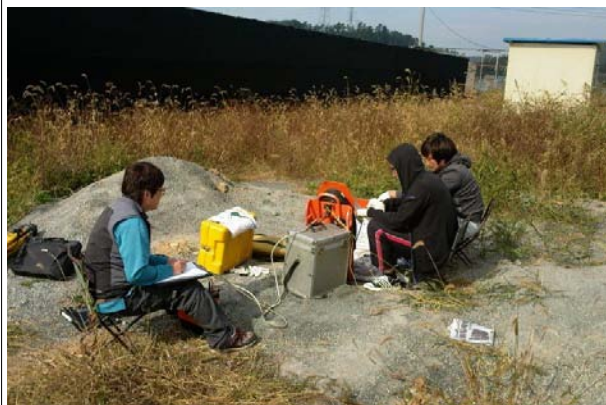
완군2지구 BH-1호공 물리검층 전경
