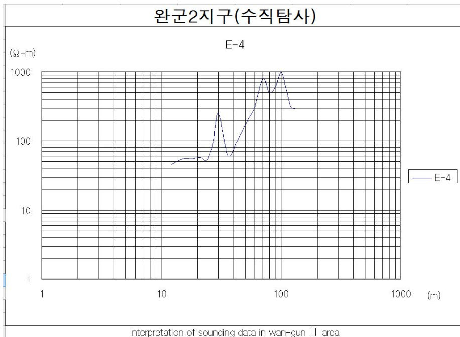
<그림 4-1-16> WG2-04 수직탐사 결과
