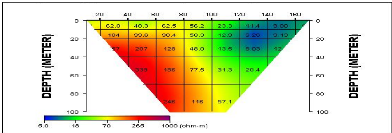
<그림 4-1-6> WG2-02 전기비저항탐사 단면도
