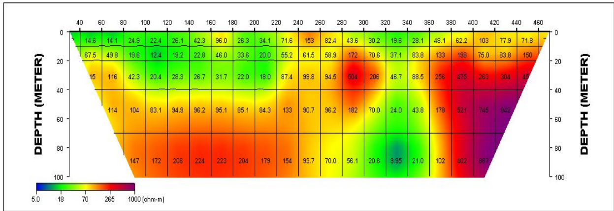
<그림 4-1-5> WG2-01 전기비저항탐사 단면도
