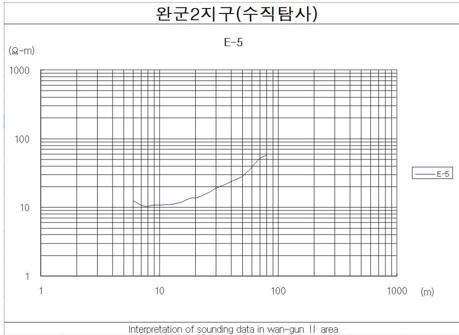
<그림 4-1-17> WG2-05 수직탐사 결과
