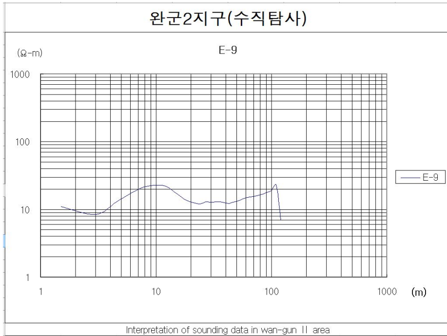
<그림 4-1-21> WG2-09 수직탐사 결과
