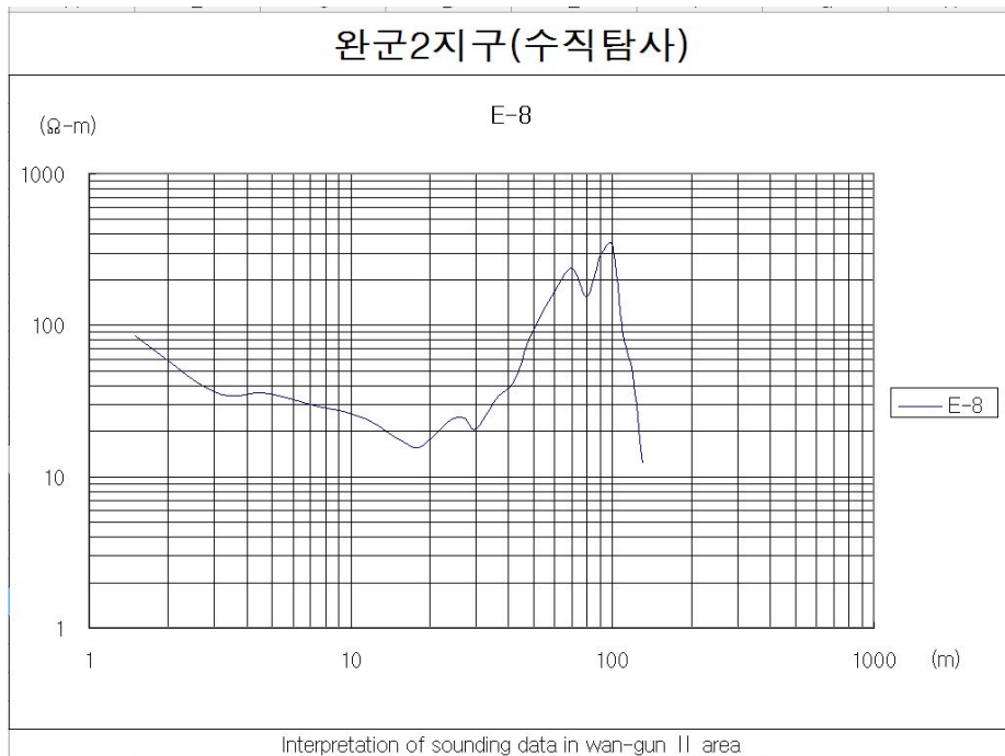
<그림 4-1-20> WG2-08 수직탐사 결과
