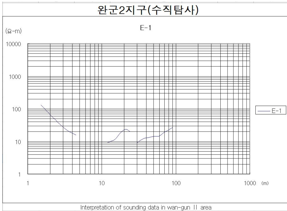
<그림 4-1-13> WG2-01 수직탐사 결과
