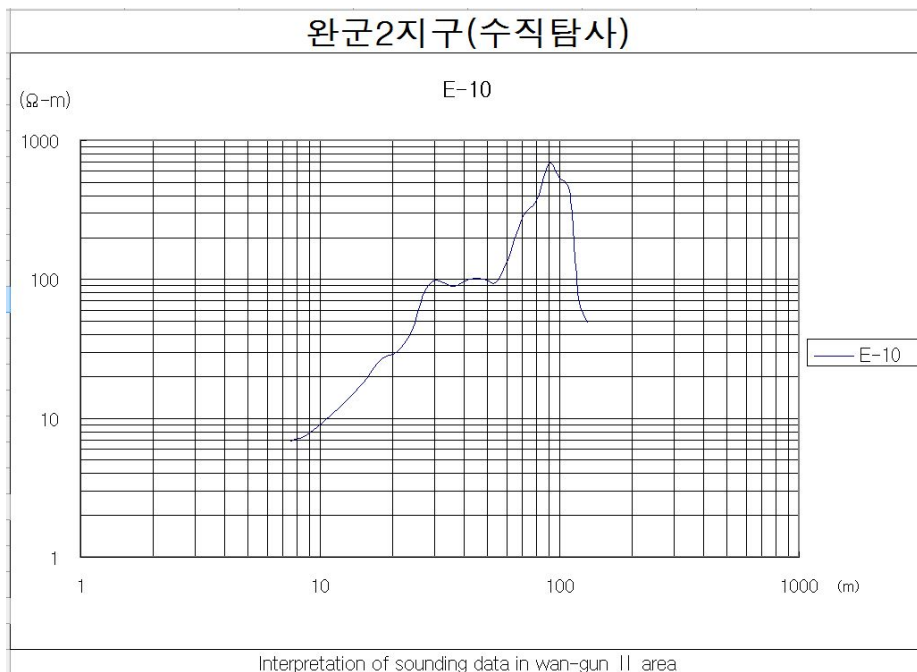
<그림 4-1-22> WG2-10 수직탐사 결과
