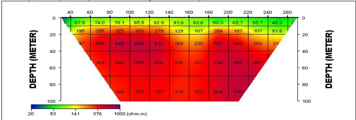
<그림4-1-7> WG2-03 전기비저항탐사 단면도
