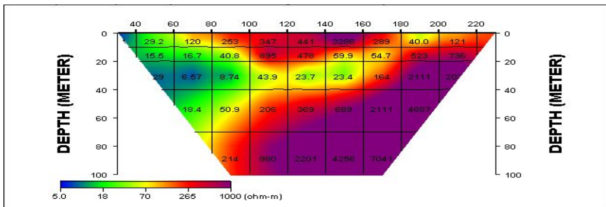
<그림 4-1-10> WG2-06 전기비저항탐사 단면도
