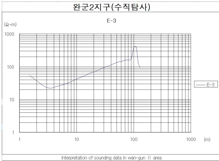
<그림 4-1-15> WG2-03 수직탐사 결과
