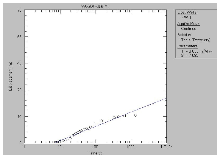
<그림 4-4-3> WG2BH-03호공 양수시험 해석 결과도
