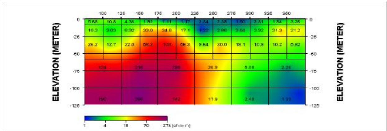
<그림 4-1-12> WG2-08 전기비저항탐사 단면도
