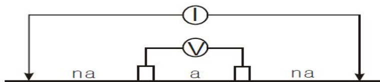
<그림 4-1-2> 슬럼버저배열 전기비저항 수직탐사 측선도
