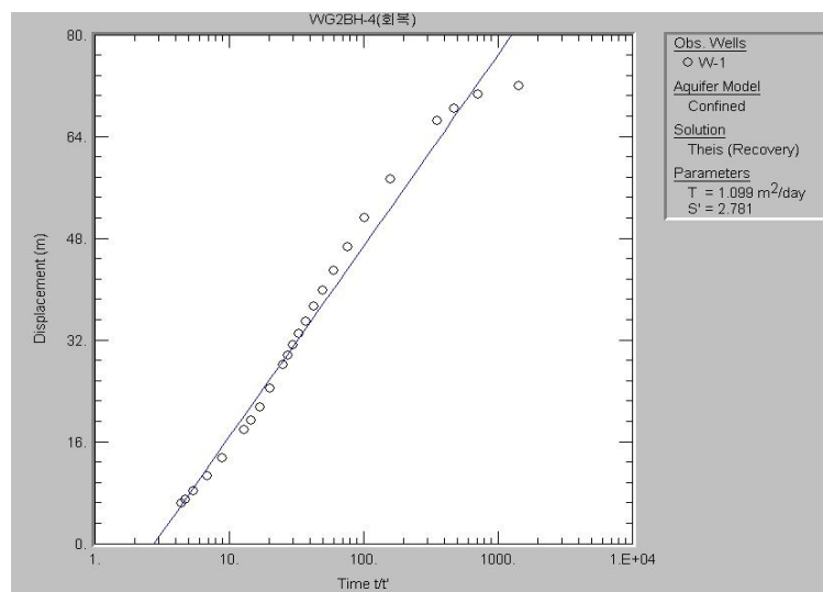
<그림 4-4-4> WG2BH-04호공 양수시험 해석 결과도
