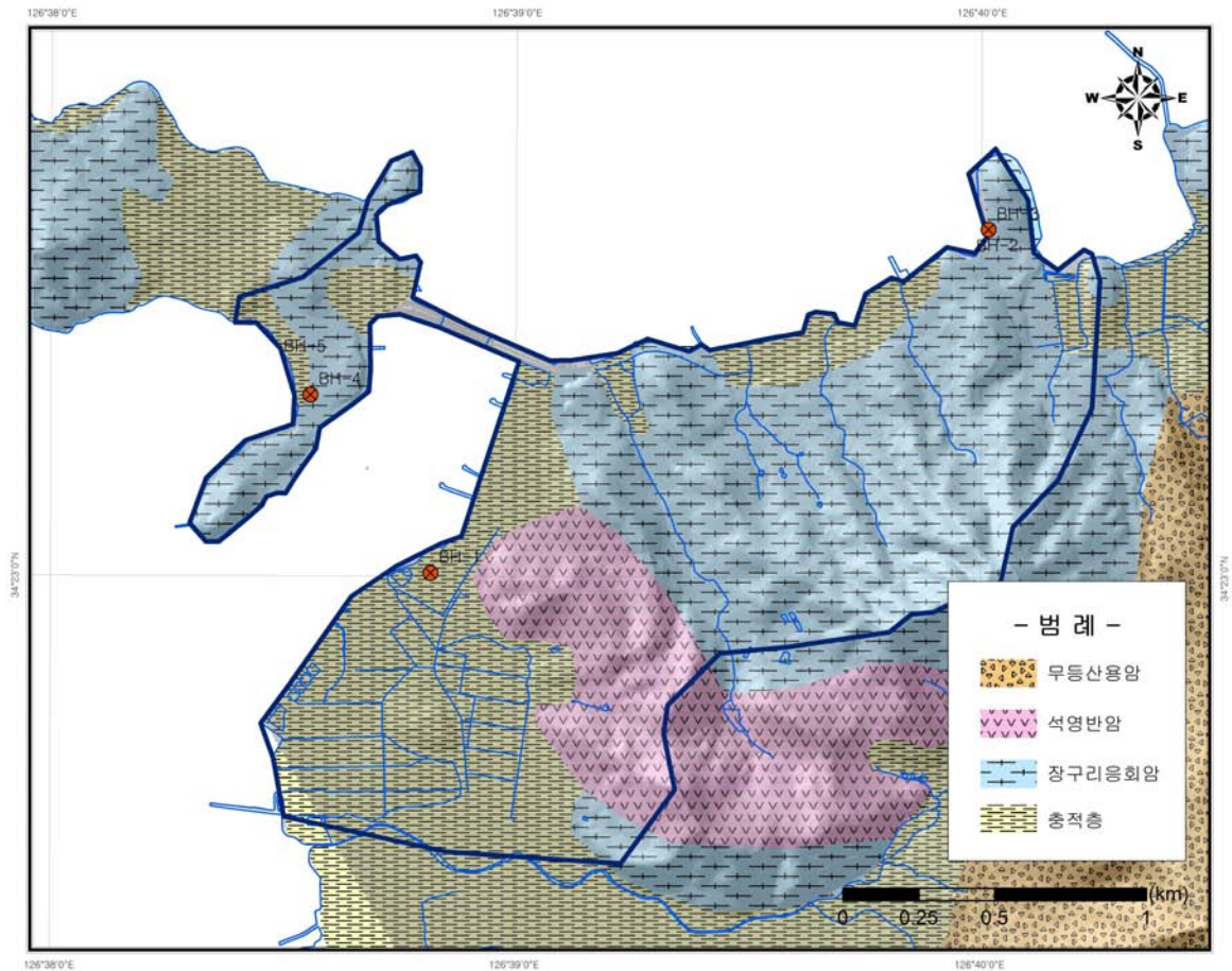
<그림 2-3-3> 완군2지구 지질도
