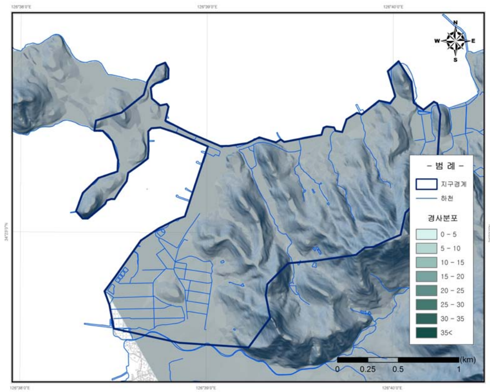
<그림 2-3-2> 완군2지구 지형경사
