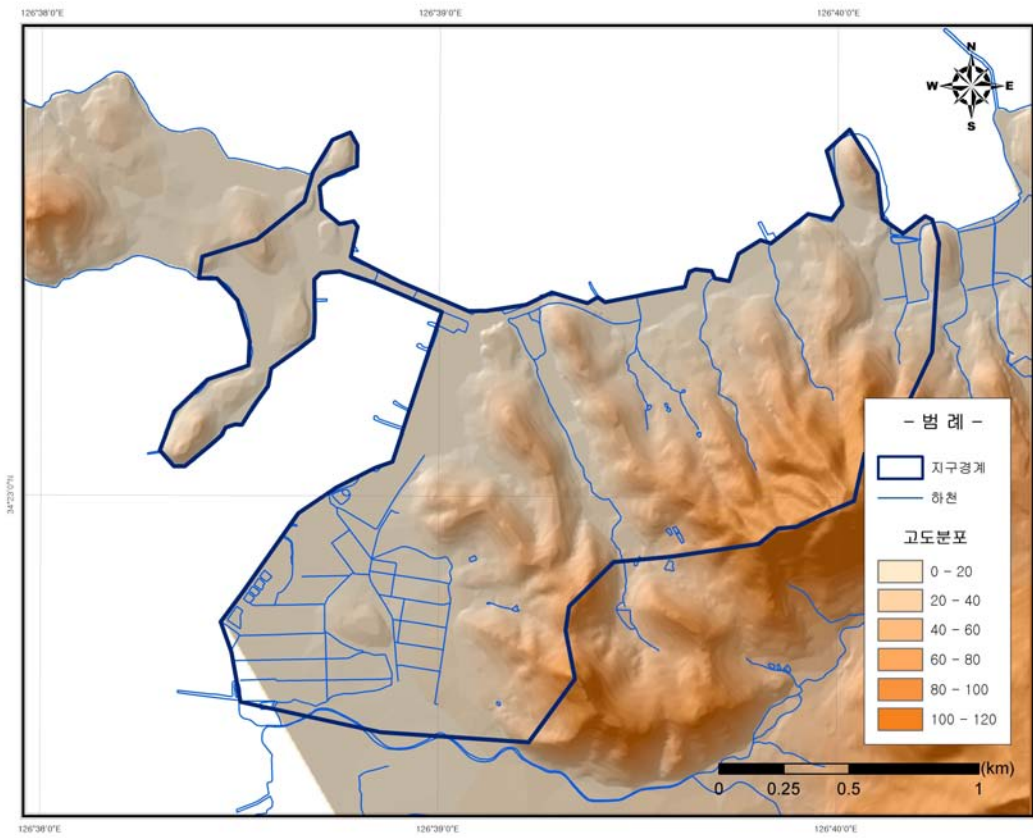
<그림 2-3-1> 완군2지구 지형고도
