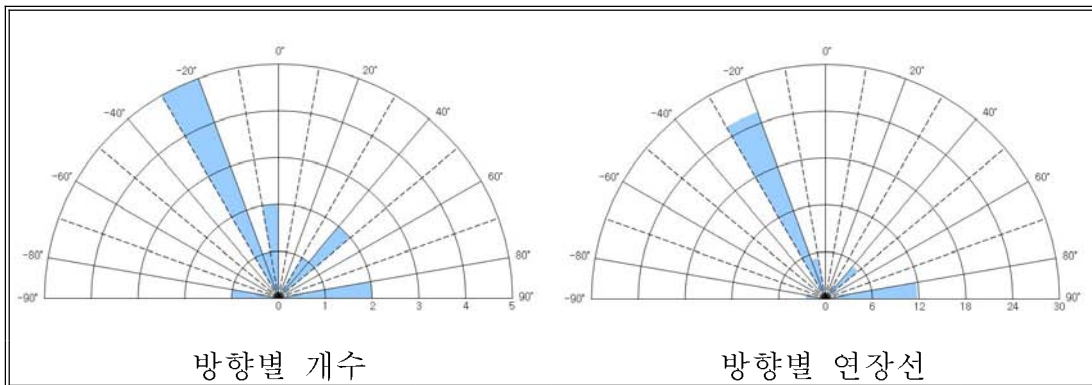
<그림 2-3-4> 완군2지구 선형구조의 방향별 특성
