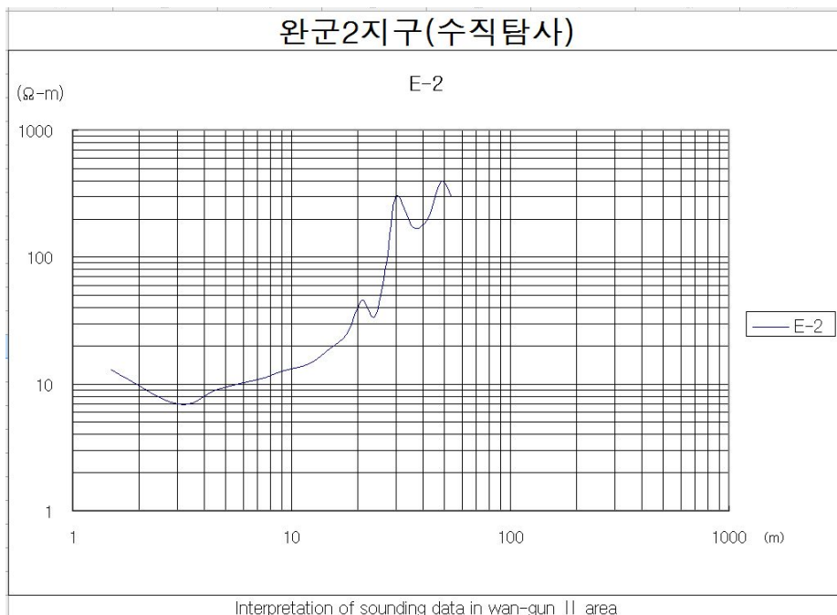
<그림 4-1-14> WG2-02 수직탐사 결과
