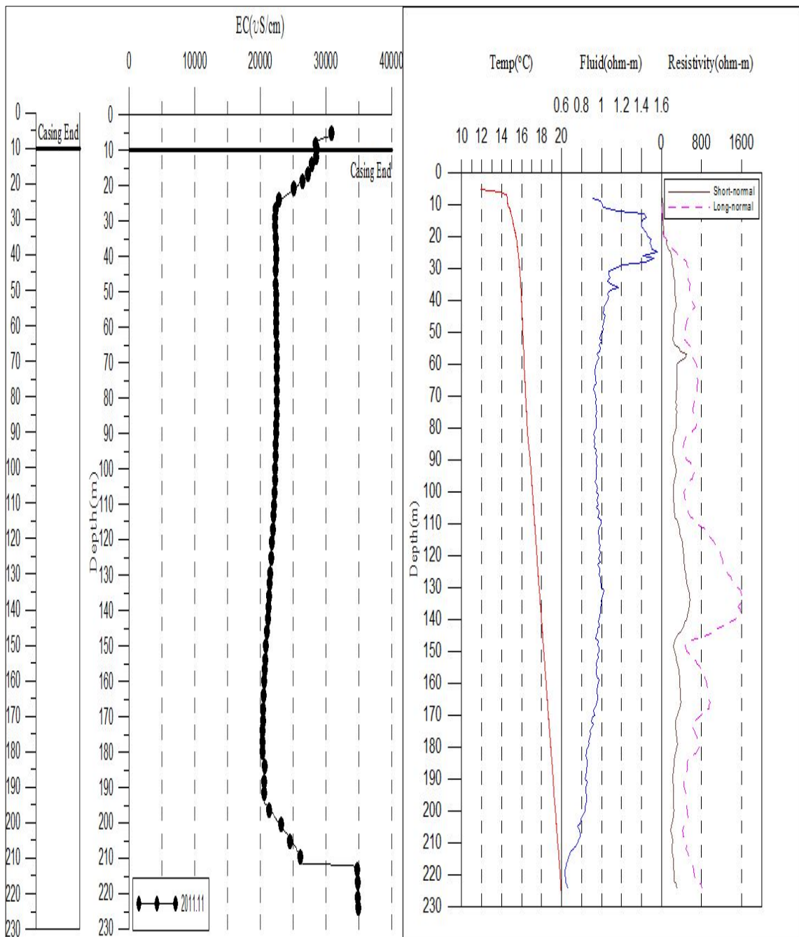
<그림 4-3-4> WG2BH-04호공의 물리검층 결과 그래프
