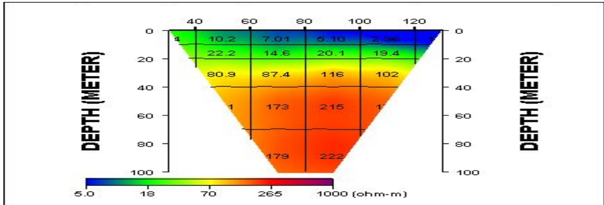
<그림 4-1-9> WG2-05 전기비저항탐사 단면도
