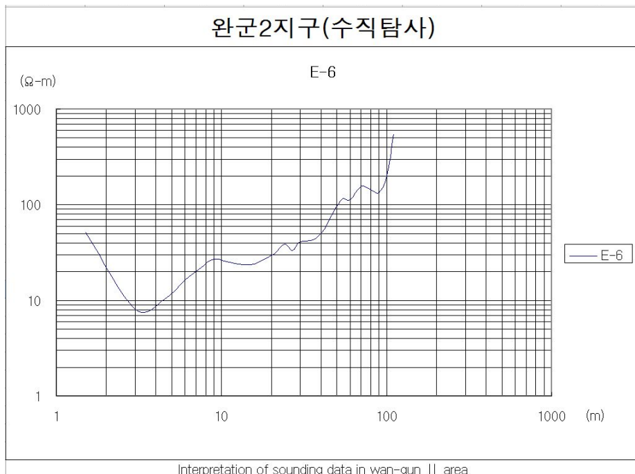
<그림 4-1-18> WG2-06 수직탐사 결과
