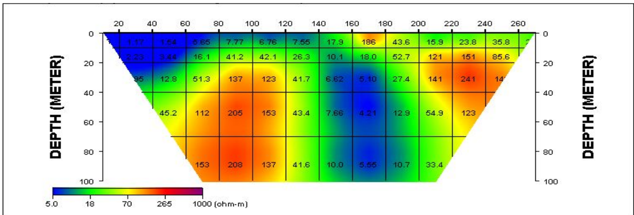
<그림 4-1-8> WG2-04 전기비저항탐사 단면도
