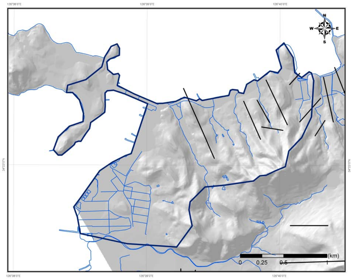
<그림 2-3-5> 완군2지구 선형구조(lineament) 분포도
