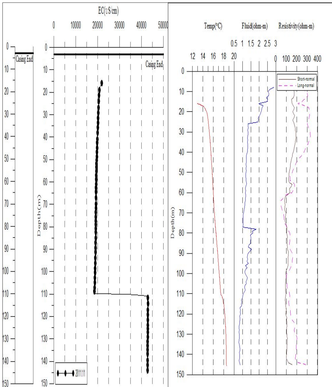
<그림 4-3-3> WG2BH-03호공의 물리검층 결과 그래프
