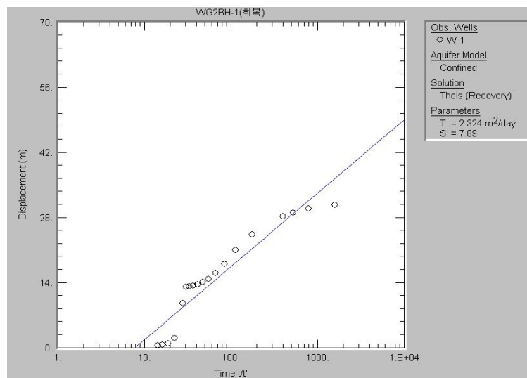
<그림 4-4-2> WG2BH-01호공 양수시험 해석 결과도
