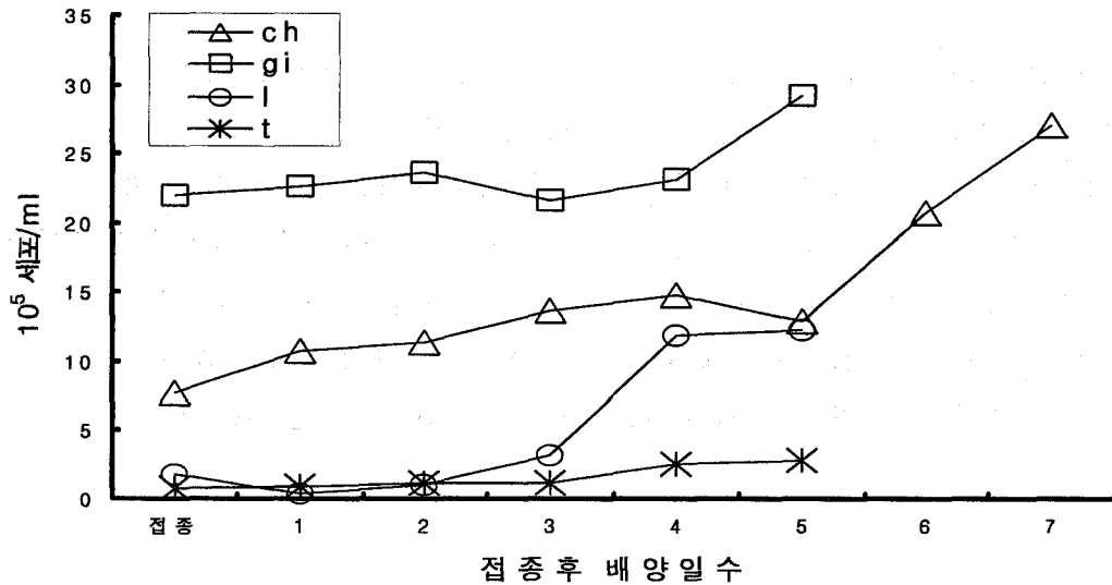
그림 3-4-5. 실외 대량배양시 식물성 먹이생물의 성장곡선.
