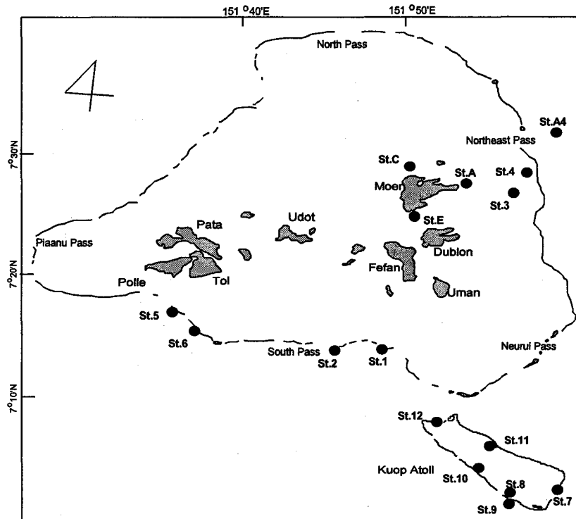
그림 3-1-2. 축 환초 조사해역도(2003. 2).
