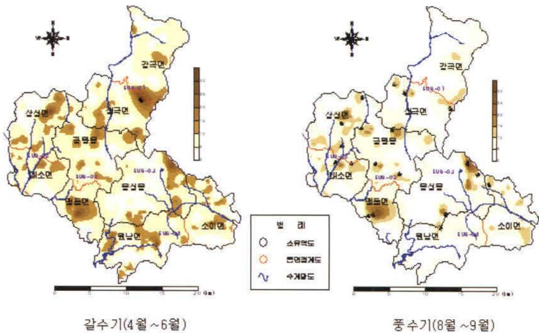
<그림 2-2-2> 질산성질소 일제조사 현황
