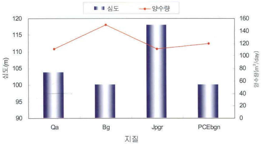
<그림 1-2-6> 지질별 암반지하수 평균심도 및 양수량
