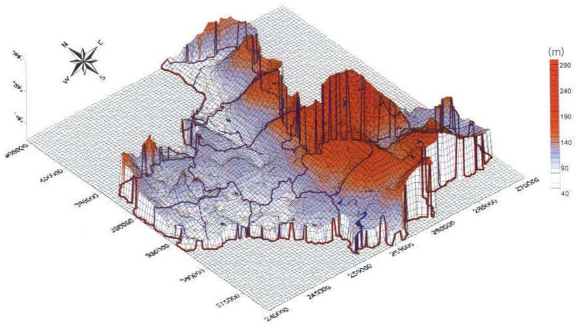
<그림 1-2-4> 풍수기 지하수두 등고선도 및 유동방향도(3D)
