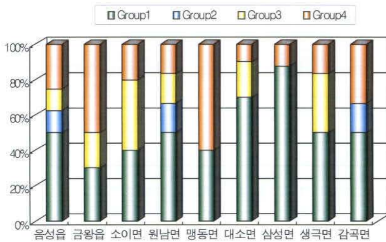
<그림 1-2-18> 읍면별 염소와 질산염에 의한 지하수분류
