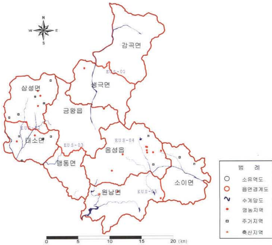
<그림1-2-21> 질소동위원소분석 조사관정 위치도
