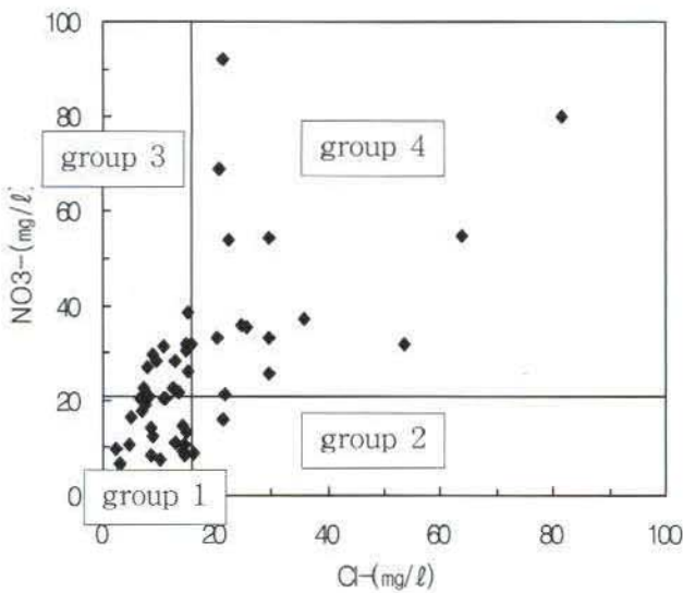
<그림 1-2-19> 염소와 질산염에 의한 지하수분류
