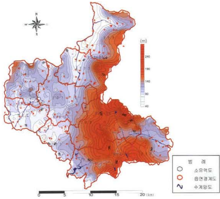
<그림 1-2-3> 풍수기 지하수두 등고선도 및 유동방향도
