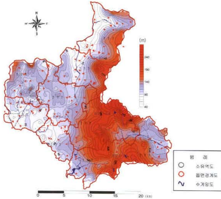
<그림 1-2-1> 갈수기 지하수두 등고선도 및 유동방향도(2D)
