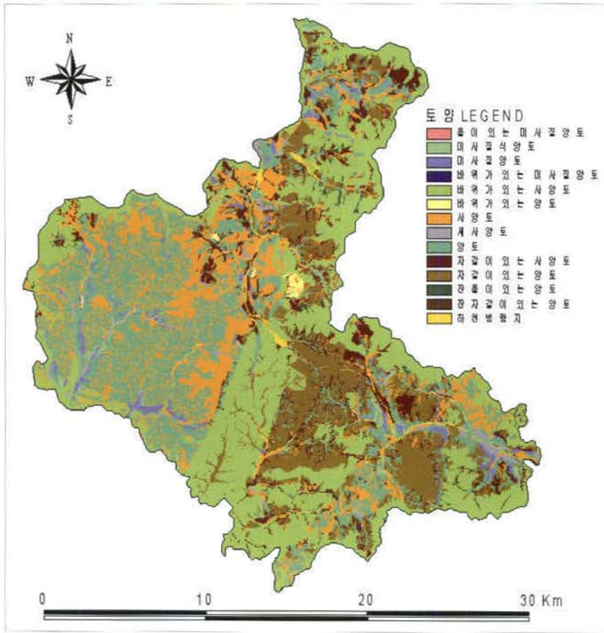
<그림 1-1-7> 음성군 토양도
