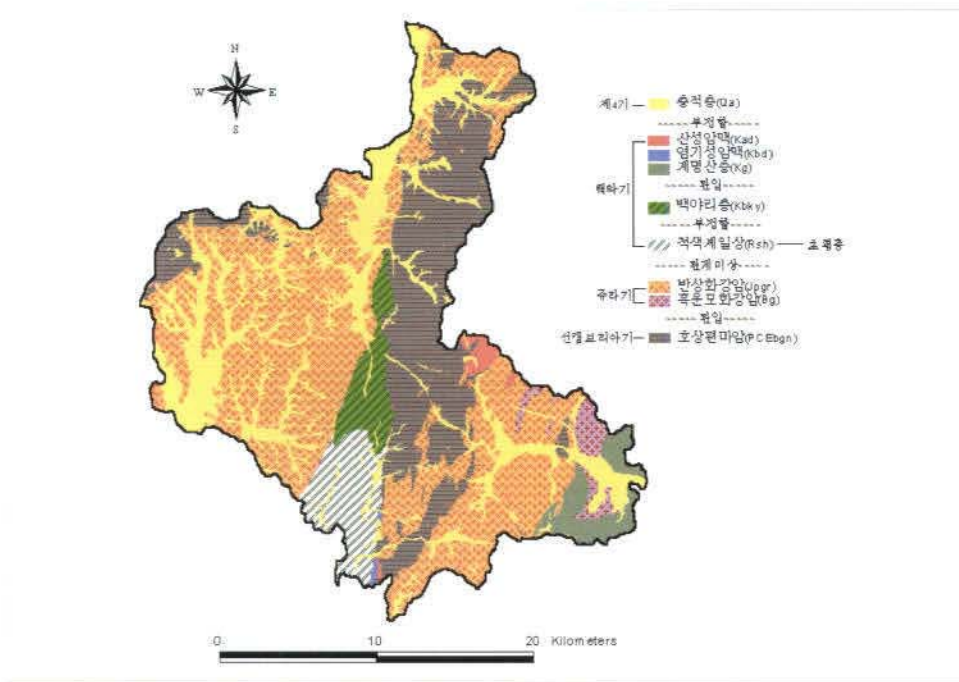
<그림 1-1-6> 음성군 지질도
