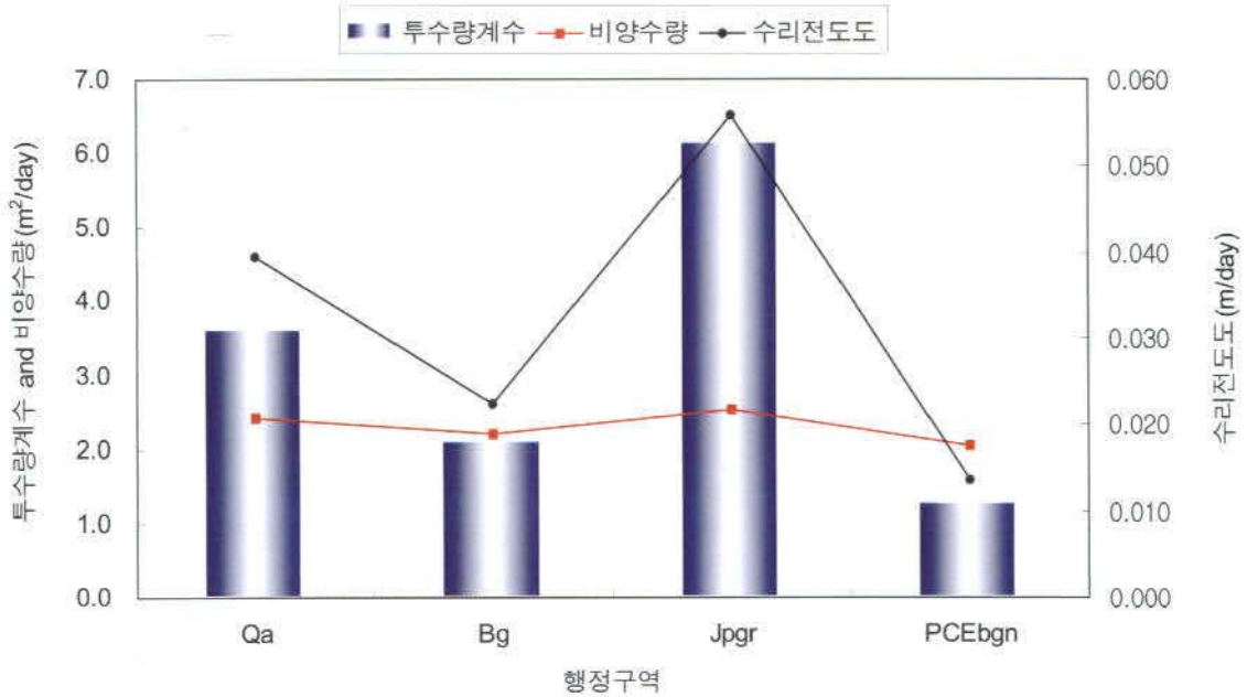
<그림 1-2-7> 지질별 암반지하수 투수랑계수, 비양수량 및 수리전도도
