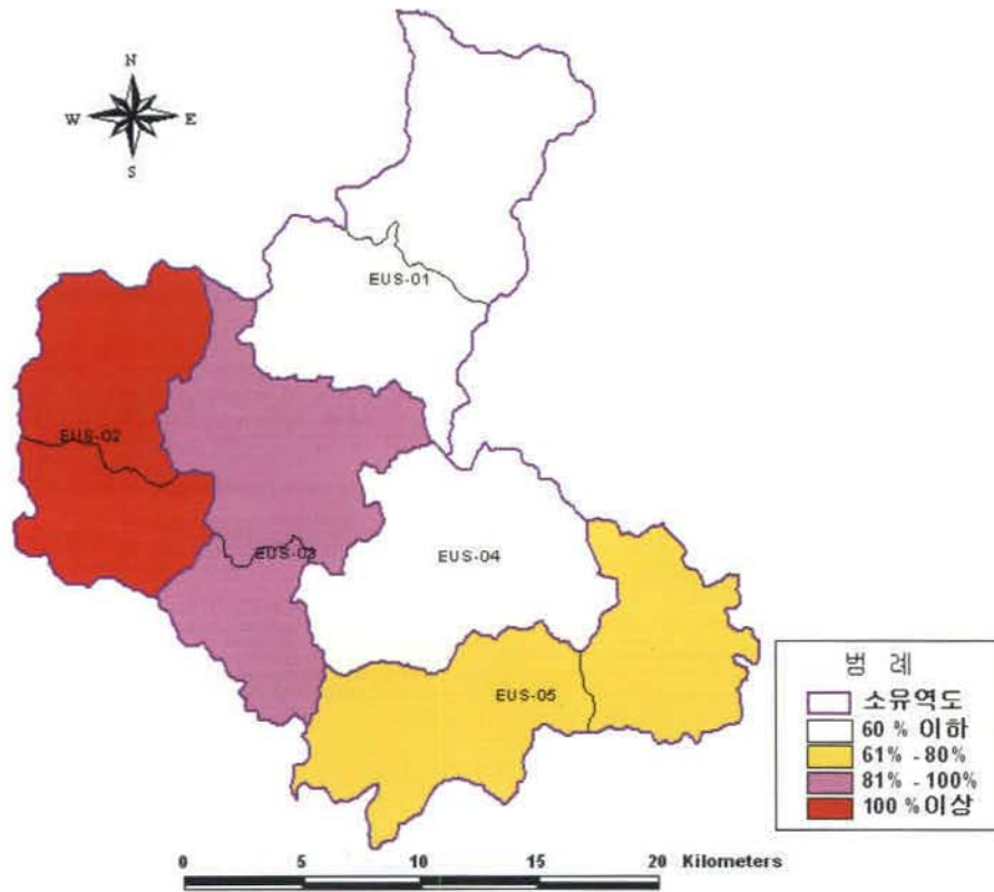
<그림 1-2-11> 유역별 지하수 이용량 대 개발가능량
