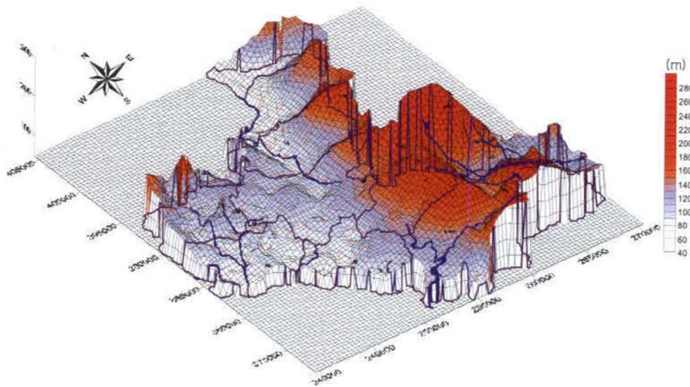
<그림 1-2-2> 갈수기 지하수두 등고선도 및 유동방향도(3D)
