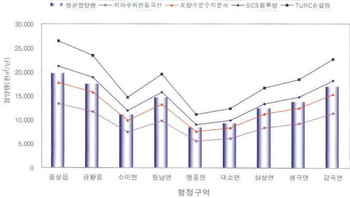
<그림 1-2-10> 읍면별 지하수 함양량
