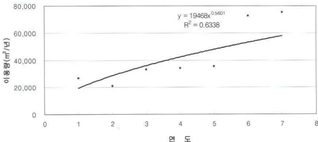
<그림 1-2-29> 지하수 이용전망 추세
