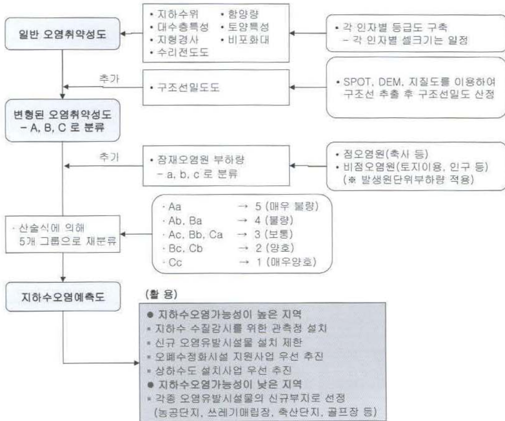
<그림 1-2-32> 지하수오염예측도 작성 모식도
