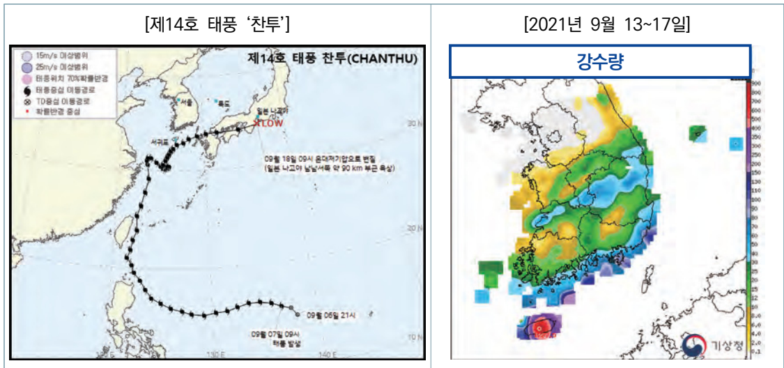
[그림 1-4-19] (왼쪽) 2021년 9월 발생 우리나라에 영향을 미친 제14호 태풍 ‘찬투’ 진로도 (오른쪽) 태풍 ‘찬투’에 의한 2021년 9월 13~17일 전국 누적강수량 분포(mm)
