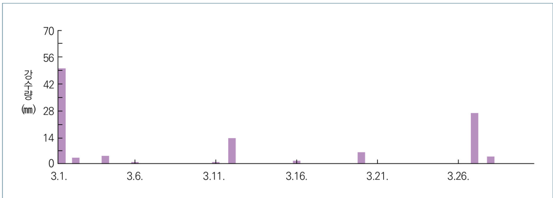
[그림 1-4-7] 3월 강수량 일별 시계열
