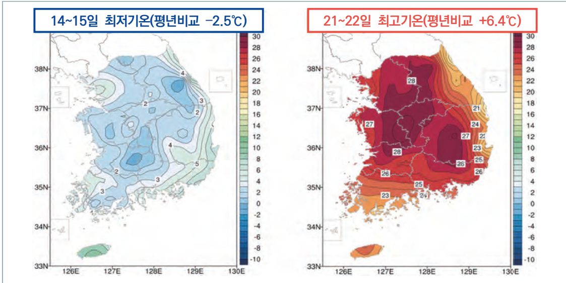
[그림 1-4-9] 14~15일 최저기온과 21~22일 최고기온 분포
