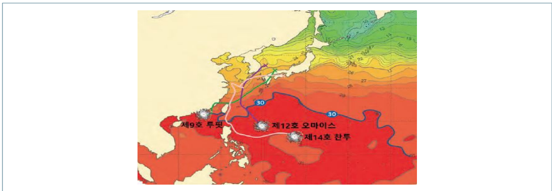
[그림 1-4-16] 2021년 영향 태풍 경로도
