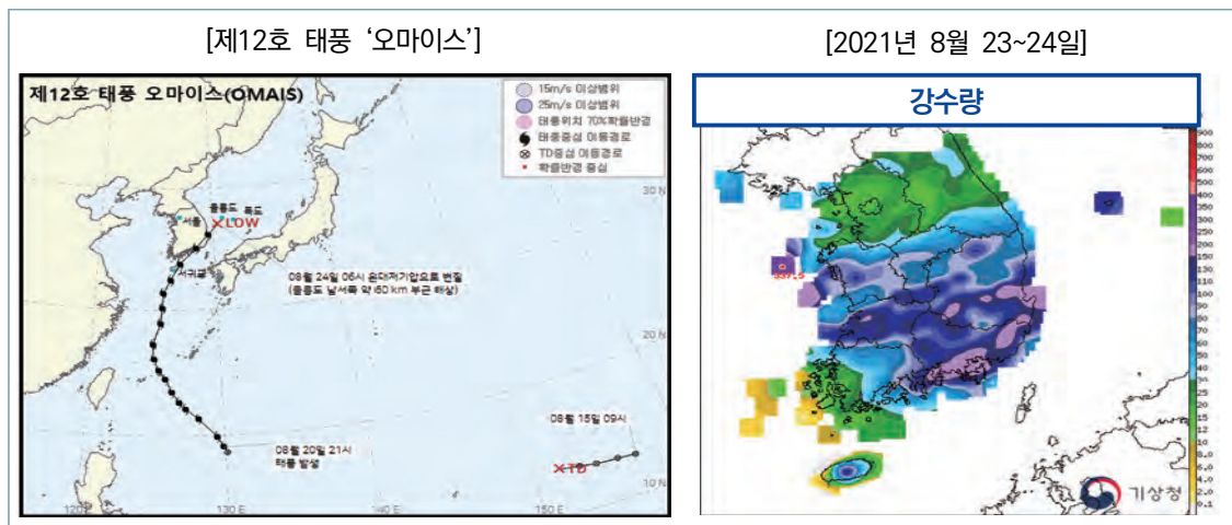
[그림 1-4-18] (왼쪽) 2021년 8월 발생 우리나라에 영향을 미친 제12호 태풍 '오마이스' 진로도 (오른쪽) 태풍 '오마이스'에 의한 2021년 8월 8~9일 전국 누적강수량 분포(mm)
