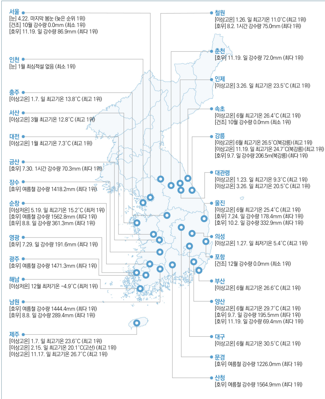
[그림 1-4-5] 우리나라의 이상기후 발생 현황(2020)
