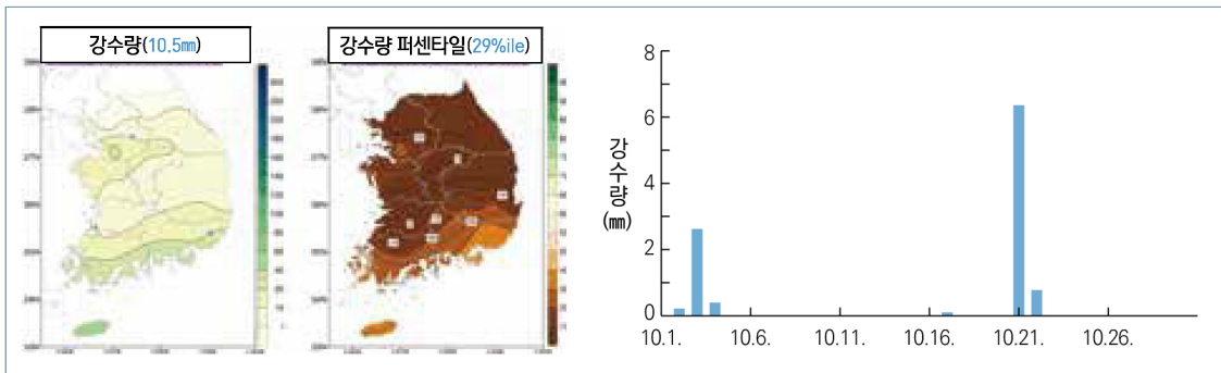
[그림 1-4-12] 전국 45개 지점의 10월 강수량(mm)과 강수량 퍼센타일 분포도 및 강수량(mm) 시계열
