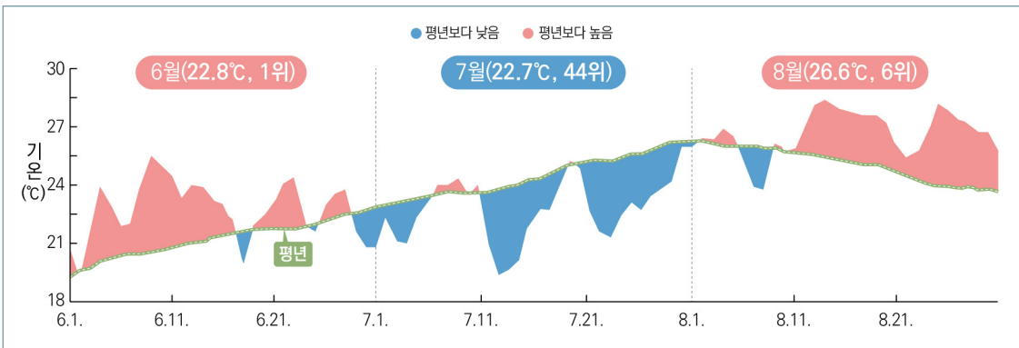
[그림 1-4-10] 2020년 6~8월 전국 평균기온의 일변화 시계열
