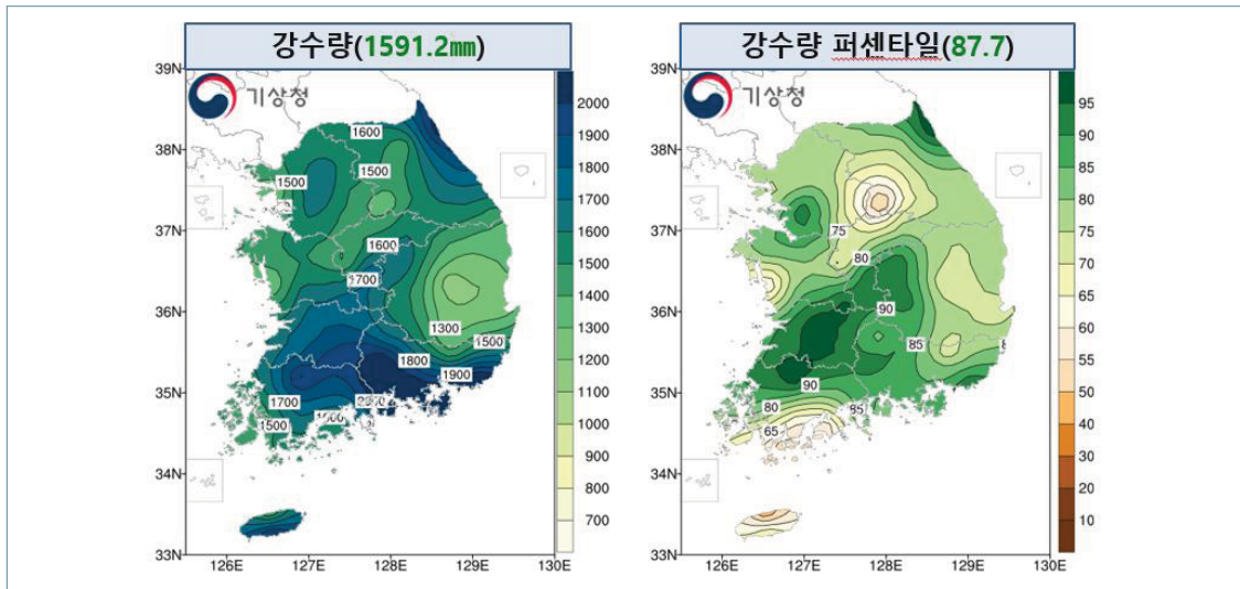
[그림 1-4-3] 연평균 누적 강수량 및 평년값 대비 연 강수량 퍼센타일 분포도
