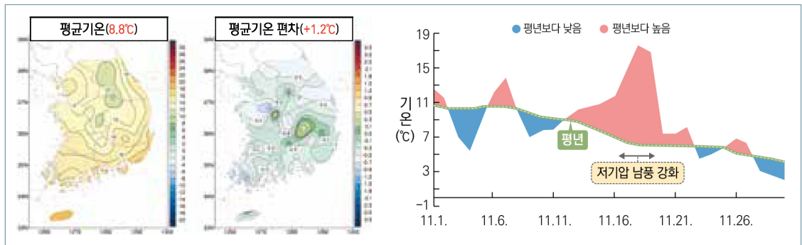
[그림 1-4-13] 전국 45개 지점의 11월 평균기온과 편차(℃) 분포도 및 일변화 시계열
