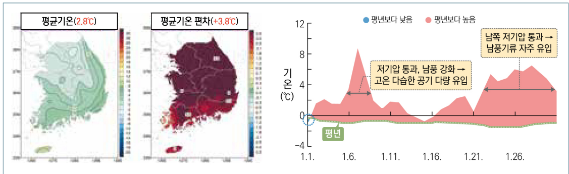
[그림 1-4-6] 전국 45개 지점의 1월 평균기온과 편차(℃) 분포도 및 일반화 시계열
