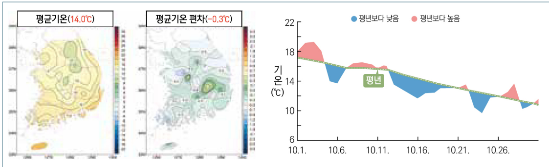
[그림 1-4-11] 전국 45개 지점의 10월 평균기온과 편차(°C) 분포도 및 일변화 시계열
