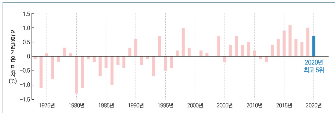
[그림 1-4-1] 우리나라 연평균기온 편차 시계열
