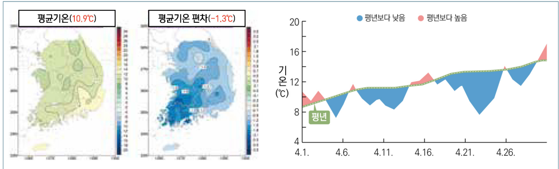
[그림 1-4-8] 전국 45개 지점의 4월 평균기온과 편차(°C) 분포도 및 일변화 시계열
