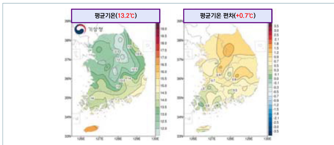
[그림 1-4-2] 연평균기온과 연평균기온 편차 분포도
