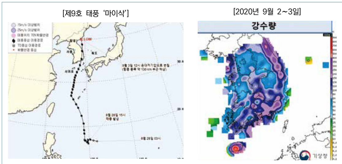
[그림 1-4-19] 제9호 태풍 ‘마이삭’ 진로도 및 태풍 ‘마이삭’에 의한 전국 누적강수량 분포도(mm)
