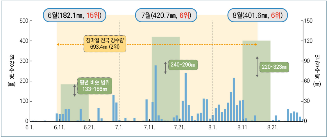
[그림 1-4-16] 2020년 6~8월 전국 강수량 일(파랑)/월(녹색) 변화 시계열
