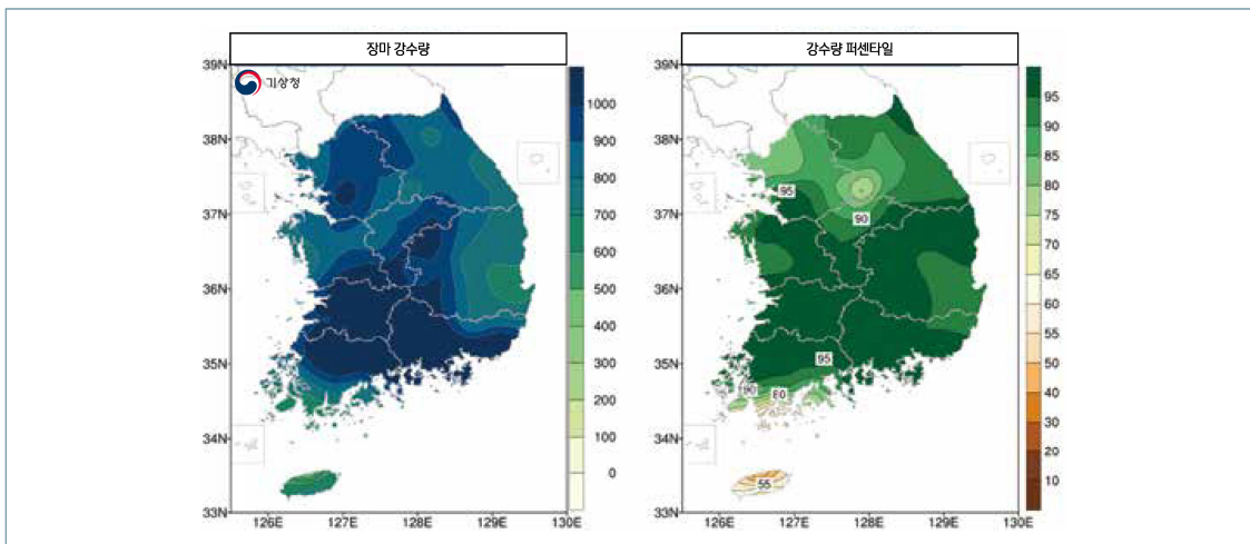
[그림 1-4-15] 장마 기간(6.10.~8.16.) 강수량(mm)과 강수량 퍼센타일(%ile) 분포도
