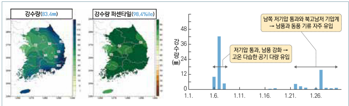
[그림 1-4-7] 전국 45개 지점의 1월 강수량(mm)과 강수량 퍼센타일 분포도 및 강수량(mm) 시계열
