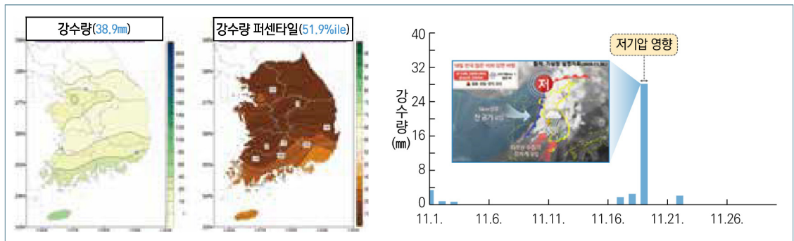
[그림 1-4-14] 전국 45개 지점의 11월 강수량(mm)과 강수량 퍼센타일 분포도 및 강수량(mm) 시계열
