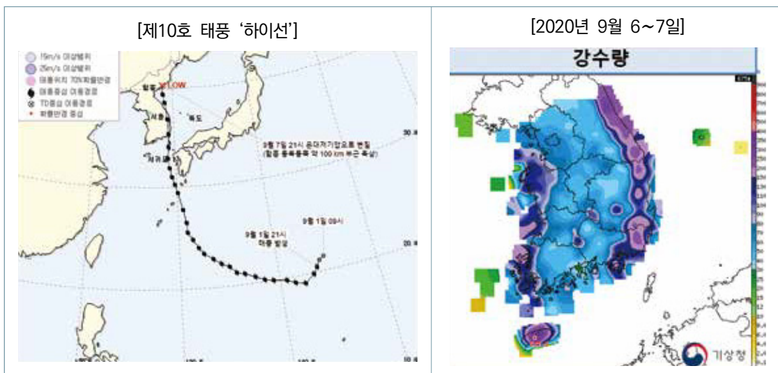
[그림 1-4-20] 제10호 태풍 ‘하이선’ 진로도 및 태풍 ‘하이선’에 의한 전국 누적강수량 분포도(mm)
