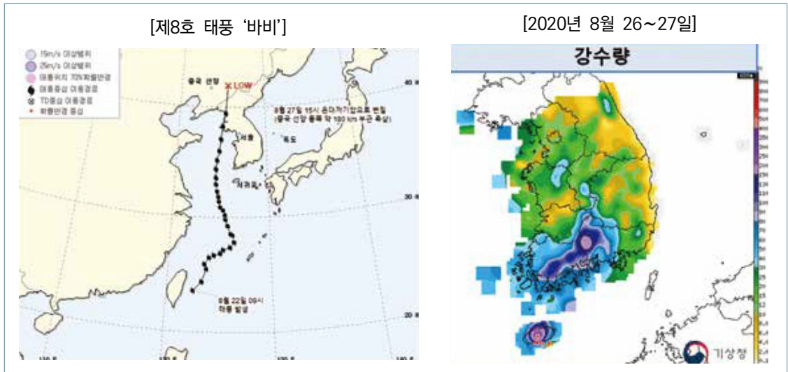
[그림 1-4-18] 제8호 태풍 ‘바비’ 진로도 및 태풍 ‘바비’에 의한 전국 누적강수량 분포도(mm)
