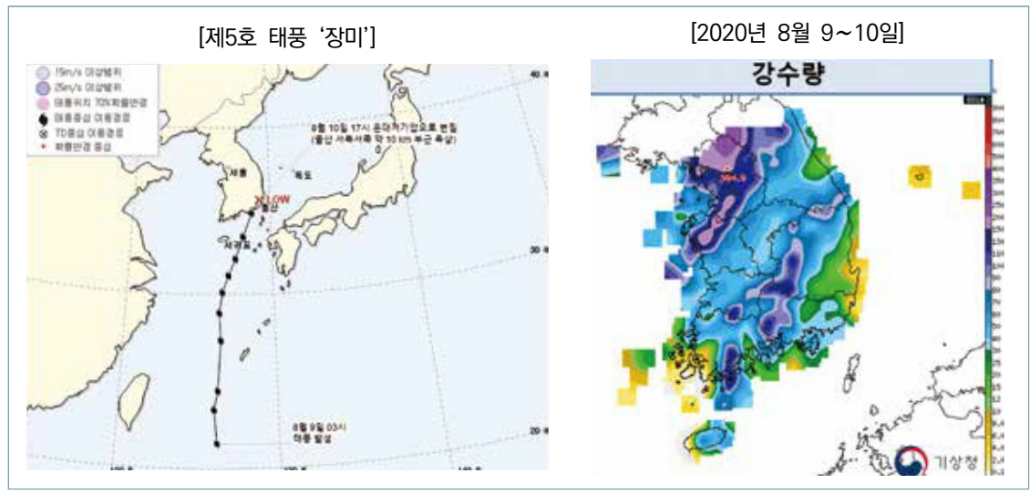
[그림 1-4-17] 제5호 태풍 ‘장미’ 진로도 및 태풍 ‘장미’에 의한 전국 누적강수량 분포도(mm)
