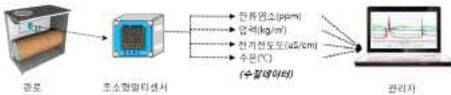
<그림 2-12> 초소형 멀티센서
