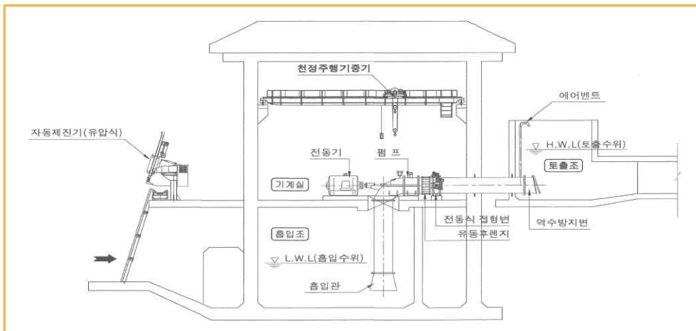
< 그림 2.18 > 횡축사류, 횡축축류 펌프의 단면도
