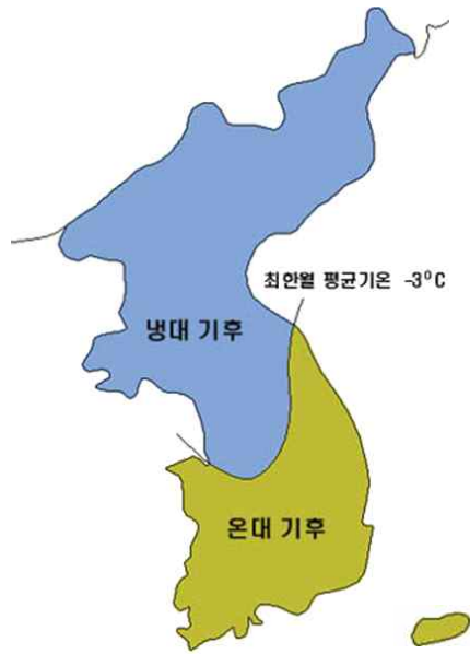
(a) 쾨펜에 의한 기후구분
