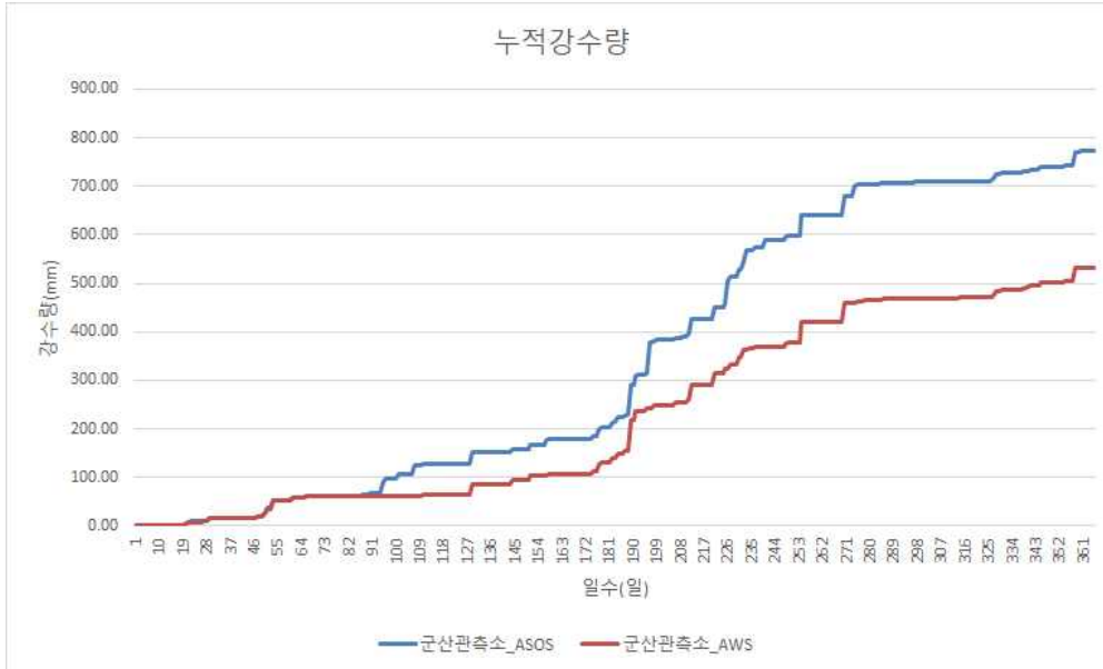
<그림 2-148> 2017년 금강지구 ASOS와 AWS 누적강수량 비교
