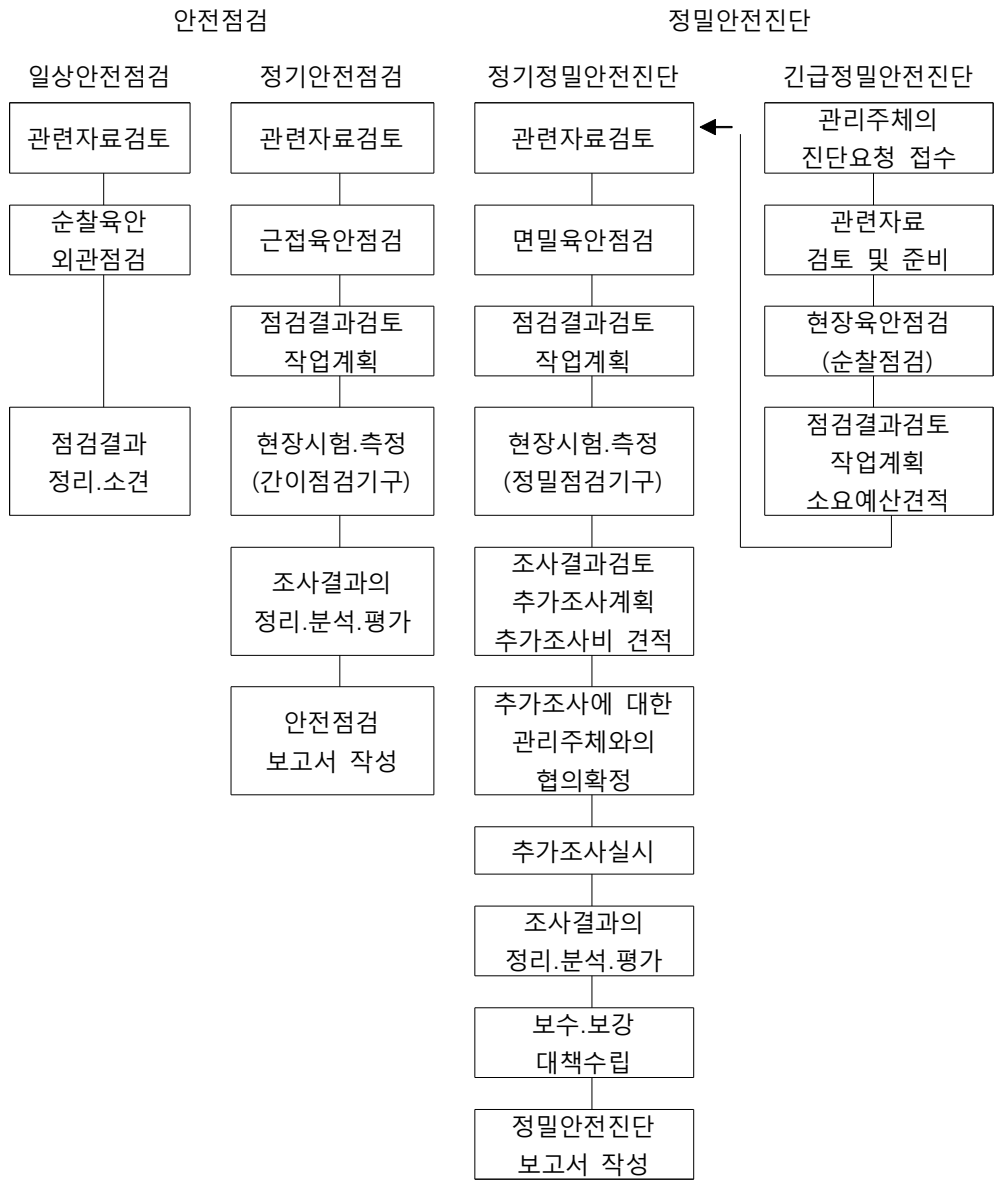
( 표 4.14 ) 안전점검 및 정밀안전진단 과업수행절차의 흐름도
