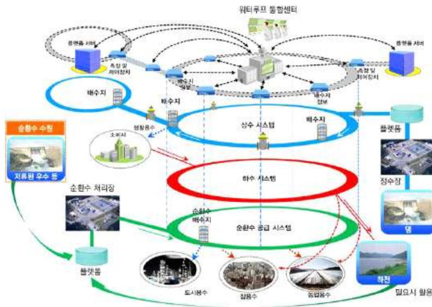
<그림 2-9> 순환수 Smart Water Grid 개념도
