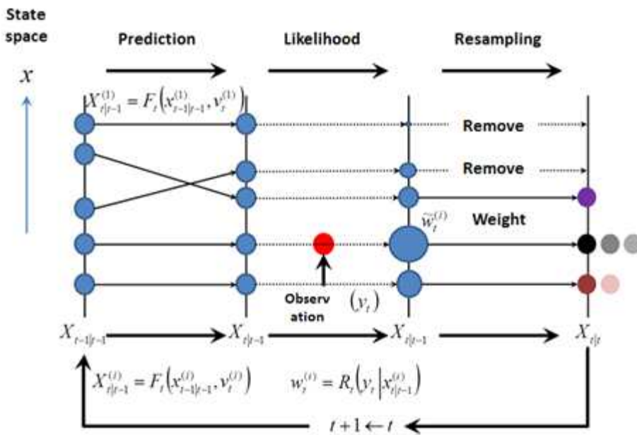
<그림 2-72> 파티클 필터의 모식도
