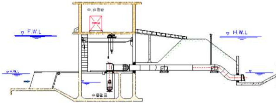
< 그림 3.25 > 수중펌프 배수장 단면도(예)
