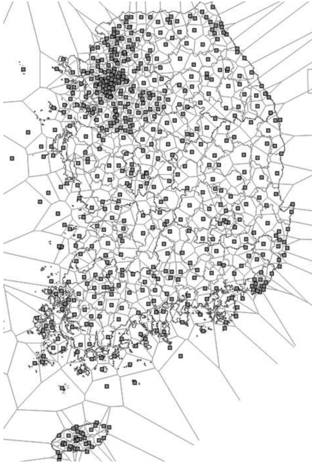
<그림 2-134> AWS 티센망도
