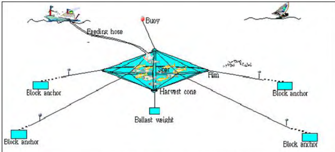
그림 106. 외해수중가두리 설치 모식도
