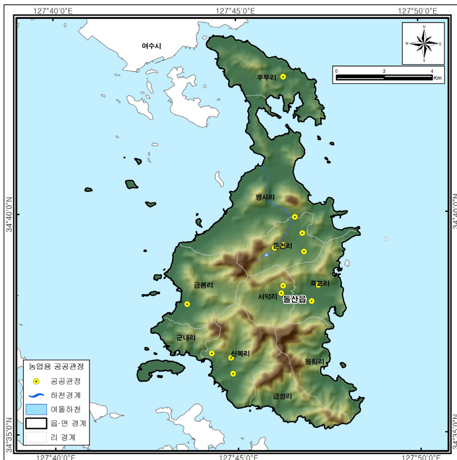
<그림 2-2-1> 현장 정밀관정조사 위치도
