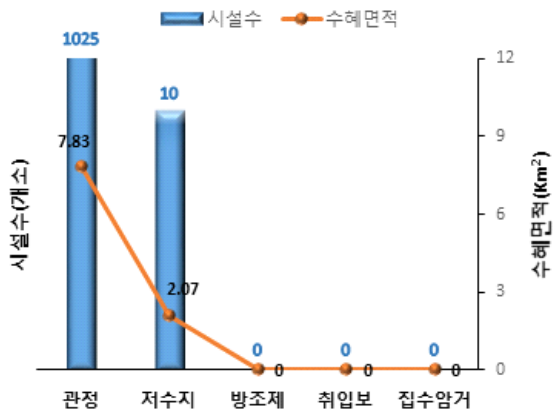
<그림 4-1-1> 농업기반 수리시설
