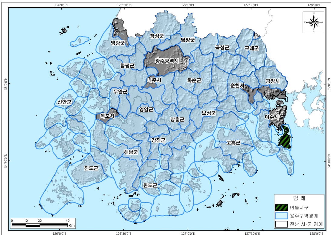
<그림 1-4-1> 여돌지구 용수구역 위치도
