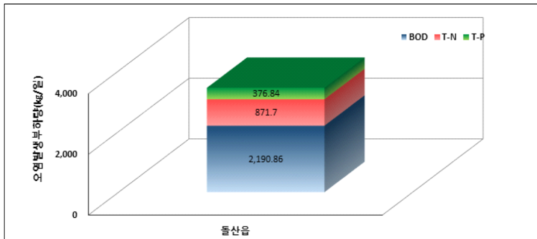
<그림 3-2-4> 읍면별 항목별 오염부하량
