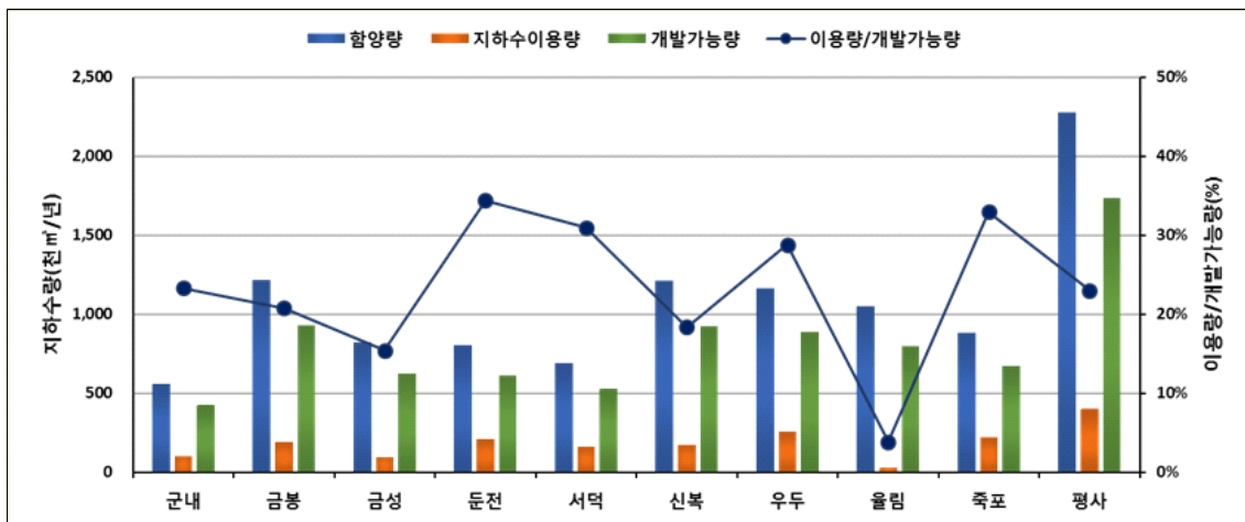
<그림 3-1-13> 리별 지하수 함양량
