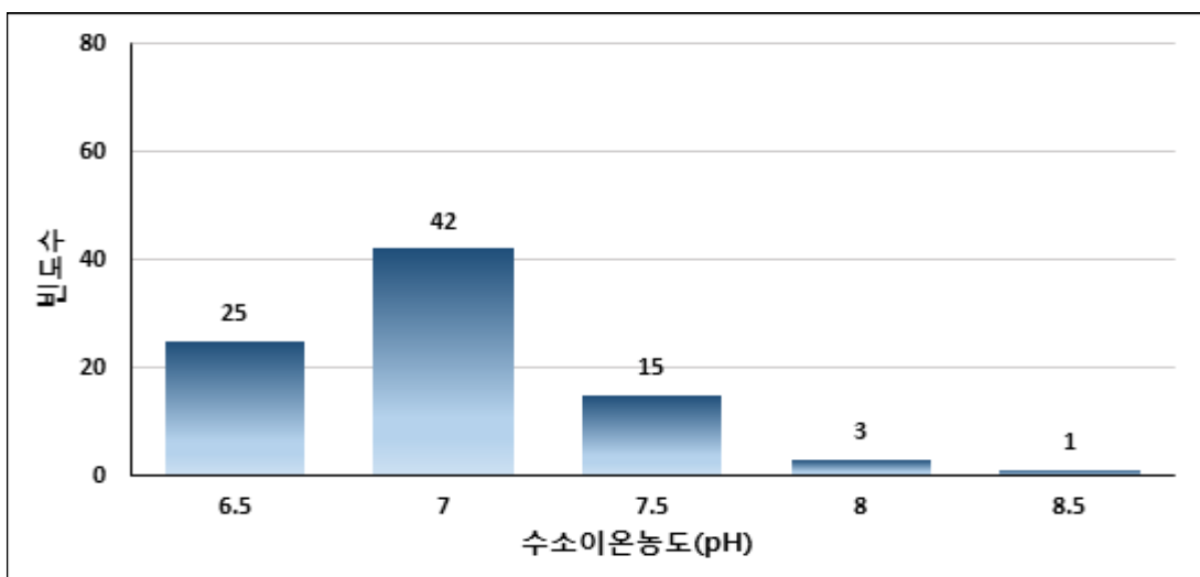
<그림 3-2-9> 여돌지구 지하수의 pH 빈도분포도
