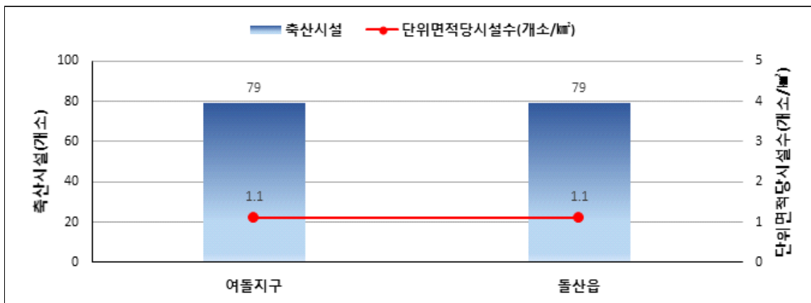
<그림 3-2-1> 점오염원 시설수 및 단위면적당 개소수
