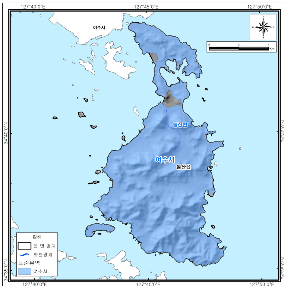
<그림 1-4-2> 여도지구 표준유역 현황
