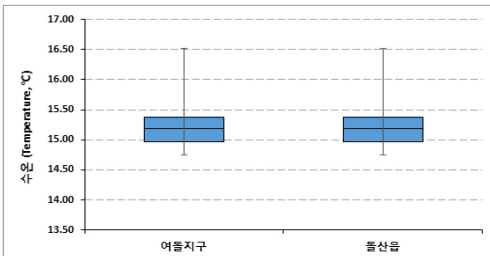
<그림 3-2-7> 여돌지구 지하수의 수온(Temperature, °C) Box-whisker
