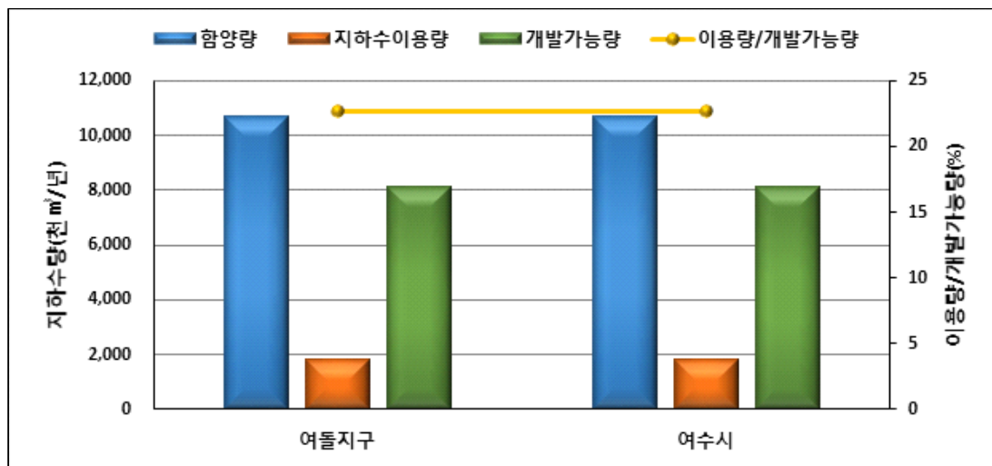
<그림 3-1-14> 표준유역별 지하수 이용량 및 개발가능량
