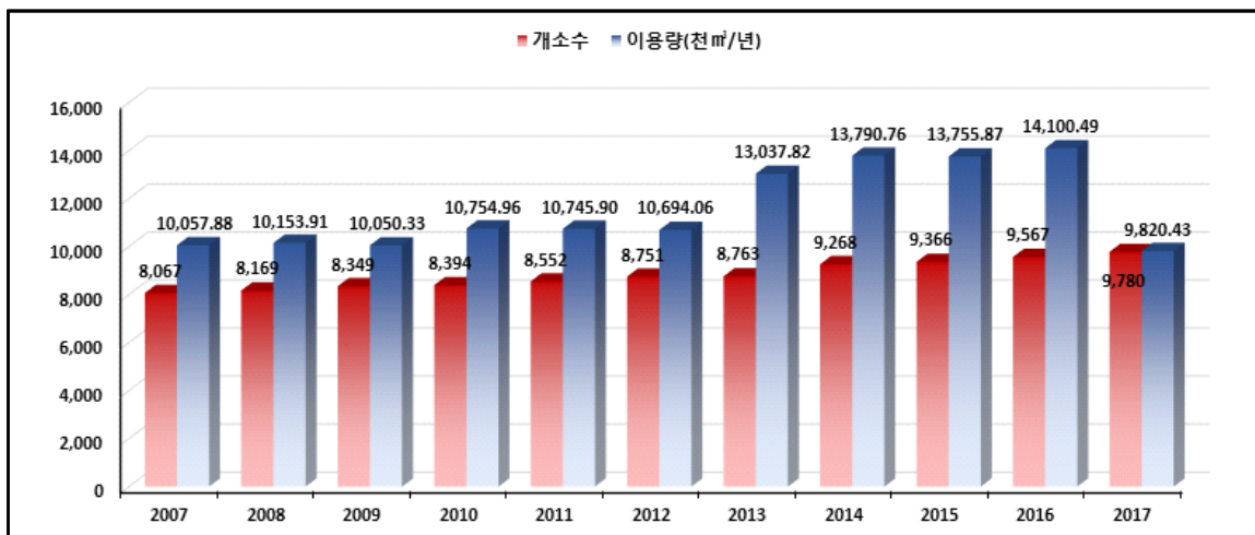
<그림 3-1-4> 연도별 지하수 이용·개발
