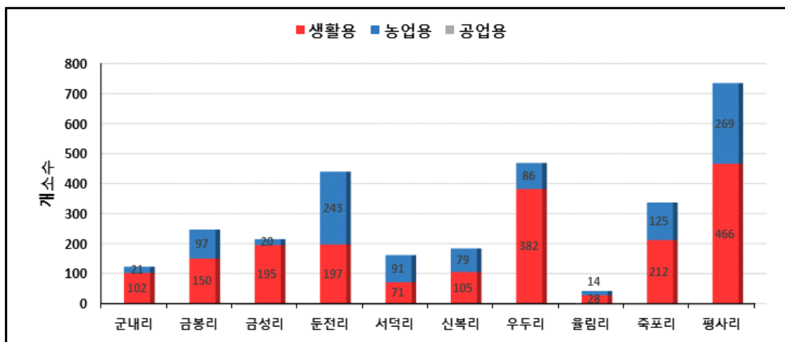
<그림 1-5-4> 리별·용도별 지하수이용현황
