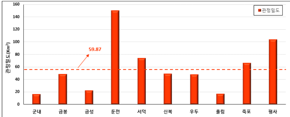
<그림 4-2-2> 리별 관정밀도 분포도
