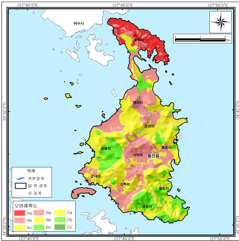
<그림 3-2-6> 여름지구 지하수오염예측도
