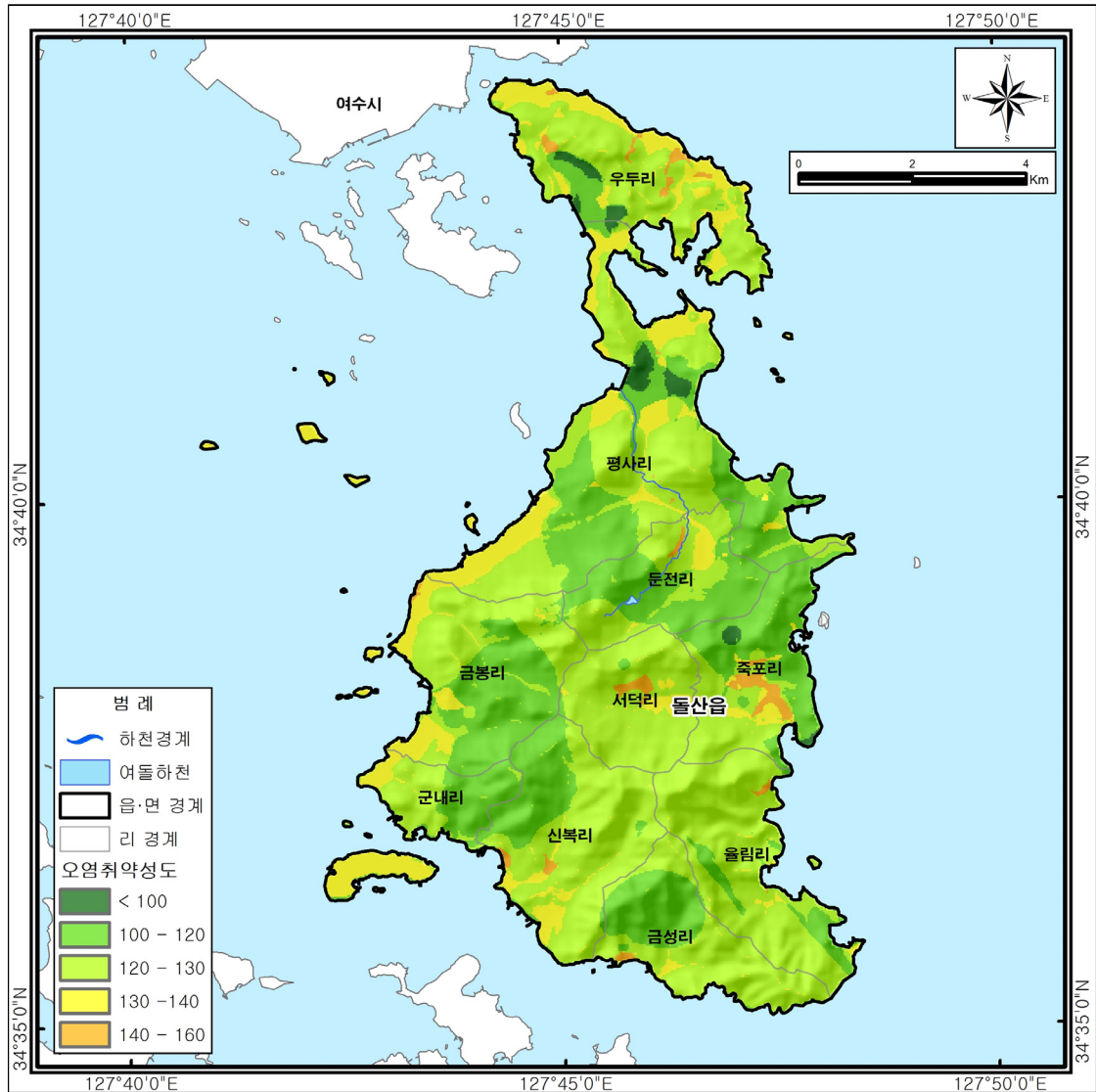
<그림 3-2-2> 여돌지구 DRASTIC INDEX Map
