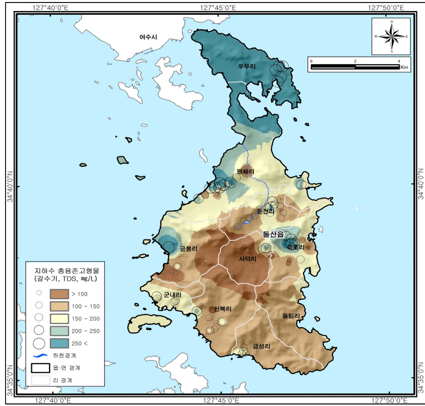
(a) 갈수기 총용존고형물 분포도
