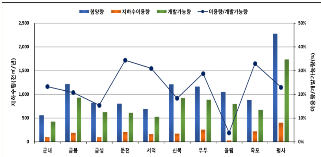
<그림 3-1-3> 리별 지하수 이용량 및 개발가능량
