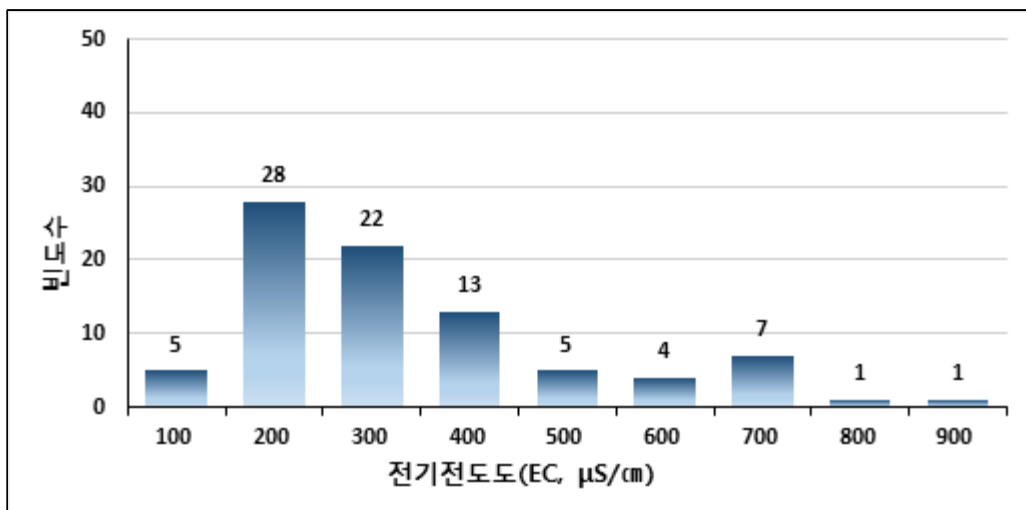
<그림 3-2-12> 여돌지구 지하수의 전기전도도(EC, \mu\text{S}/\text{cm} ) 빈도분포도
