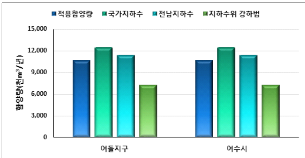
<그림 3-1-11> 표준유역별 지하수 함양량
