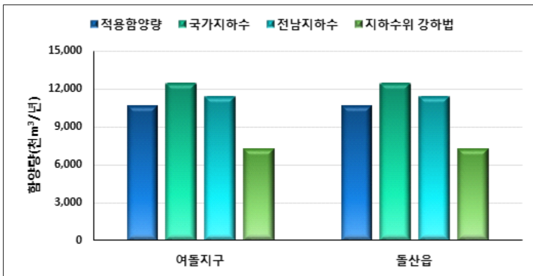
<그림 3-1-12> 읍면별 지하수 함양량
