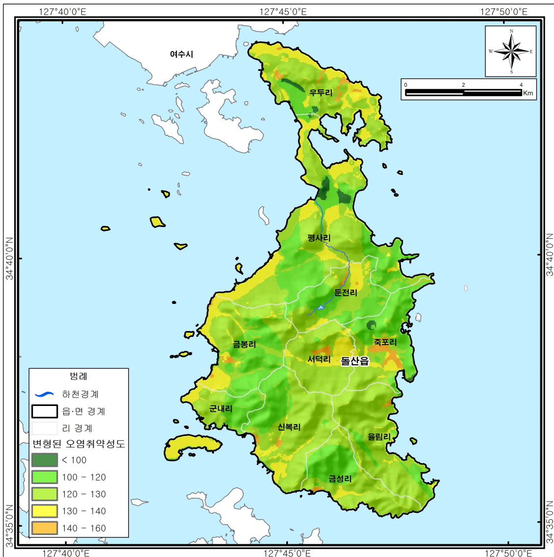
<그림 3-2-3> 여돌지구 Modified DRASTIC INDEX Map
