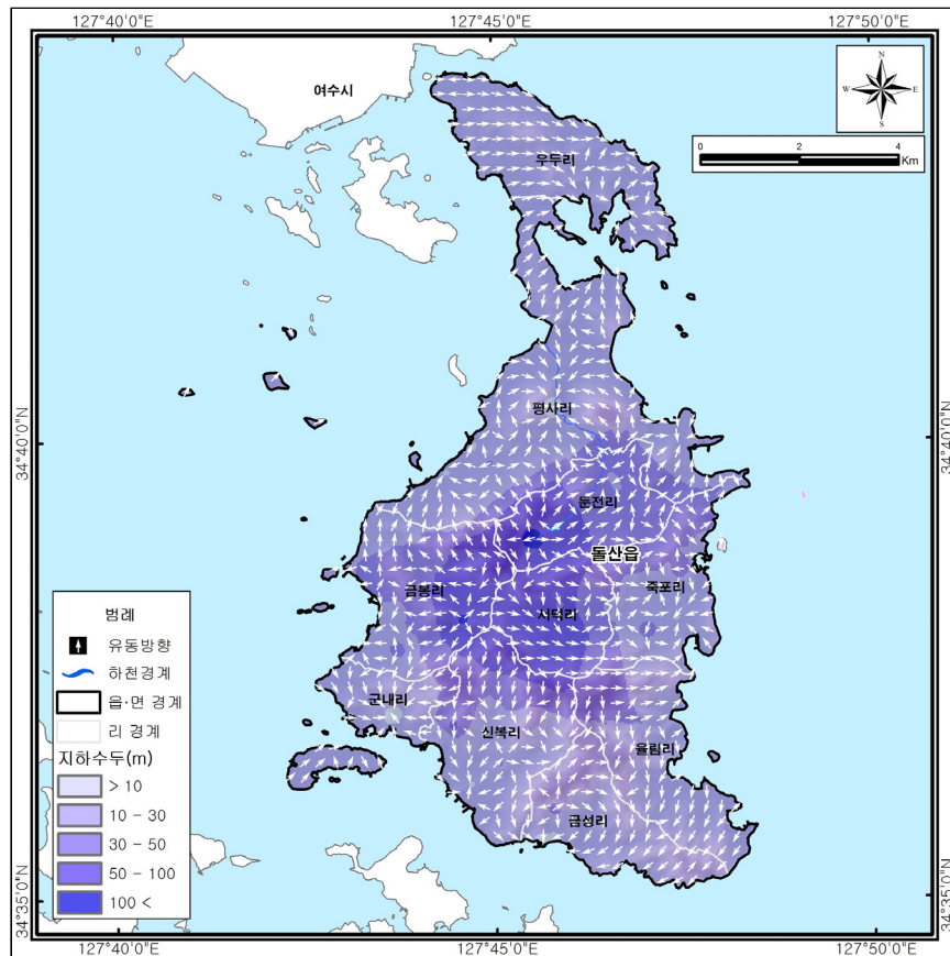
<그림 3-1-3> 지하수두 및 유동방향도
