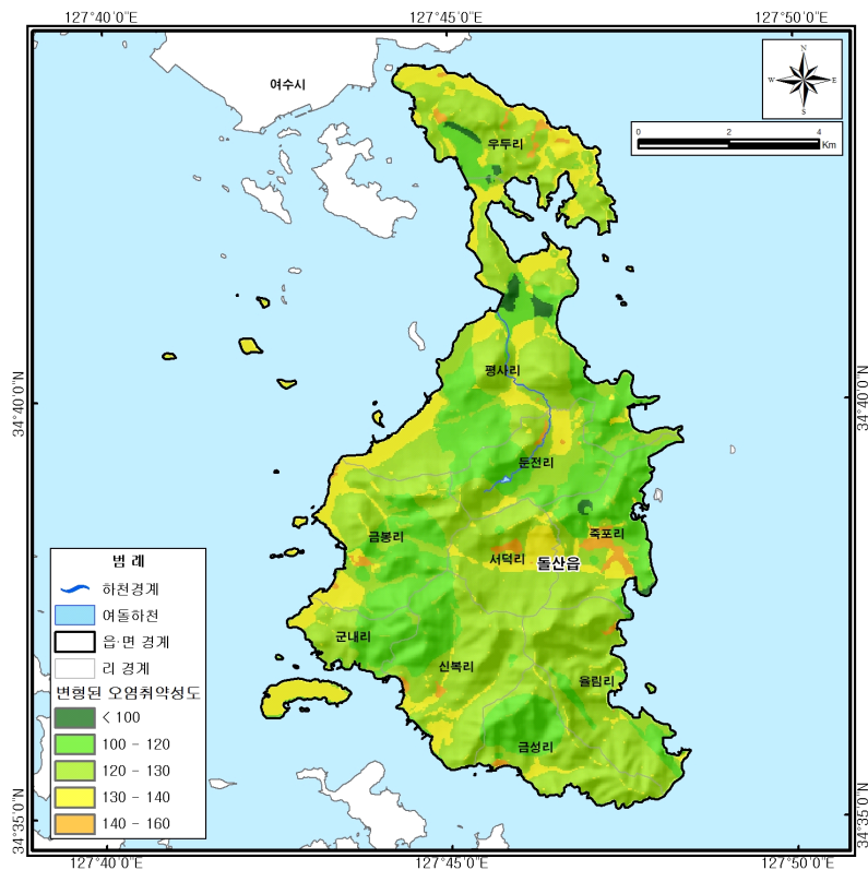
<그림 3-3-11> 여돌지구 변형된 오염취약성도(M-DRASTIC)
