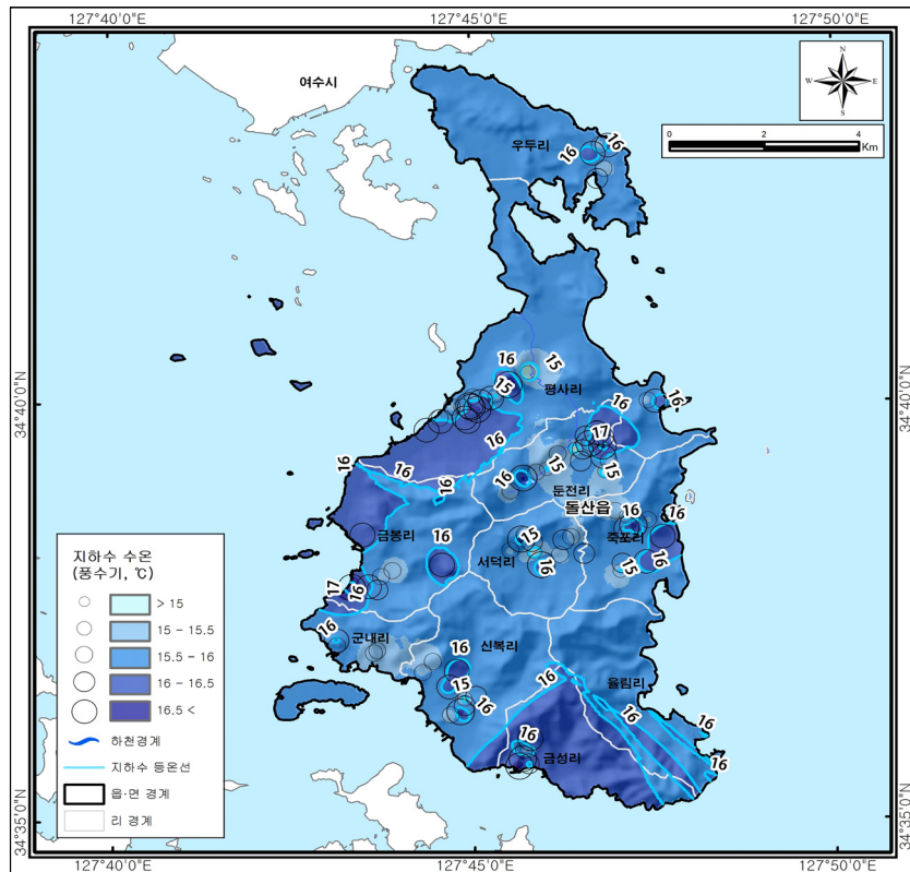
(b) 풍수기 수온분포도
