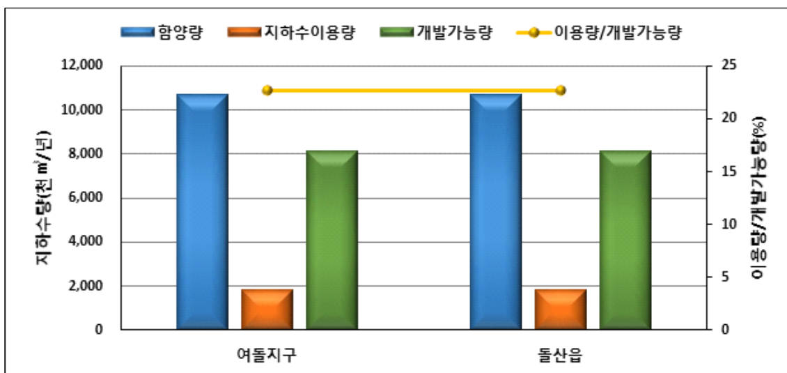
<그림 3-1-15> 읍면별 지하수 이용량 및 개발가능량
