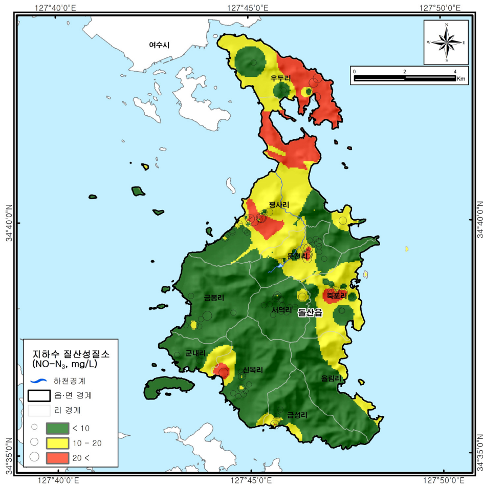
<그림 3-2-18> 여들지구 지하수의 질산성질소(mg/L) 분포도
