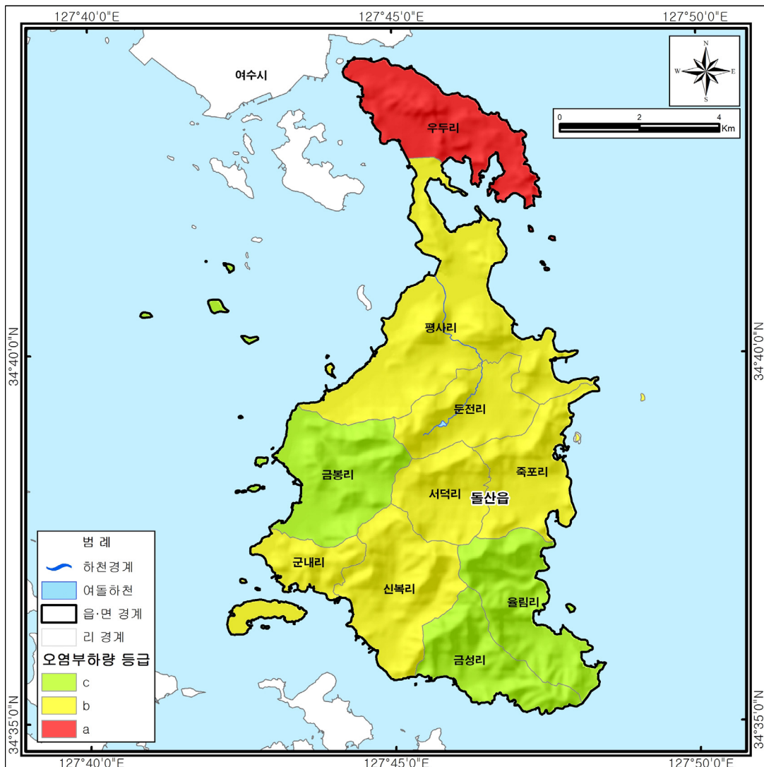
<그림 3-2-4> 발생단위별 잠재오염원 부하량 등급도
