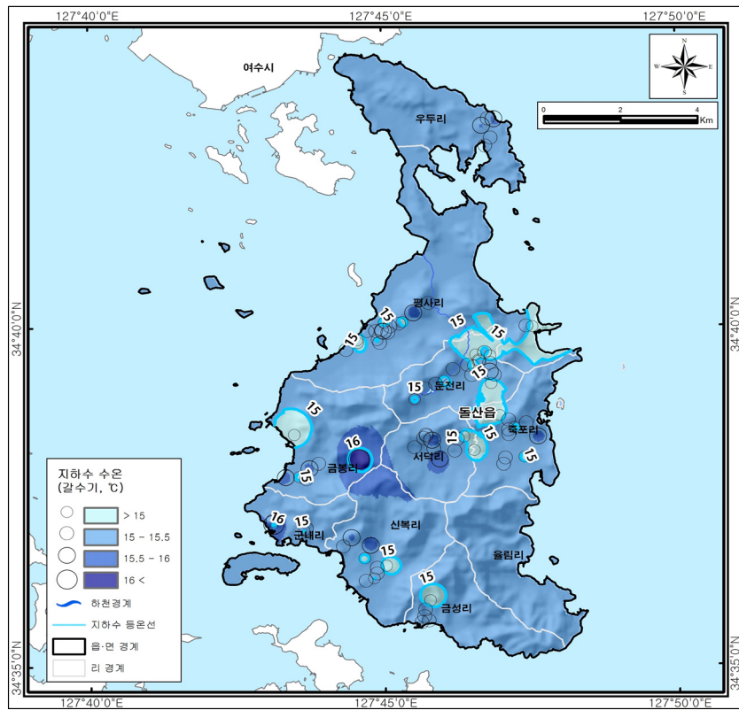
(a) 갈수기 수온분포도
