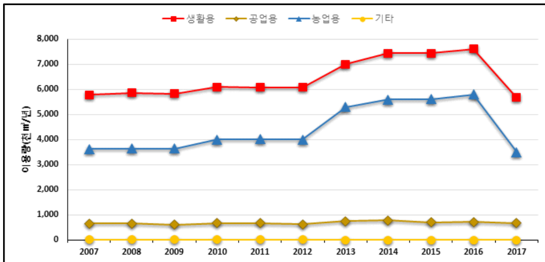
<그림 3-1-5> 여수시 용도별 지하수 이용량 추이
