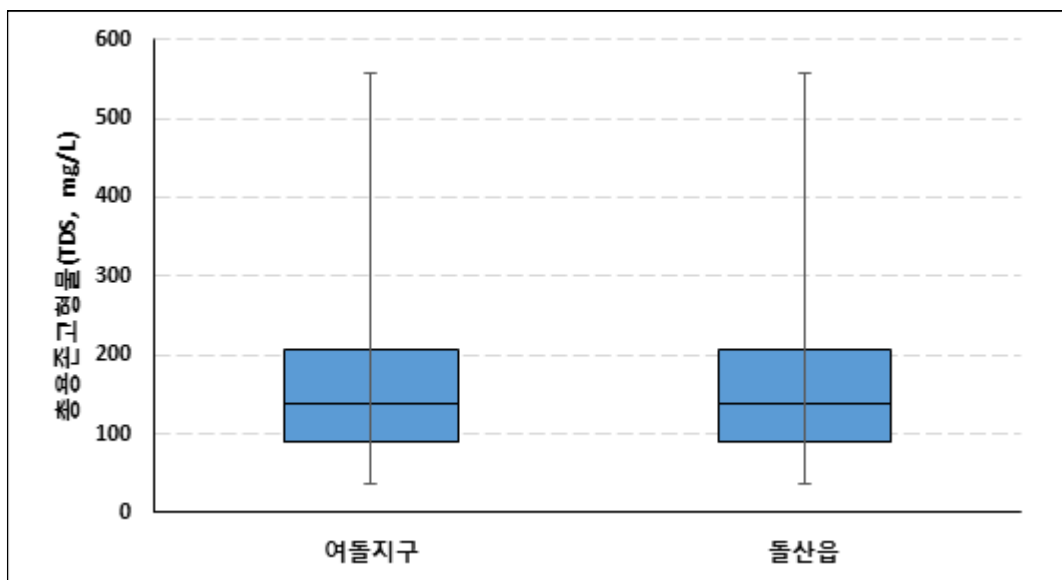
<그림 3-2-16> 여들지구 지하수의 총용존고형물(TDS, mg/L) Box-whisker
