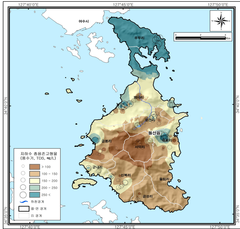
(b) 풍수기 총용존고형물 분포도
