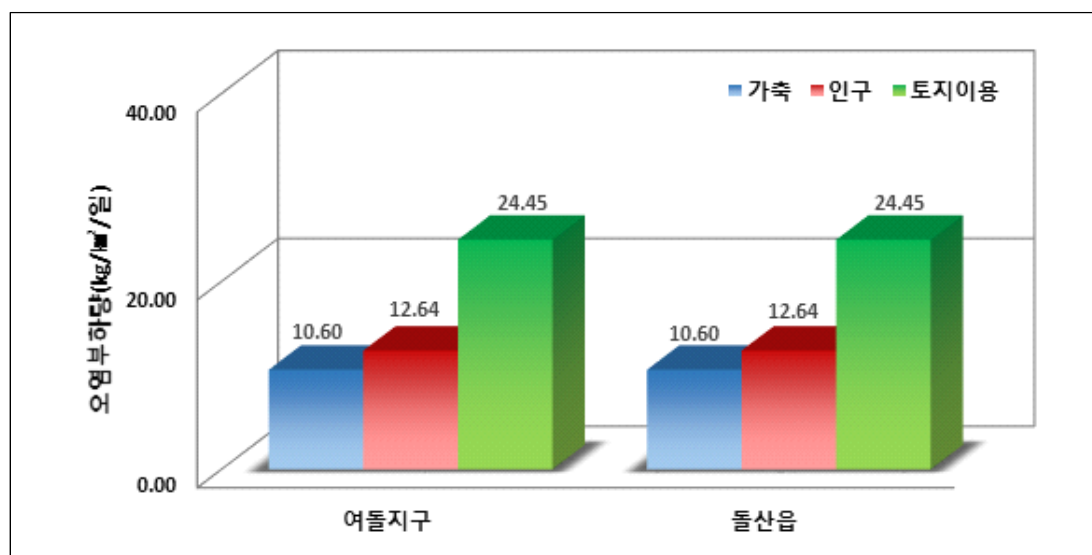
<그림 3-2-3> 읍면별 항목별 단위면적당 오염부하량
