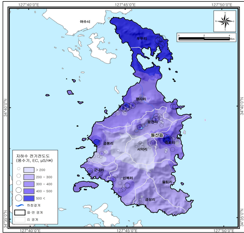
(b) 풍수기 전기전도도 분포도
