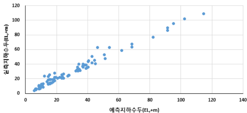
<그림 3-1-2> 실측 지하수두와 예측지하수두
