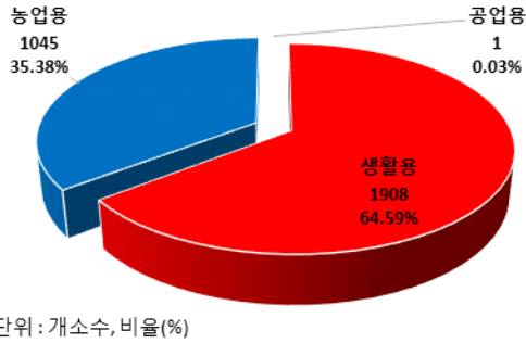
<그림 2-2-2> 용도별 지하수 개소수 <그림 2-2-3> 용도별 지하수 이용량
