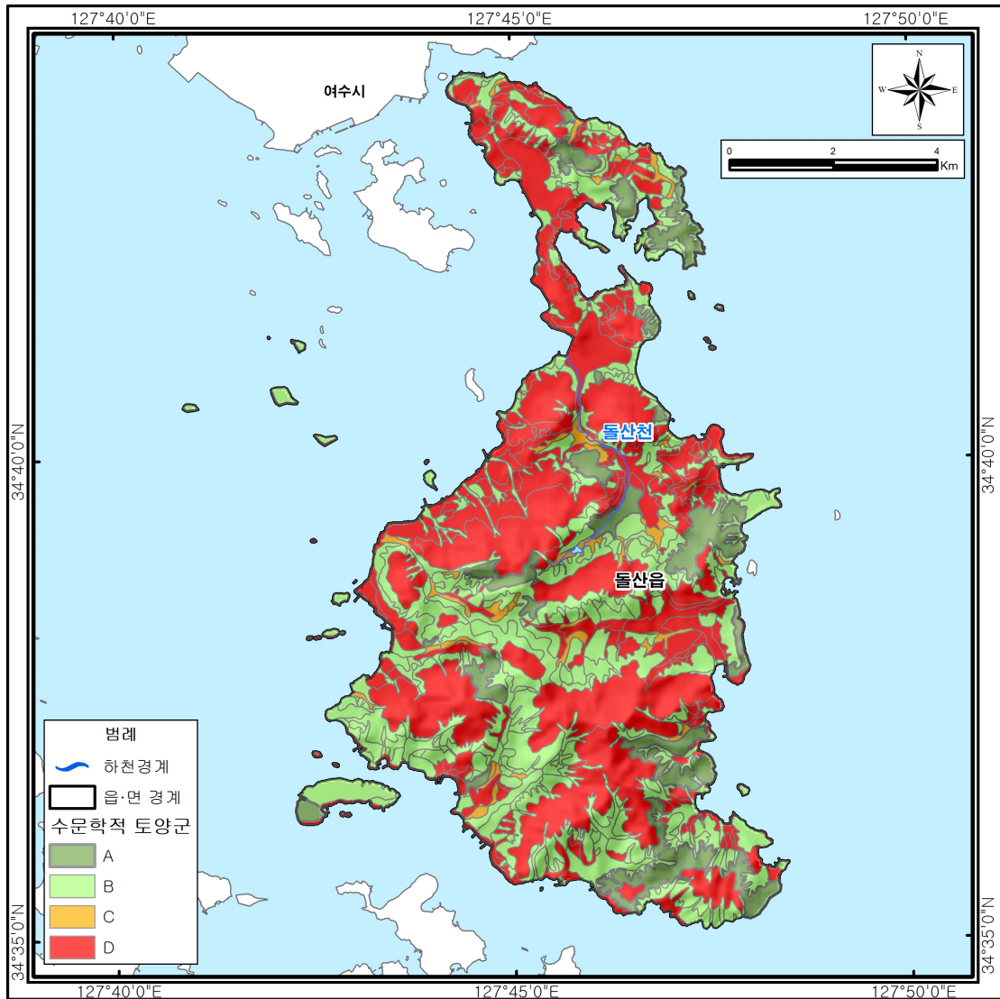
<그림 1-4-6> 여도지구 NRCS 토양도
