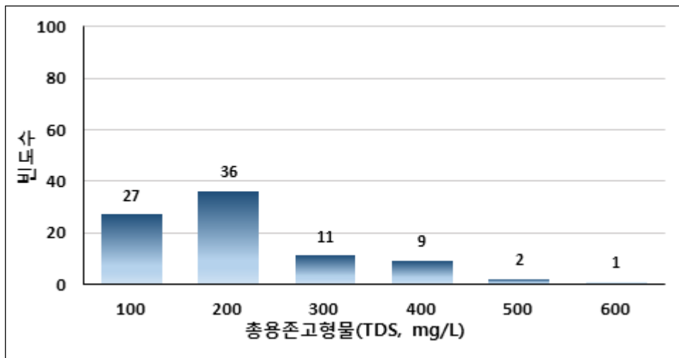
<그림 3-2-15> 여들지구 지하수의 총용존고형물(TDS, mg/L) 빈도분포도
