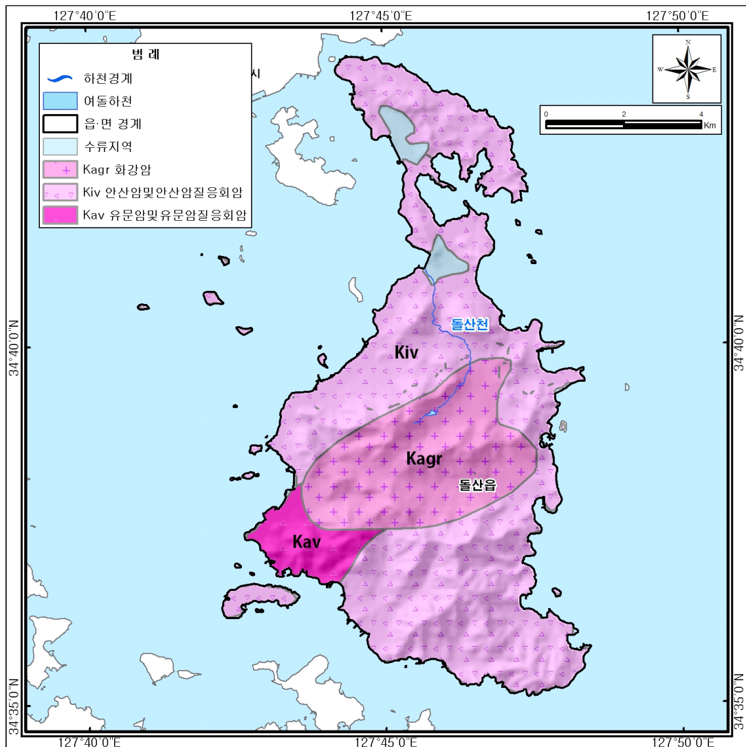
<그림 1-4-4> 여돌지구 지질도
