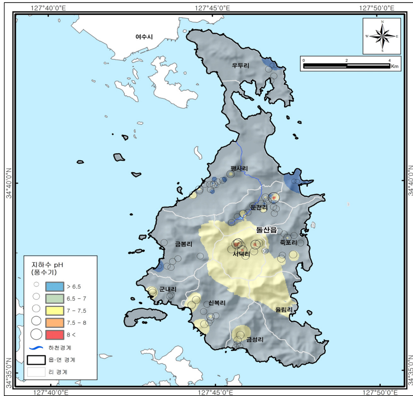
(b) 퐁수기 pH 분포도
