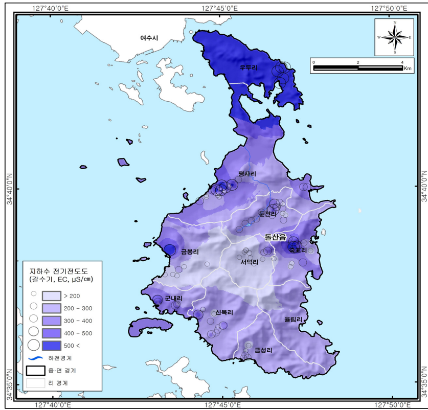
(a) 갈수기 전기전도도 분포도
