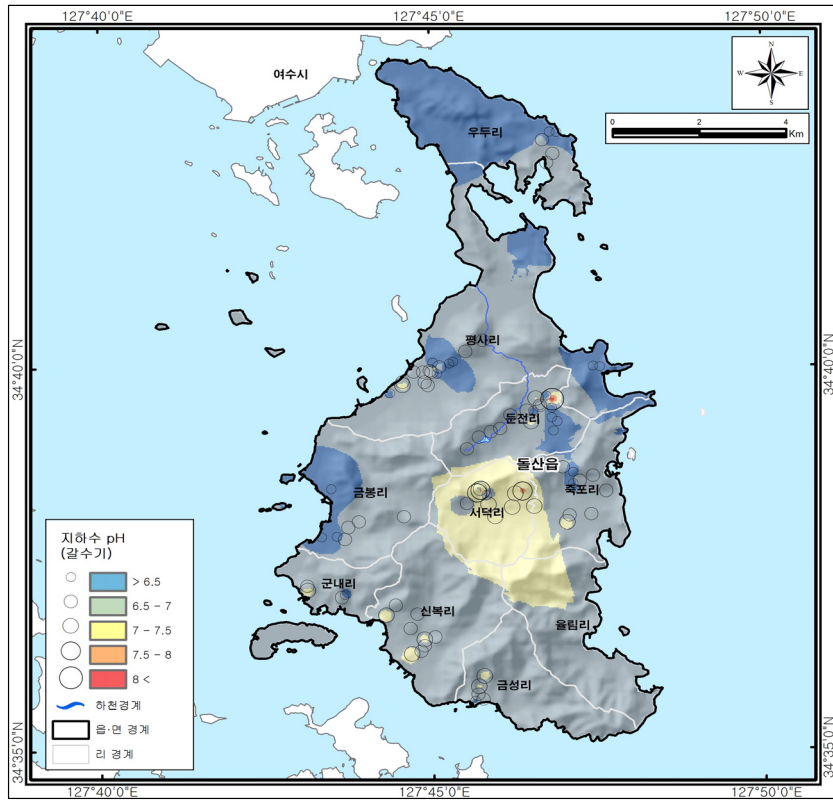
(a) 갈수기 pH 분포도
