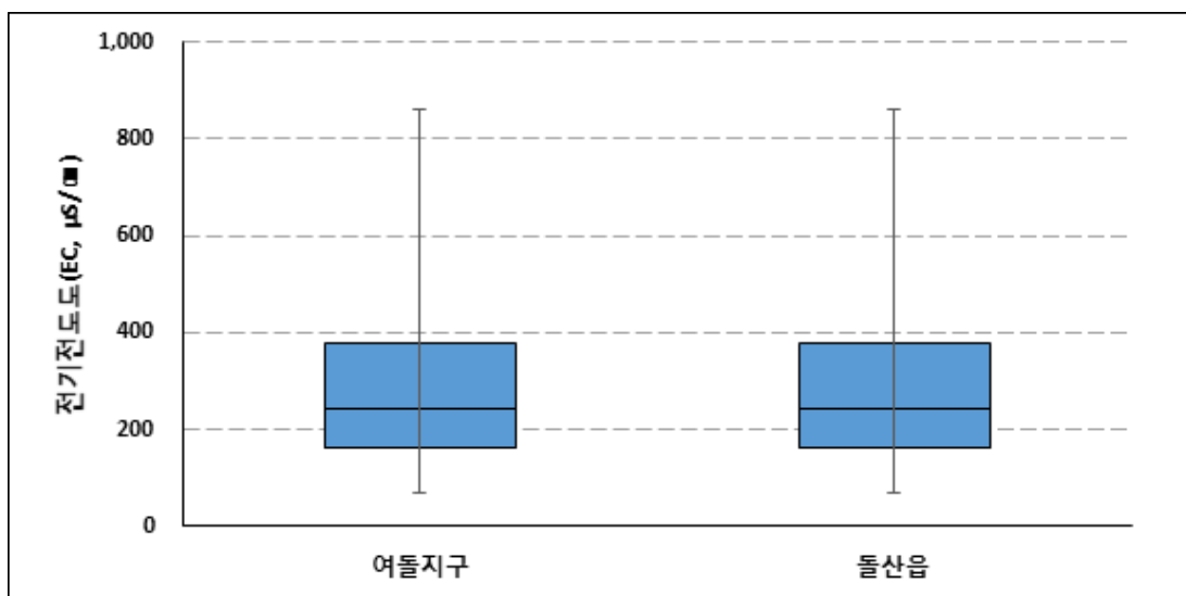
<그림 3-2-13> 여돌지구 지하수의 전기전도도(EC, \mu\text{S}/\text{cm} ) Box-whisker
