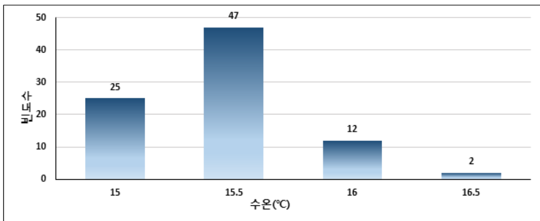
<그림 3-2-6> 여돌지구 지하수의 수온(Temperature, °C) 빈도분포도
