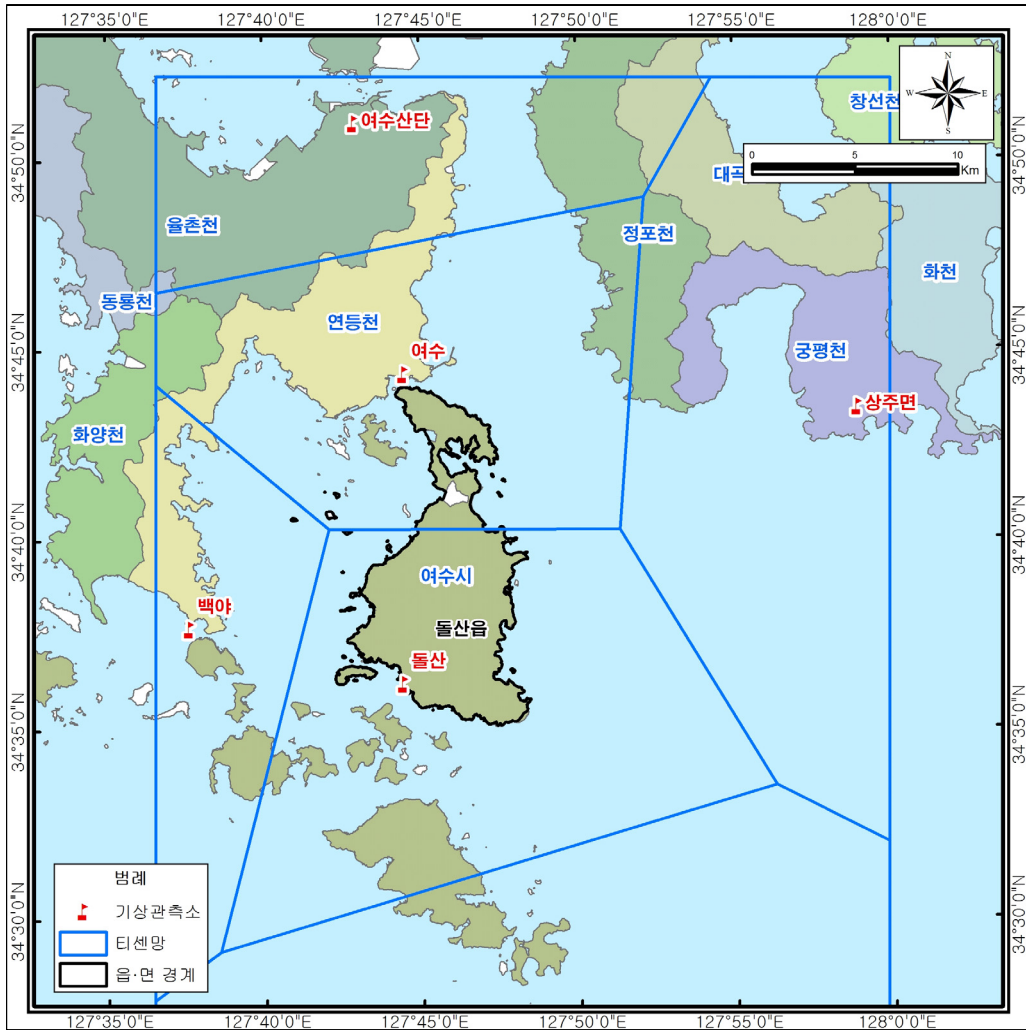
<그림 3-1-9> 조사지역 Thiessen망도
