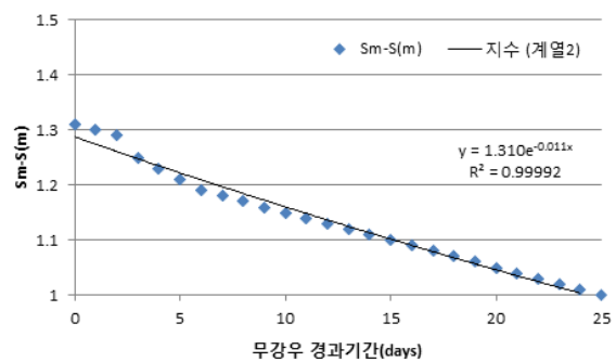
<그림 3-1-10> 지하수 수위 무강우 일수 산정 및 감수곡선
