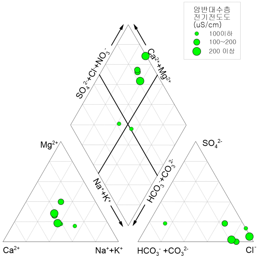
<그림 3-2-25> 여돌지구 암반 지하수의 Piper Diagram
