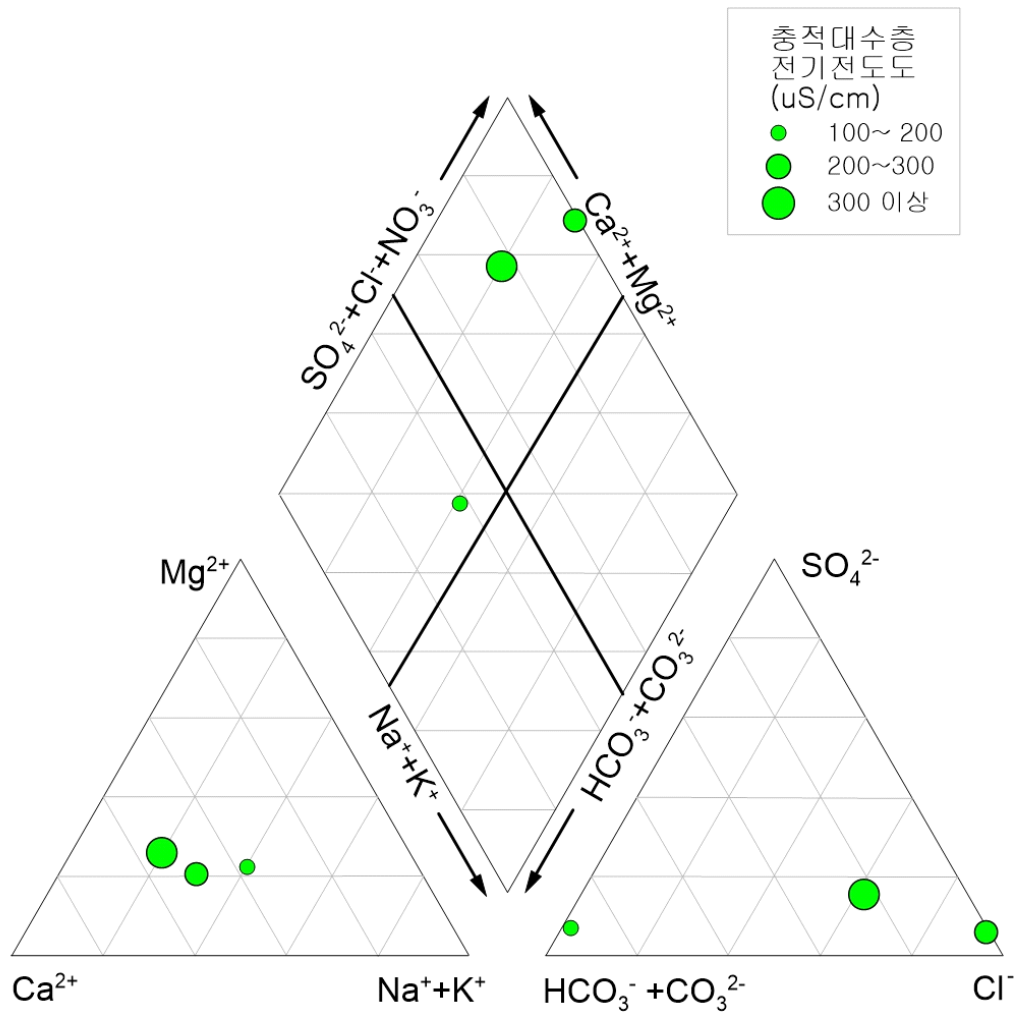
<그림 3-2-26> 여돌지구 총적 지하수의 Piper Diagram
