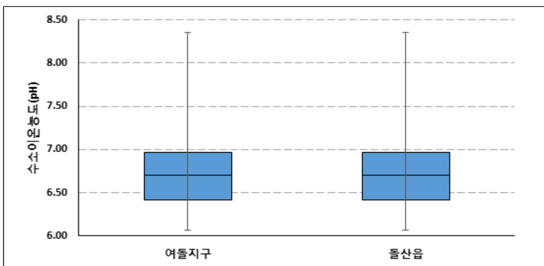
<그림 3-2-10> 여돌지구 지하수의 pH Box-whisker
