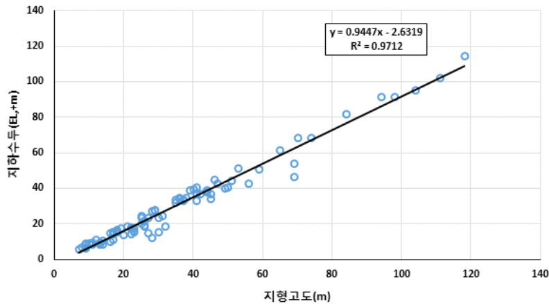
<그림 3-1-1> 지형고도와 지하수두 선형회귀분석
