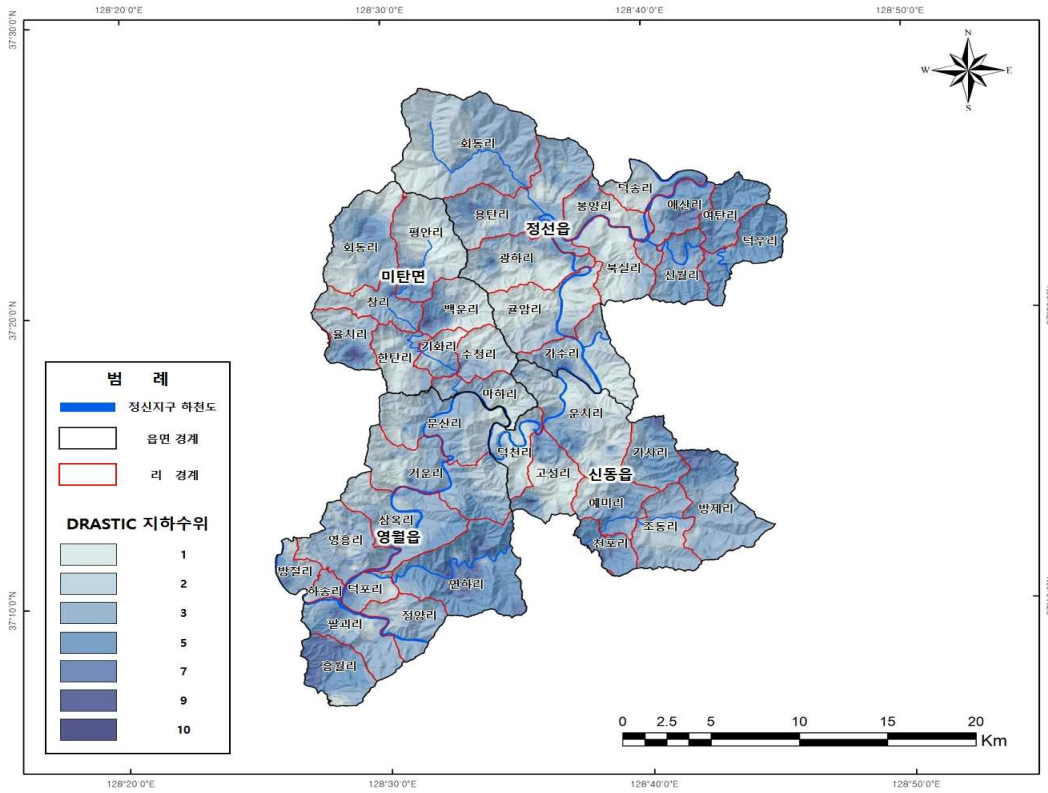
<그림 3-3-2> 지하수위
