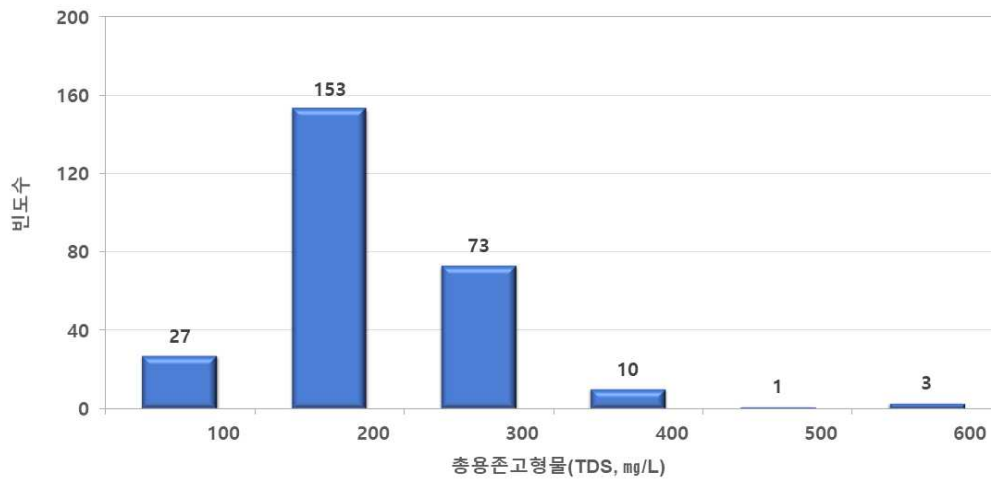
<그림 3-2-15> 지하수 총용존고형물(TDS, mg/L) 빈도분포도
