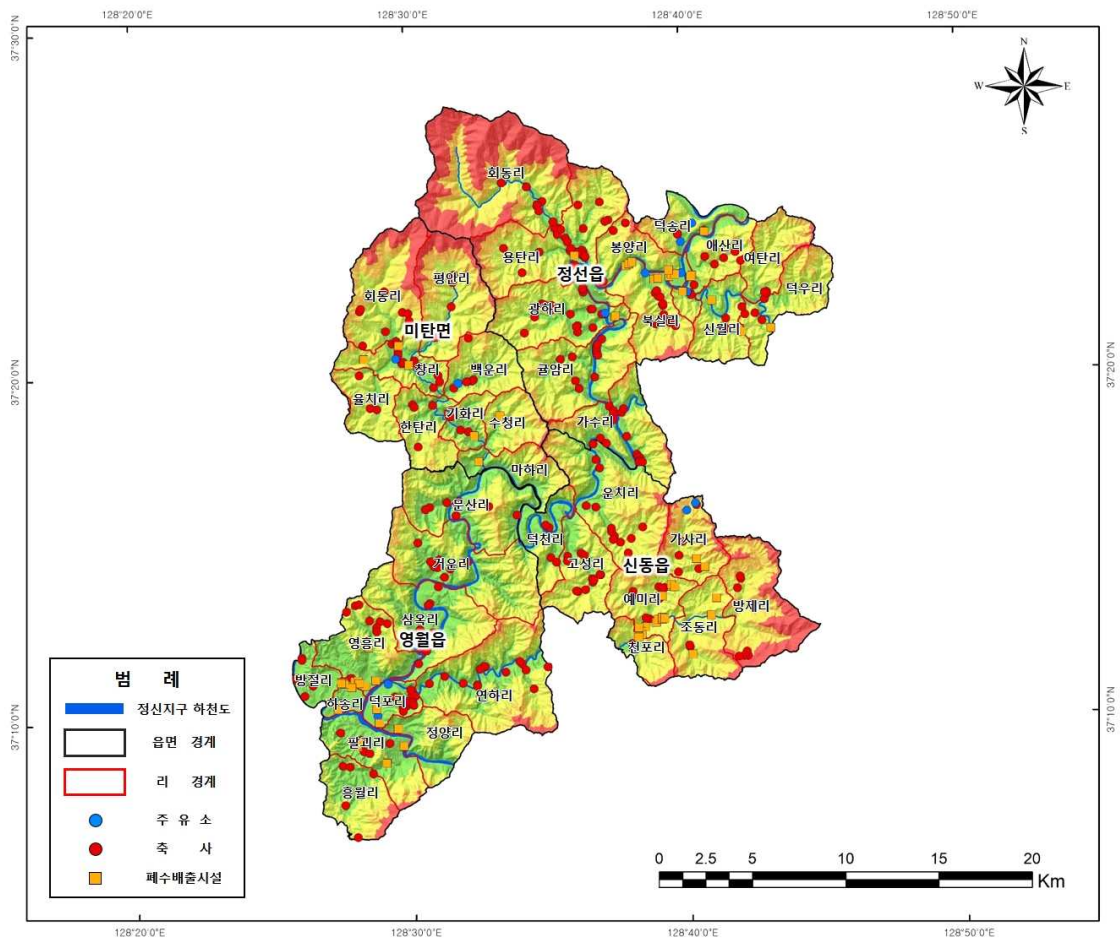
<그림 3-2-2> 환경기초시설 및 점오염원 분포현황도
