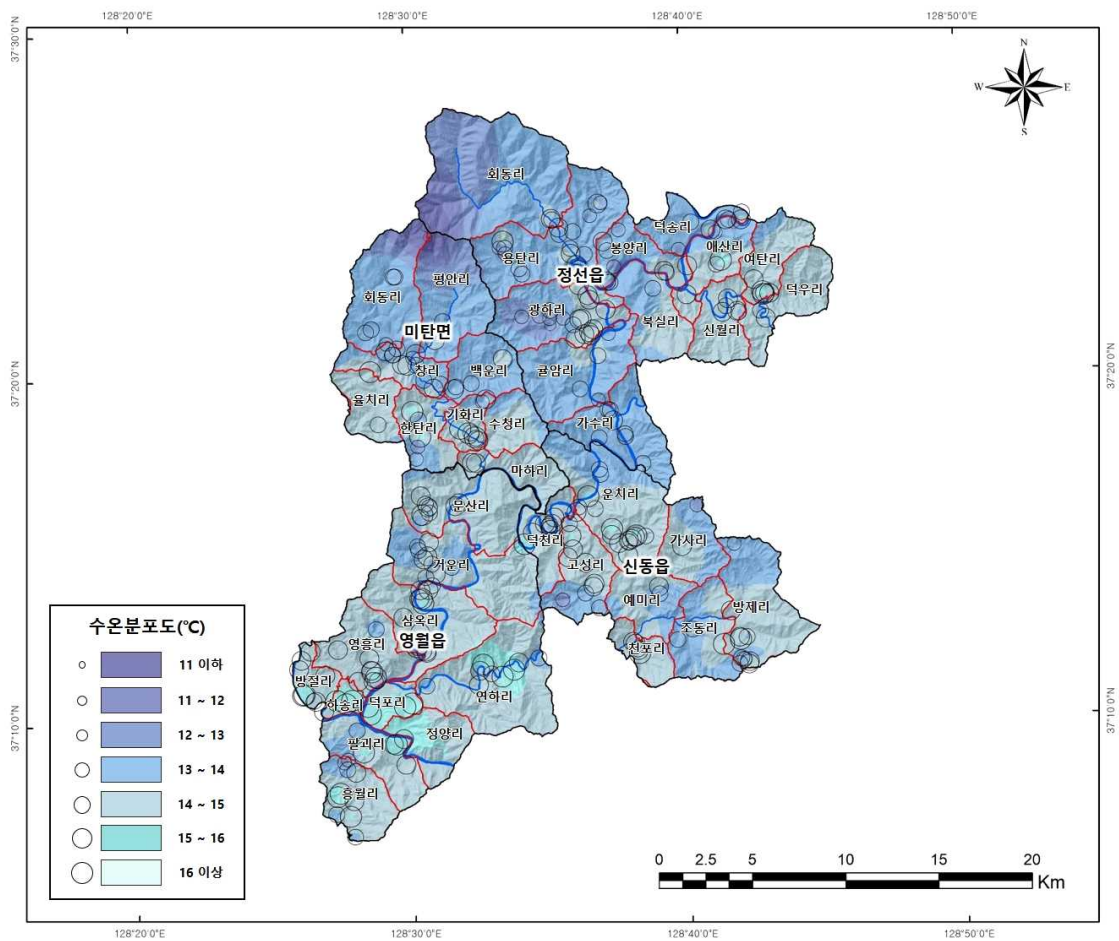
<그림 3-2-8> 정신지구 지하수의 수온(°C) 분포도
