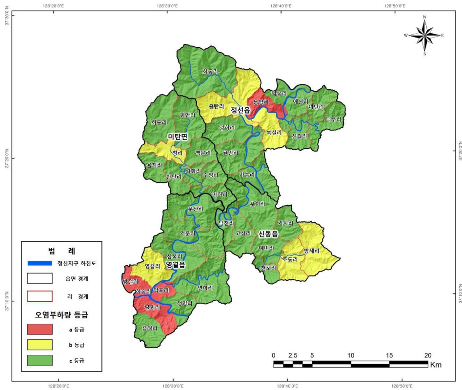
<그림 3-2-7> 발생단위별 잠재오염원 부하량 등급도
