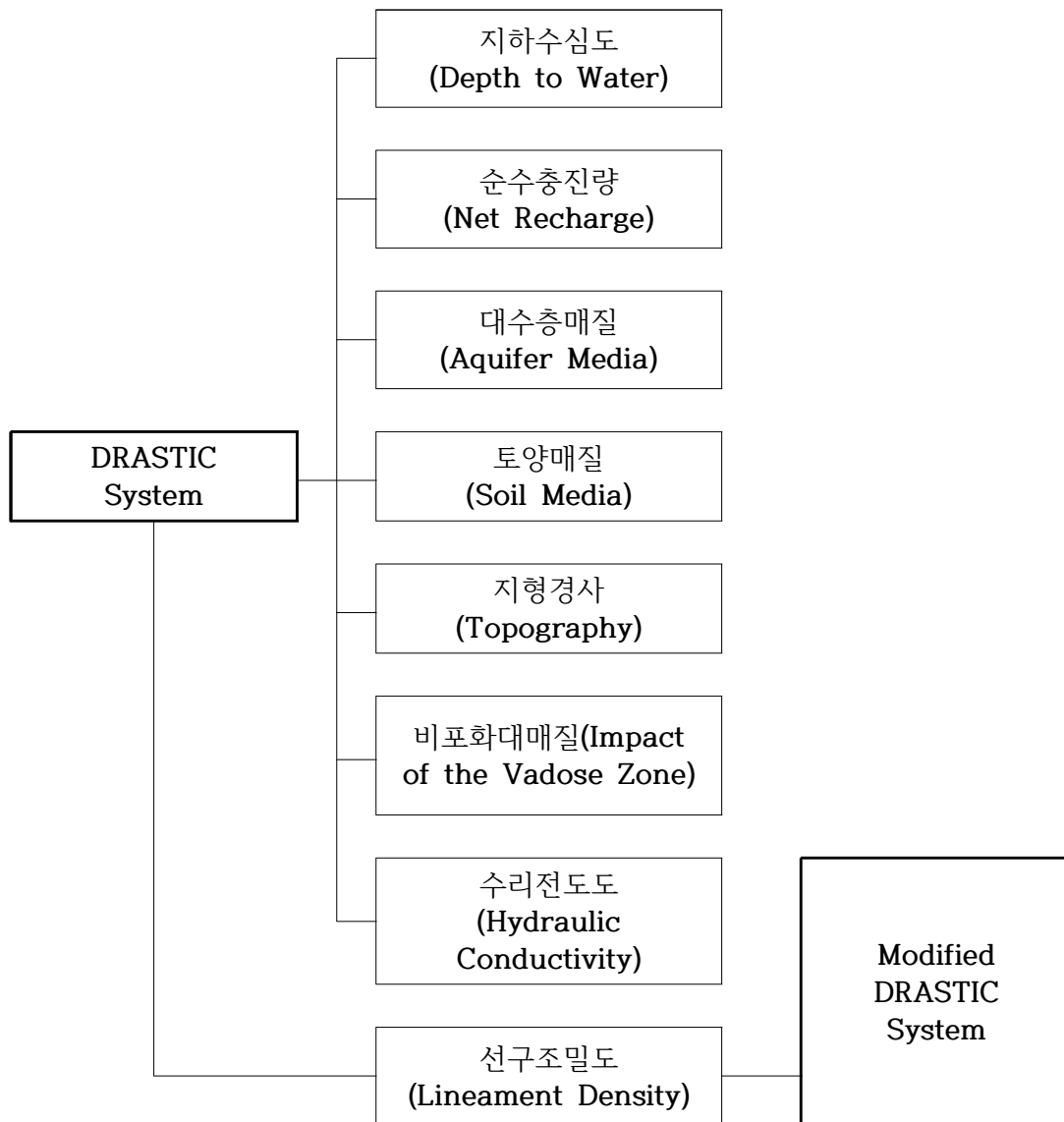
<그림 3-3-1> DRASTIC 흐름도
