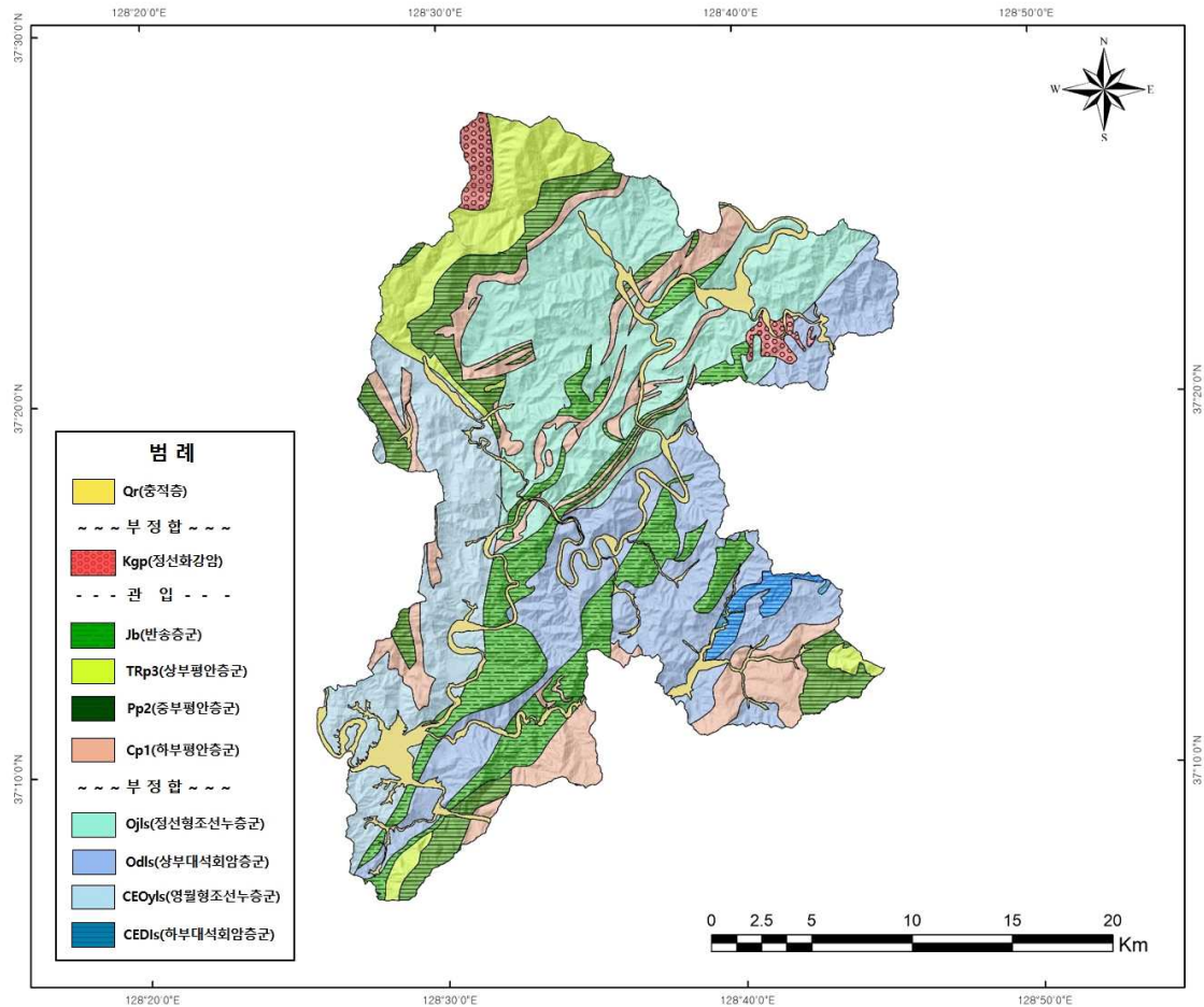
<그림 1-4-4> 정신지구 지질도
