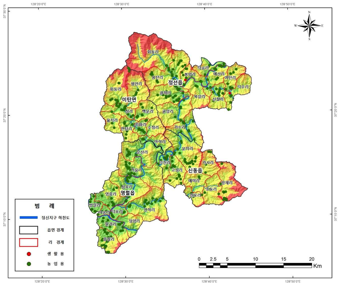
<그림 1-4-5> 용도별 지하수개발 위치도(금회조사)
