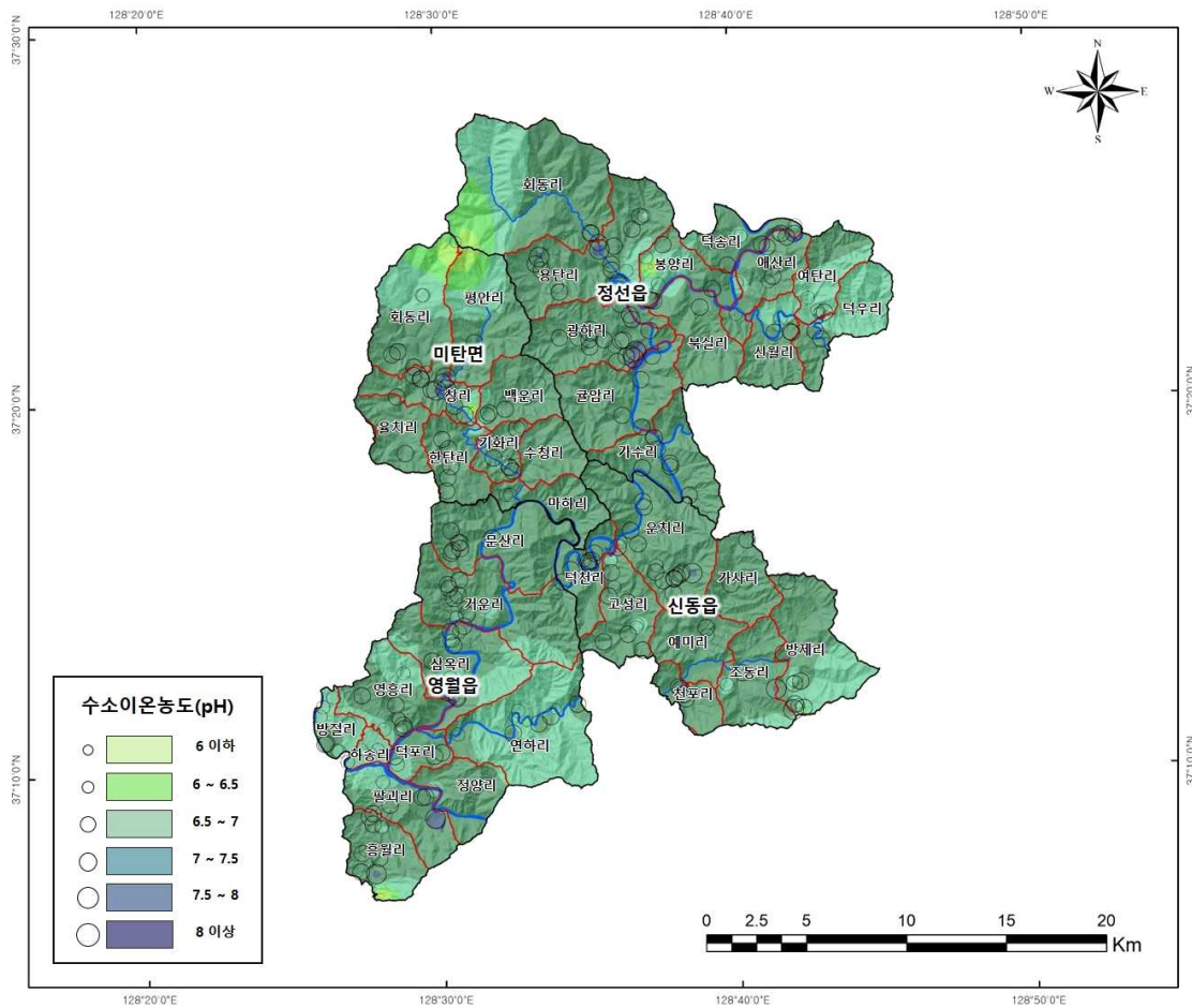
<그림 3-2-11> 정선지구 지하수 pH 분포도
