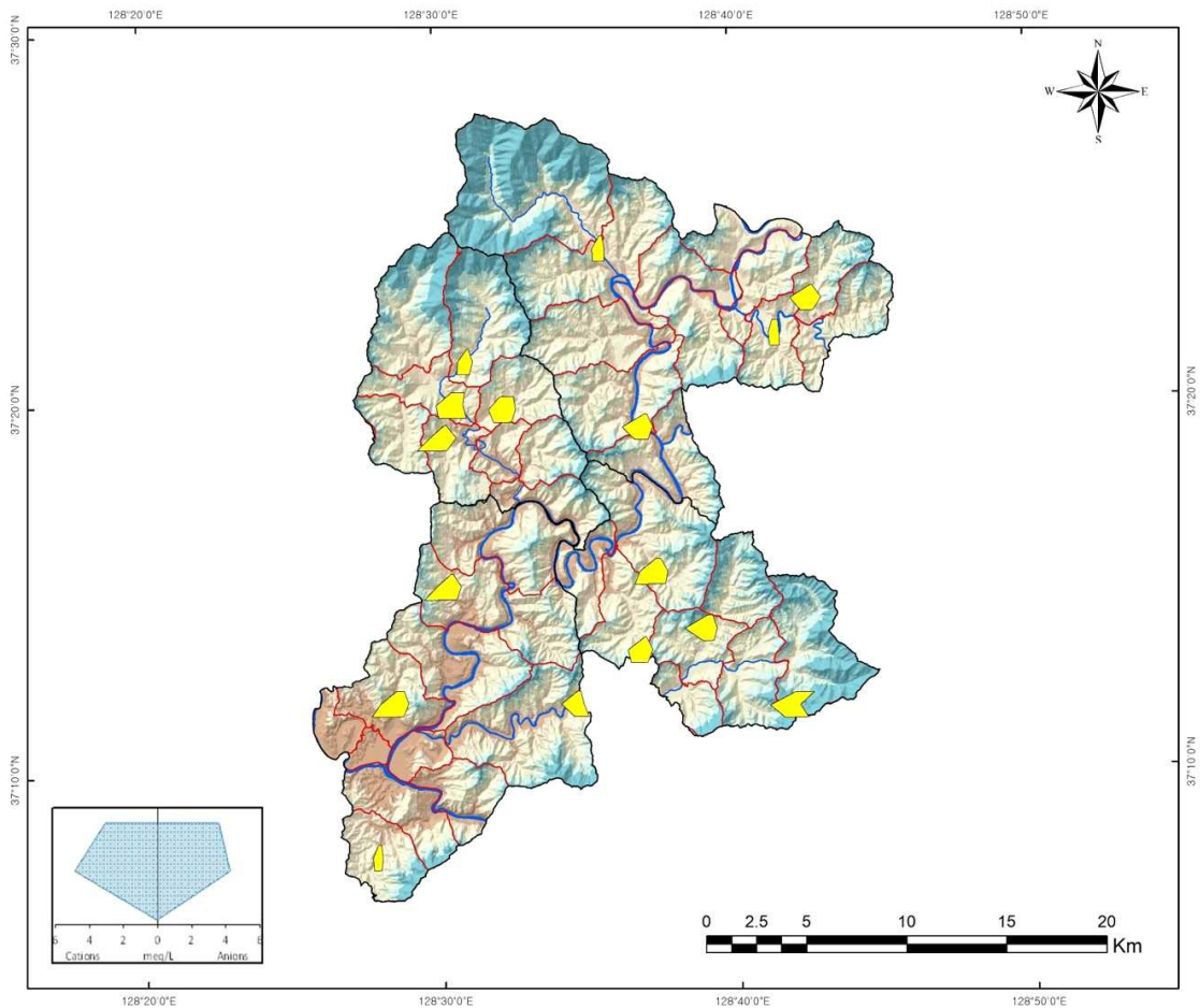
<그림 3-2-25> 정신지구 지하수의 Stiff Diagram
