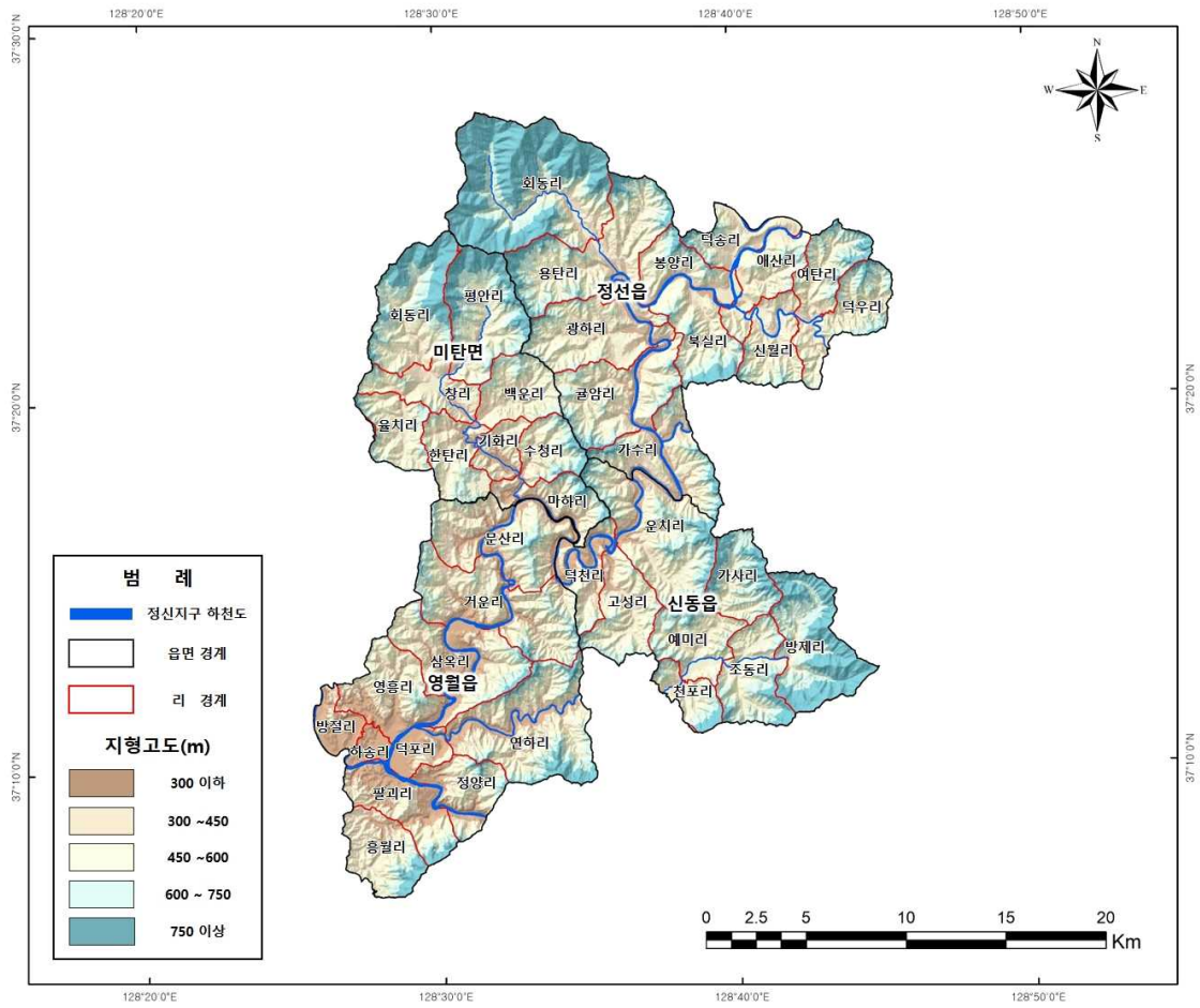
<그림 1-4-3> 지형고도 분포
