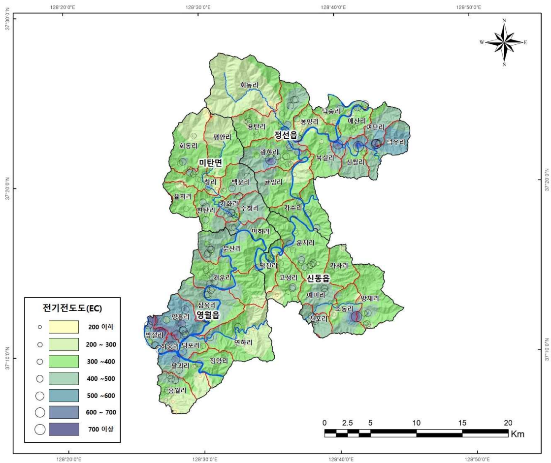
<그림 3-2-14> 지하수 전기전도도(EC, \mu\text{S}/\text{cm} ) 분포도
