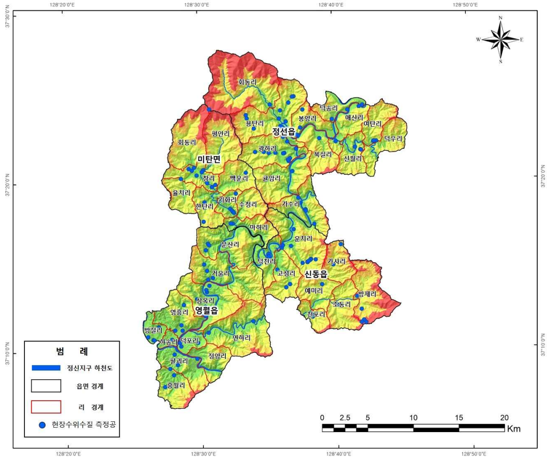
<그림 3-2-5> 정신지구 간이수질 측정공 위치도
