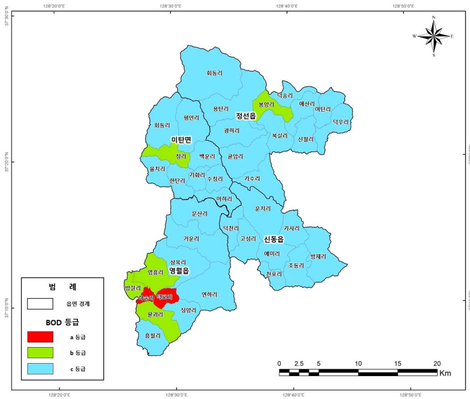
<그림 3-2-5> BOD 발생부하량 등급도
