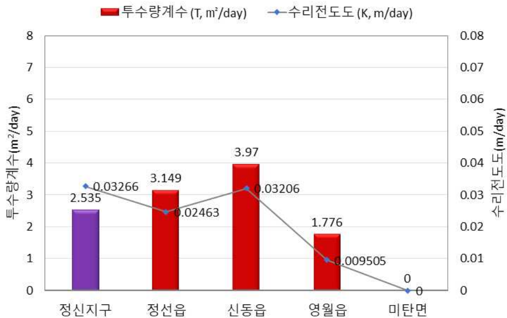
<그림 3-1-4> 읍면별 지하수 투수량계수 및 수리전도도(기하평균)
