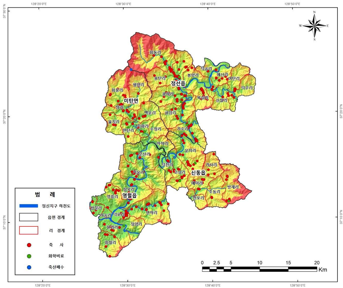
<그림 3-2-19> 질소동위원소 오염원별 위치도
