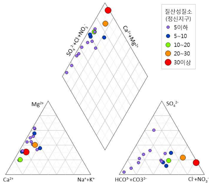
<그림 3-2-23> 지하수 Piper Diagram(질산성질소)
