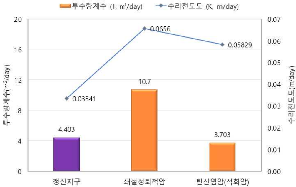
<그림 3-1-6> 수문지질별 지하수 투수량계수 및 수리전도도(산술평균)
