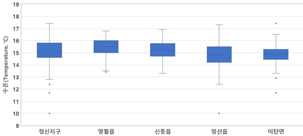
<그림 3-2-7> 정신지구 지하수의 수온(T) Box-whisker
