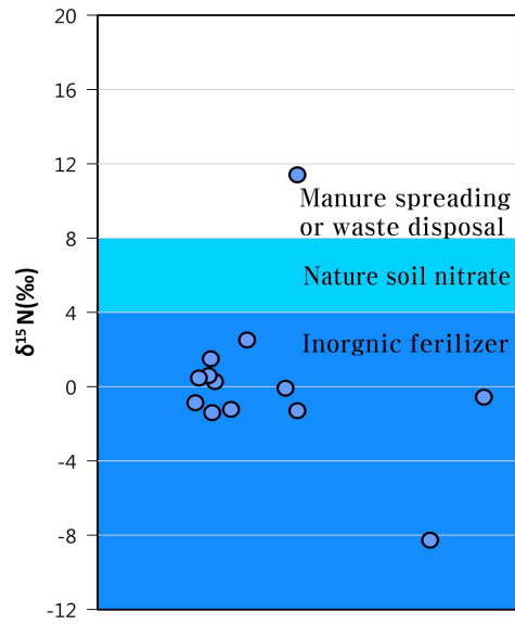
<그림 3-2-20> NO 3 -N과 δ 15 N의 관계
