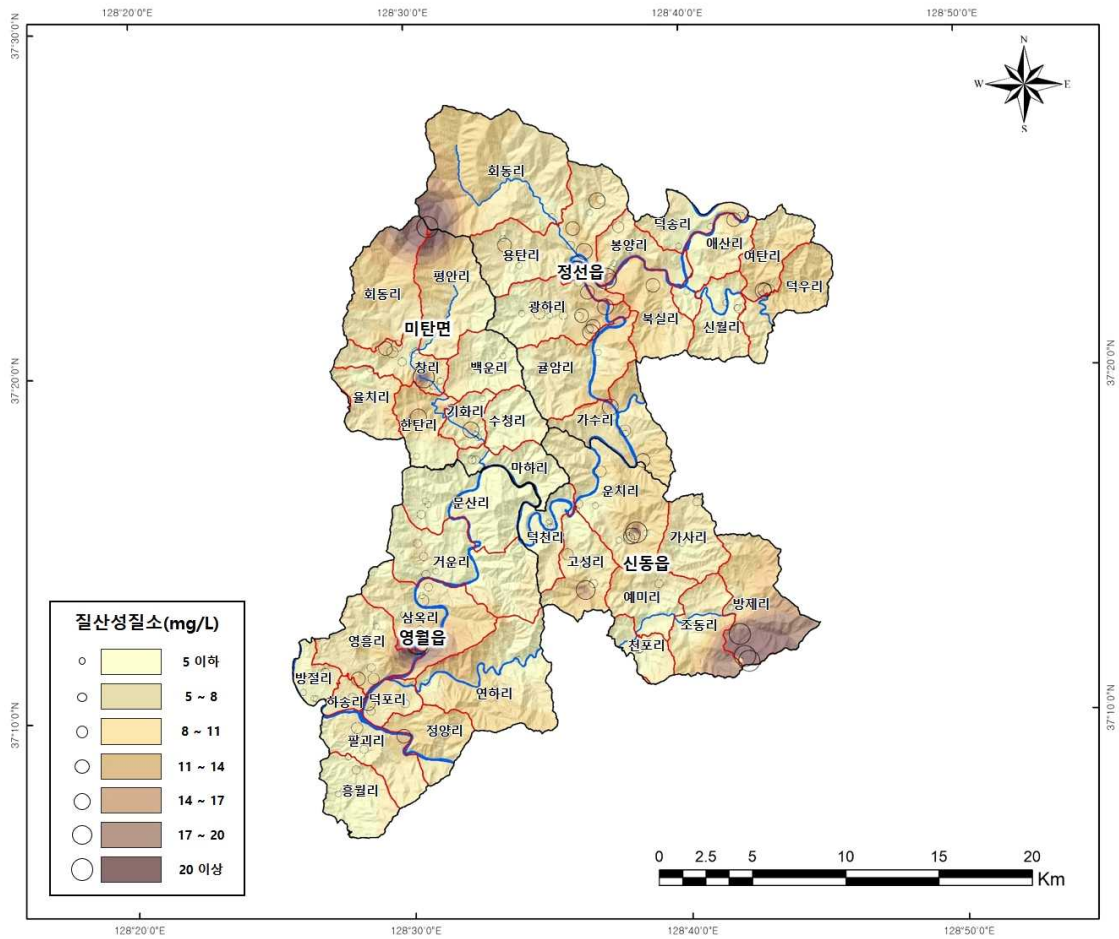
<그림 3-2-18> 정신지구 지하수의 질산성질소(mg/L) 분포도
