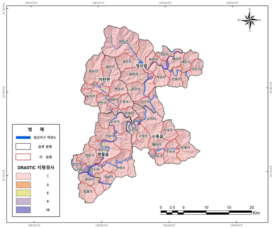
<그림 3-3-6> 지형경사
