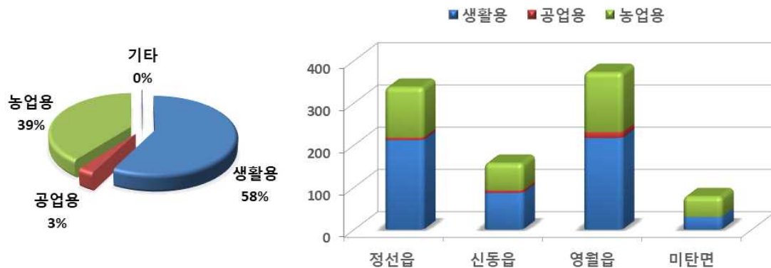
<그림 1-4-4> 읍면별 · 용도별 지하수 개발현황
