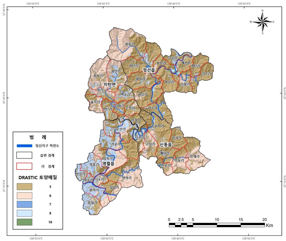
<그림 3-3-5> 토양 매질
