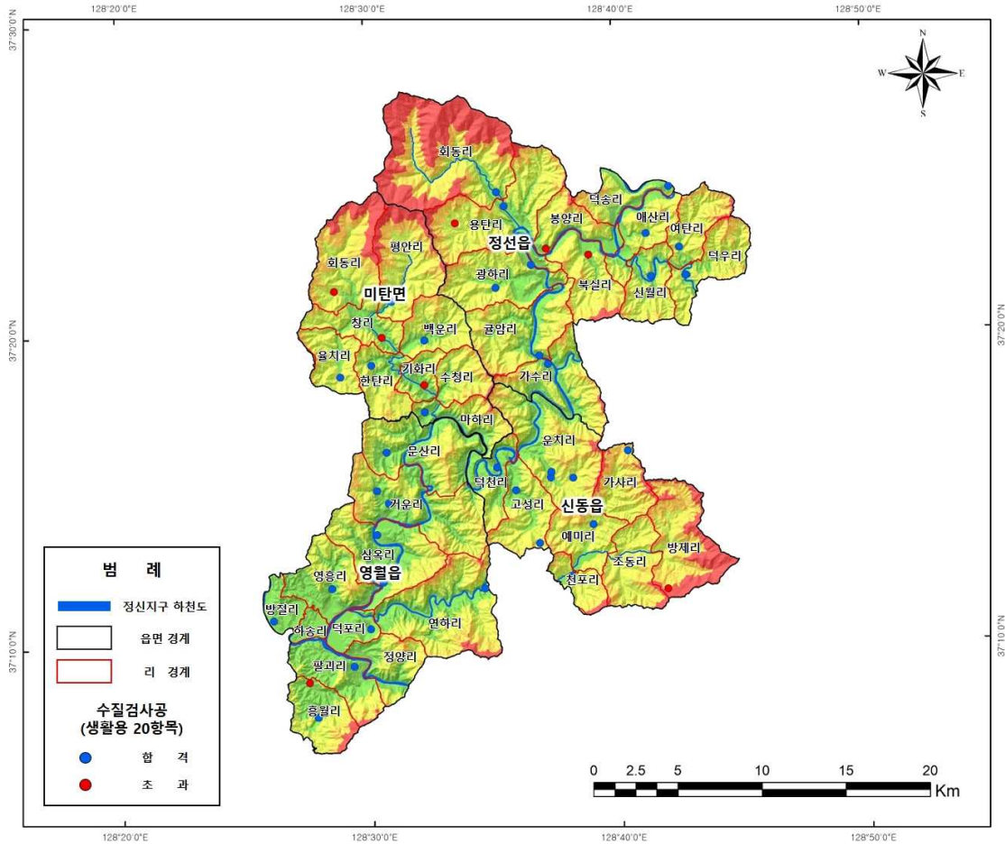
<그림 3-2-21> 수질검사 및 초과지점 분포도
