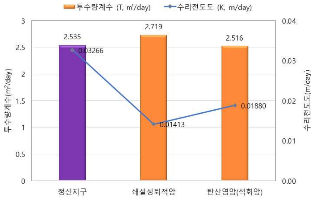
<그림 3-1-7> 수문지질별 지하수 투수량계수 및 수리전도도(기하평균)
