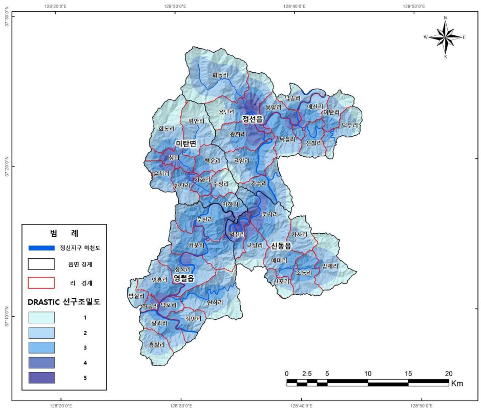
<그림 3-3-10> 선구조밀도
