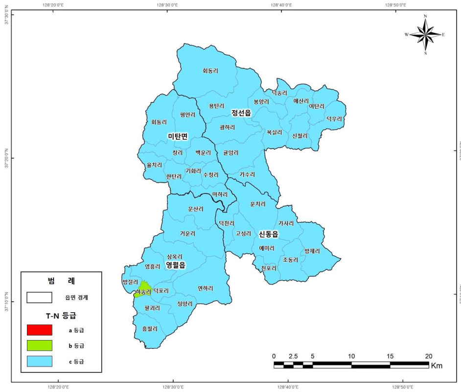
<그림 3-2-4> T-N 발생부하량 등급도
