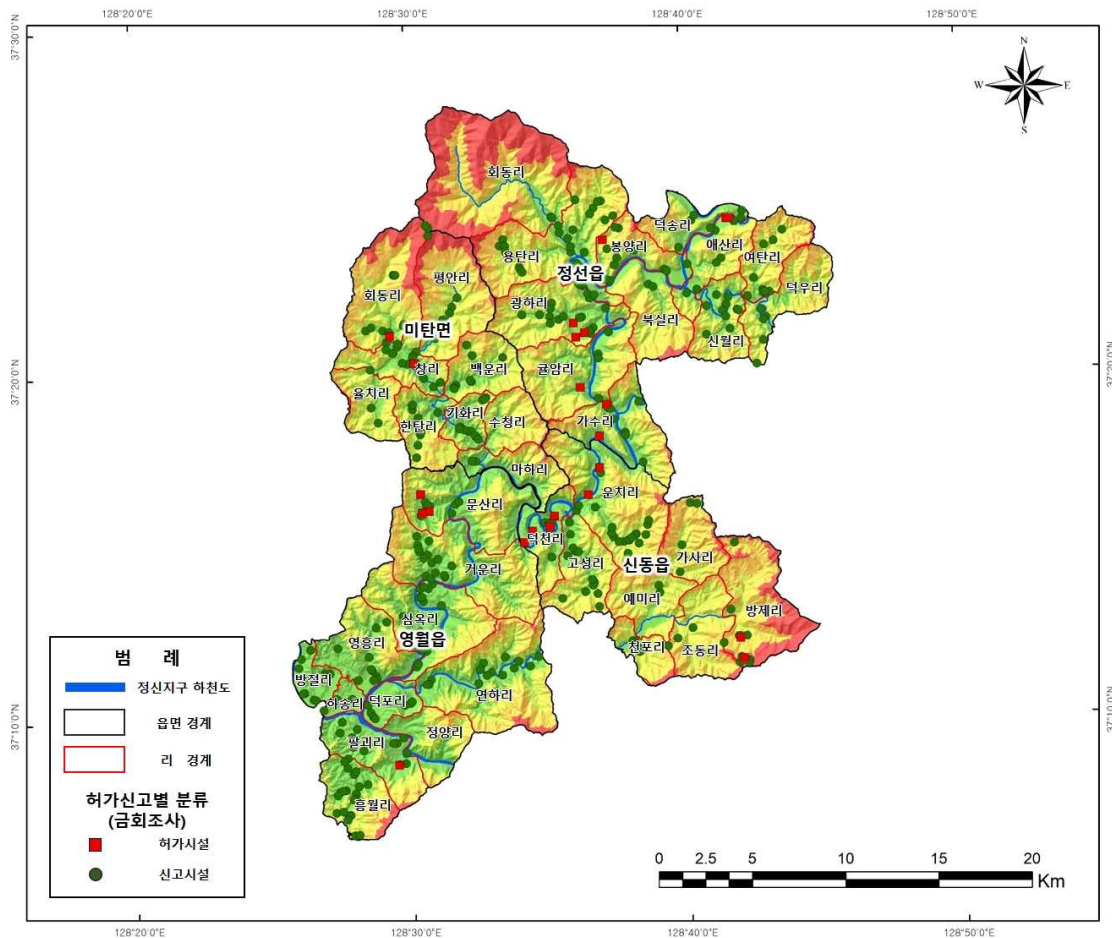
<그림 2-1-1> 허가/신고 형태별 관정 현황도
