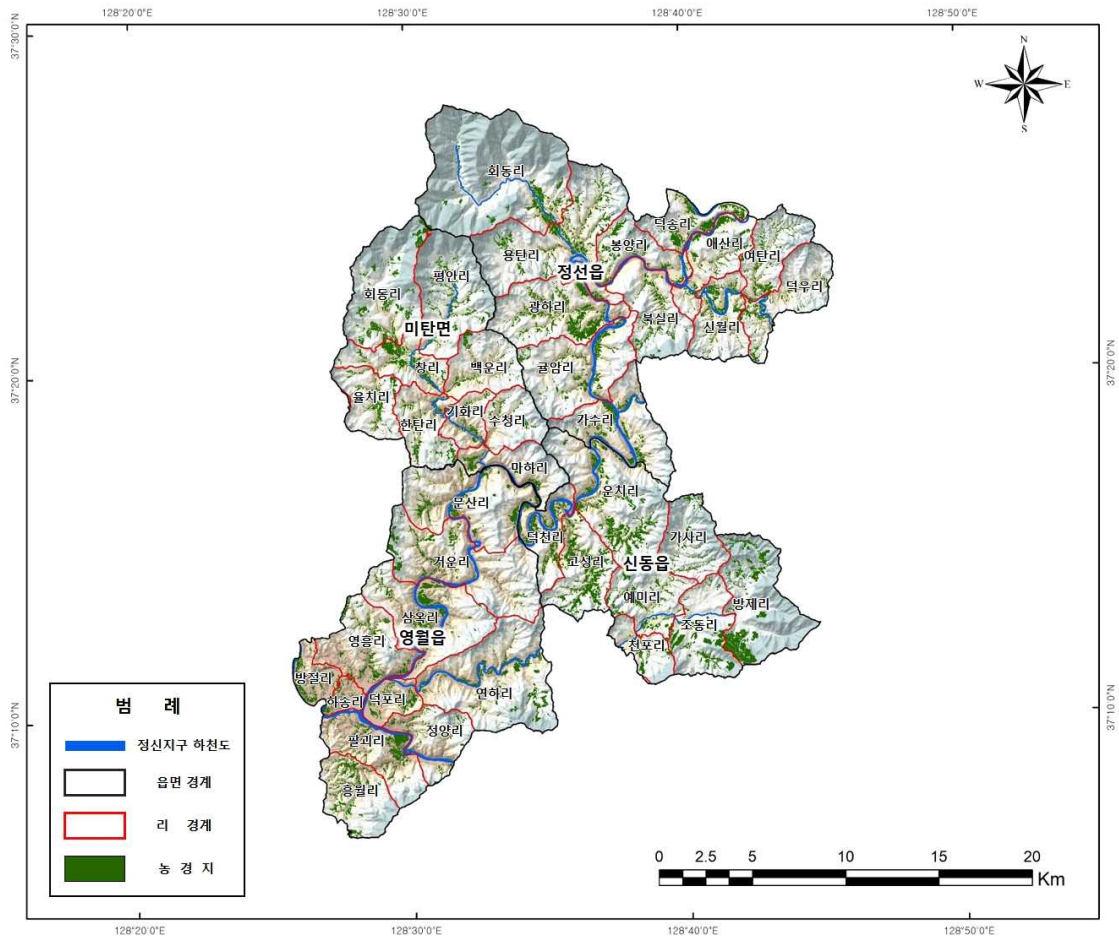
<그림 1-3-1> 농지분포도
