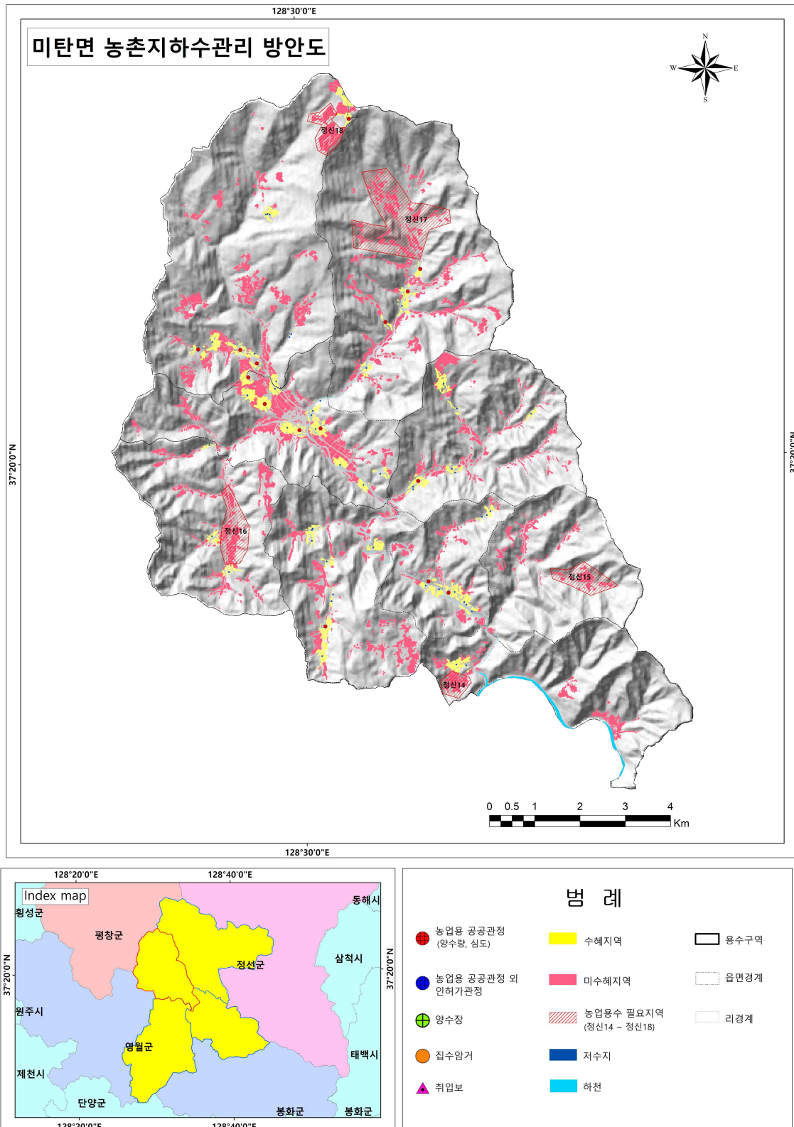
<그림 4-3-6> 미탄면 농촌지하수관리 방안도
