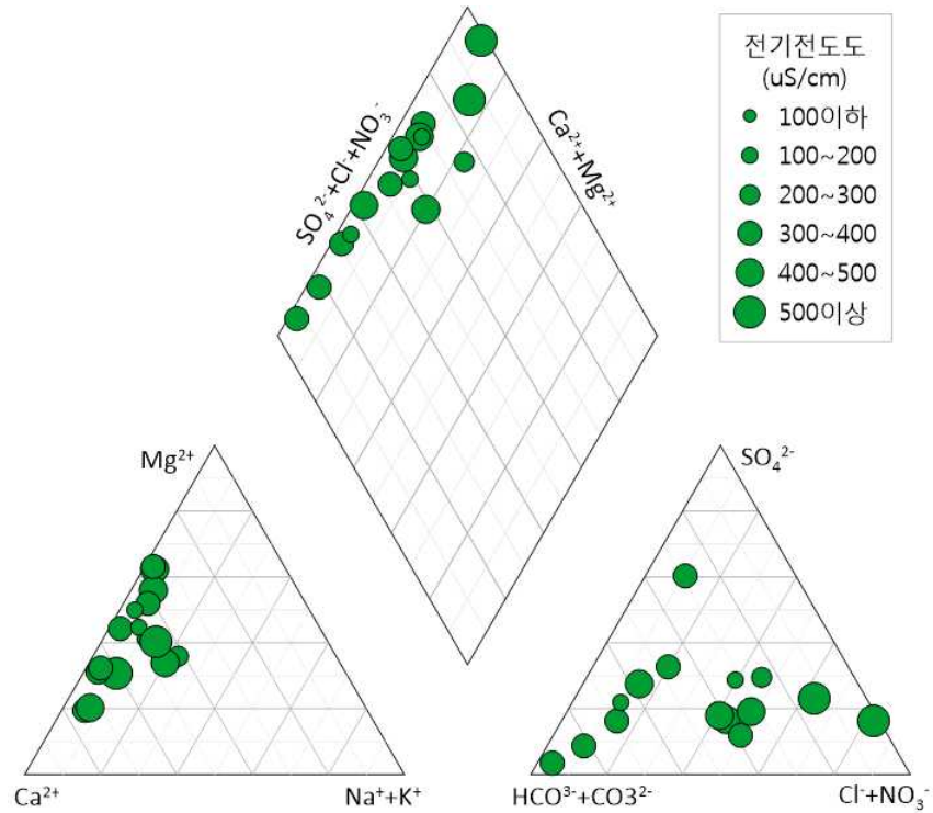
<그림 3-2-24> 지하수 Piper Diagram(전기전도도)
