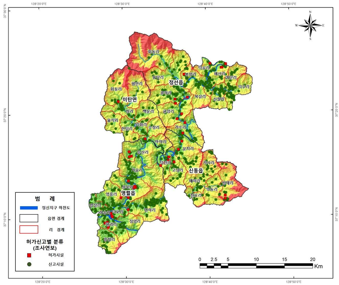
<그림 1-4-3> 허가/신고 형태별 관정 현황도(조사연보)
