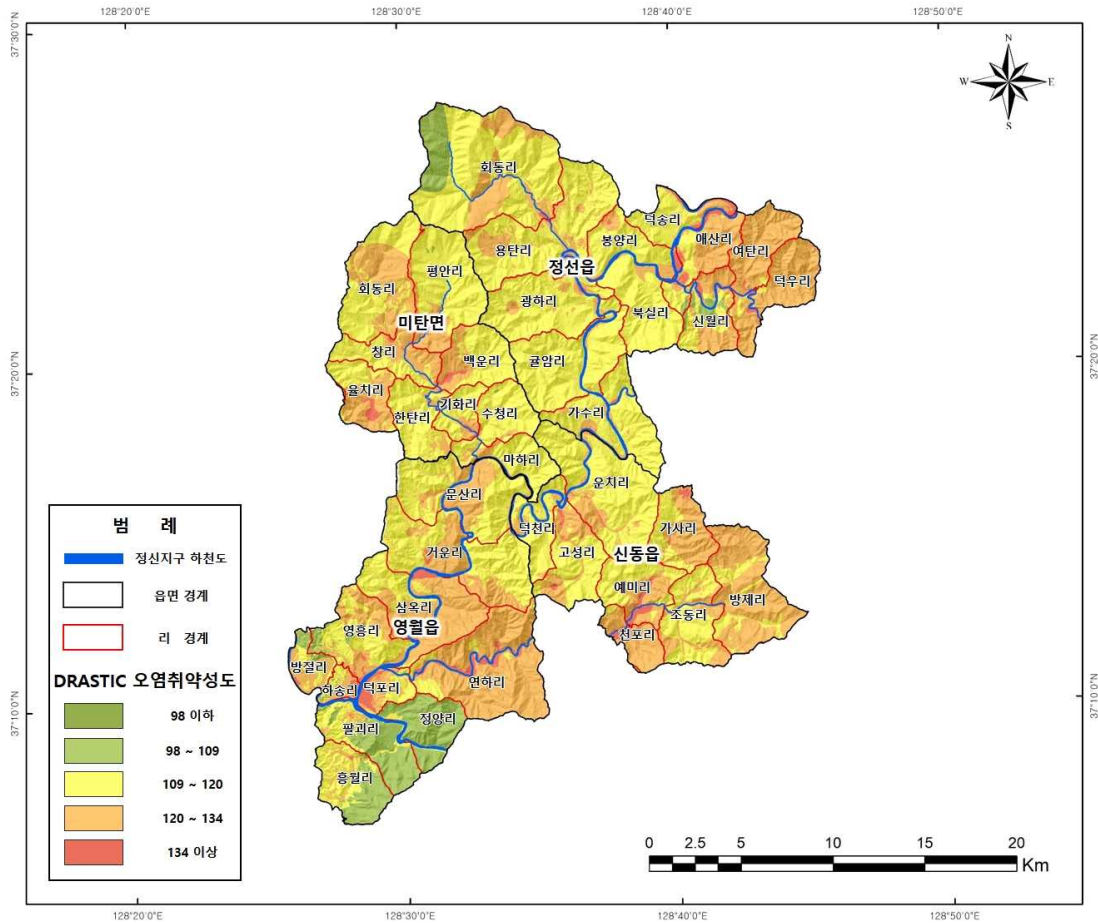
<그림 3-3-9> 오염취약성도(DRASTIC Index Map)
