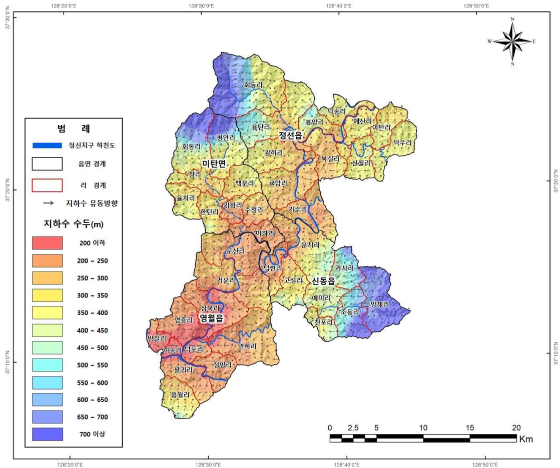
<그림 3-1-1> 지하수두 및 유동방향도
