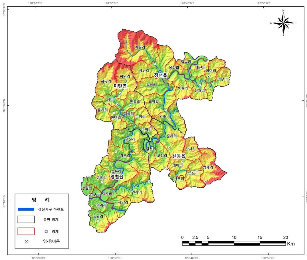
<그림 3-2-22> 양·음이온 분석시료 채수 위치도
