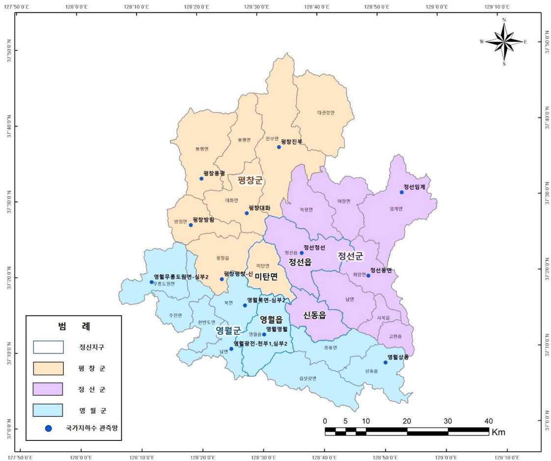
<그림 1-4-7> 국가 지하수관측망 위치도
