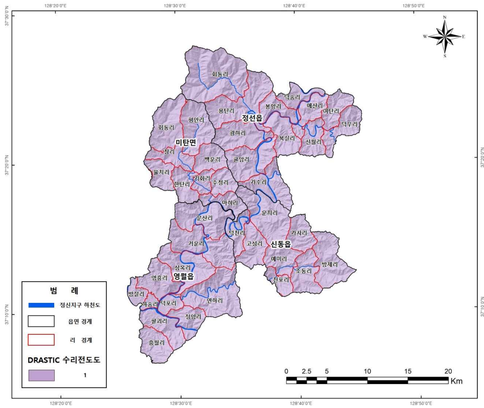
<그림 3-3-8> 수리전도도
