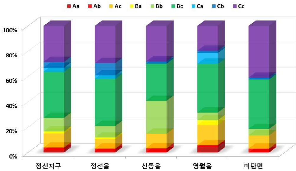
<그림 3-2-10> 지하수오염예측도 등급별 면적비
