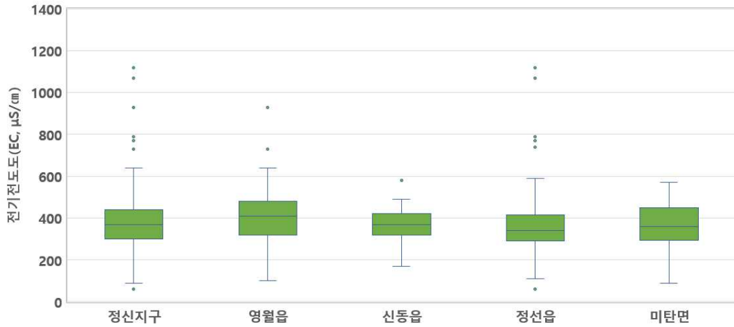
<그림 3-2-13> 지하수 전기전도도(EC, \mu\text{S}/\text{cm} ) Box-whisker
