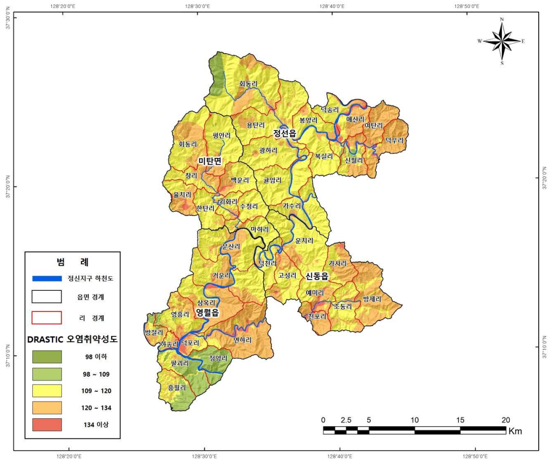
<그림 3-2-2> 정신지구 오염취약성 지수(DRASTIC INDEX Map)
