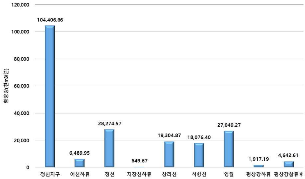
<그림 3-1-9> 표준유역별 지하수 함양량
