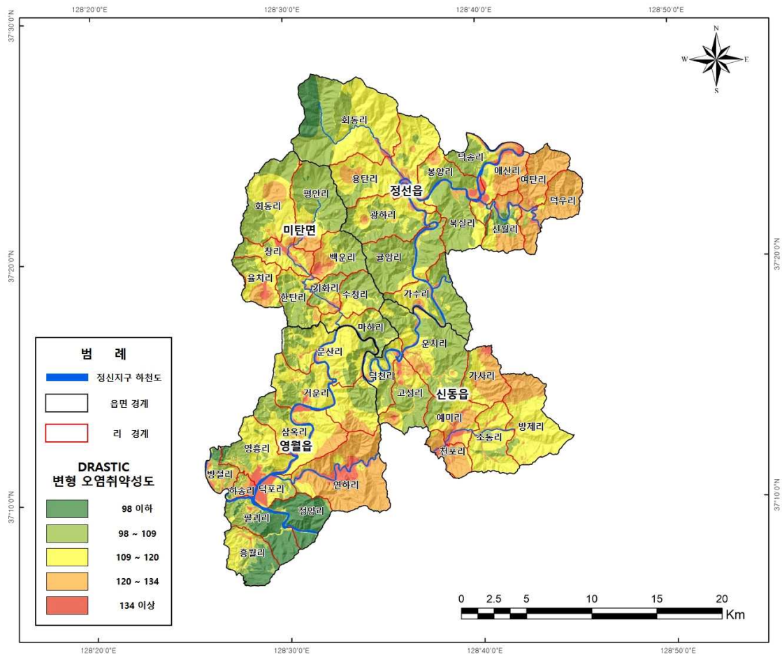
<그림 3-2-3> 정신지구 변형오염취약성지수(Modified DRASTIC INDEX Map)
