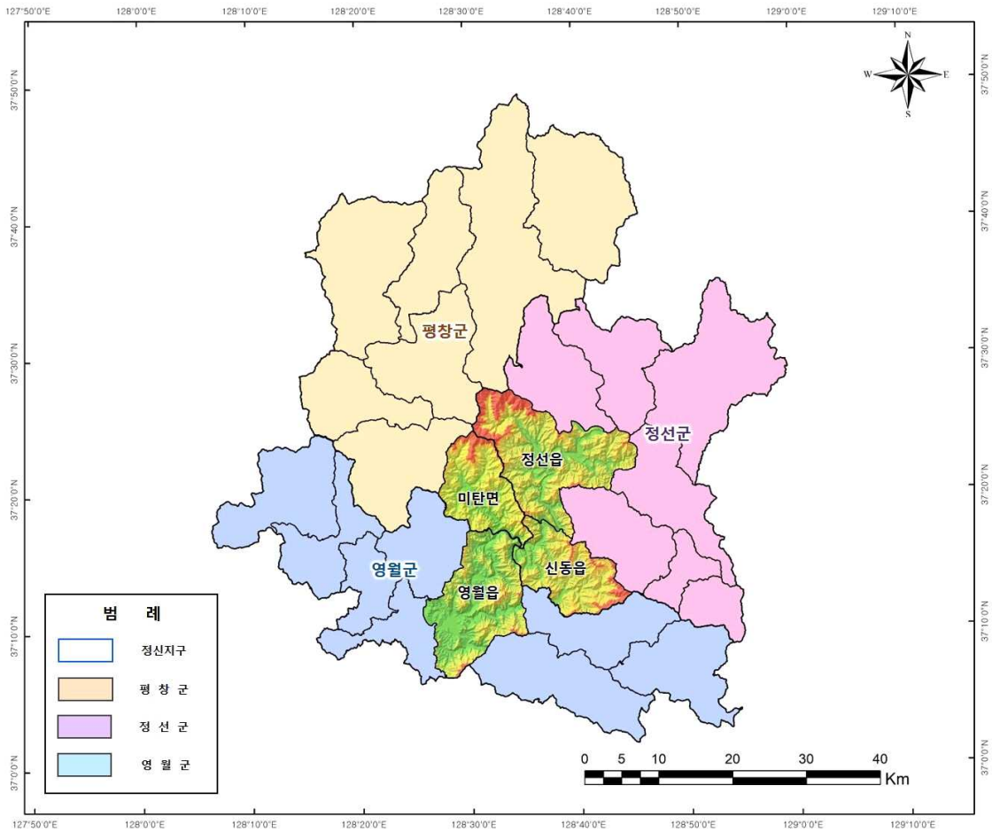
<그림 1-4-1> 정신지구 용수구역 위치도
