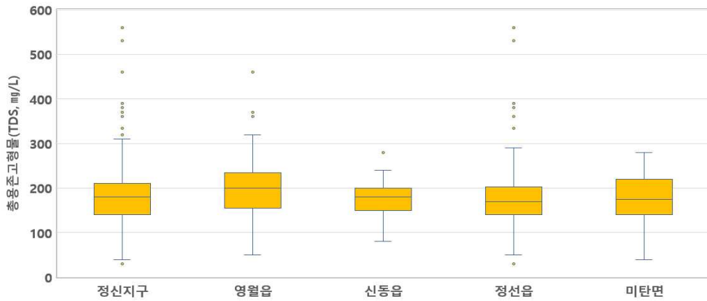
<그림 3-2-16> 지하수 총용존고형물(TDS, mg/L) Box-whisker
