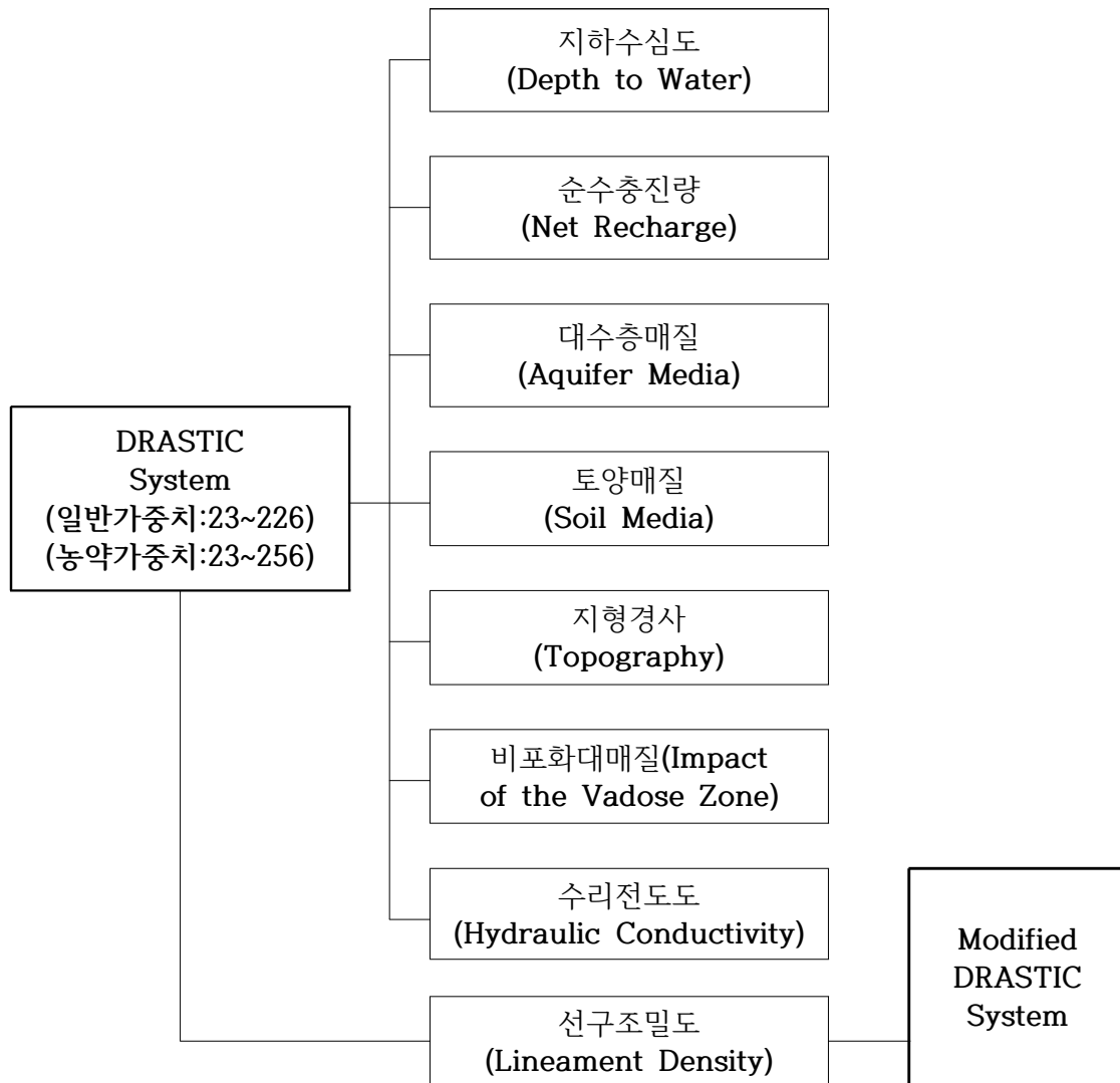
<그림 3-2-1> DRASTIC 흐름도
