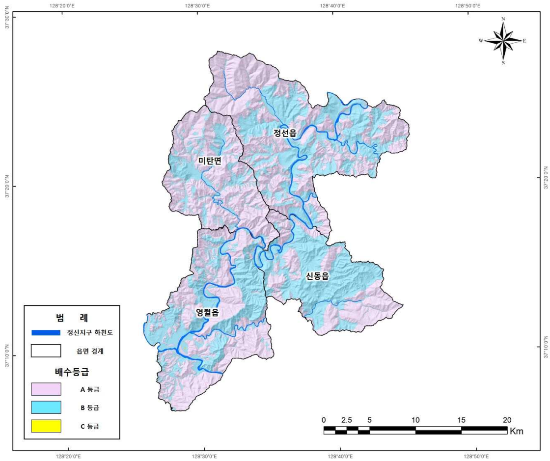
<그림 1-4-6> 정선지구 NRCS 토양도
