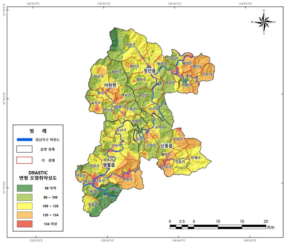
<그림 3-3-11> 변형오염취약성도(Modified DRASTIC INDEX Map)
