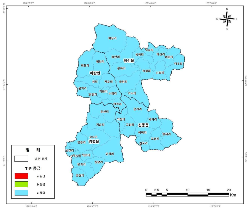
<그림 3-2-6> T-P 발생부하량 등급도
