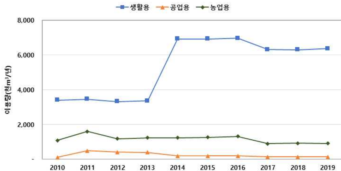
<그림 3-1-4> 정신지구 용도별 관정수 및 이용량 추이
