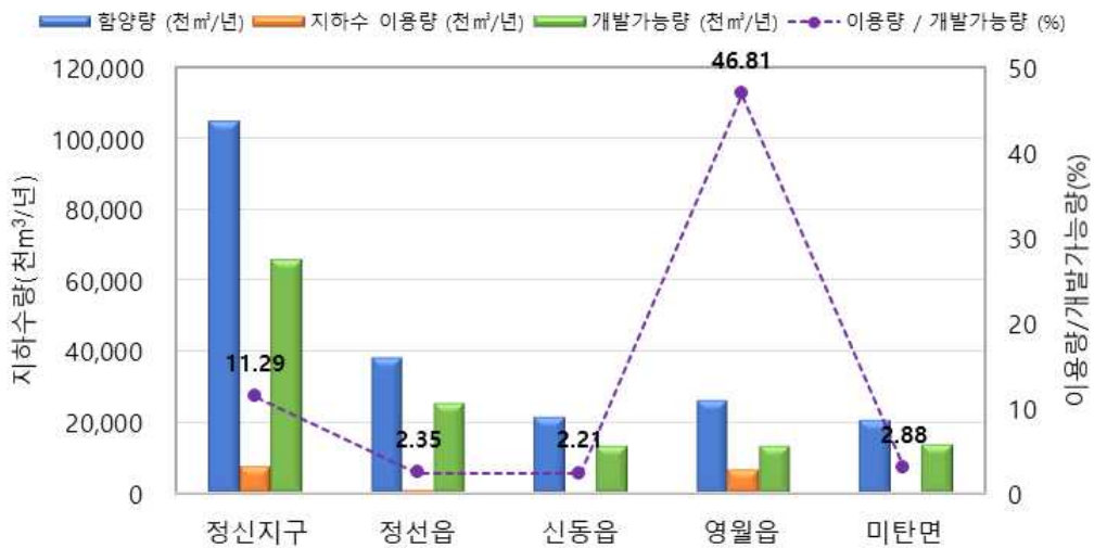
<그림 3-1-12> 읍면별 지하수 이용량 및 개발가능량
