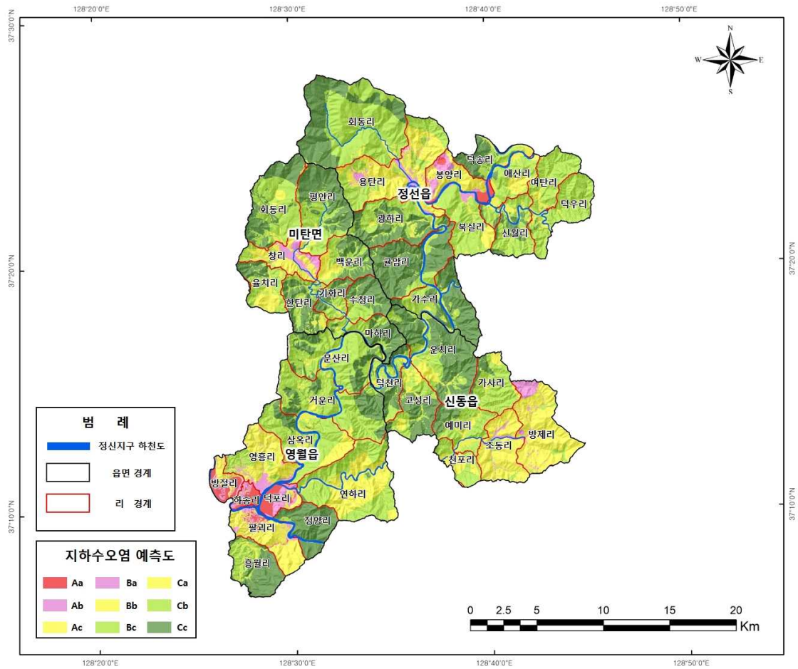
<그림 3-2-9> 정신지구 지하수오염예측도
