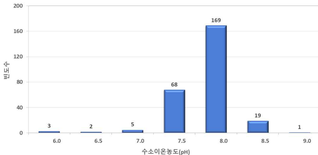
<그림 3-2-9> 정선지구 지하수 pH 빈도분포도
