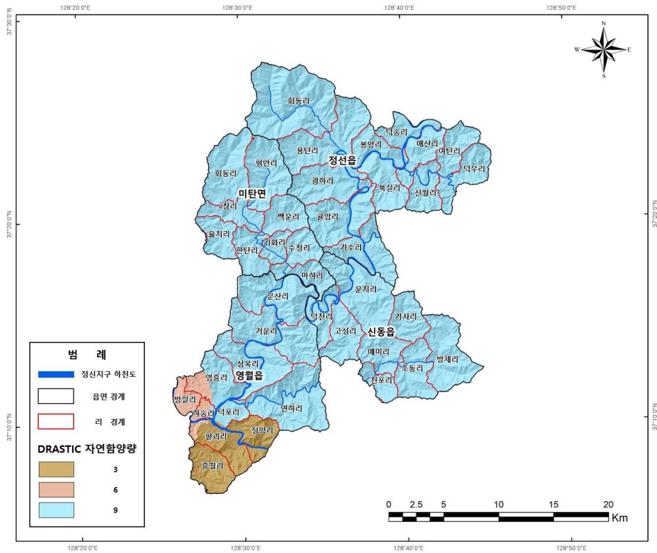
<그림 3-3-3> 자연함양량
