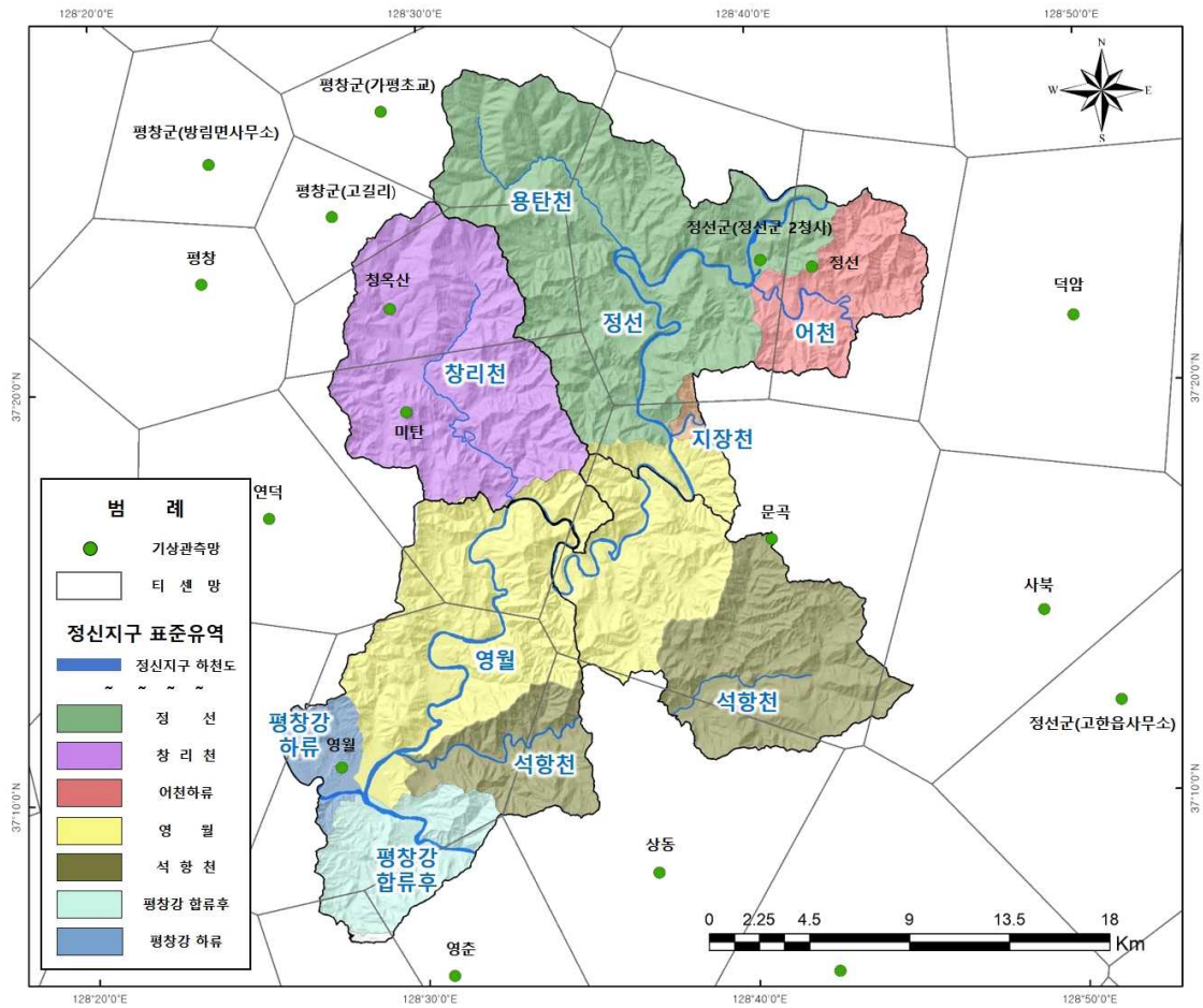
<그림 3-1-8> 조사지역 Thiessen망도
