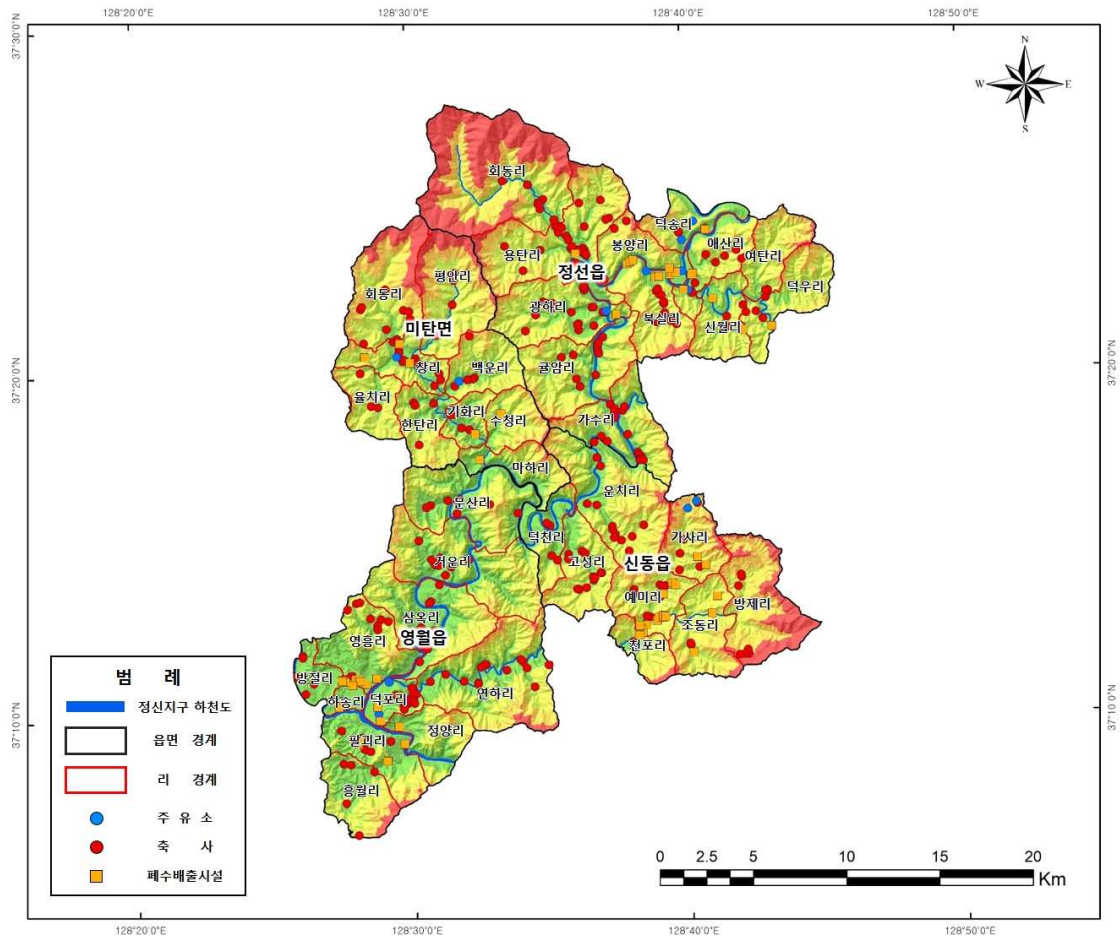
<그림 1-4-2> 정신지구 점오염원 위치도
