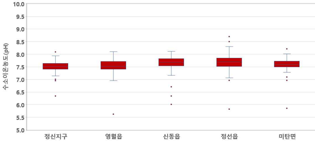
<그림 3-2-10> 정선지구 지하수 pH Box-whisker
