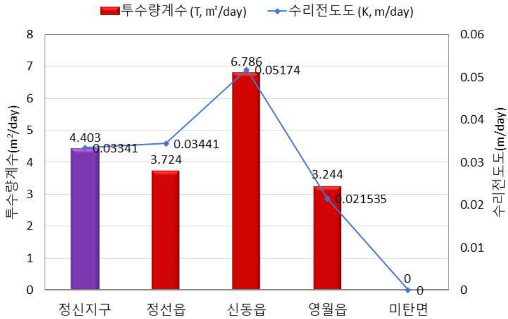
<그림 3-1-3> 읍면별 지하수 투수량계수 및 수리전도도(산술평균)
