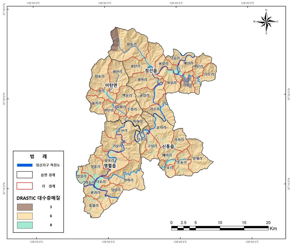
<그림 3-3-4> 대수층 매질
