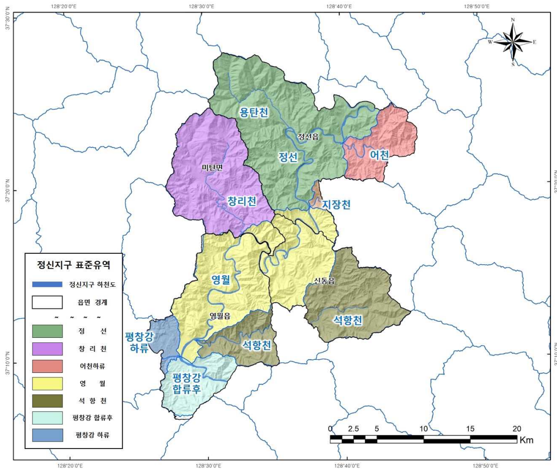
<그림 1-4-2> 정신지구 표준유역 현황
