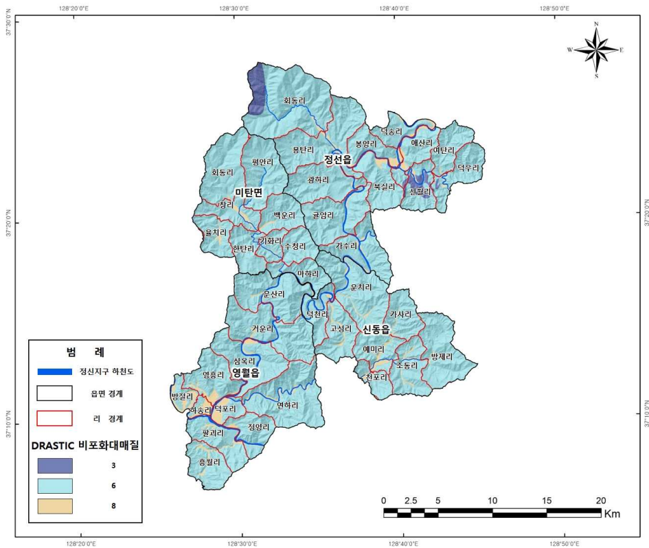
<그림 3-3-7> 비포화대 매질
