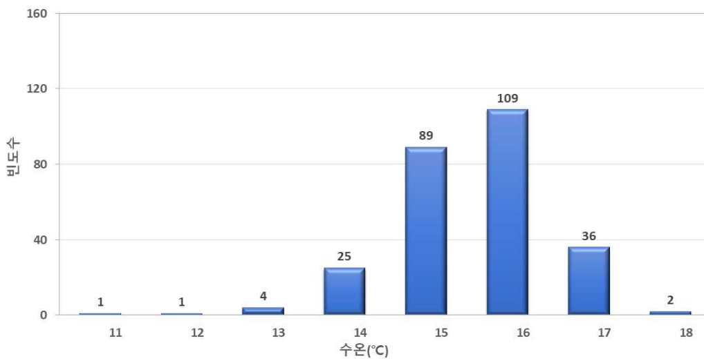
<그림 3-2-6> 정신지구 지하수의 수온(T) 빈도분포도
