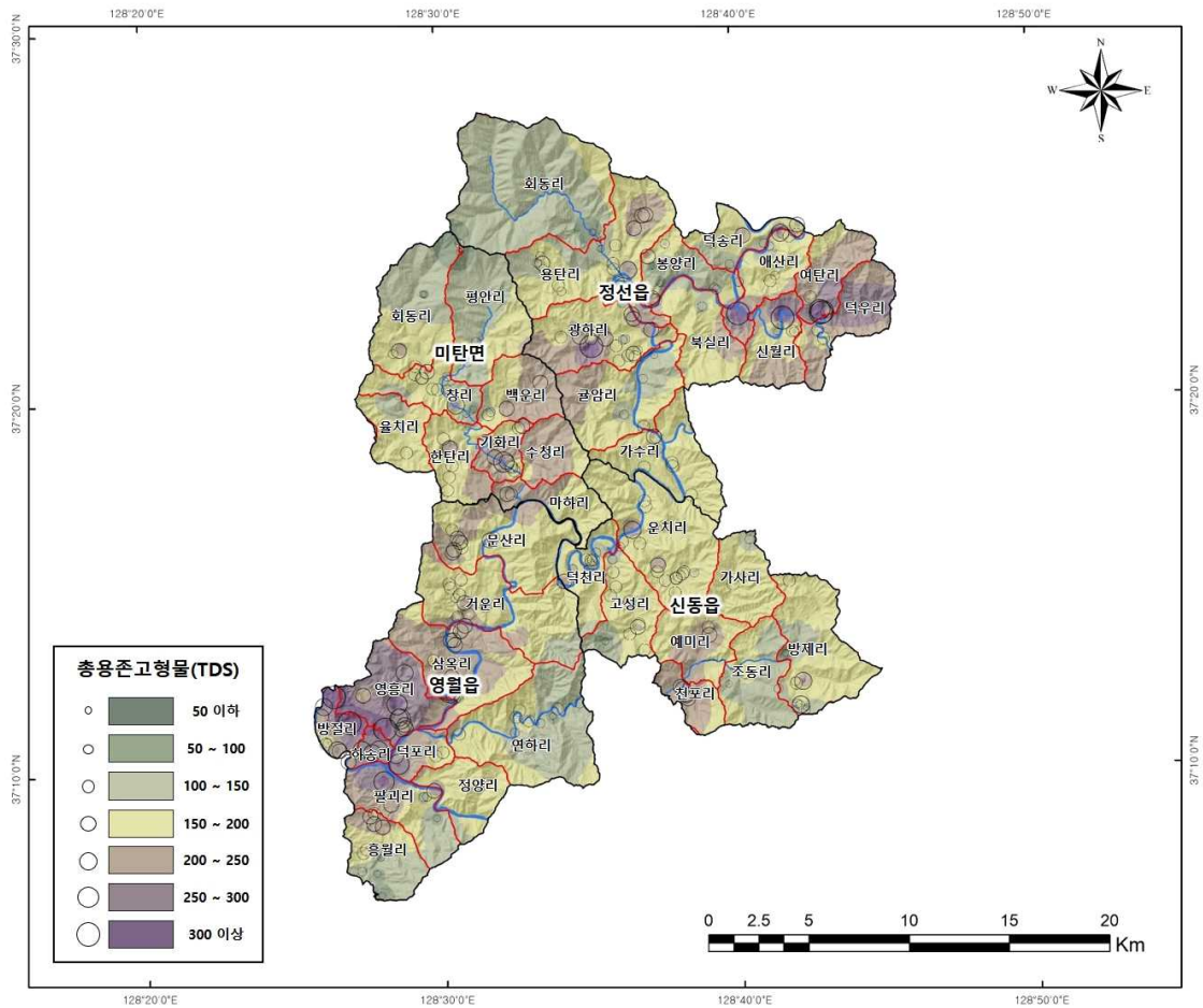
<그림 3-2-17> 지하수 총용존고형물(TDS, mg/L) 분포도
