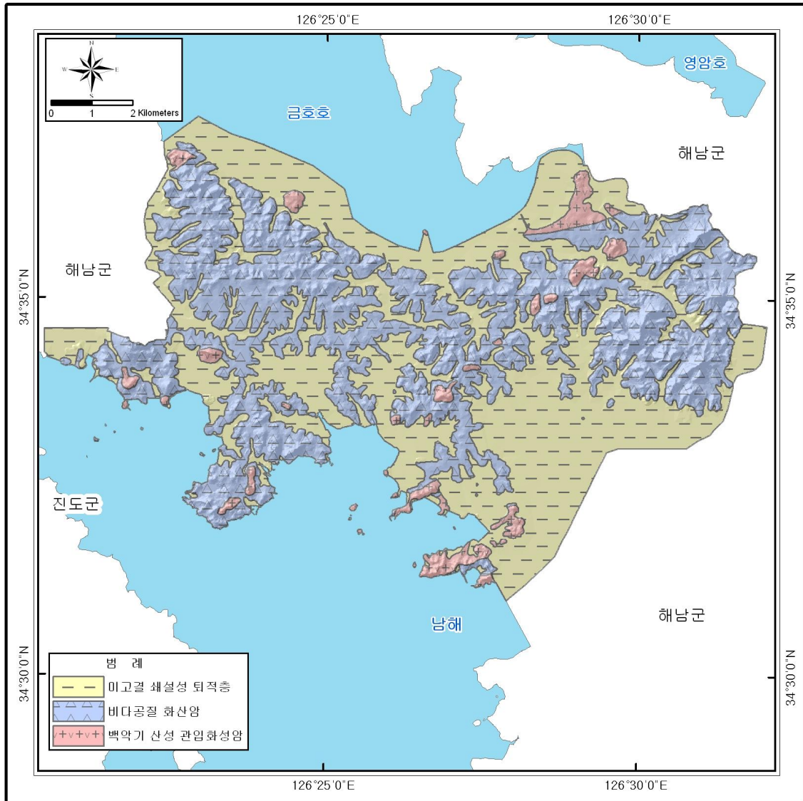
<그림 1-4-5> 해황지구 수문지질도
