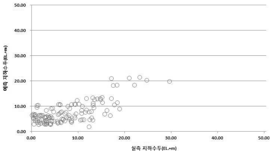
<그림 3-1-2> 실측 지하수두와 예측 지하수두
