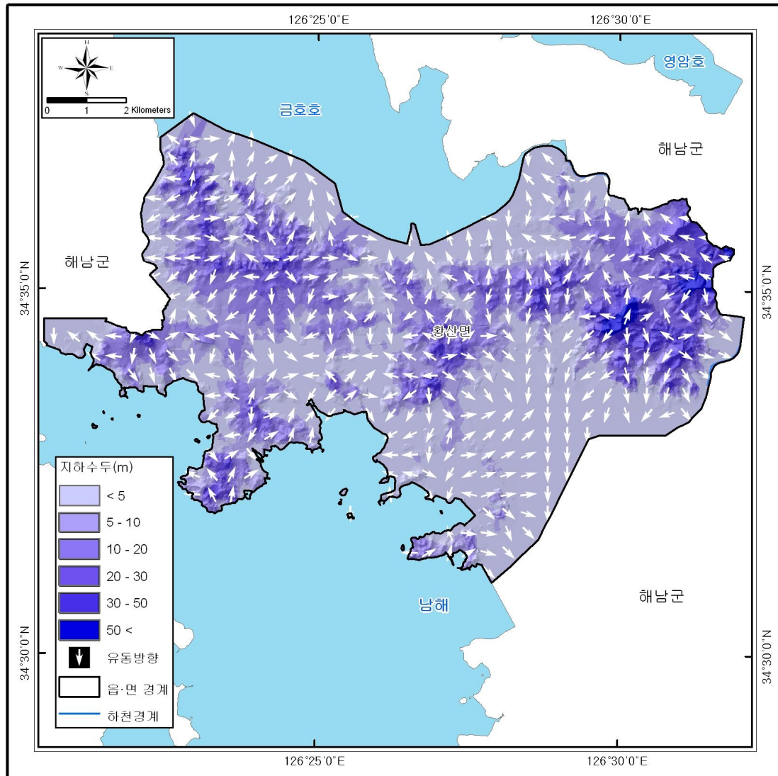
<그림 3-1-3> 지하수두 및 유동방향도
