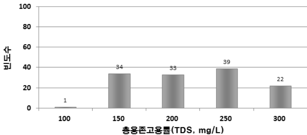
<그림 3-2-15> 해황지구 지하수의 총용존고형물(TDS, mg/L) 빈도분포도
