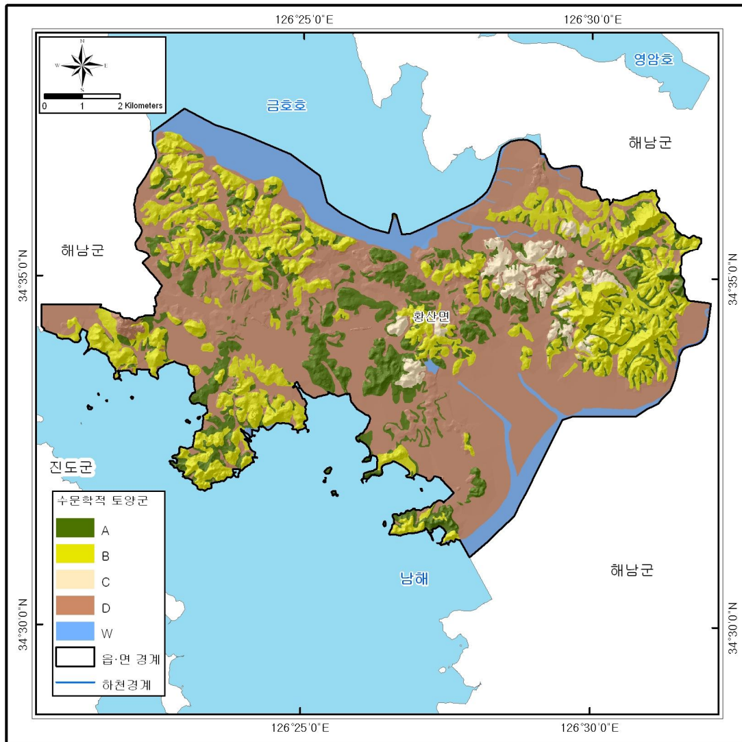
<그림 1-4-7> 해황지구 NRCS 토양도
