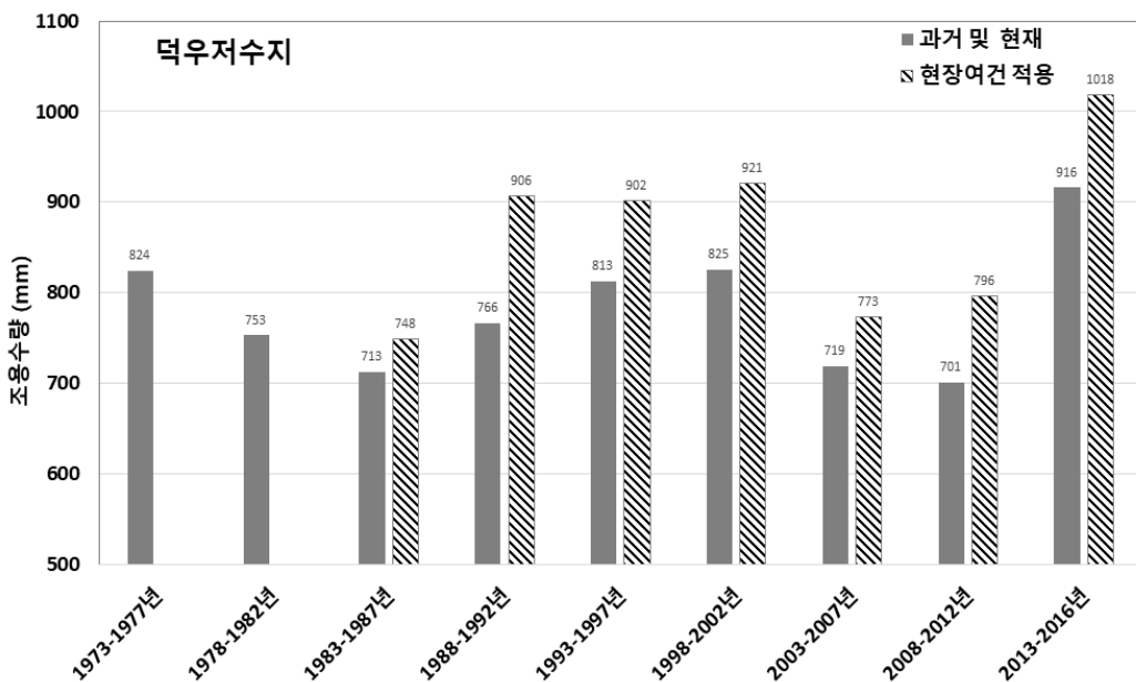
[그림 5.67] 덕우저수지 5년 단위 시나리오별 연평균 조용수량 분석
