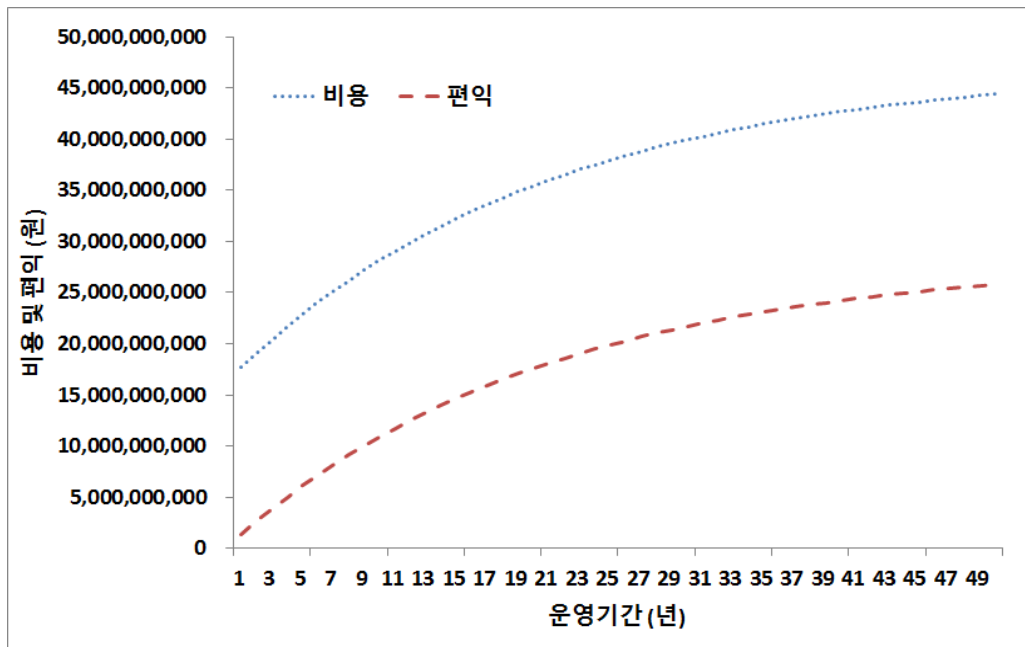
[그림 6.11] 냉정저수지 경제성 분석 결과
