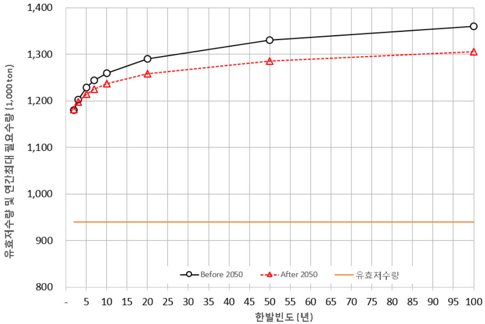
[그림 5.99] 냉정저수지 미래 이수안전도 분석
