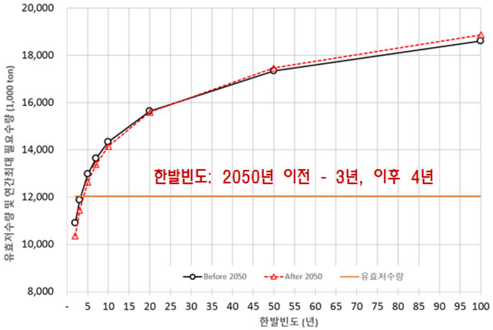
[그림 5.94] 금광저수지 미래 이수안전도 분석
