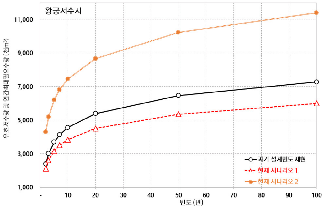
[그림 5.87] 왕궁저수지 이수안전도 분석
