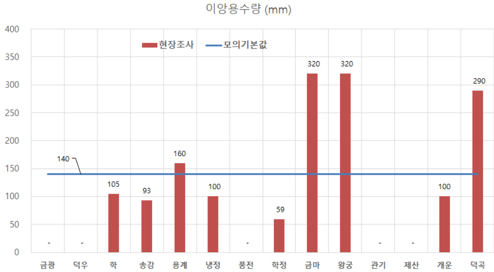
[그림 4.5] 시험지구 이앙용수량 조사
