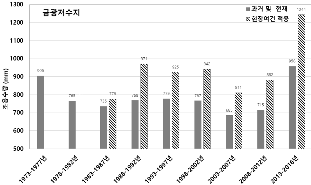
[그림 5.66] 금광저수지 5년 단위 시나리오별 연평균 조용수량 분석
