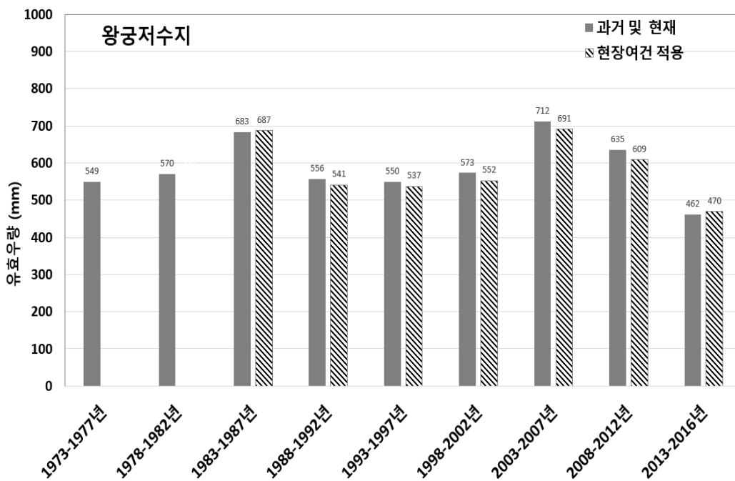
[그림 5.48] 왕궁저수지 5년 단위 시나리오별 연평균 유효수량 분석
