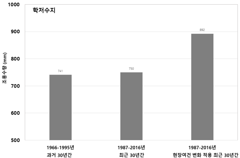
[그림 5.55] 학저수지 30년 단위 시나리오별 연평균 조용수량 비교
