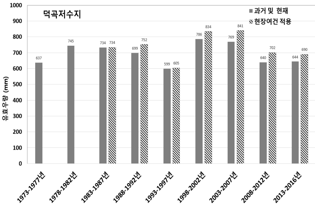
[그림 5.52] 덕곡저수지 5년 단위 시나리오별 연평균 유효우량 분석
