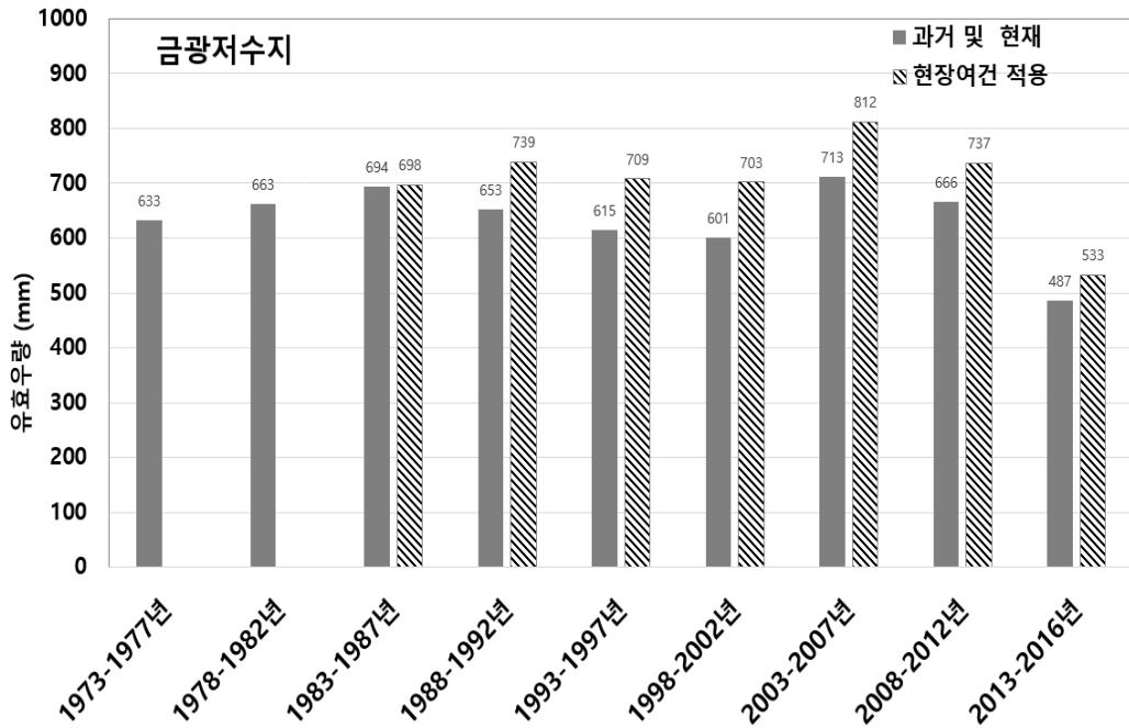
[그림 5.40] 금광저수지 5년 단위 시나리오별 연평균 유효우량 분석
