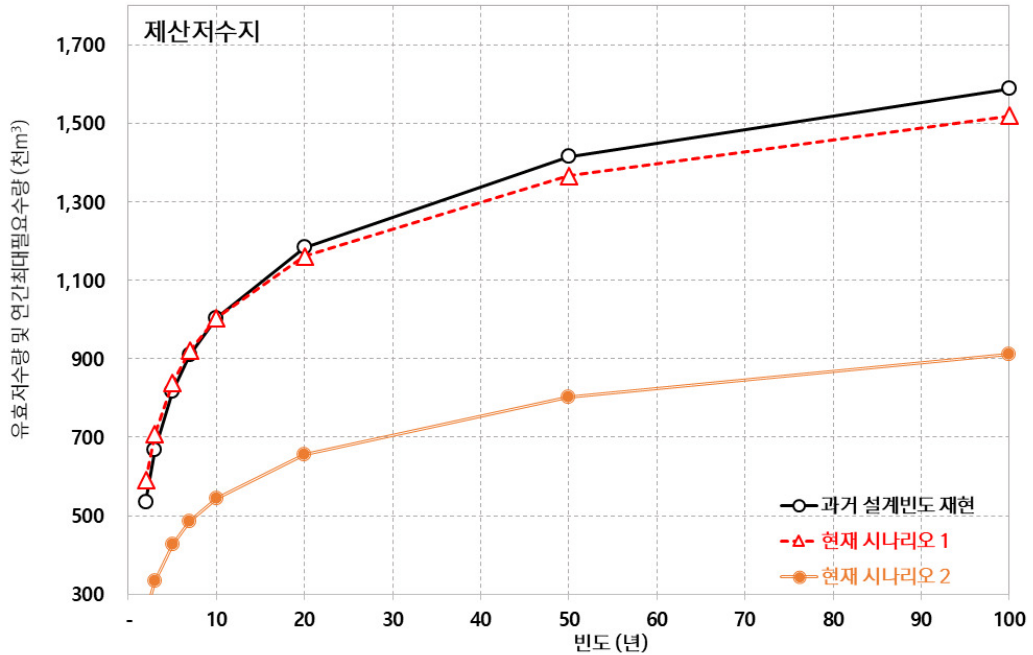
[그림 5.89] 제산저수지 이수안전도 분석
