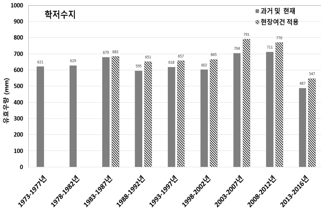
[그림 5.42] 학저수지 5년 단위 시나리오별 연평균 유효우량 분석
