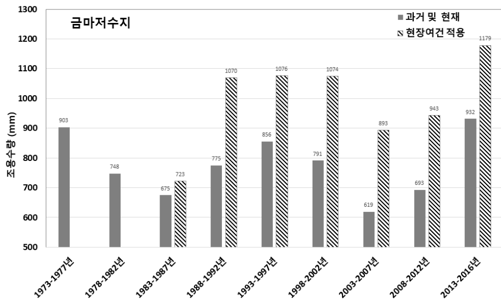
[그림 5.73] 금마저수지 5년 단위 시나리오별 연평균 조용수량 분석
