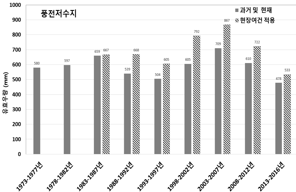
[그림 5.46] 풍전저수지 5년 단위 시나리오별 연평균 유효수량 분석
