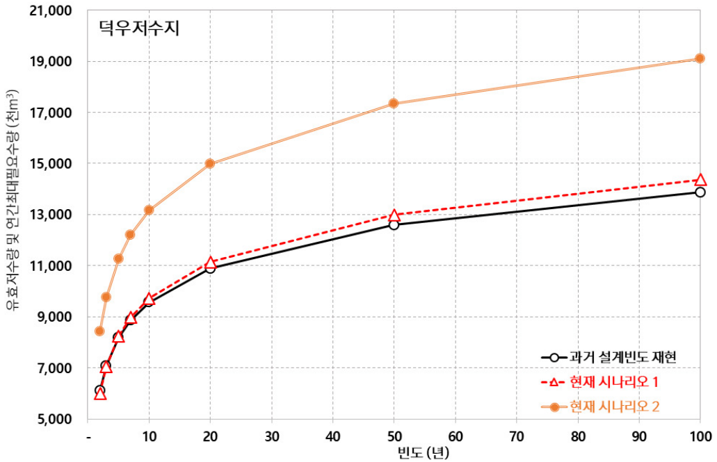
[그림 5.80] 덕우저수지 이수안전도 분석
