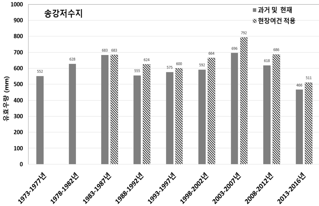
[그림 5.43] 송강저수지 5년 단위 시나리오별 연평균 유효수량 분석
