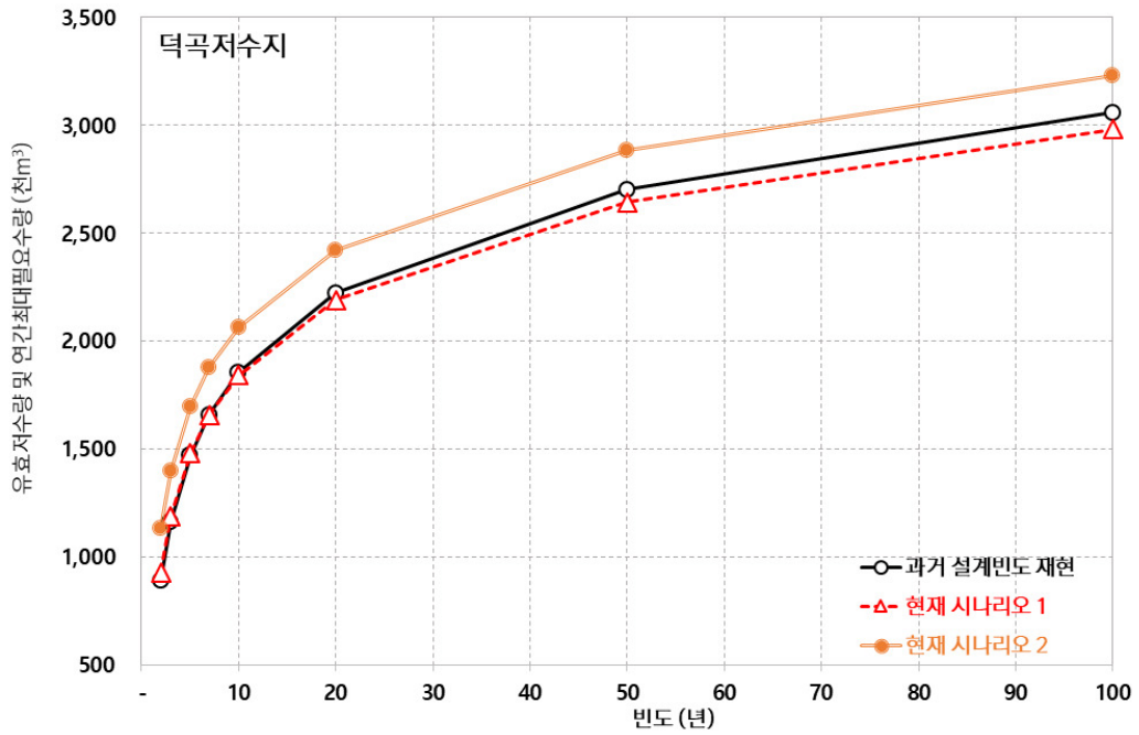
[그림 5.91] 덕곡저수지 이수안전도 분석
