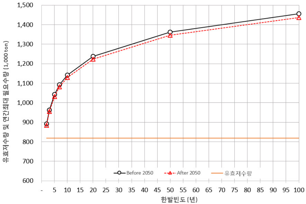
[그림 5.101] 금마저수지 미래 이수안전도 분석
