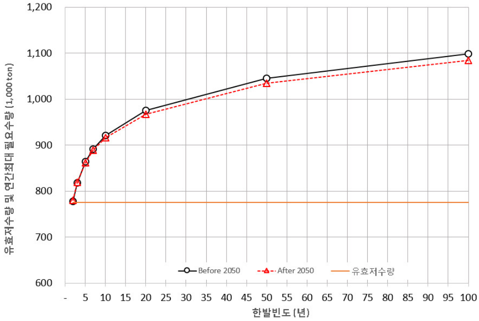
[그림 5.98] 학정저수지 미래 이수안전도 분석
