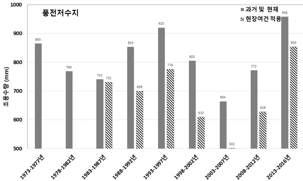
[그림 5.72] 풍전저수지 5년 단위 시나리오별 연평균 조용수량 분석
