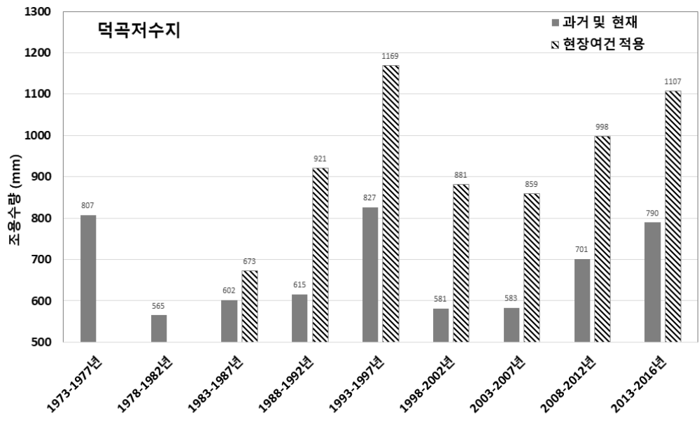
[그림 5.78] 덕곡저수지 5년 단위 시나리오별 연평균 조용수량 분석
