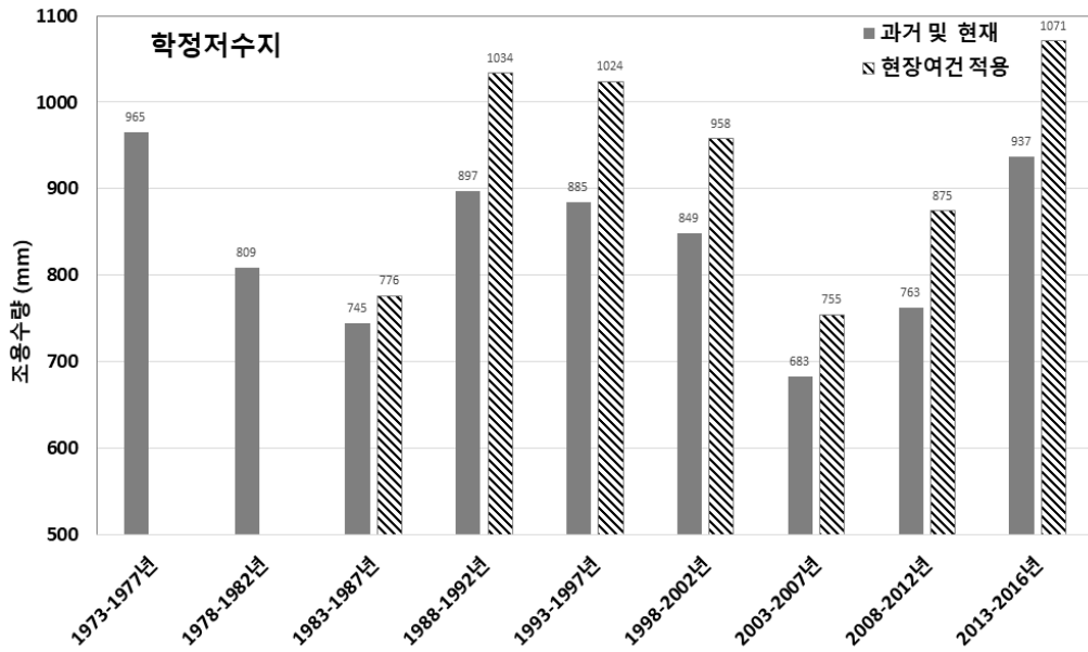
[그림 5.70] 학정저수지 5년 단위 시나리오별 연평균 조용수량 분석
