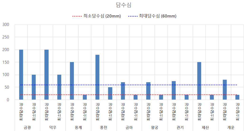
[그림 4.8] 시험지구 담수심 조사
