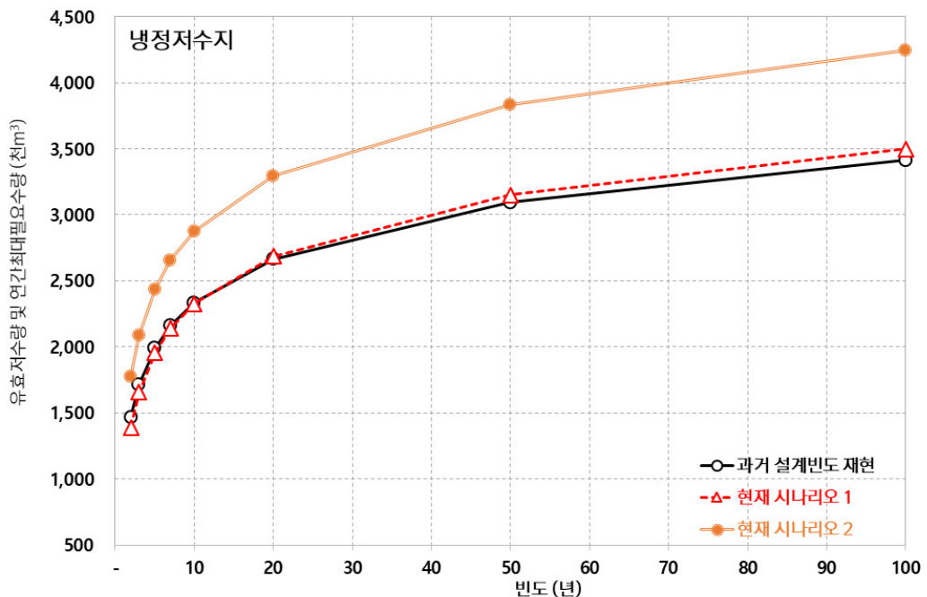
[그림 5.84] 냉정저수지 이수안전도 분석
