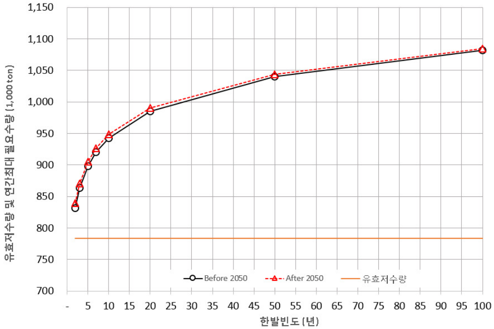
[그림 5.103] 관기저수지 미래 이수안전도 분석
