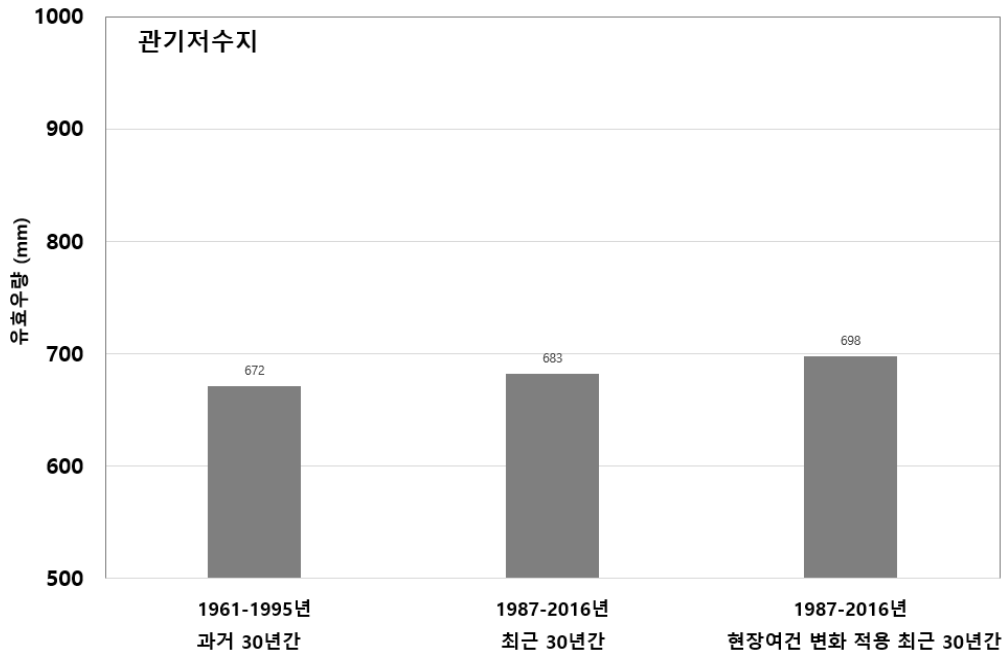
[그림 5.36] 관기저수지 30년 단위 시나리오별 연평균 유효우량 비교
