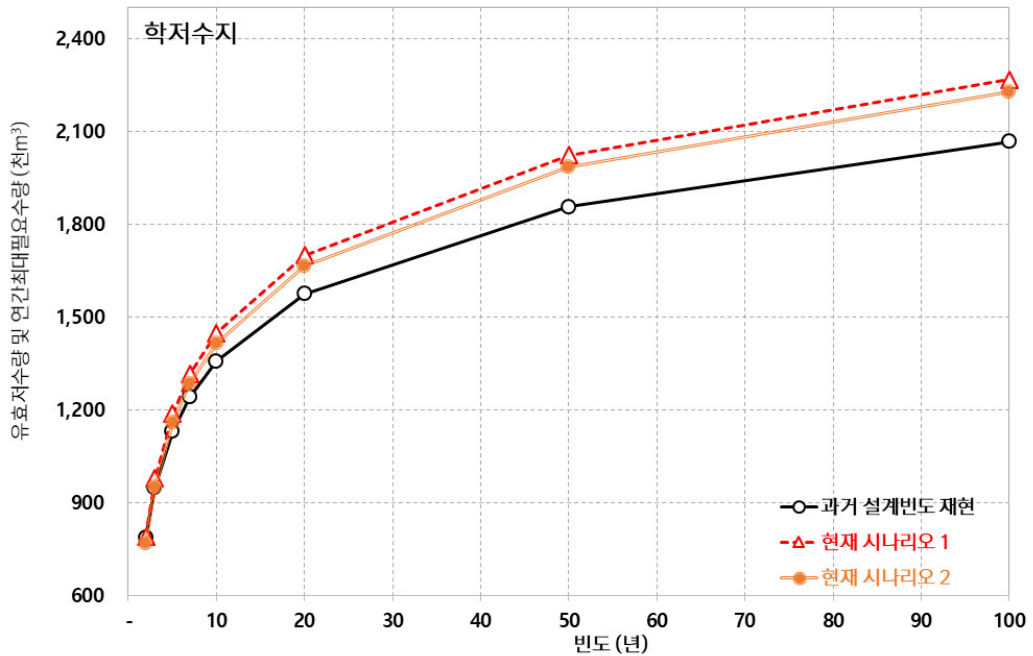
[그림 5.81] 학저수지 이수안전도 분석
