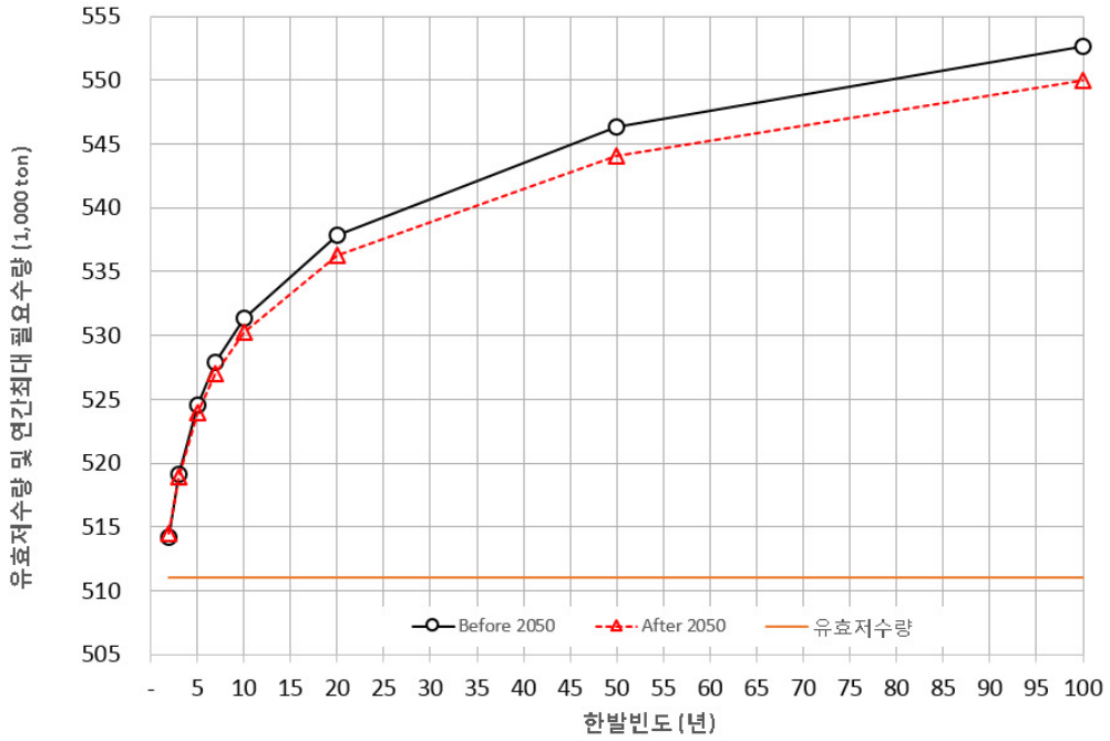
[그림 5.104] 제산저수지 미래 이수안전도 분석
