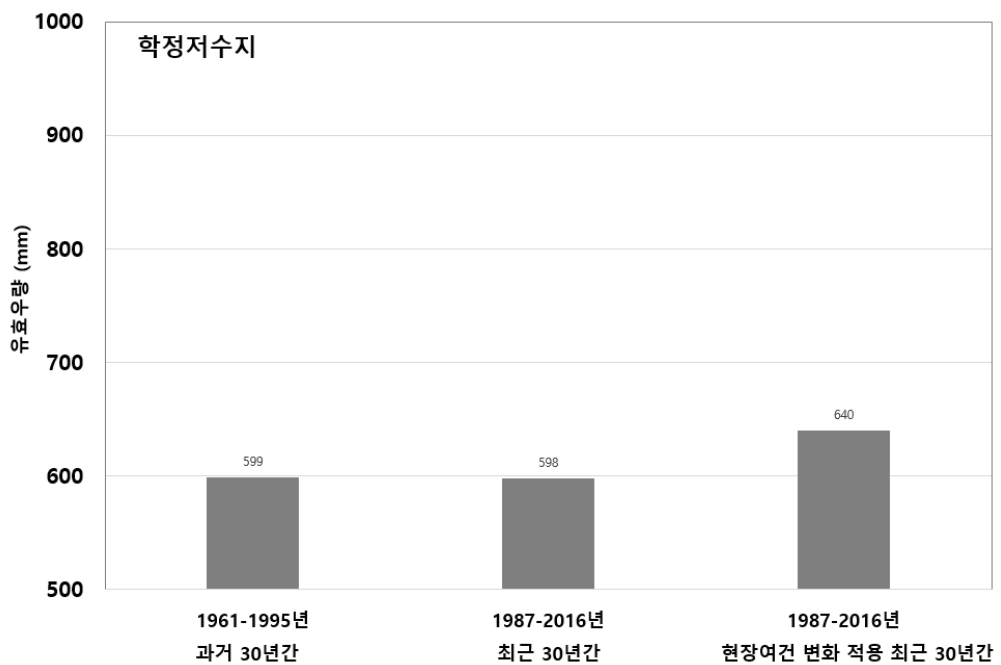
[그림 5.31] 학정저수지 30년 단위 시나리오별 연평균 유효우량 비교
