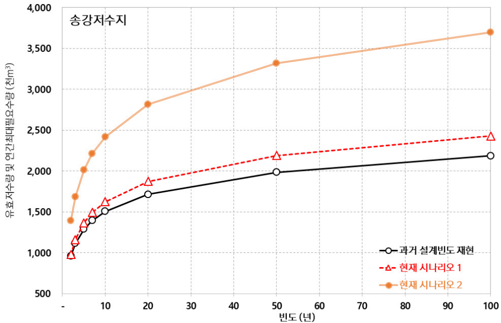
[그림 5.82] 송강저수지 이수안전도 분석
