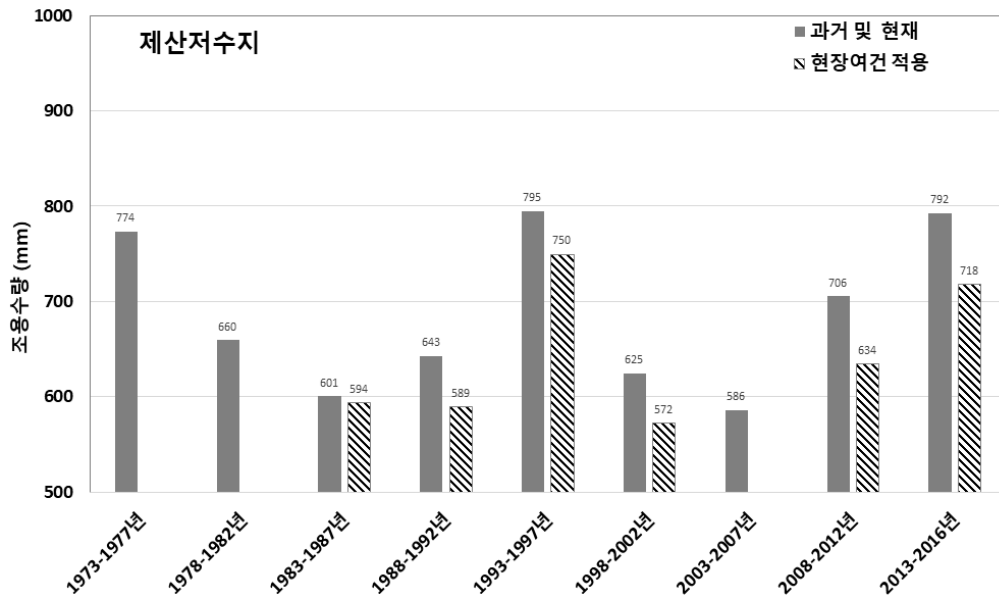
[그림 5.76] 제산저수지 5년 단위 시나리오별 연평균 조용수량 분석
