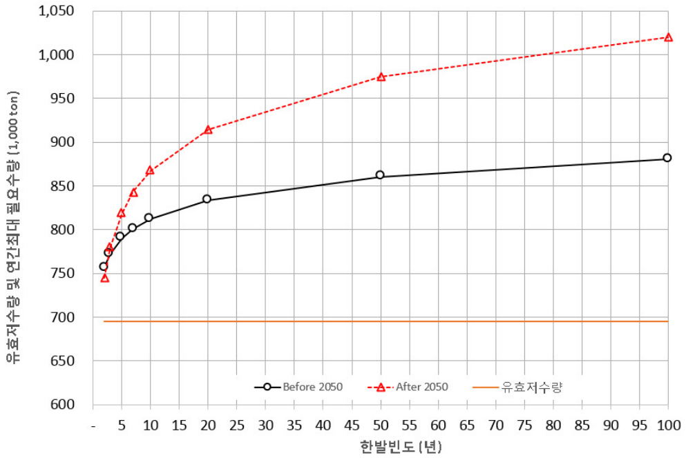
[그림 5.106] 덕곡저수지 미래 이수안전도 분석
