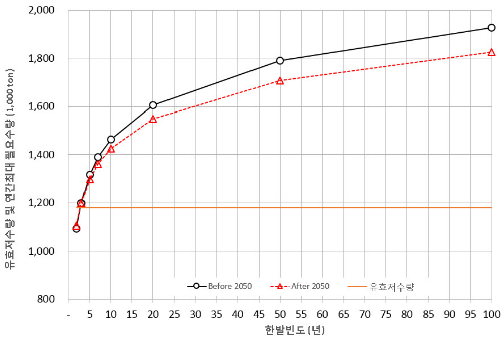
[그림 5.105] 개운저수지 미래 이수안전도 분석
