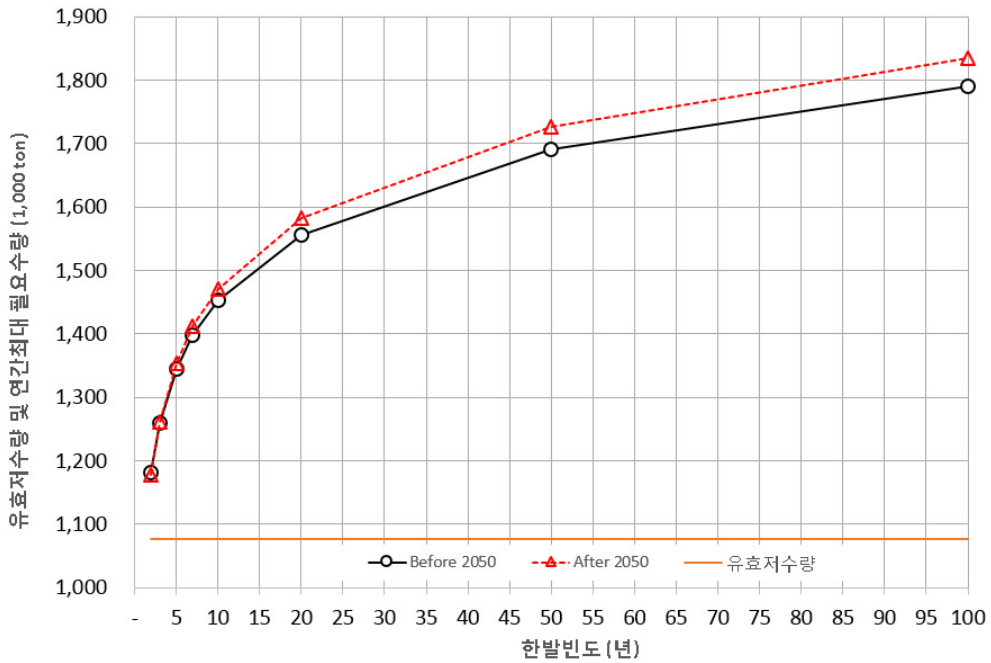
[그림 5.97] 송강저수지 미래 이수안전도 분석
