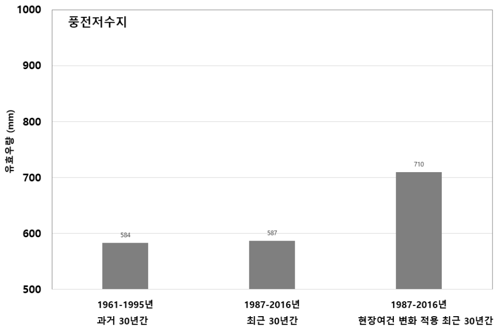
[그림 5.33] 풍전저수지 30년 단위 시나리오별 연평균 유효우량 비교
