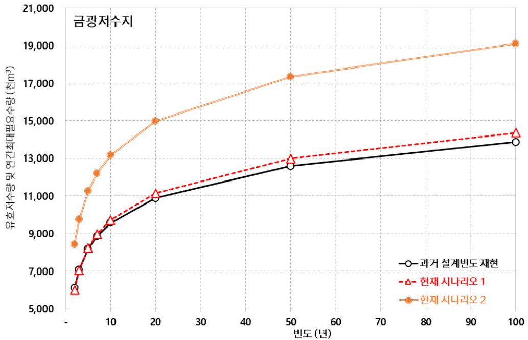
[그림 5.79] 금광저수지 이수안전도 분석
