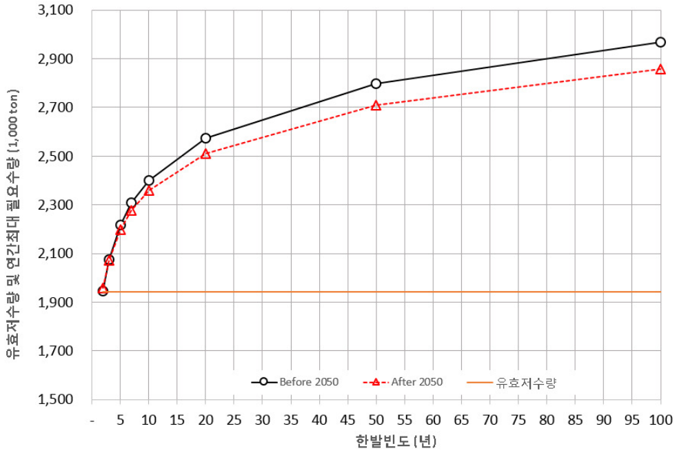
[그림 5.102] 왕궁저수지 미래 이수안전도 분석
