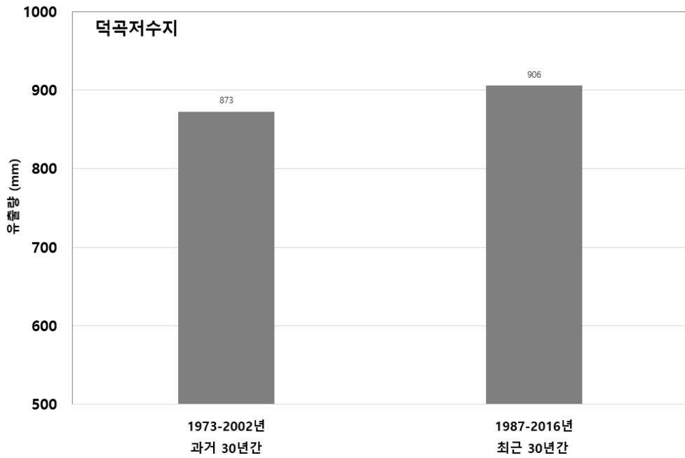
[그림 5.13] 덕곡저수지 30년 단위 연평균 유출량 비교
