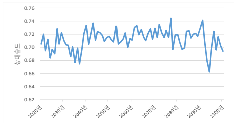
[RCP 4.5 상대습도]
