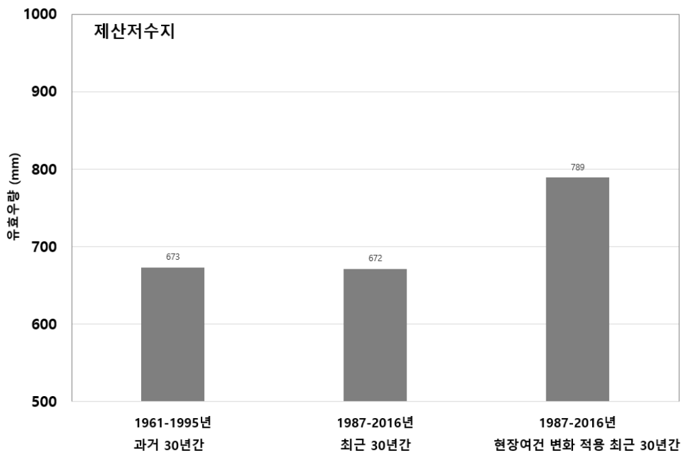
[그림 5.37] 제산저수지 30년 단위 시나리오별 연평균 유효우량 비교
