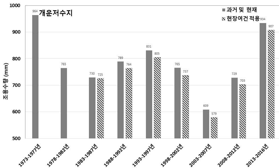
[그림 5.77] 개운저수지 5년 단위 시나리오별 연평균 조용수량 분석
