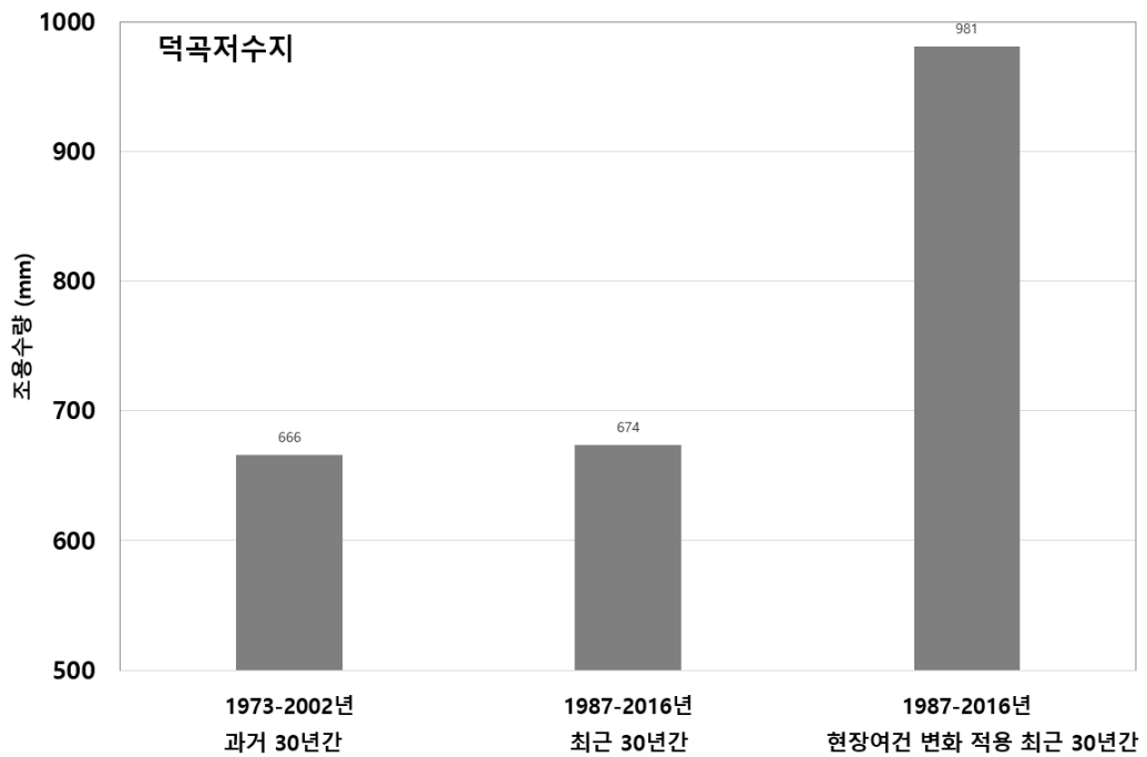
[그림 5.65] 덕곡저수지 30년 단위 시나리오별 연평균 조용수량 비교
