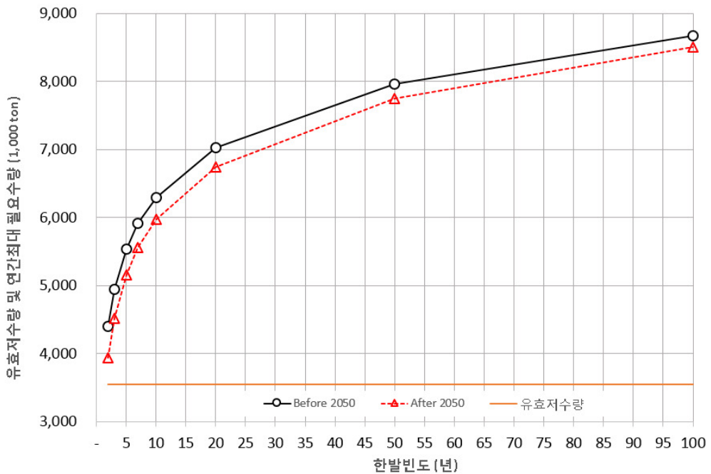
[그림 5.95] 덕우저수지 미래 이수안전도 분석
