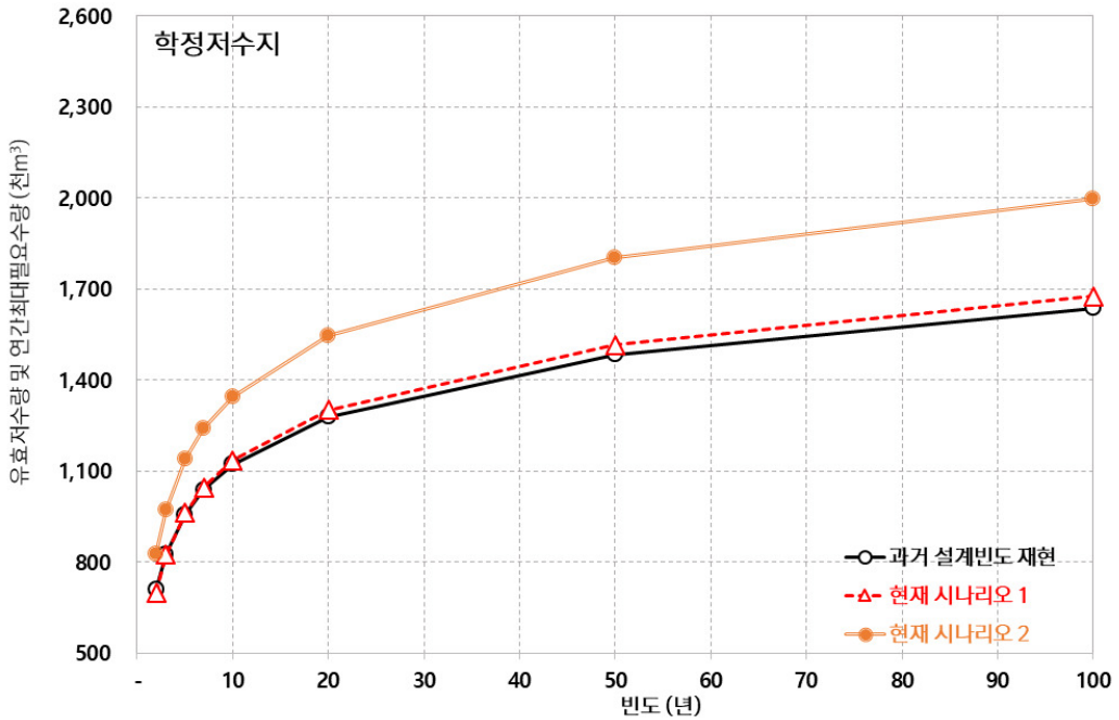
[그림 5.83] 학정저수지 이수안전도 분석
