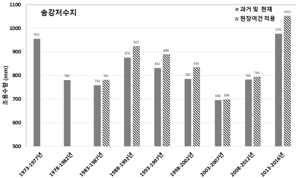
[그림 5.69] 송강저수지 5년 단위 시나리오별 연평균 조용수량 분석
