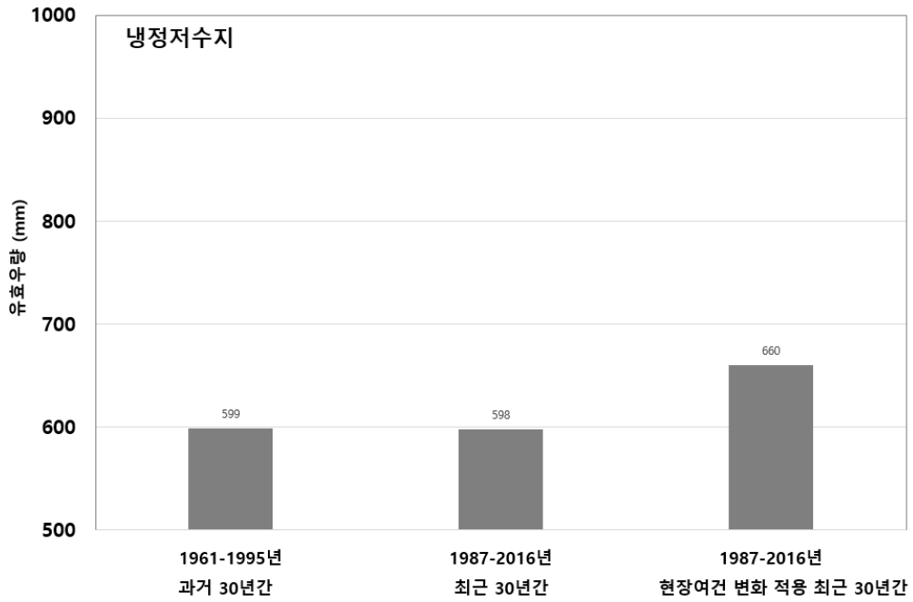
[그림 5.32] 냉정저수지 30년 단위 시나리오별 연평균 유효우량 비교
