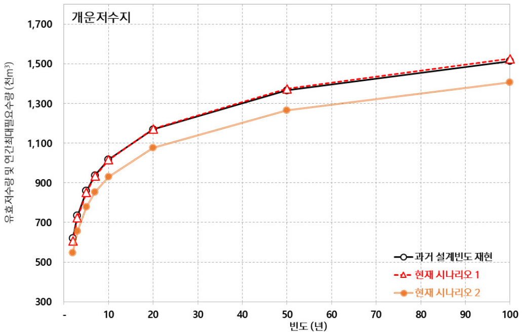
[그림 5.90] 개운저수지 이수안전도 분석
