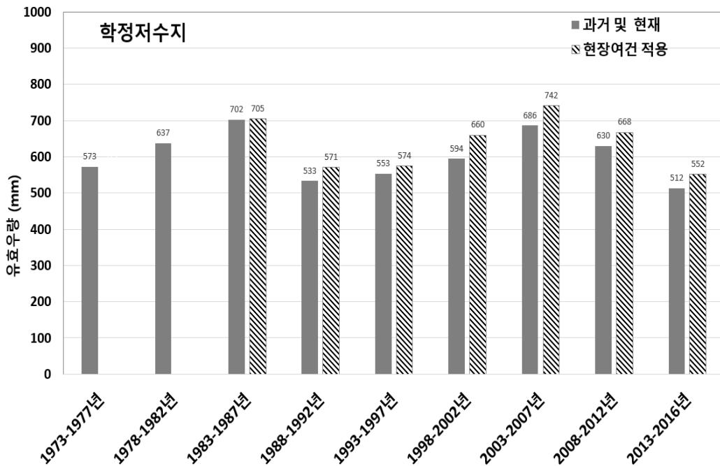
[그림 5.44] 학정저수지 5년 단위 시나리오별 연평균 유효수량 분석
