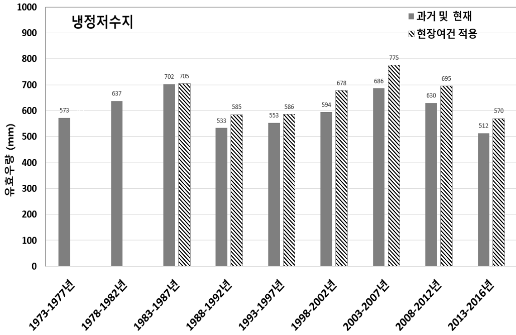
[그림 5.45] 냉정저수지 5년 단위 시나리오별 연평균 유효수량 분석
