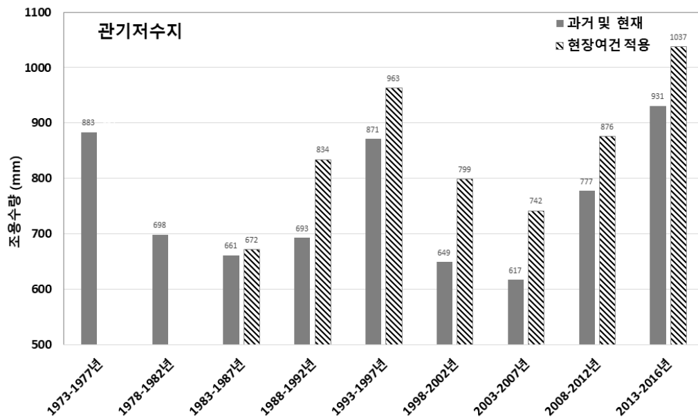
[그림 5.75] 관기저수지 5년 단위 시나리오별 연평균 조용수량 분석
