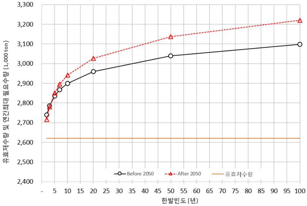
[그림 5.100] 풍전저수지 미래 이수안전도 분석
