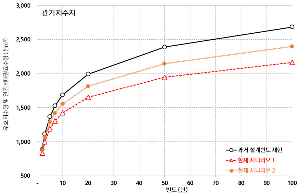
[그림 5.88] 관기저수지 이수안전도 분석
