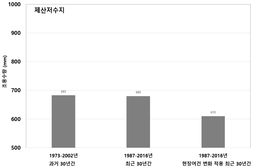
[그림 5.63] 제산저수지 30년 단위 시나리오별 연평균 조용수량 비교
