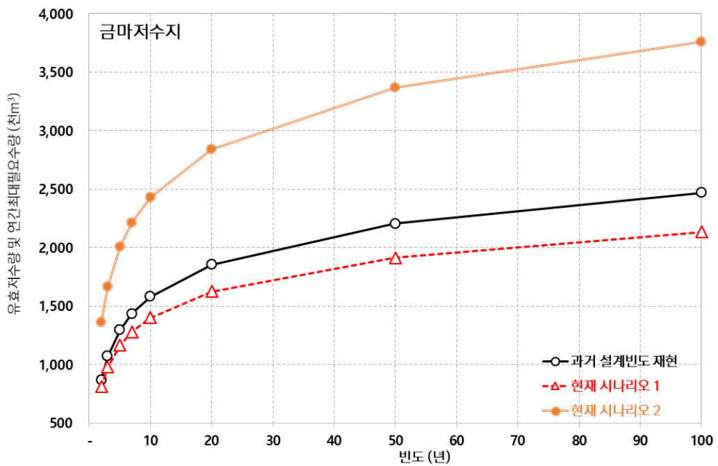
[그림 5.86] 금마저수지 이수안전도 분석
