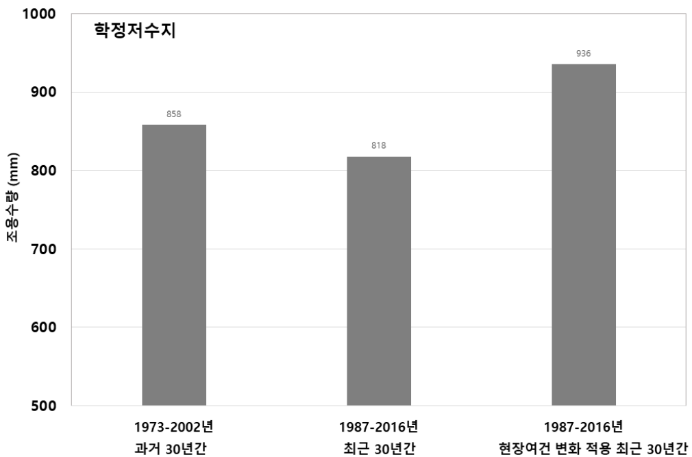
[그림 5.57] 학정저수지 30년 단위 시나리오별 연평균 조용수량 비교
