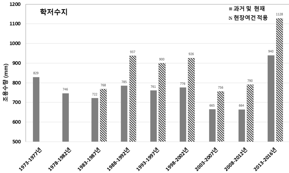
[그림 5.68] 학저수지 5년 단위 시나리오별 연평균 조용수량 분석
