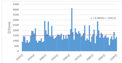
[RCP 4.5 강우량]
