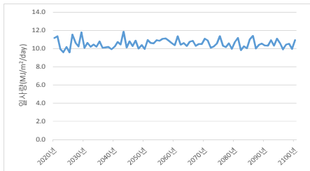
[RCP 4.5 일사량]
