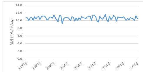
[RCP 8.5 일사량]
