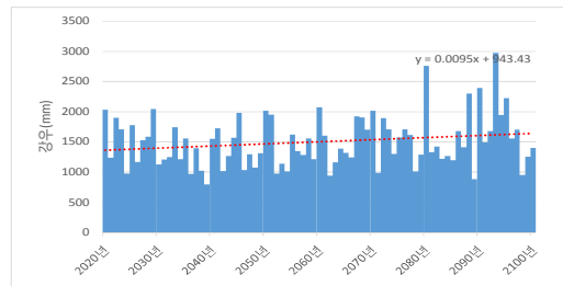
[RCP 8.5 강우량]
