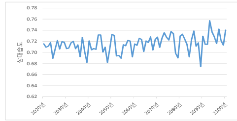
[RCP 8.5 상대습도]
