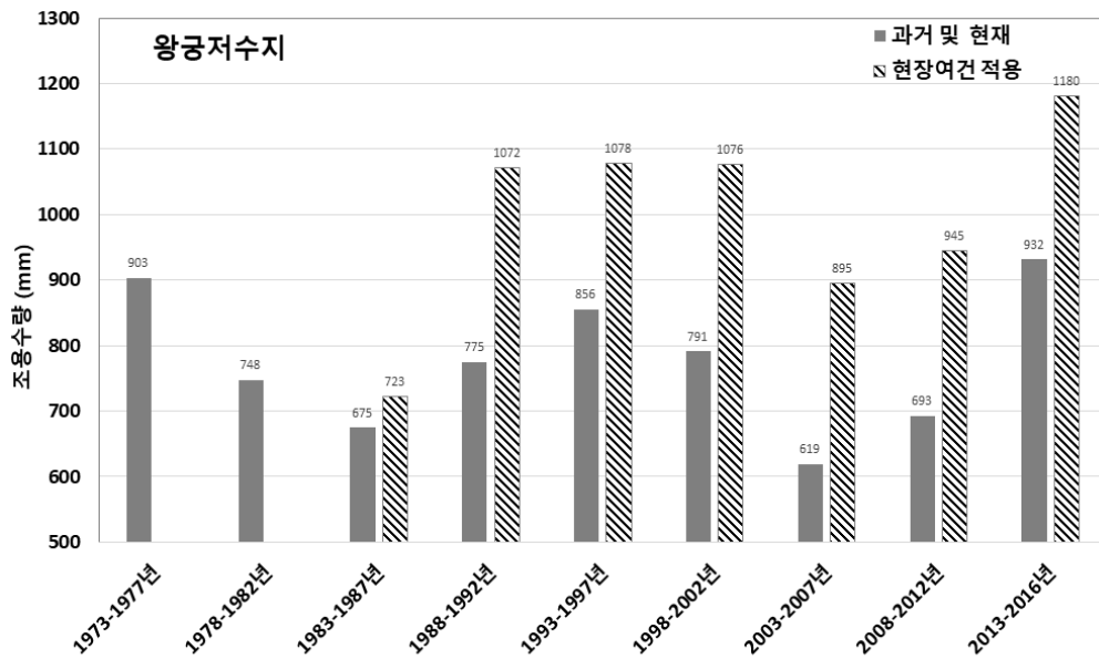
[그림 5.74] 왕궁저수지 5년 단위 시나리오별 연평균 조용수량 분석
