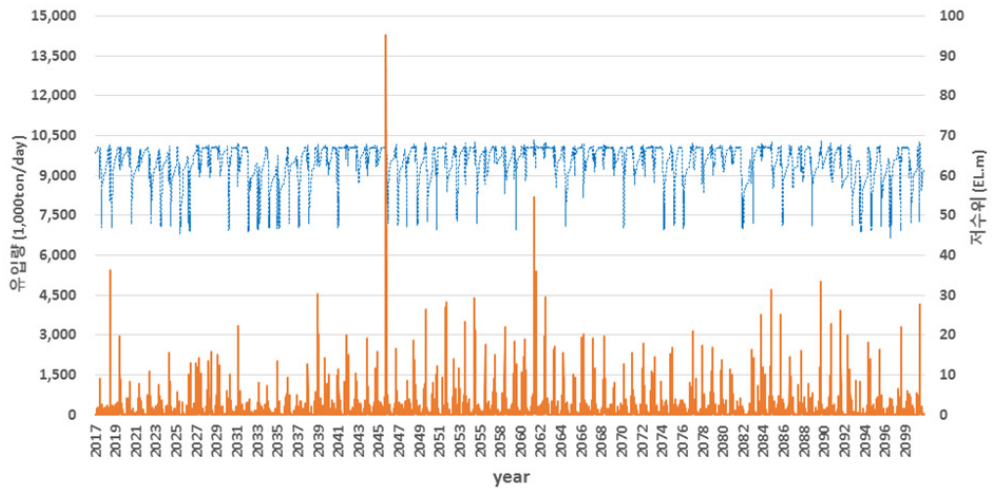
[그림 5.93] 기후변화 시나리오를 이용한 미래 물수지 분석 (금광저수지)
