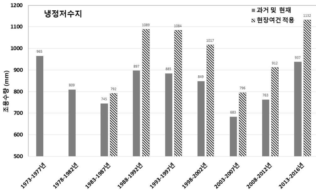
[그림 5.71] 냉정저수지 5년 단위 시나리오별 연평균 조용수량 분석
