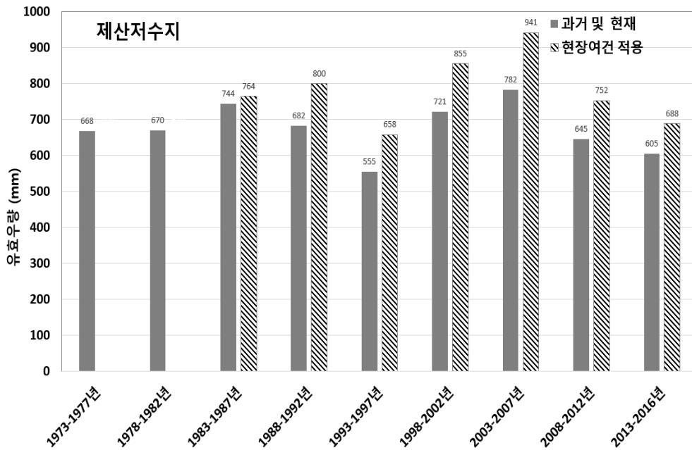
[그림 5.50] 제산저수지 5년 단위 시나리오별 연평균 유효수량 분석
