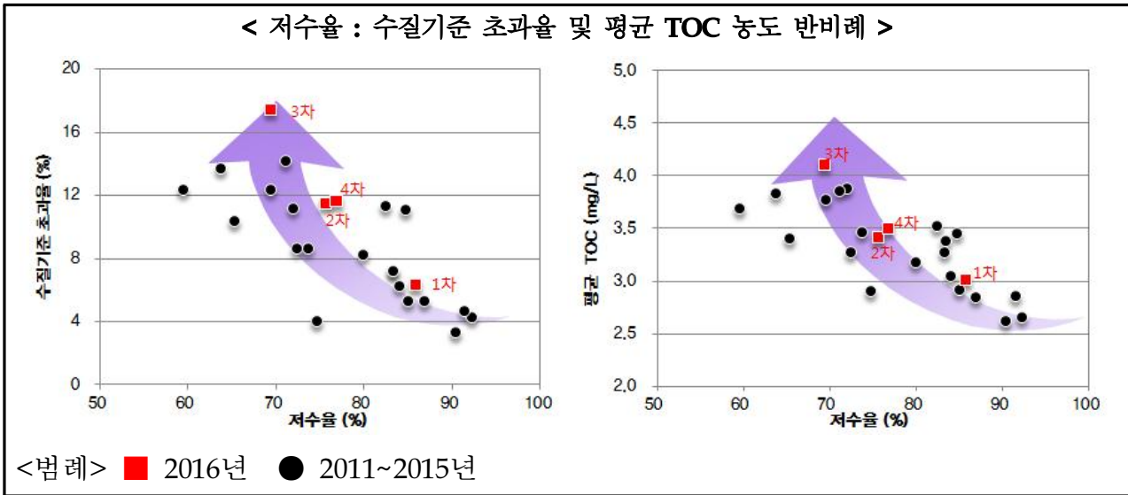
<그림 4.1-10> 조사시기별 호소수질기준 IV등급 초과율, 평균 TOC 농도 및 저수율 관계
