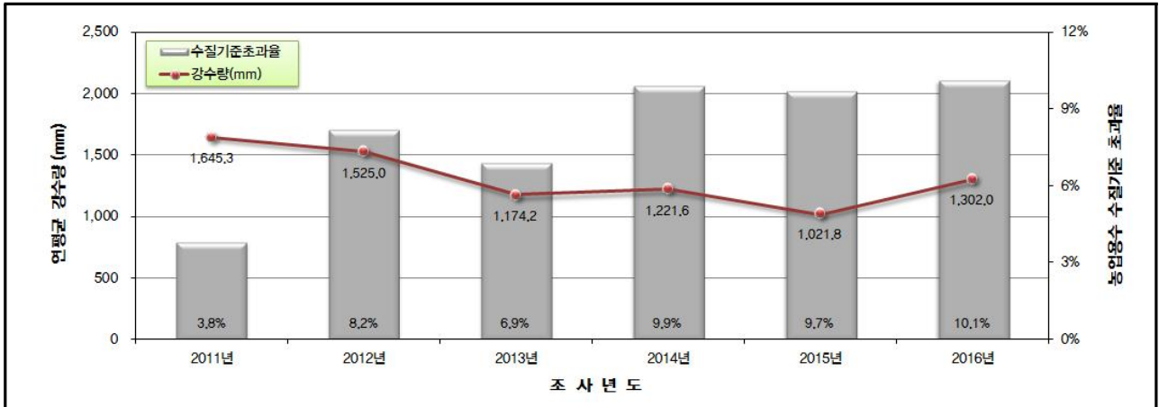
<연도별 호소수질기준 IV등급 초과율 및 연평균 강수량 변화추이>
