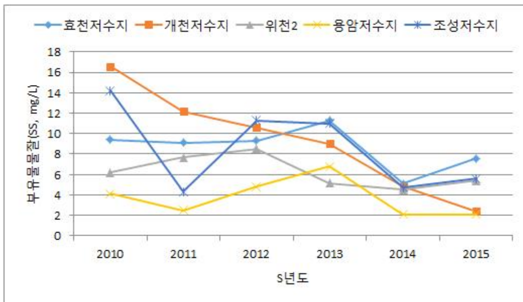
<그림 1-4-5> 연도별 부유물질량(SS) 변화
