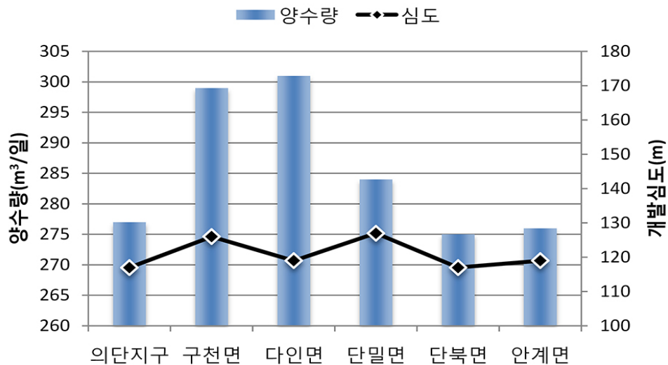
<그림 3-1-2> 읍면별 암반지하수의 평균 양수량 및 개발심도
