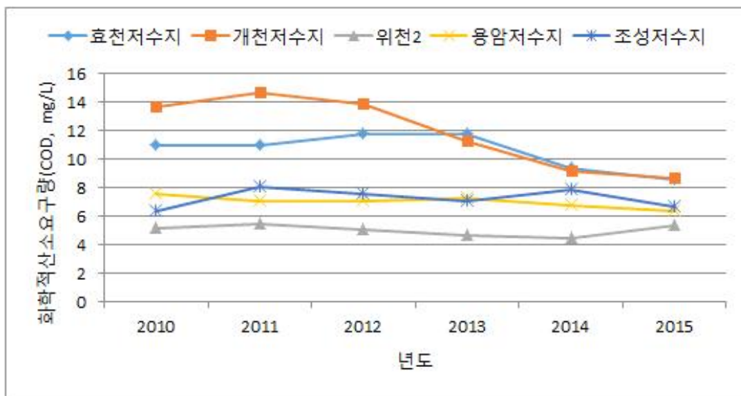
<그림 1-4-3> 연도별 화학적산소요구량(COD) 변화
