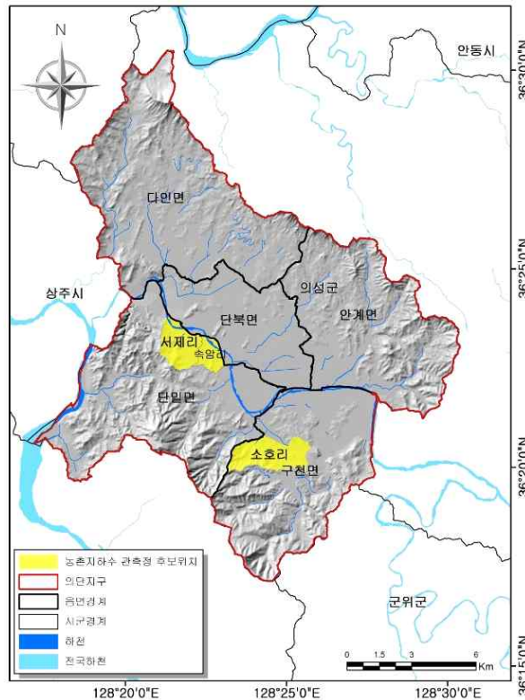
<그림 5-2-2> 농촌지하수 관측정 후보위치도
