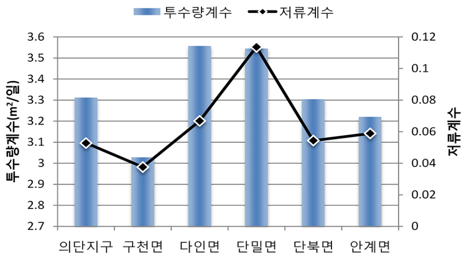
<그림 3-1-3> 읍면별 투수량계수 및 저류계수
