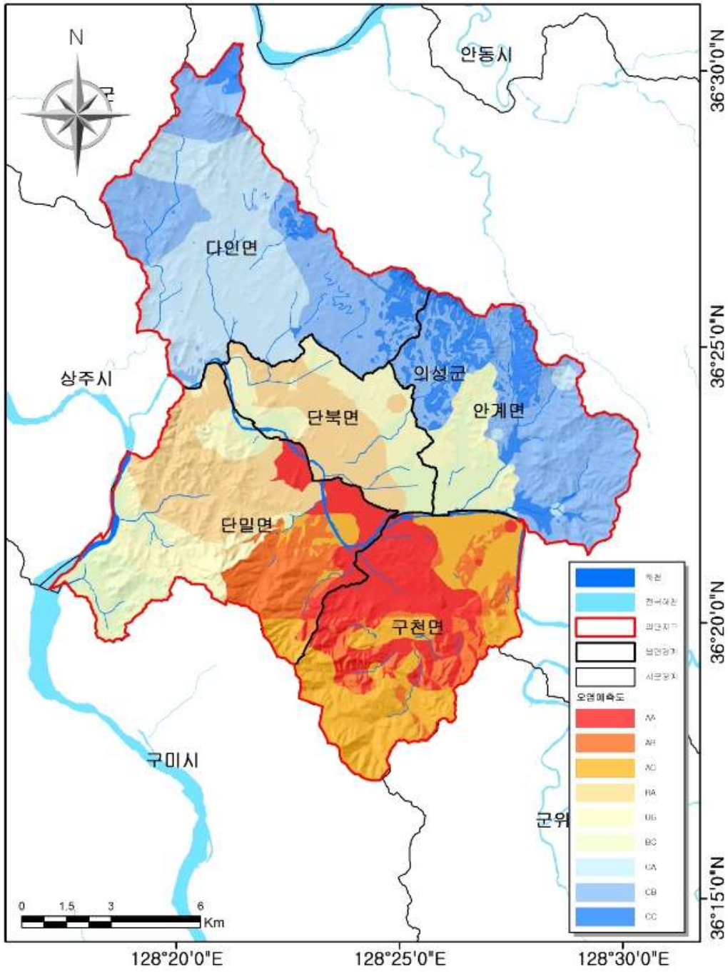
<그림 3-3-5> 의단지구 지하수오염예측도
