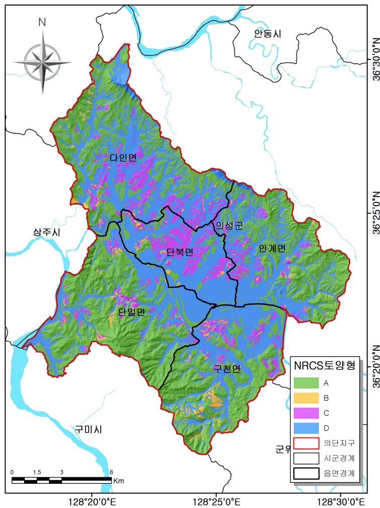
<그림 1-4-13> 의단지구 NRCS 토양도
