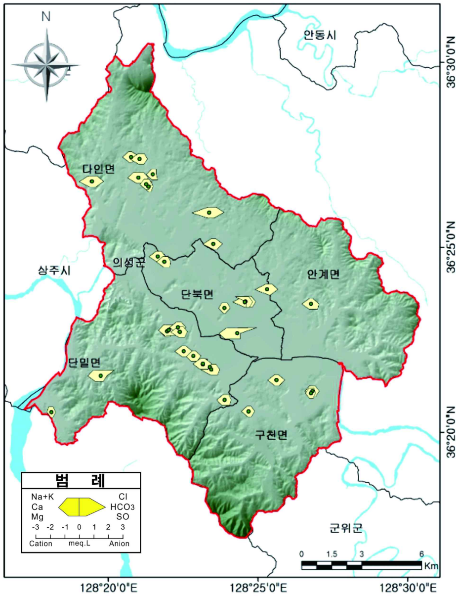
<그림 3-2-16> 의단지구 Stiff 다이어그램
