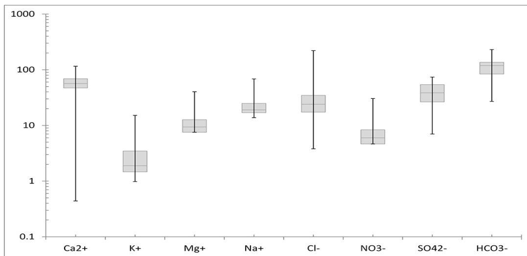
<그림 3-2-13> 주요 양·음이온 농도분포 상자도표
