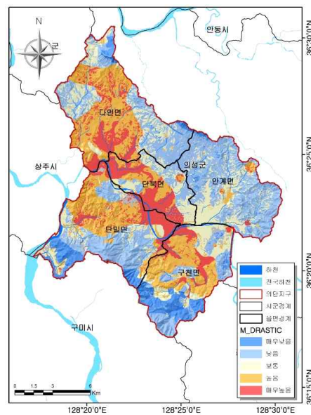
<그림 3-3-2> 의단지구 Modified Drastic Index Map
