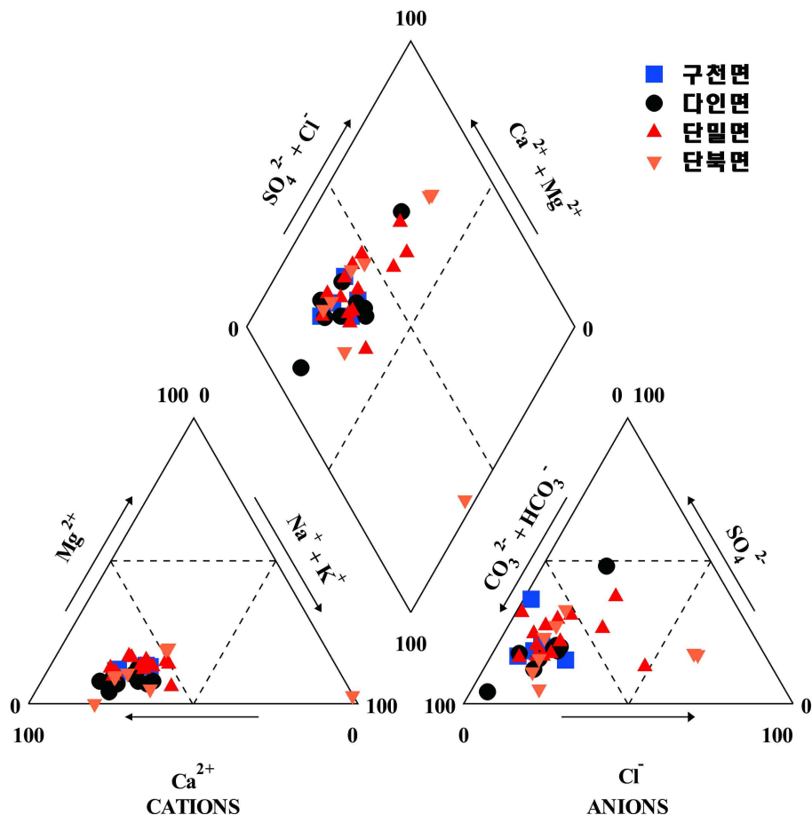
<그림 3-2-15> 의단지구 지하수의 Piper Diagram
