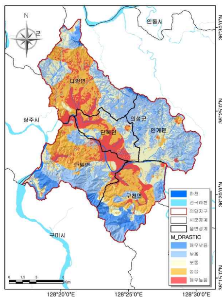
(c) 변형된 오염취약성도 <그림 3-3-3> 변형된 오염취약성도
