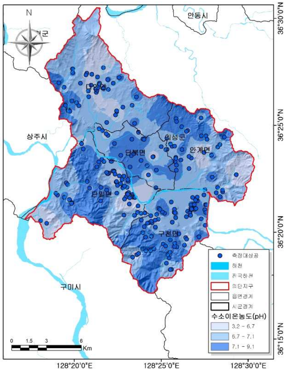
<그림 3-2-6> 의단지구 지하수의 pH 분포도
