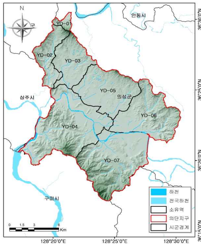
<그림 1-4-7> 의단지구 소유역 현황
