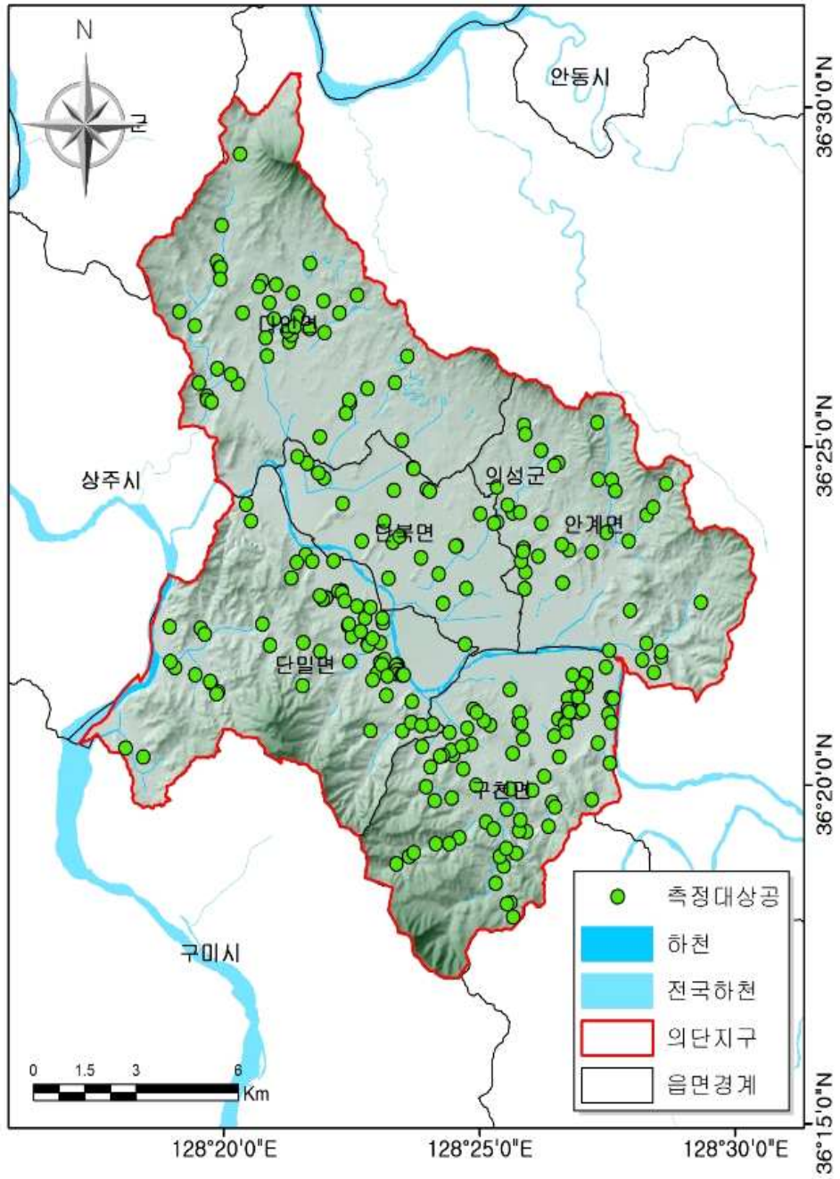
<그림 3-2-4> 의단지구 간이수질 측정대상공 위치도
