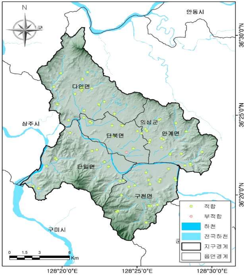
<그림 3-2-18> 수질검사 결과 분포도
