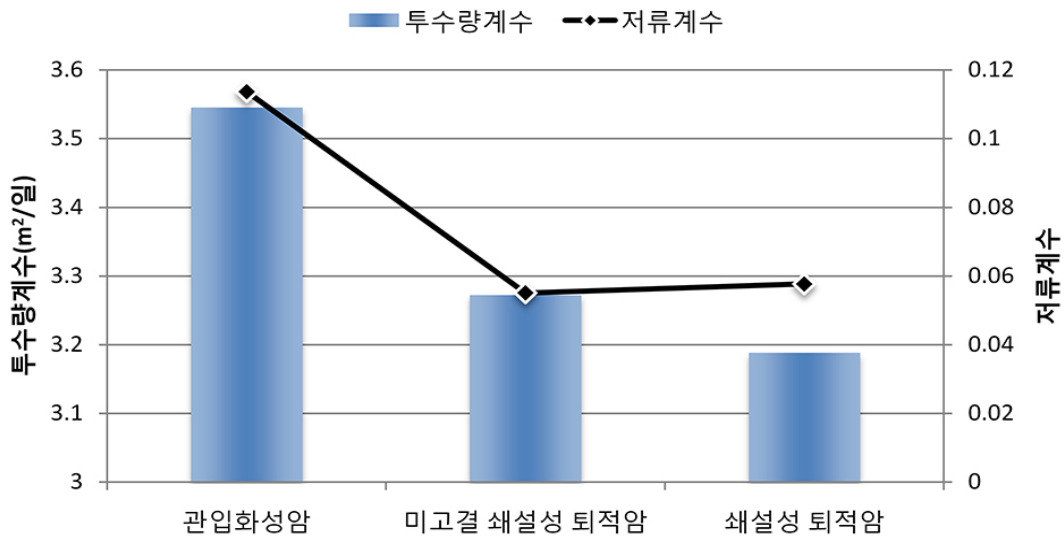
<그림 3-1-7> 수문지질단위별 암반지하수 투수량계수 및 저류계수
