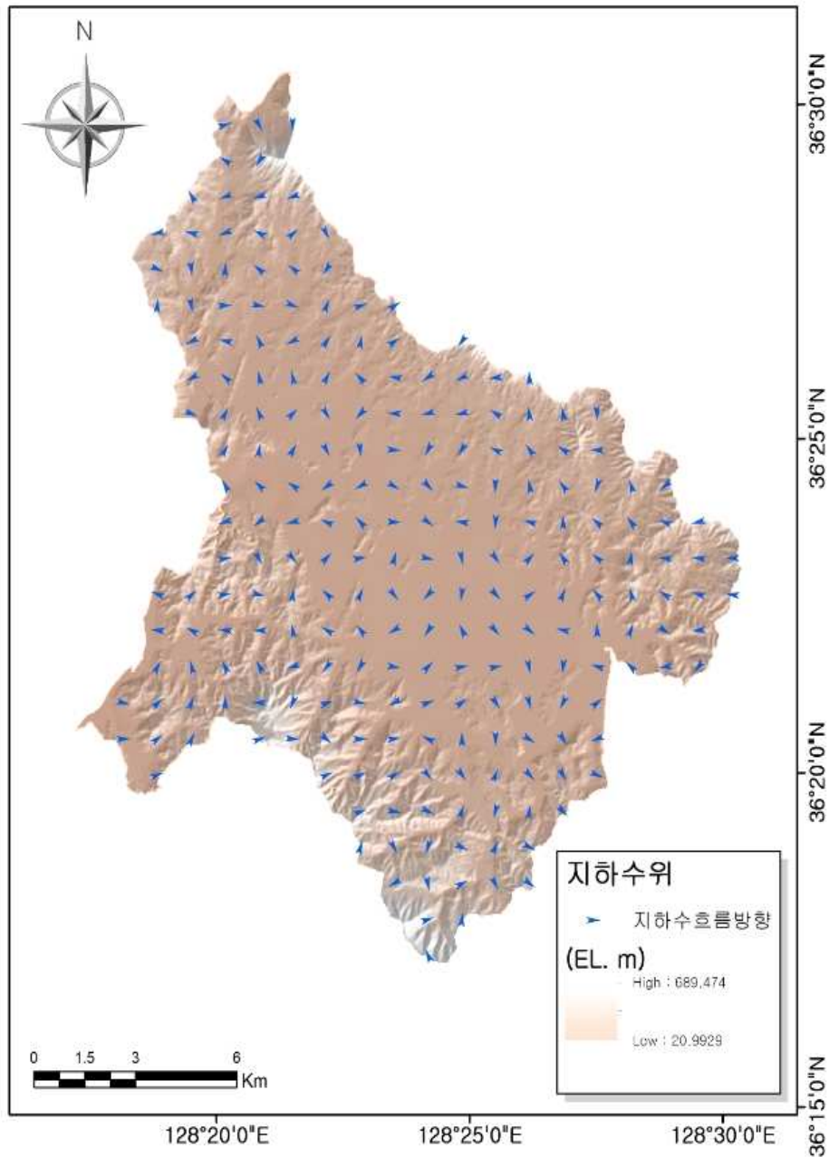
<그림 3-1-1> 지하수위 분포도 및 지하수유동체계
