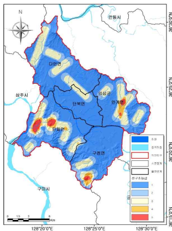
(a) 선구조 가중밀도도
