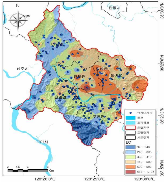
<그림 3-2-7> 의단지구 지하수의 전기전도도(EC, \mu\text{S}/\text{cm} ) 분포도
