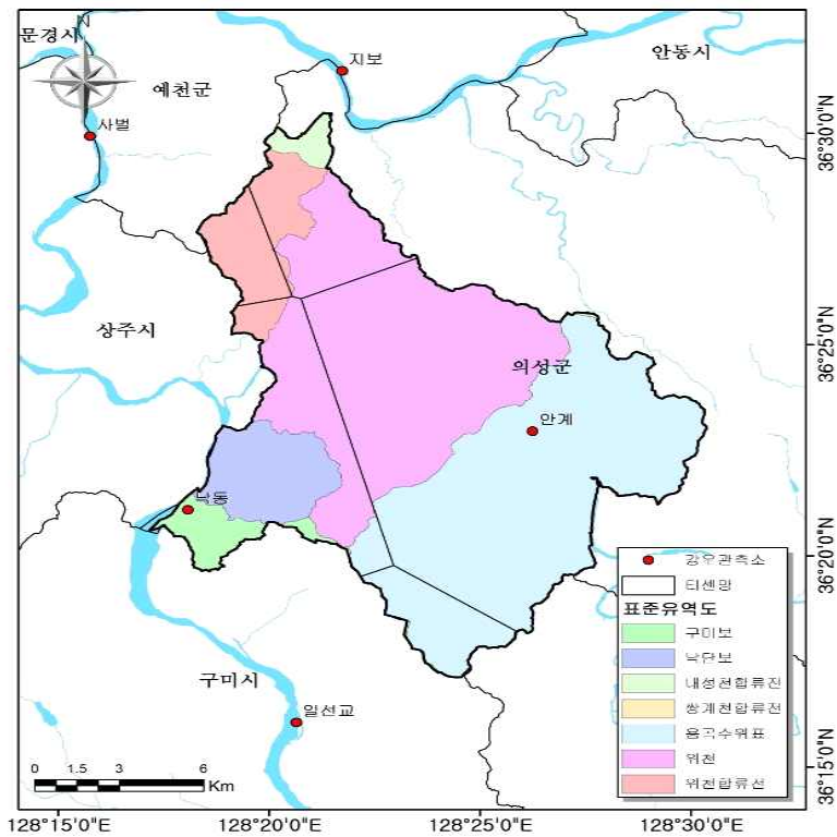
<그림 3-1-8> 의단지구 티센망도
