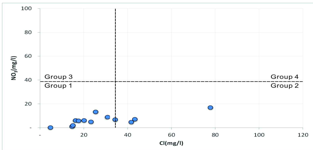
(b)지하수 그룹 분류
