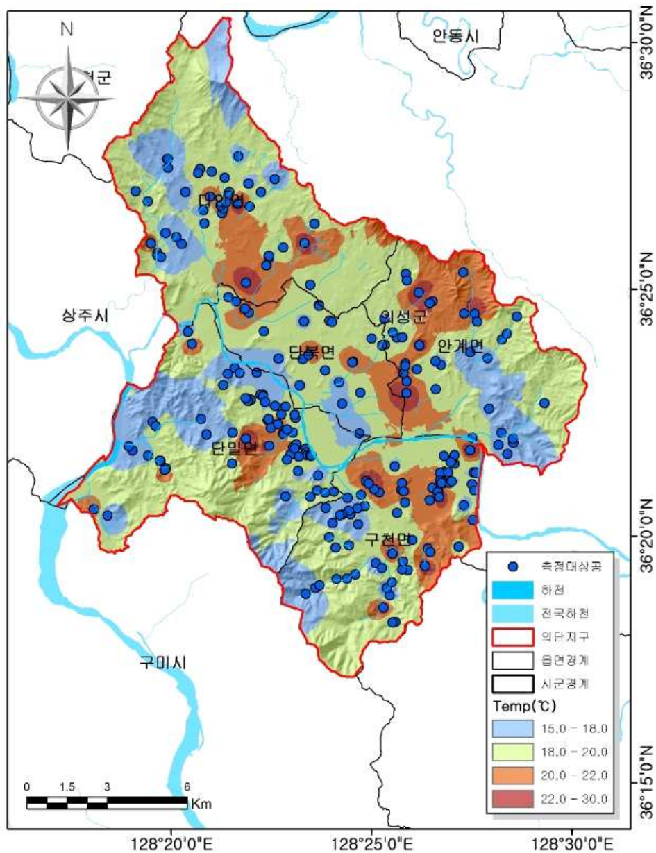
<그림 3-2-5> 의단지구 지하수의 수온(°C) 분포도
