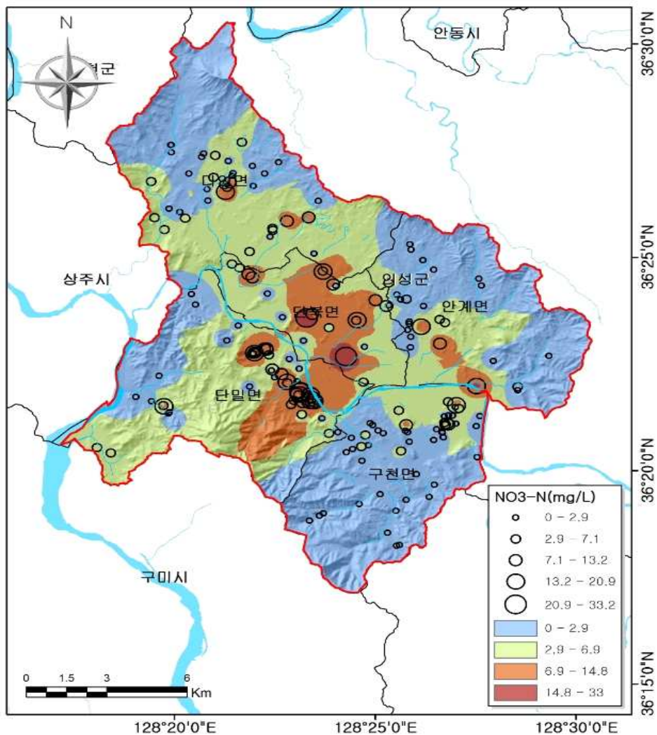
<그림 3-2-9> 의단지구 질산성질소(NO 3 -N, mg/L) 분포도
