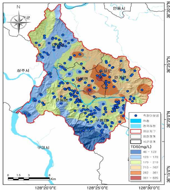
<그림 3-2-8> 의단지구 지하수의 총용존고용물(TDS, mg/L) 분포도
