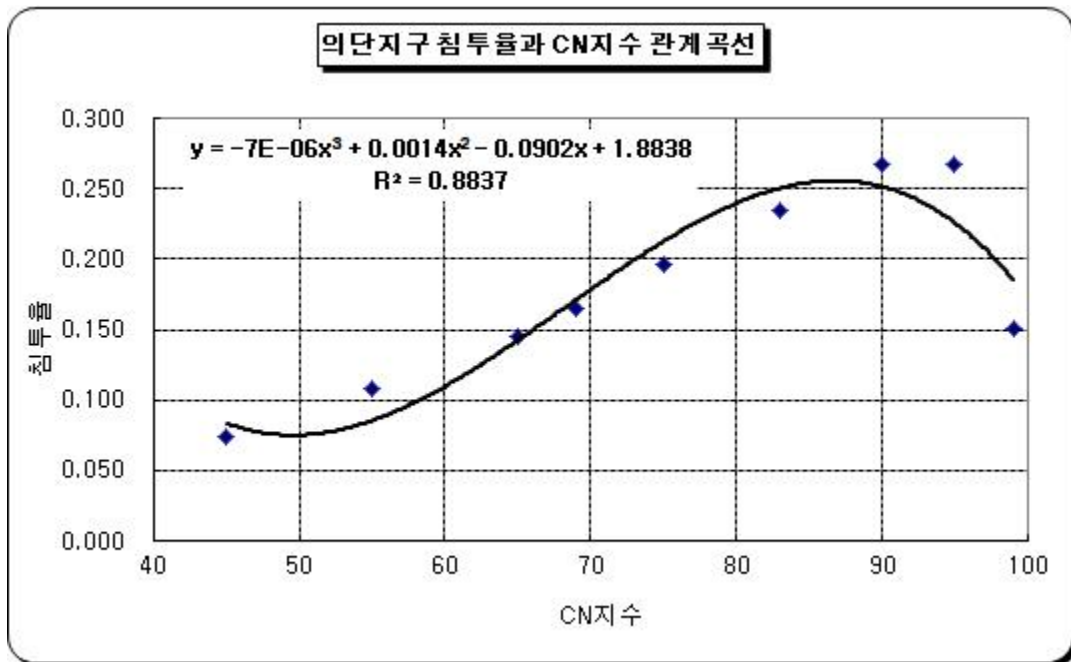
<그림 3-1-10> 함양률(침투율)과 CN지수와의 관계
