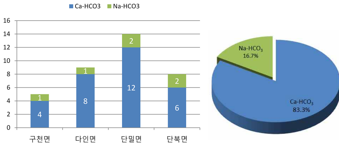
<그림 3-2-17> 의단지구 지하수 유형
