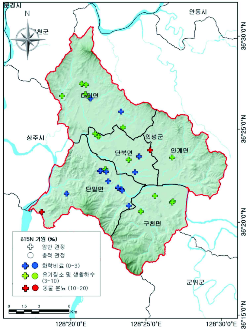
<그림 3-2-10> 질소동위원소 시료채수 위치도
