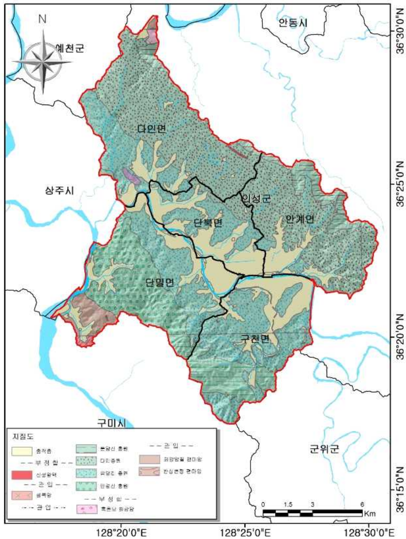
<그림 1-4-10> 의단지구 지질도
