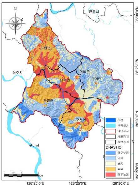
<그림 3-3-1> 의단지구 Drastic Index Map
