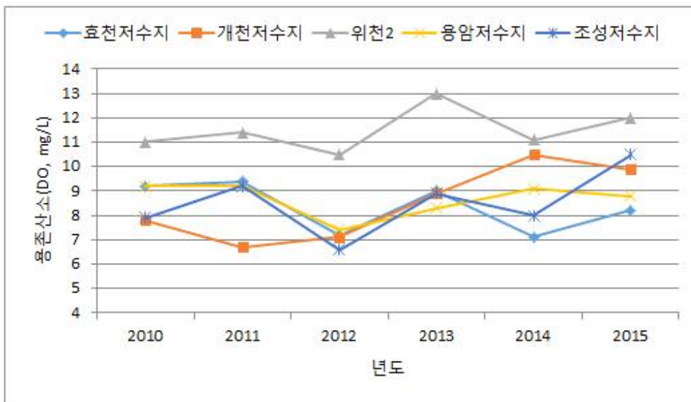
<그림 1-4-4> 연도별 용존산소량(DO) 변화
