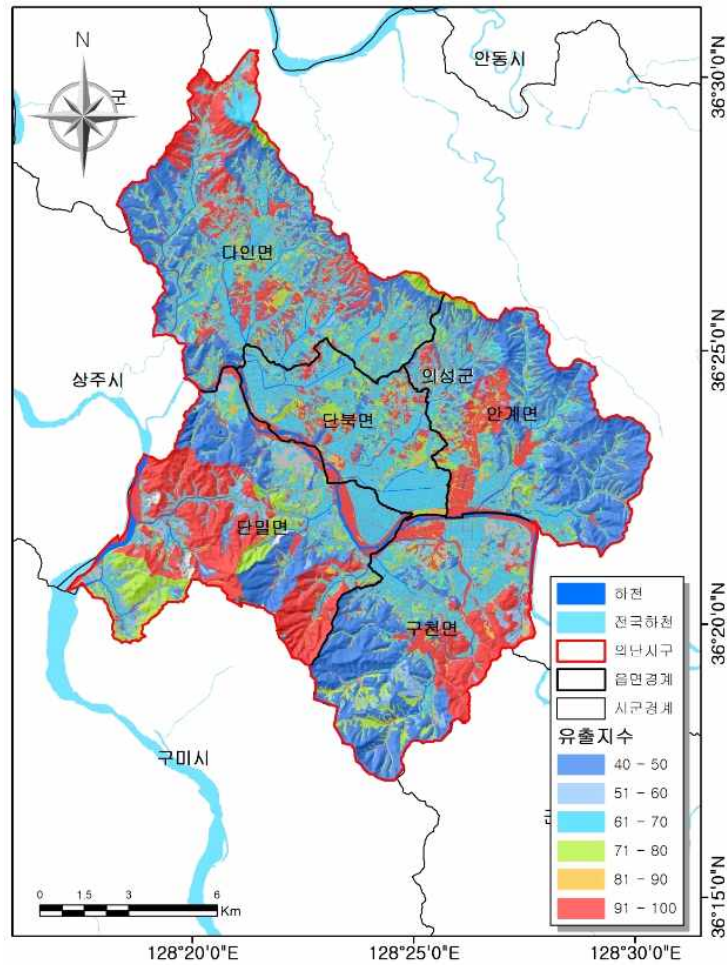
<그림 3-1-9> 유출곡선지수(CN) 분포도
