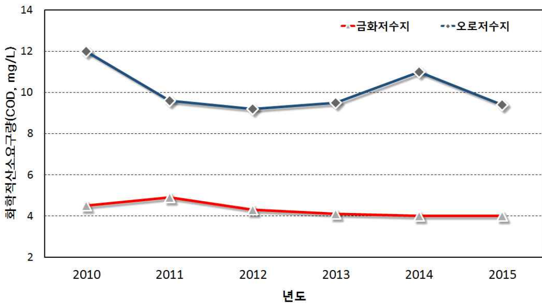
<그림 1-4-3> 연도별 화학적산소요구량(COD) 변화
