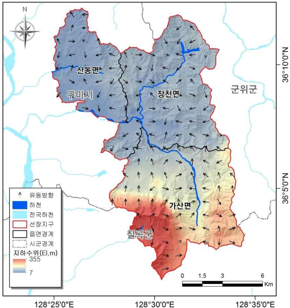
<그림 3-1-1> 지하수위 분포도 및 지하수유동체계
