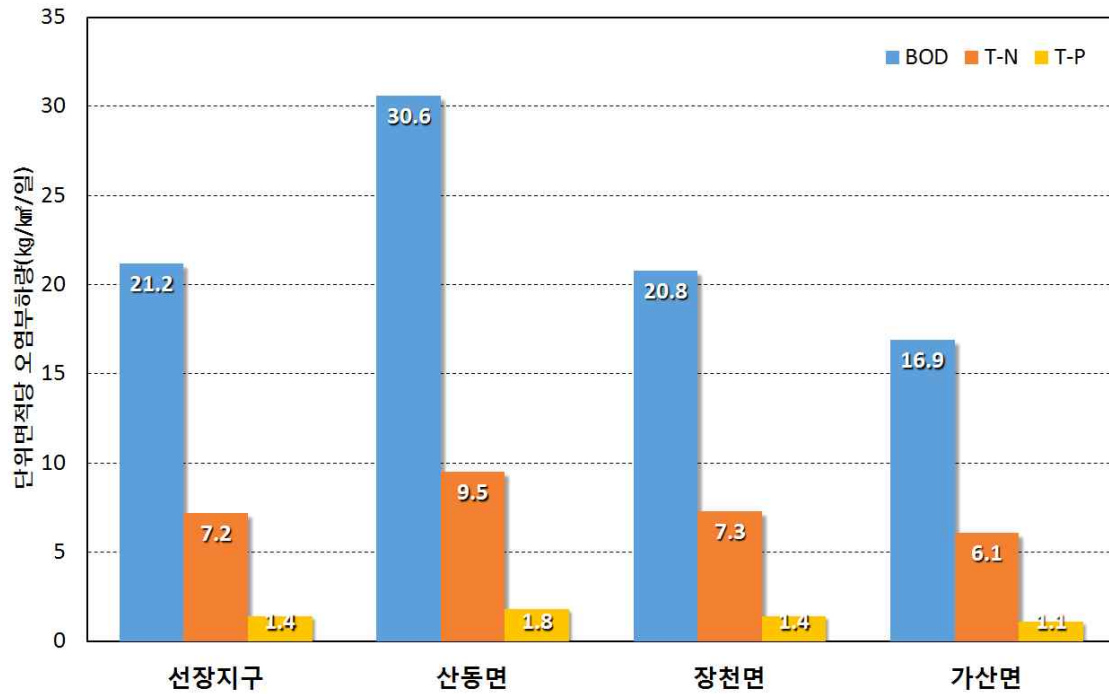
<그림 3-2-2> 읍면별 항목별 단위면적당 오염부하량
