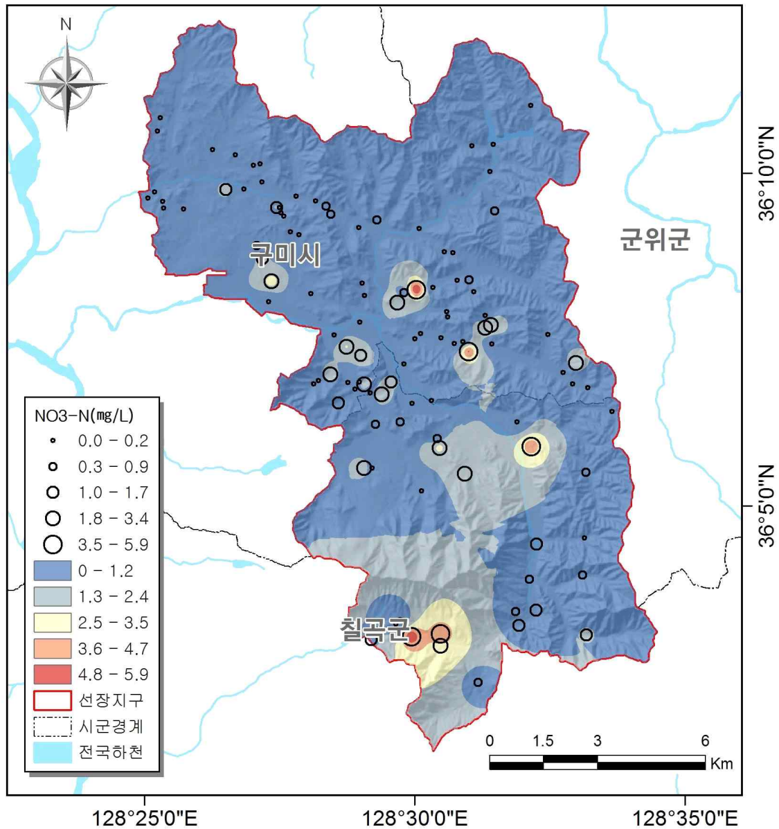
<그림 3-2-9> 선장지구 질산성질소( \text{NO}_3\text{-N} , mg/L) 분포도
