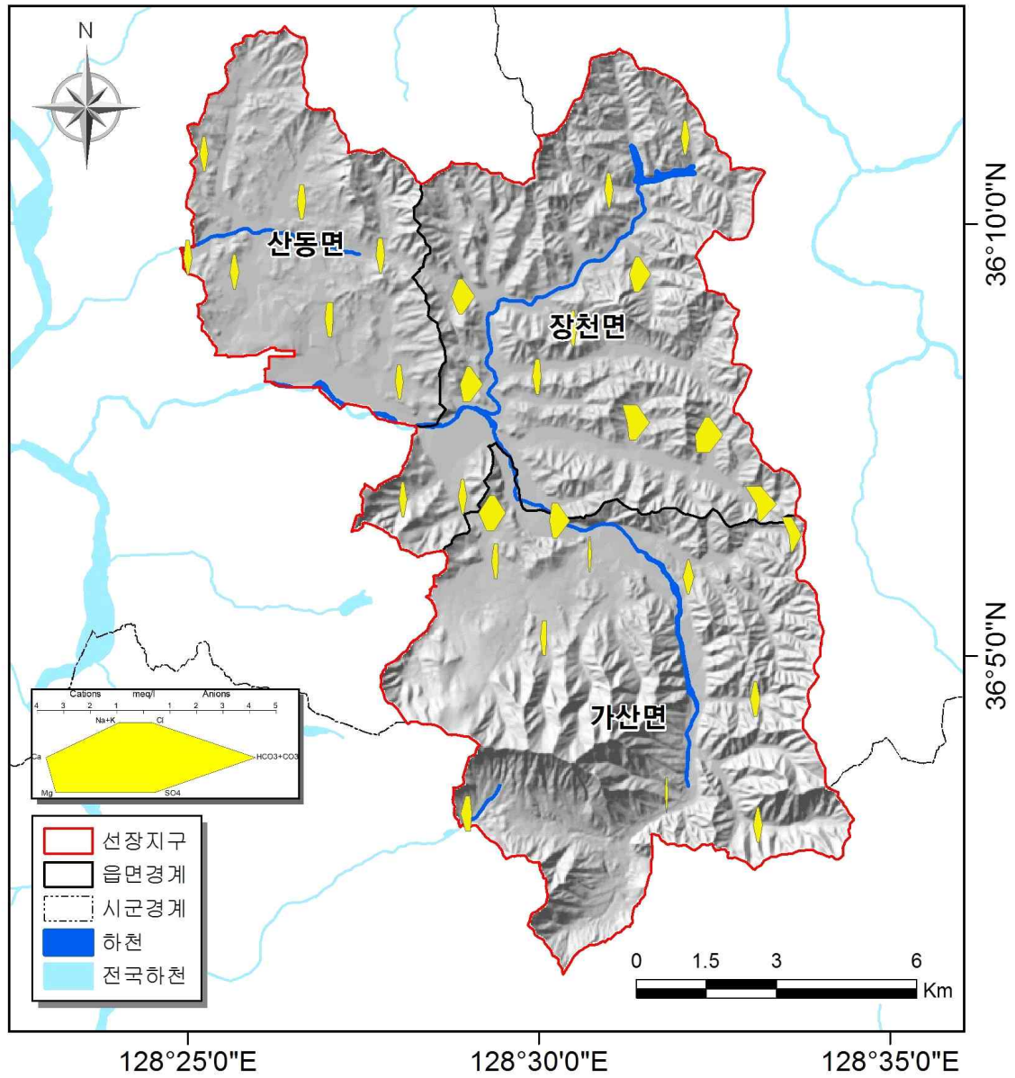
<그림 3-2-16> 선장지구 Stiff 다이어그램
