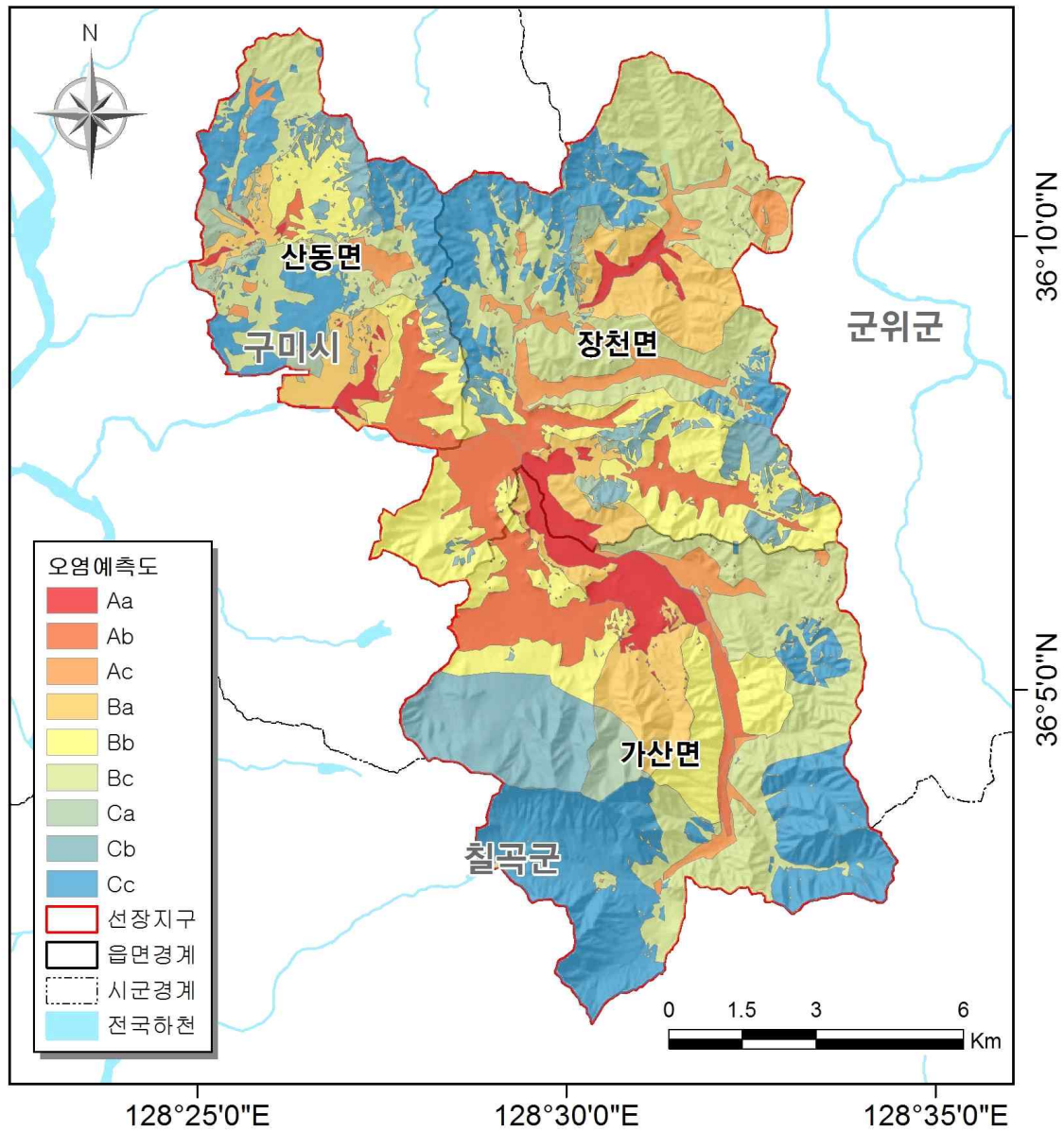
<그림 3-3-5> 선장지구 지하수오염예측도
