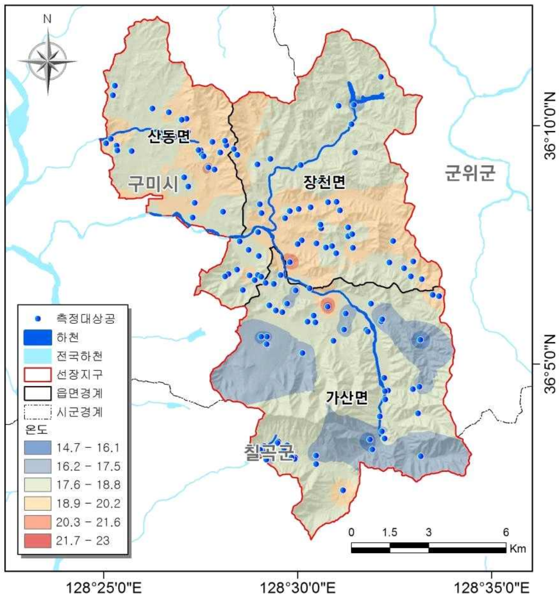
<그림 3-2-5> 선장지구 지하수의 수온(°C) 분포도
