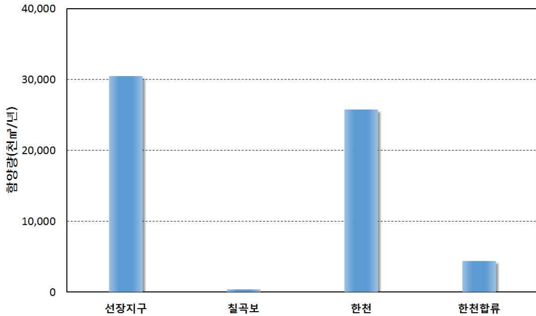
<그림 3-1-11> 표준유역별 지하수 함양량
