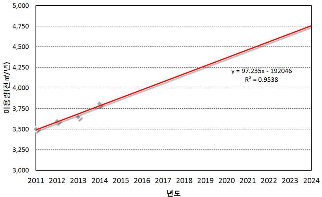
<그림 3-2-6 선장지구 지하수 이용전망 추세>
