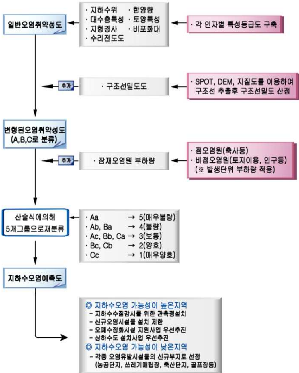
<그림 3-3-4> 지하수오염예측도 작성 모식도
