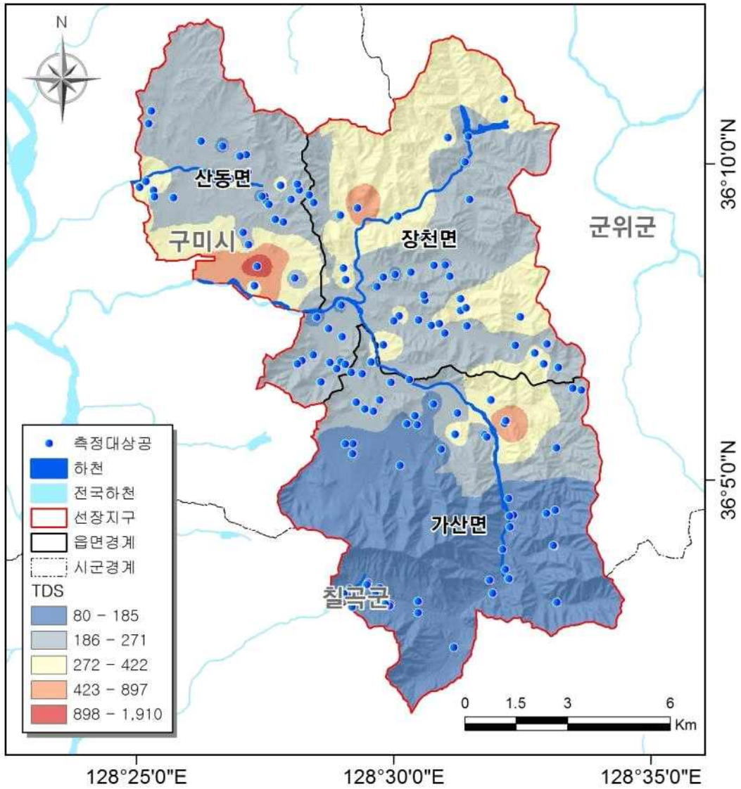
<그림 3-2-8> 선장지구 지하수의 총용존고용물(TDS, mg/L) 분포도
