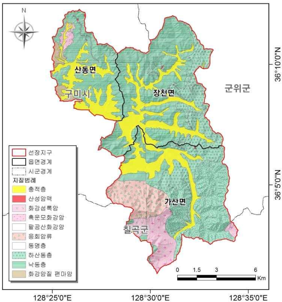
<그림 1-4-10> 선장지구 지질도
