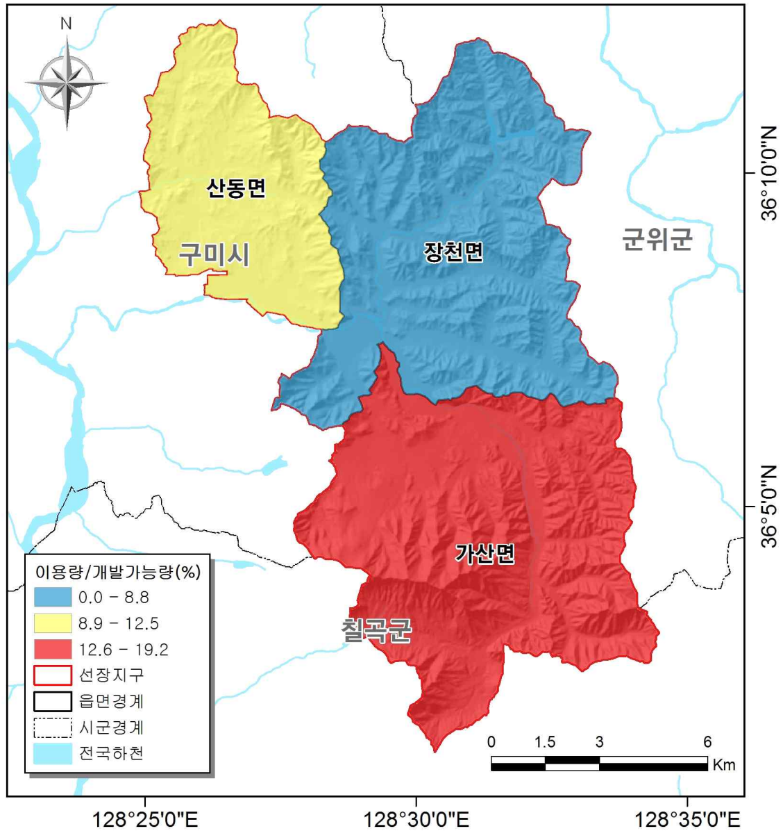
<그림 3-1-16> 행정구역별 이용량 대 개발가능량
