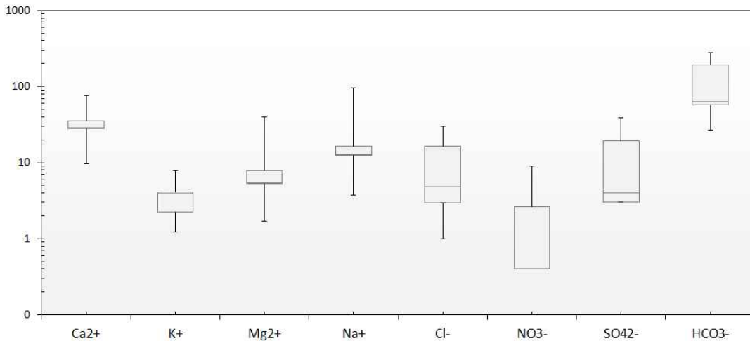
<그림 3-2-13> 주요 양·음이온 농도분포 상자도표
