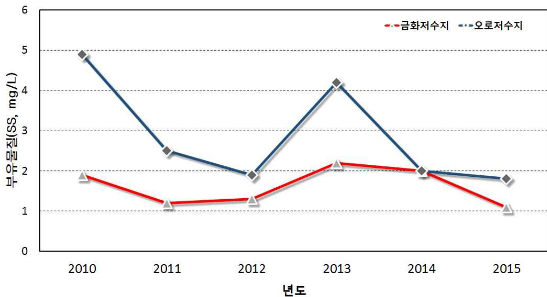
<그림 1-4-5> 연도별 부유물질량(SS) 변화
