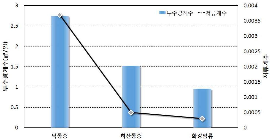
<그림 3-1-5> 지질별 암반지하수 투수량계수 및 저류계수
