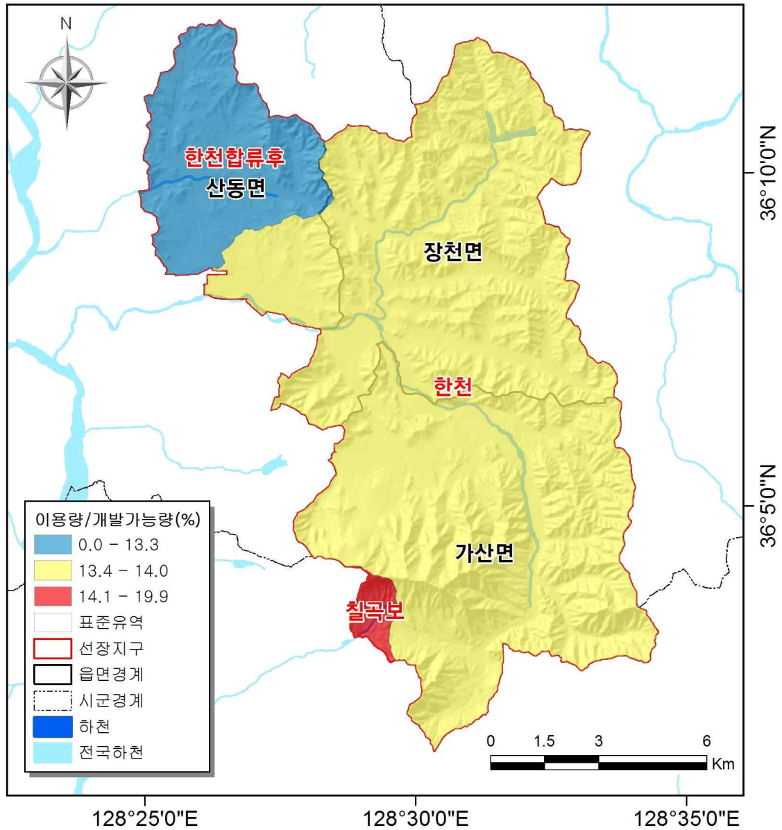
<그림 3-1-14> 표준구역별 이용량 대 개발가능량
