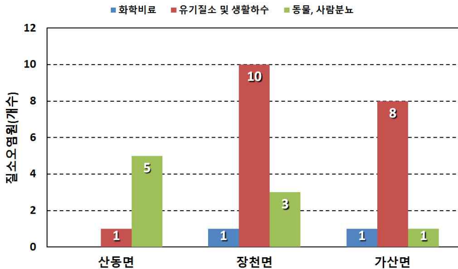
<그림 3-2-12> 읍면별 질소오염원 구성비
