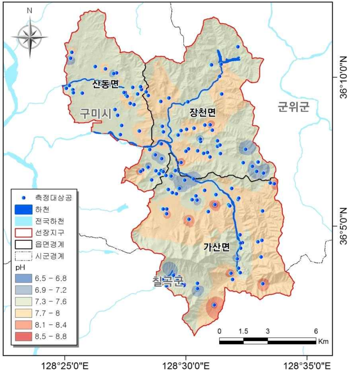
<그림 3-2-6> 선장지구 지하수의 pH 분포도
