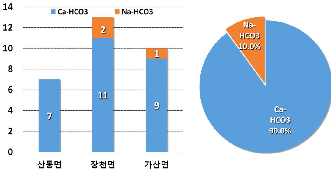
<그림 3-2-17> 선장지구 지하수 유형
