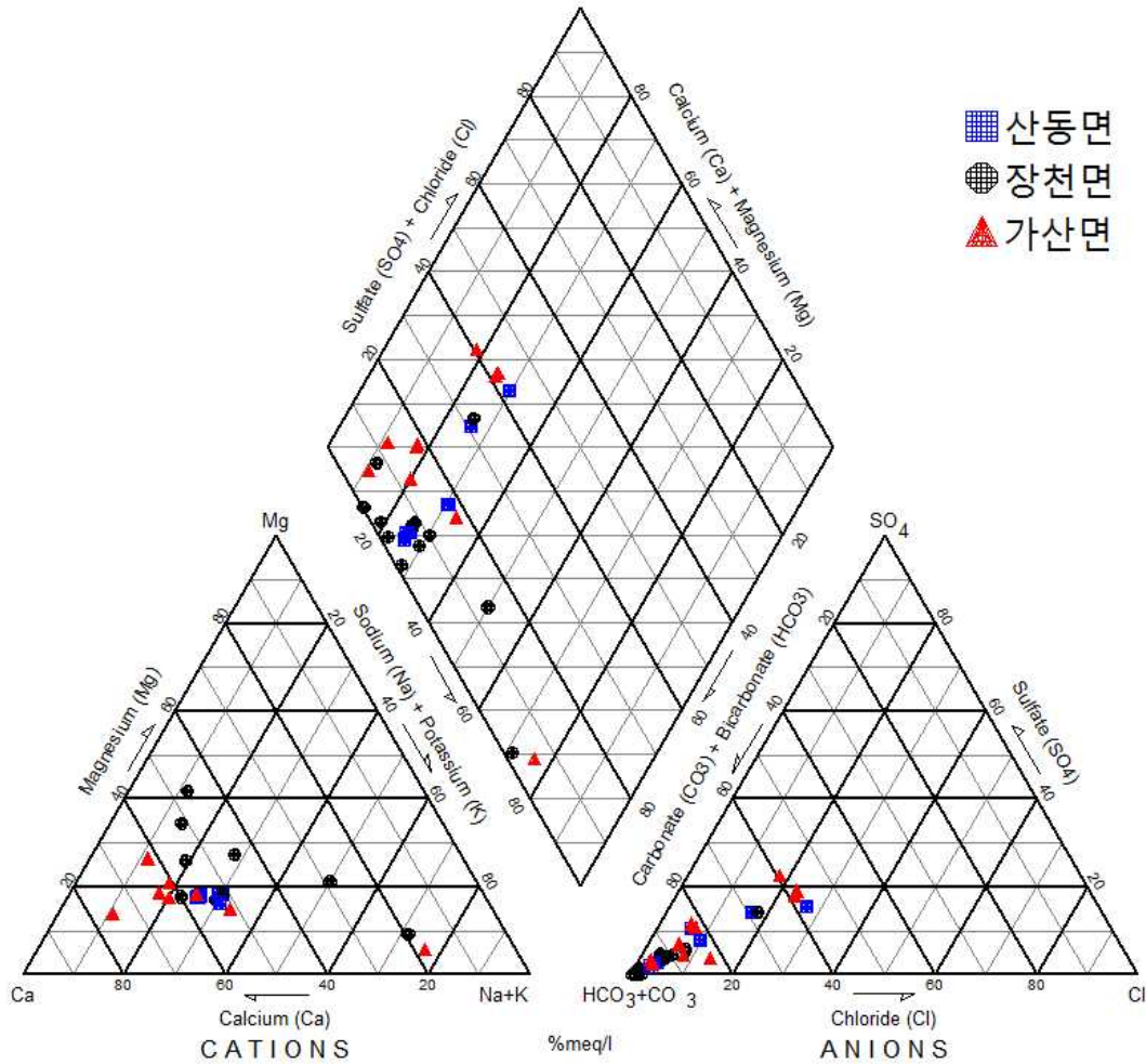
<그림 3-2-15> 선장지구 지하수의 Piper Diagram
