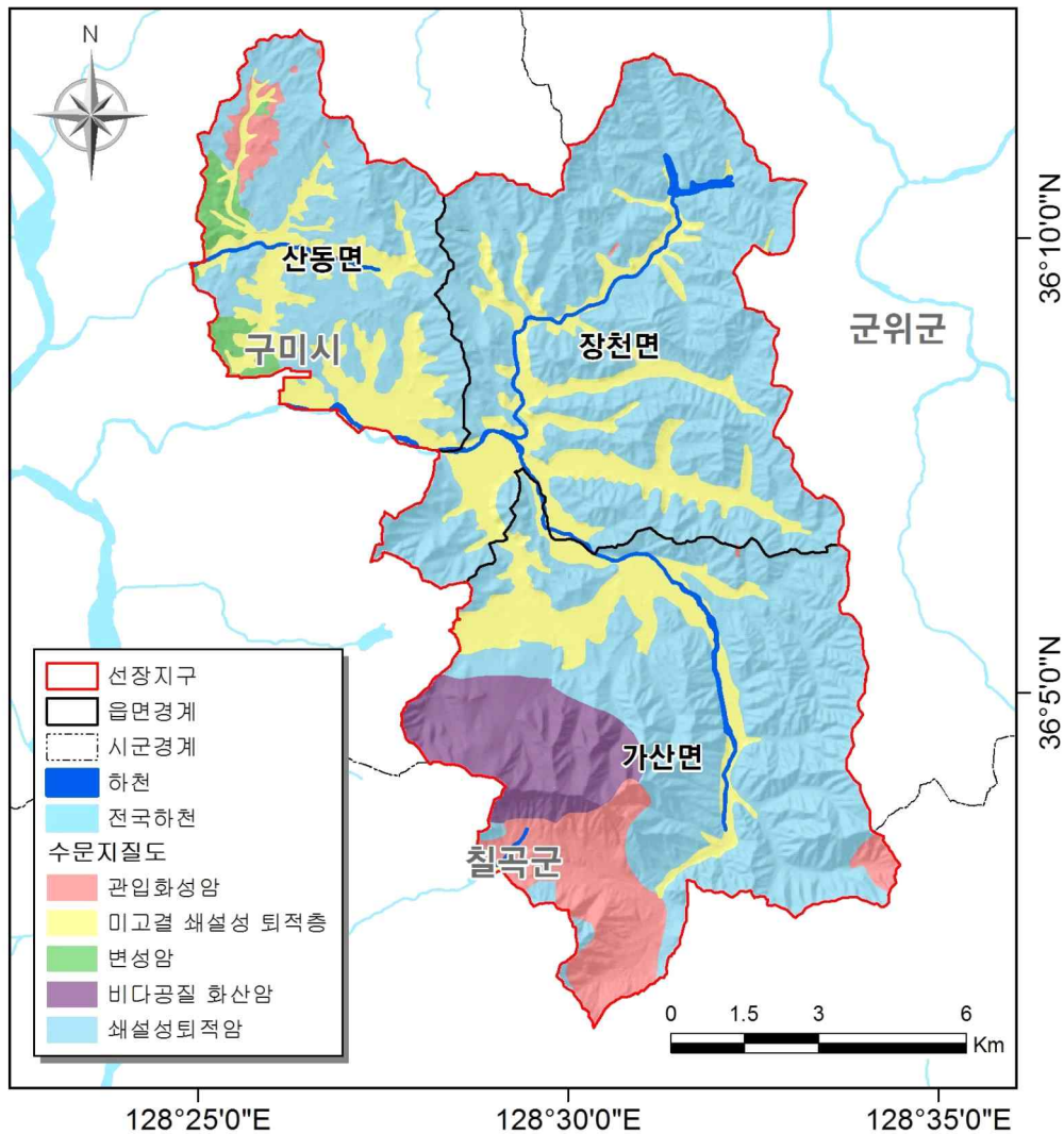
<그림 1-4-11> 선장지구 수문지질도
