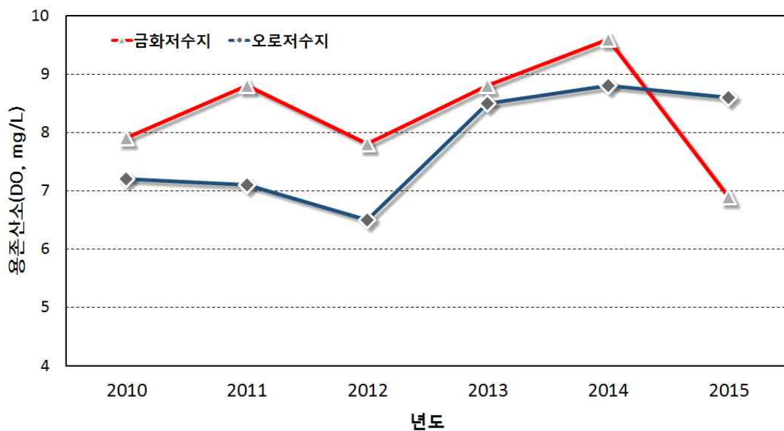
<그림 1-4-4> 연도별 용존산소량(DO) 변화
