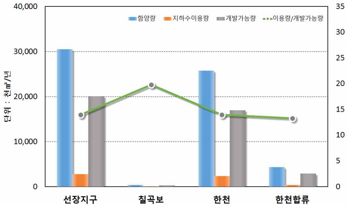
<그림 3-1-13> 표준유역별 지하수 함양량, 이용량 및 개발가능량
