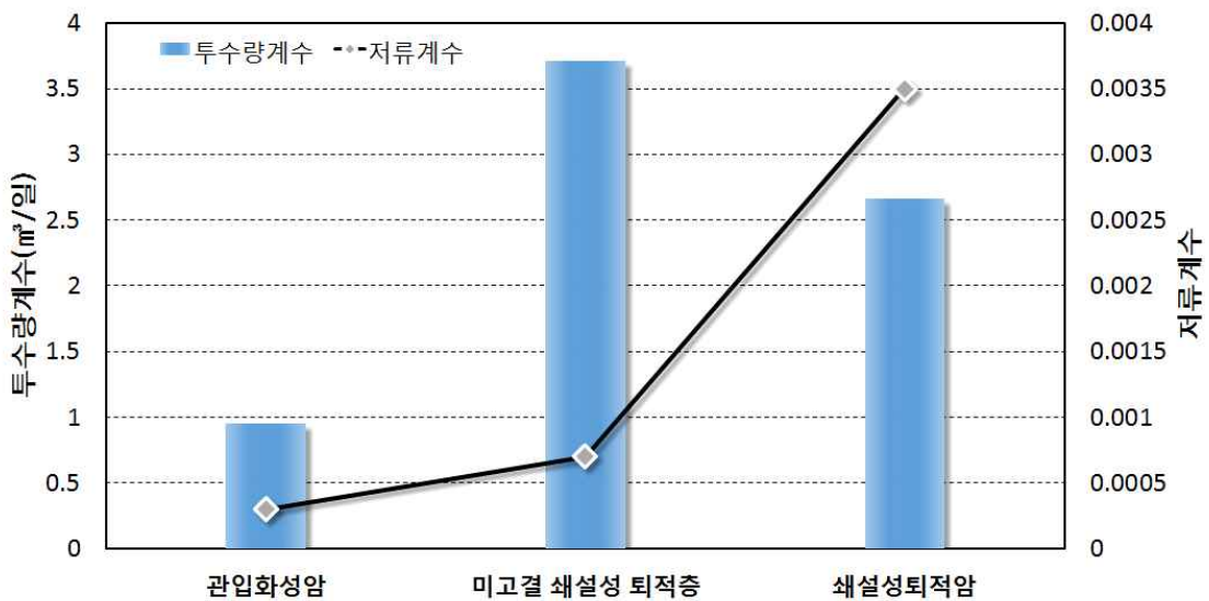
<그림 3-1-7> 수문지질단위별 암반지하수 투수량계수 및 저류계수
