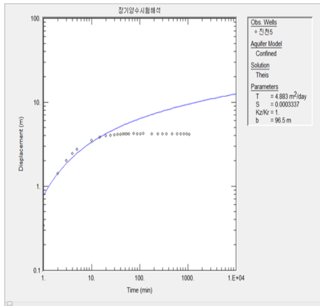
<진천5 관측공 양수시험>
