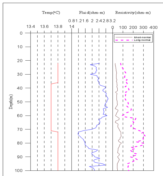
<청양6 관측공 물리검층>
