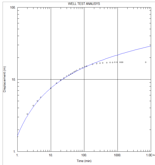
<청양6 관측공 양수시험>
