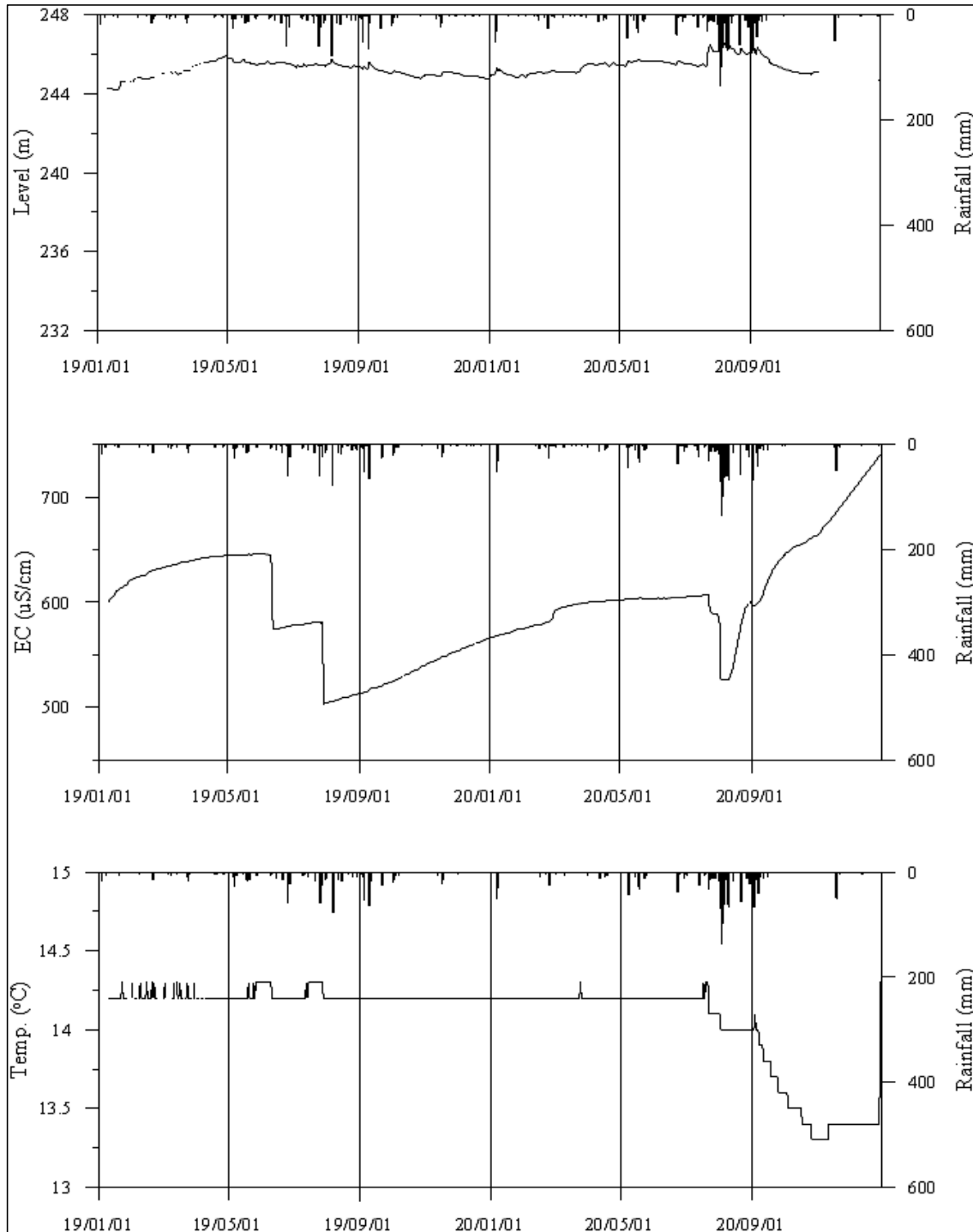
<인제3 관측공의 장기관측자료 (2019.1.1 ~ 2020.12.31)> (a)지하수위, (b)전기전도도, (c)수온
