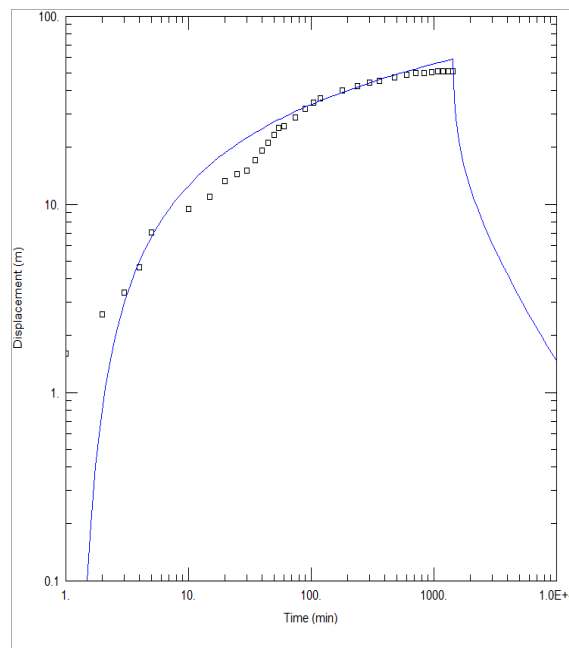
<김천5 관측공 양수시험>
