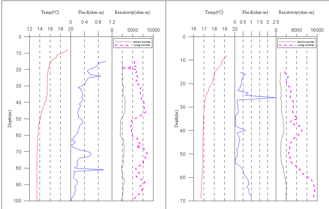
<영월7 관측공 물리검층>
