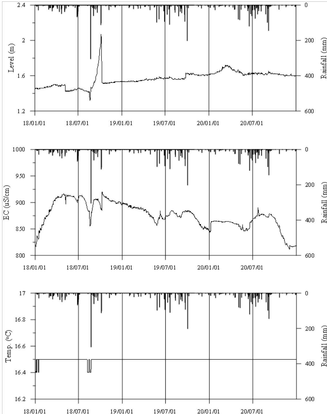
<진도3 관측공의 장기관측자료 (2018.1.1.~2020.12.31)> (a)지하수위, (b)전기전도도, (c)수온
