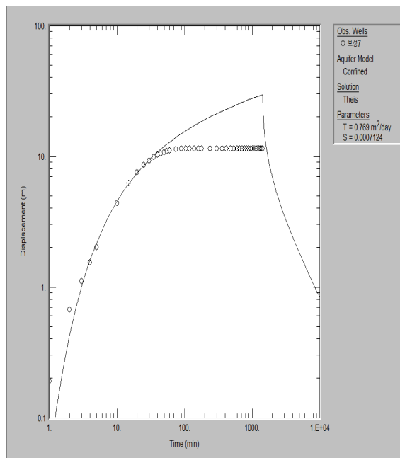
<보성7 관측공 양수시험>
