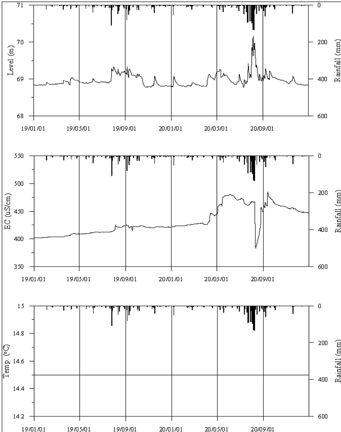
<용인4 관측공의 장기관측자료 (2019.1.1 ~ 2020.12.31)> (a)지하수위, (b)전기전도도, (c)수온
