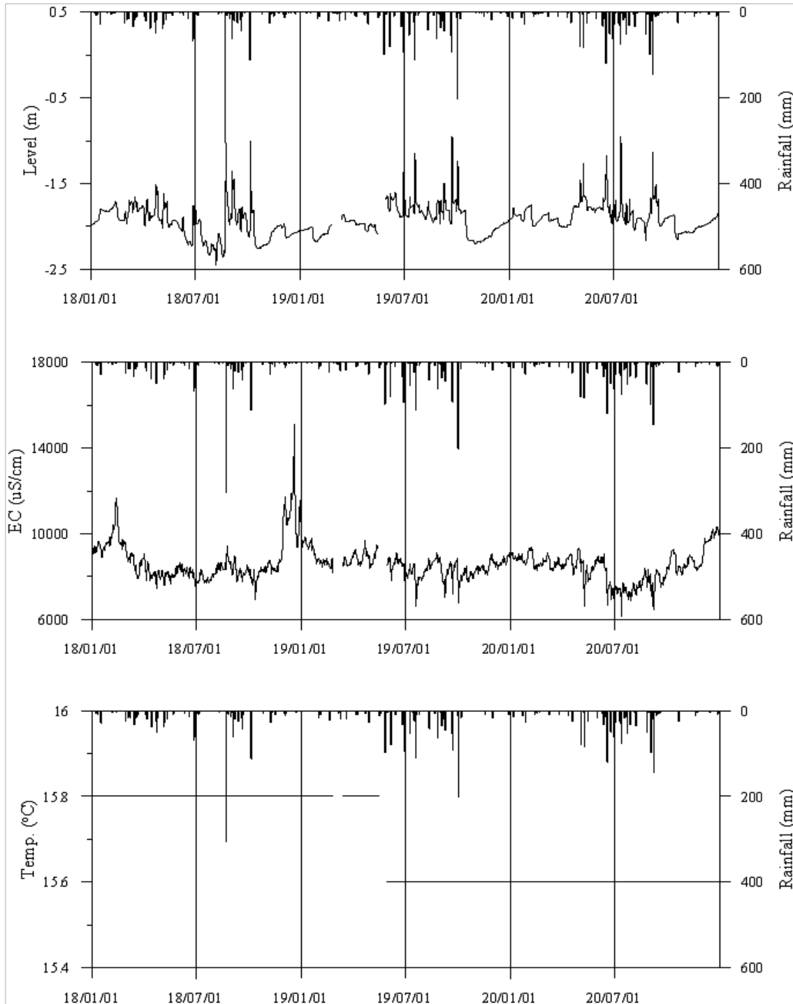
<진도4 관측공의 장기관측자료 (2018.1.1.~2020.12.31)> (a)지하수위, (b)전기전도도, (c)수온
