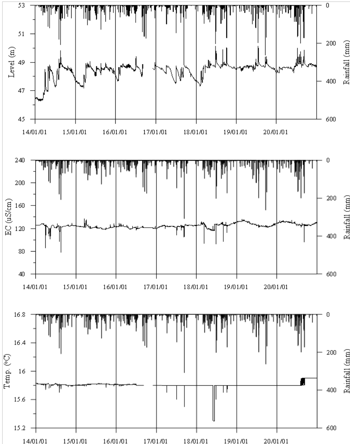
<거제2 관측공의 장기관측자료 (2014.1.1 ~ 2020.12.31)> (a)지하수위, (b)전기전도도, (c)수온
