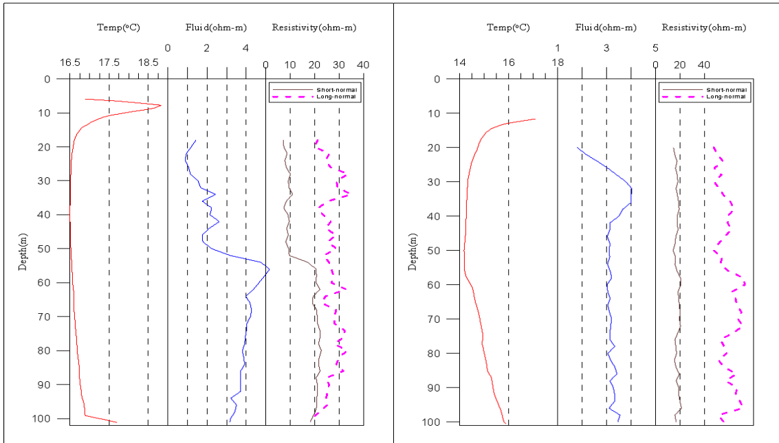
<사천1(신) 관측공 물리검층>
