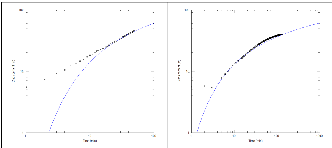
<여주7 관측공 양수시험>
