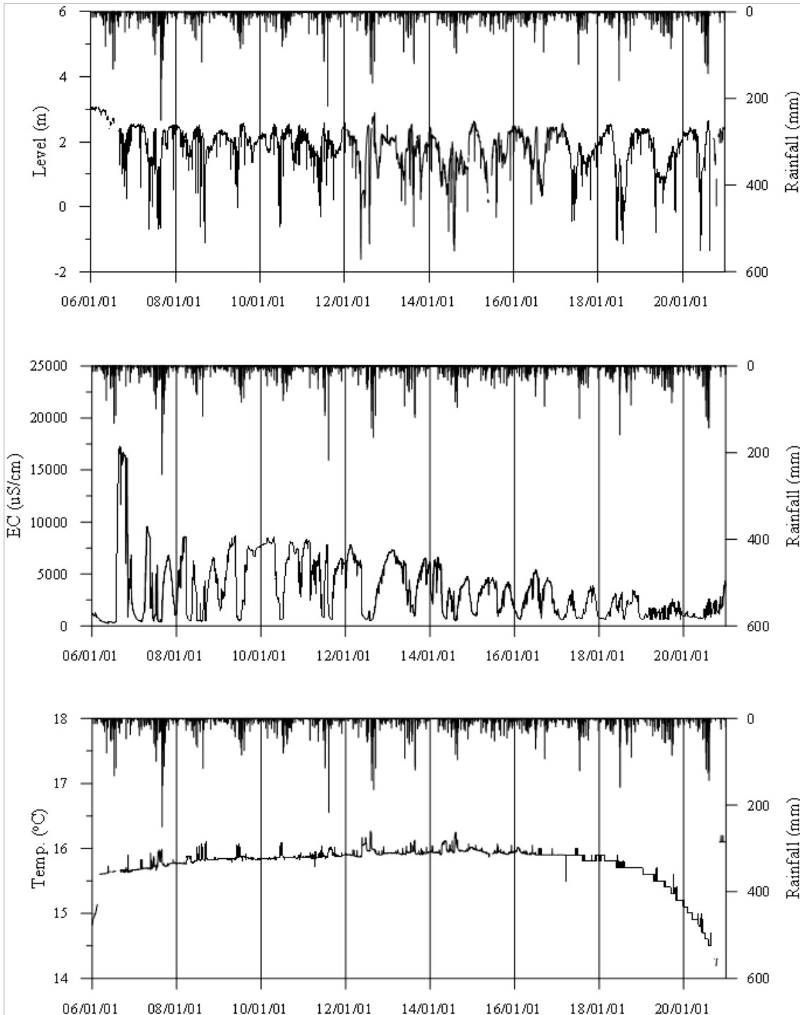
<부안1 관측공의 장기관측자료 (2006.1.1 ~ 2020.12.31)> (a)지하수위, (b)전기전도도, (c)수온
