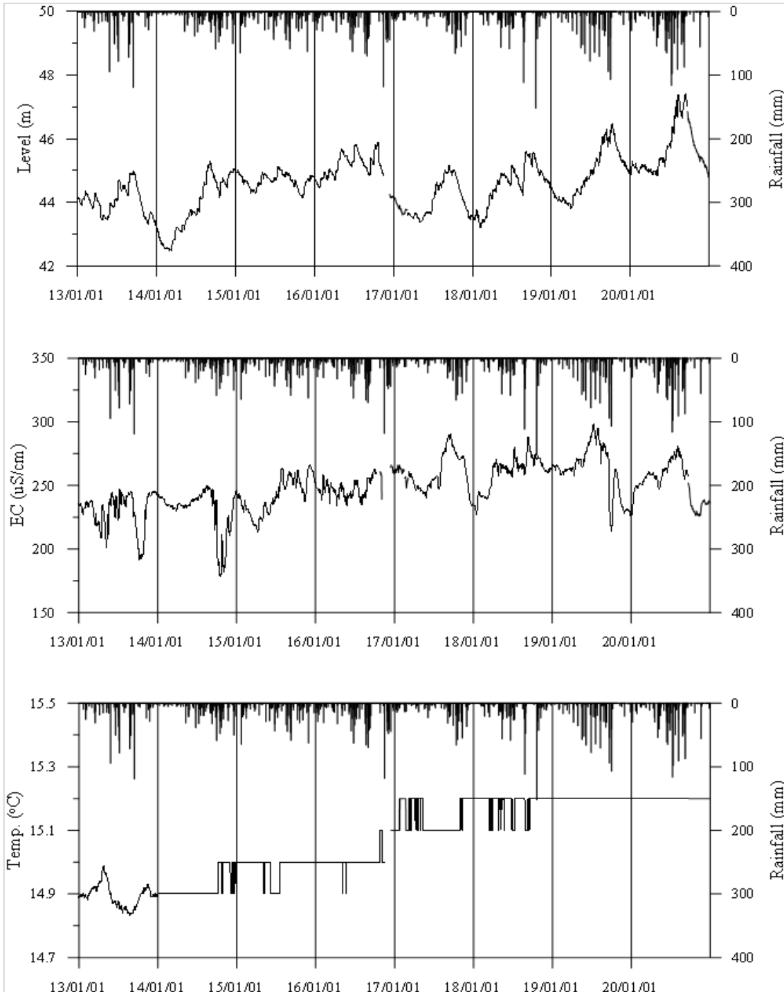
<함평1 관측공의 장기관측자료 (2013.1.1~2020.12.31)> (a)지하수위, (b)전기전도도, (c)수온
