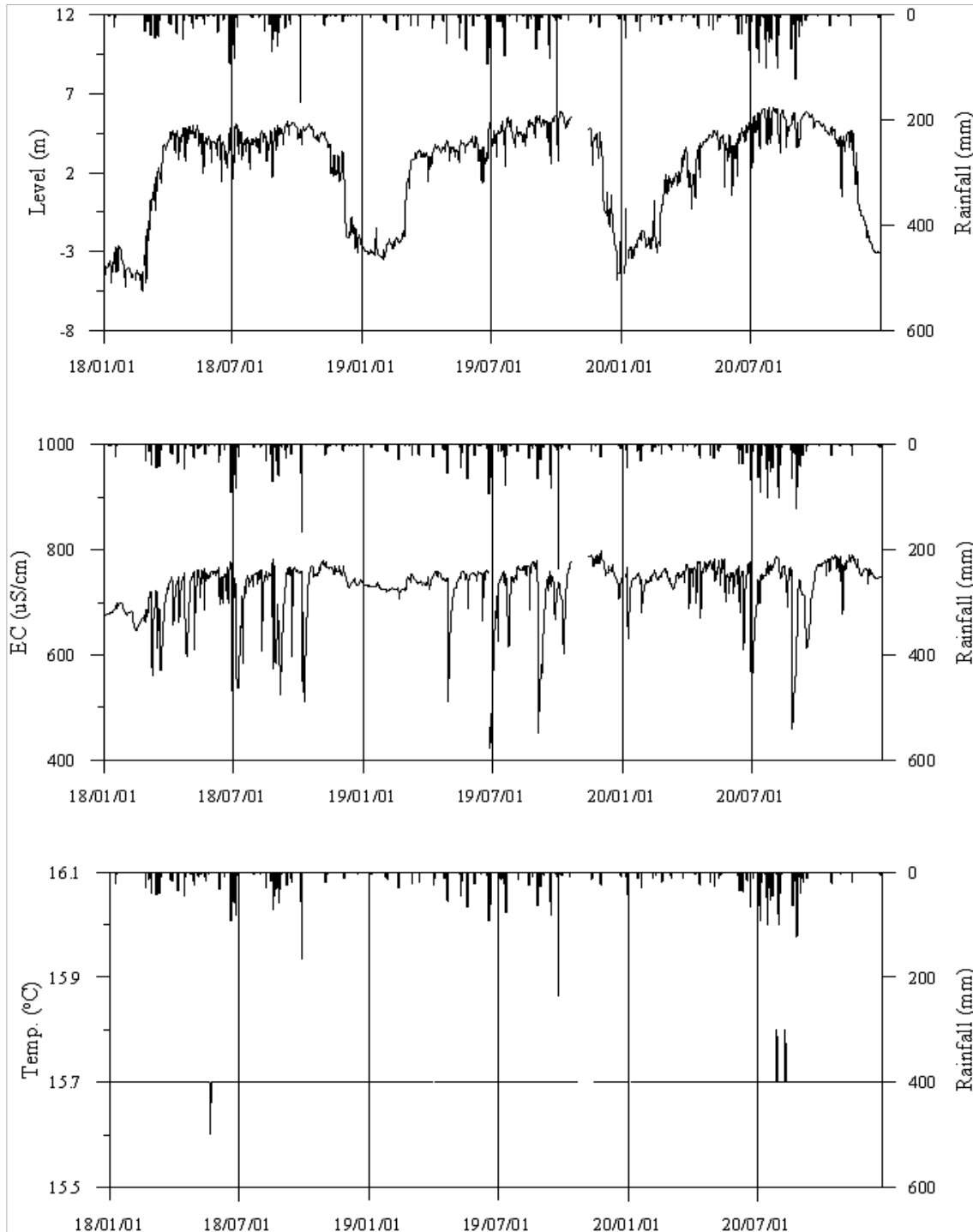
<의령4 관측공의 장기관측자료 (2018.1.1 ~ 2020.12.31)> (a)지하수위, (b)전기전도도, (c)수온
