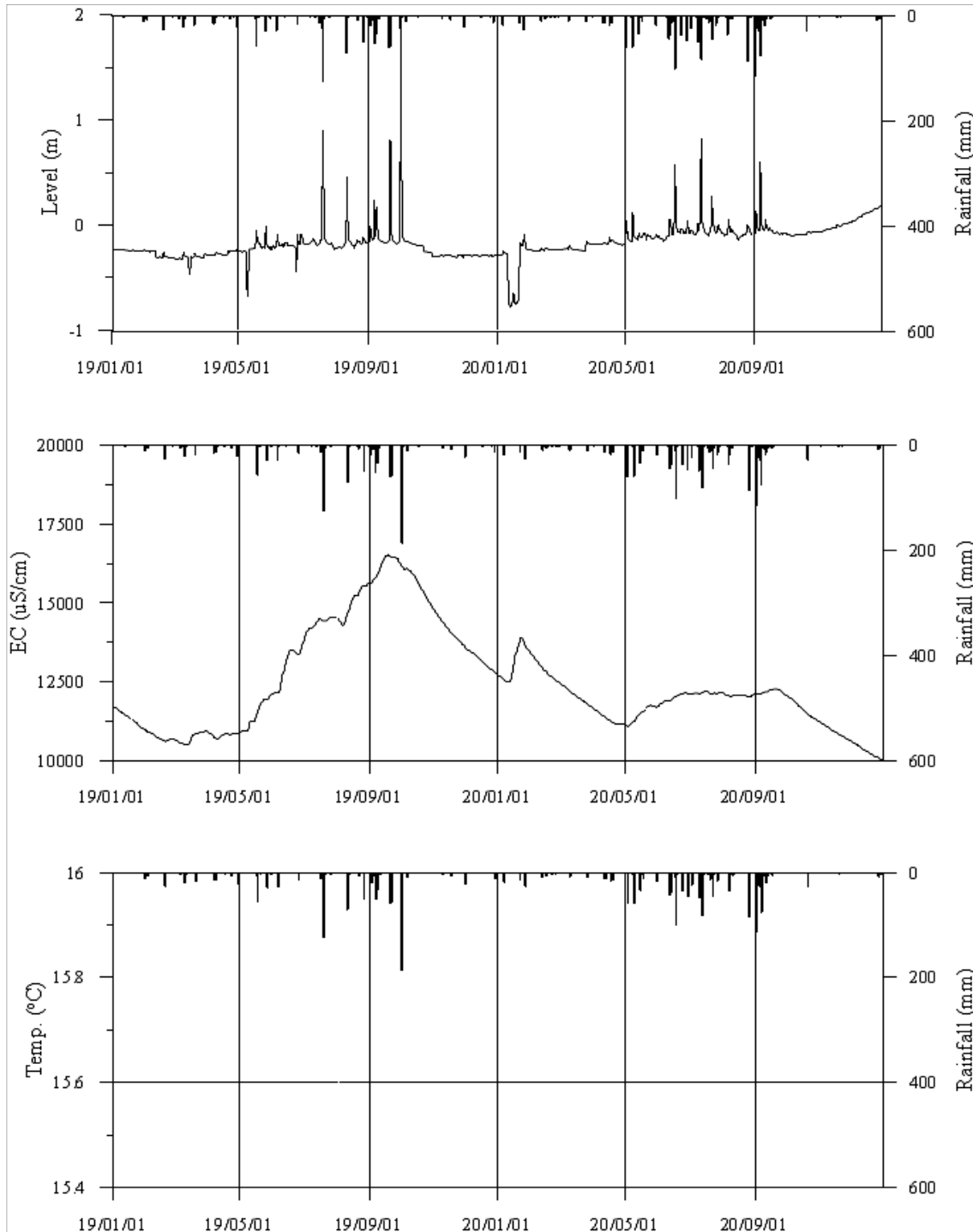
<해남3 관측공의 장기관측자료 (2019.1.1~2020.12.31)> (a)지하수위, (b)전기전도도, (c)수온
