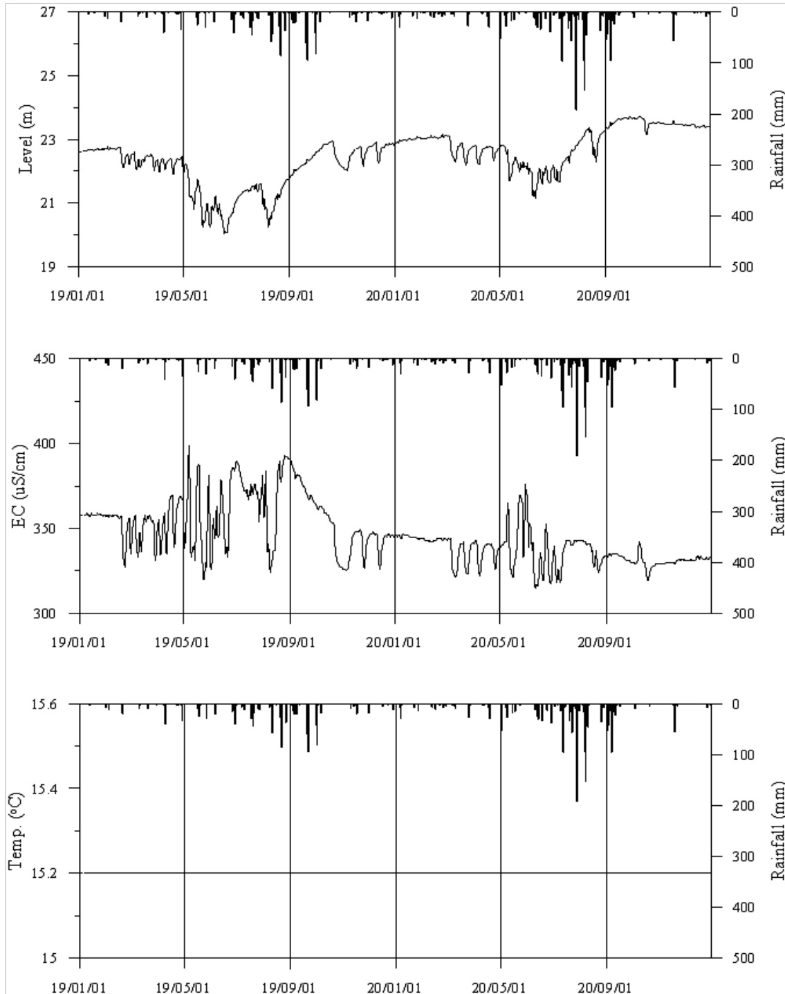
<영광6 관측공의 장기관측자료 (2017.1.1 ~ 2020.12.31)> (a)지하수위, (b)전기전도도, (c)수온
