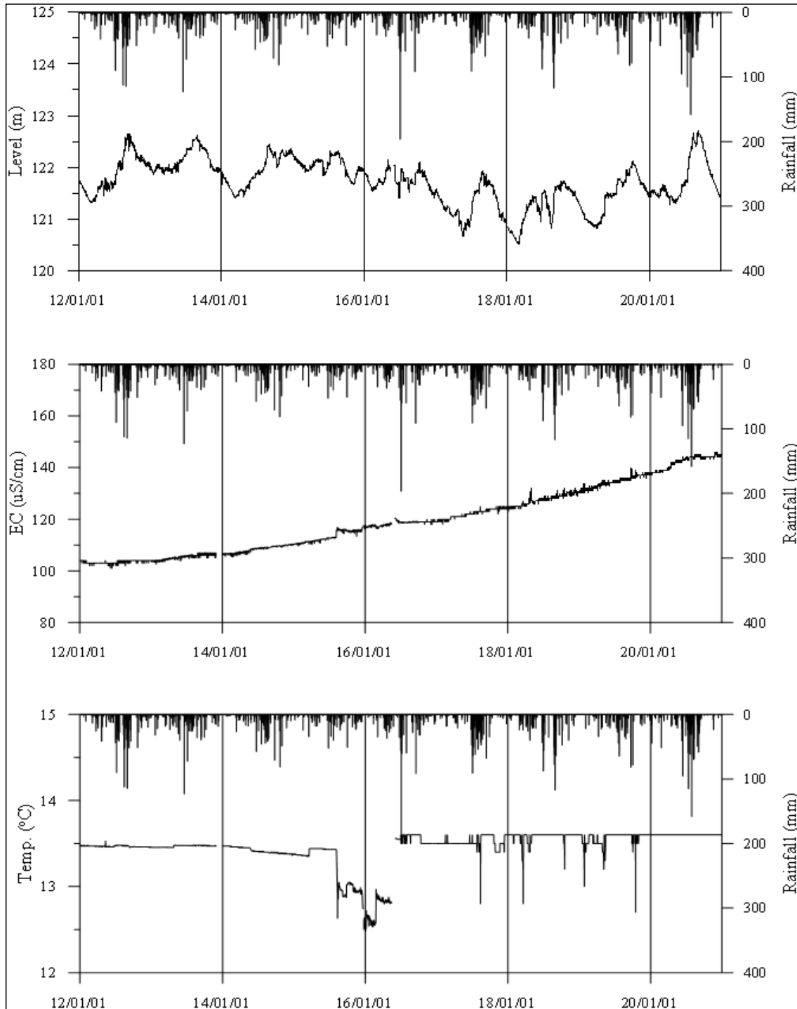
<옥천2 관측공의 장기관측자료 (2012.1.1 ~ 2020.12.31)> (a)지하수위, (b)전기전도도, (c)수온
