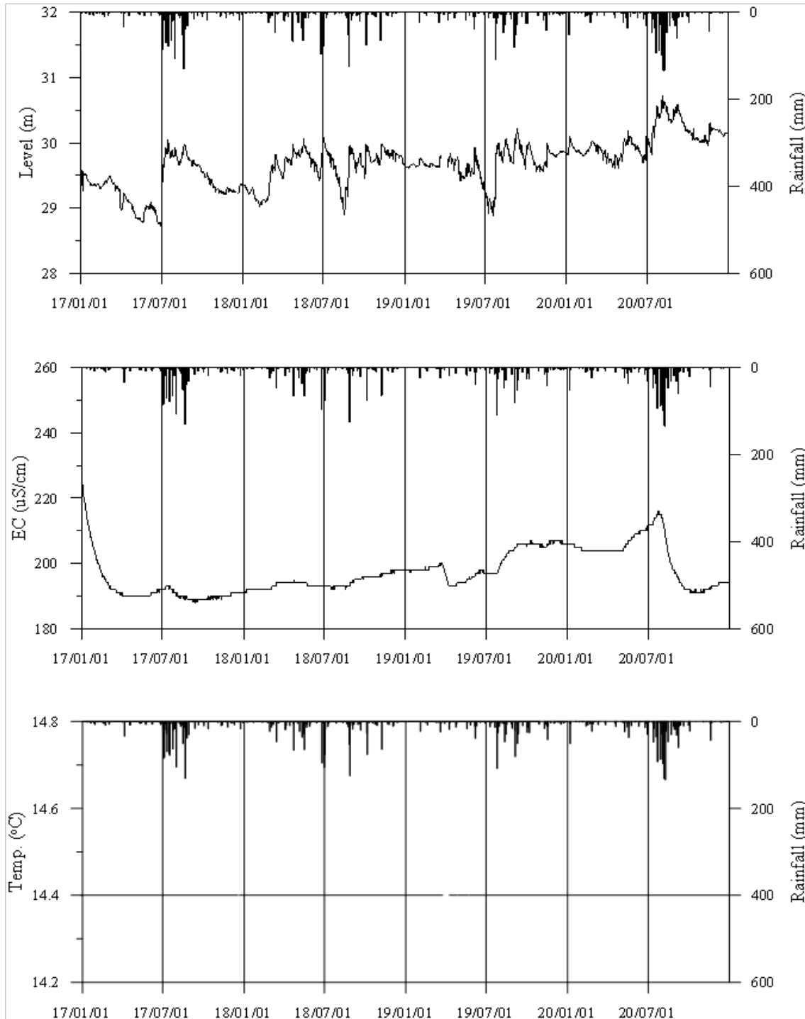
<화성3 관측공의 장기관측자료 (2017.1.1 ~ 2020.12.31)> (a)지하수위, (b)전기전도도, (c)수온
