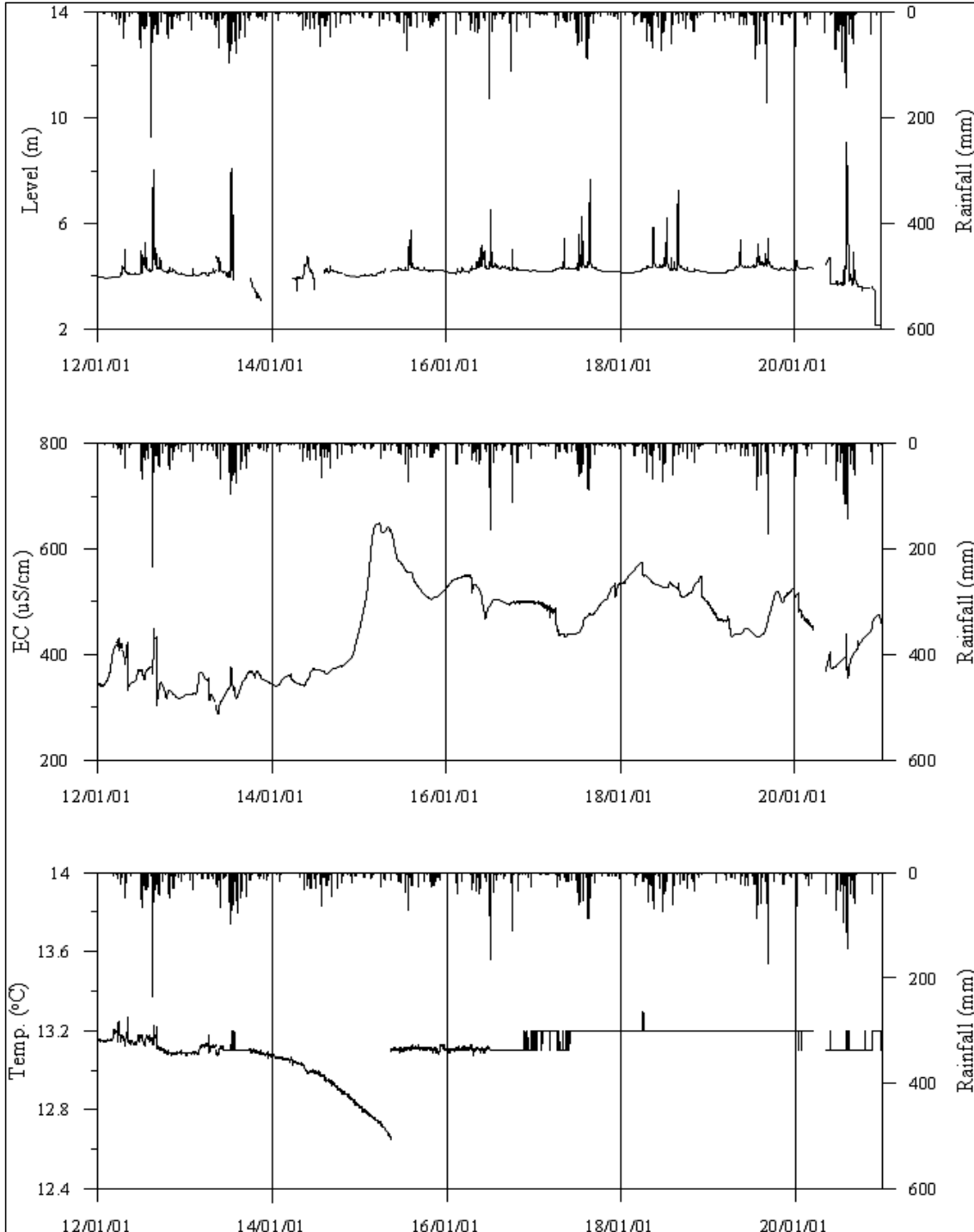
<과주1 관측공의 장기관측자료 (2012.1.1 ~ 2020.12.31)> (a)지하수위, (b)전기전도도, (c)수온
