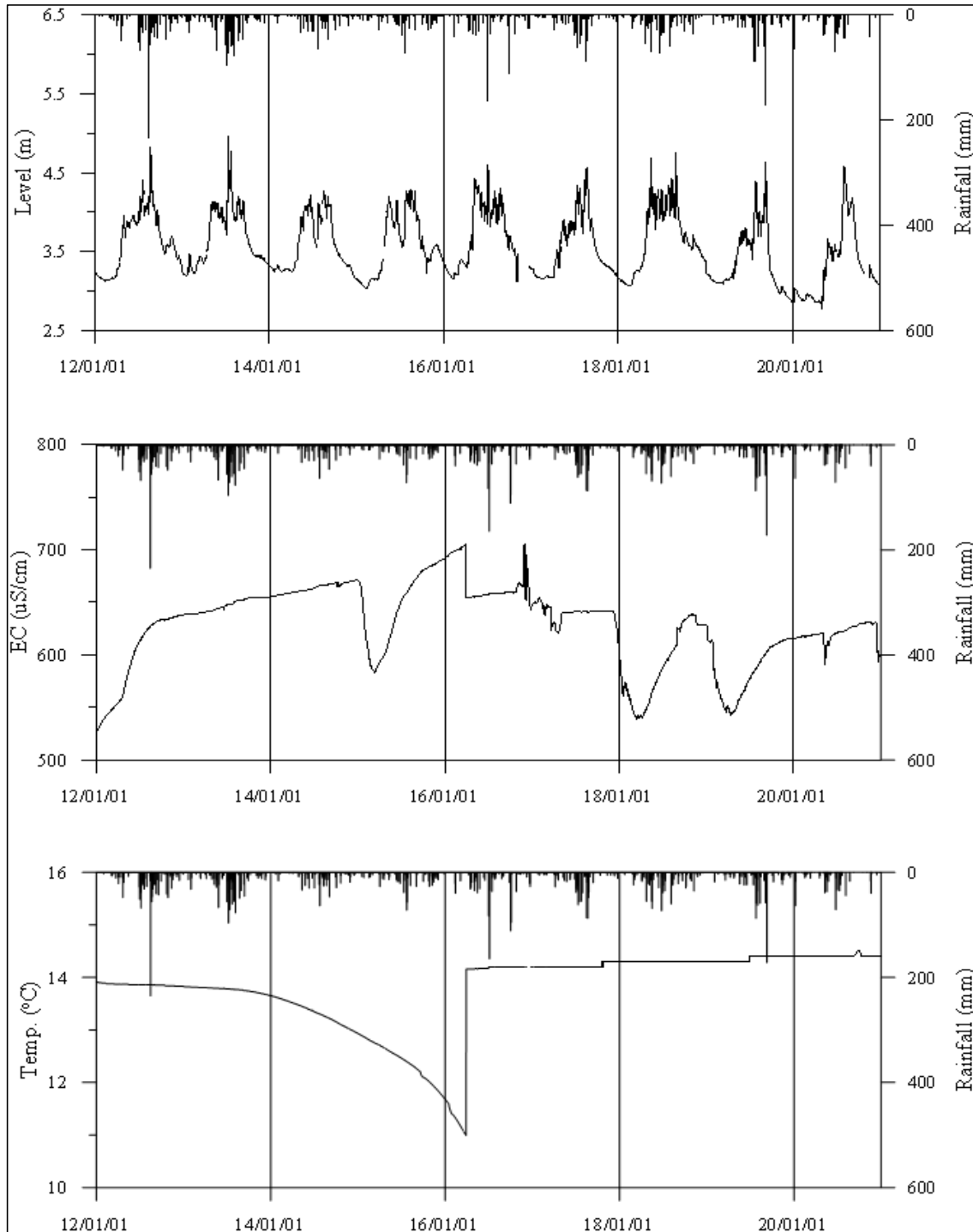
<파주2 관측공의 장기관측자료 (2012.1.1 ~ 2020.12.31)> (a)지하수위, (b)전기전도도, (c)수온
