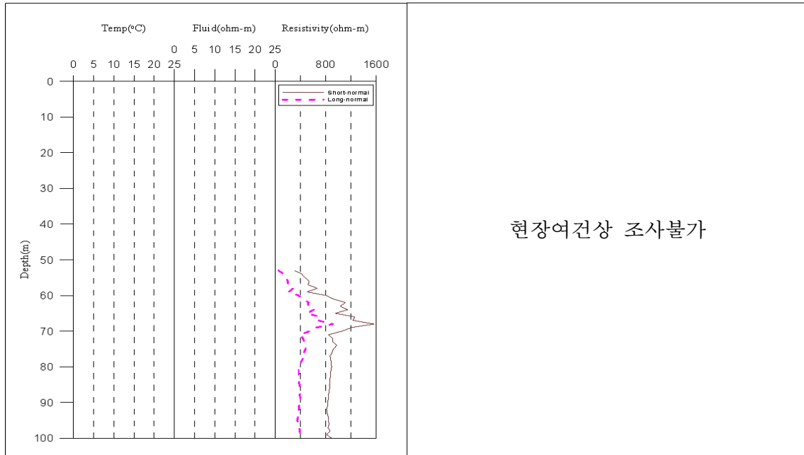
<기장1 관측공 물리검층>
