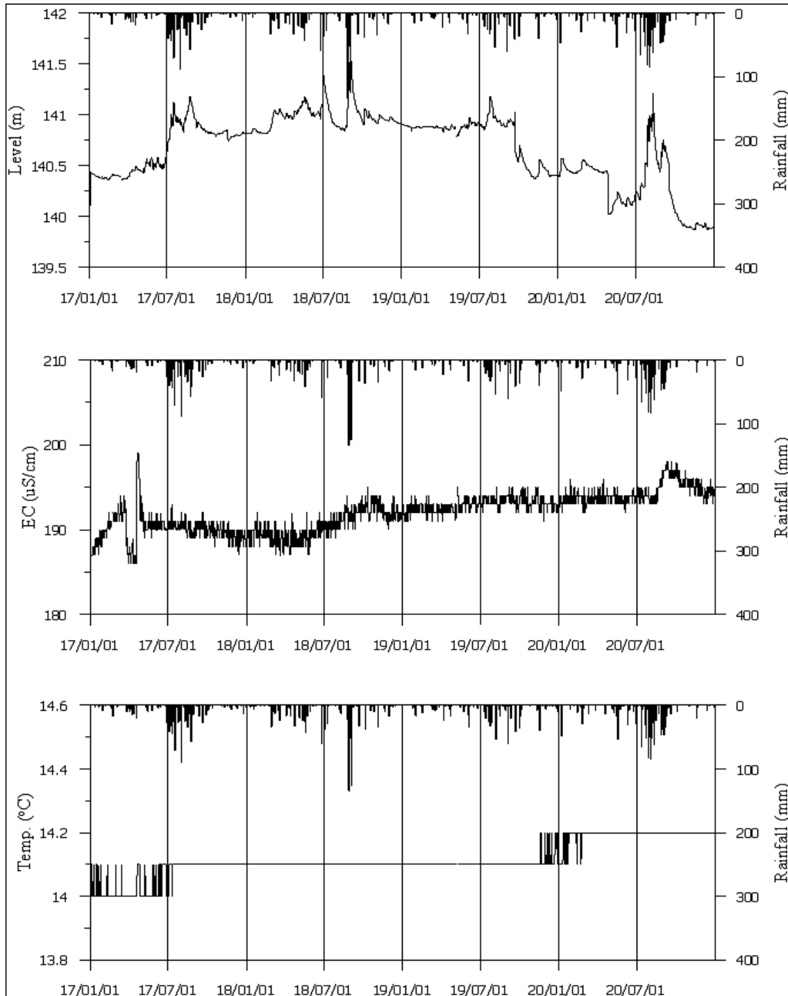
<음성5 관측공의 장기관측자료 (2017.1.1 ~ 2020.12.31)> (a)지하수위, (b)전기전도도, (c)수온
