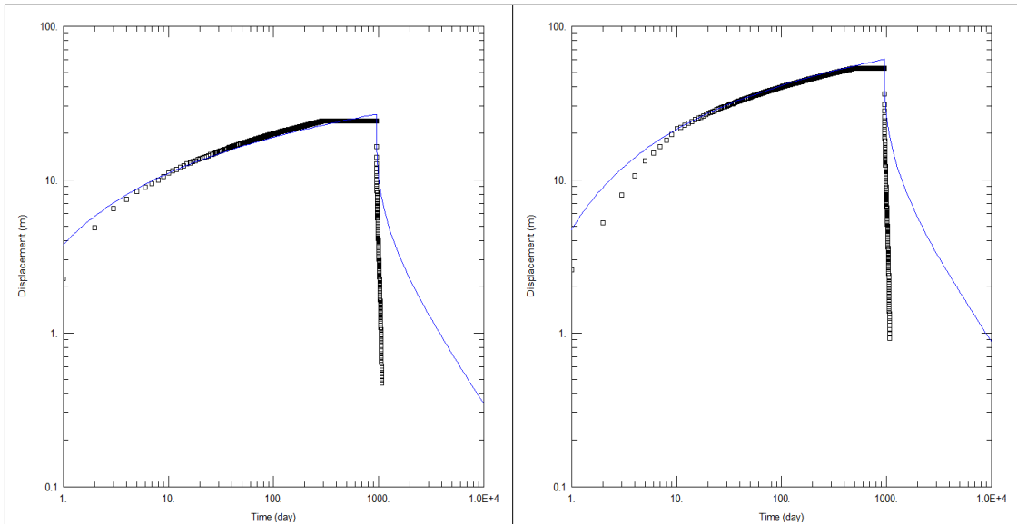
<영월3 관측공 양수시험>
