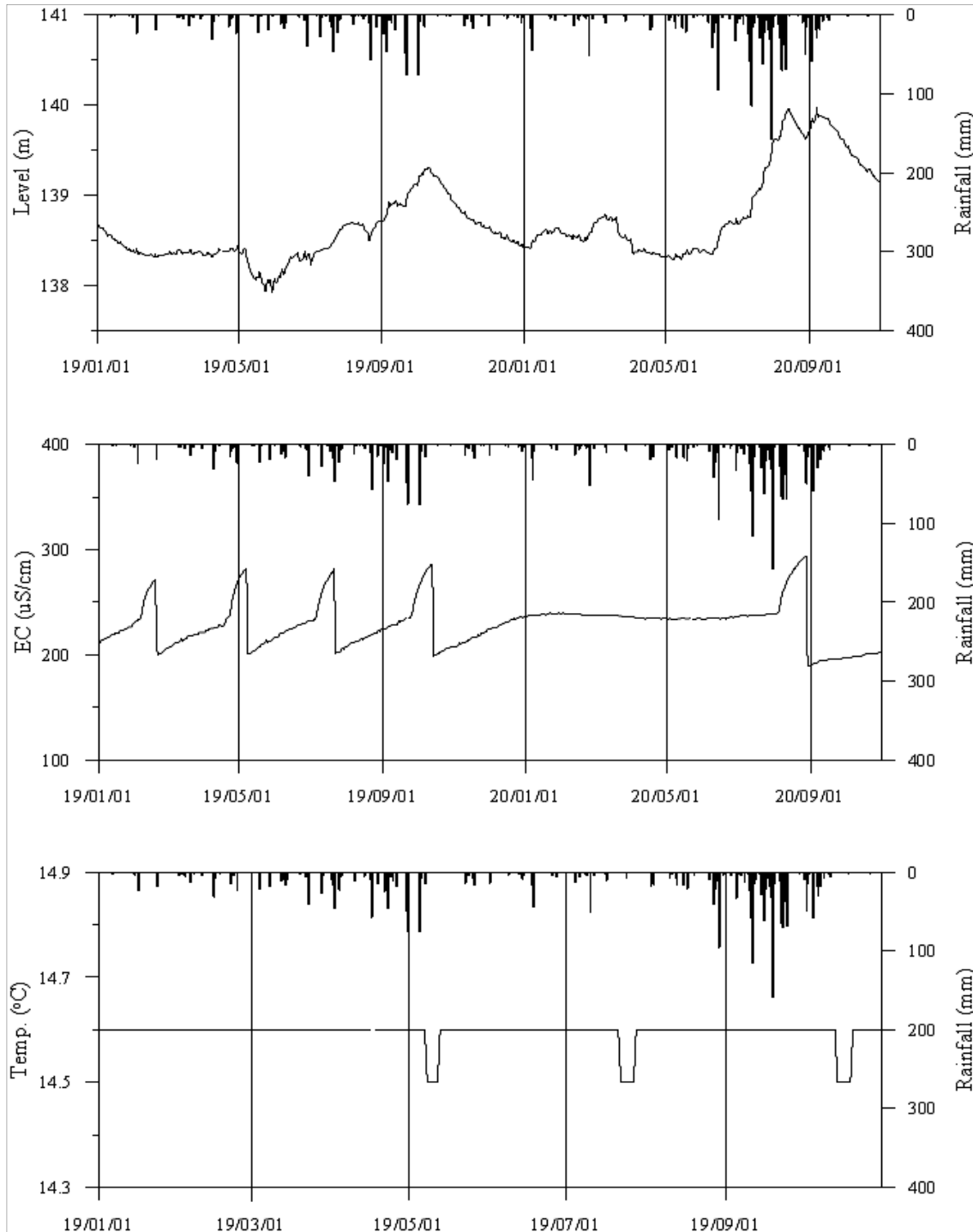
<금산4 관측공의 장기관측자료 (2019.1.1 ~ 2020.12.31)> (a)지하수위, (b)전기전도도, (c)수온
