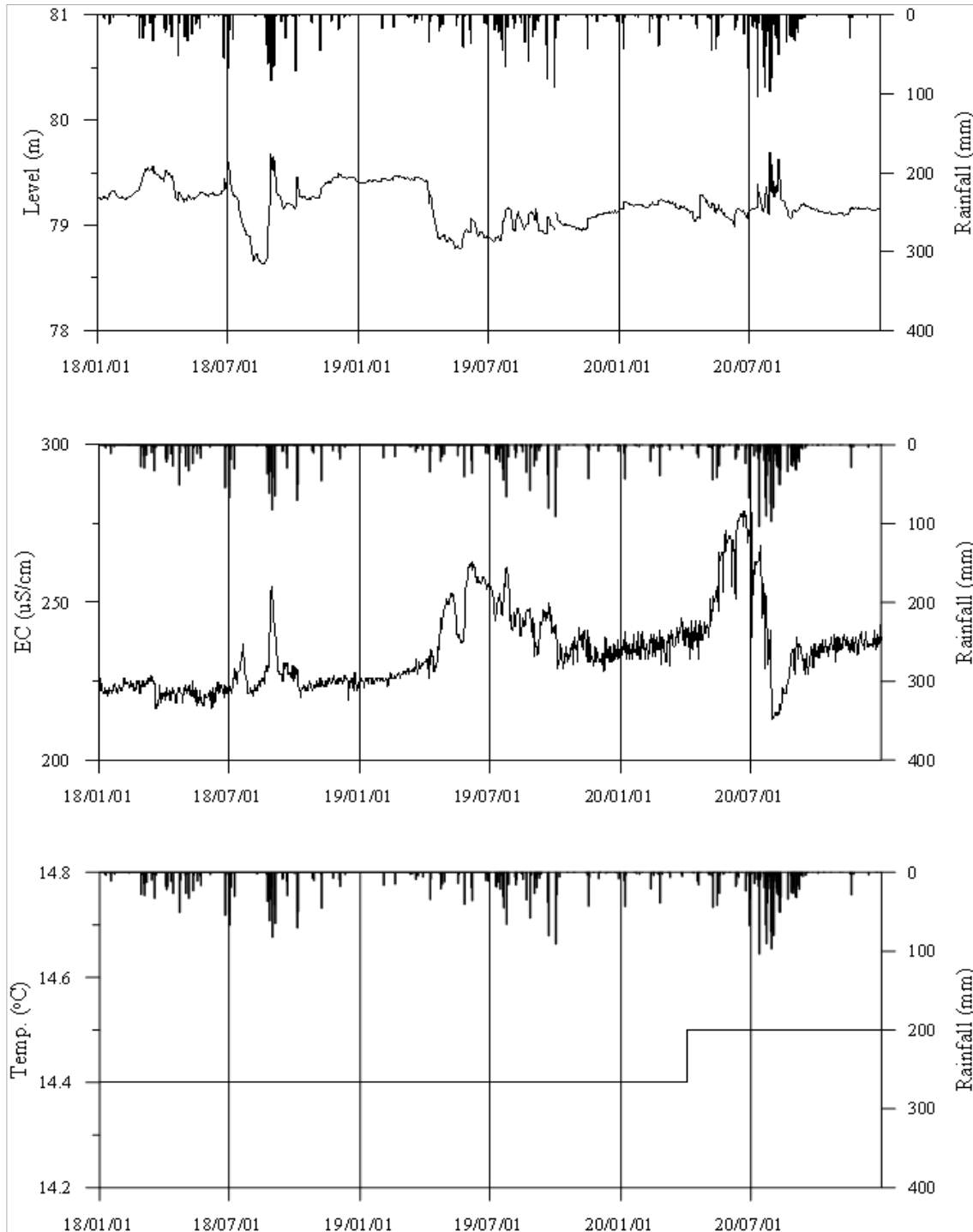
<문경4 관측공의 장기관측자료 (2018.1.1 ~ 2020.12.31.)> (a)지하수위, (b)전기전도도, (c)수온
