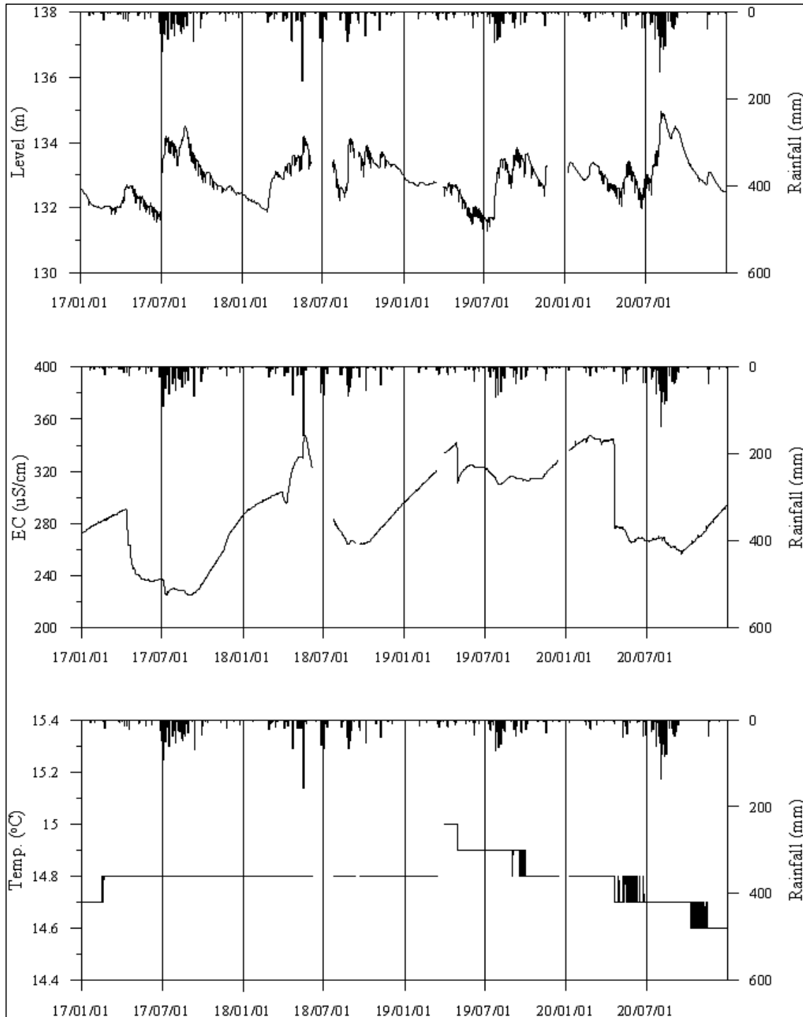
<홍천3 관측공의 장기관측자료 (2017.1.1 ~ 2020.12.31)> (a)지하수위, (b)전기전도도, (c)수온
