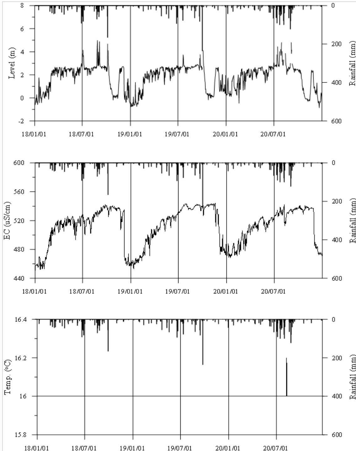
<의령2 관측공의 장기관측자료 (2018.1.1 ~ 2020.12.31)> (a)지하수위, (b)전기전도도, (c)수온
