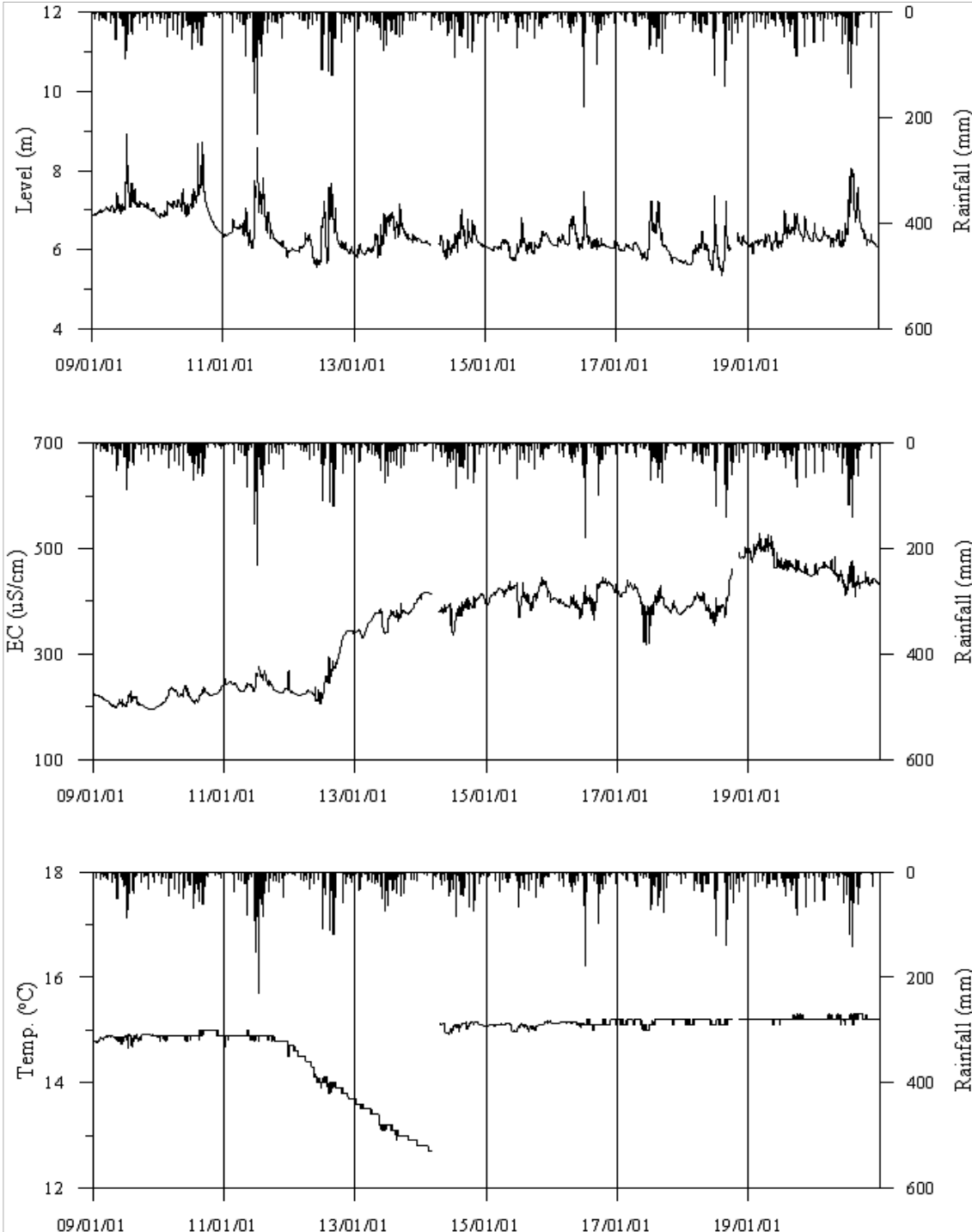
<공주1 관측공의 장기관측자료 (2009.1.1 ~ 2020.12.31)> (a)지하수위, (b)전기전도도, (c)수온
