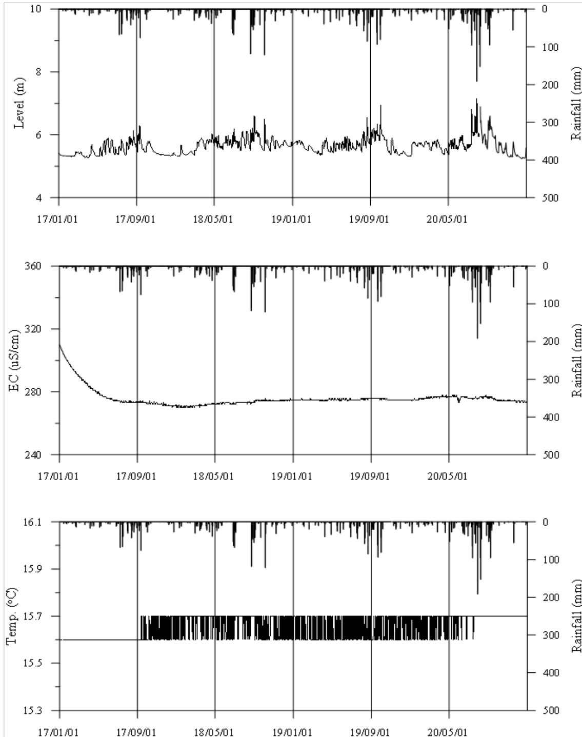
<영광3 관측공의 장기관측자료 (2017.1.1 ~ 2020.12.31)> (a)지하수위, (b)전기전도도, (c)수온
