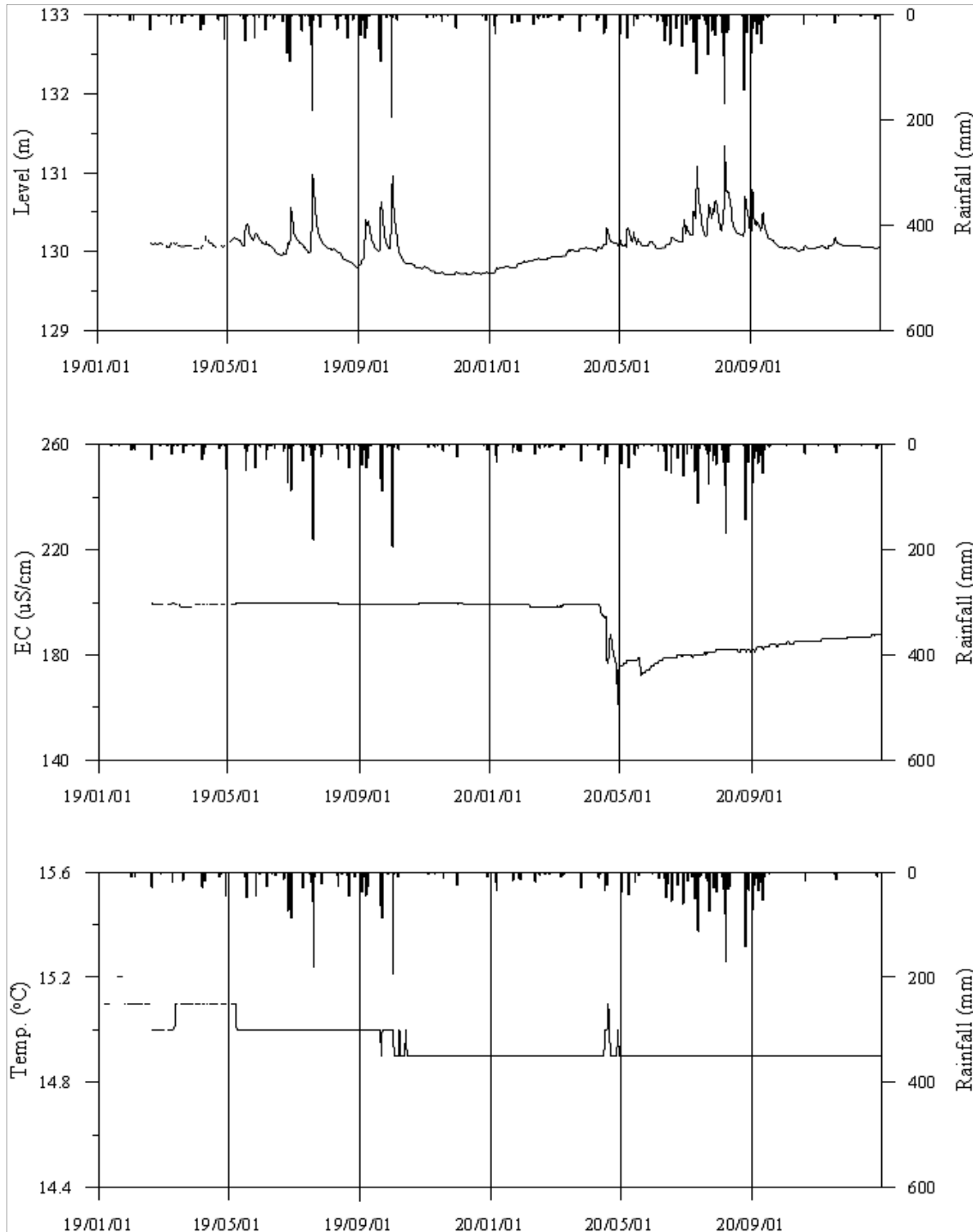
<순천7 관측공의 장기관측자료 (2019.1.1~2020.12.31)> (a)지하수위, (b)전기전도도, (c)수온
