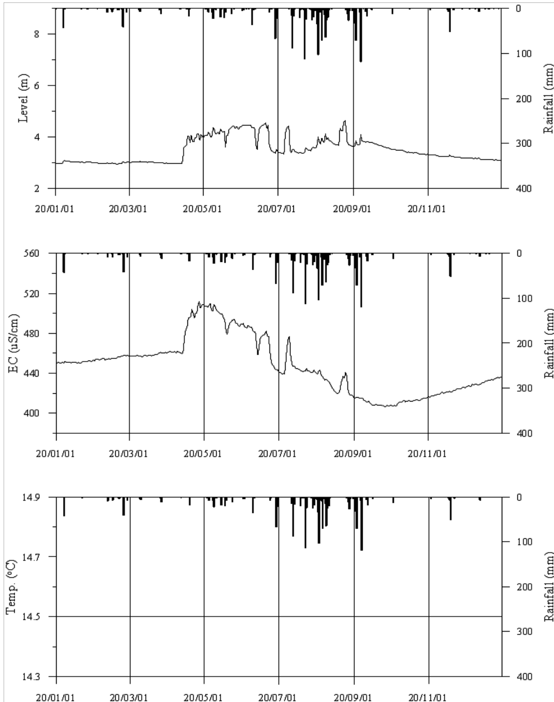
<당진2 관측공의 장기관측자료 (2020.1.1 ~ 2020.12.31)> (a)지하수위, (b)전기전도도, (c)수온
