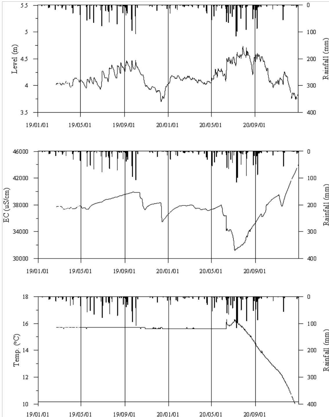
<함평7 관측공의 장기관측자료 (2019.1.1~2020.12.31)> (a)지하수위, (b)전기전도도, (c)수온
