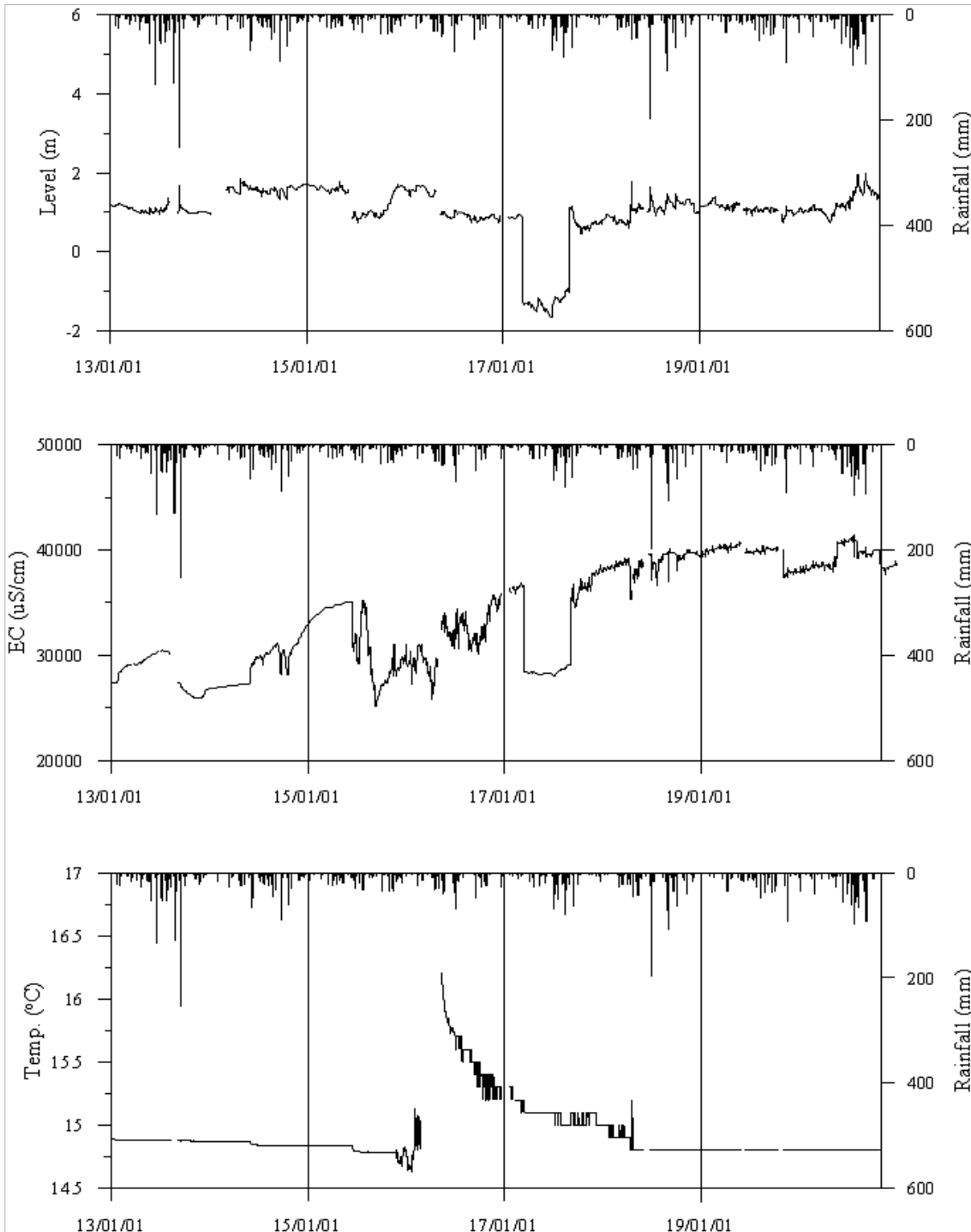
<보령1 관측공의 장기관측자료 (2013.1.1 ~ 2020.12.31)> (a)지하수위, (b)전기전도도, (c)수온
