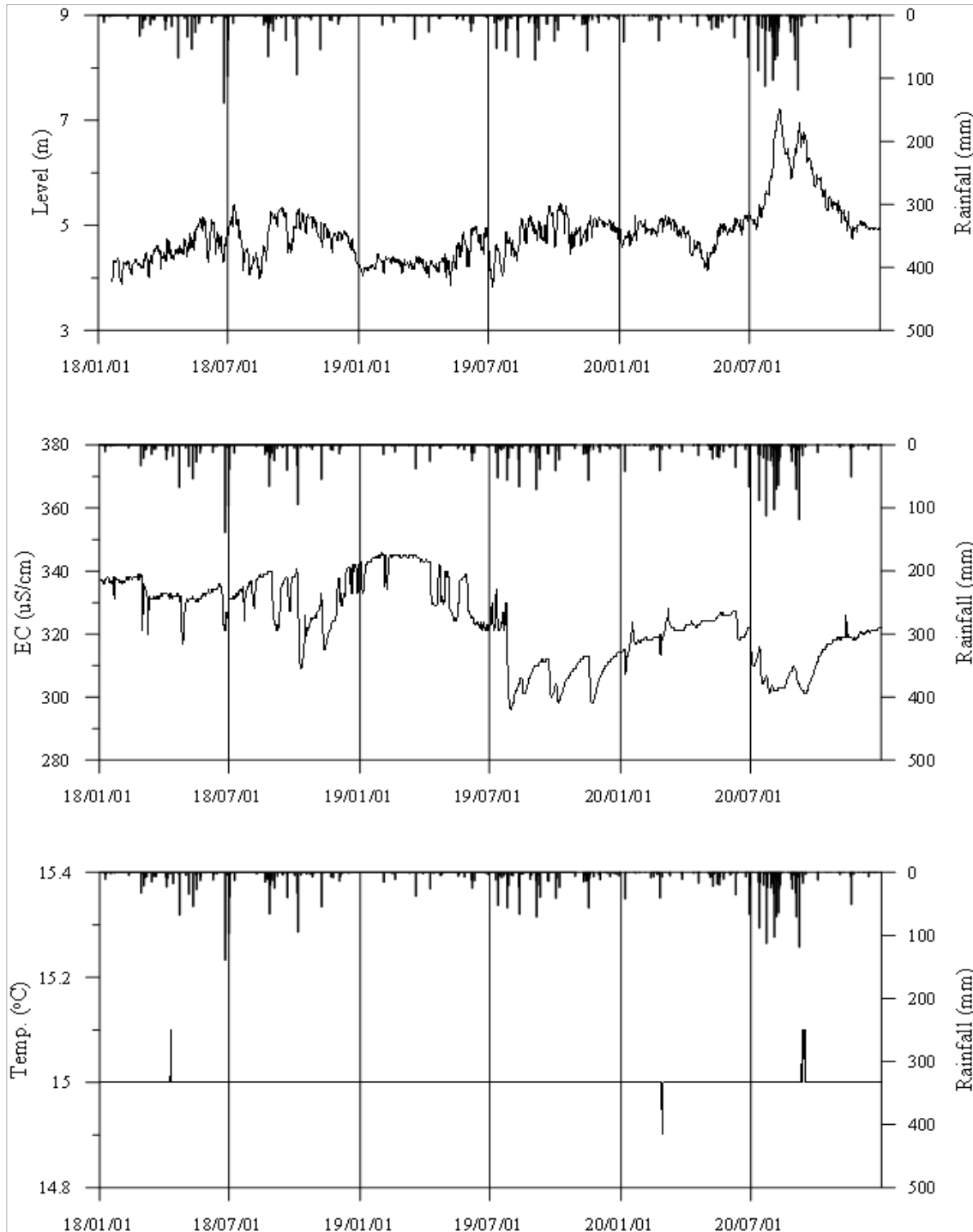
<예산3 관측공의 장기관측자료 (2018.1.1 ~ 2020.12.31)> (a)지하수위, (b)전기전도도, (c)수온
