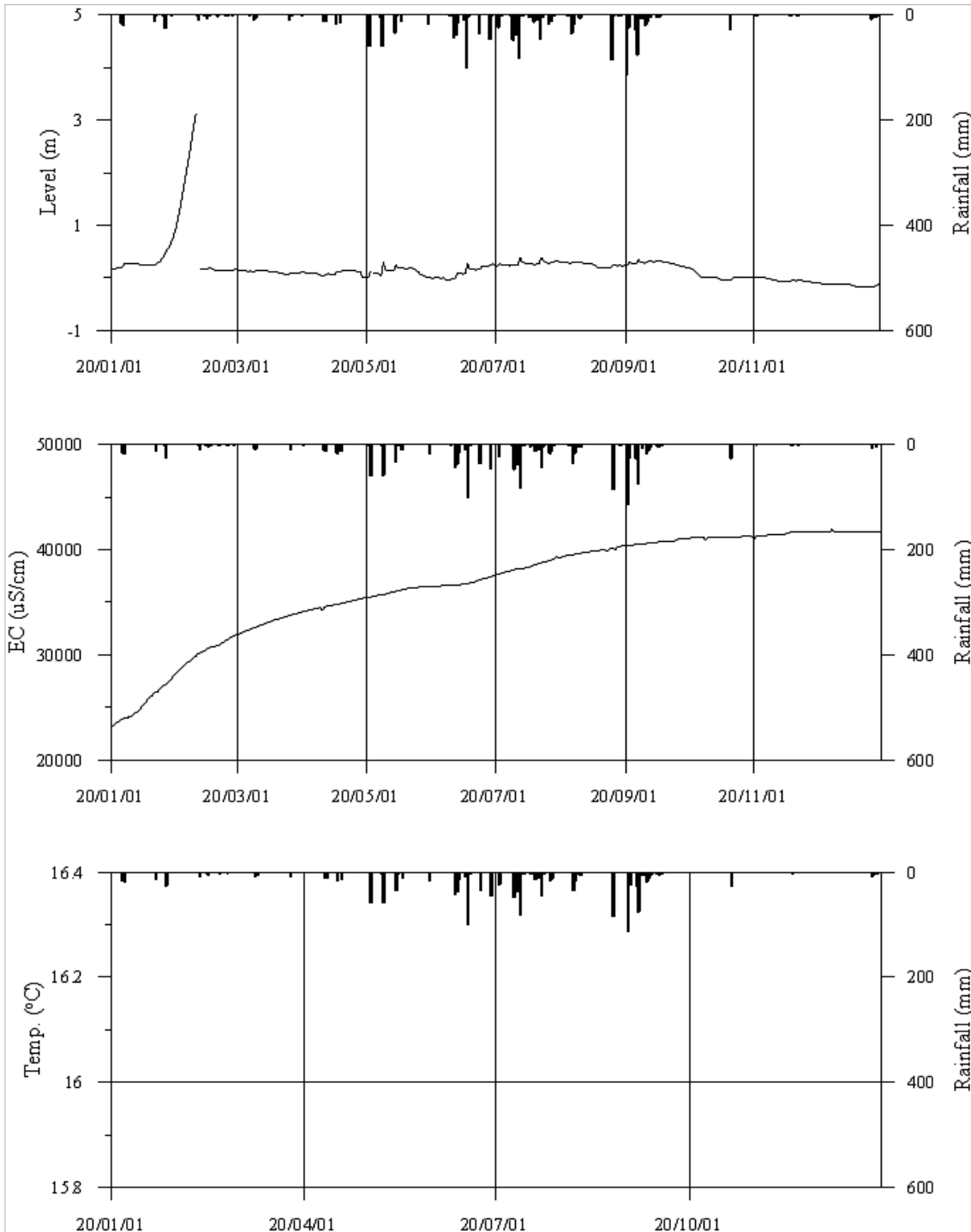
<해남12 관측공의 장기관측자료 (2020.1.1~2020.12.31)> (a)지하수위, (b)전기전도도, (c)수온
