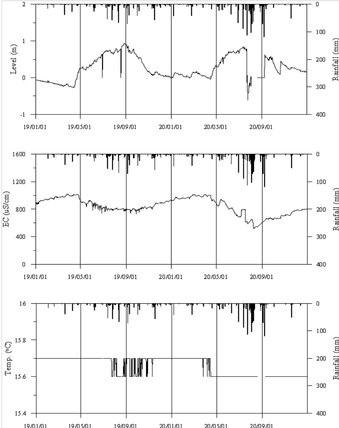
<서산1 관측공의 장기관측자료 (2019.1.1 ~ 2020.12.31)> (a)지하수위, (b)전기전도도, (c)수온
