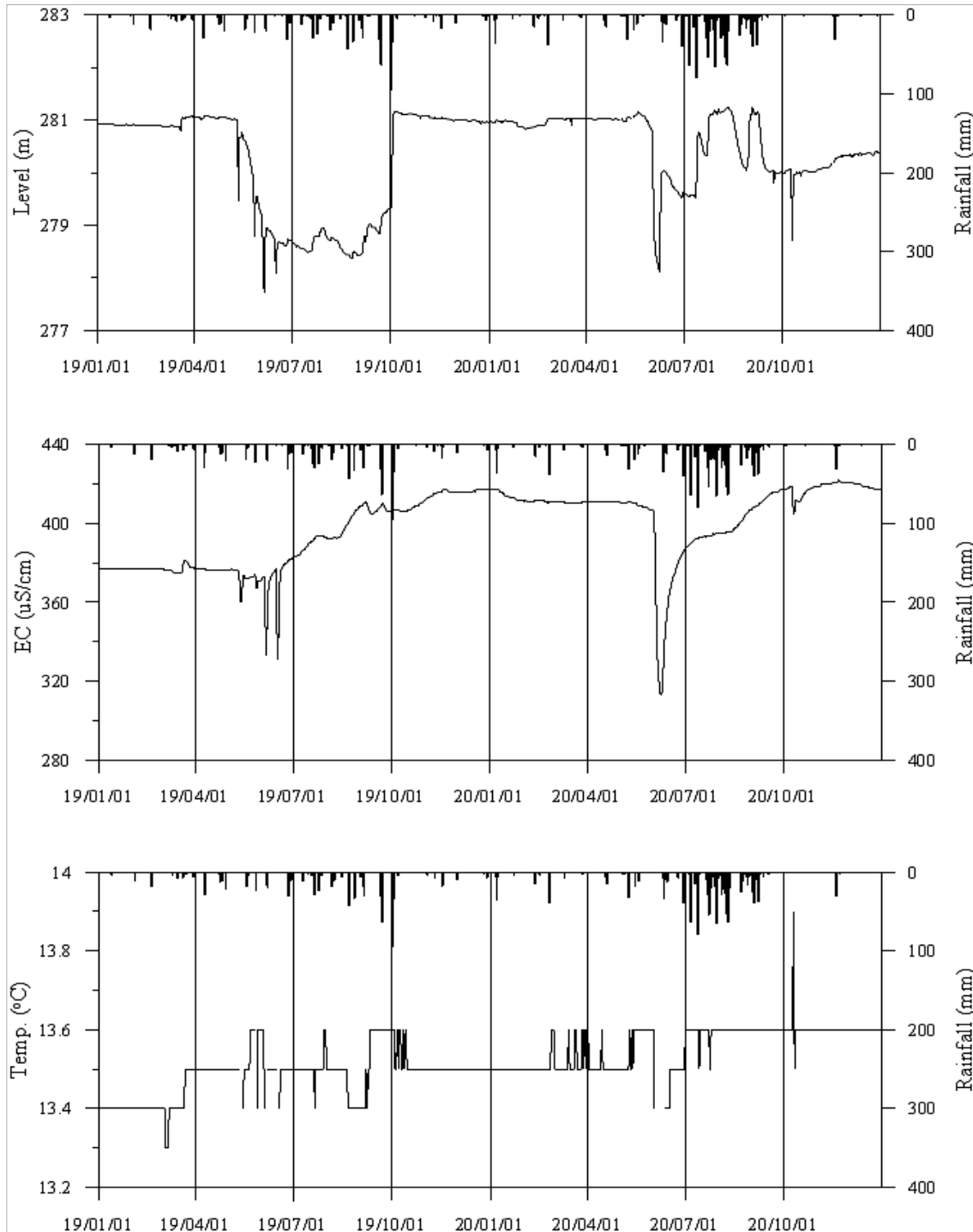
<안동6 관측공의 장기관측자료 (2019.1.1 ~ 2020.12.31)> (a)지하수위, (b)전기전도도, (c)수온
