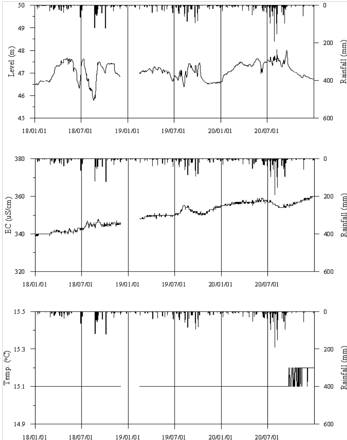
<장성5 관측공의 장기관측자료 (2018.1.1 ~ 2020.12.31)> (a)지하수위, (b)전기전도도, (c)수온
