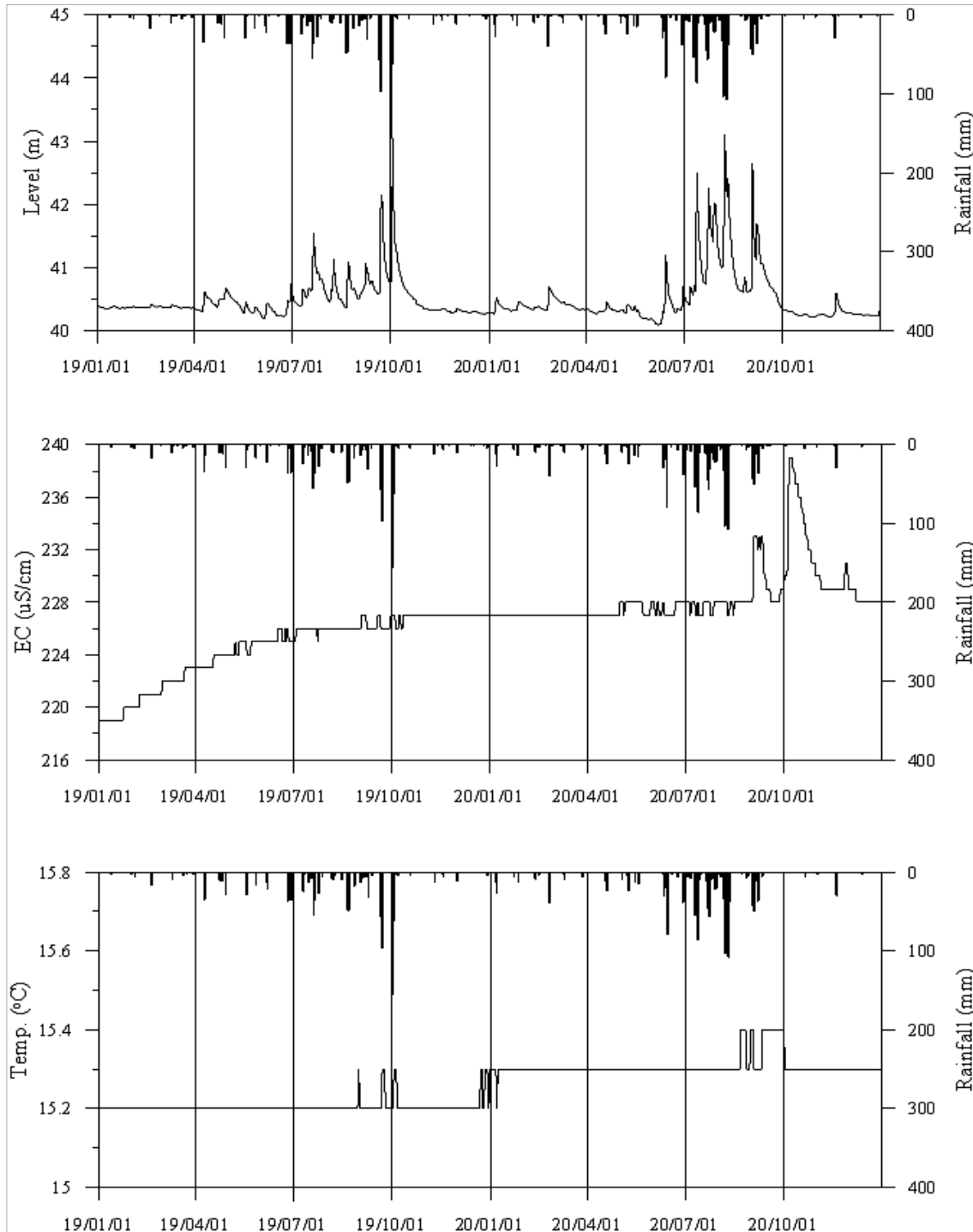
<김천3 관측공의 장기관측자료 (2019.1.1 ~ 2020.12.31.)> (a)지하수위, (b)전기전도도, (c)수온
