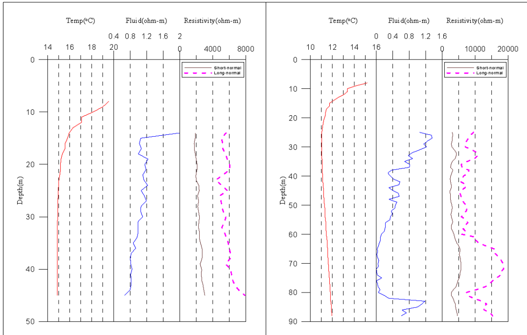
<영월3 관측공 물리검층>
