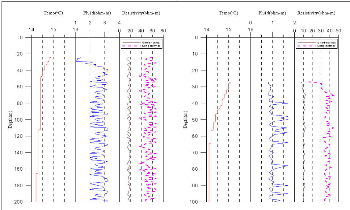
<예천2 관측공 물리검층>
