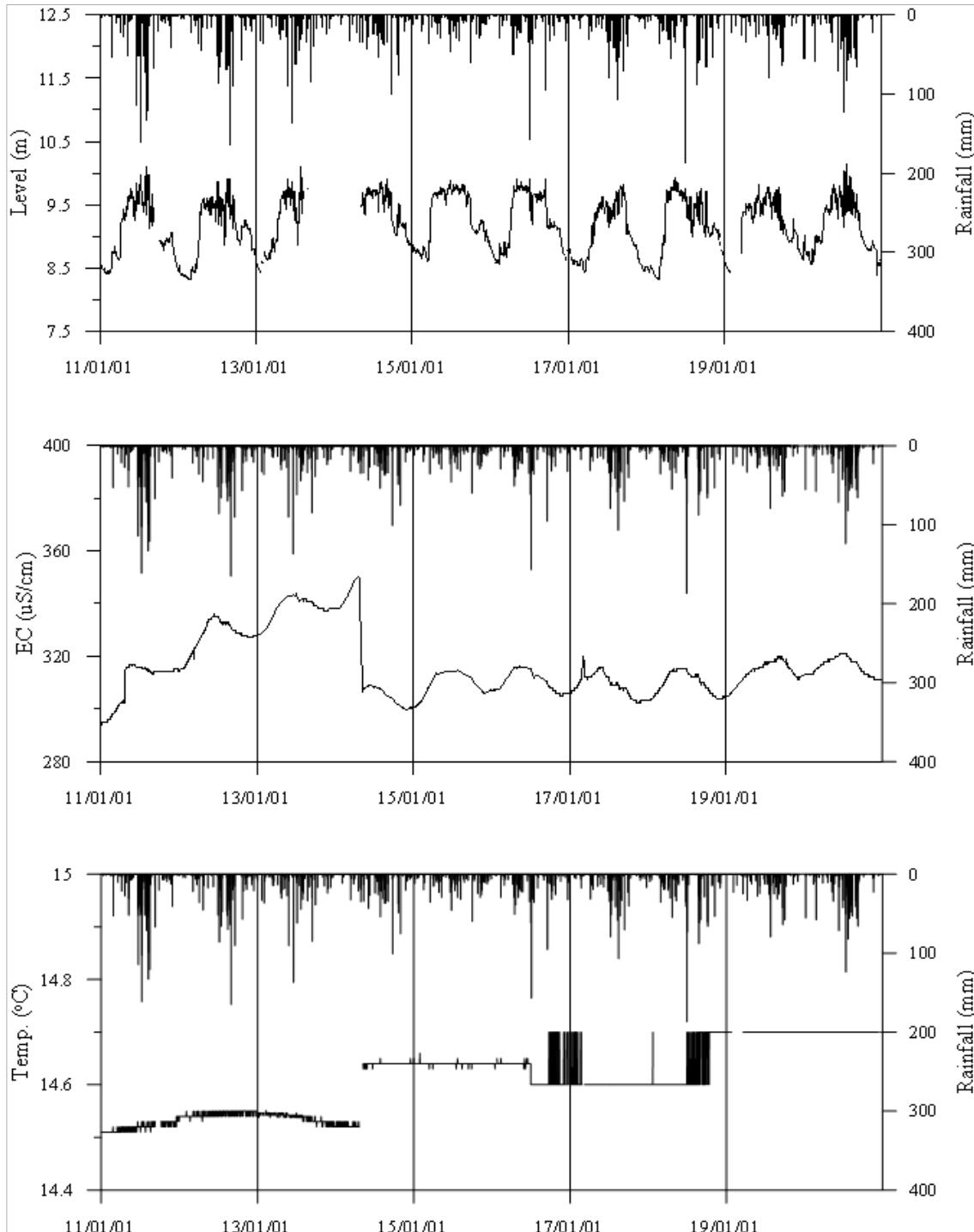
<부여1 관측공의 장기관측자료 (2011.1.1 ~ 2020.12.31)> (a)지하수위, (b)전기전도도, (c)수온
