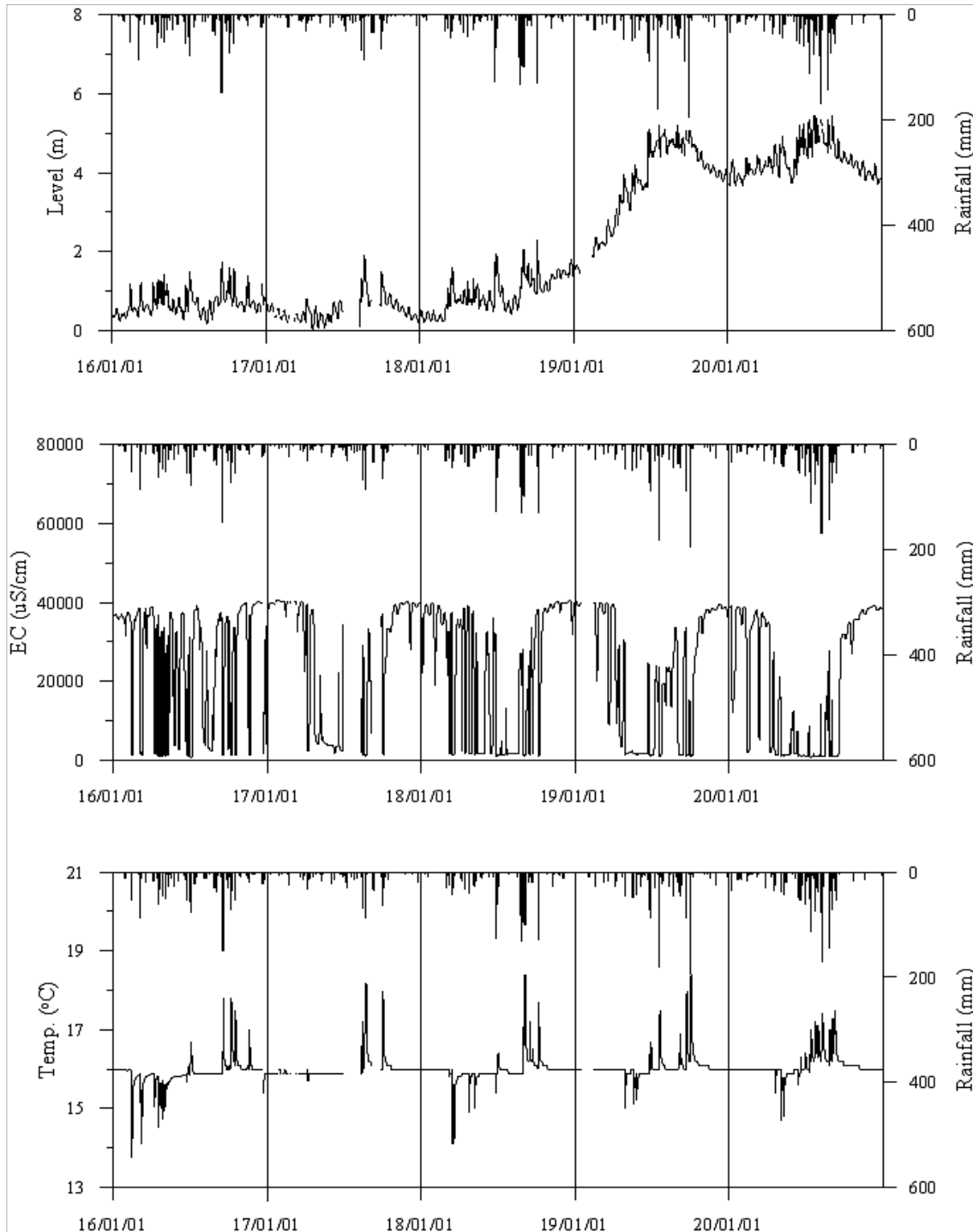
<순천4 관측공의 장기관측자료 (2016.1.1~2020.12.31)> (a)지하수위, (b)전기전도도, (c)수온
