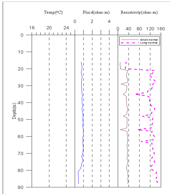
<봉화7 관측공 물리검층>
