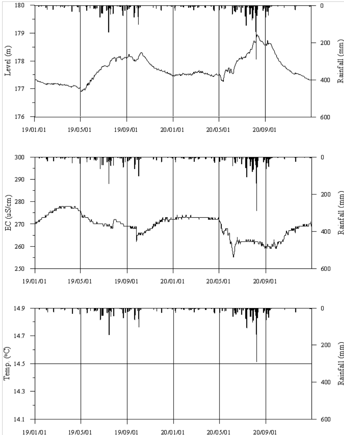
<남원5 관측공의 장기관측자료 (2019.1.1 ~ 2020.12.31)> (a)지하수위, (b)전기전도도, (c)수온
