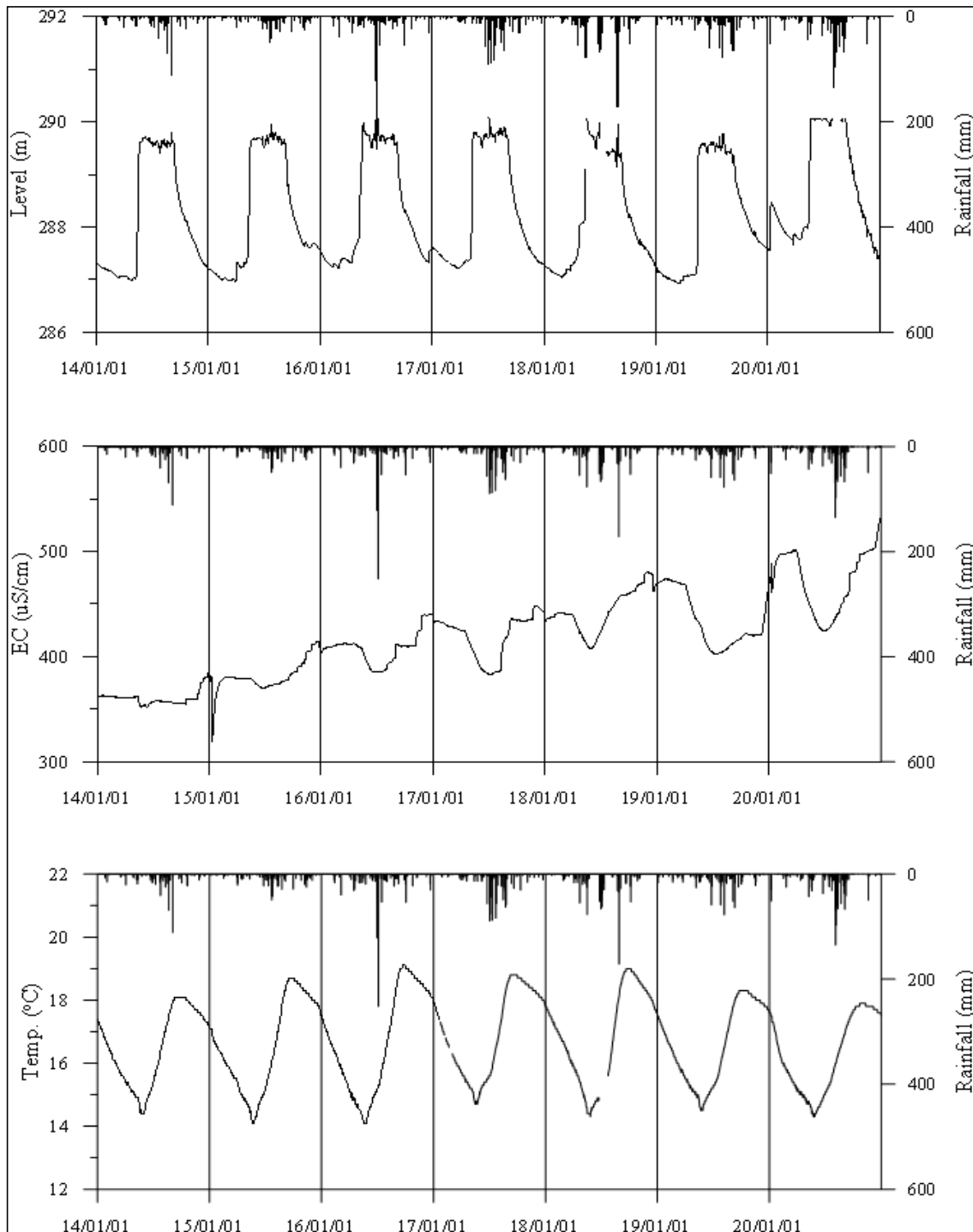
<인제3 관측공의 장기관측자료 (2014.1.1 ~ 2020.12.31)> (a)지하수위, (b)전기전도도, (c)수온
