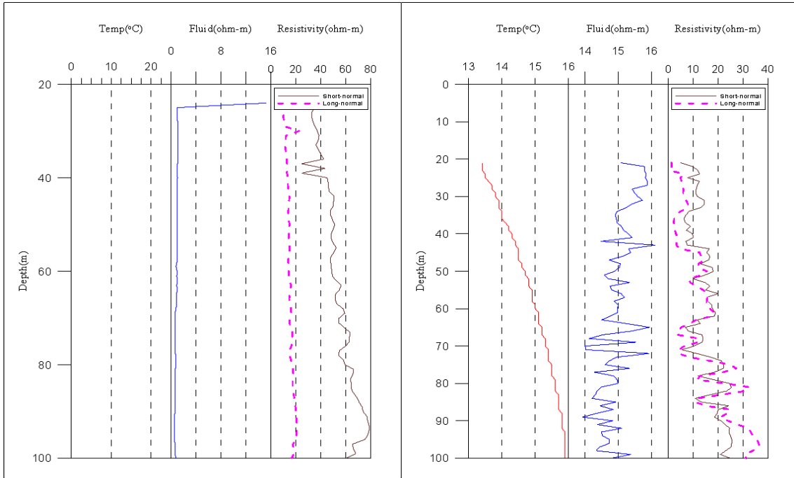
<안동4(신) 관측공 물리검층>
