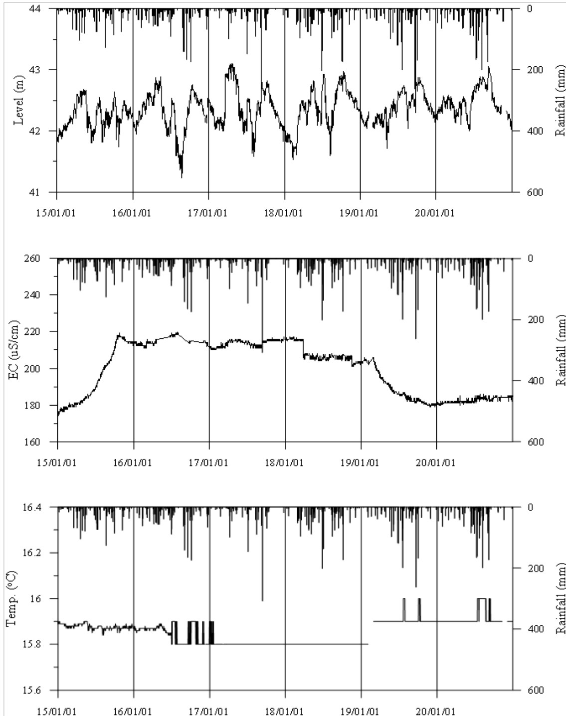
<거제3 관측공의 장기관측자료 (2015.1.1 ~ 2020.12.31)> (a)지하수위, (b)전기전도도, (c)수온
