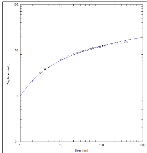
<파주3 관측공 양수시험>
