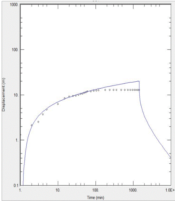
<영양1 관측공 양수시험>
