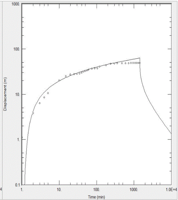
<영양2 관측공 양수시험>
