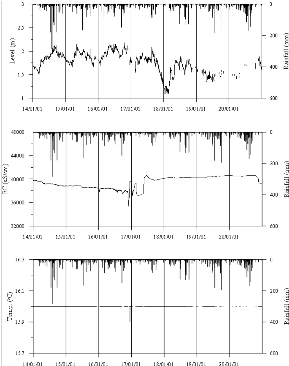
<순천1 관측공의 장기관측자료 (2014.1.1~2020.12.31)> (a)지하수위, (b)전기전도도, (c)수온
