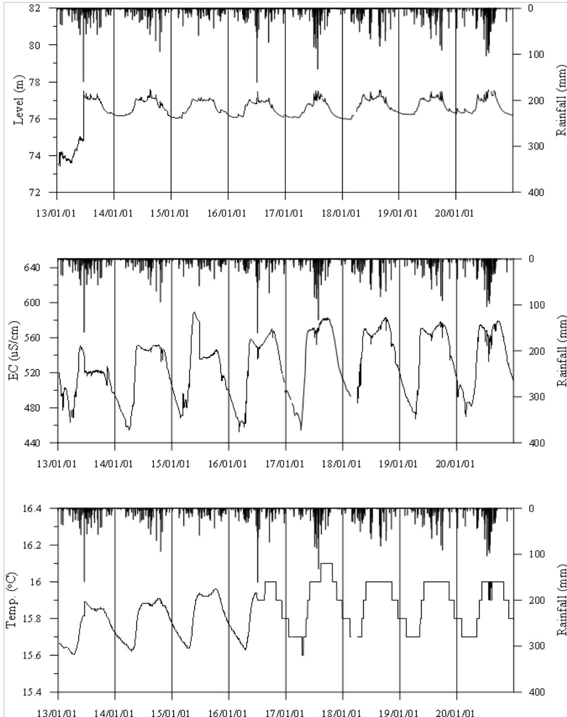
<문경1 관측공의 장기관측자료 (2013.1.1 ~ 2020.12.31)> (a)지하수위, (b)전기전도도, (c)수온
