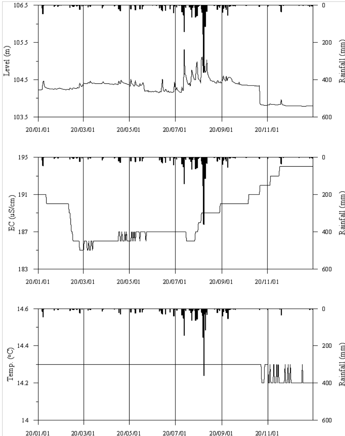
<순창6 관측공의 장기관측자료 (2020.1.1 ~ 2020.12.31)> (a)지하수위, (b)전기전도도, (c)수온
