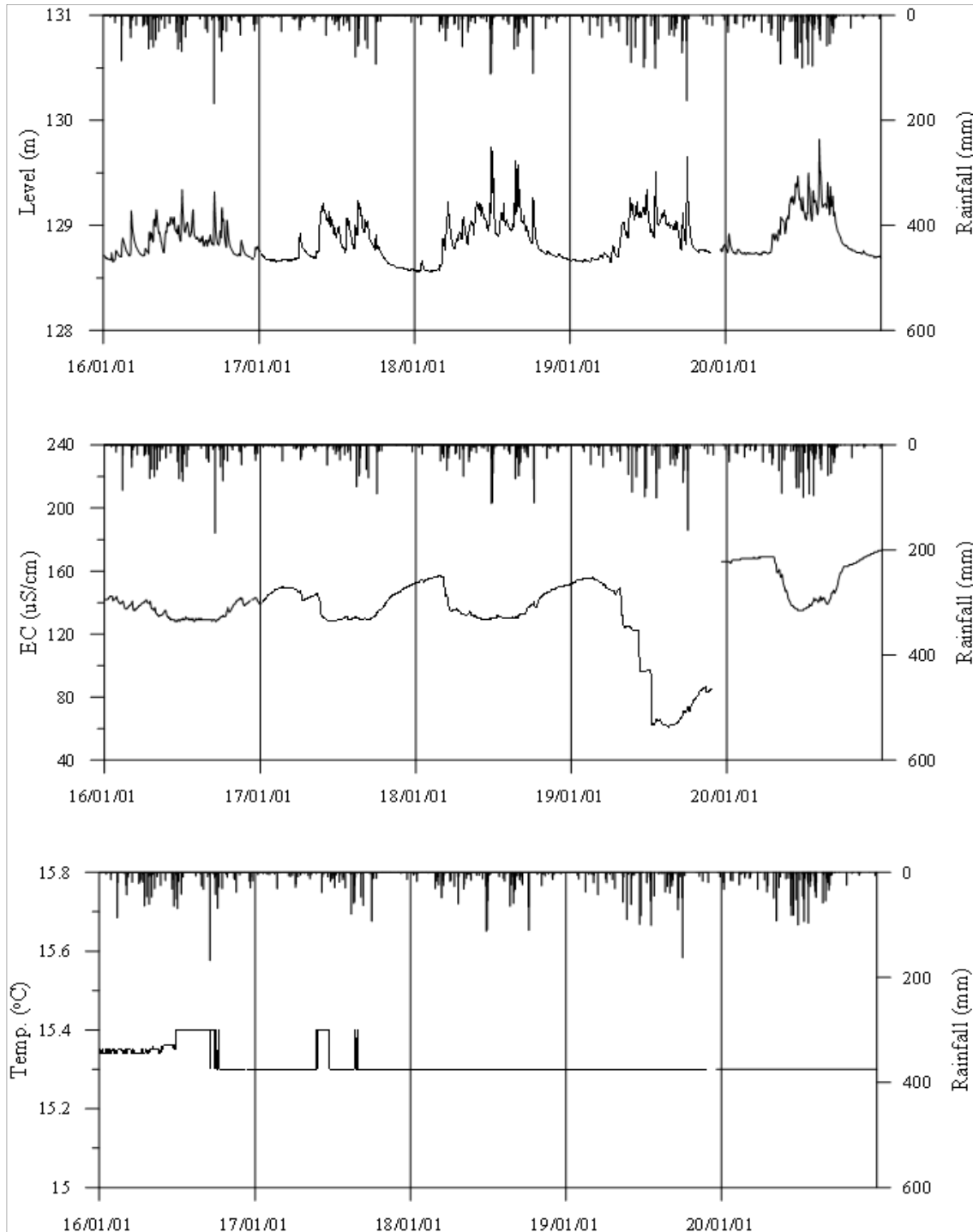
<보성5 관측공의 장기관측자료 (2016.1.1 ~ 2020.12.31)> (a)지하수위, (b)전기전도도, (c)수온
