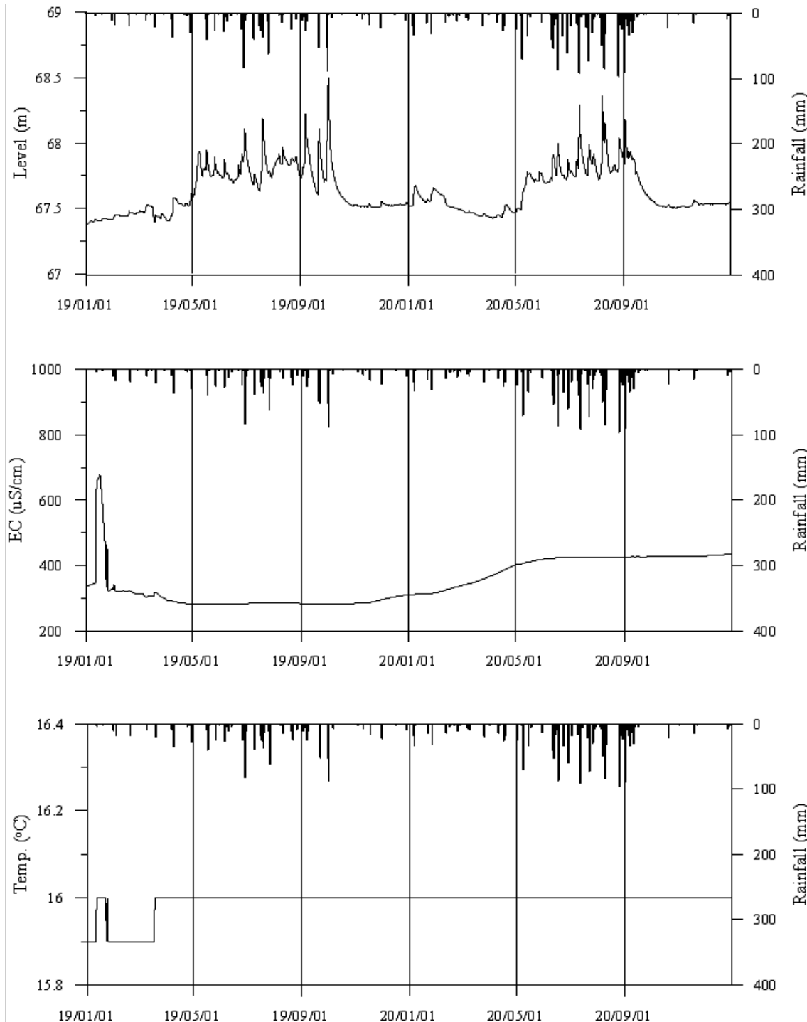
<화순6 관측공의 장기관측자료 (2019.1.1 ~ 2020.12.31)> (a)지하수위, (b)전기전도도, (c)수온
