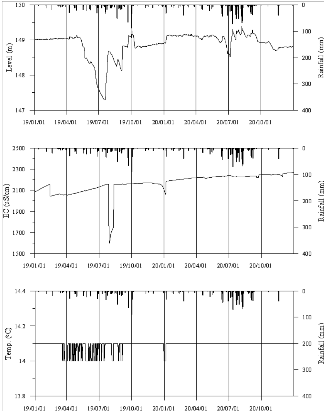
<의성8 관측공의 장기관측자료 (2019.1.1 ~ 2020.12.31.)> (a)지하수위, (b)전기전도도, (c)수온
