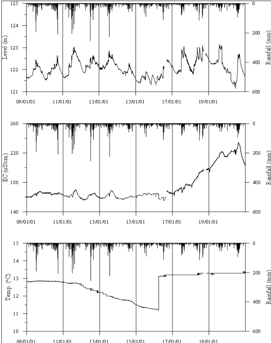
<횡성1 관측공의 장기관측자료 (2009.1.1 ~ 2020.12.31)> (a)지하수위, (b)전기전도도, (c)수온
