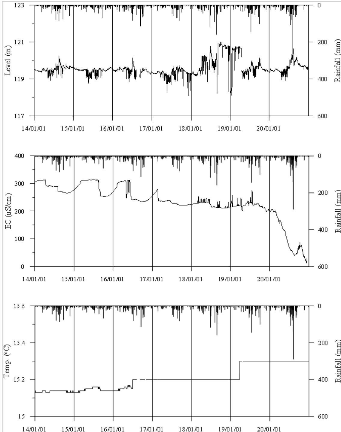
<남원3 관측공의 장기관측자료 (2014.1.1 ~ 2020.12.31)> (a)지하수위, (b)전기전도도, (c)수온
