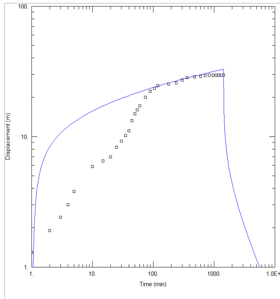
<영주4 관측공 양수시험>
