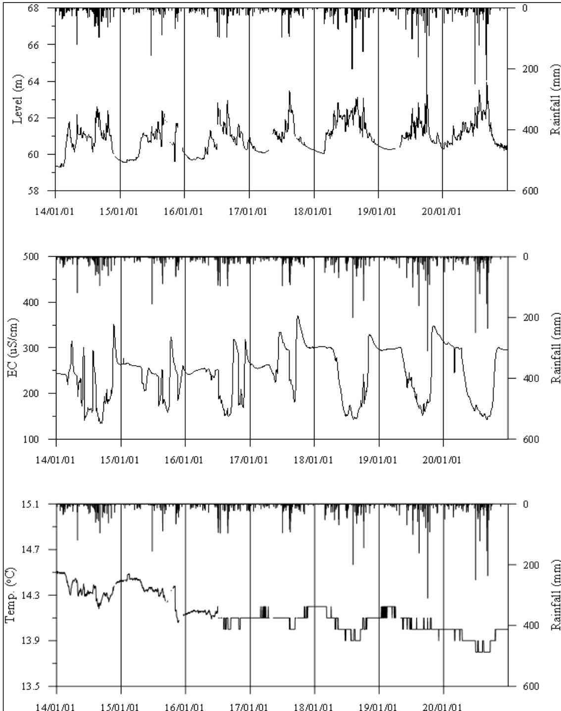
<강릉1 관측공의 장기관측자료 (2014.1.1 ~ 2020.12.31)> (a)지하수위, (b)전기전도도, (c)수온
