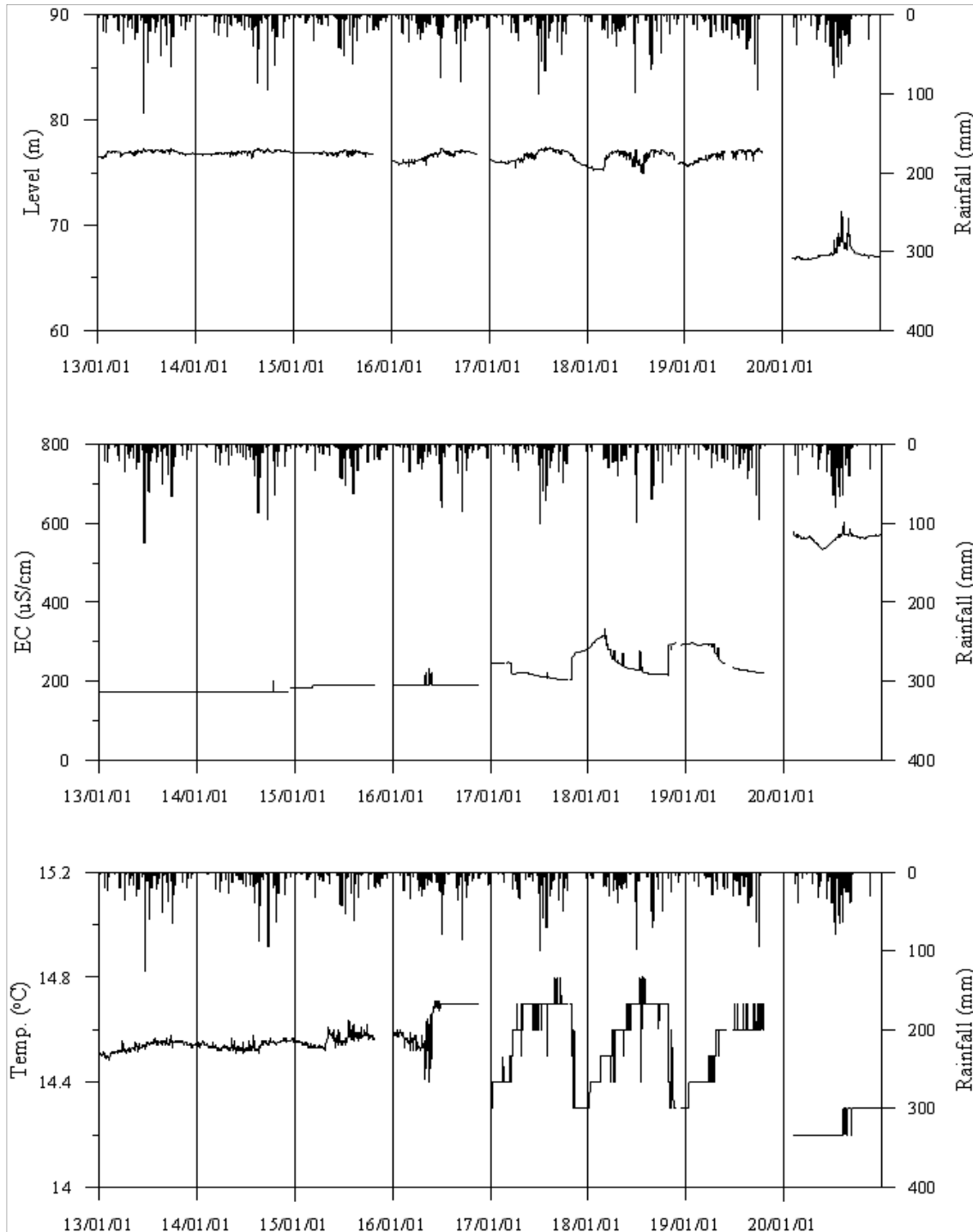
<안동4(구) 관측공의 장기관측자료 (2013.1.1 ~ 2020.12.31)> (a)지하수위, (b)전기전도도, (c)수온
