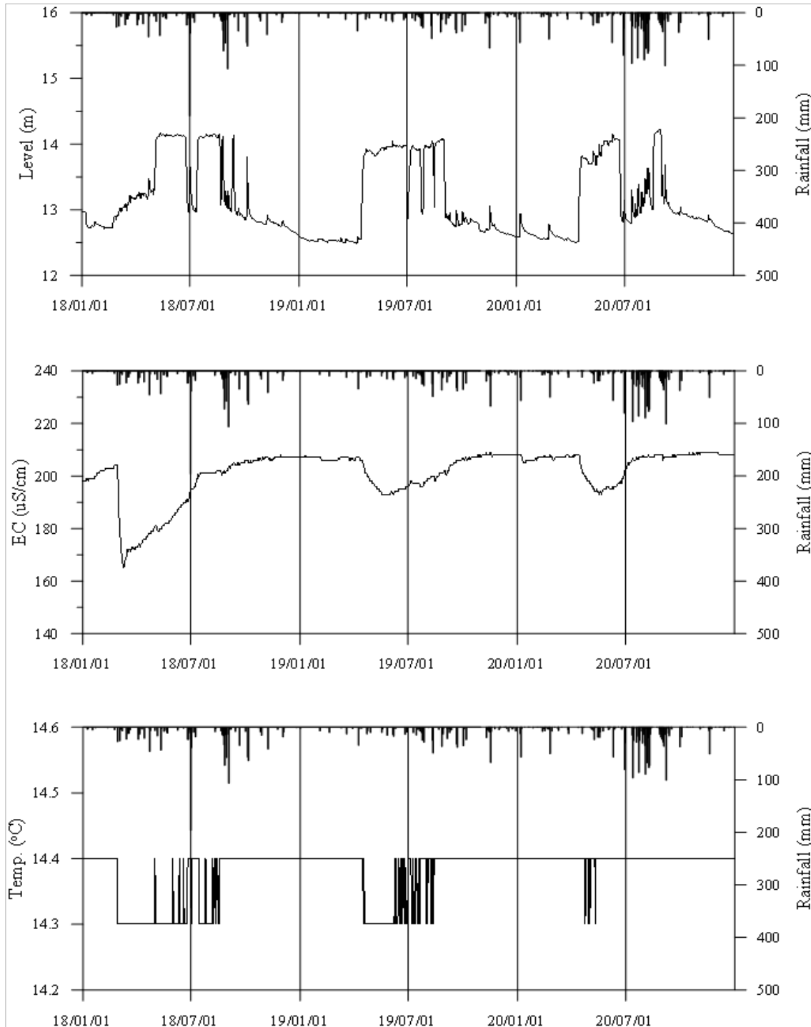
<홍성4 관측공의 장기관측자료 (2018.1.1 ~ 2020.12.31)> (a)지하수위, (b)전기전도도, (c)수온
