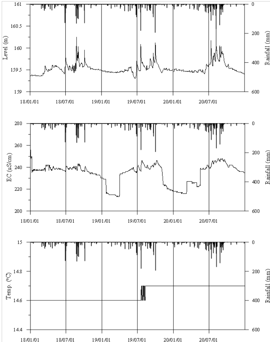
<순천5 관측공의 장기관측자료 (2018.1.1~2020.12.31)> (a)지하수위, (b)전기전도도, (c)수온
