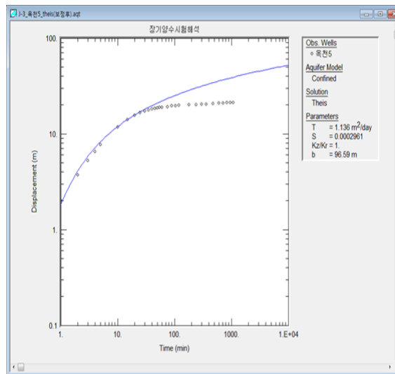
<옥천5 관측공 양수시험>
