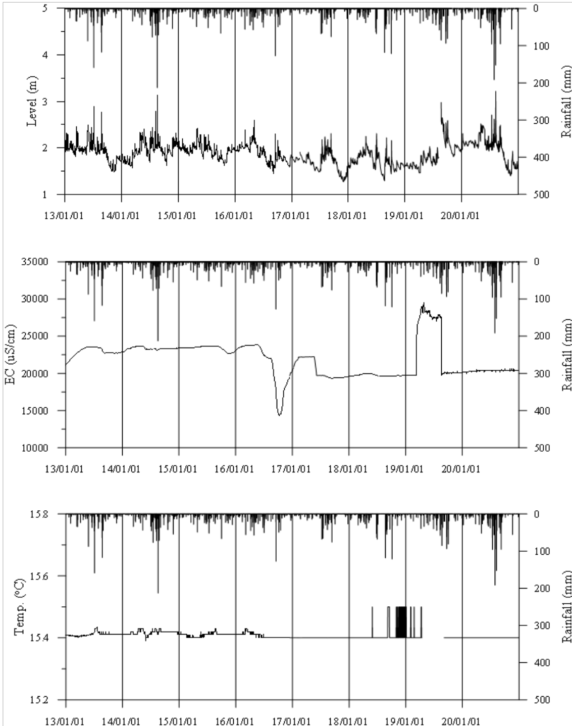
<영광1 관측공의 장기관측자료 (2013.1.1 ~ 2020.12.31)> (a)지하수위, (b)전기전도도, (c)수온
