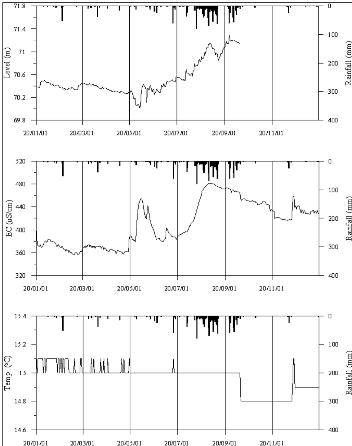
<청주4 관측공의 장기관측자료 (2020.1.1 ~ 2020.12.31)> (a)지하수위, (b)전기전도도, (c)수온
