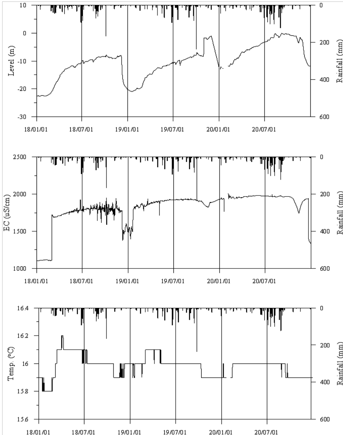
<의령5 관측공의 장기관측자료 (2018.1.1 ~ 2020.12.31)> (a)지하수위, (b)전기전도도, (c)수온
