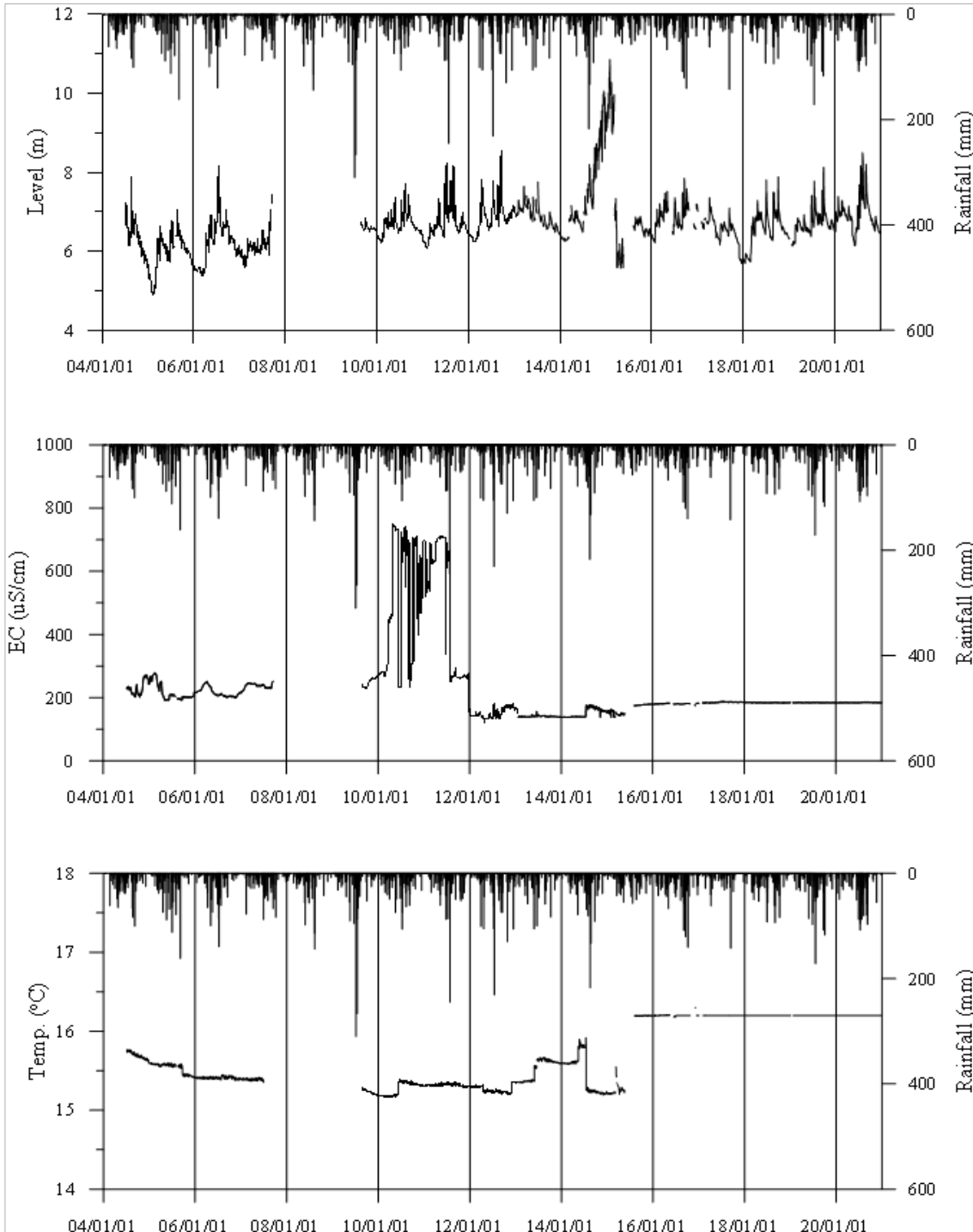
<김해1 관측공의 장기관측자료 (2004.1.1 ~ 2020.12.31)> (a)지하수위, (b)전기전도도, (c)수온
