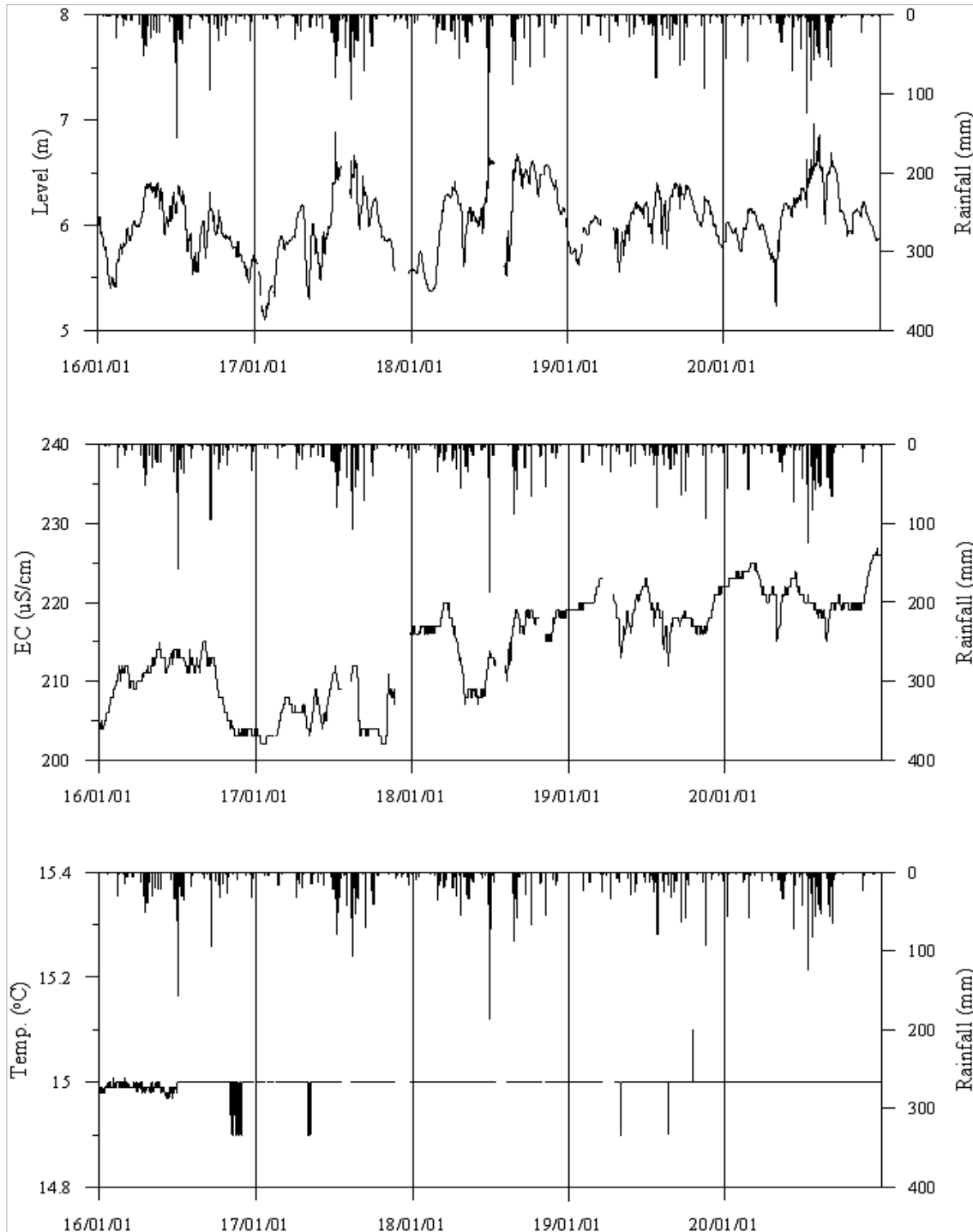
<부여3 관측공의 장기관측자료 (2016.1.1 ~ 2020.12.31)> (a)지하수위, (b)전기전도도, (c)수온
