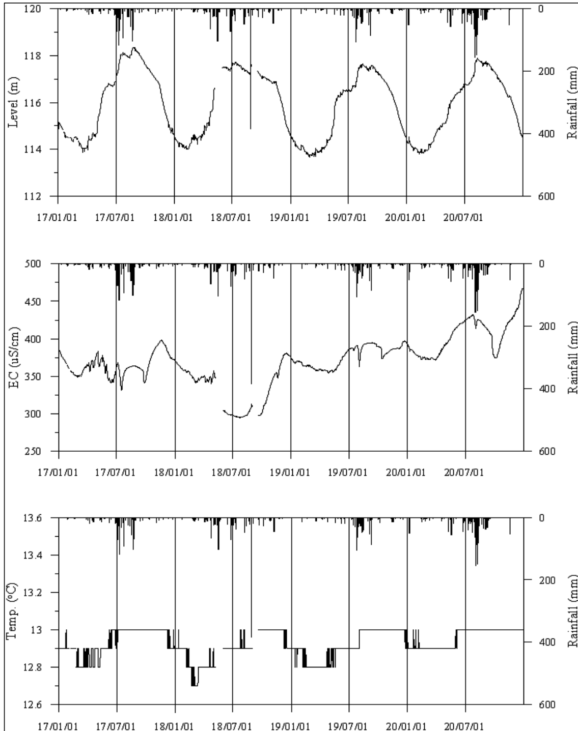
<포천2 관측공의 장기관측자료 (2017.1.1 ~ 2020.12.31)> (a)지하수위, (b)전기전도도, (c)수온
