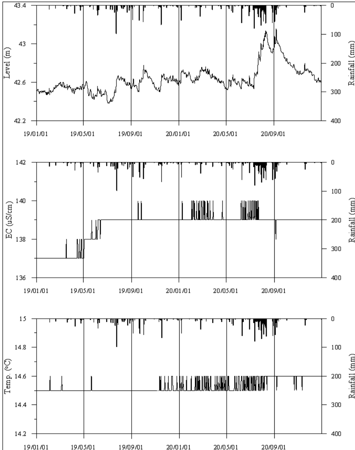
<청주2 관측공의 장기관측자료 (2019.1.1 ~ 2020.12.31)> (a)지하수위, (b)전기전도도, (c)수온
