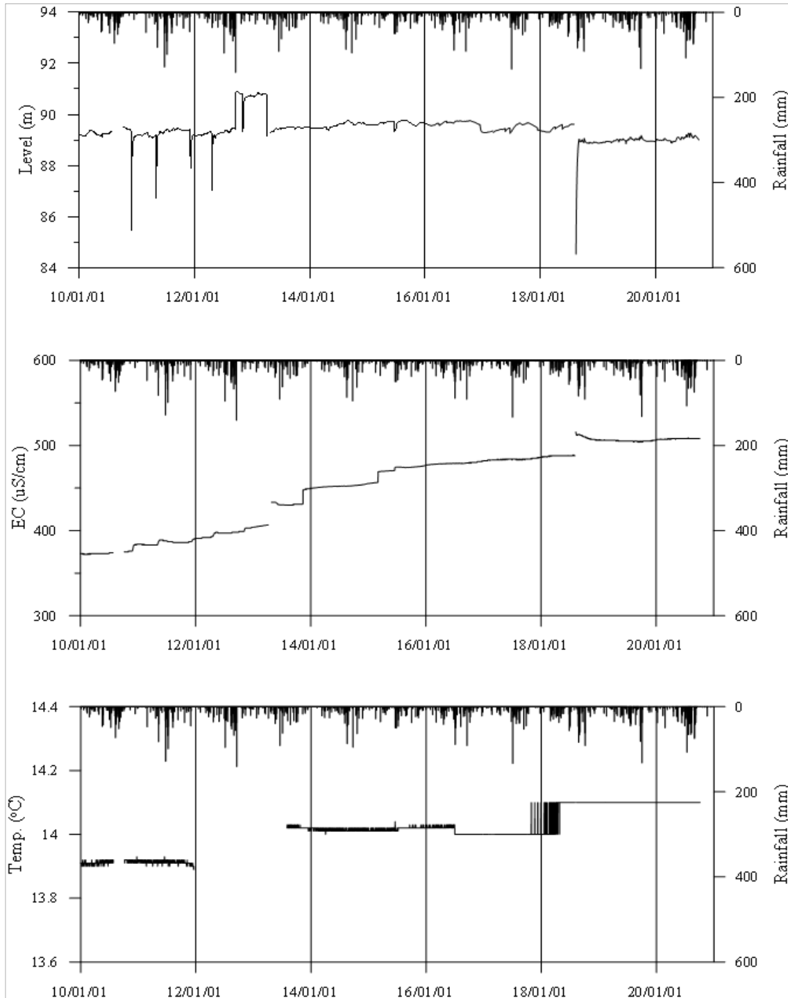
<상주3 관측공의 장기관측자료 (2010.1.1 ~ 2020.12.31)> (a)지하수위, (b)전기전도도, (c)수온
