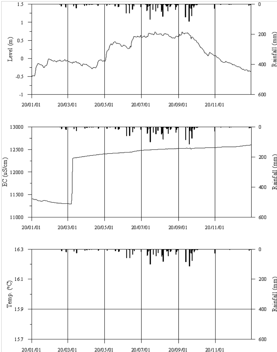
<해남9 관측공의 장기관측자료 (2020.1.1~2020.12.31)> (a)지하수위, (b)전기전도도, (c)수온
