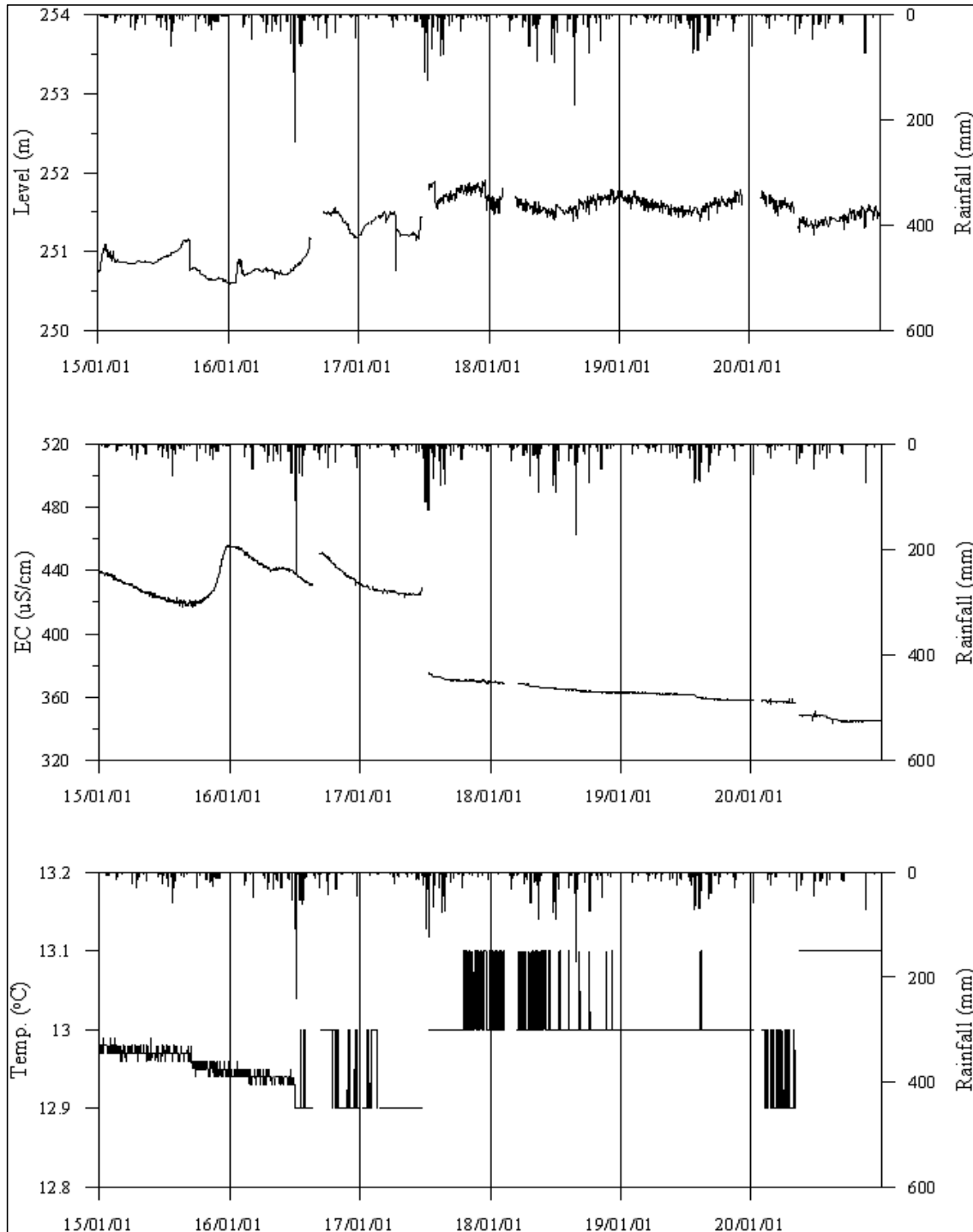
<춘천3 관측공의 장기관측자료 (2015.1.1 ~ 2020.12.31)> (a)지하수위, (b)전기전도도, (c)수온
