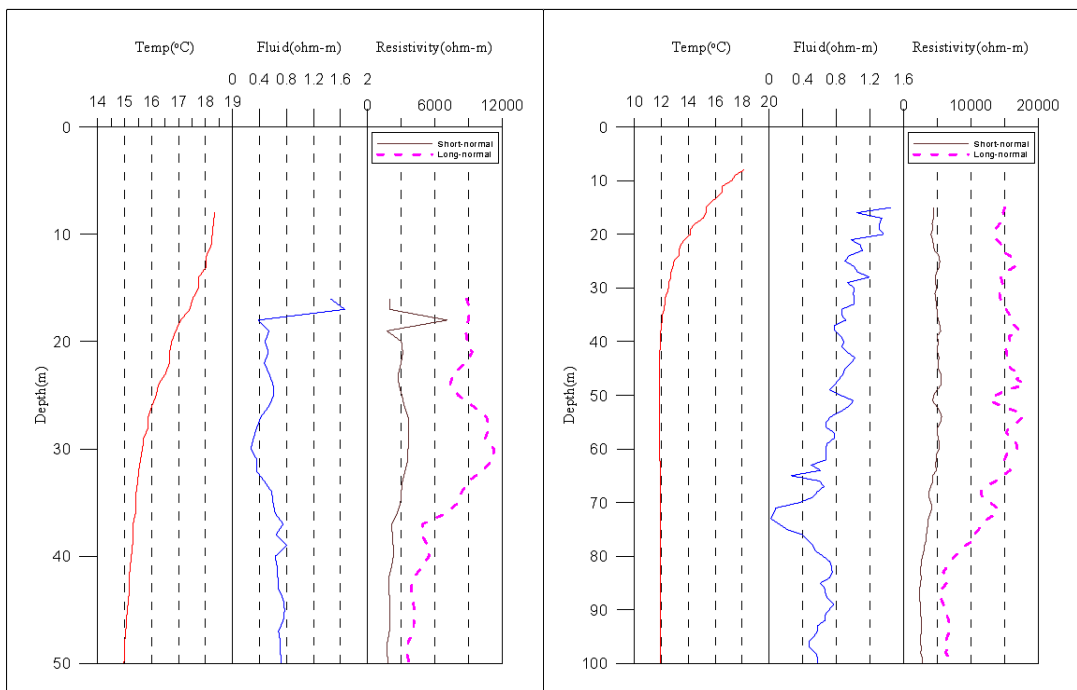
<영월5 관측공 물리검층>
