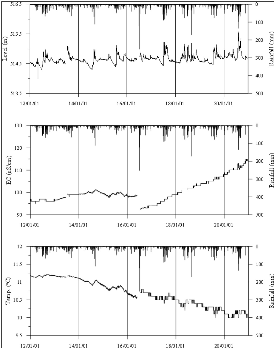
<양구2 관측공의 장기관측자료 (2012.1.1 ~ 2020.12.31)> (a)지하수위, (b)전기전도도, (c)수온
