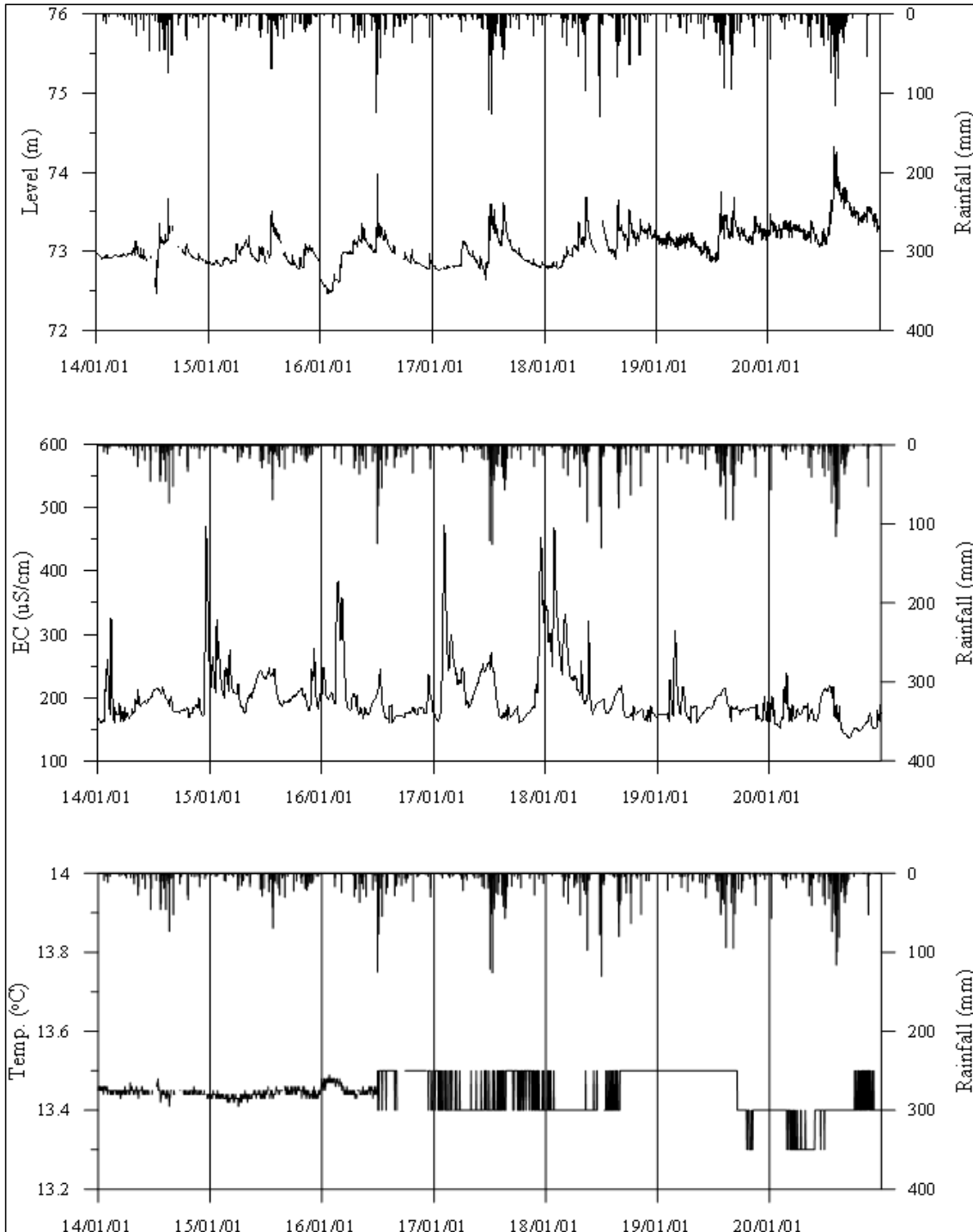
<남양주1 관측공의 장기관측자료 (2014.1.1 ~ 2020.12.31)> (a)지하수위, (b)전기전도도, (c)수온
