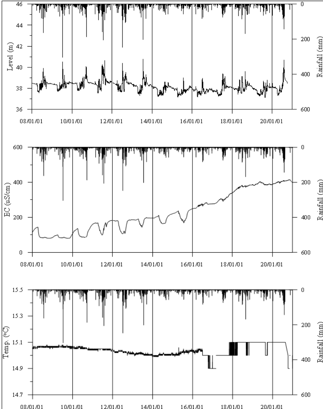
<이천1 관측공의 장기관측자료 (2008.1.1 ~ 2020.12.31)> (a)지하수위, (b)전기전도도, (c)수온
