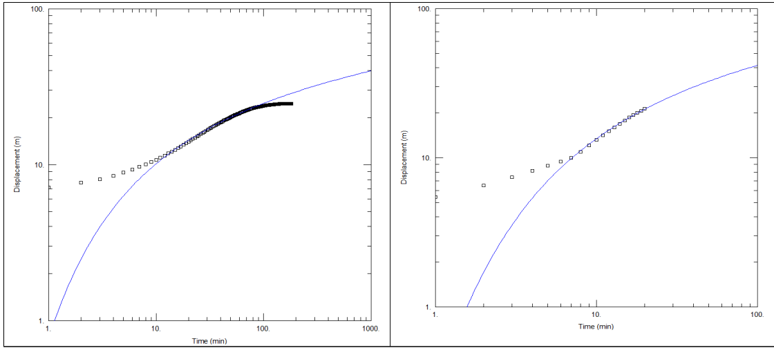
<가평4 관측공 양수시험>
