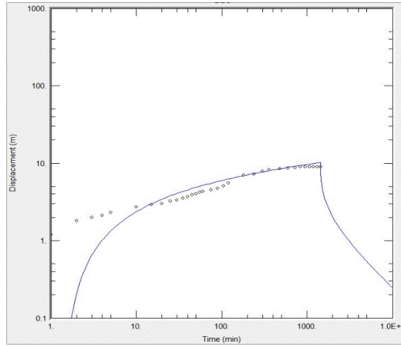
<청송6 관측공 양수시험>
