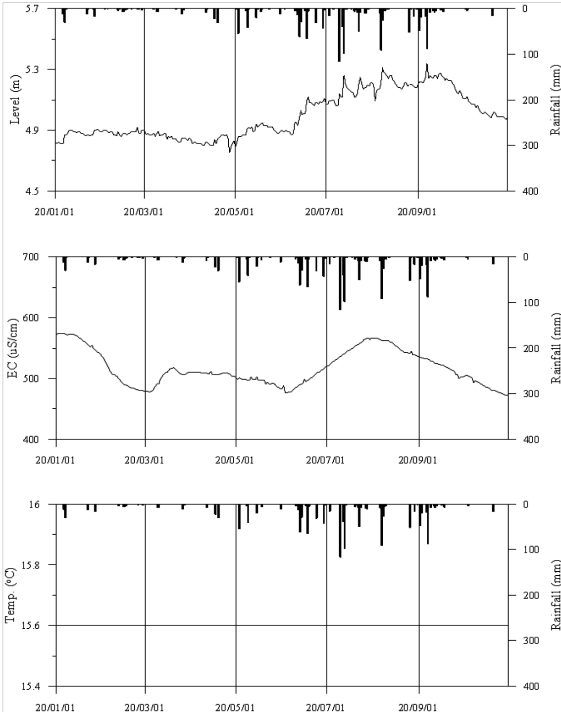
<영암5 관측공의 장기관측자료 (2020.1.1~2020.10.31)> (a)지하수위, (b)전기전도도, (c)수온
