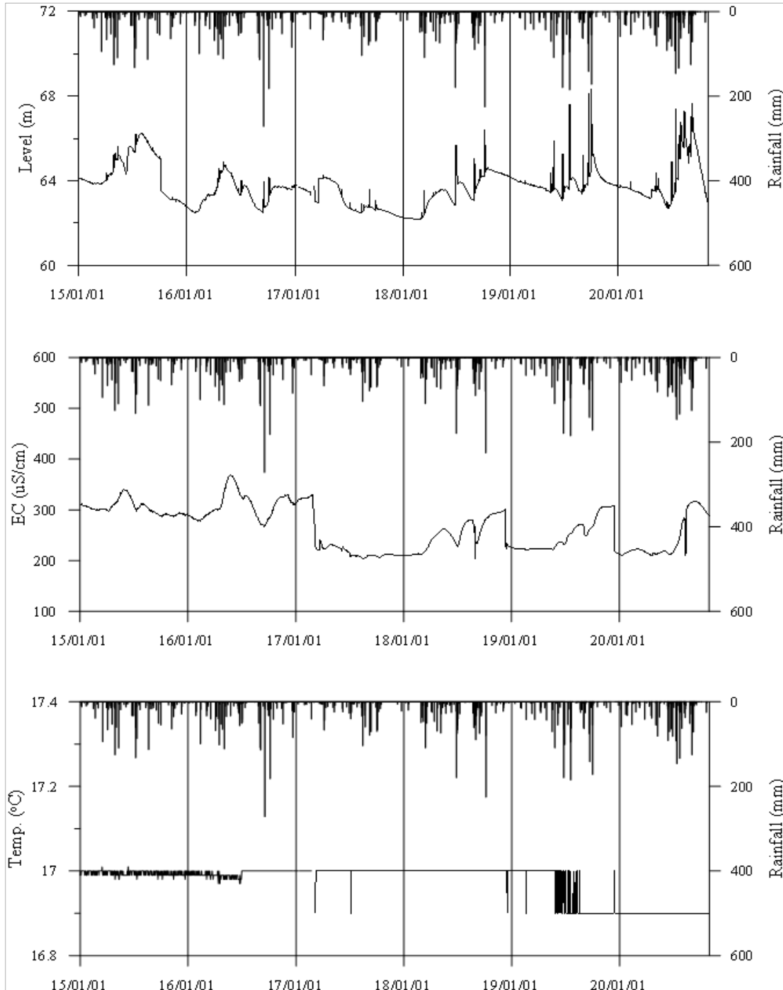
<남해1 관측공의 장기관측자료 (2015.1.1 ~ 2020.10.31)> (a)지하수위, (b)전기전도도, (c)수온
