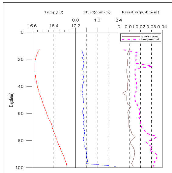
<순천8 관측공 물리검층>
