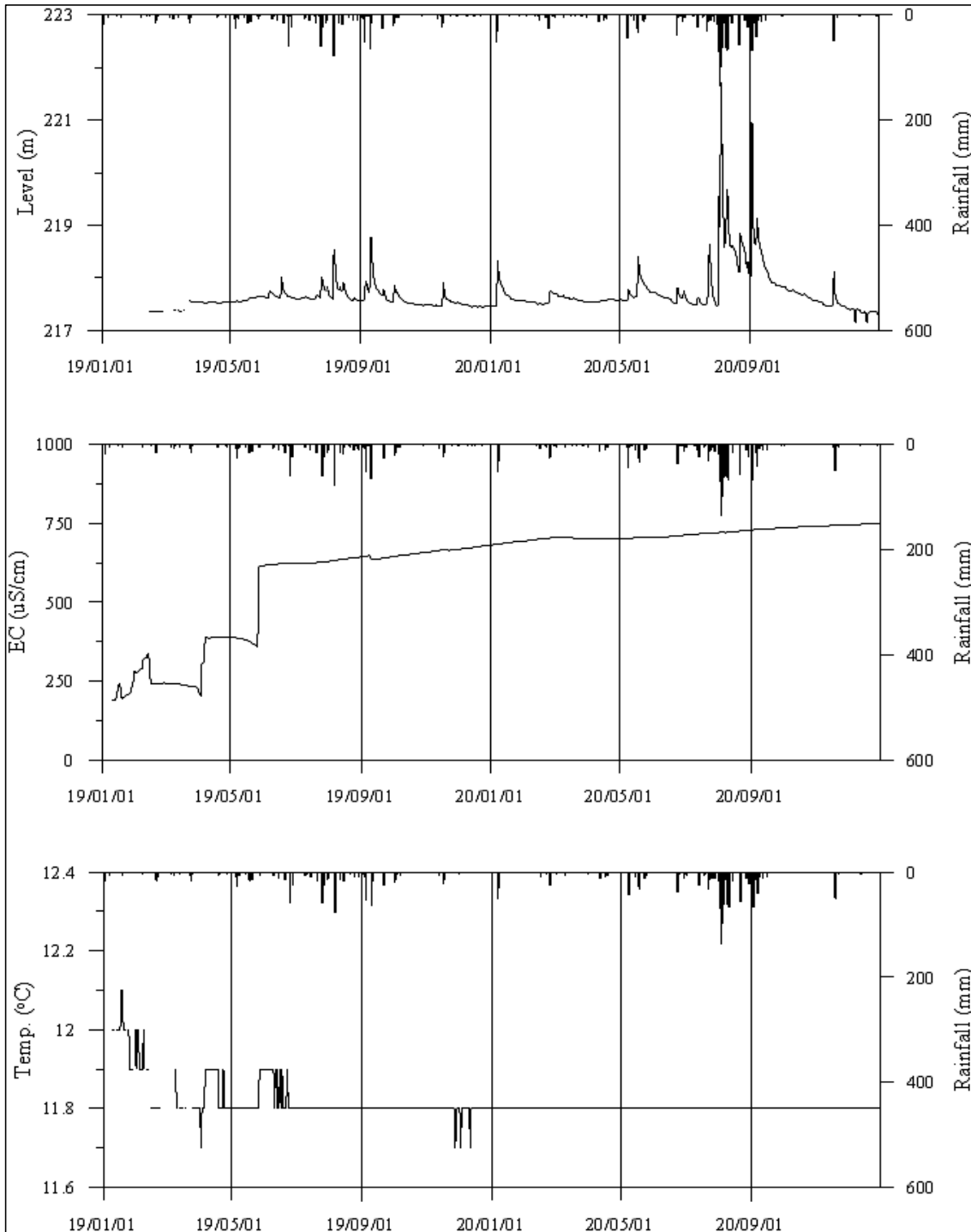
<인제4 관측공의 장기관측자료 (2019.1.1 ~ 2020.12.31)> (a)지하수위, (b)전기전도도, (c)수온
