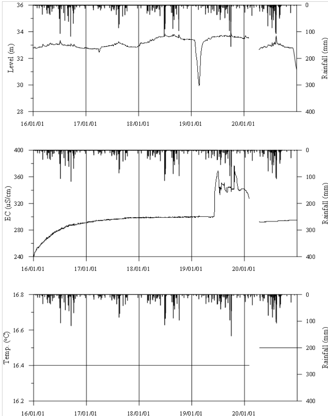
<구미4 관측공의 장기관측자료 (2016.1.1 ~ 2020.12.31)> (a)지하수위, (b)전기전도도, (c)수온
