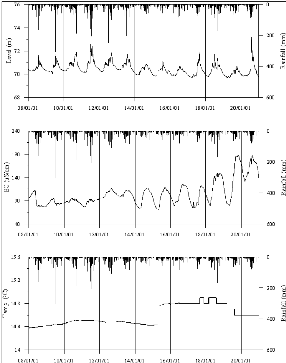
<이천2 관측공의 장기관측자료 (2008.1.1 ~ 2020.12.31)> (a)지하수위, (b)전기전도도, (c)수온
