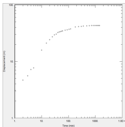
<사천5 관측공 양수시험>
