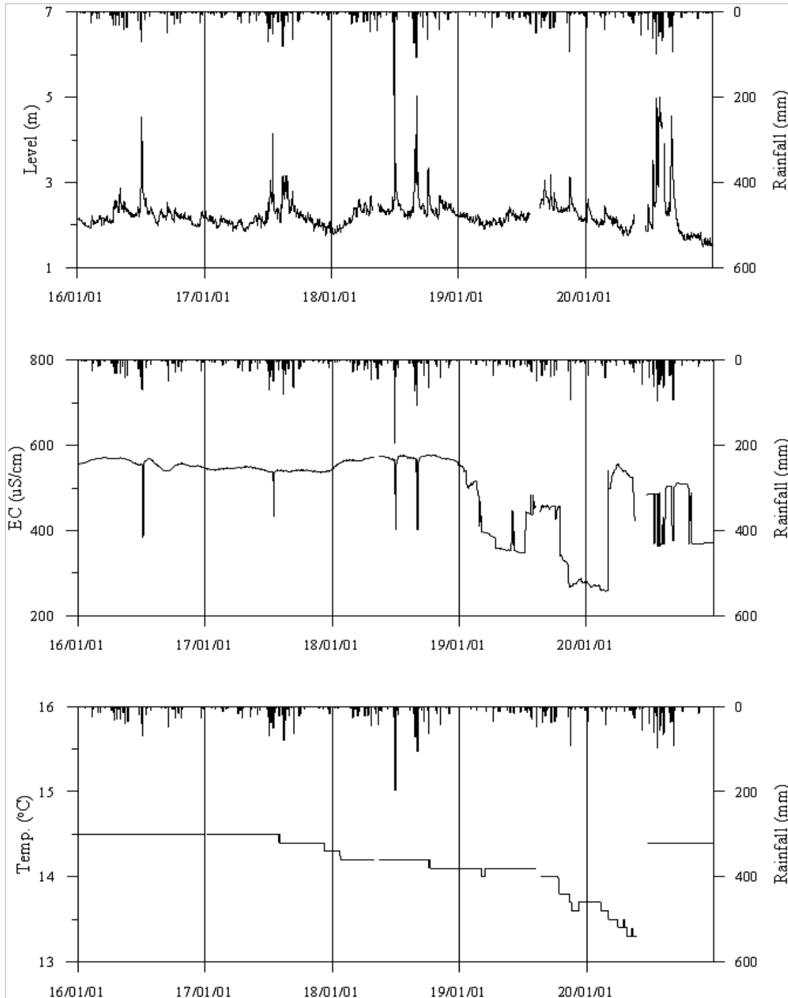
<청양3 관측공의 장기관측자료 (2016.1.1 ~ 2020.12.31)> (a)지하수위, (b)전기전도도, (c)수온
