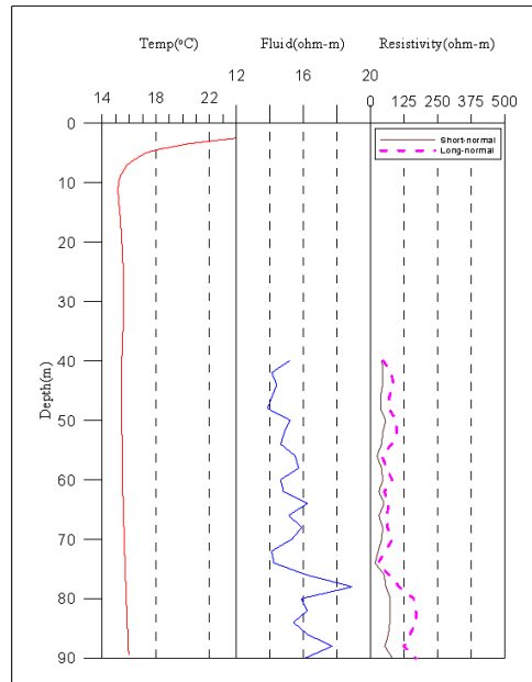
<함양2 관측공 물리검층>
