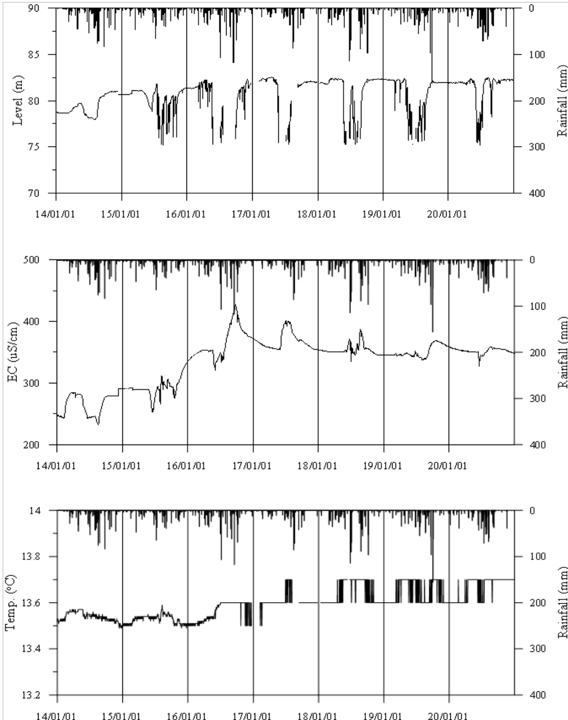
<군위1 관측공의 장기관측자료 (2014.1.1 ~ 2020.12.31)> (a)지하수위, (b)전기전도도, (c)수온
