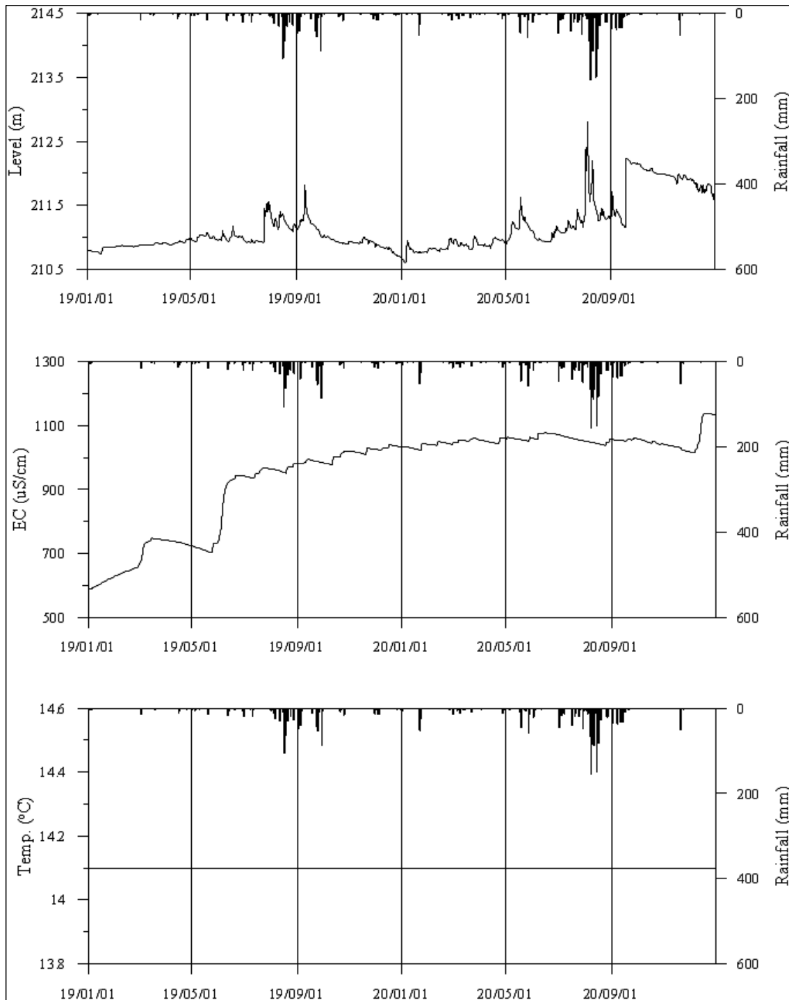
<철원4 관측공의 장기관측자료 (2018.12.1 ~ 2020.12.31)> (a)지하수위, (b)전기전도도, (c)수온
