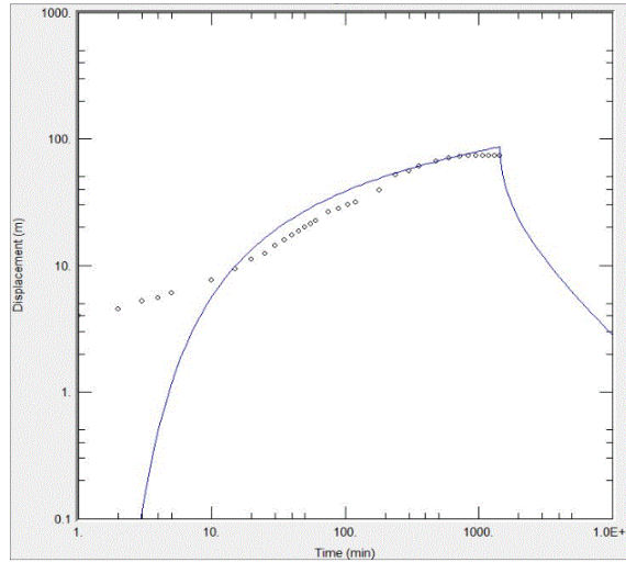
<봉화7 관측공 양수시험>
