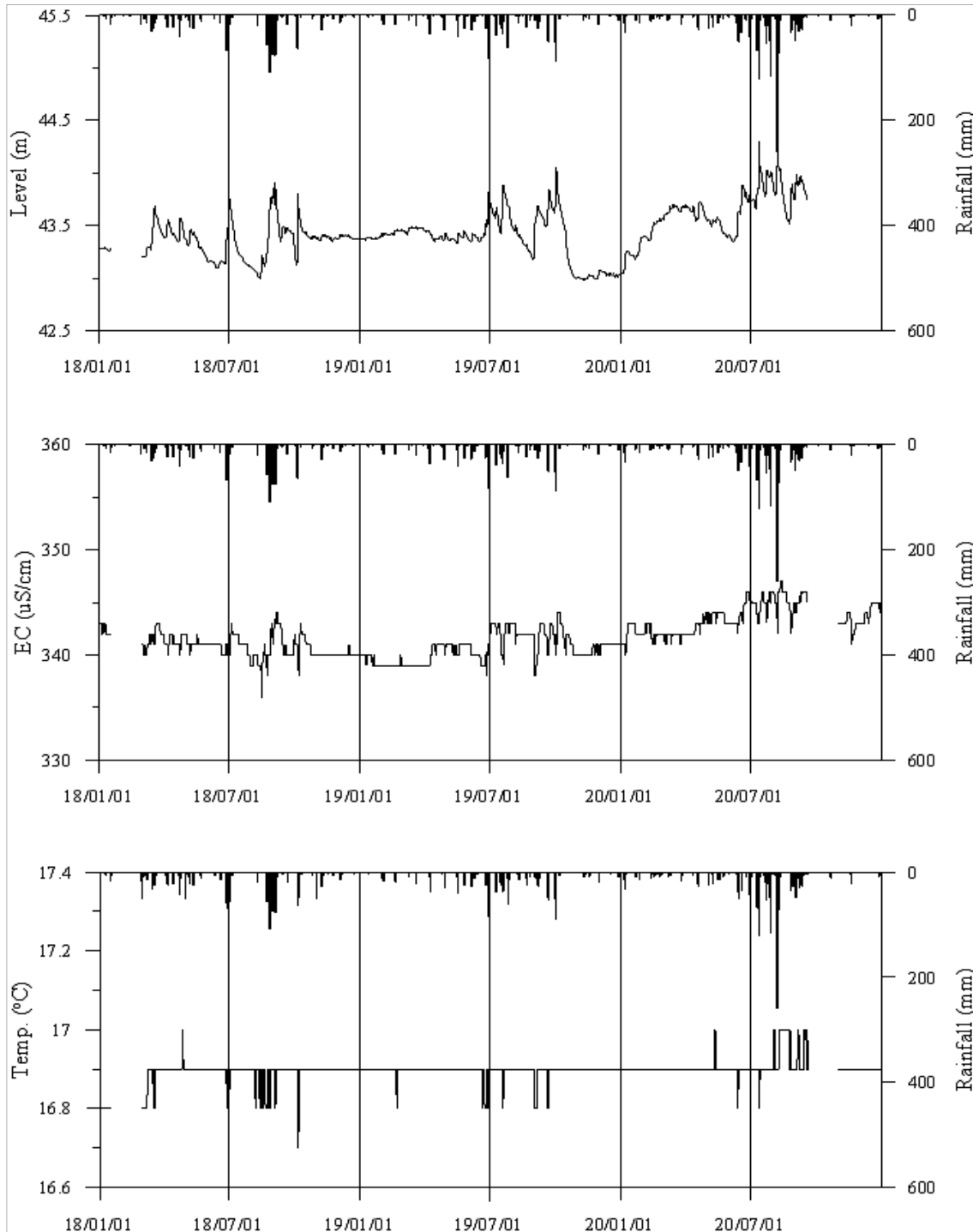
<화순3 관측공의 장기관측자료 (2018.1.1 ~ 2020.12.31)> (a)지하수위, (b)전기전도도, (c)수온
