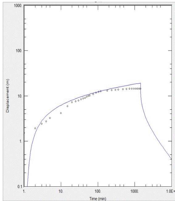
<칠곡4 관측공 양수시험>
