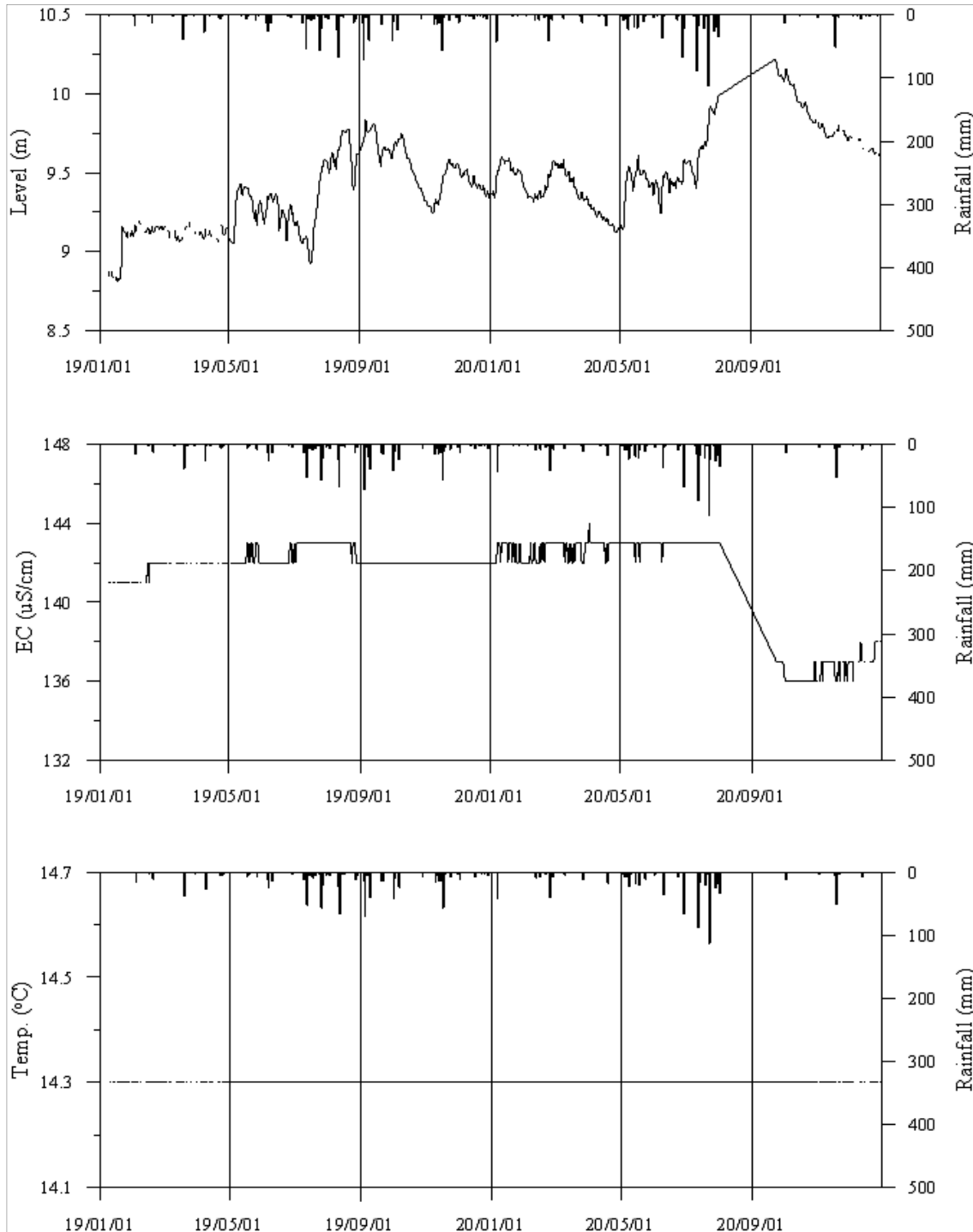
<예산5 관측공의 장기관측자료 (2019.1.1 ~ 2020.12.31)> (a)지하수위, (b)전기전도도, (c)수온
