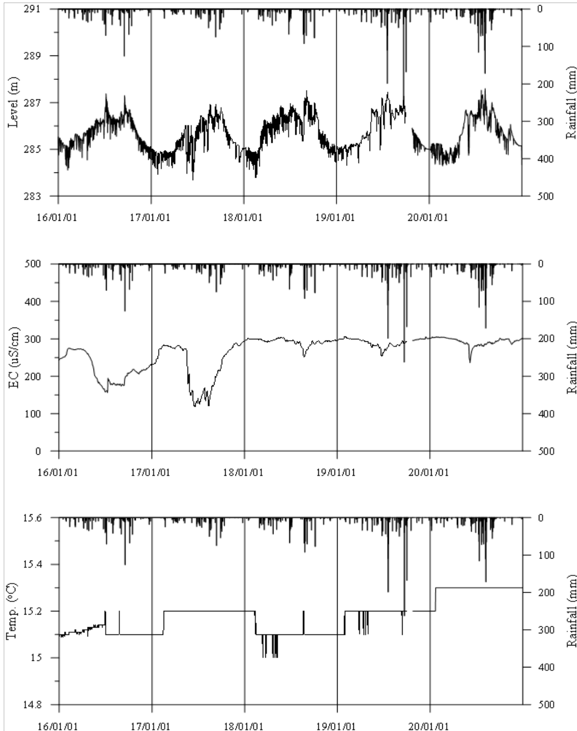
<거창2 관측공의 장기관측자료 (2016.1.1 ~ 2020.12.31)> (a)지하수위, (b)전기전도도, (c)수온
