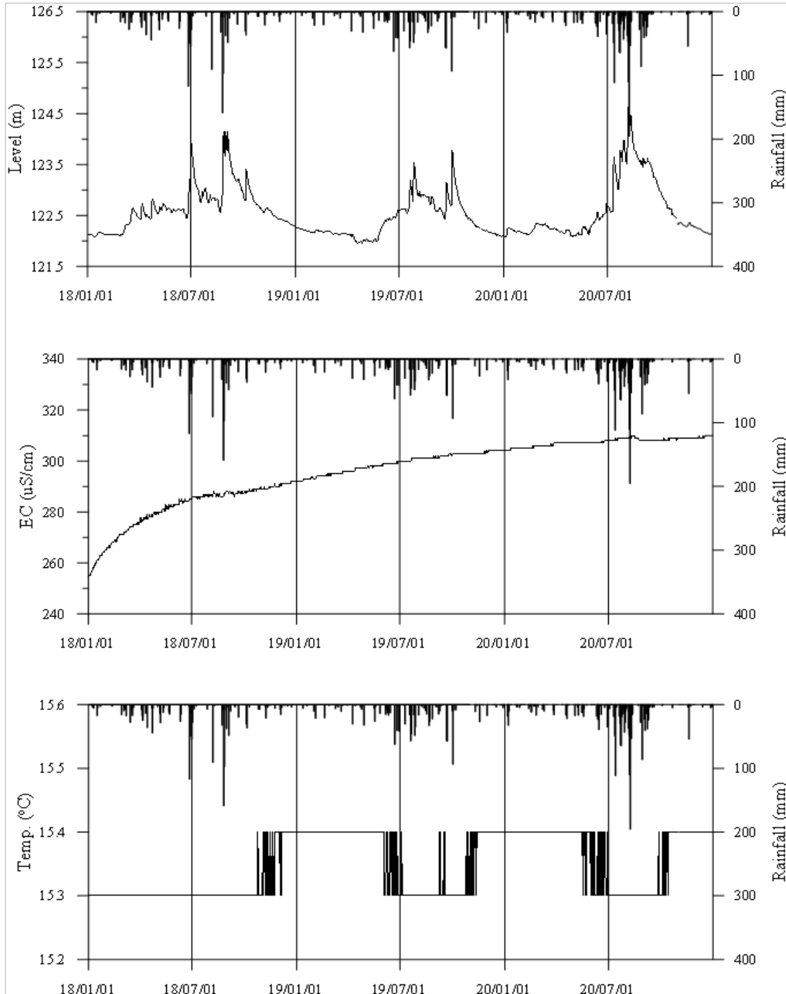
<임실1 관측공의 장기관측자료 (2018.1.1 ~ 2020.12.31)> (a)지하수위, (b)전기전도도, (c)수온
