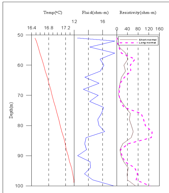
<보성7 관측공 물리검층>
