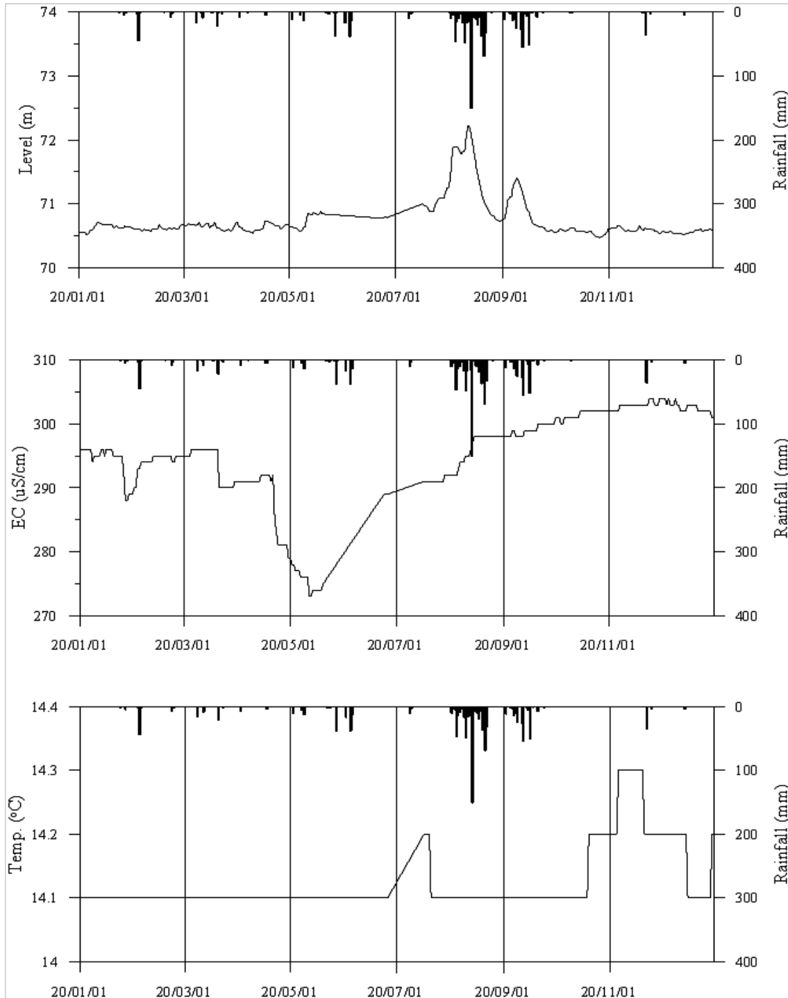
<봉화7 관측공의 장기관측자료 (2020.1.1 ~ 2020.12.31)> (a)지하수위, (b)전기전도도, (c)수온
