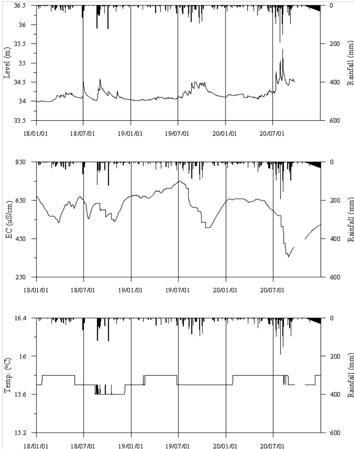
<장성4 관측공의 장기관측자료 (2018.1.1 ~ 2020.12.31)> (a)지하수위, (b)전기전도도, (c)수온
