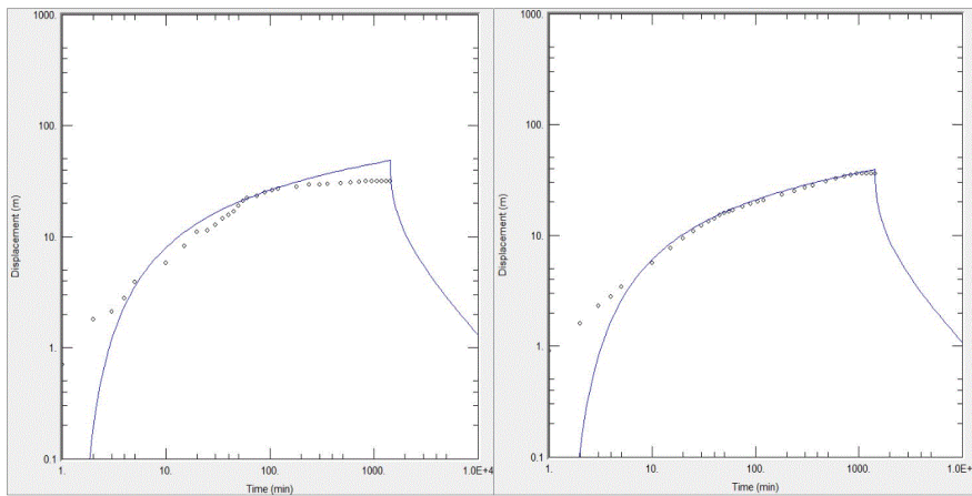
<울진1 관측공 양수시험>
