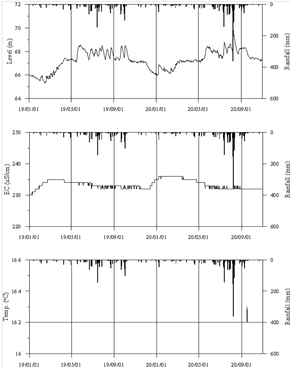
<담양5 관측공의 장기관측자료 (2019.1.1~2020.10.31)> (a)지하수위, (b)전기전도도, (c)수온
