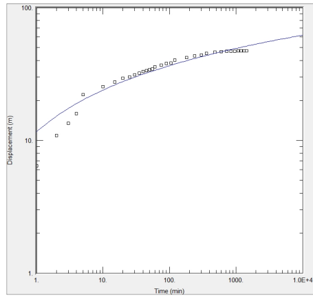
<경남고성2 관측공 양수시험>
