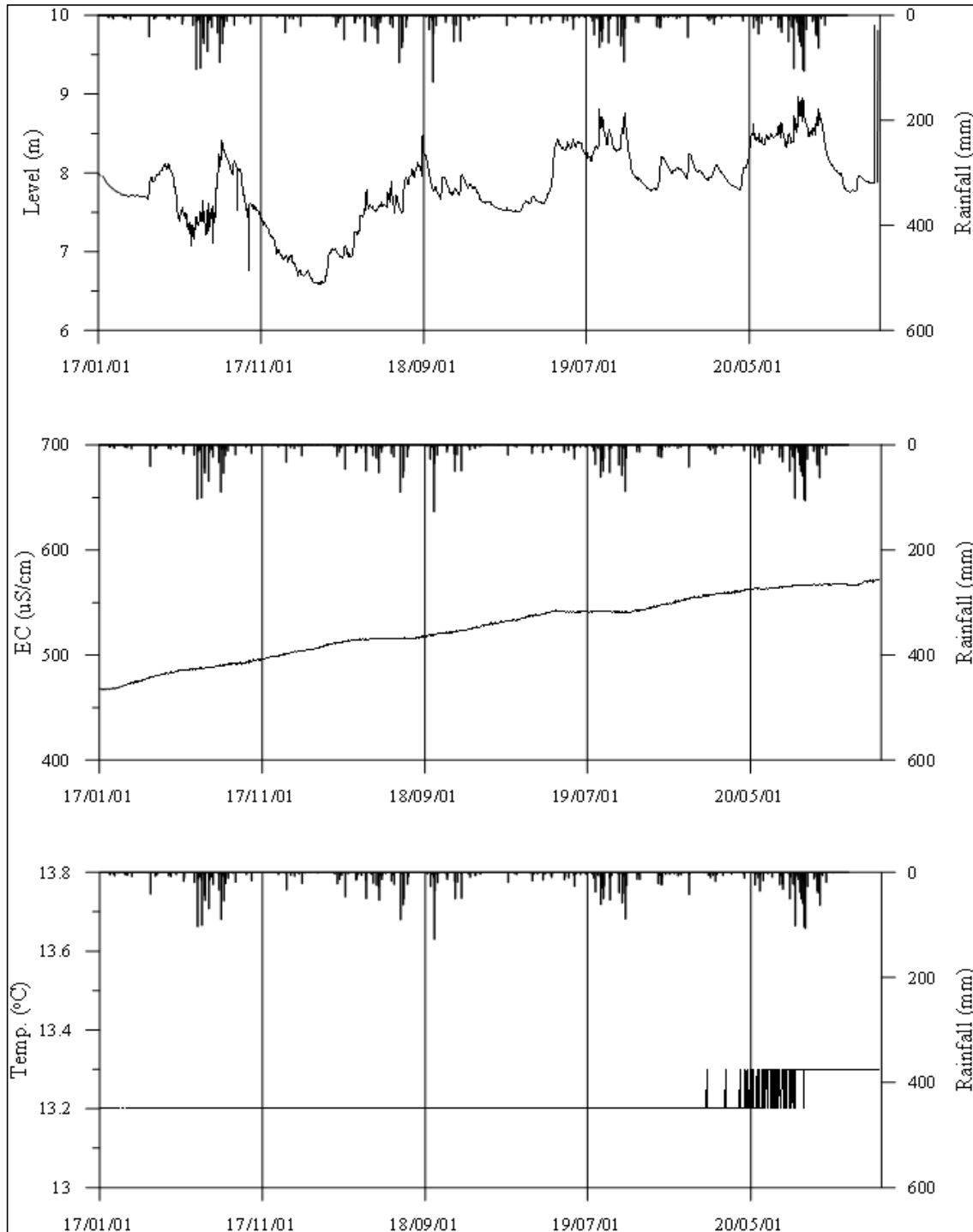
<김포3 관측공의 장기관측자료 (2017.1.1 ~ 2020.12.31)> (a)지하수위, (b)전기전도도, (c)수온
