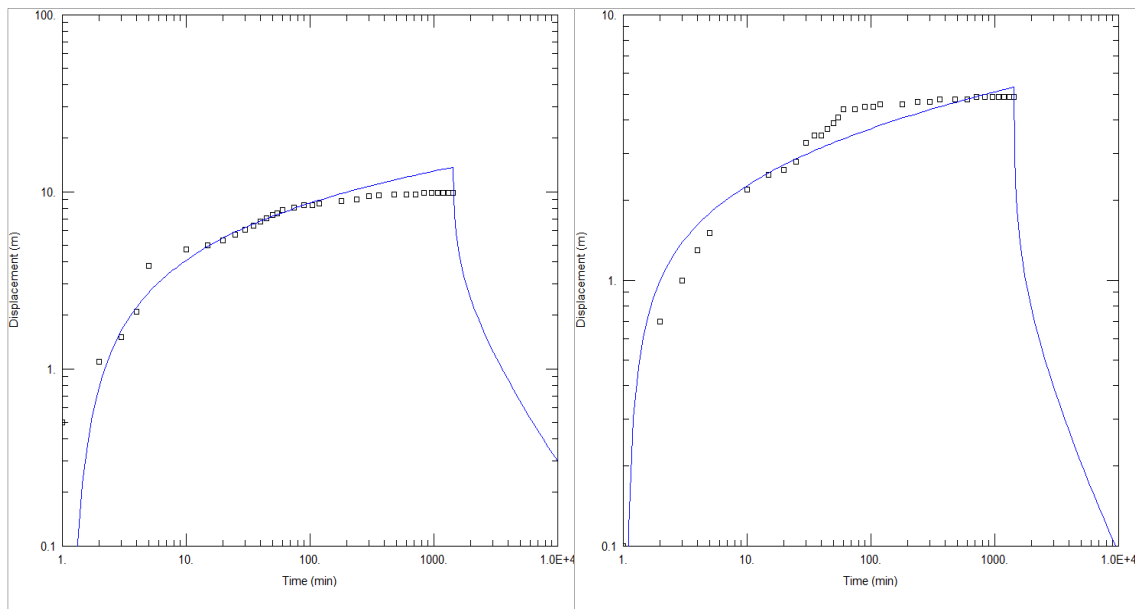
<예천2 관측공 양수시험>
