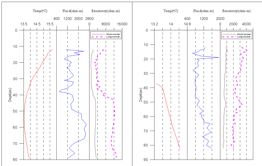
<가평4 관측공 물리검층>
