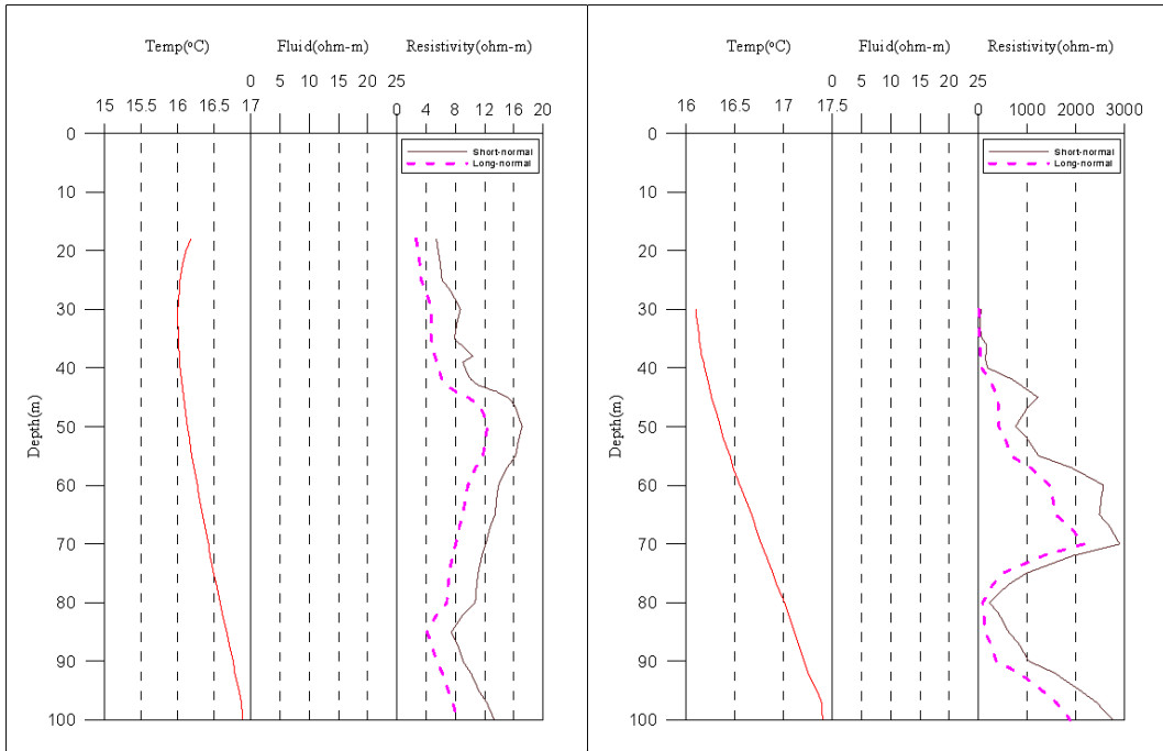
<여수1 관측공 물리검층>
