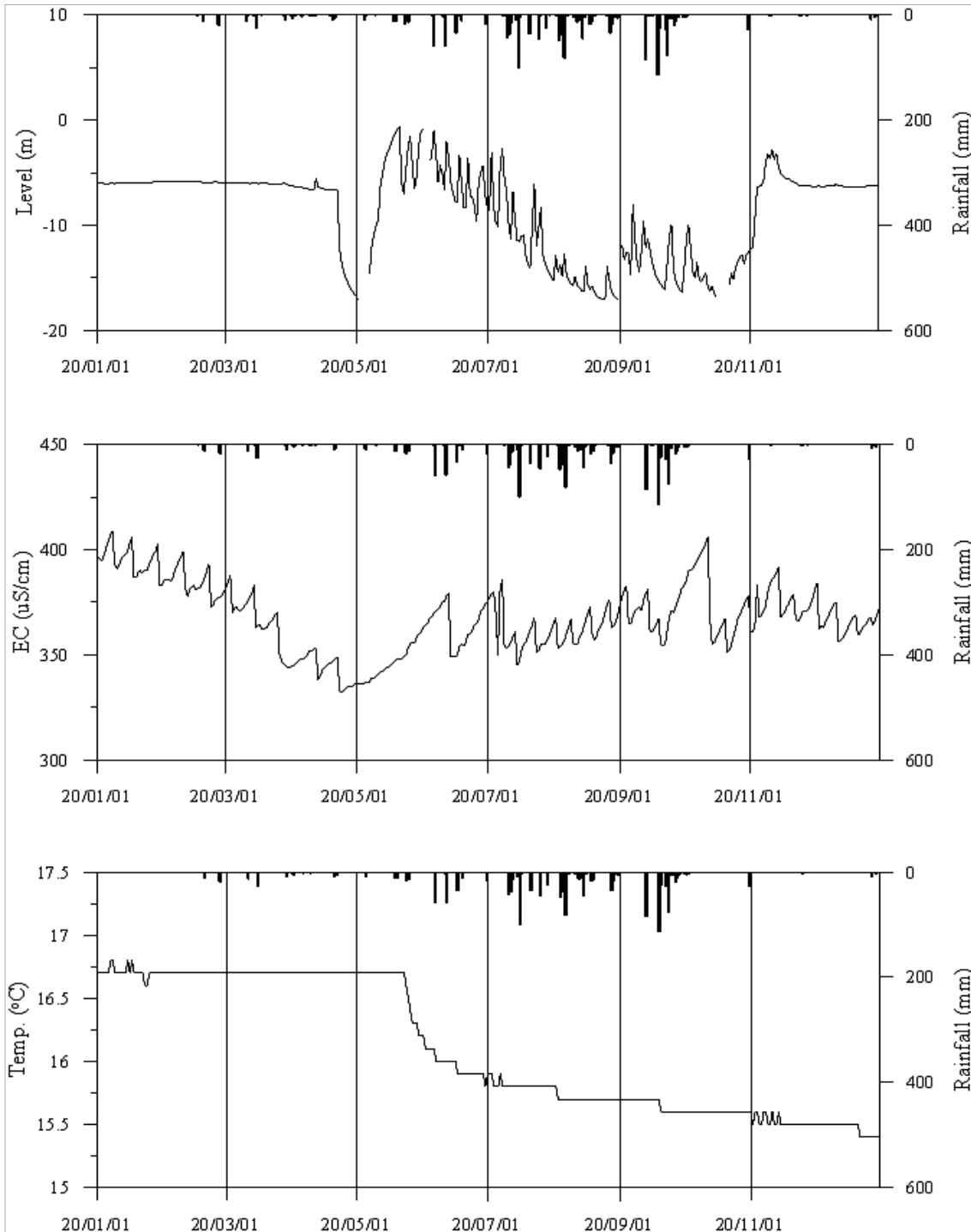
<해남10 관측공의 장기관측자료 (2020.1.1~2020.12.31)> (a)지하수위, (b)전기전도도, (c)수온
