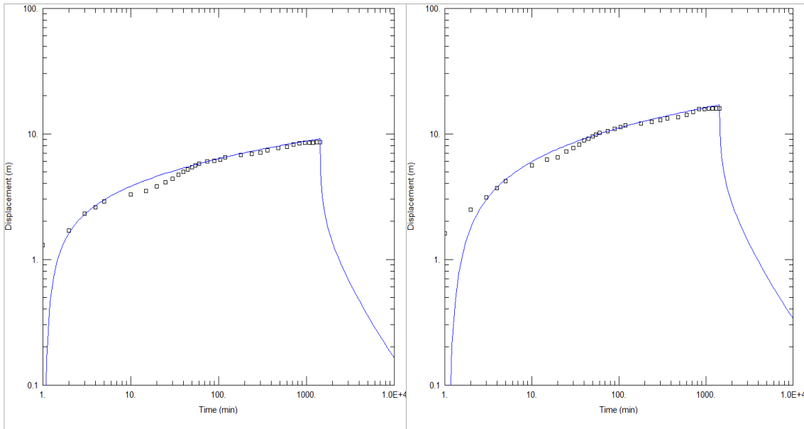
<안동7 관측공 양수시험>
