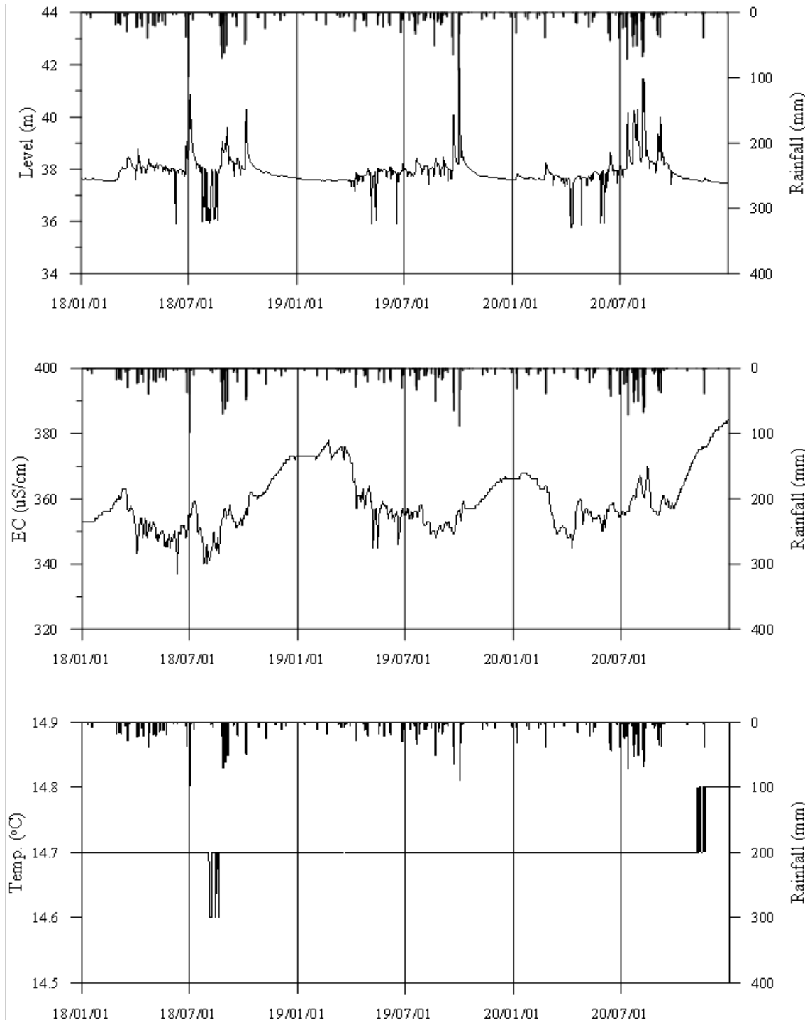
<의성3 관측공의 장기관측자료 (2018.1.1 ~ 2020.12.31.)> (a)지하수위, (b)전기전도도, (c)수온
