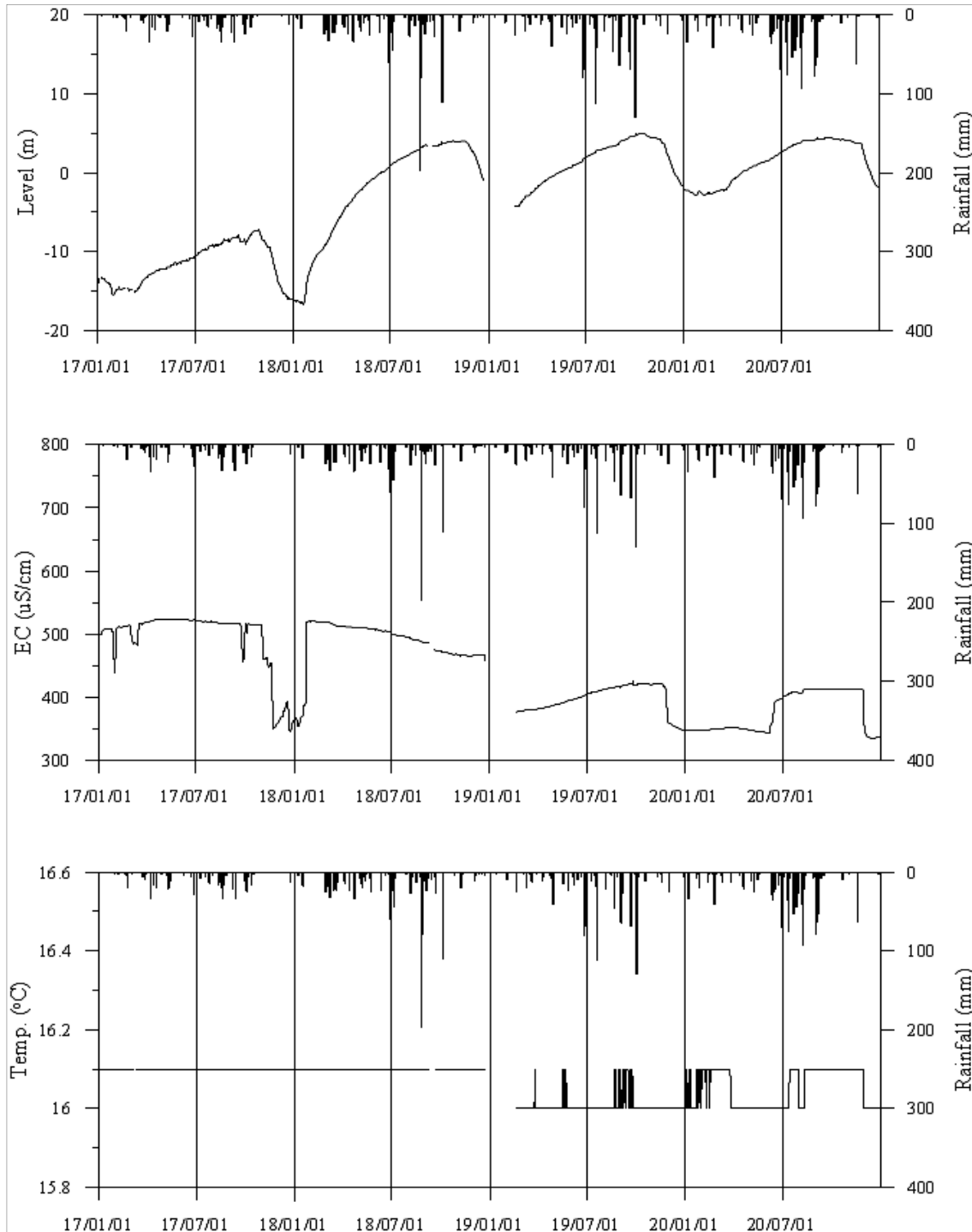
<밀양4 관측공의 장기관측자료 (2017.1.1 ~ 2020.12.31)> (a)지하수위, (b)전기전도도, (c)수온
