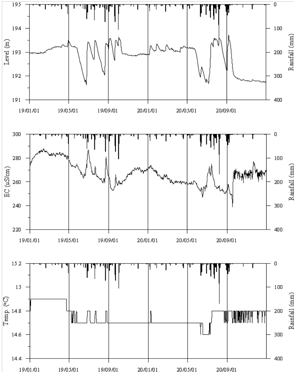
<청도3 관측공의 장기관측자료 (2019.1.1 ~ 2020.12.31.)> (a)지하수위, (b)전기전도도, (c)수온
