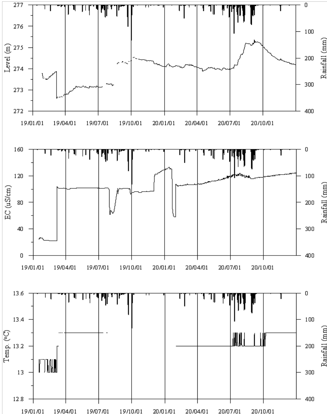
<상주8 관측공의 장기관측자료 (2019.1.1 ~ 2020.12.31)> (a)지하수위, (b)전기전도도, (c)수온
