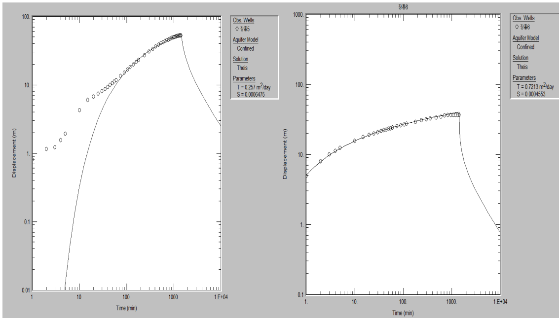
<장흥5 관측공 양수시험>
