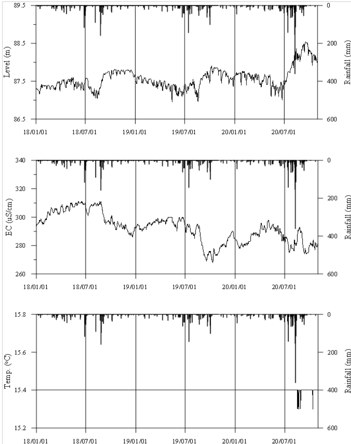
<곡성5 관측공의 장기관측자료 (2018.1.1~2020.12.31)> (a)지하수위, (b)전기전도도, (c)수온
