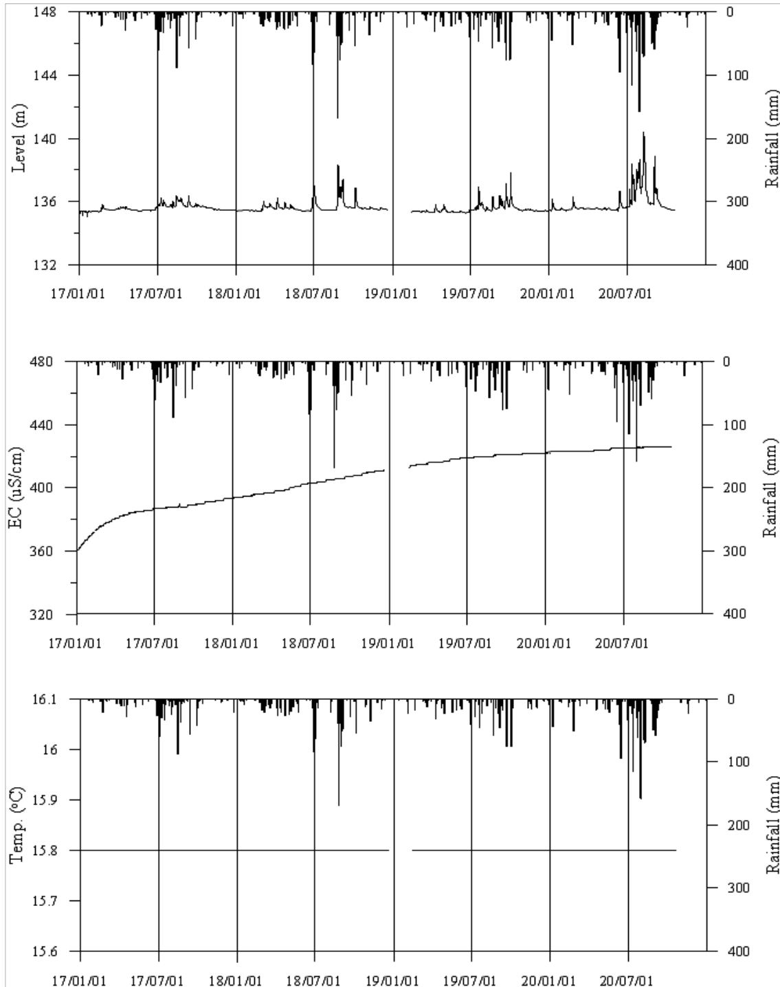
<금산2 관측공의 장기관측자료 (2017.1.1 ~ 2020.12.31)> (a)지하수위, (b)전기전도도, (c)수온
