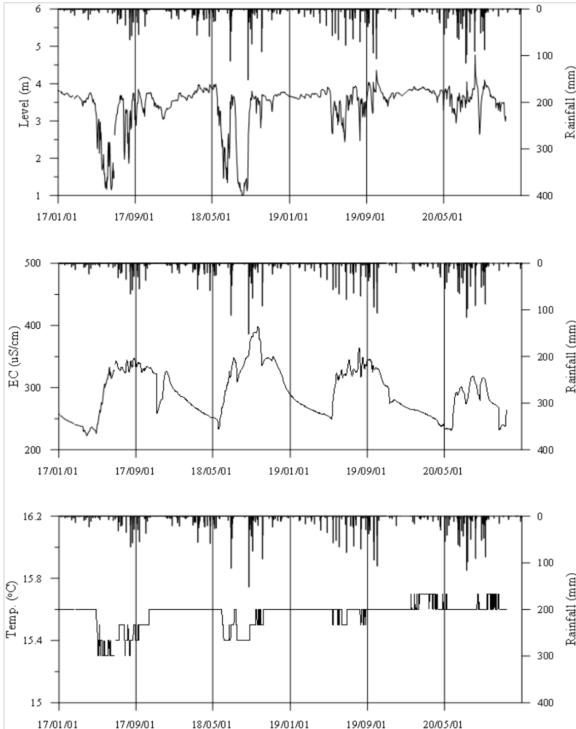
<무안6 관측공의 장기관측자료 (2017.1.1 ~ 2020.12.31)> (a)지하수위, (b)전기전도도, (c)수온
