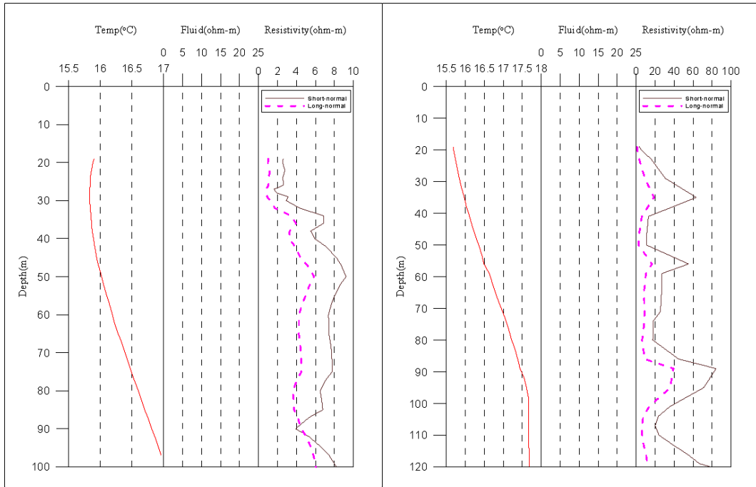
<해남13 관측공 물리검층>
