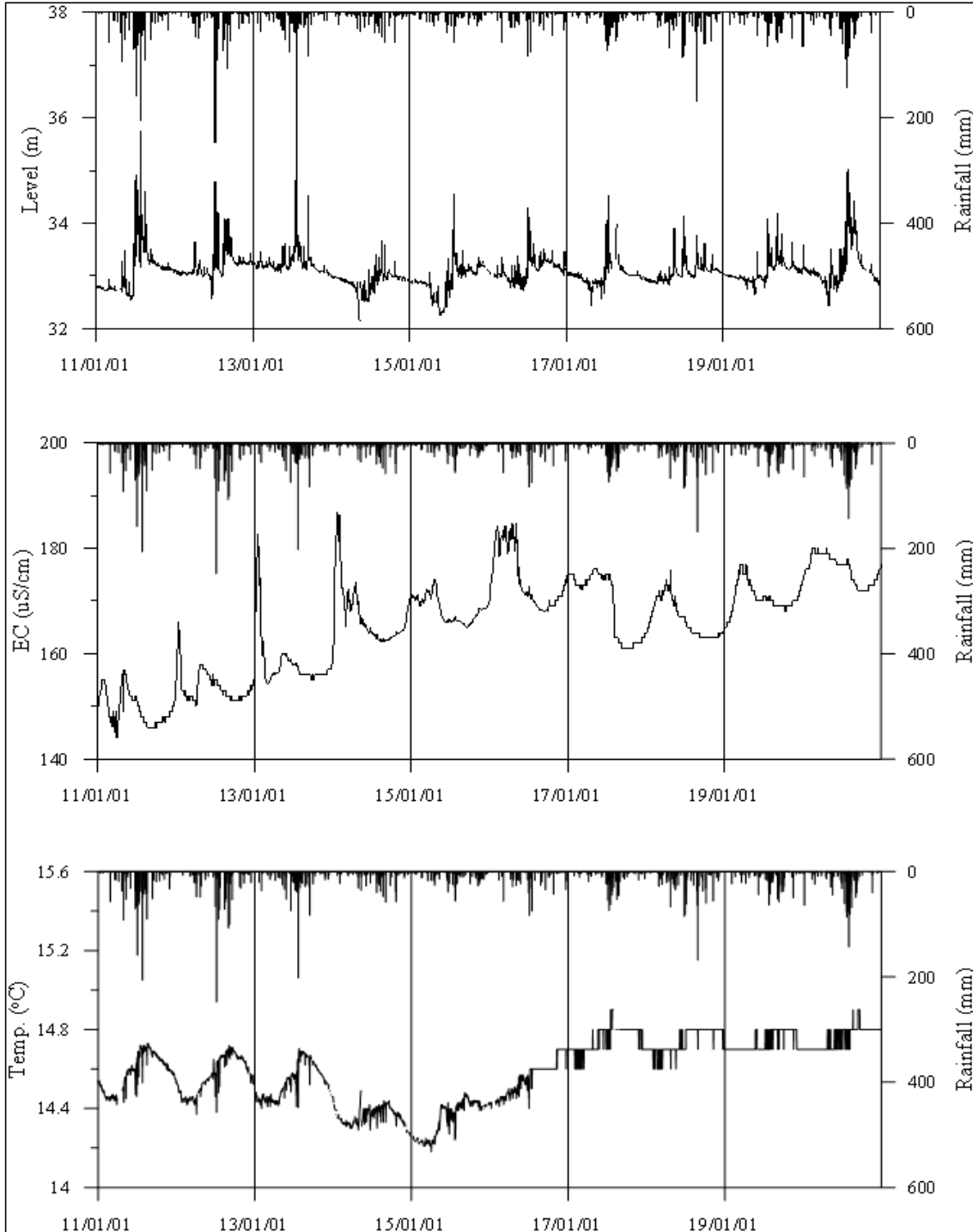
<여주1 관측공의 장기관측자료 (2011.1.1 ~ 2020.12.31)> (a)지하수위, (b)전기전도도, (c)수온
