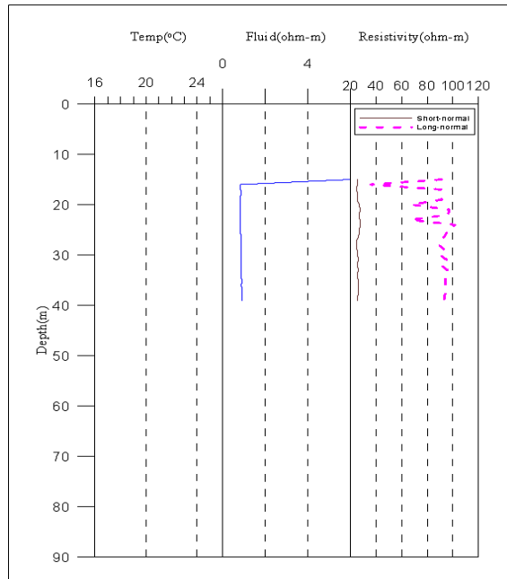
<영양5 관측공 물리검층>
