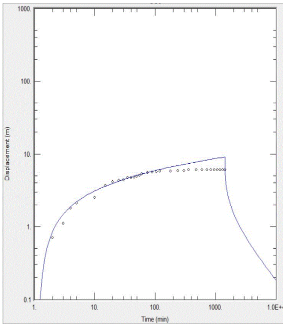
<영양3 관측공 양수시험>
