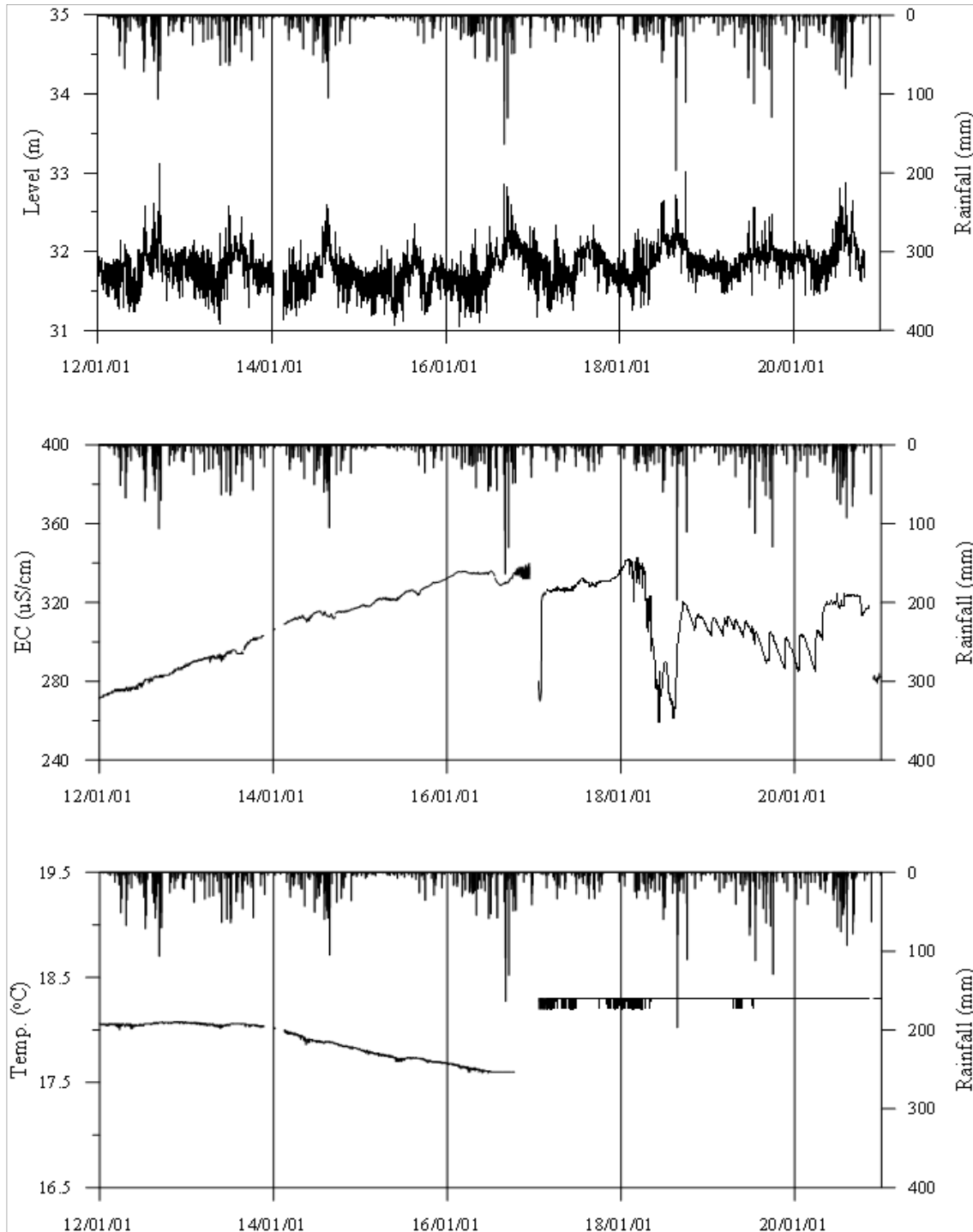
<밀양2 관측공의 장기관측자료 (2012.1.1 ~ 2020.12.31)> (a)지하수위, (b)전기전도도, (c)수온
