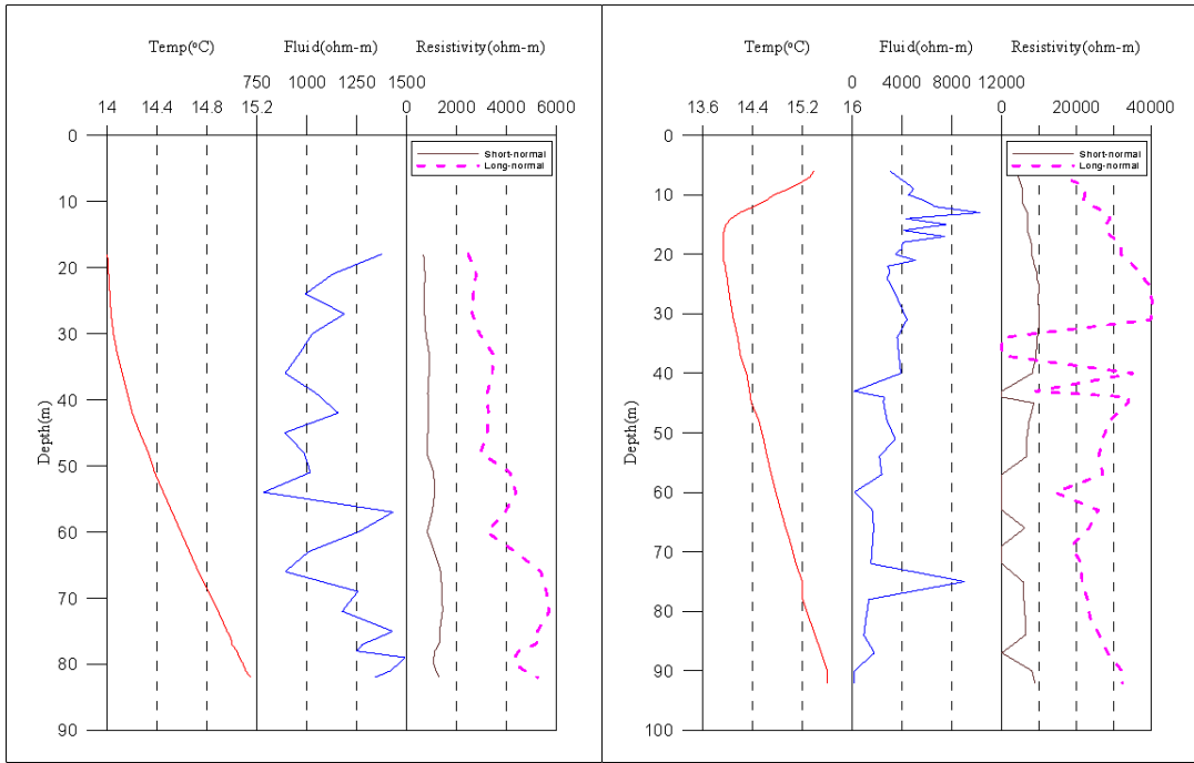
<여주5 관측공 물리검층>
