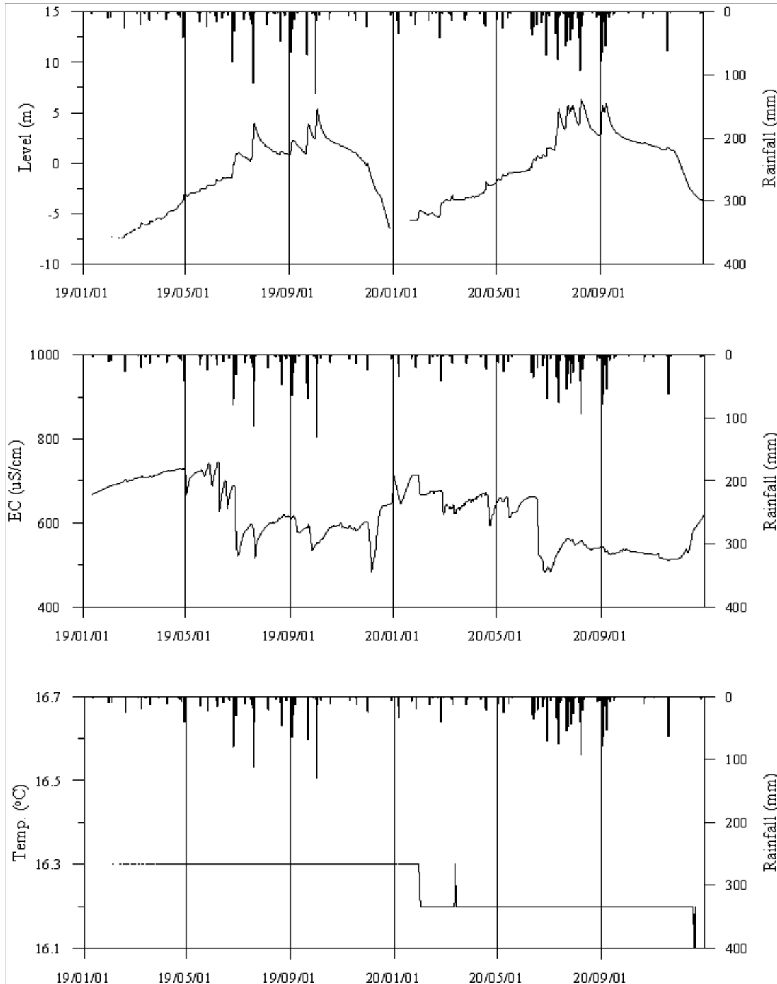
<밀양6 관측공의 장기관측자료 (2019.1.1 ~ 2020.12.31)> (a)지하수위, (b)전기전도도, (c)수온
