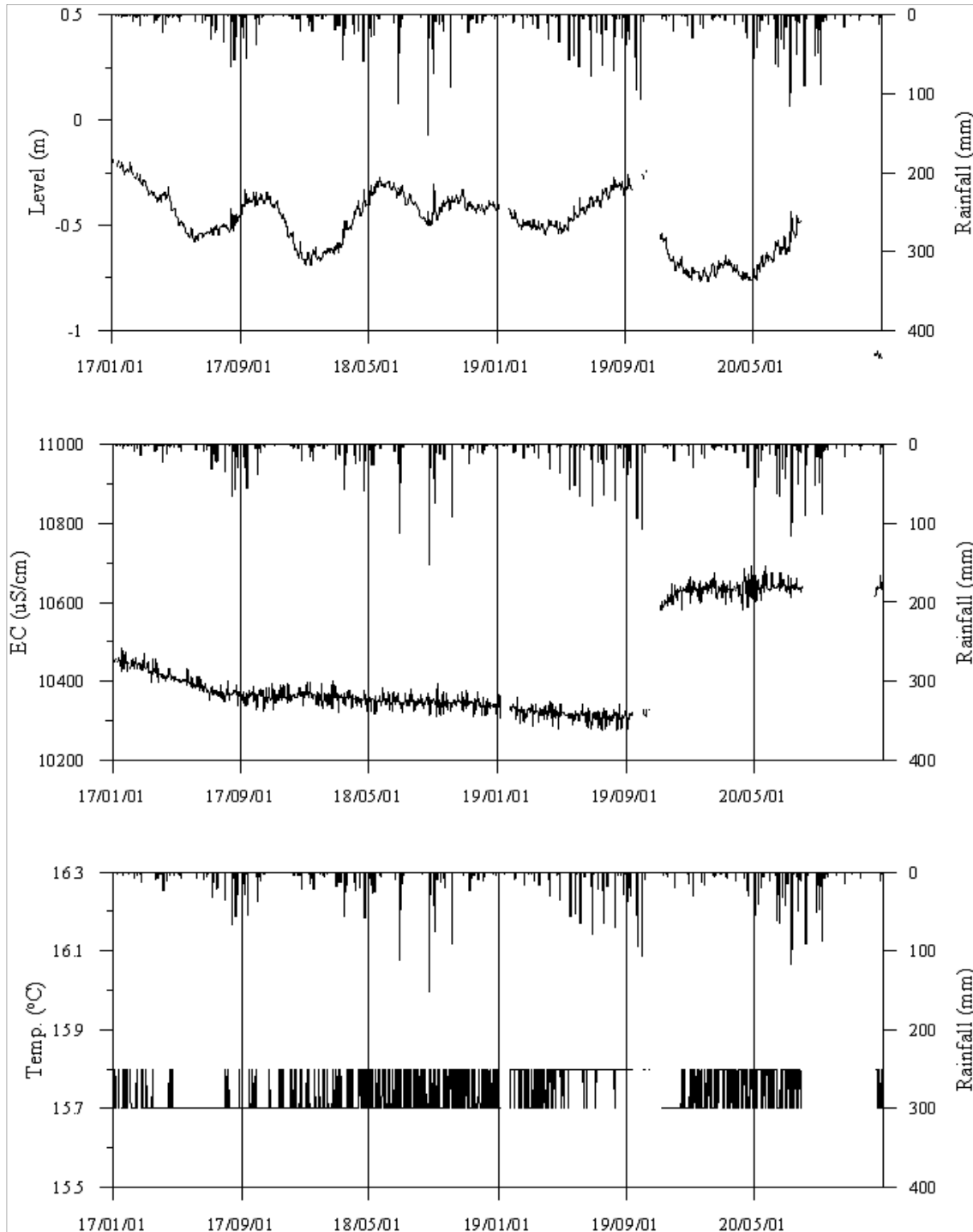
<무안5 관측공의 장기관측자료 (2017.1.1 ~ 2020.12.31)> (a)지하수위, (b)전기전도도, (c)수온
