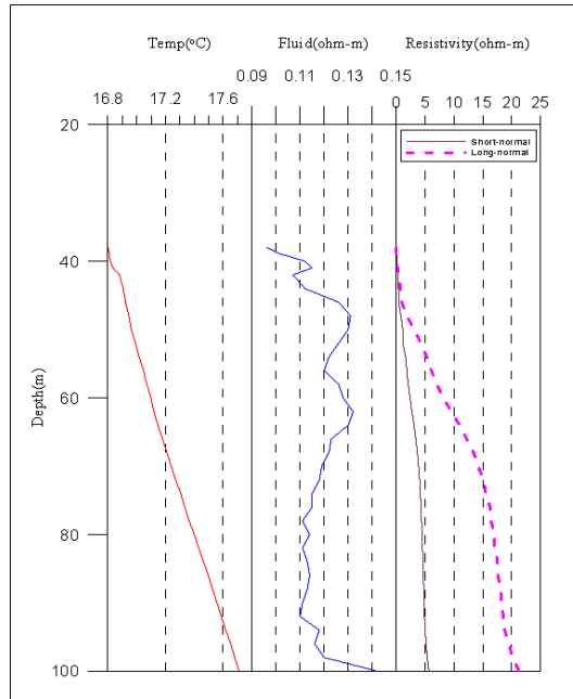
<고흥9 관측공 물리검층>
