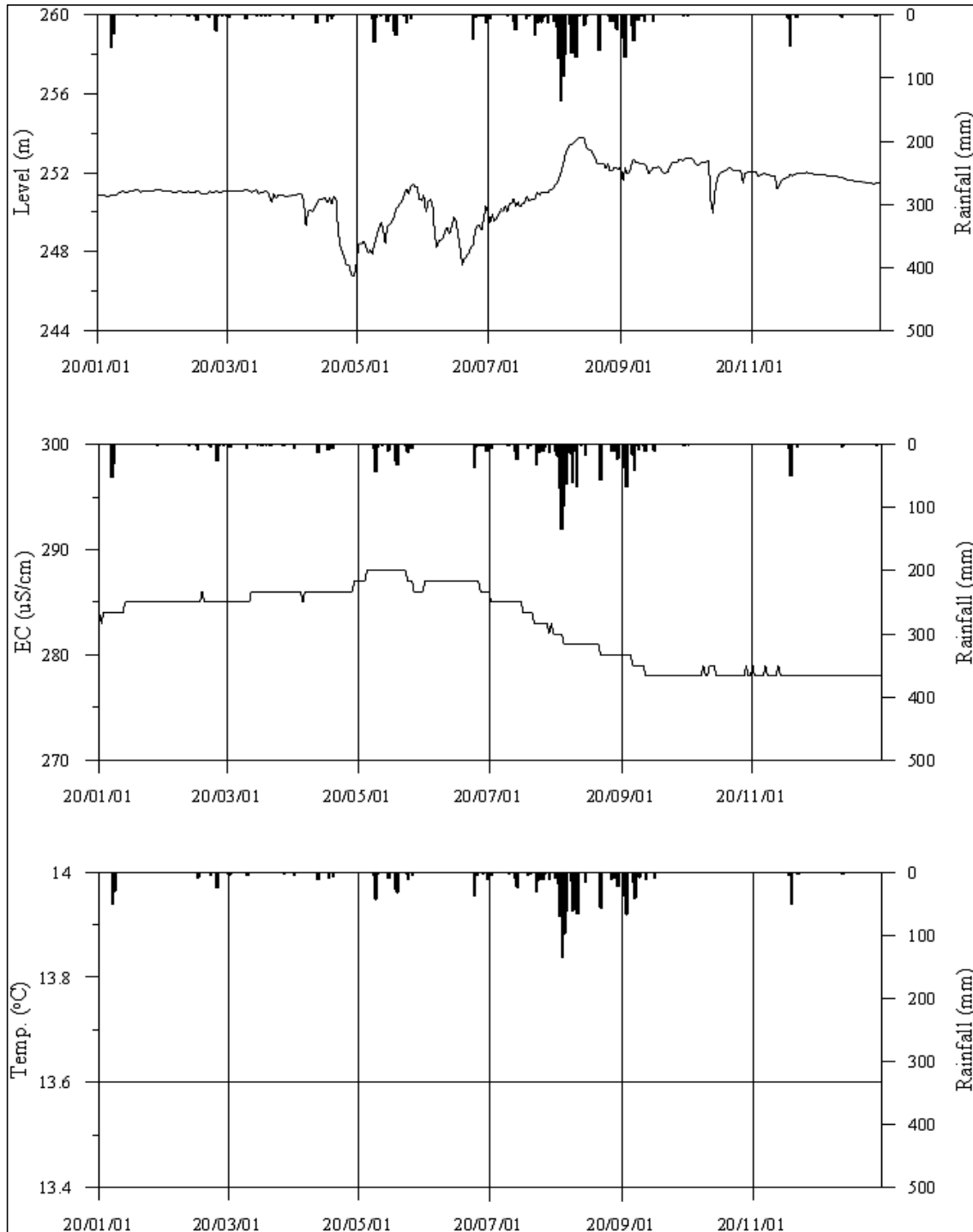
<양구3 관측공의 장기관측자료 (2020.1.1 ~ 2020.12.31)> (a)지하수위, (b)전기전도도, (c)수온
