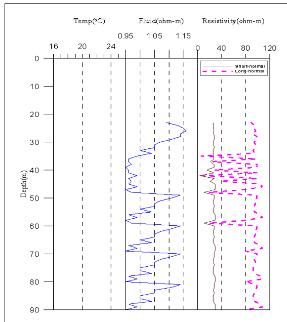
<청송6 관측공 물리검층>
