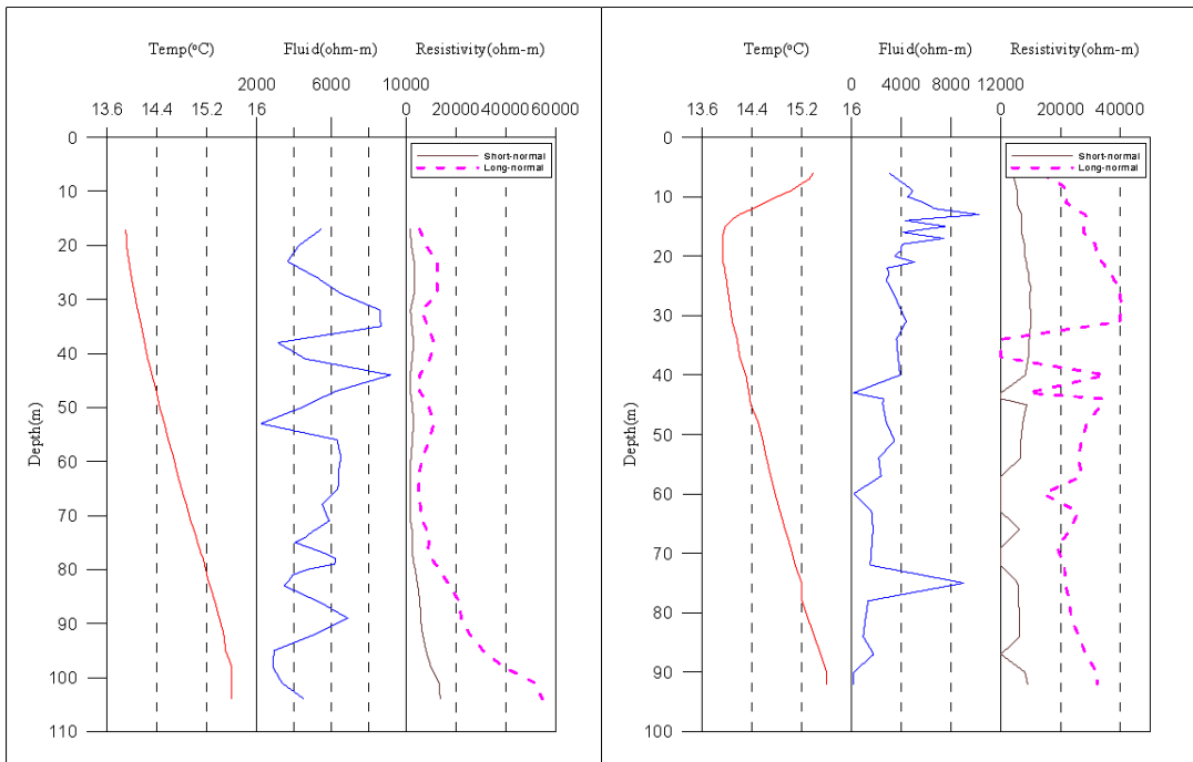
<여주7 관측공 물리검층>
