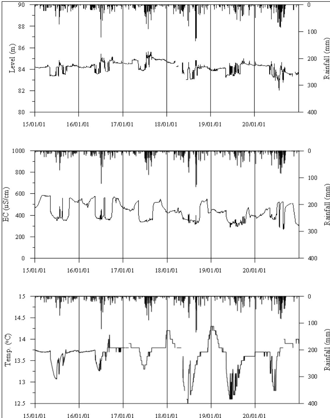
<충주1 관측공의 장기관측자료 (2015.1.1 ~ 2020.12.31)> (a)지하수위, (b)전기전도도, (c)수온
