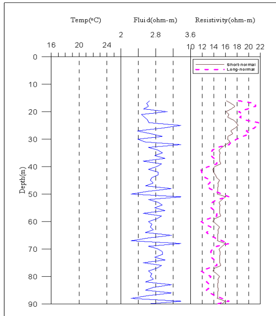
<의성10 관측공 물리검층>
