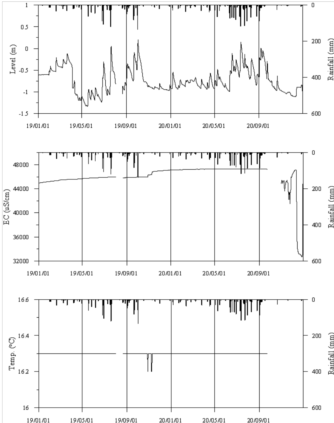
<고흥8 관측공의 장기관측자료 (2019.1.1~2020.12.31)> (a)지하수위, (b)전기전도도, (c)수온
