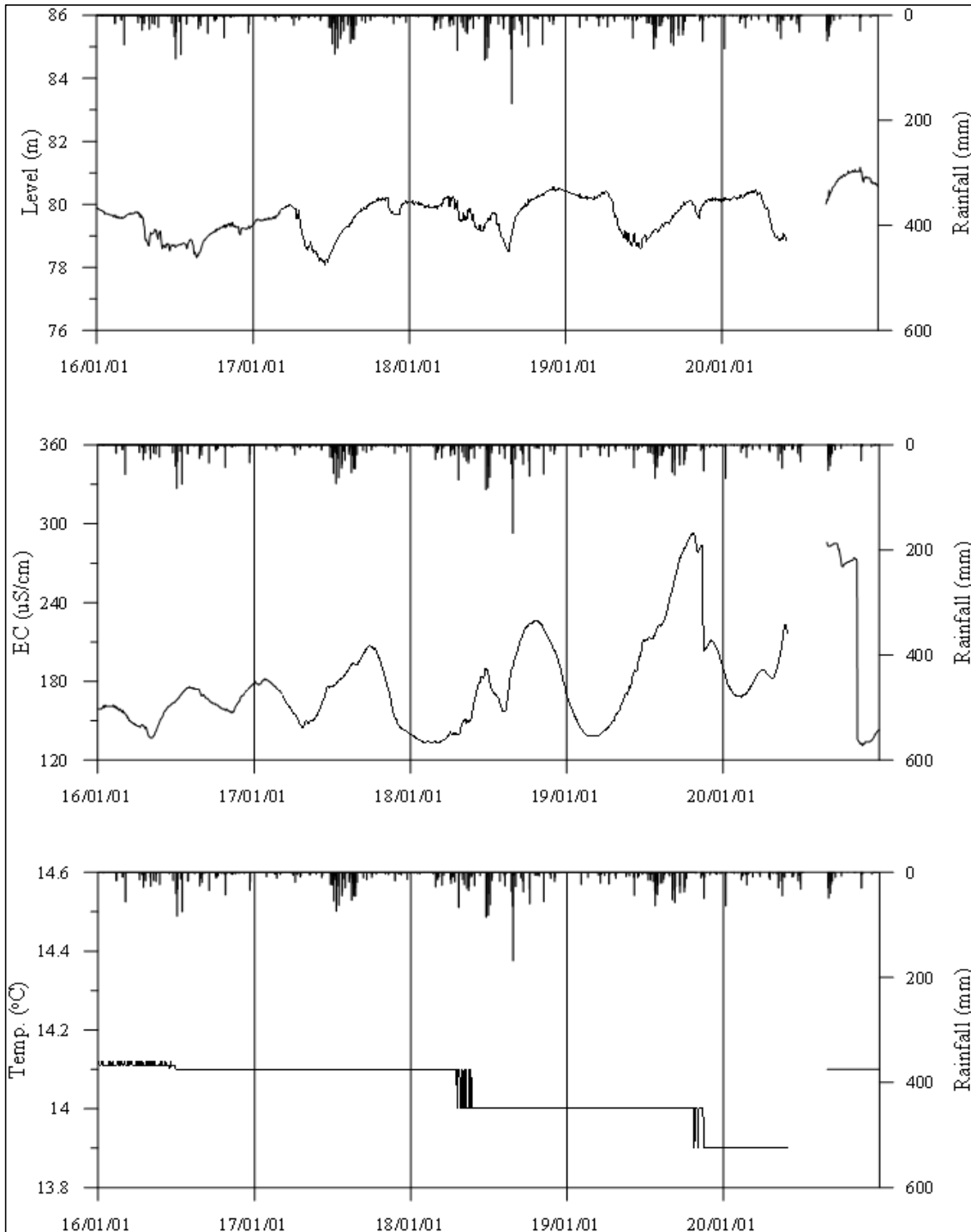
<이천4 관측공의 장기관측자료 (2016.1.1 ~ 2020.12.31)> (a)지하수위, (b)전기전도도, (c)수온
