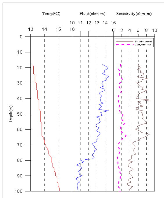
<안동8 관측공 물리검층>
