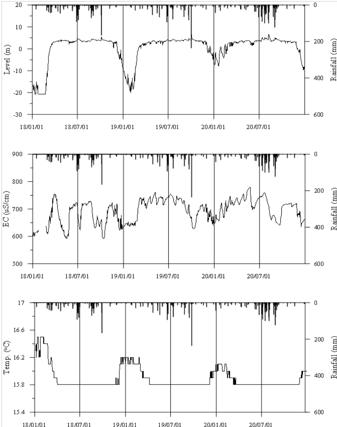
<의령1 관측공의 장기관측자료 (2018.1.1 ~ 2020.12.31)> (a)지하수위, (b)전기전도도, (c)수온
