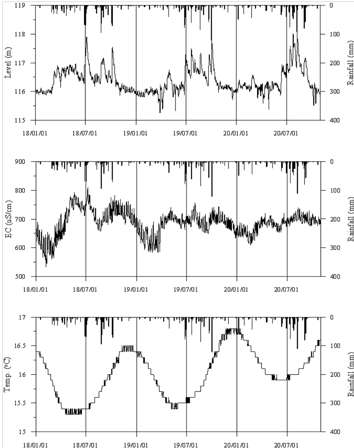
<영천5 관측공의 장기관측자료 (2018.1.1 ~ 2020.12.31)> (a)지하수위, (b)전기전도도, (c)수온
