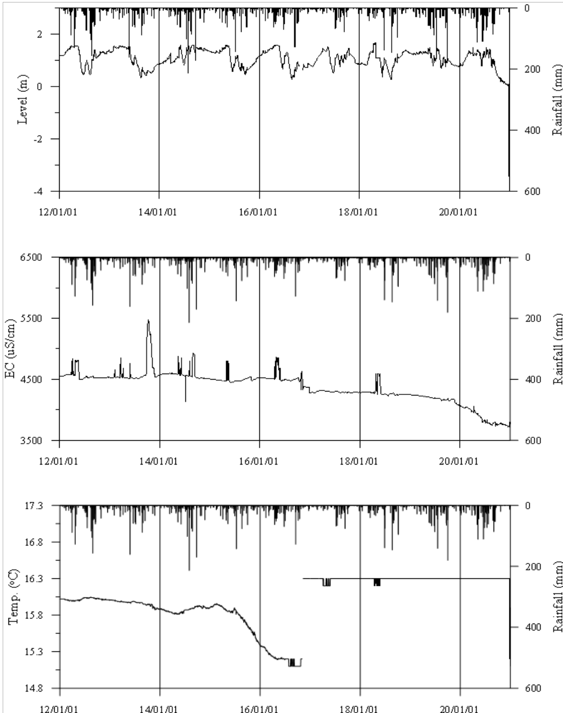
<장흥1 관측공의 장기관측자료 (2012.1.1 ~ 2020.12.31)> (a)지하수위, (b)전기전도도, (c)수온
