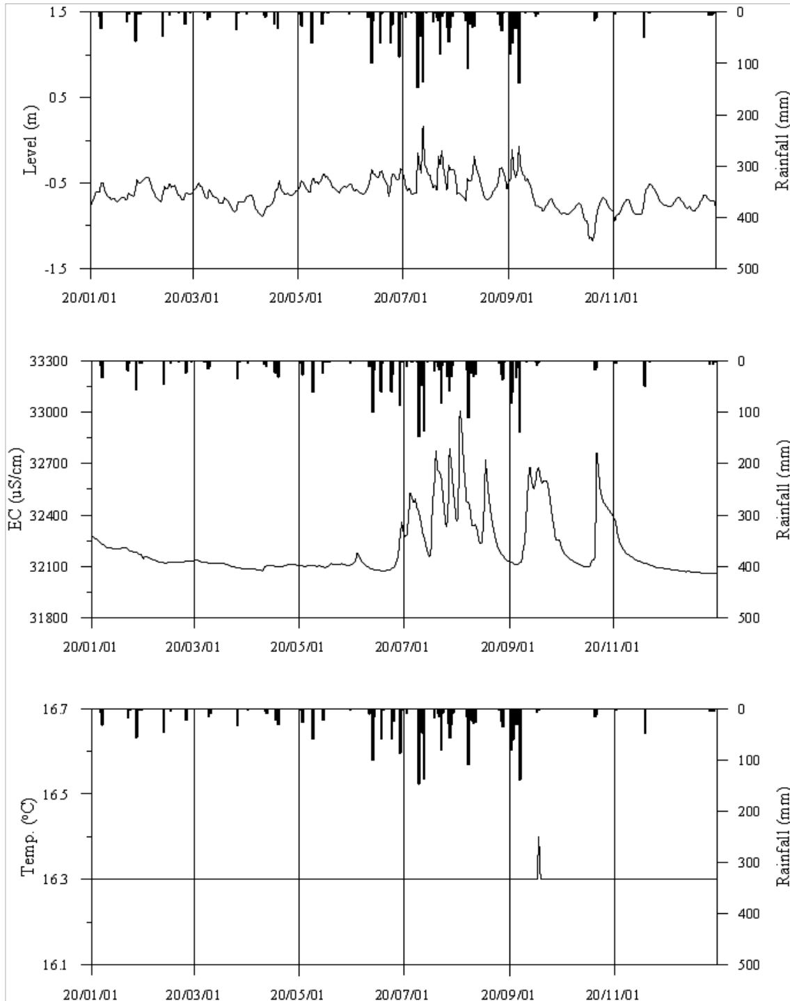
<경남고성2 관측공의 장기관측자료 (2020.1.1 ~ 2020.12.31)> (a)지하수위, (b)전기전도도, (c)수온
