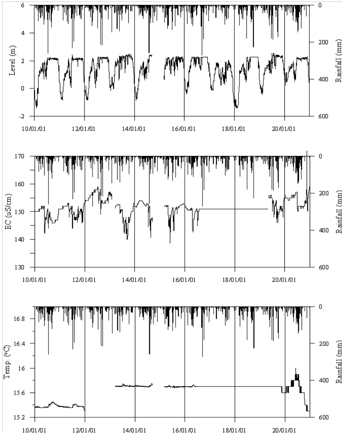
<하동2 관측공의 장기관측자료 (2010.1.1 ~ 2020.12.31)> (a)지하수위, (b)전기전도도, (c)수온
