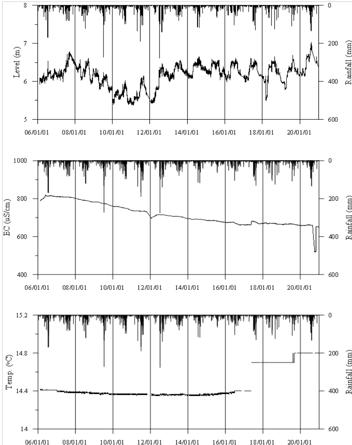
<화성4 관측공의 장기관측자료 (2006.1.1 ~ 2020.12.31)> (a)지하수위, (b)전기전도도, (c)수온
