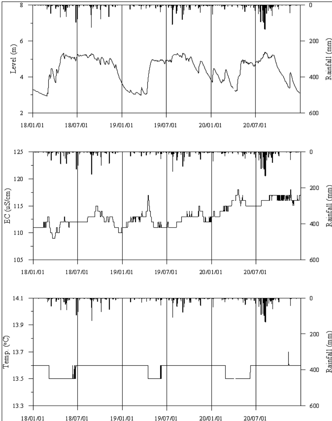
<평택4 관측공의 장기관측자료 (2018.1.1 ~ 2020.12.31)> (a)지하수위, (b)전기전도도, (c)수온
