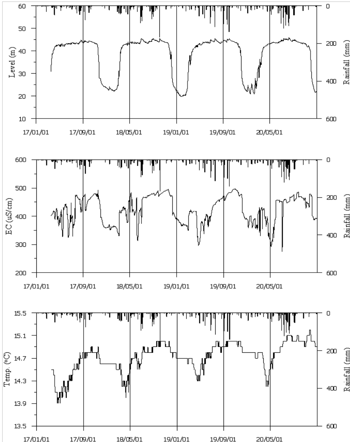
<진주2(신) 관측공의 이동설치 후 장기관측자료 (2017.1.1 ~ 2020.12.31)> (a)지하수위, (b)전기전도도, (c)수온
