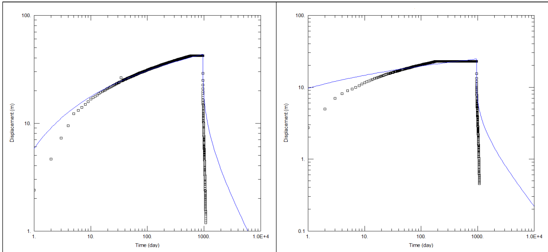
<영월7 관측공 양수시험>
