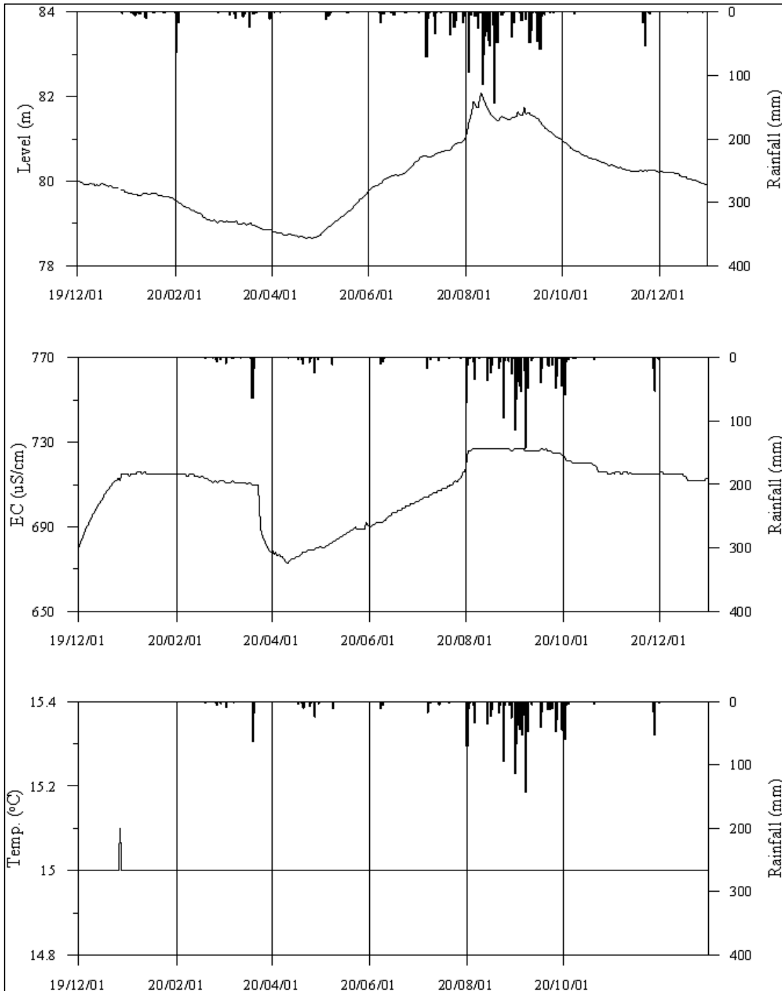
<양주2 관측공의 장기관측자료 (2019.12.1 ~ 2020.12.31)> (a)지하수위, (b)전기전도도, (c)수온
