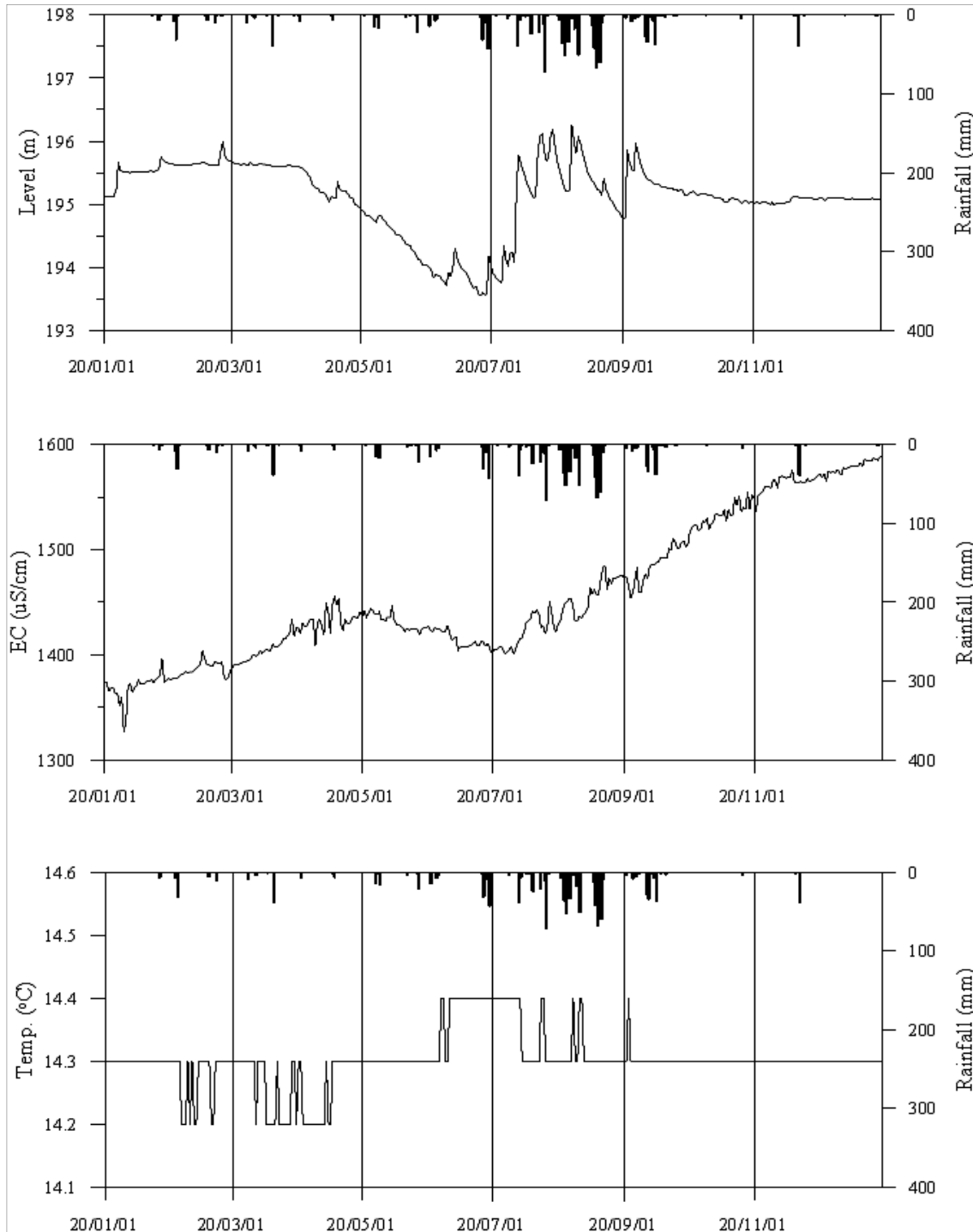
<의성10 관측공의 장기관측자료 (2020.1.1 ~ 2020.12.31.)> (a)지하수위, (b)전기전도도, (c)수온
