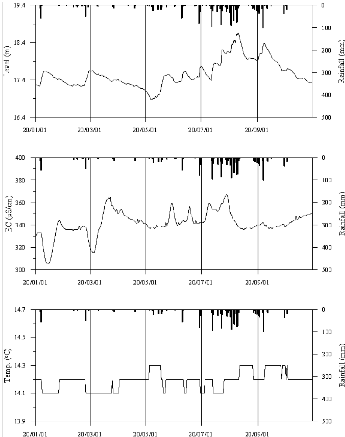
<홍성5 관측공의 장기관측자료 (2020.1.1 ~ 2020.10.31)> (a)지하수위, (b)전기전도도, (c)수온
