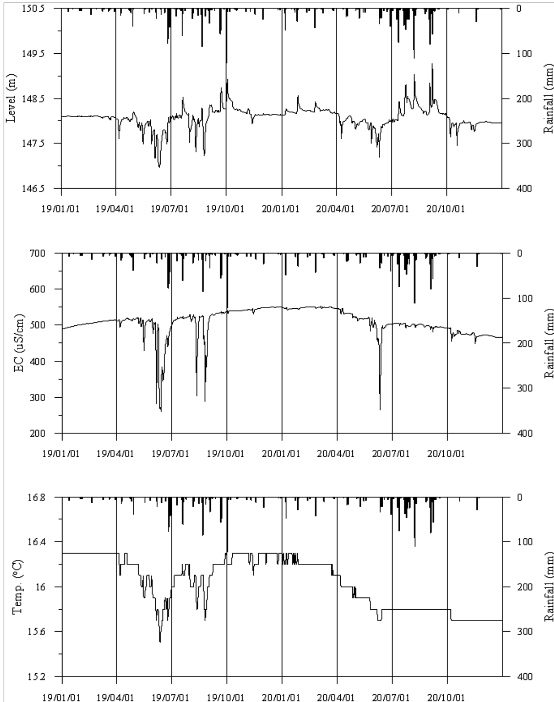
<영천7 관측공의 장기관측자료 (2019.1.1 ~ 2020.12.31)> (a)지하수위, (b)전기전도도, (c)수온
