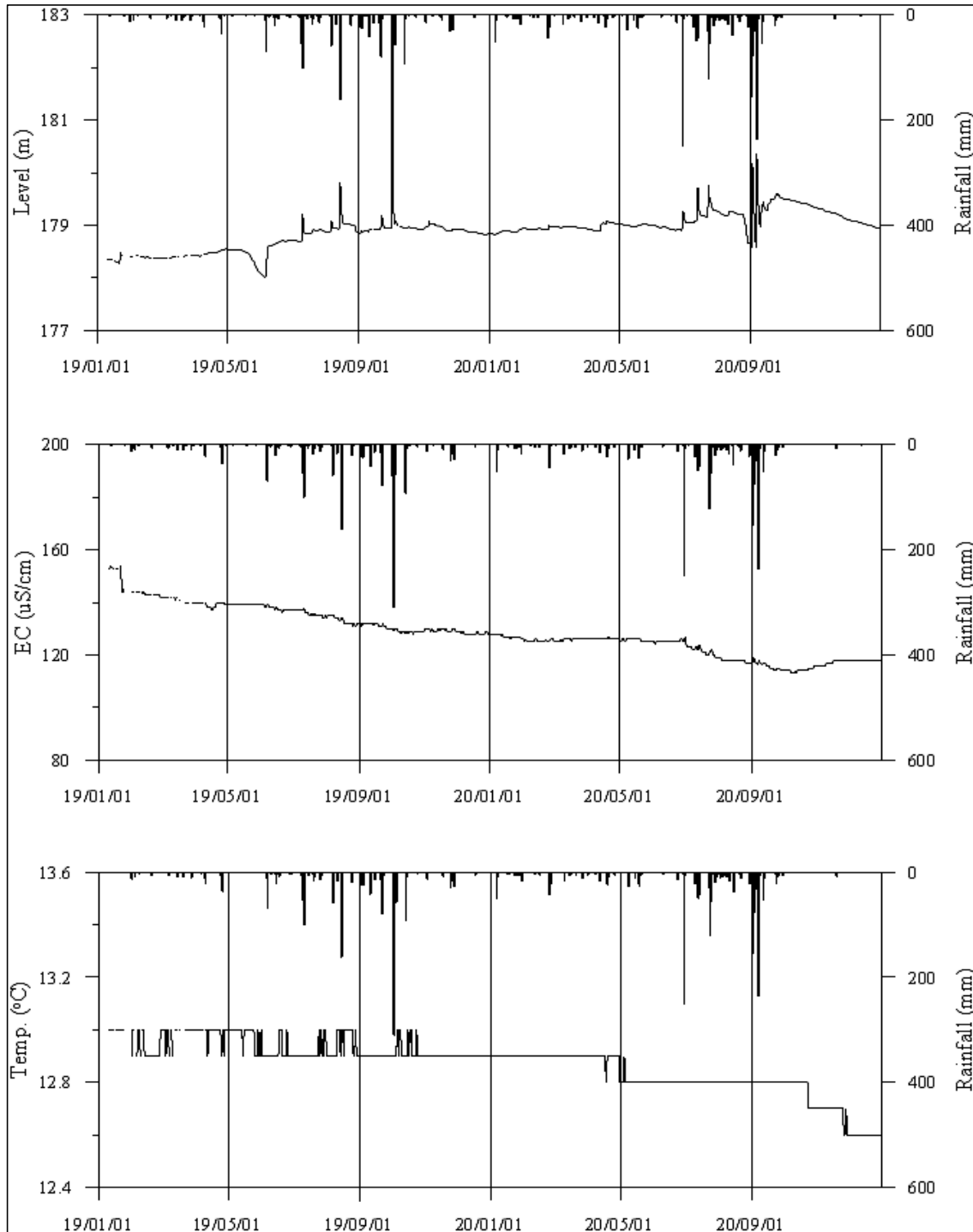
<강릉5 관측공의 장기관측자료 (2019.1.1 ~ 2020.12.31)> (a)지하수위, (b)전기전도도, (c)수온
