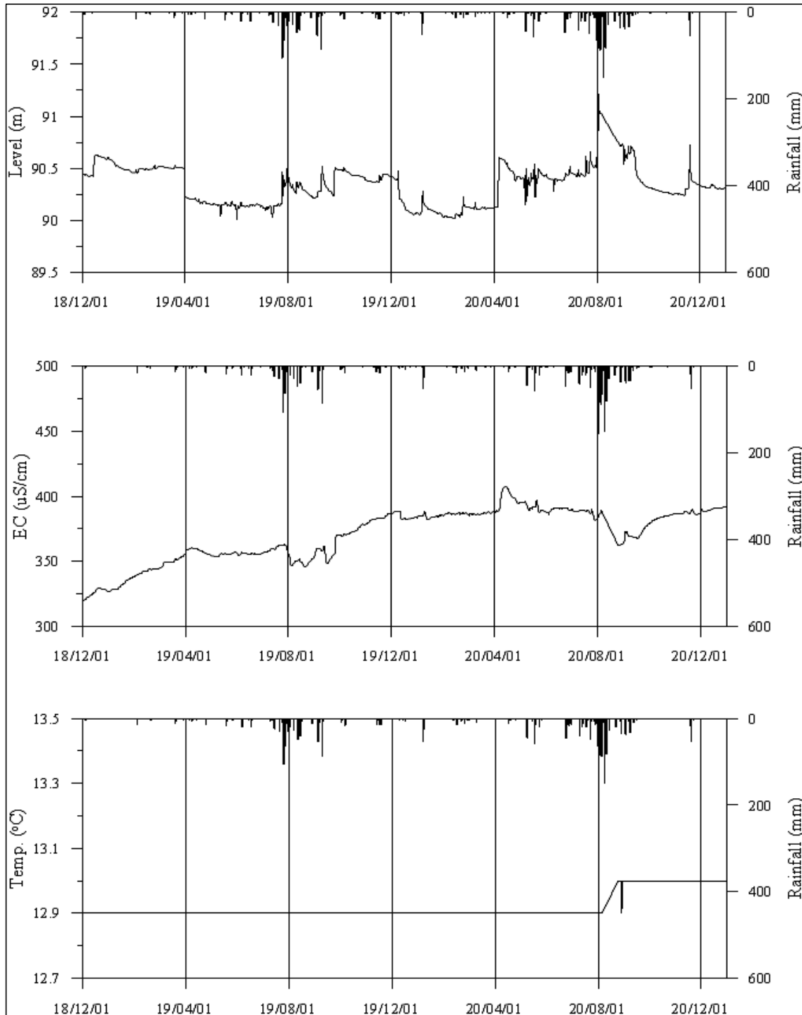
<포천4 관측공의 장기관측자료 (2018.12.1 ~ 2020.12.31)> (a)지하수위, (b)전기전도도, (c)수온
