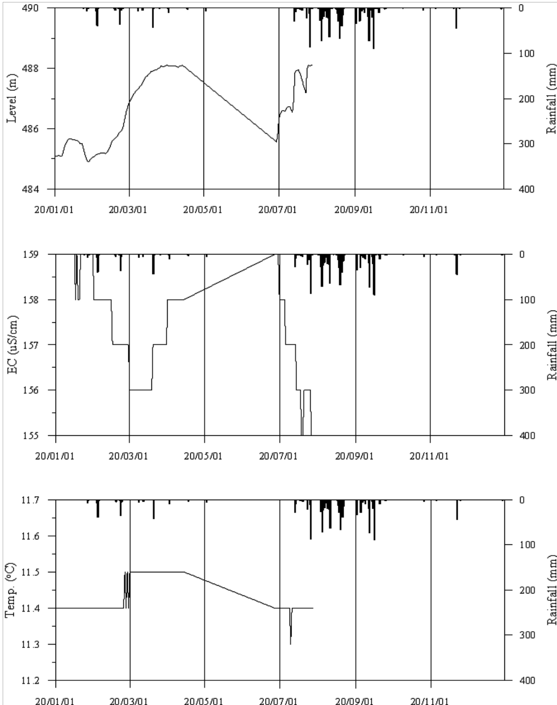
<영양1 관측공의 장기관측자료 (2020.1.1 ~ 2020.12.31.)> (a)지하수위, (b)전기전도도, (c)수온
