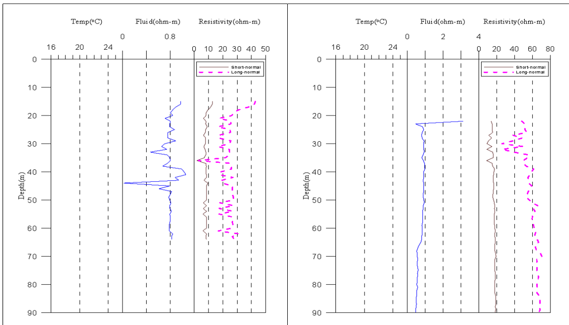
<영양3 관측공 물리검층>
