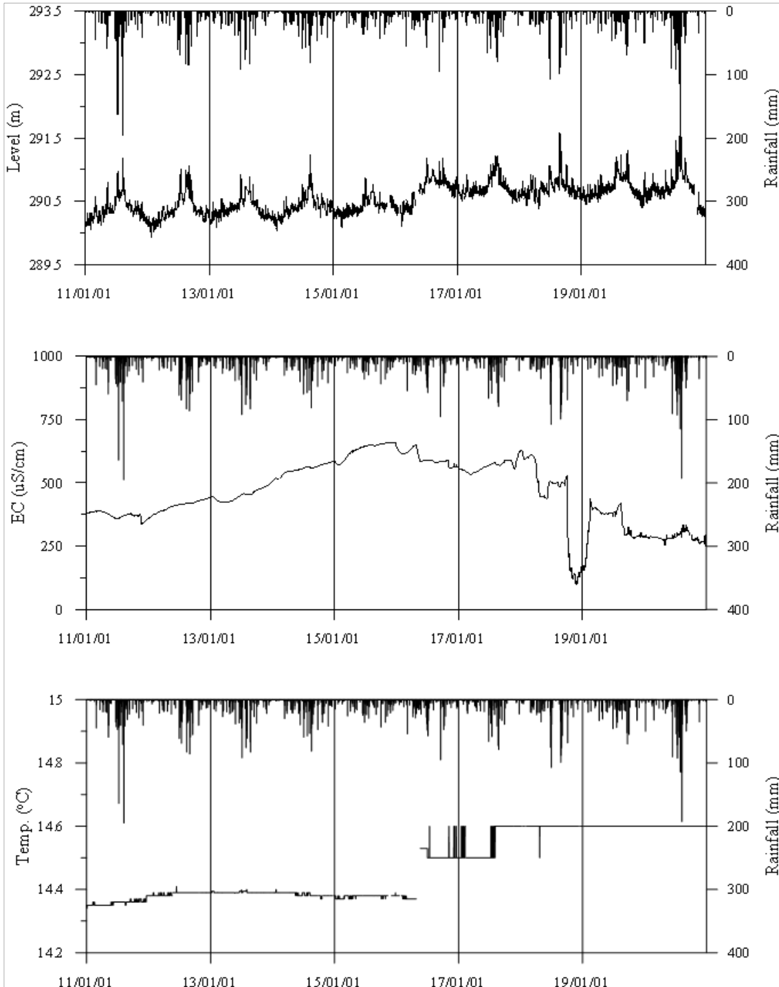
<진안1 관측공의 장기관측자료 (2011.1.1 ~ 2020.12.31)> (a)지하수위, (b)전기전도도, (c)수온
