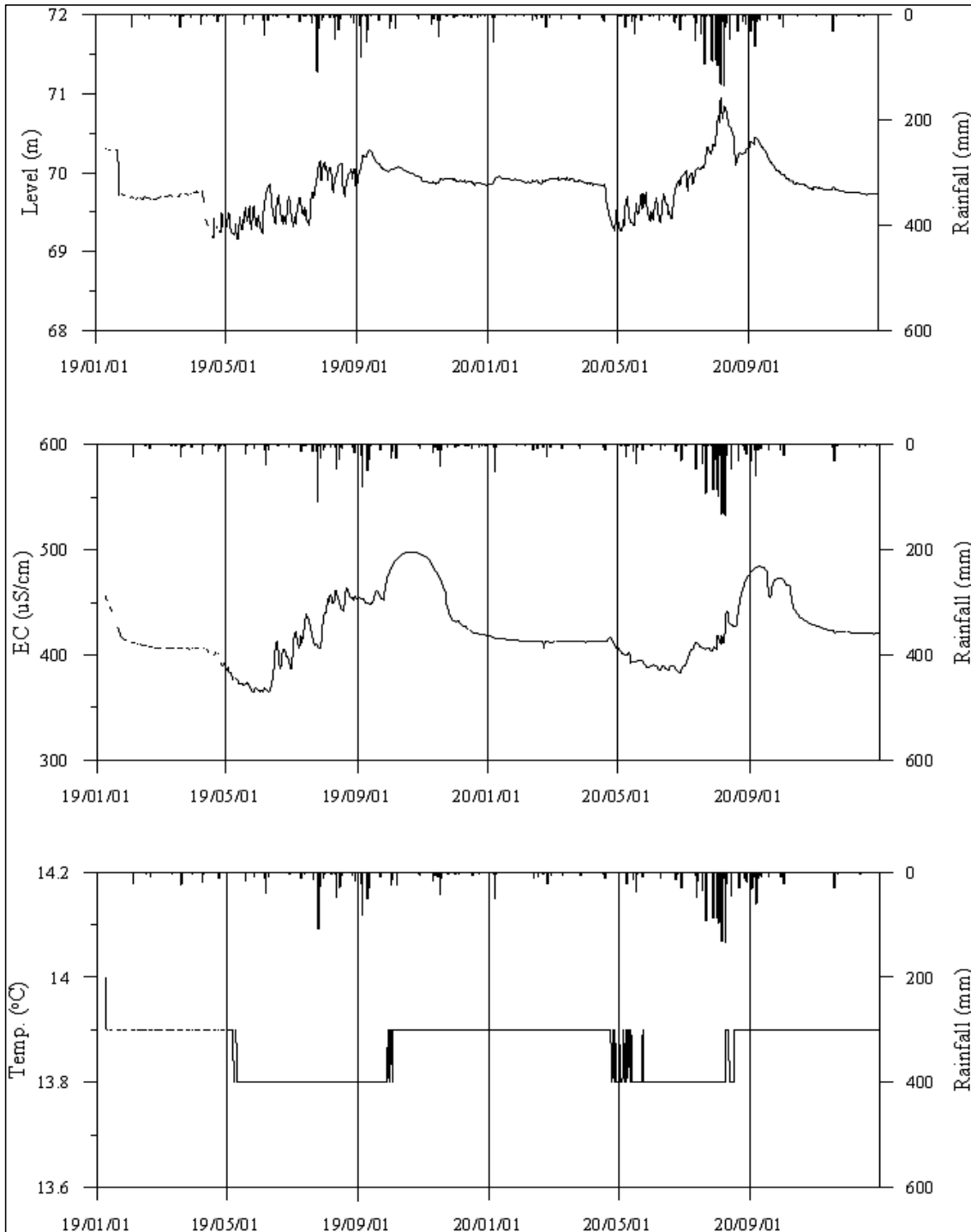
<용인5 관측공의 장기관측자료 (2019.1.1 ~ 2020.12.31)> (a)지하수위, (b)전기전도도, (c)수온
