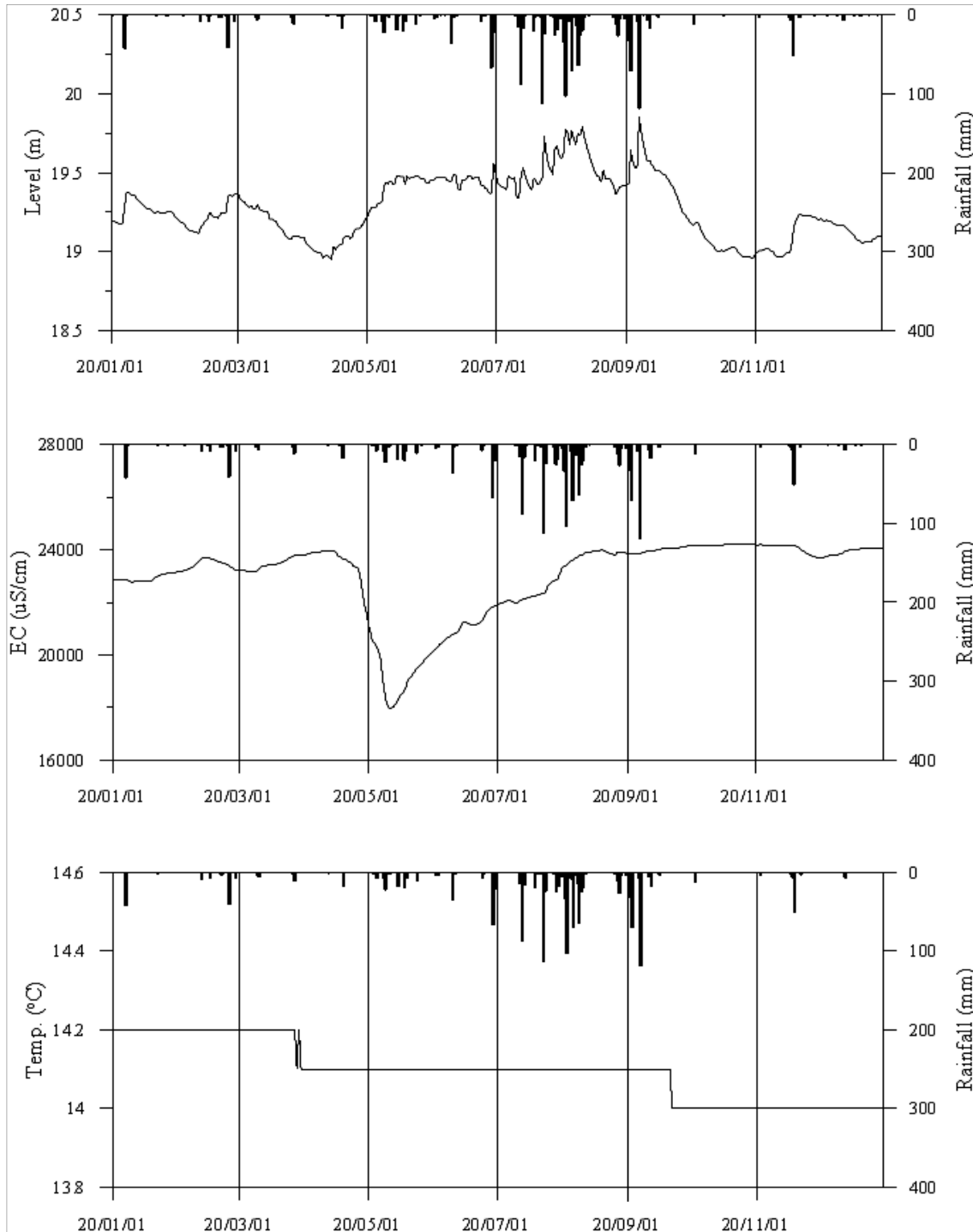
<당진3 관측공의 장기관측자료 (2020.1.1 ~ 2020.12.31)> (a)지하수위, (b)전기전도도, (c)수온
