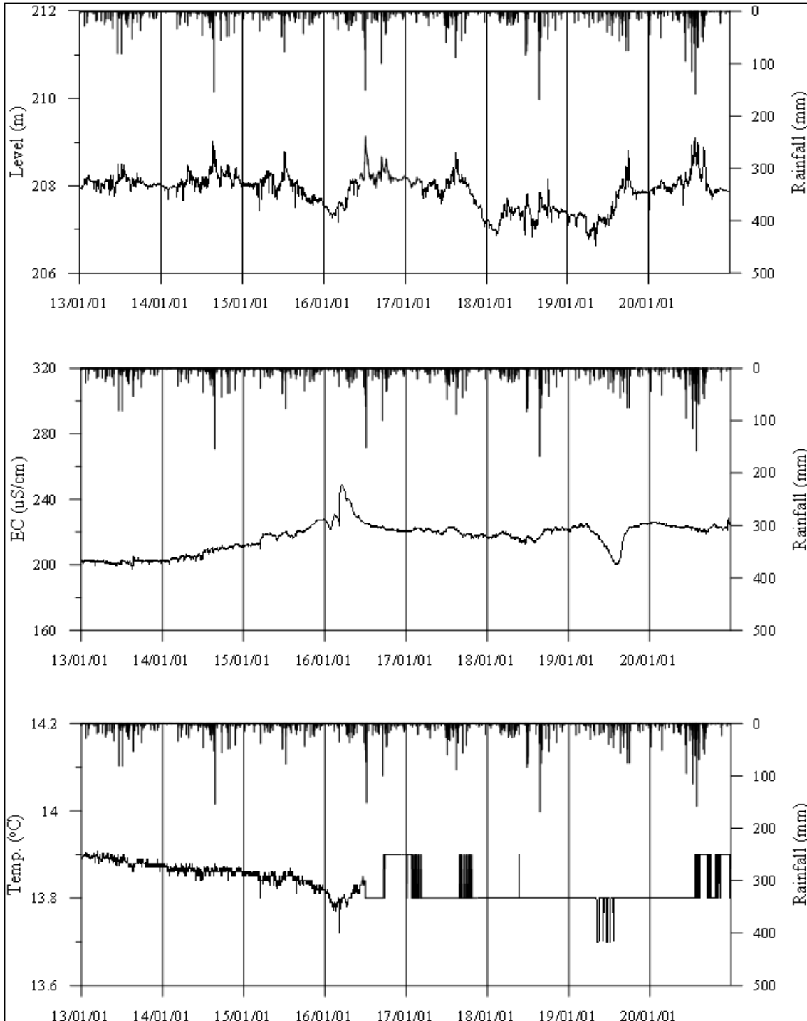
<영동1 관측공의 장기관측자료 (2013.1.1 ~ 2020.12.31)> (a)지하수위, (b)전기전도도, (c)수온
