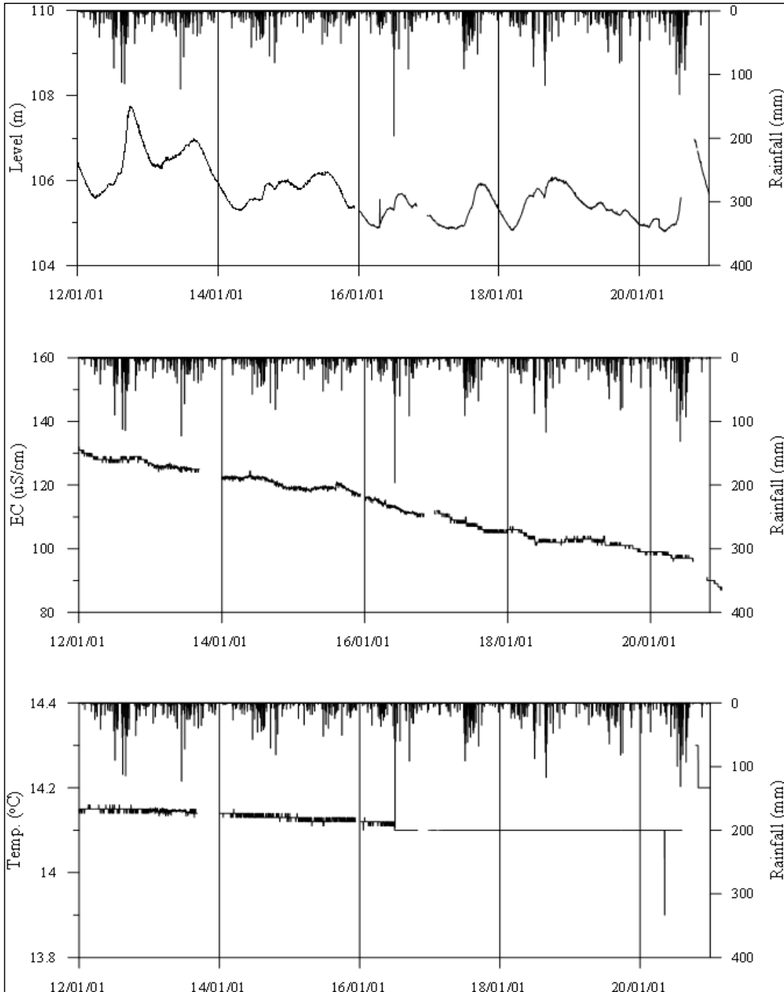
<옥천1 관측공의 장기관측자료 (2012.1.1 ~ 2020.12.31)> (a)지하수위, (b)전기전도도, (c)수온
