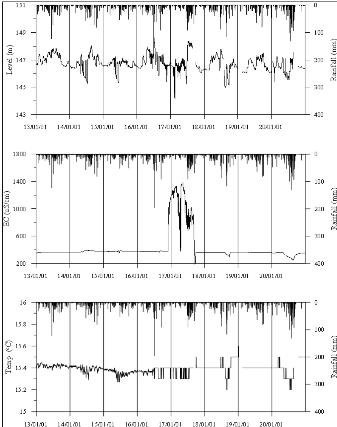
<보은2 관측공의 장기관측자료 (2013.1.1 ~ 2020.12.31)> (a)지하수위, (b)전기전도도, (c)수온
