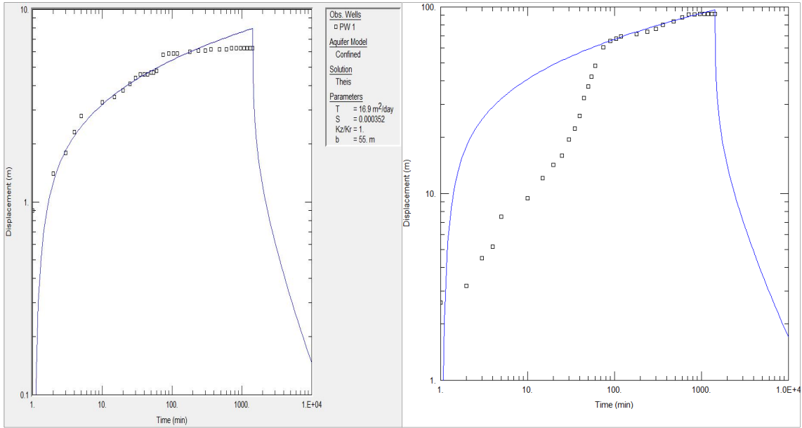
<영주2 관측공 양수시험>
