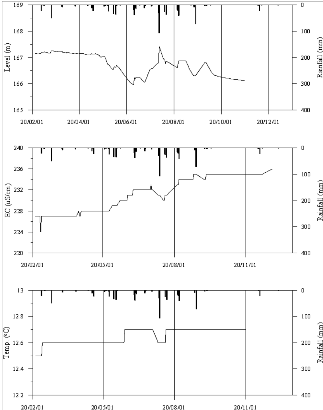
<상주9 관측공의 장기관측자료 (2020.2.1 ~ 2020.12.31)> (a)지하수위, (b)전기전도도, (c)수온
