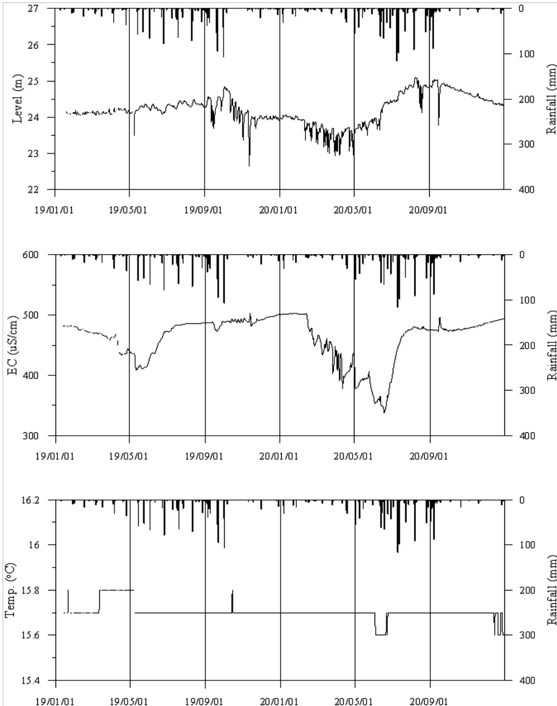
<무안8 관측공의 장기관측자료 (2019.1.1 ~ 2020.12.31)> (a)지하수위, (b)전기전도도, (c)수온
