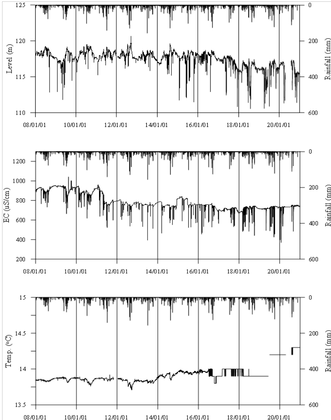
<영천3 관측공의 장기관측자료 (2008.1.1 ~ 2020.12.31)> (a)지하수위, (b)전기전도도, (c)수온
