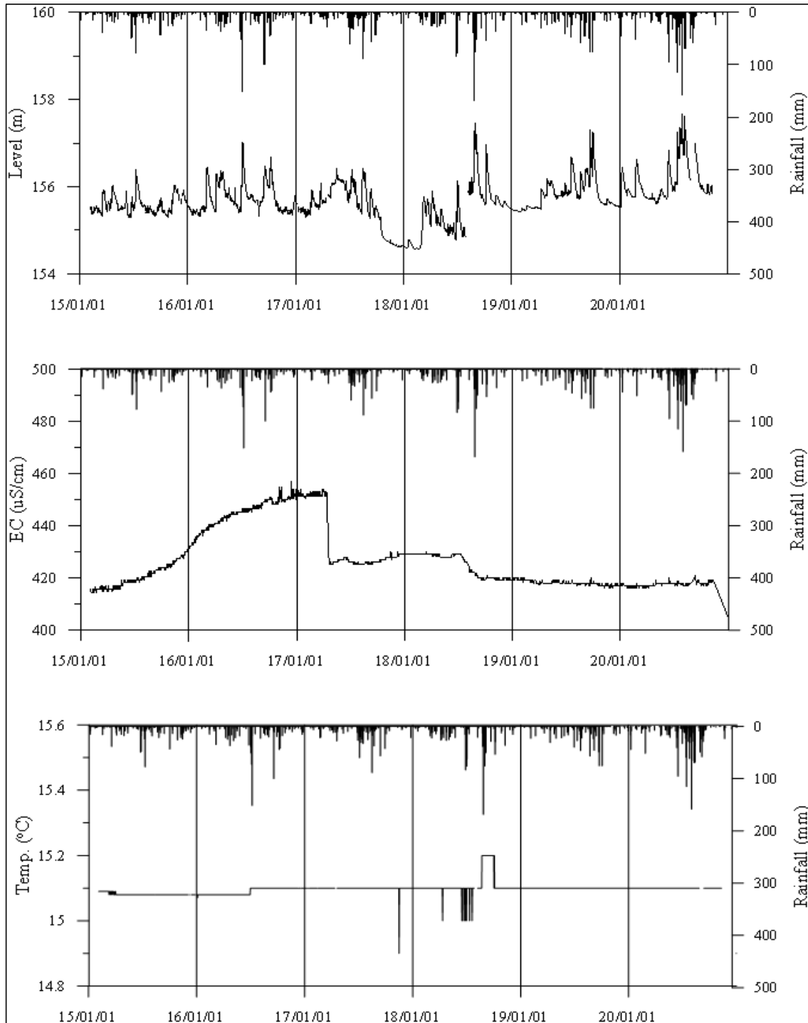
<영동3 관측공의 장기관측자료 (2015.1.1 ~ 2020.12.31)> (a)지하수위, (b)전기전도도, (c)수온
