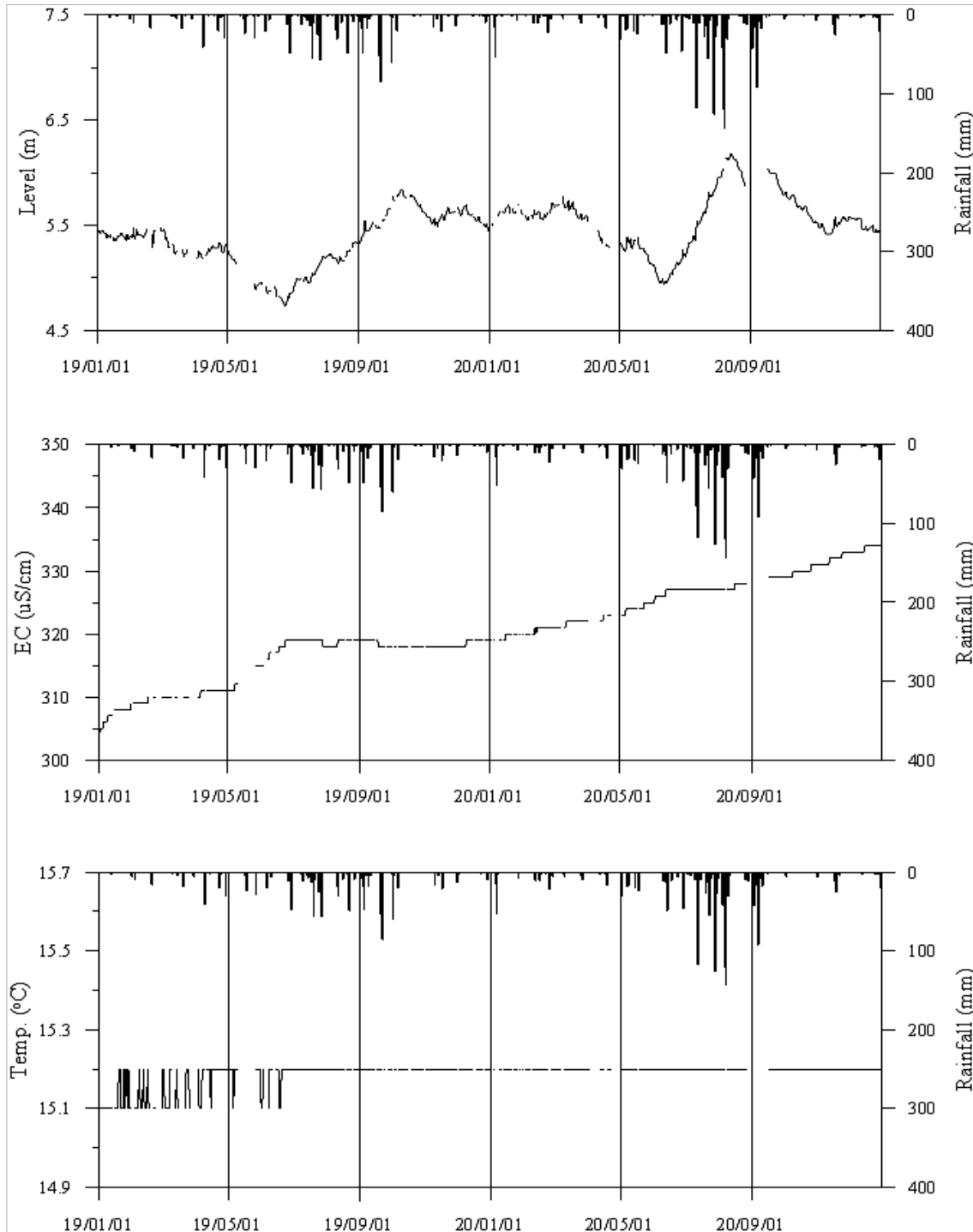
<부안2(신) 관측공의 장기관측자료 (2019.1.1 ~ 2020.12.31)> (a)지하수위, (b)전기전도도, (c)수온
