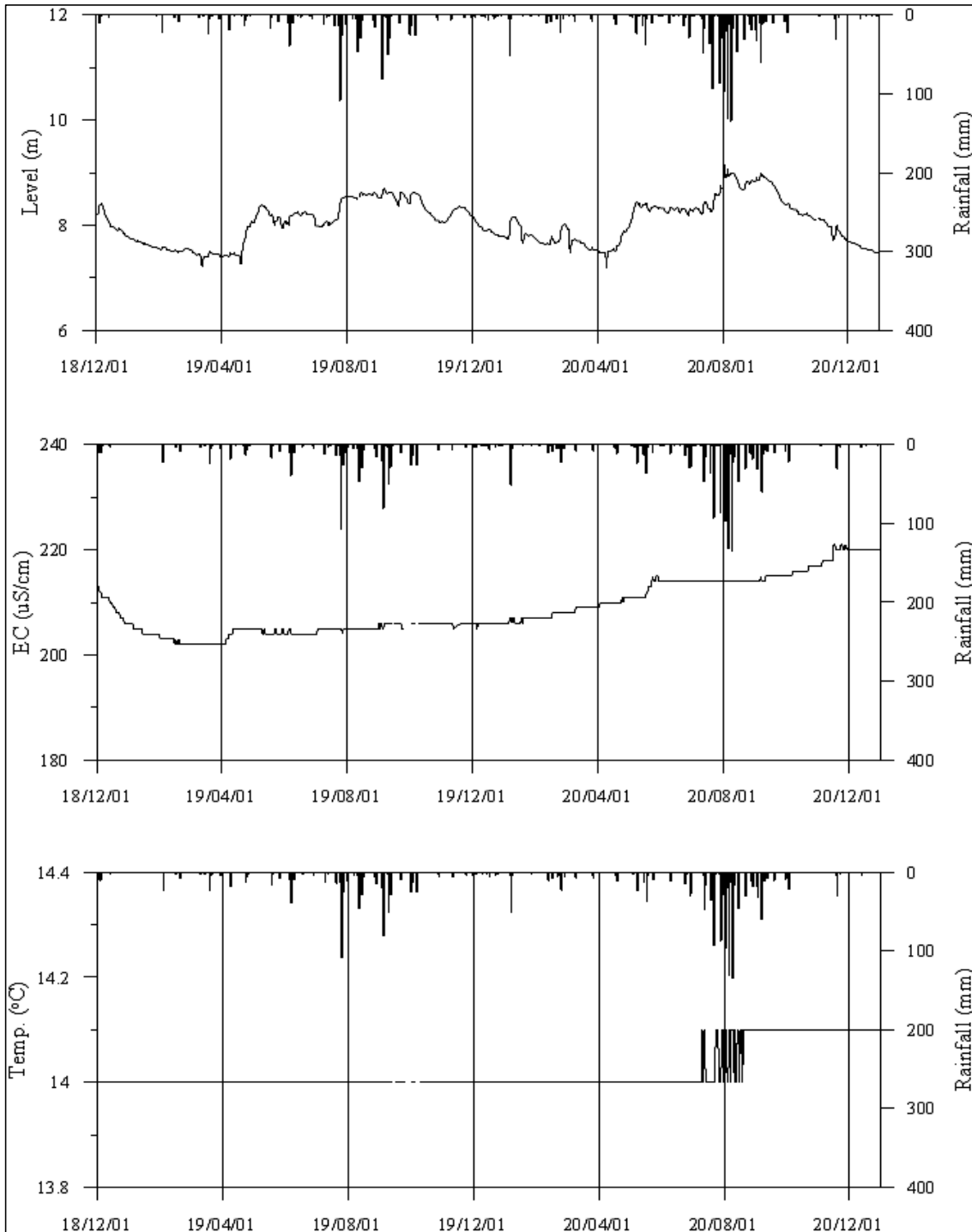
<안성5 관측공의 장기관측자료 (2018.12.1 ~ 2020.12.31)> (a)지하수위, (b)전기전도도, (c)수온
