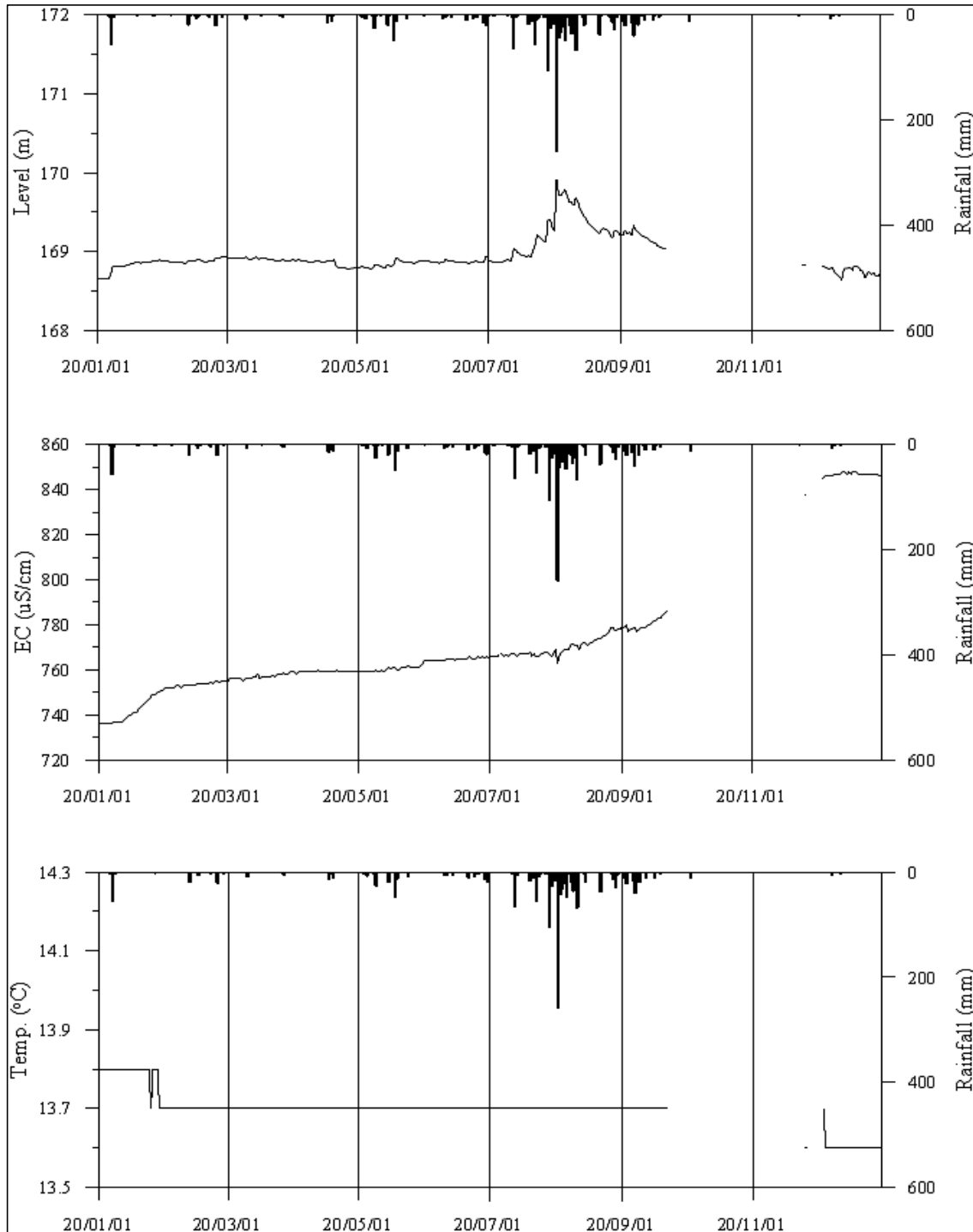
<제천3 관측공의 장기관측자료 (2020.1.1 ~ 2020.12.31)> (a)지하수위, (b)전기전도도, (c)수온
