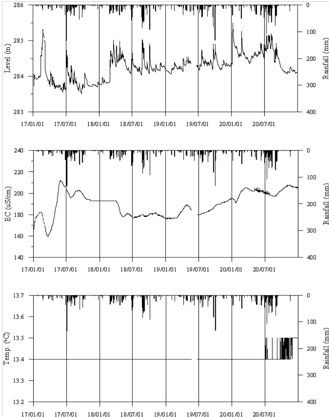
<상주6 관측공의 장기관측자료 (2016.1.1 ~ 2020.12.31)> (a)지하수위, (b)전기전도도, (c)수온
