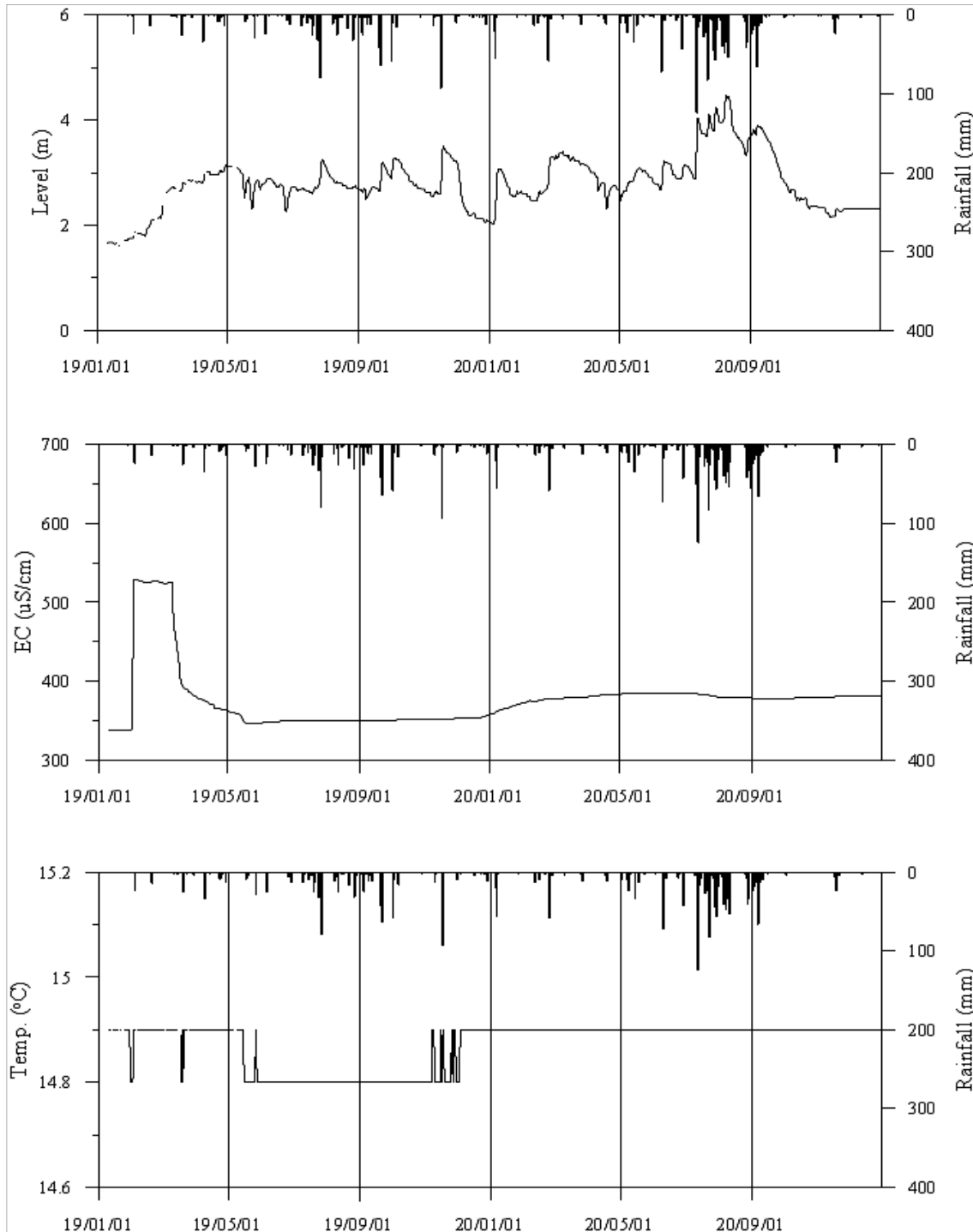
<부여5 관측공의 장기관측자료 (2019.1.1 ~ 2020.12.31)> (a)지하수위, (b)전기전도도, (c)수온
