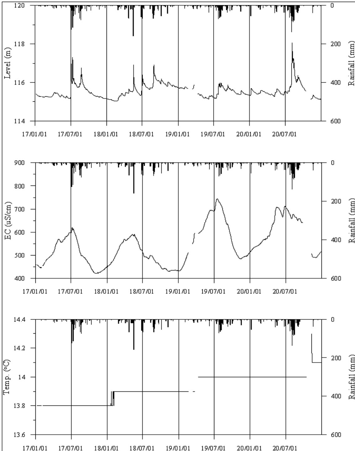
<홍천4 관측공의 장기관측자료 (2017.1.1 ~ 2020.12.31)> (a)지하수위, (b)전기전도도, (c)수온
