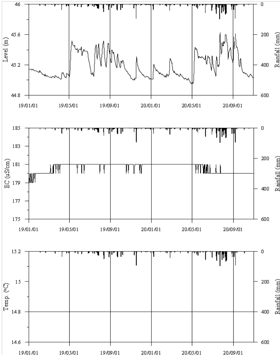
<보령4 관측공의 장기관측자료 (2019.1.1 ~ 2020.12.31)> (a)지하수위, (b)전기전도도, (c)수온
