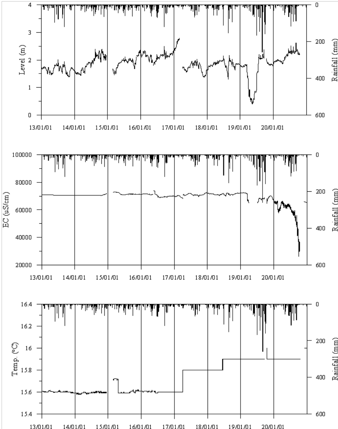
<신안1 관측공의 장기관측자료 (2013.1.1~2020.12.31)> (a)지하수위, (b)전기전도도, (c)수온
