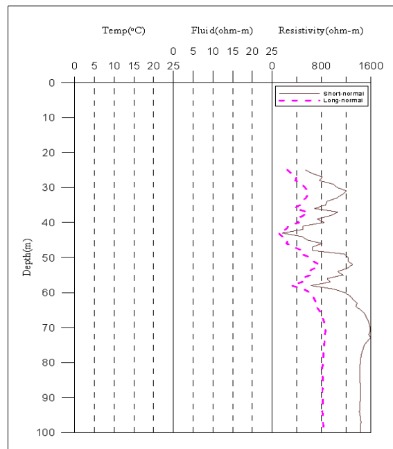
<기장3 관측공 물리검층>
