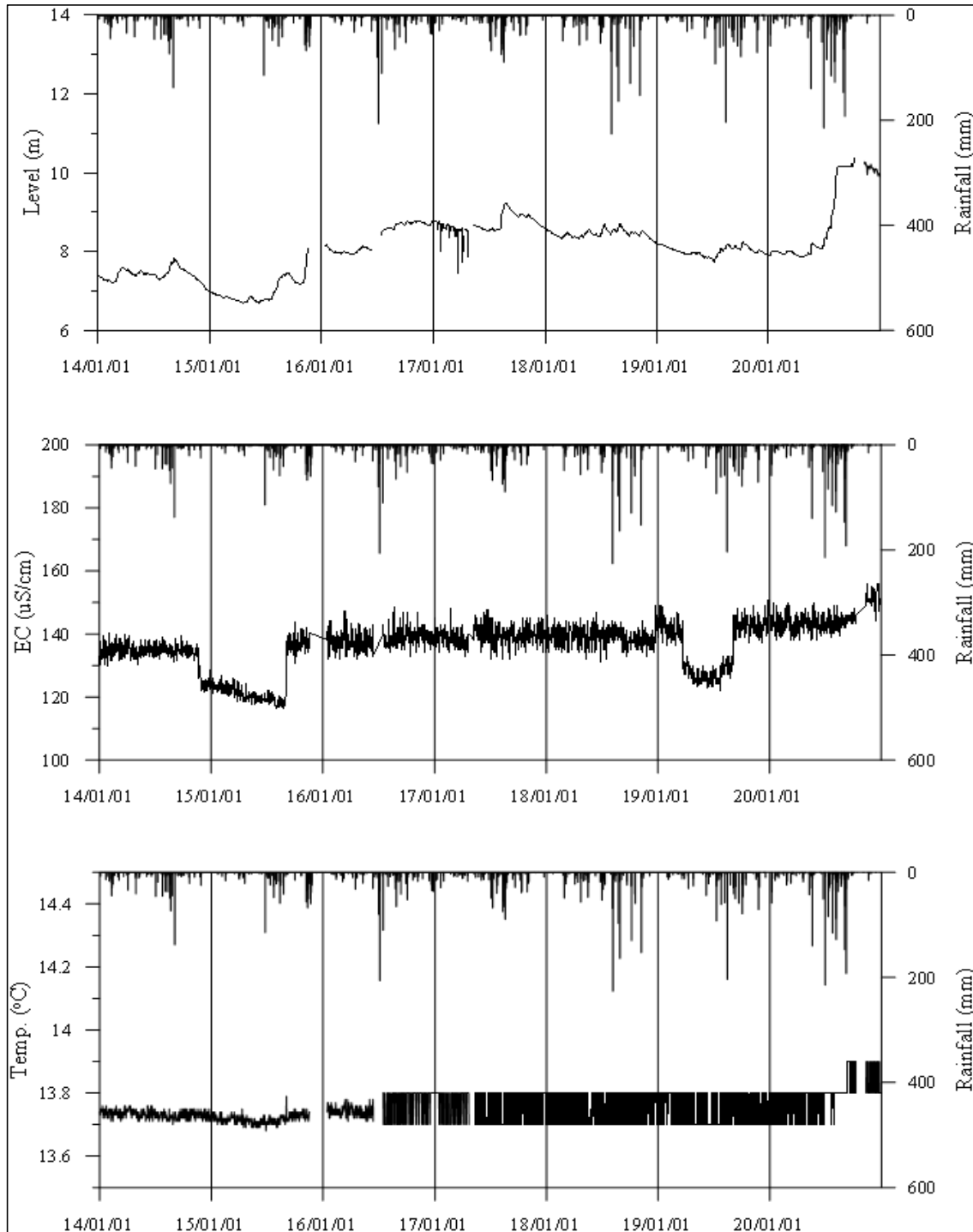
<고성2 관측공의 장기관측자료 (2014.1.1 ~ 2020.12.31)> (a)지하수위, (b)전기전도도, (c)수온
