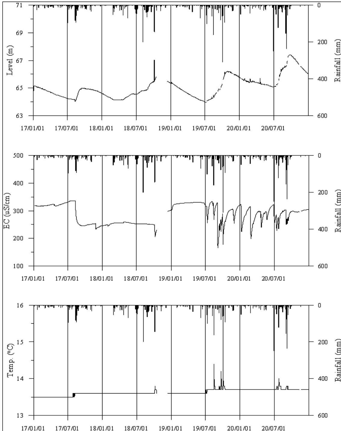
<강릉4 관측공의 장기관측자료 (2017.1.1 ~ 2020.12.31)> (a)지하수위, (b)전기전도도, (c)수온
