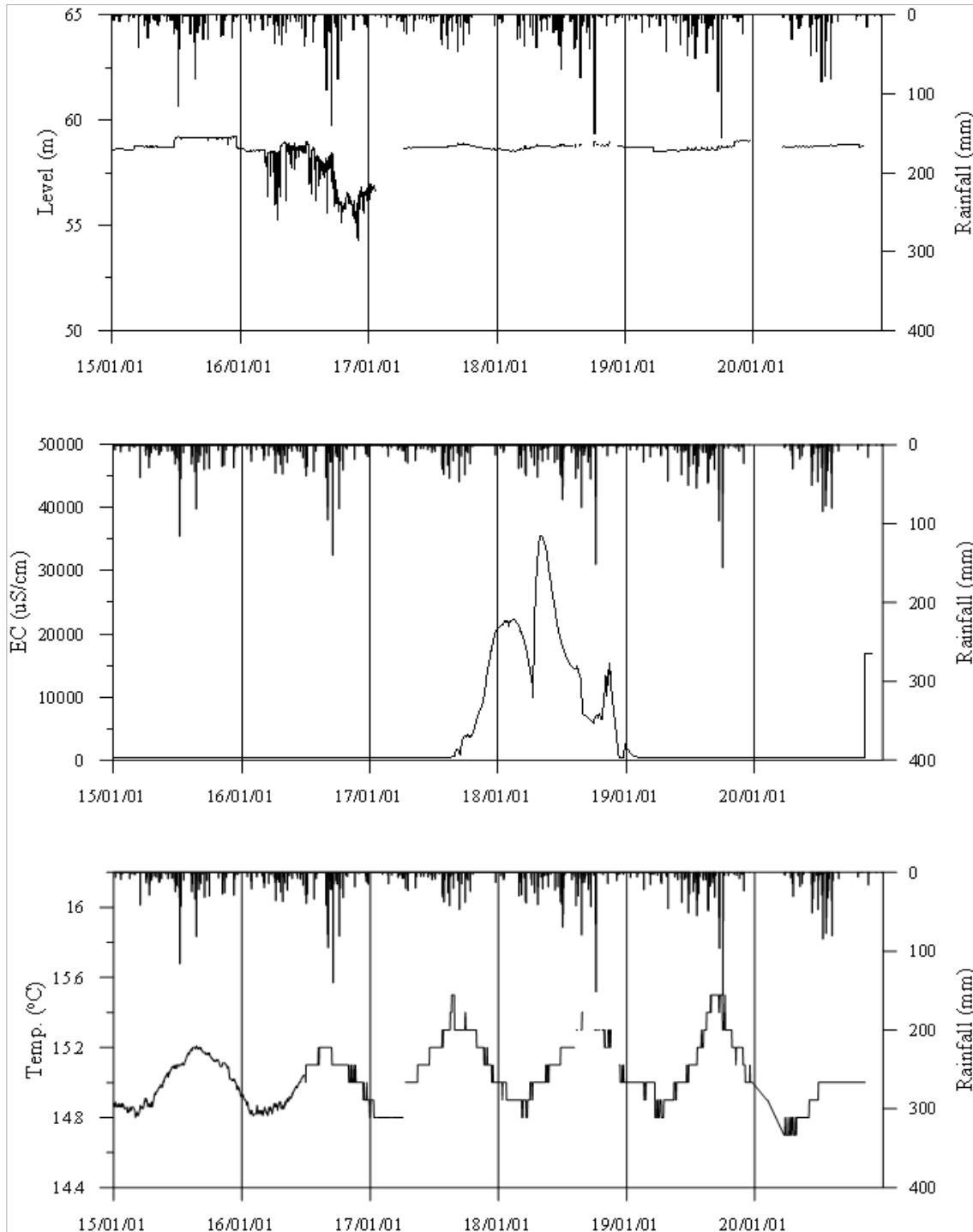
<경주2 관측공의 장기관측자료 (2015.1.1 ~ 2020.12.31)> (a)지하수위, (b)전기전도도, (c)수온
