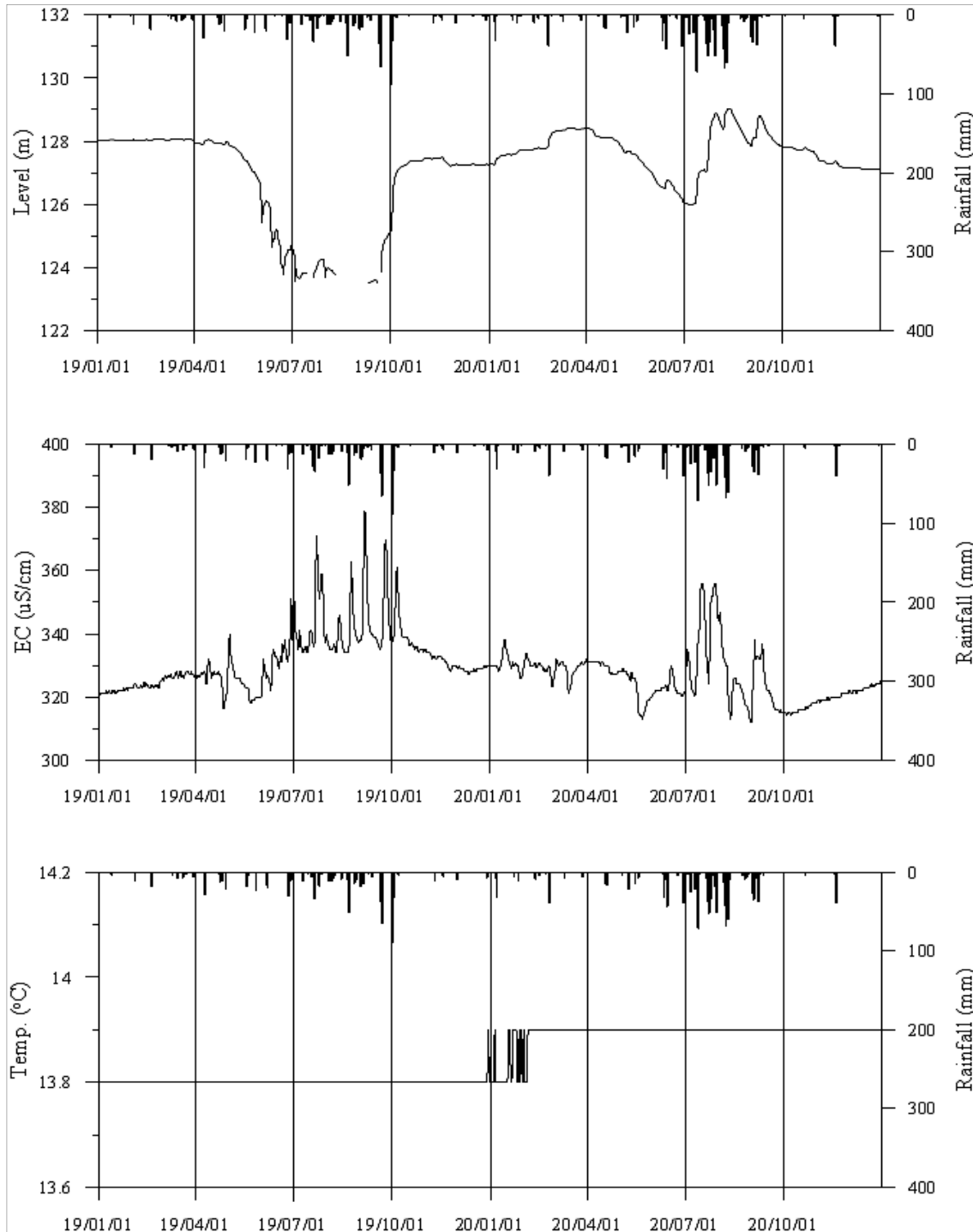
<의성6 관측공의 장기관측자료 (2019.1.1 ~ 2020.12.31.)> (a)지하수위, (b)전기전도도, (c)수온
