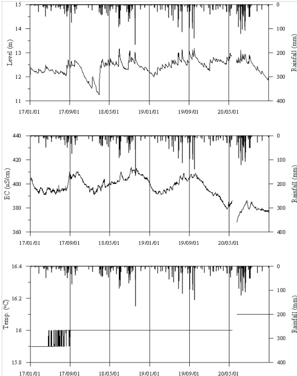
<사천3 관측공의 장기관측자료 (2017.1.1 ~ 2020.12.31)> (a)지하수위, (b)전기전도도, (c)수온
