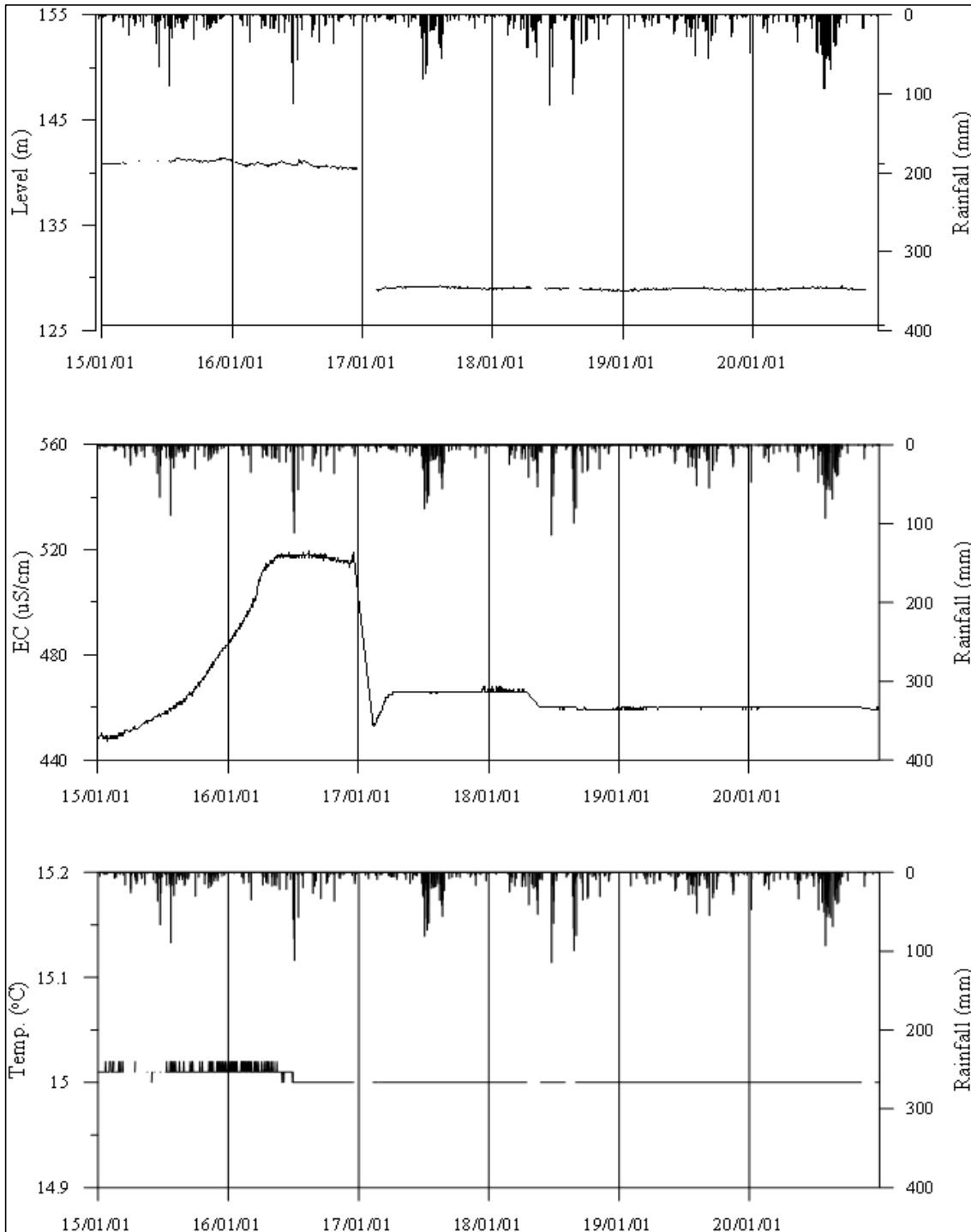
<황성3 관측공의 장기관측자료 (2015.1.1 ~ 2020.12.31)> (a)지하수위, (b)전기전도도, (c)수온
