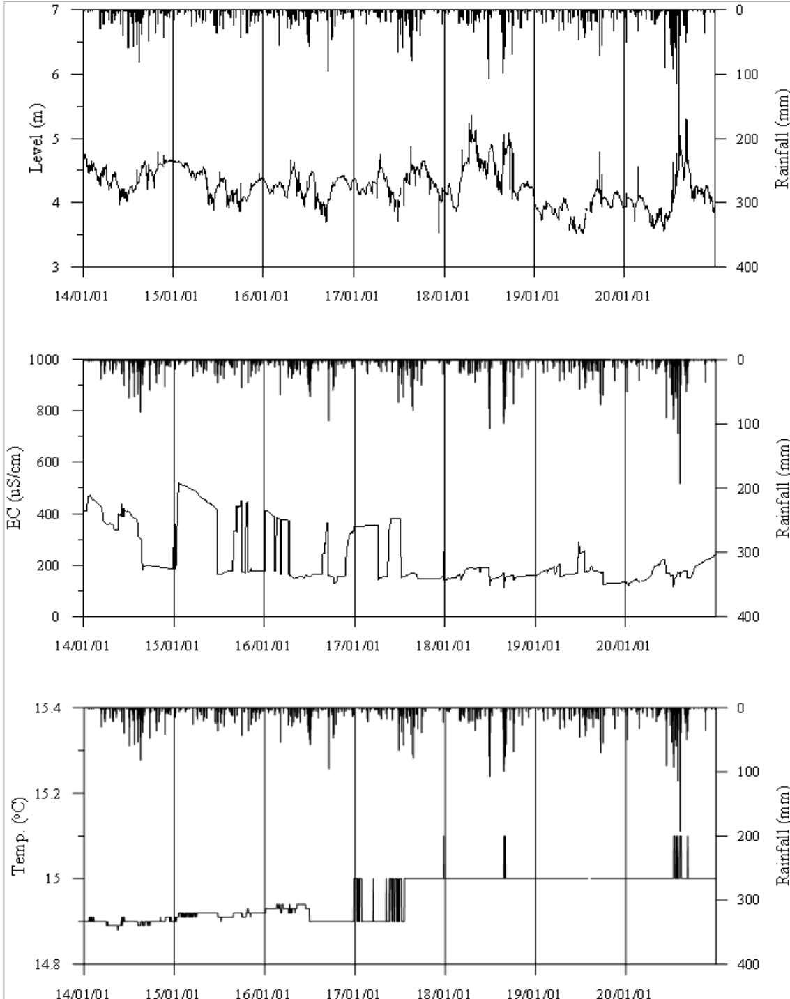
<익산1 관측공의 장기관측자료 (2014.1.1 ~ 2020.12.31)>
