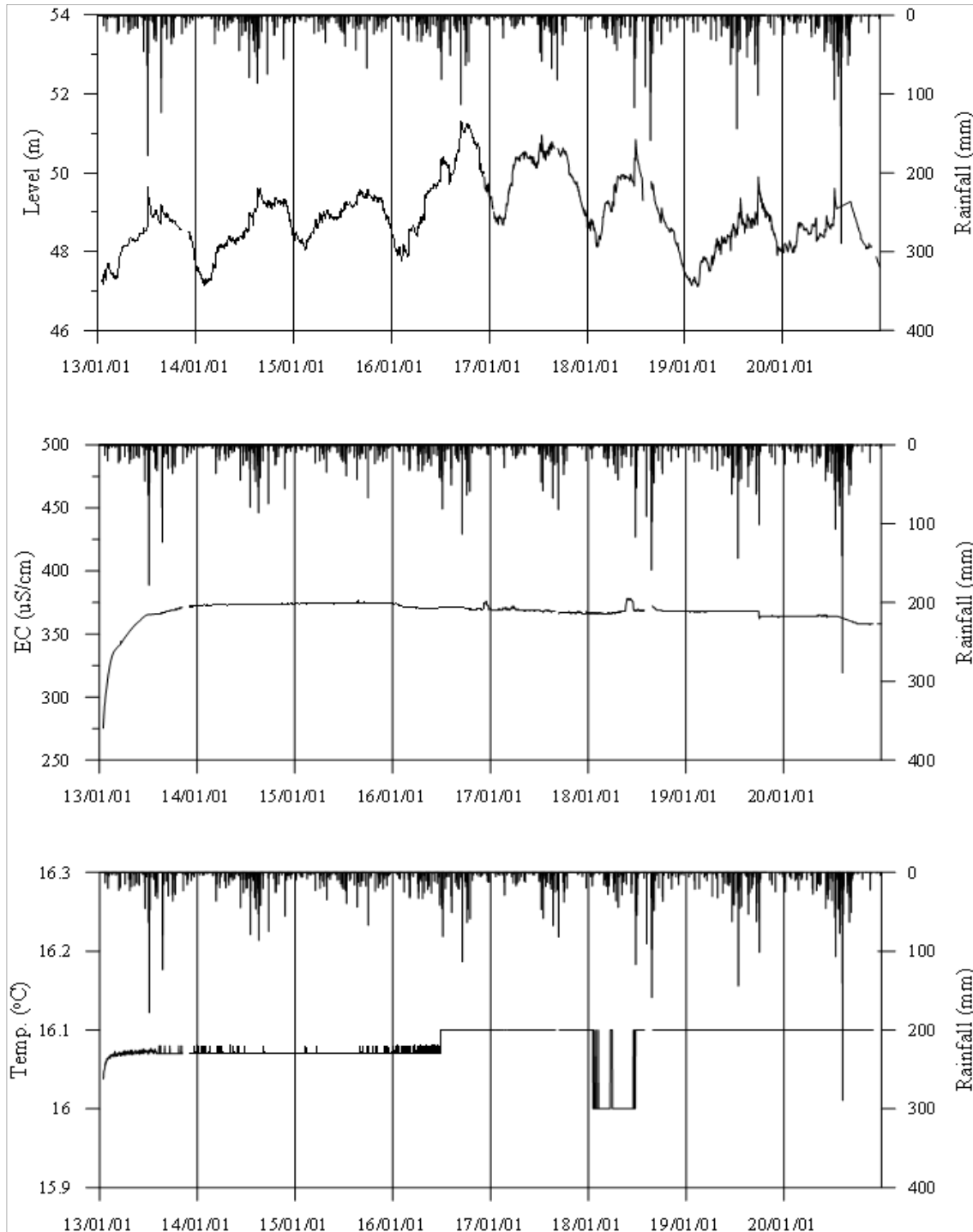
<남원2 관측공의 장기관측자료 (2013.1.1 ~ 2020.12.31)> (a)지하수위, (b)전기전도도, (c)수온
