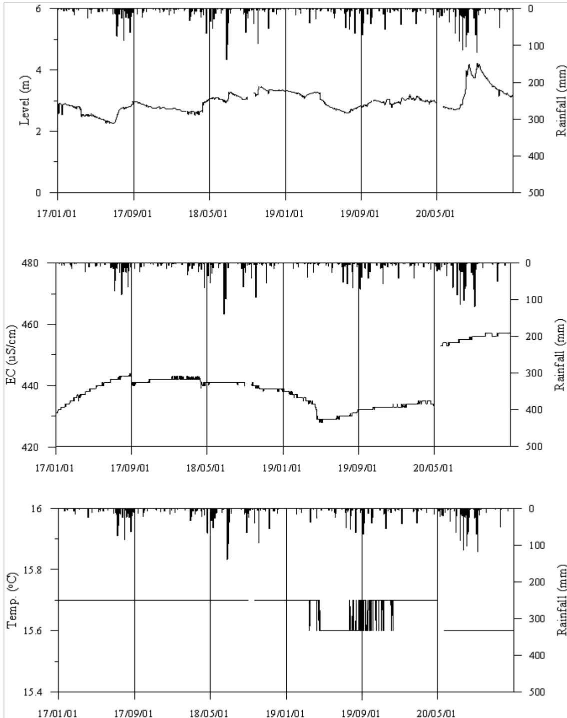
<예산2 관측공의 장기관측자료 (2017.1.1 ~ 2020.12.31)> (a)지하수위, (b)전기전도도, (c)수온
