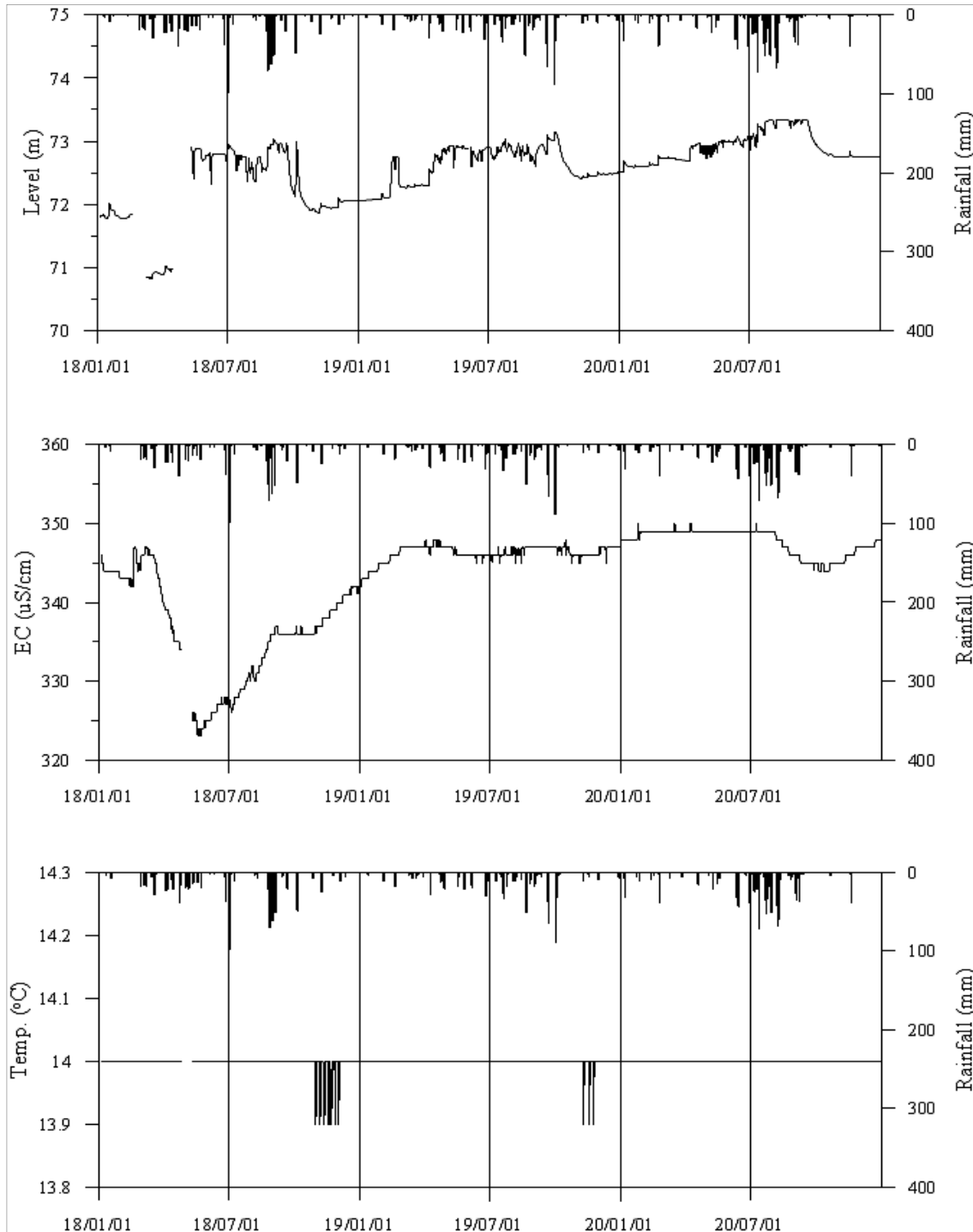
<의성2 관측공의 장기관측자료 (2018.1.1 ~ 2020.12.31.)> (a)지하수위, (b)전기전도도, (c)수온
