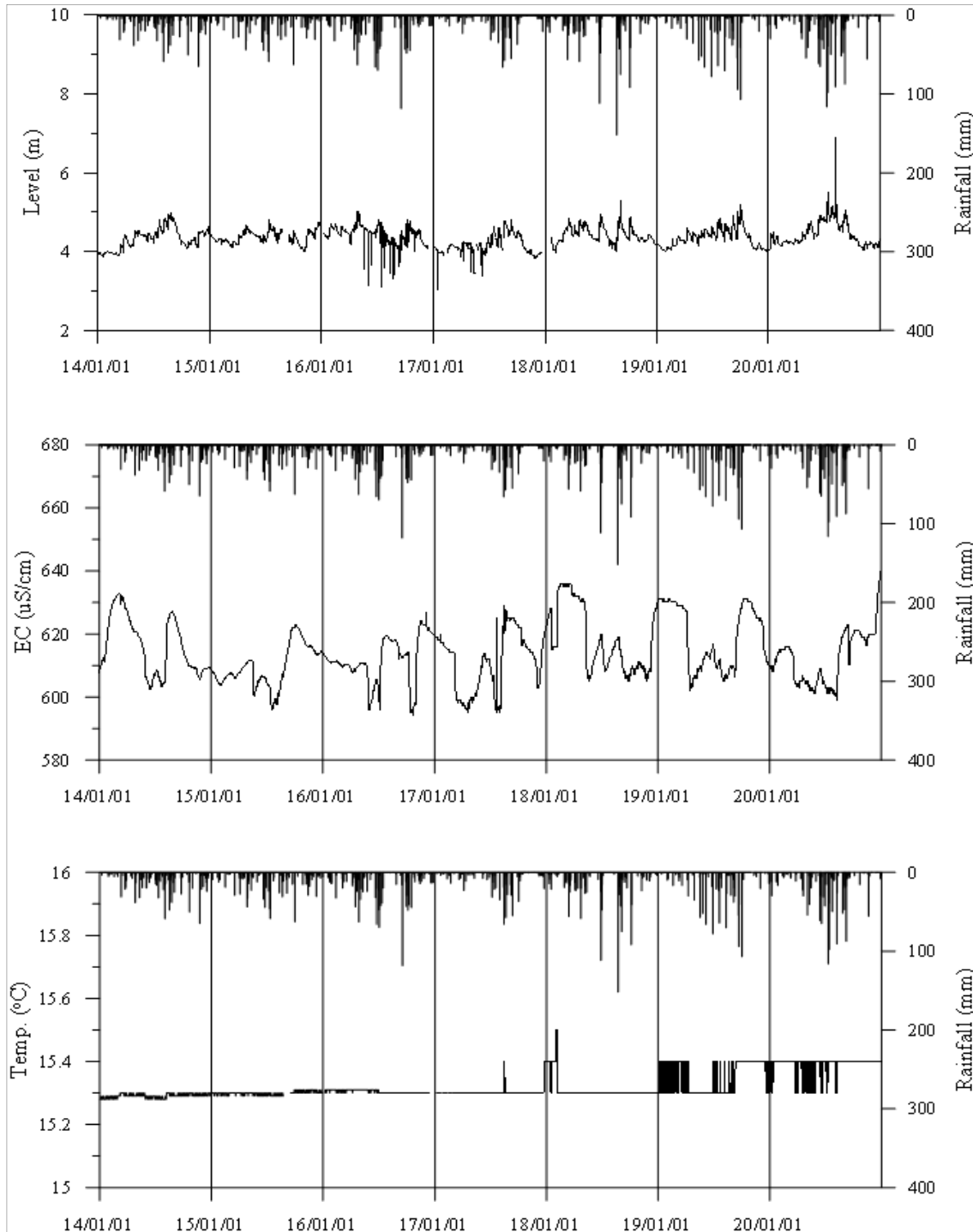
<함평3 관측공의 장기관측자료 (2014.1.1~2020.12.31)> (a)지하수위, (b)전기전도도, (c)수온
