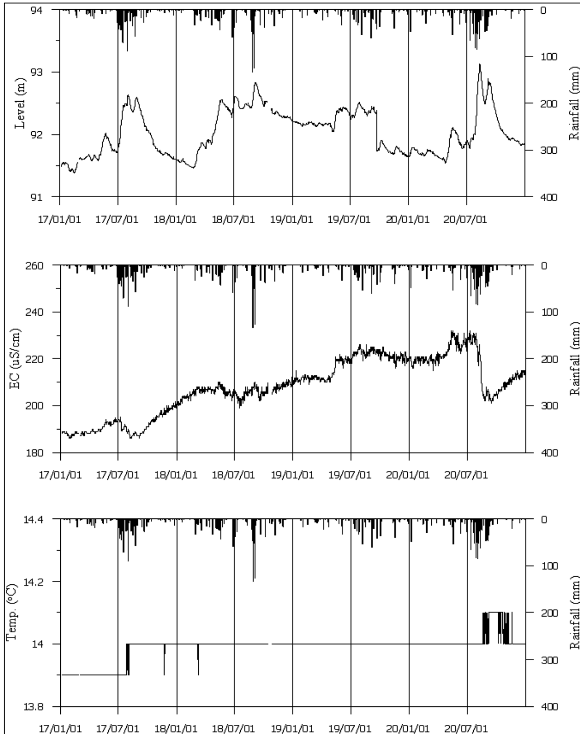
<음성4 관측공의 장기관측자료 (2017.1.1 ~ 2020.12.31)> (a)지하수위, (b)전기전도도, (c)수온
