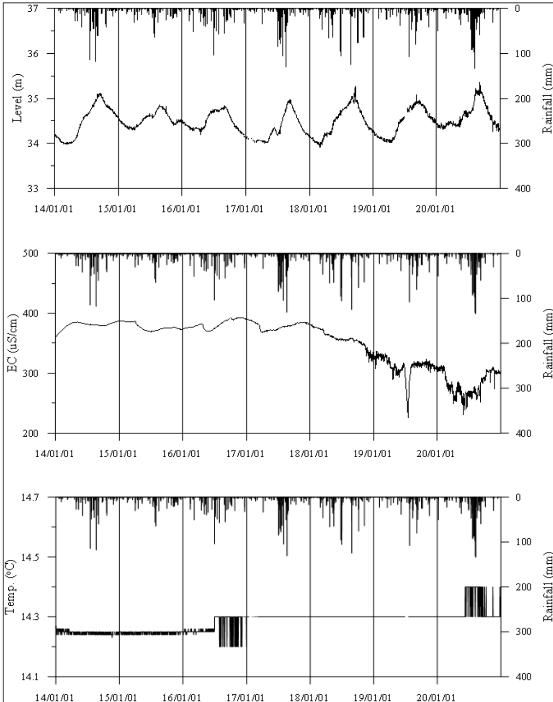
<안성2 관측공의 장기관측자료 (2014.1.1 ~ 2020.12.31)> (a)지하수위, (b)전기전도도, (c)수온
