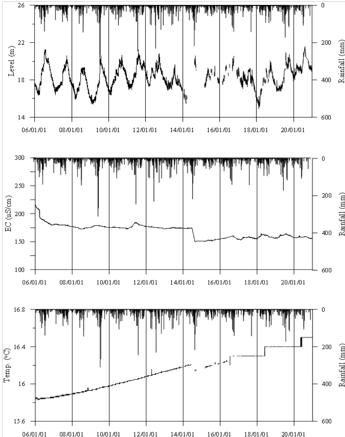
<김해3 관측공의 장기관측자료 (2006.1.1 ~ 2020.12.31)> (a)지하수위, (b)전기전도도, (c)수온
