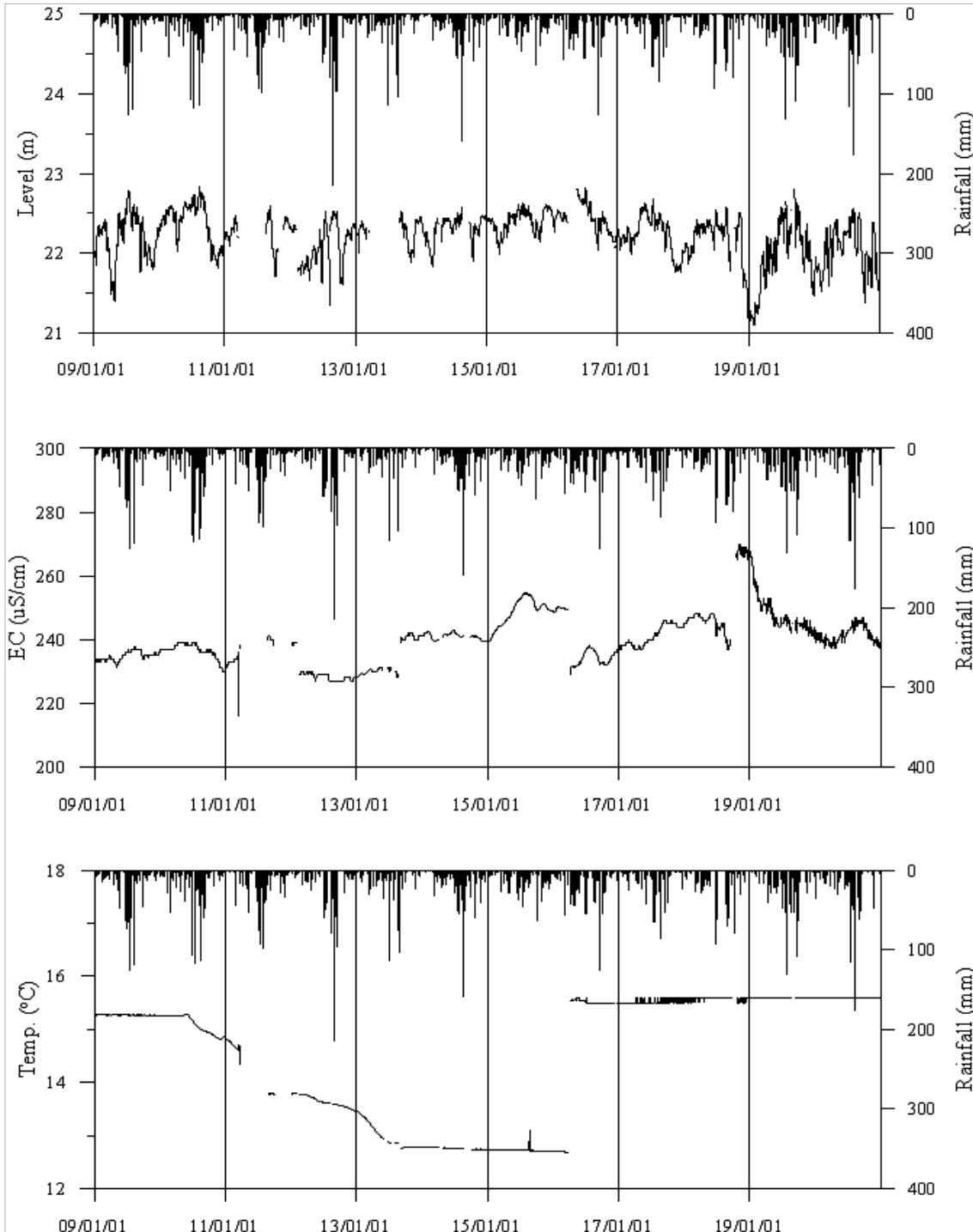
<정읍1 관측공의 장기관측자료 (2009.1.1 ~ 2020.12.31)> (a)지하수위, (b)전기전도도, (c)수온
