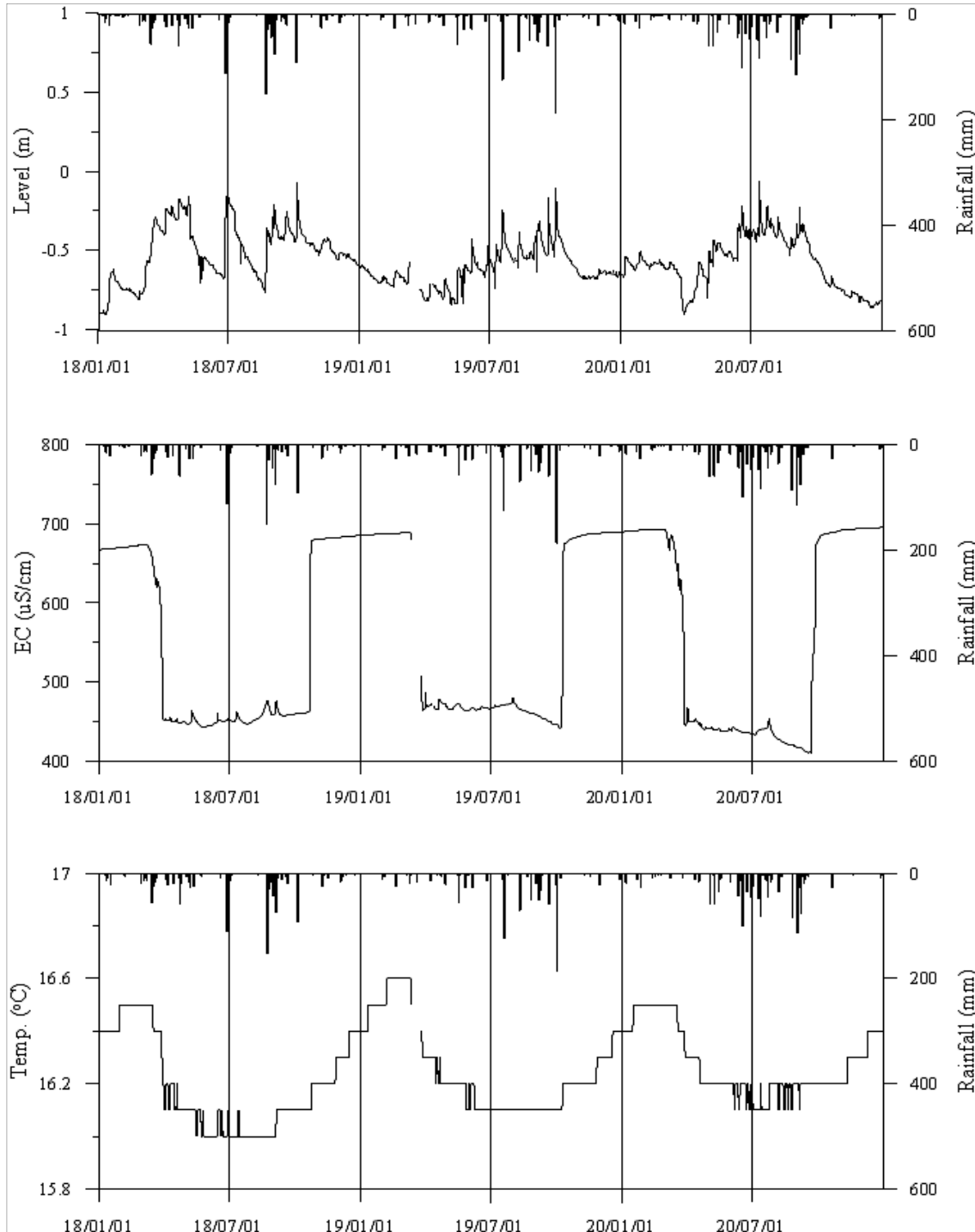
<해남1 관측공의 장기관측자료 (2018.1.1~2020.12.31)> (a)지하수위, (b)전기전도도, (c)수온
