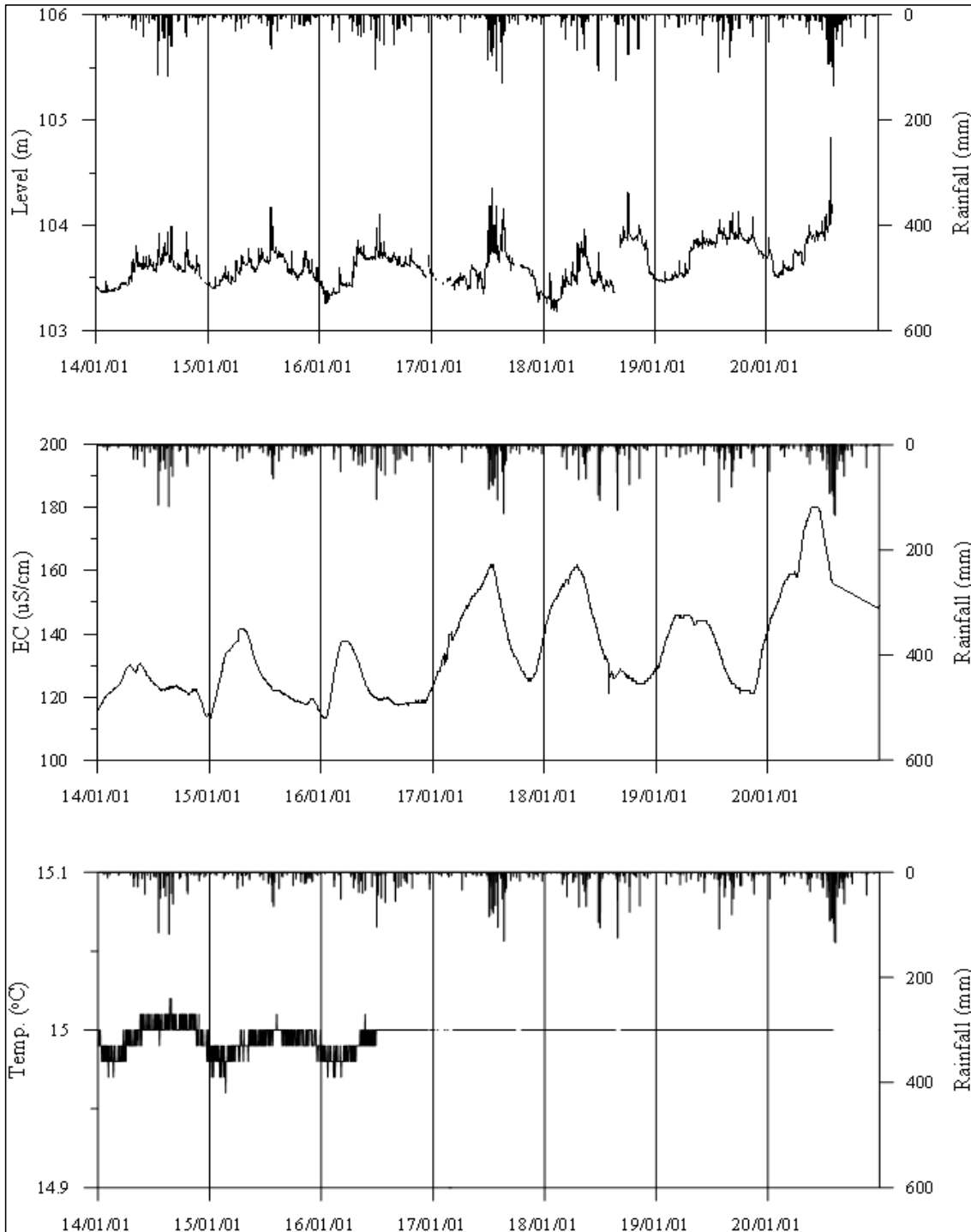
<용인2 관측공의 장기관측자료 (2014.1.1 ~ 2020.12.31)> (a)지하수위, (b)전기전도도, (c)수온
