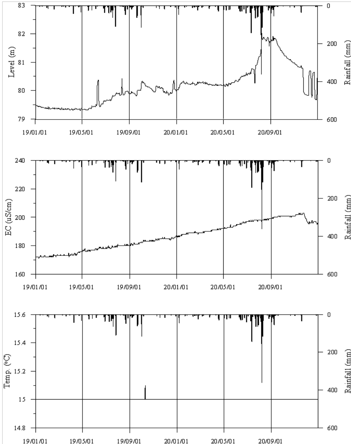
<순창5 관측공의 장기관측자료 (2019.1.1 ~ 2020.12.31)> (a)지하수위, (b)전기전도도, (c)수온
