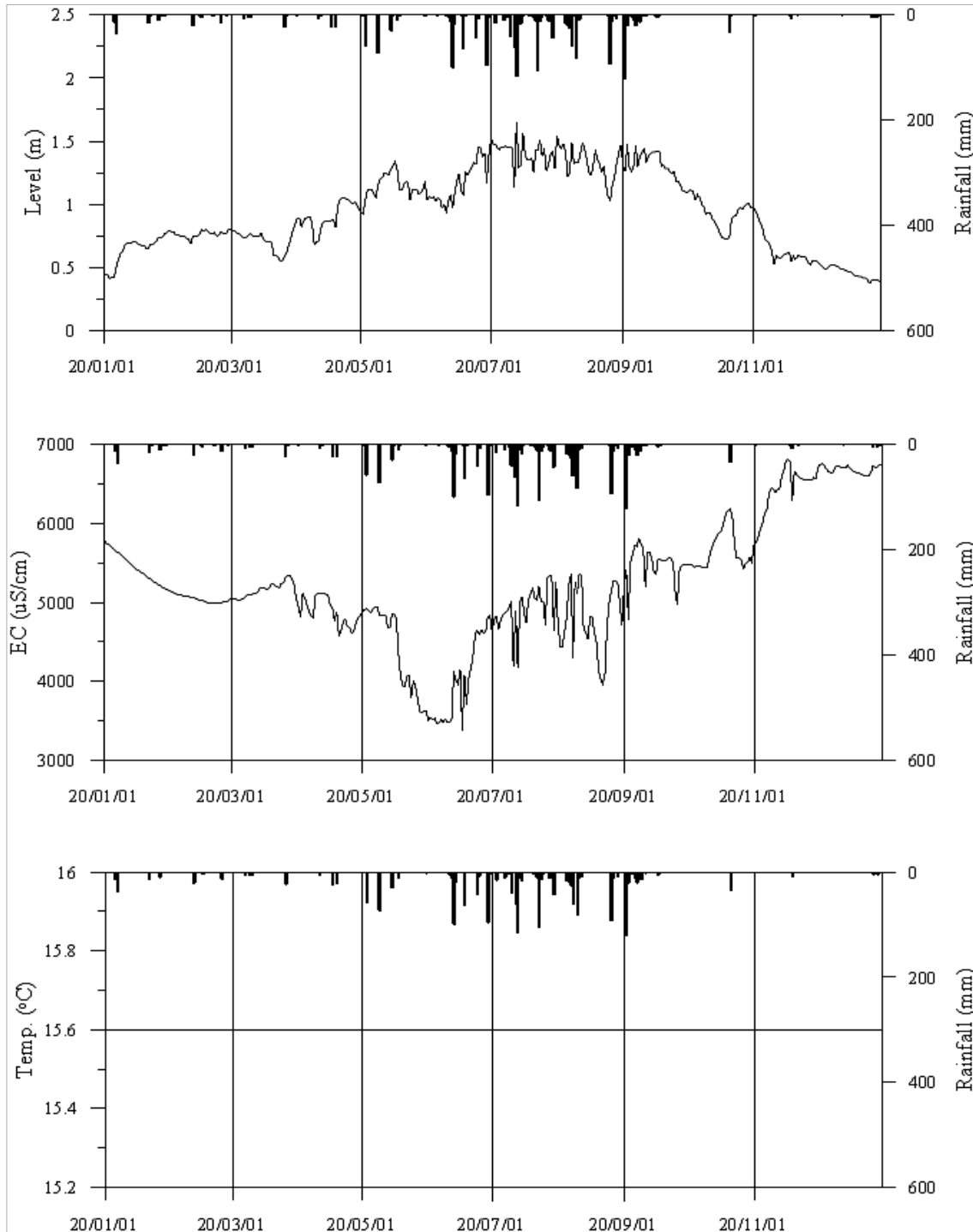
<순천8 관측공의 장기관측자료 (2020.1.1~2020.12.31)> (a)지하수위, (b)전기전도도, (c)수온
