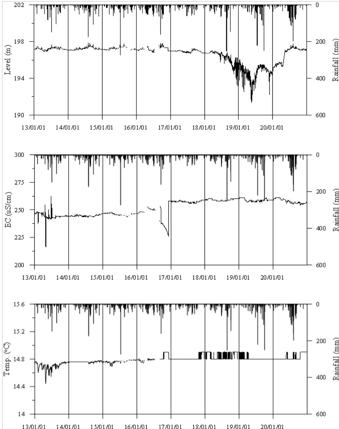
<산청1 관측공의 장기관측자료 (2013.1.1 ~ 2020.12.31)> (a)지하수위, (b)전기전도도, (c)수온
