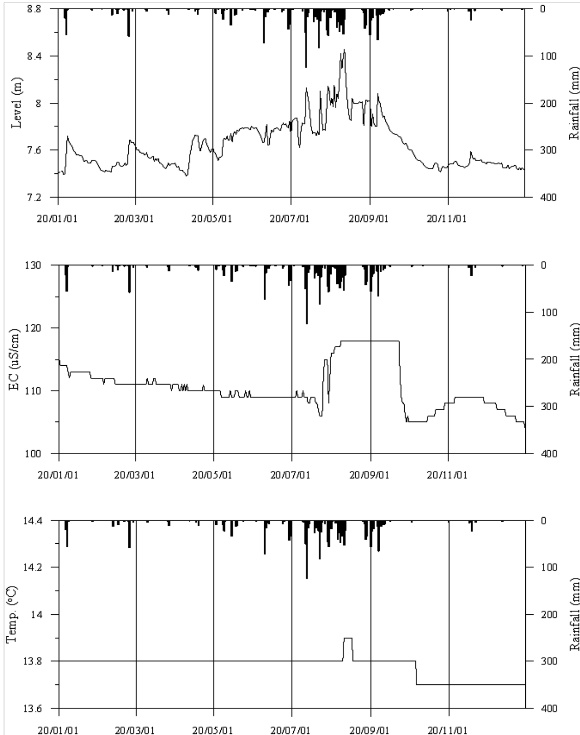
<청양5 관측공의 장기관측자료 (2020.1.1 ~ 2020.12.31)> (a)지하수위, (b)전기전도도, (c)수온
