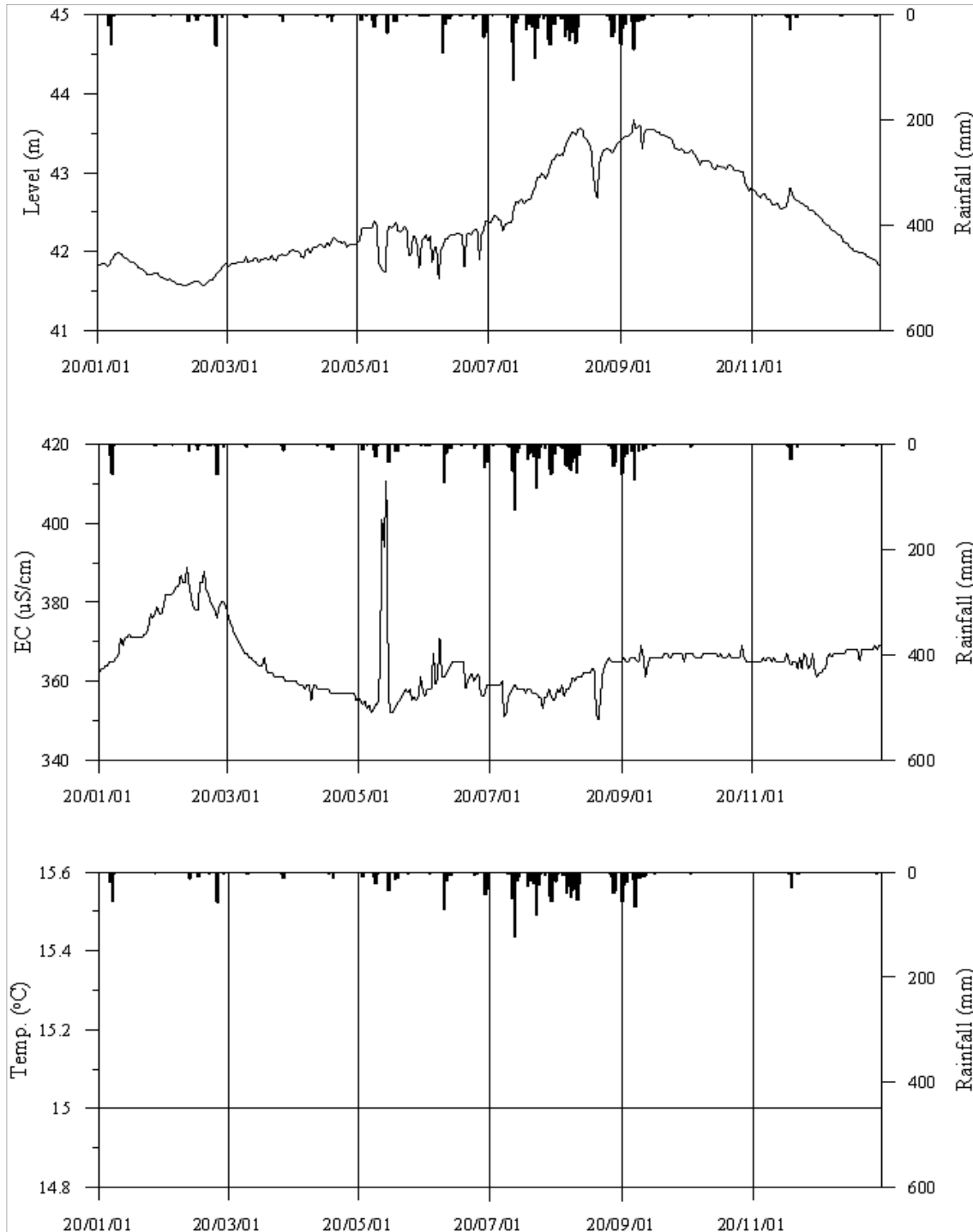
<공주5 관측공의 장기관측자료 (2020.1.1 ~ 2020.12.31)> (a)지하수위, (b)전기전도도, (c)수온
