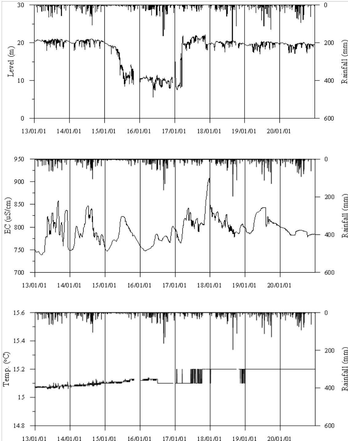
<창녕1 관측공의 장기관측자료 (2013.1.1 ~ 2020.12.31)> (a)지하수위, (b)전기전도도, (c)수온
