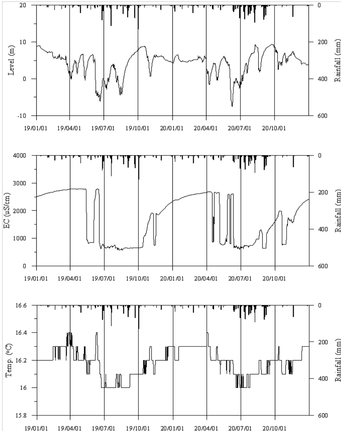
<창녕4 관측공의 장기관측자료 (2019.1.1 ~ 2020.12.31)> (a)지하수위, (b)전기전도도, (c)수온
