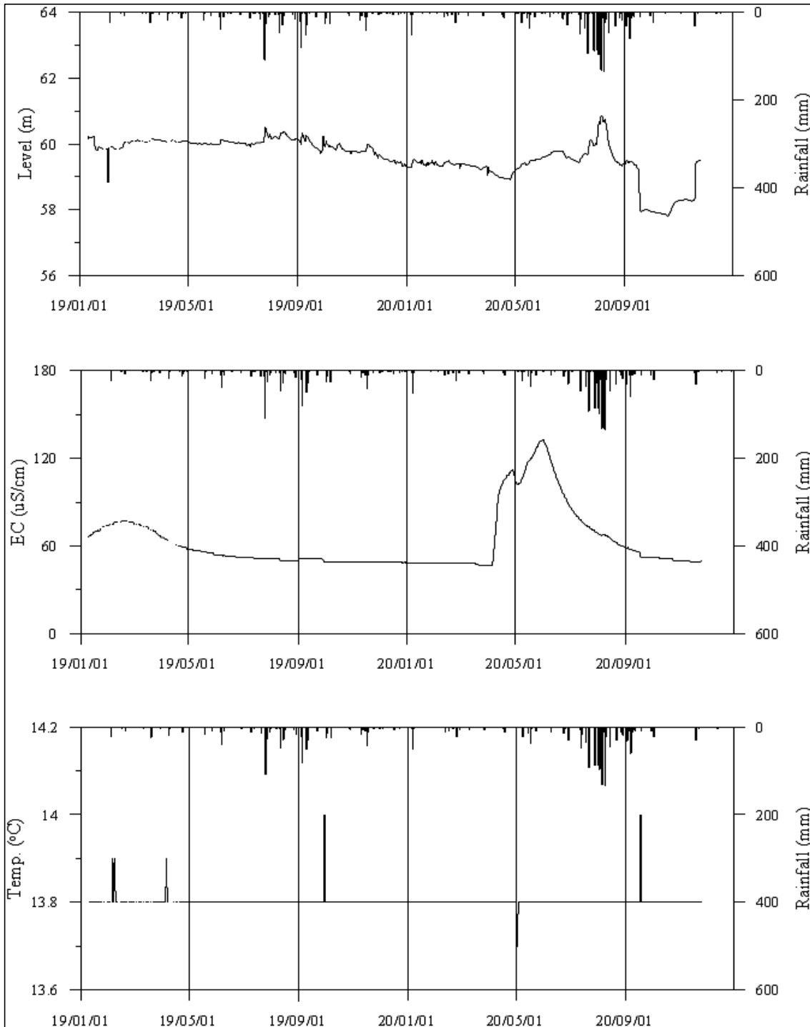
<용인6 관측공의 장기관측자료 (2019.1.1 ~ 2020.12.31)> (a)지하수위, (b)전기전도도, (c)수온
