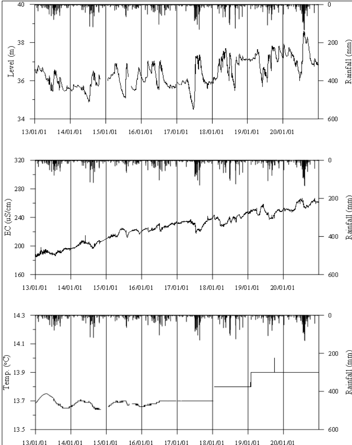
<용인1 관측공의 장기관측자료 (2013.1.1 ~ 2020.12.31)> (a)지하수위, (b)전기전도도, (c)수온
