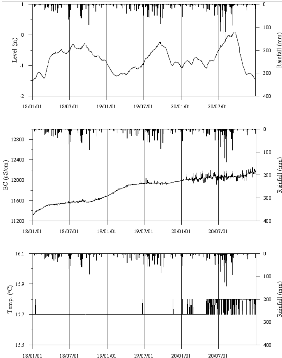
<부안4 관측공의 장기관측자료 (2018.1.1 ~ 2020.12.31)> (a)지하수위, (b)전기전도도, (c)수온
