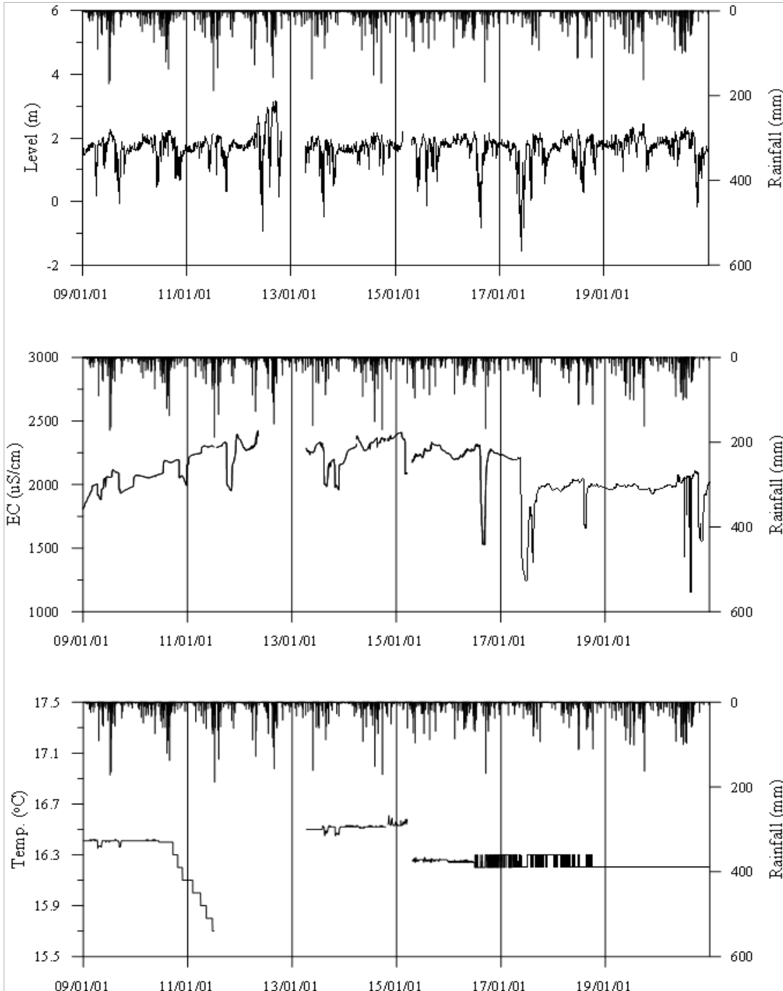
<보성1 관측공의 장기관측자료 (2009.1.1 ~ 2020.12.31)> (a)지하수위, (b)전기전도도, (c)수온
