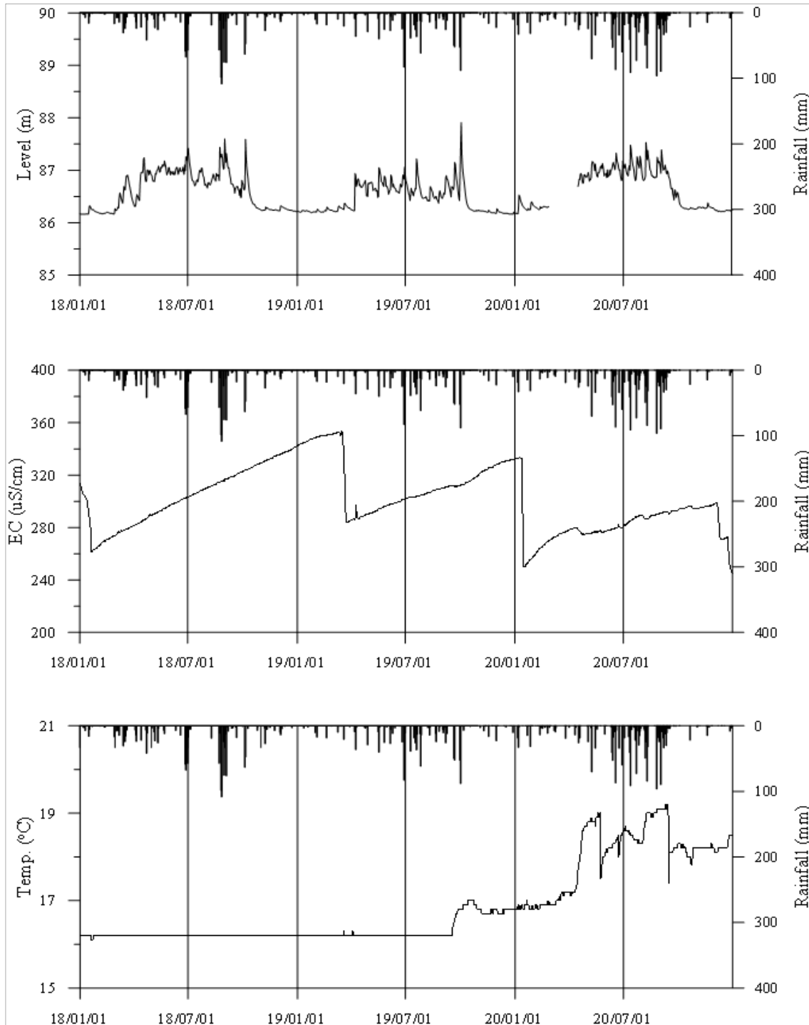
<화순5 관측공의 장기관측자료 (2018.1.1 ~ 2020.12.31)> (a)지하수위, (b)전기전도도, (c)수온
