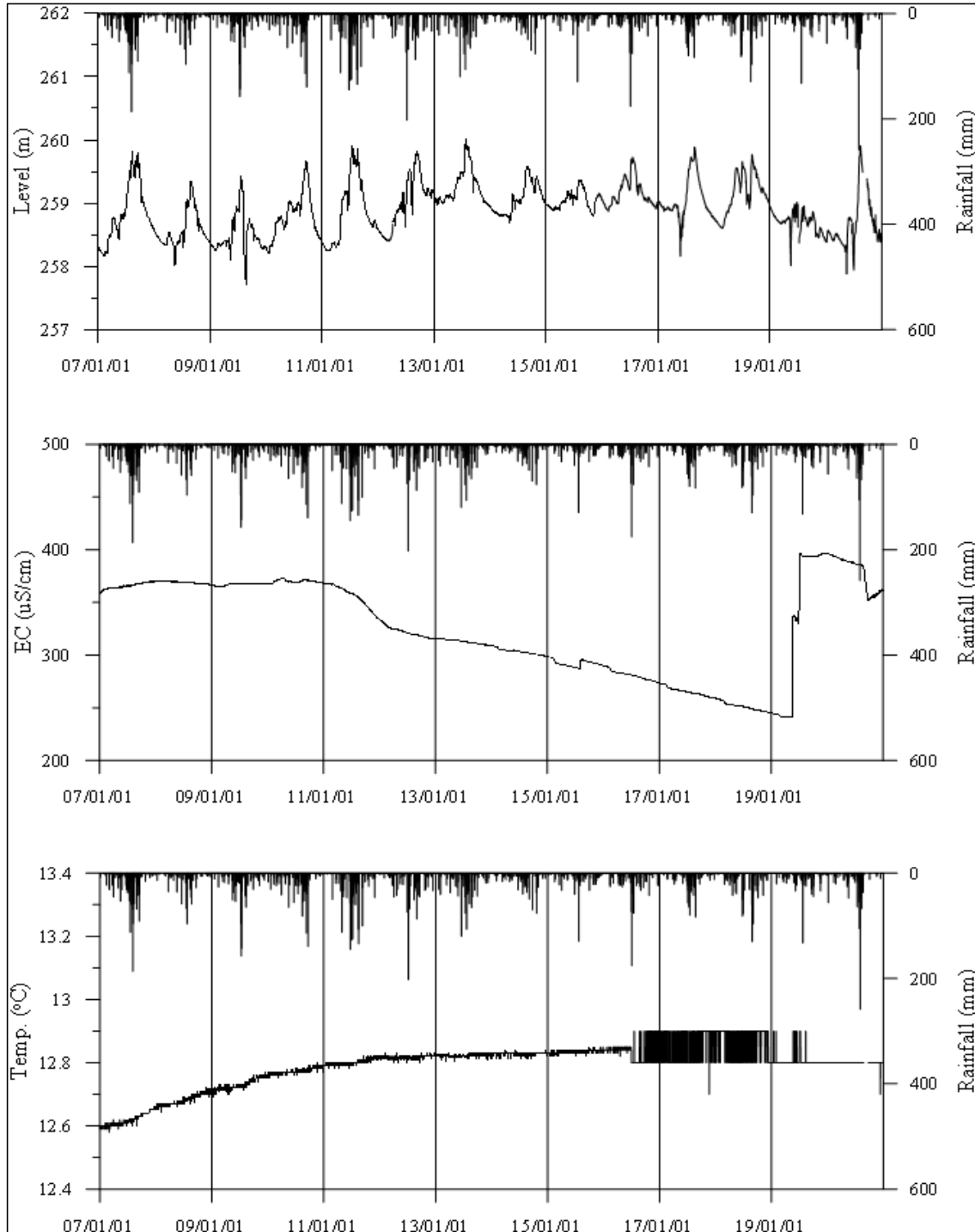
<제천1 관측공의 장기관측자료 (2007.1.1 ~ 2020.12.31)> (a)지하수위, (b)전기전도도, (c)수온
