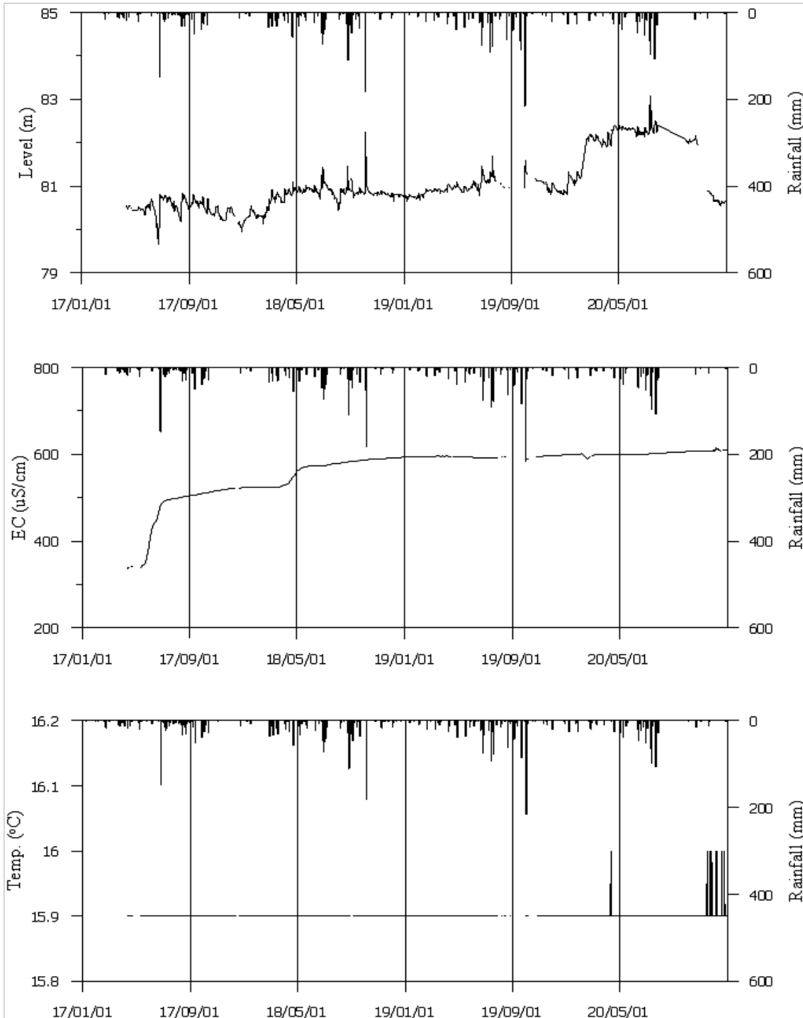
<합천1(신) 관측공의 이동설치 후 장기관측자료 (2017.1.1 ~ 2020.12.31)> (a)지하수위, (b)전기전도도, (c)수온
