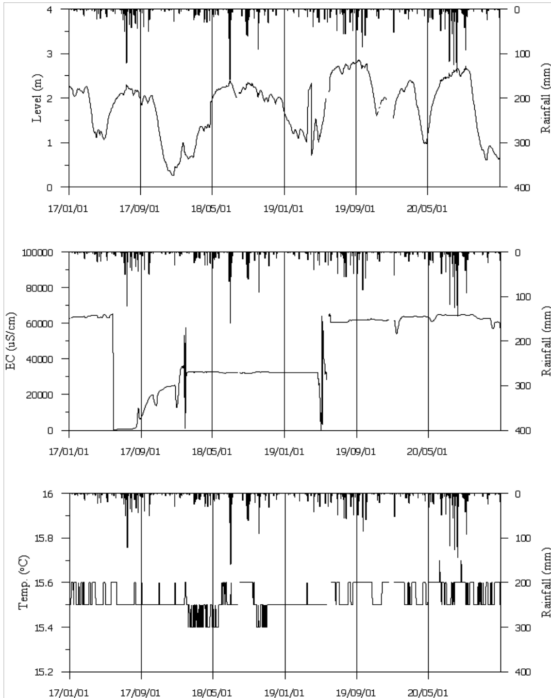
<부안3 관측공의 장기관측자료 (2017.1.1 ~ 2020.12.31)> (a)지하수위, (b)전기전도도, (c)수온
