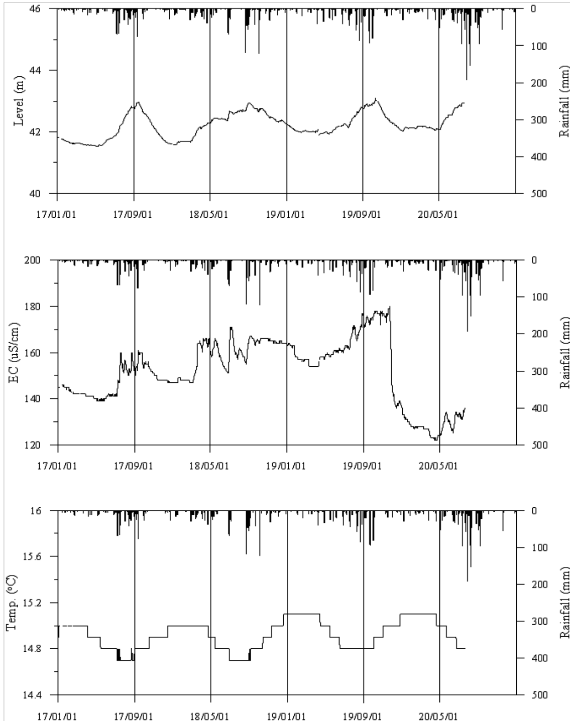
<영광5 관측공의 장기관측자료 (2017.1.1 ~ 2020.12.31)> (a)지하수위, (b)전기전도도, (c)수온
