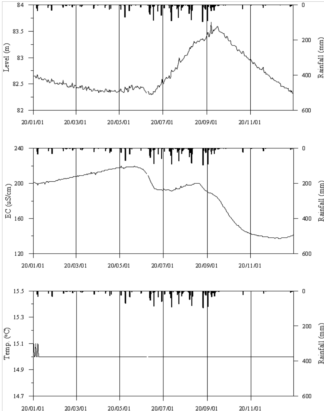
<장흥6 관측공의 장기관측자료 (2020.1.1 ~ 2020.12.31)> (a)지하수위, (b)전기전도도, (c)수온
