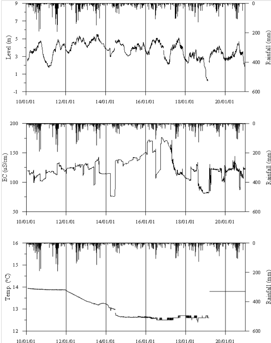
<김포1 관측공의 장기관측자료 (2010.1.1 ~ 2020.12.31)> (a)지하수위, (b)전기전도도, (c)수온
