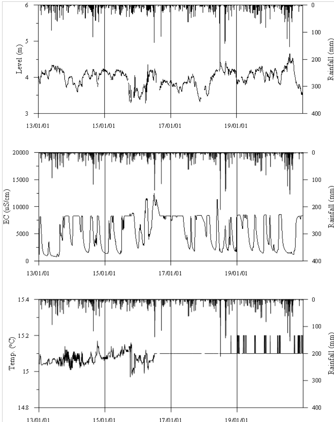
<서천1 관측공의 장기관측자료 (2013.1.1 ~ 2020.12.31)> (a)지하수위, (b)전기전도도, (c)수온
