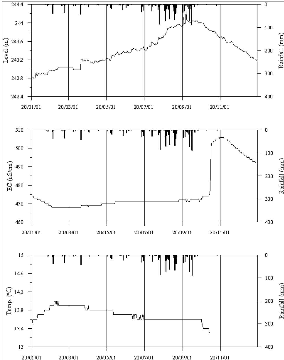
<영양4 관측공의 장기관측자료 (2020.1.1 ~ 2020.12.31.)> (a)지하수위, (b)전기전도도, (c)수온
