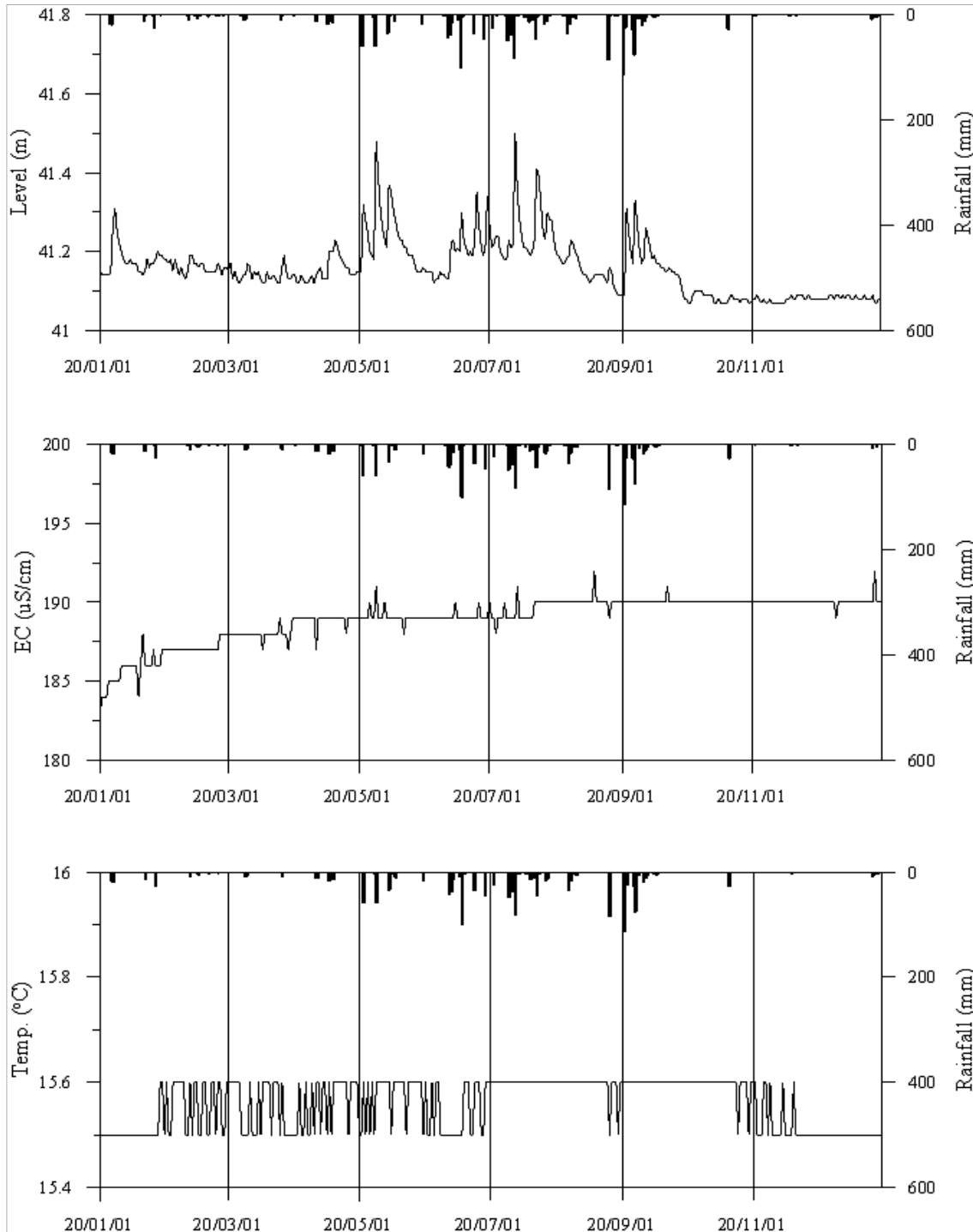
<해남11 관측공의 장기관측자료 (2020.1.1~2020.12.31)> (a)지하수위, (b)전기전도도, (c)수온
