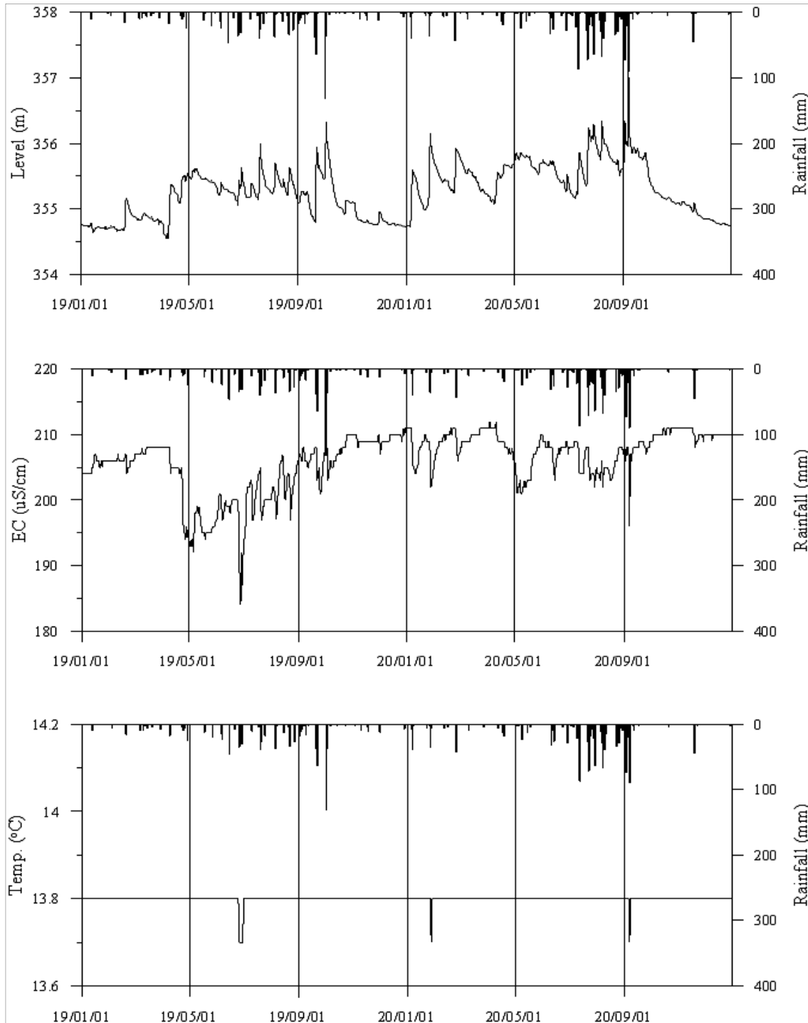
<청송5 관측공의 장기관측자료 (2019.1.1 ~ 2020.12.31)> (a)지하수위, (b)전기전도도, (c)수온
