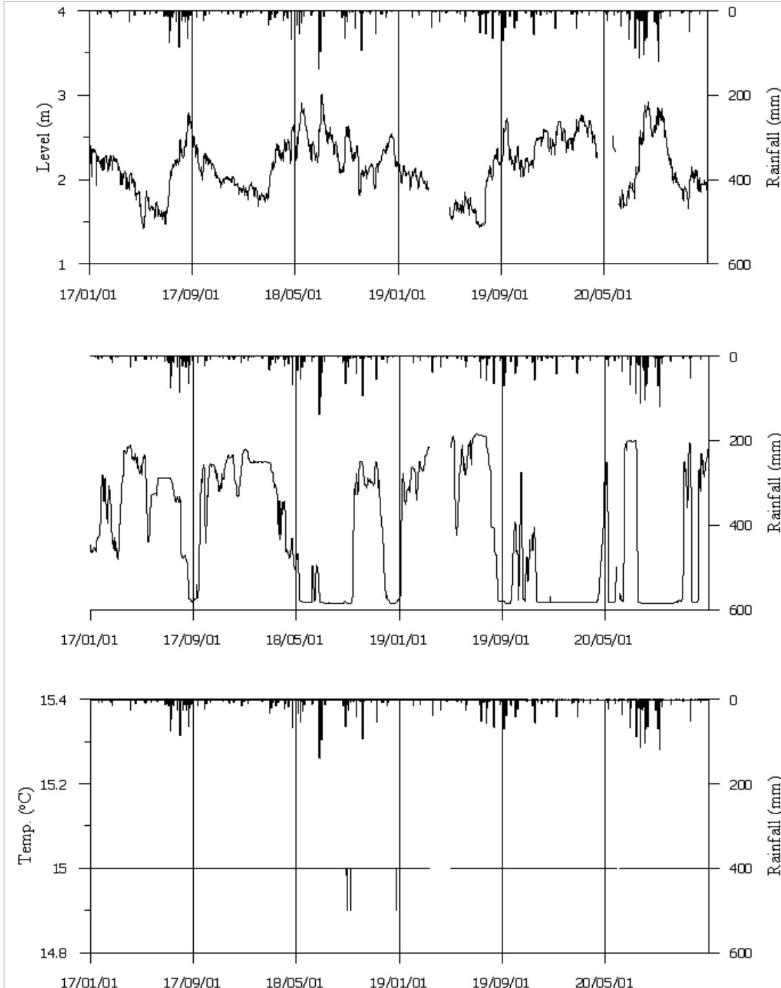
<태안1 관측공의 장기관측자료 (2017.1.1 ~ 2020.12.31)> (a)지하수위, (b)전기전도도, (c)수온
