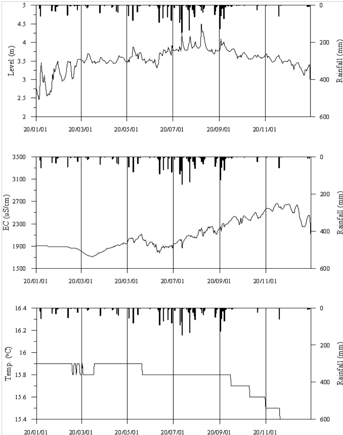
<하동5 관측공의 장기관측자료 (2020.1.1 ~ 2020.12.31)> (a)지하수위, (b)전기전도도, (c)수온
