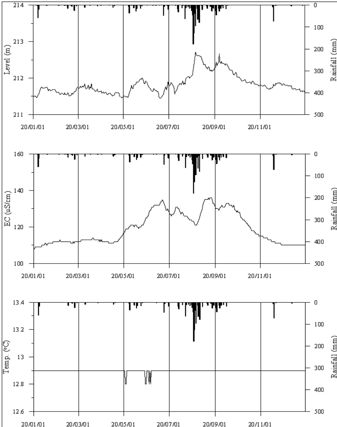
<화전4 관측공의 장기관측자료 (2020.1.1 ~ 2020.12.31)> (a)지하수위, (b)전기전도도, (c)수온
