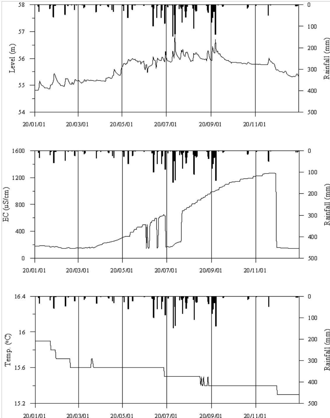
<경남고성1 관측공의 장기관측자료 (2020.1.1 ~ 2020.12.31)> (a)지하수위, (b)전기전도도, (c)수온
