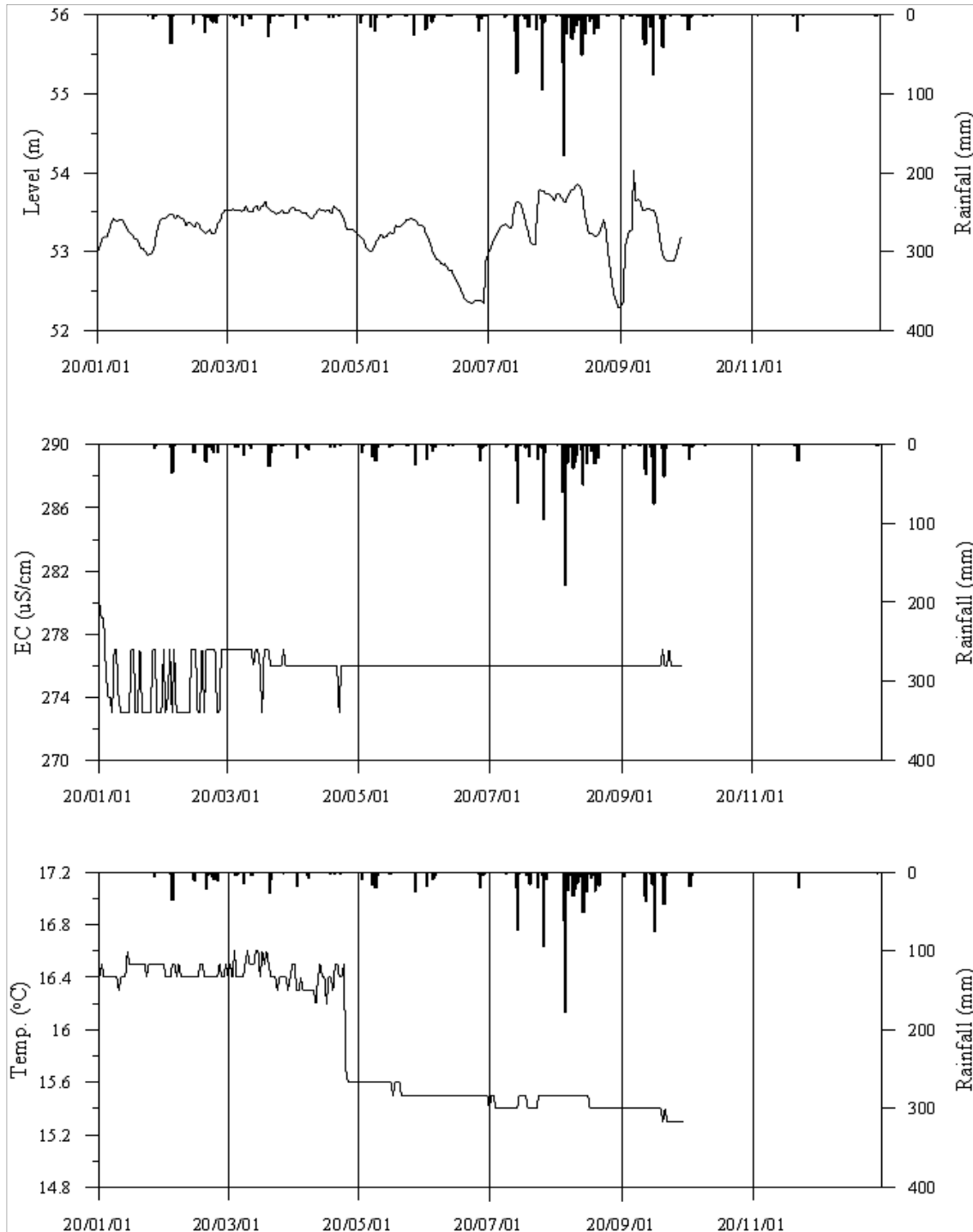
<울진3 관측공의 장기관측자료 (2020.1.1 ~ 2020.12.31.)> (a)지하수위, (b)전기전도도, (c)수온
