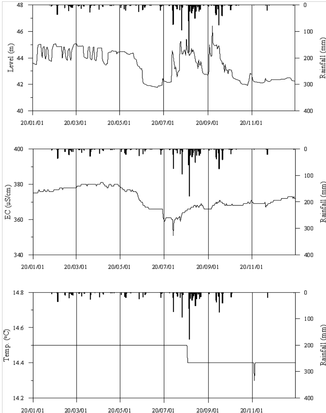
<울진2 관측공의 장기관측자료 (2020.1.1 ~ 2020.12.31.)> (a)지하수위, (b)전기전도도, (c)수온
