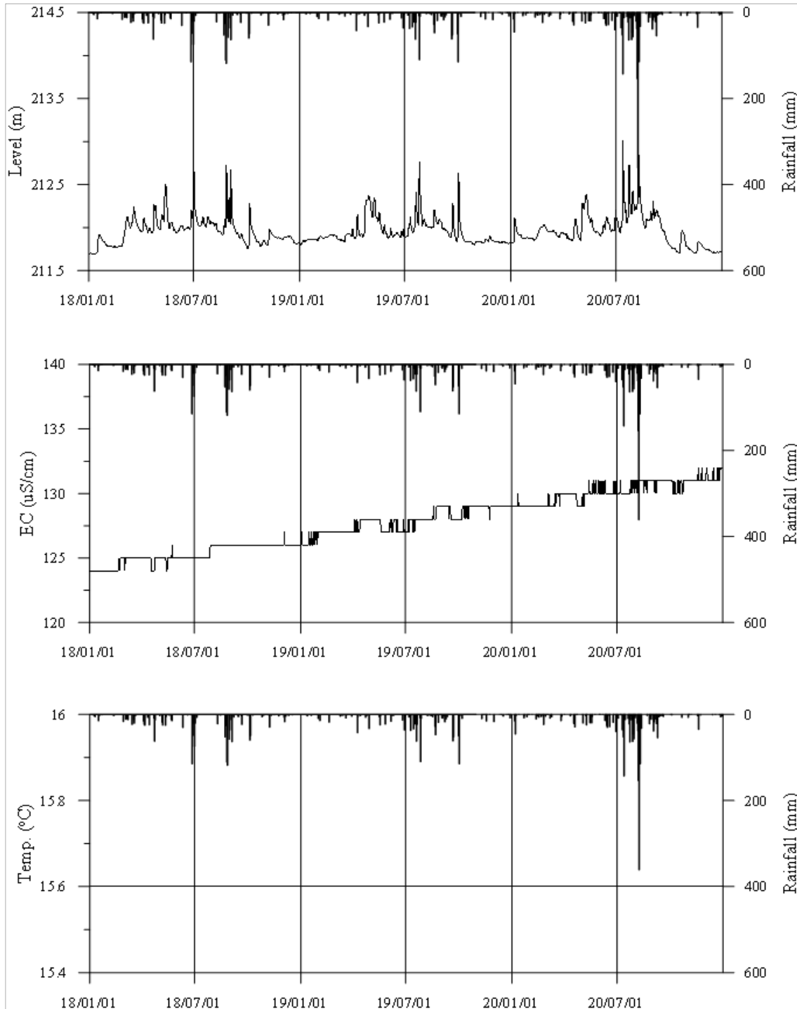
<순창3 관측공의 장기관측자료 (2018.1.1 ~ 2020.12.31)> (a)지하수위, (b)전기전도도, (c)수온
