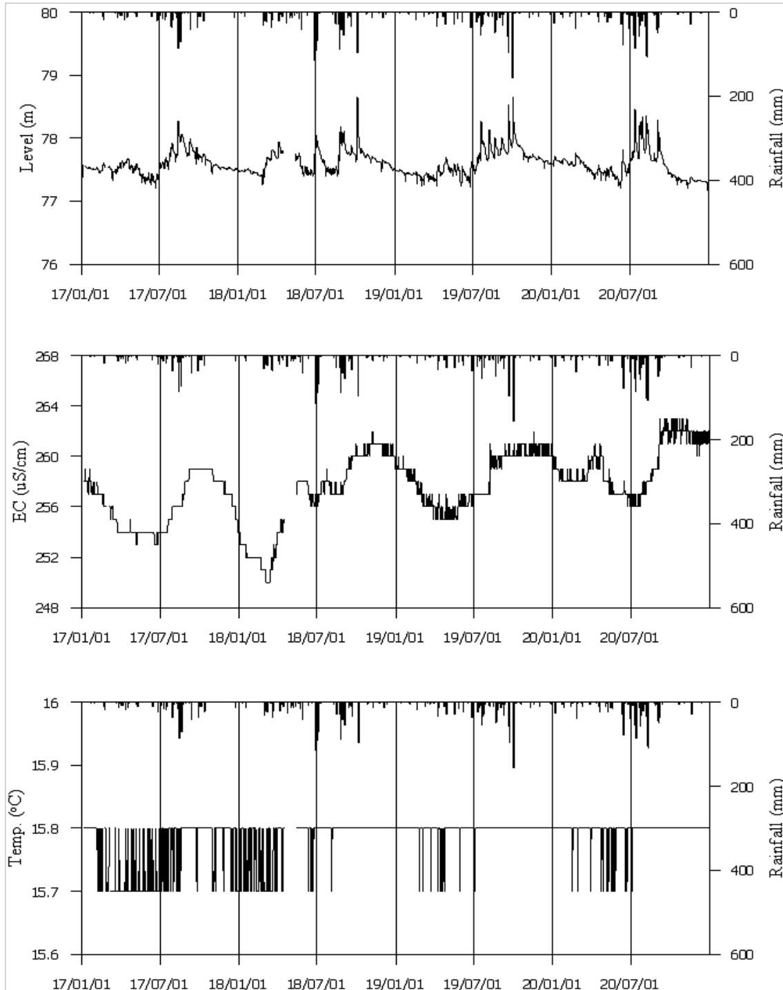
<김천1 관측공의 장기관측자료 (2017.1.1 ~ 2020.12.31.)> (a)지하수위, (b)전기전도도, (c)수온
