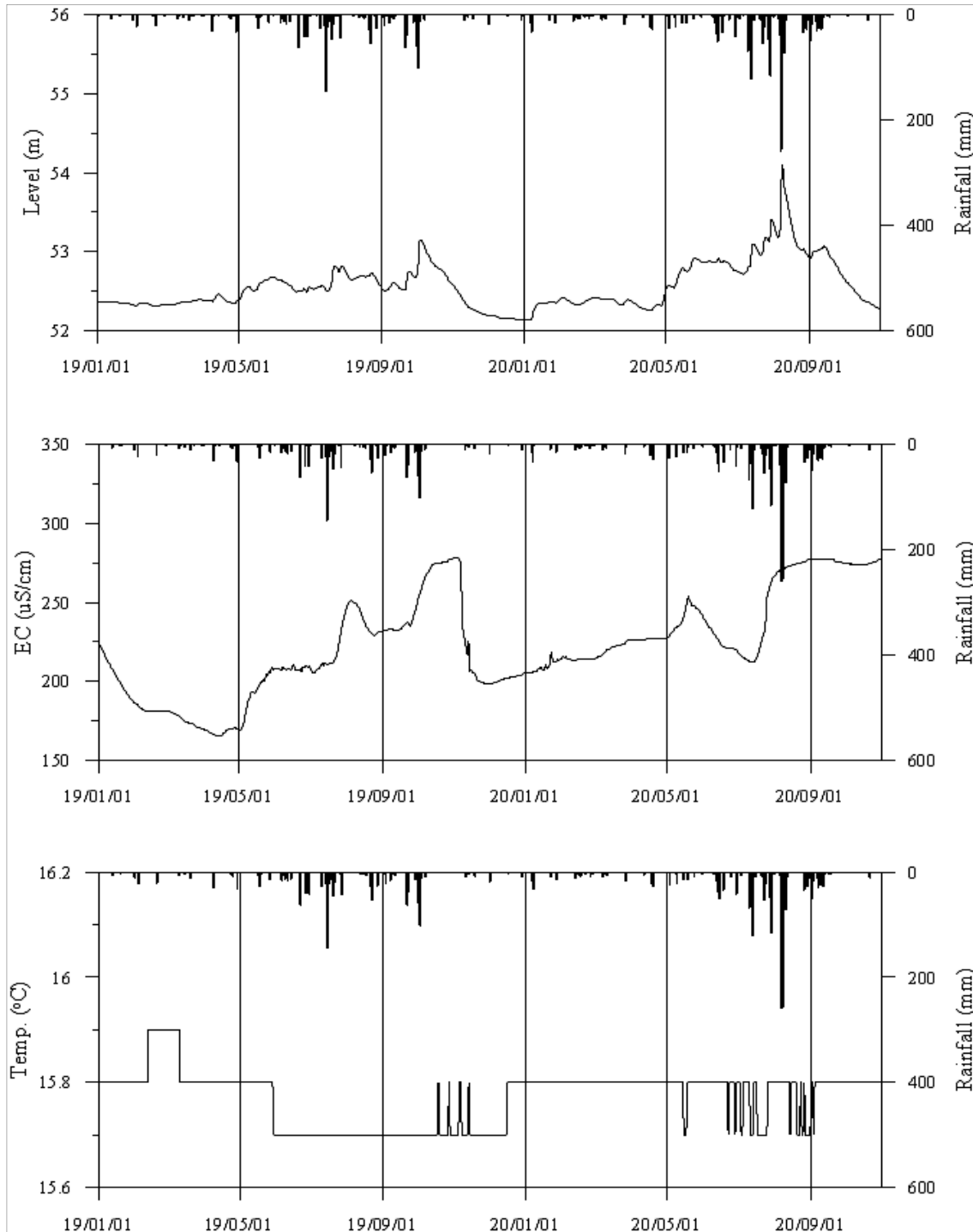
<담양2 관측공의 장기관측자료 (2019.1.1.~2020.10.31)> (a)지하수위, (b)전기전도도, (c)수온
