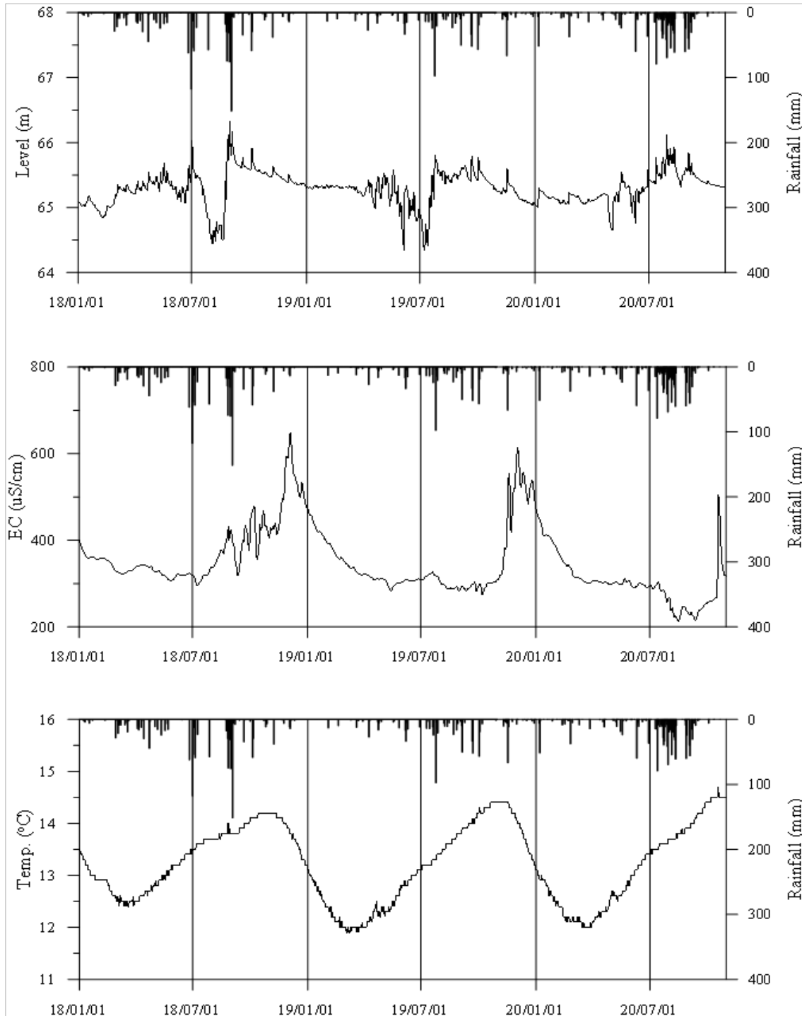
<증평2 관측공의 장기관측자료 (2018.1.1 ~ 2020.10.31)> (a)지하수위, (b)전기전도도, (c)수온
