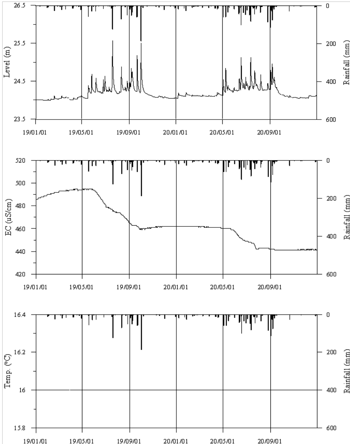
<해남4 관측공의 장기관측자료 (2019.1.1~2020.12.31)> (a)지하수위, (b)전기전도도, (c)수온
