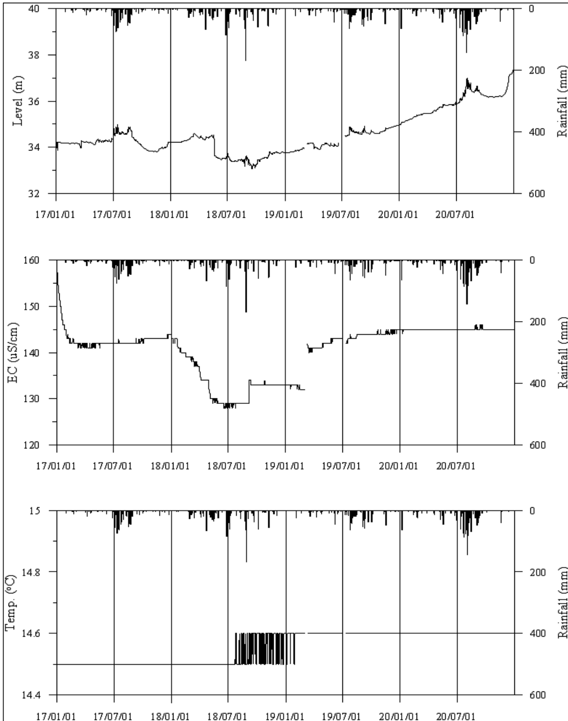
<여주3 관측공의 장기관측자료 (2017.1.1. ~ 2020.12.31)> (a)지하수위, (b)전기전도도, (c)수온
