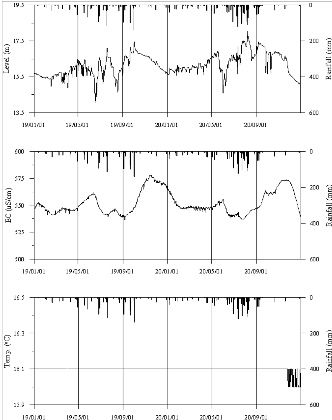
<진주6 관측공의 장기관측자료 (2019.1.1 ~ 2020.12.31)> (a)지하수위, (b)전기전도도, (c)수온
