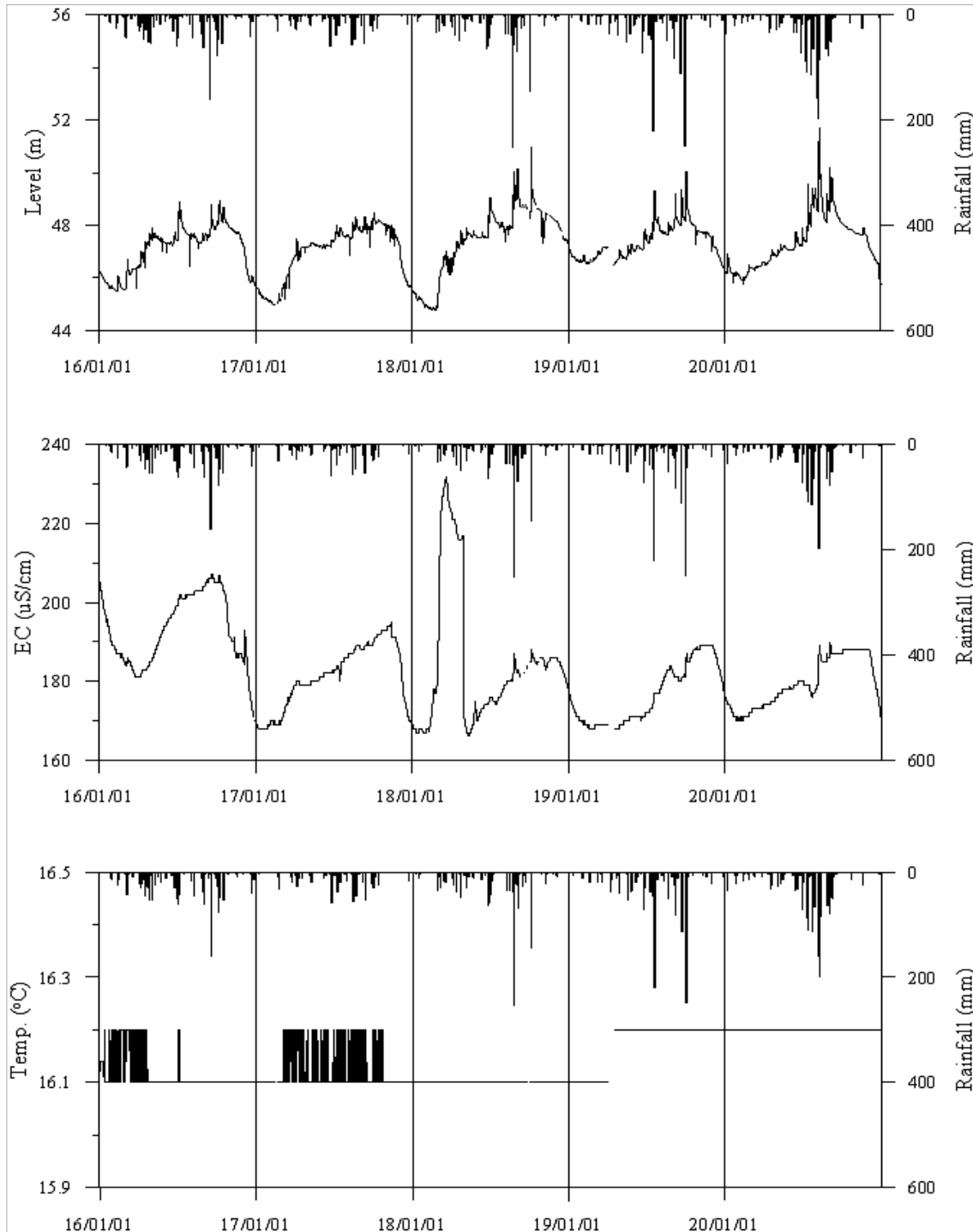
<산청4 관측공의 장기관측자료 (2016.1.1 ~ 2020.12.31)> (a)지하수위, (b)전기전도도, (c)수온
