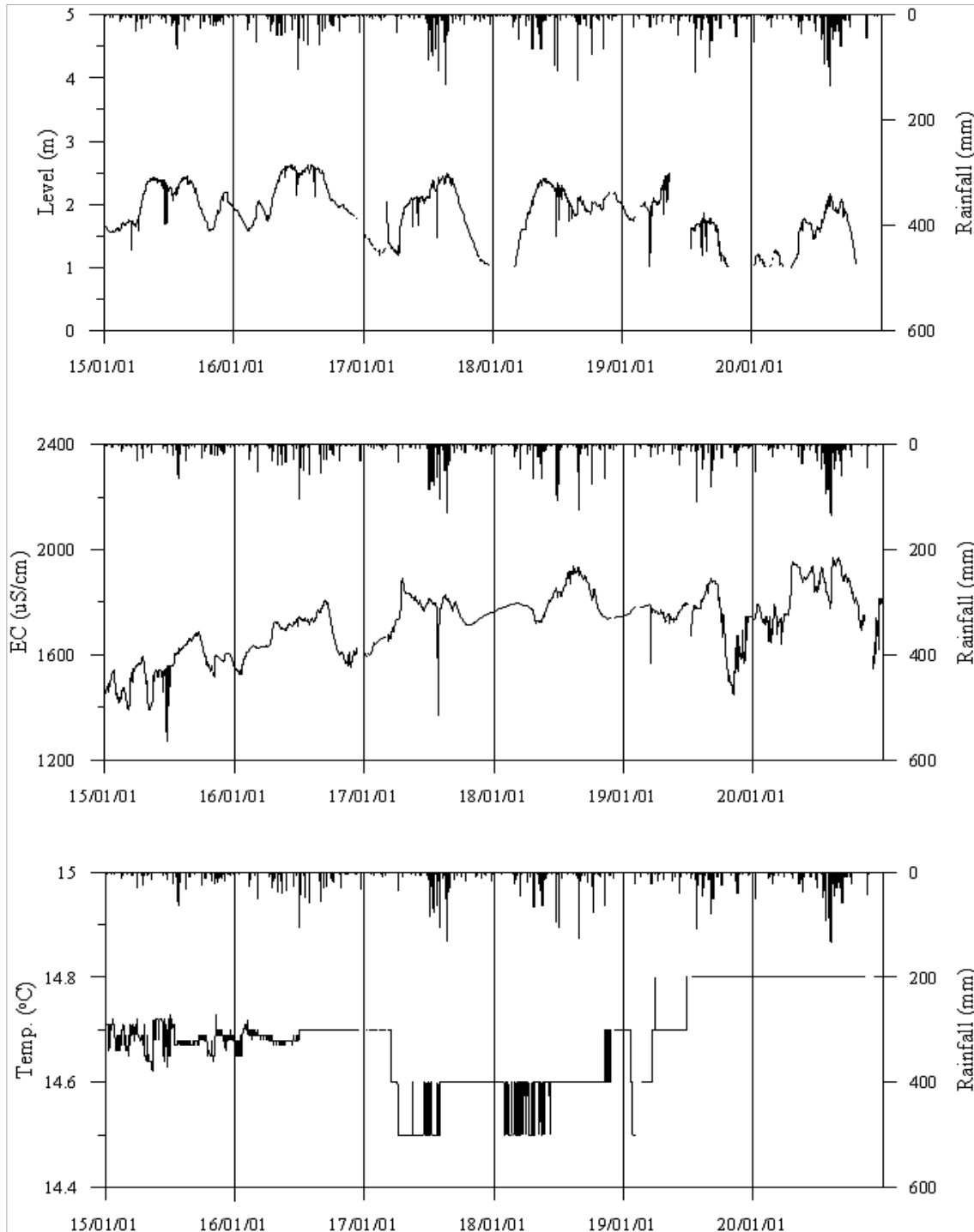
<화성2 관측공의 장기관측자료 (2015.1.1 ~ 2020.12.31)> (a)지하수위, (b)전기전도도, (c)수온
