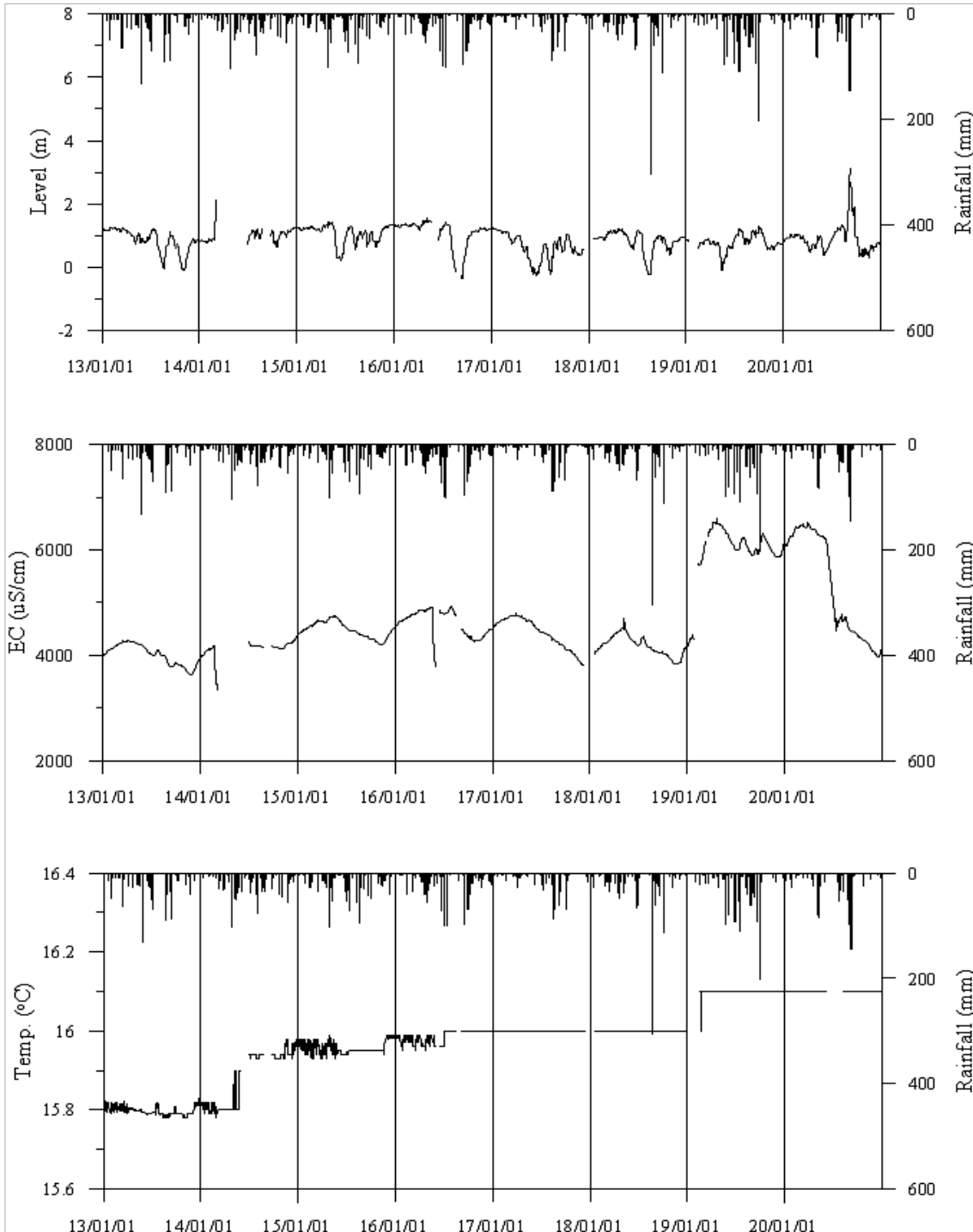
<진도1 관측공의 장기관측자료 (2013.1.1.~2020.12.31)> (a)지하수위, (b)전기전도도, (c)수온
