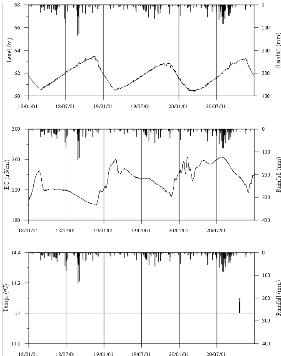
<충주4 관측공의 장기관측자료 (2018.1.1 ~ 2020.12.31)> (a)지하수위, (b)전기전도도, (c)수온
