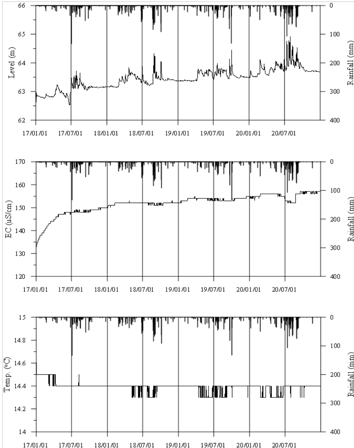
<상주4 관측공의 장기관측자료 (2017.1.1 ~ 2020.12.31)> (a)지하수위, (b)전기전도도, (c)수온
