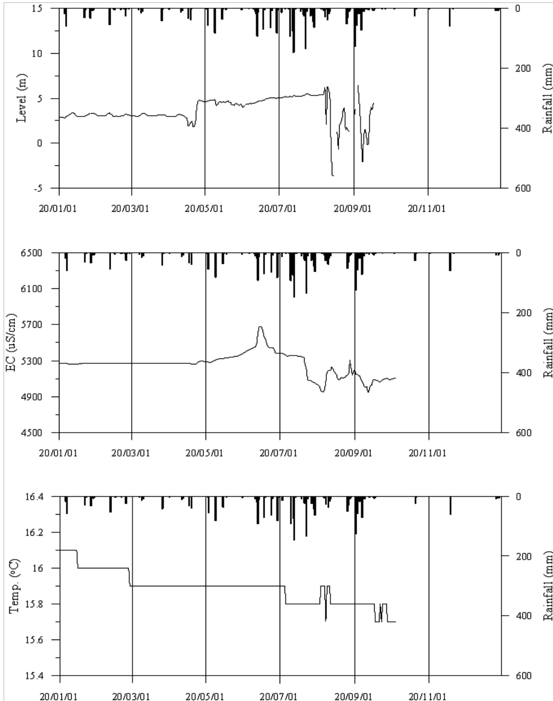
<하동6 관측공의 장기관측자료 (2020.1.1 ~ 2020.12.31)> (a)지하수위, (b)전기전도도, (c)수온
