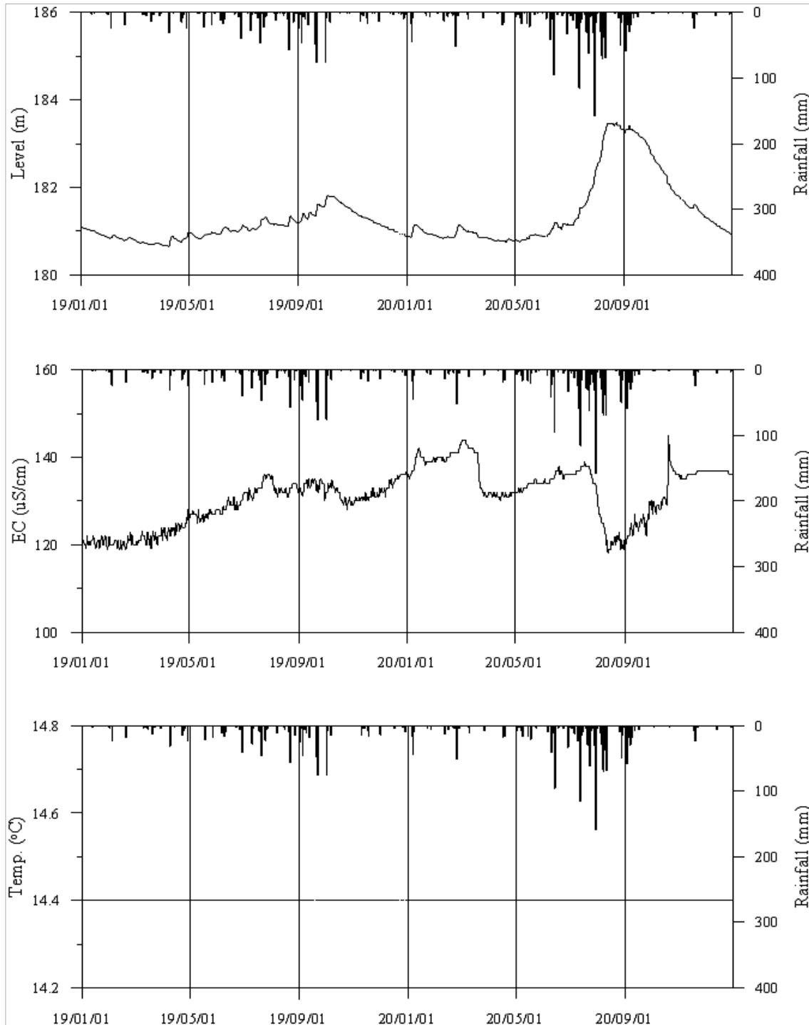
<금산6 관측공의 장기관측자료 (2019.1.1 ~ 2020.12.31)> (a)지하수위, (b)전기전도도, (c)수온
