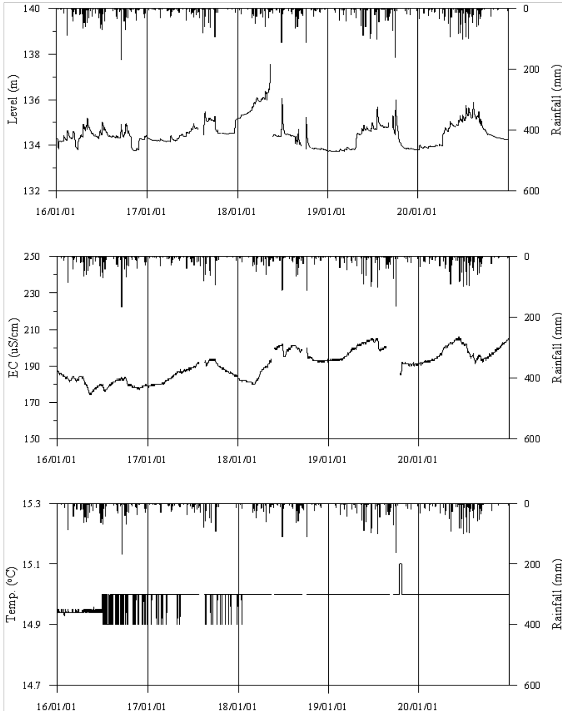
<보성2 관측공의 장기관측자료 (2016.1.1 ~ 2020.12.31)> (a)지하수위, (b)전기전도도, (c)수온
