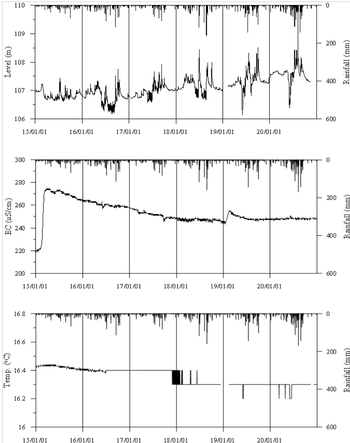
<곡성2 관측공의 장기관측자료 (2015.1.1~2020.12.31)> (a)지하수위, (b)전기전도도, (c)수온
