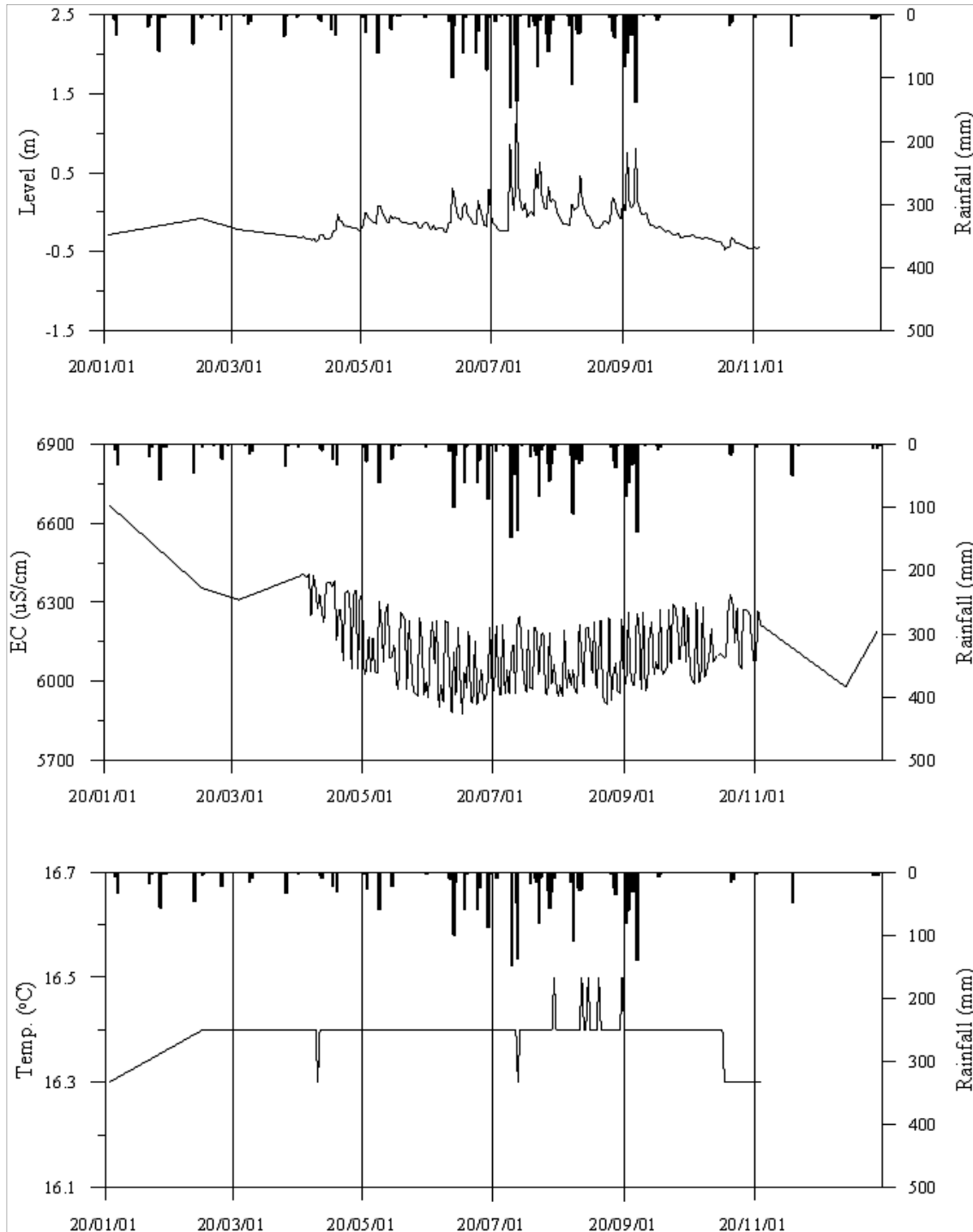
<경남고성3 관측공의 장기관측자료 (2020.1.1 ~ 2020.12.31)> (a)지하수위, (b)전기전도도, (c)수온
