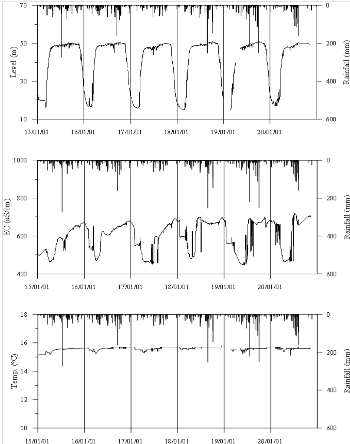
<산청3 관측공의 장기관측자료 (2015.1.1 ~ 2020.12.31)> (a)지하수위, (b)전기전도도, (c)수온
