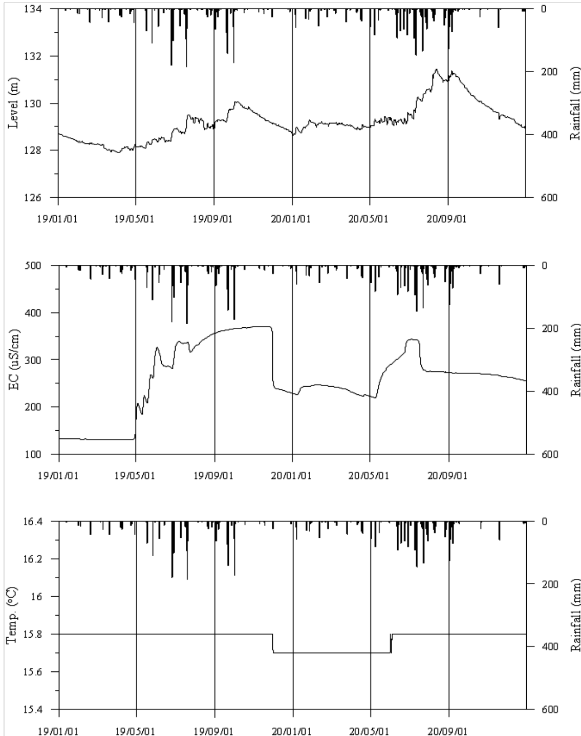
<하동4 관측공의 장기관측자료 (2019.1.1 ~ 2020.12.31)> (a)지하수위, (b)전기전도도, (c)수온
