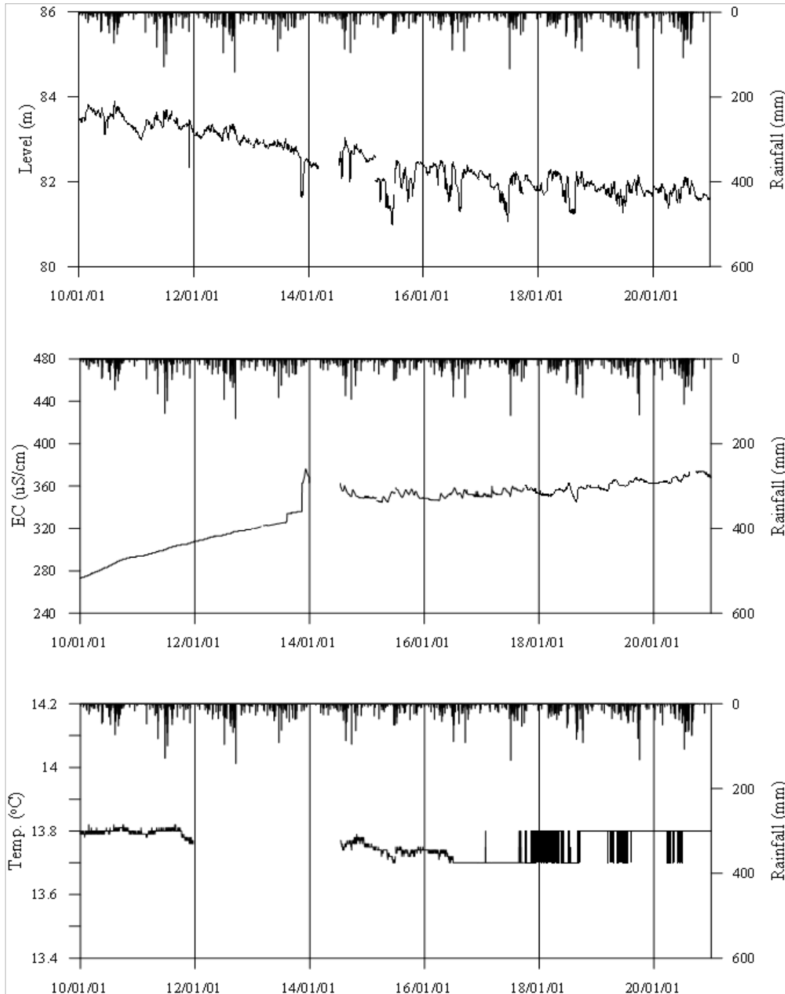
<상주2 관측공의 장기관측자료 (2010.1.1 ~ 2020.12.31)> (a)지하수위, (b)전기전도도, (c)수온
