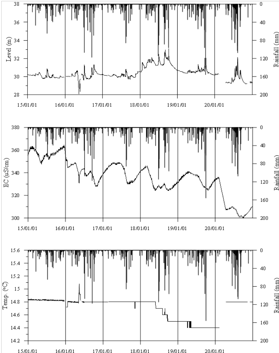
<구미1 관측공의 장기관측자료 (2015.1.1 ~ 2020.12.31)> (a) 지하수위, (b) 전기전도도, (c) 수온
