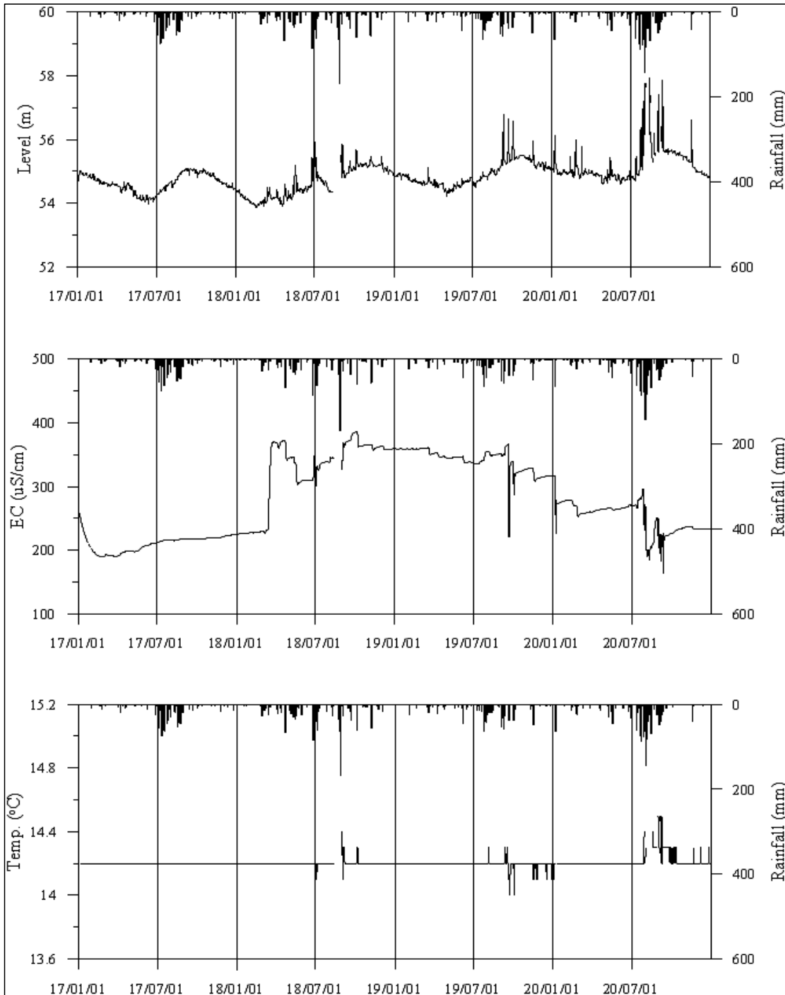
<여주4 관측공의 장기관측자료 (2017.1.1. ~ 2020.12.31)> (a)지하수위, (b)전기전도도, (c)수온
