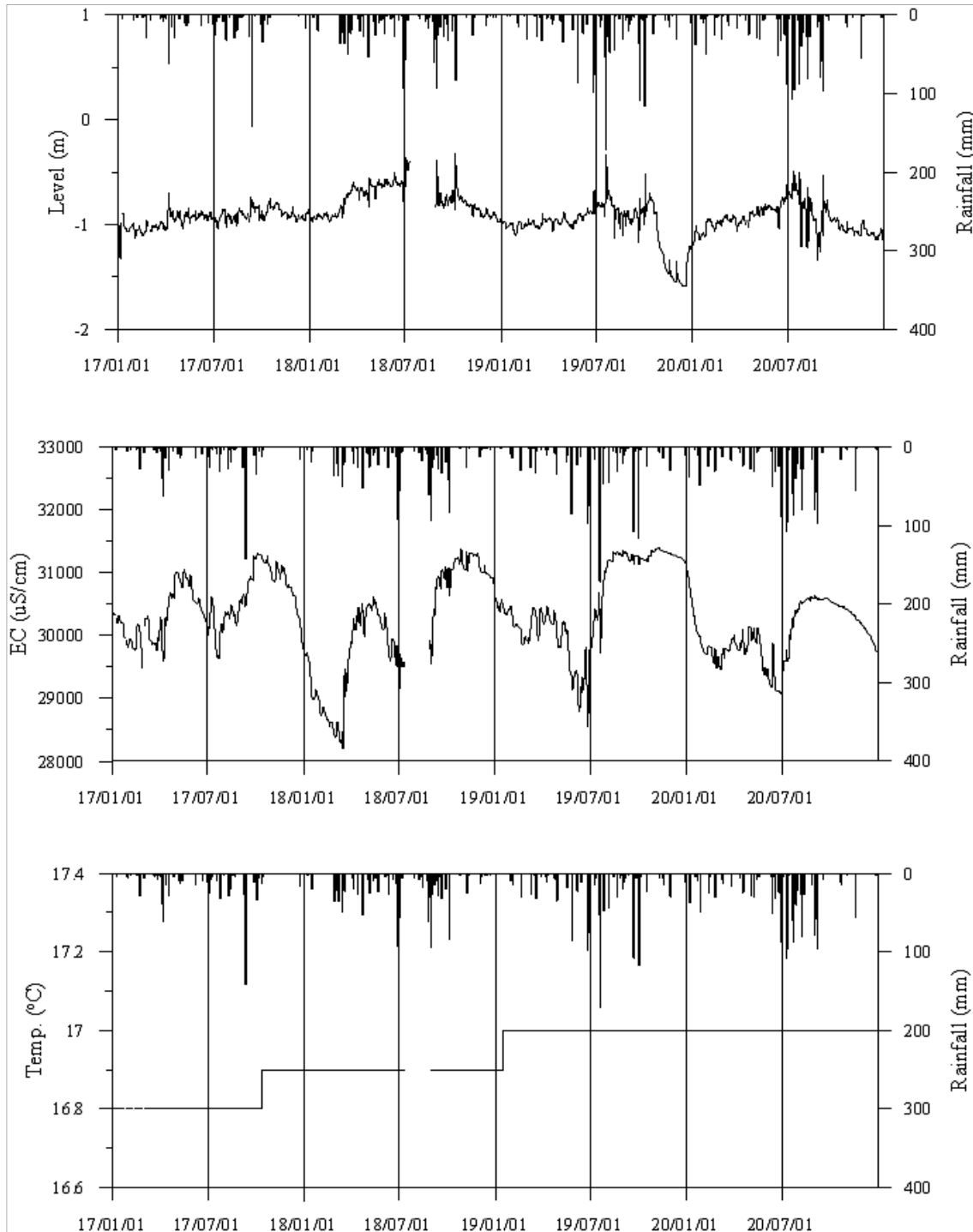
<김해4 관측공의 장기관측자료 (2017.1.1 ~ 2020.12.31)> (a)지하수위, (b)전기전도도, (c)수온
