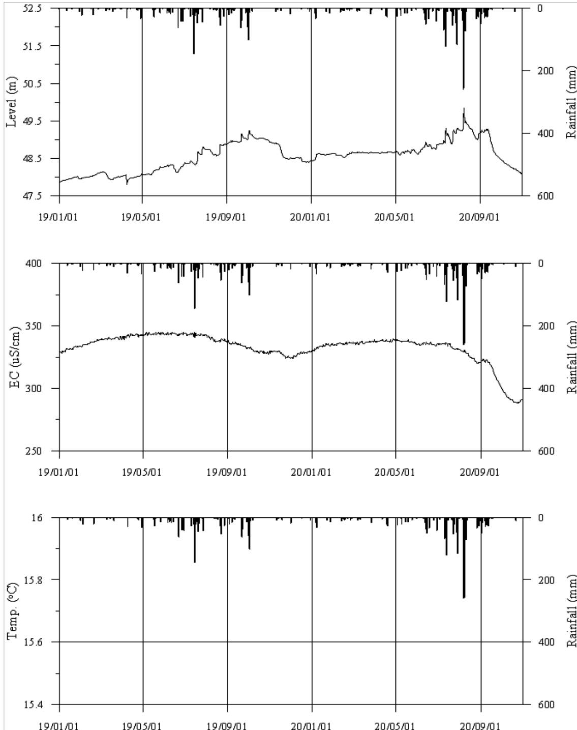
<담양1 관측공의 장기관측자료 (2019.1.1~2020.10.31)> (a)지하수위, (b)전기전도도, (c)수온
