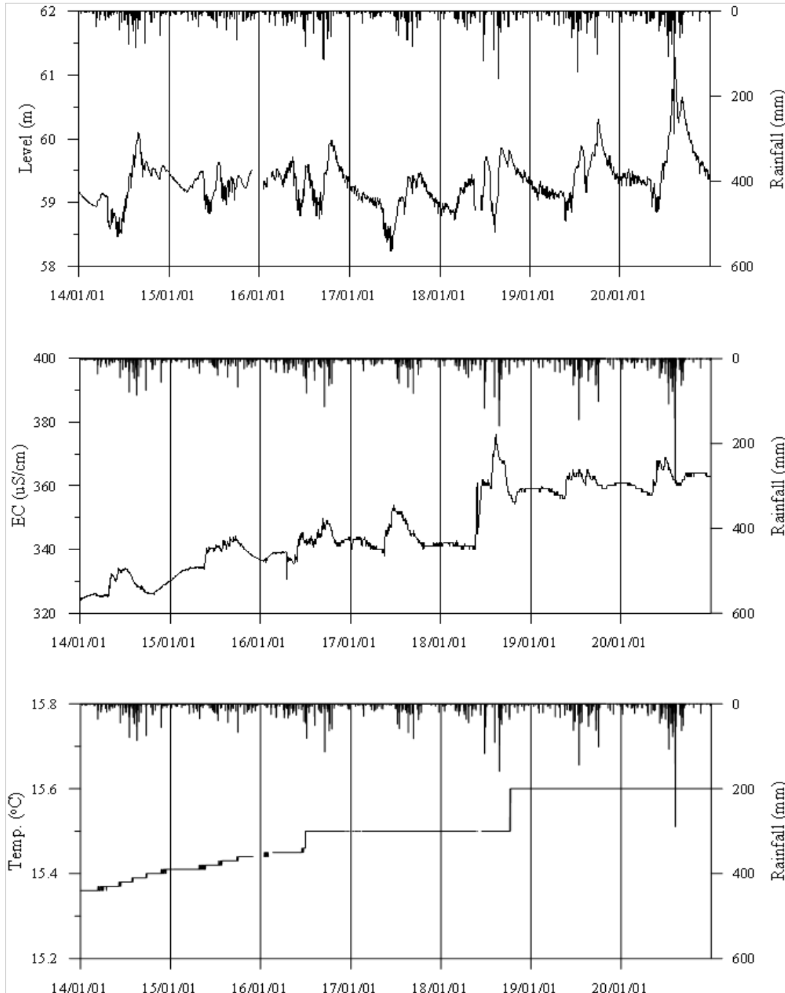
<곡성1 관측공의 장기관측자료 (2014.1.1~2020.12.31)> (a)지하수위, (b)전기전도도, (c)수온
