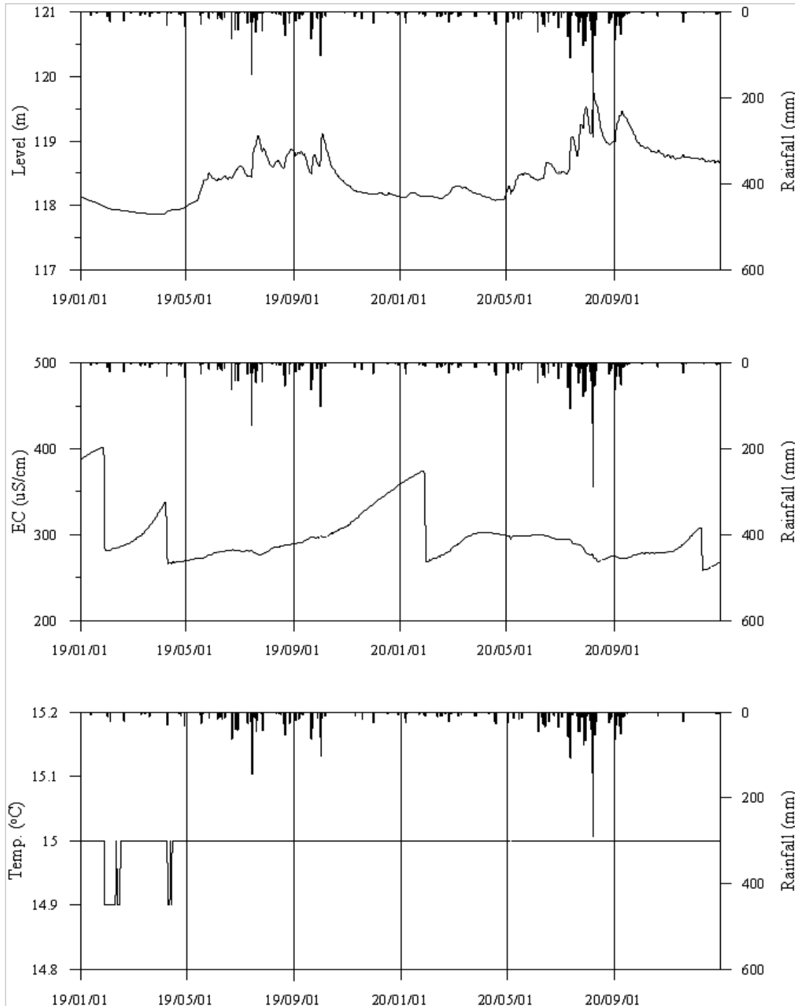
<남원4 관측공의 장기관측자료 (2019.1.1 ~ 2020.12.31)> (a)지하수위, (b)전기전도도, (c)수온
