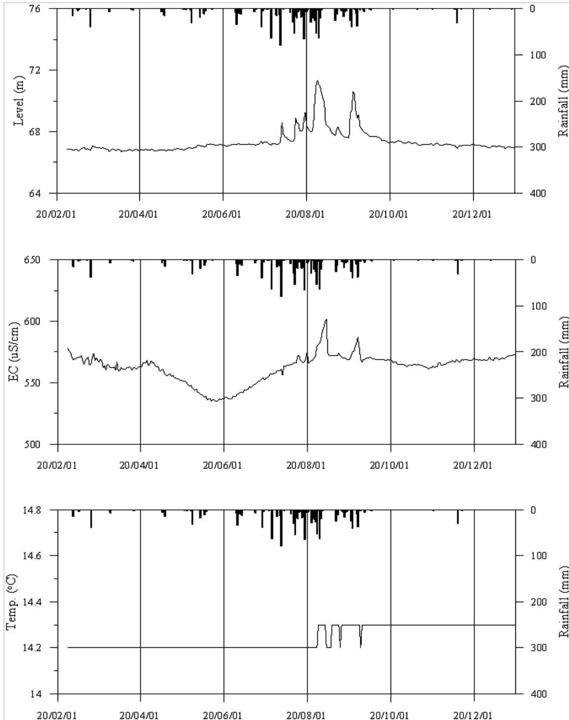
<안동4(신) 관측공의 장기관측자료 (2020.2.1 ~ 2020.12.31)> (a)지하수위, (b)전기전도도, (c)수온
