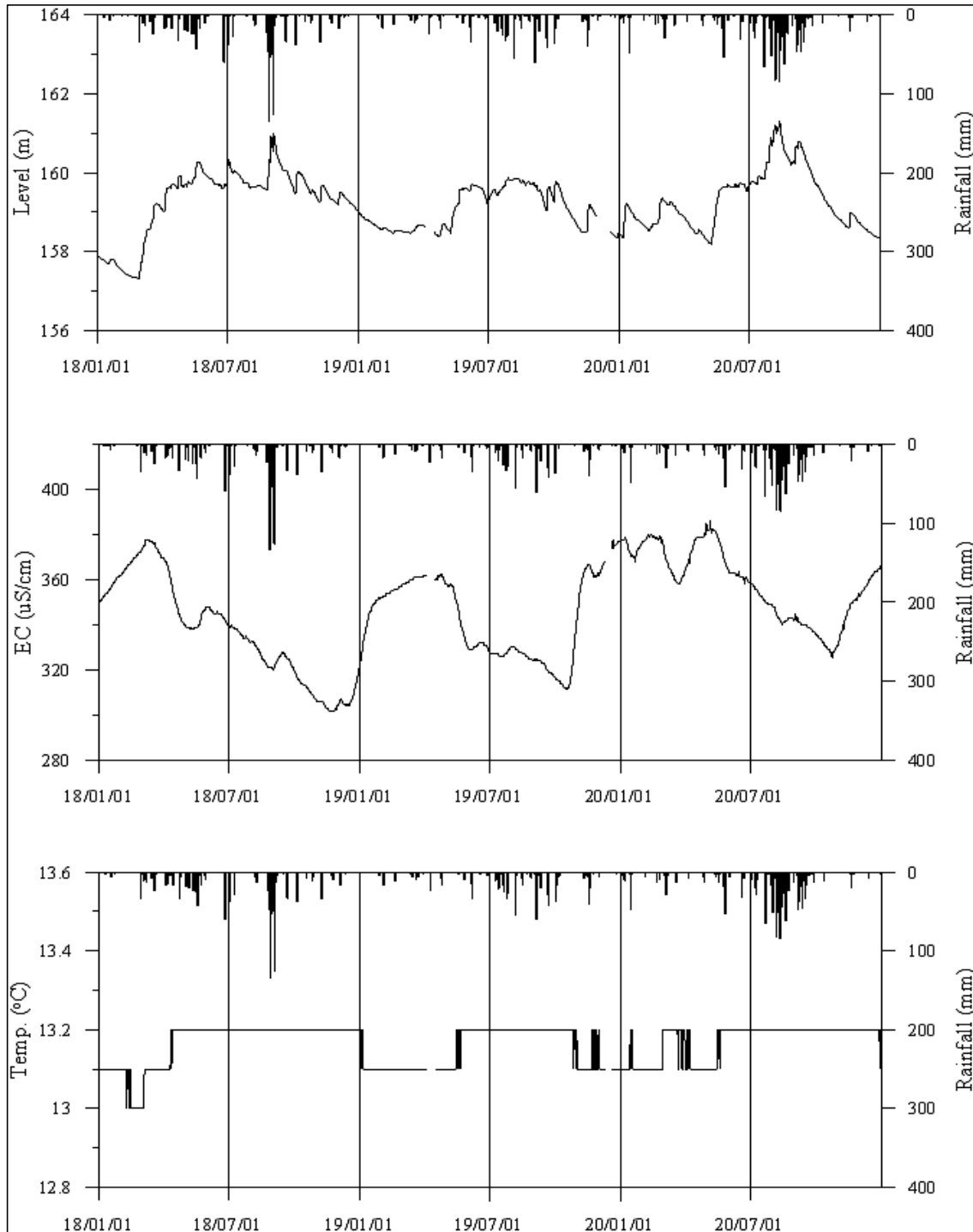
<충주3 관측공의 장기관측자료 (2018.1.1 ~ 2020.12.31)> (a)지하수위, (b)전기전도도, (c)수온
