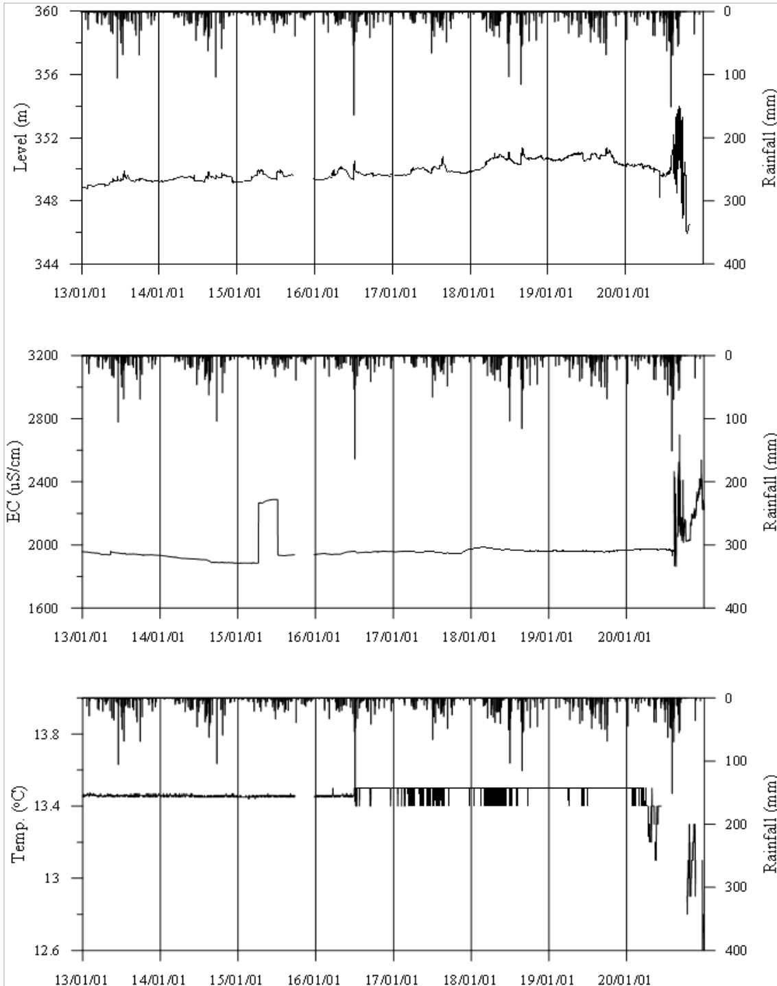
<봉화1 관측공의 장기관측자료 (2013.1.1 ~ 2020.12.31)> (a)지하수위, (b)전기전도도, (c)수온
