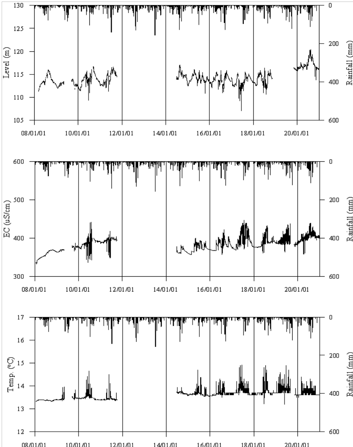
<영천1 관측공의 장기관측자료 (2008.1.1 ~ 2020.12.31)> (a)지하수위, (b)전기전도도, (c)수온
