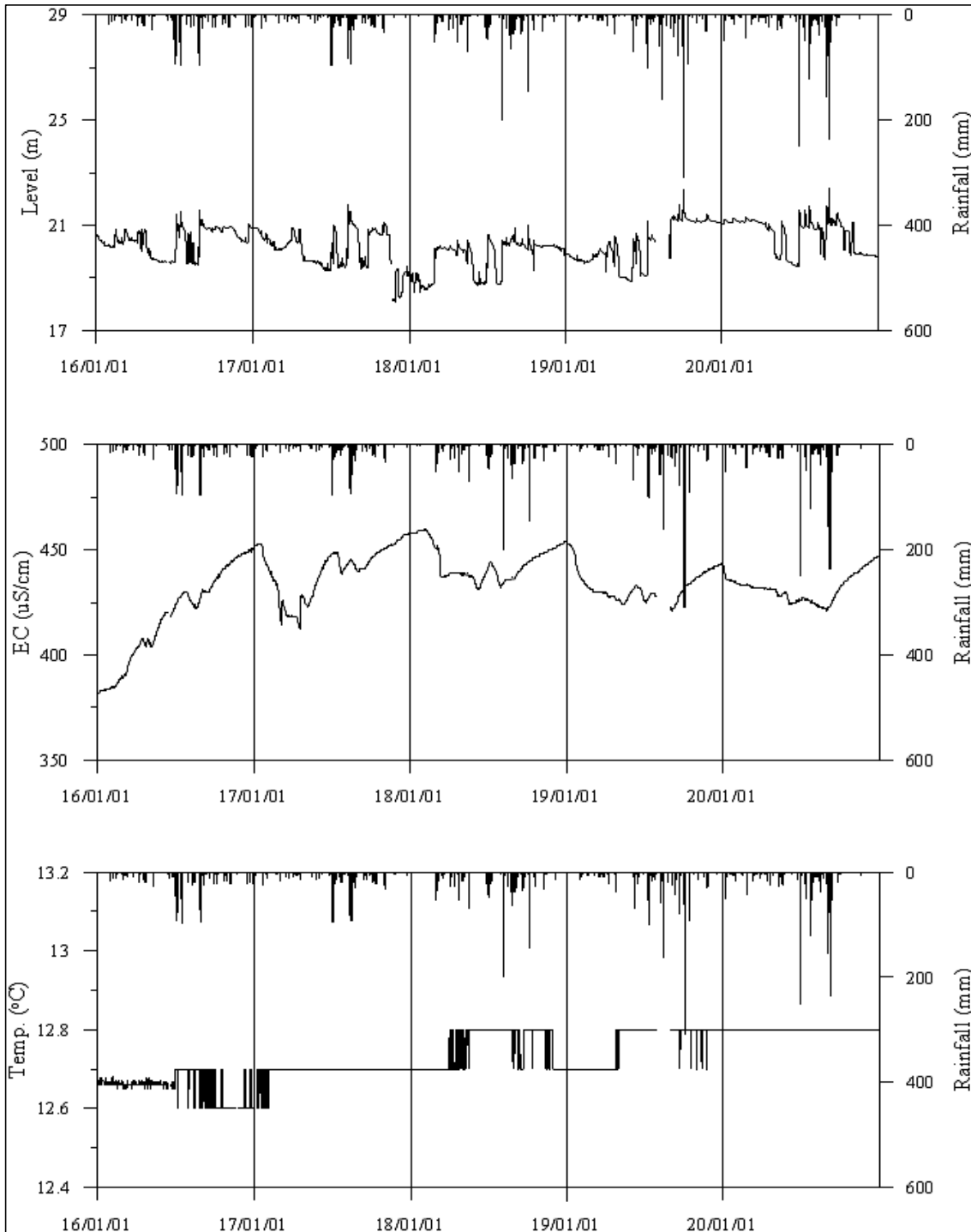
<강릉3 관측공의 장기관측자료 (2016.1.1 ~ 2020.12.31)> (a)지하수위, (b)전기전도도, (c)수온
