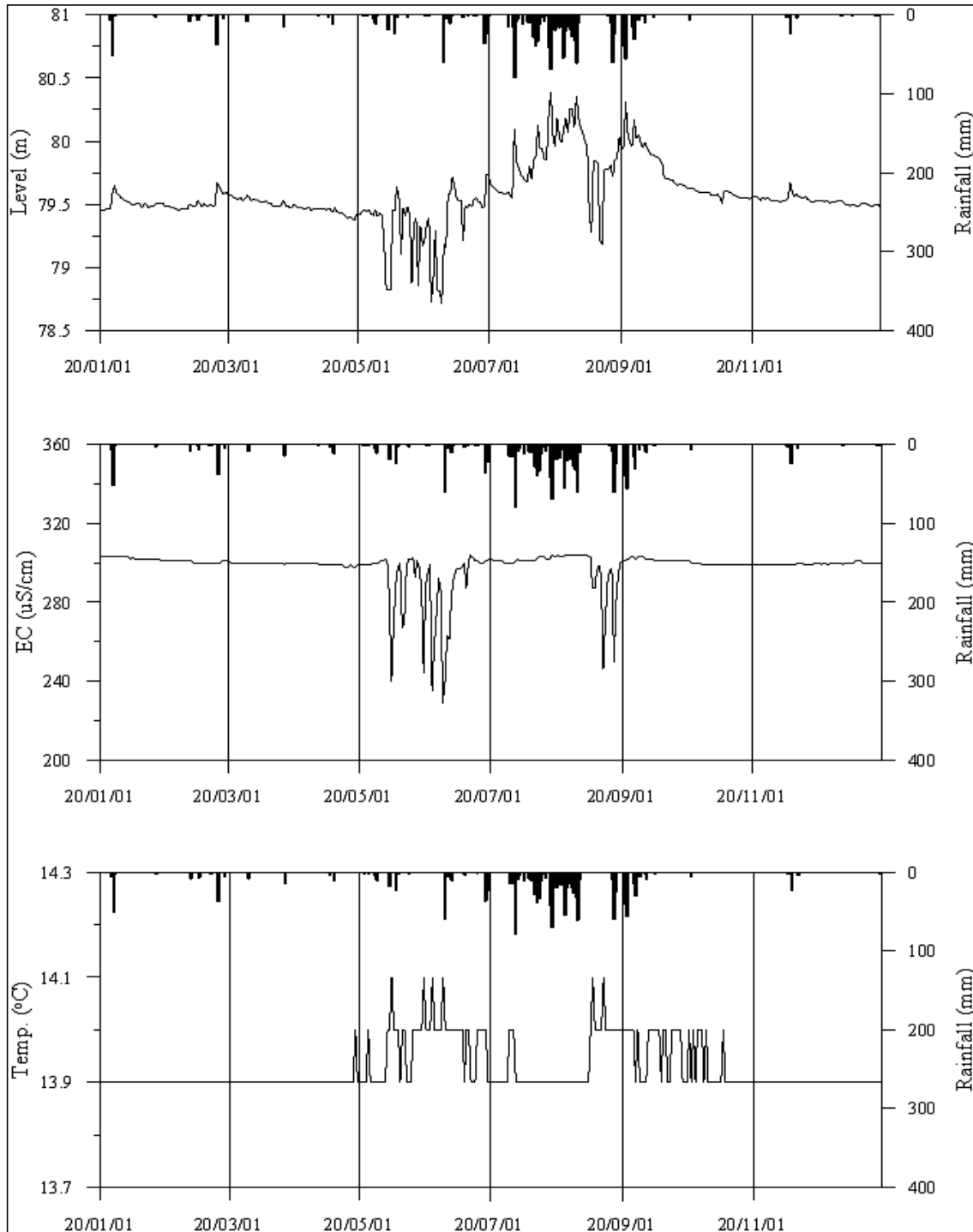
<청주3 관측공의 장기관측자료 (2020.1.1 ~ 2020.12.31)> (a)지하수위, (b)전기전도도, (c)수온
