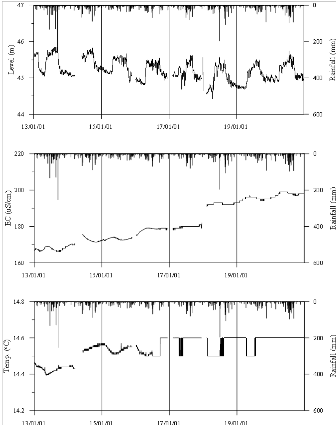
<청양1 관측공의 장기관측자료 (2013.1.1 ~ 2020.12.31)> (a)지하수위, (b)전기전도도, (c)수온
