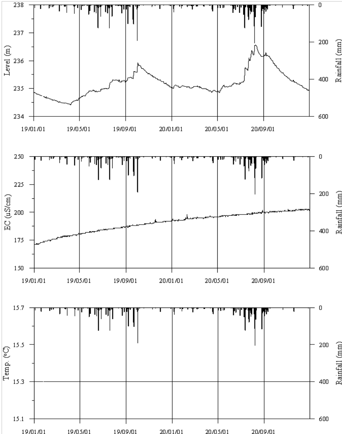
<함양1 관측공의 장기관측자료 (2019.1.1 ~ 2020.12.31)> (a)지하수위, (b)전기전도도, (c)수온
