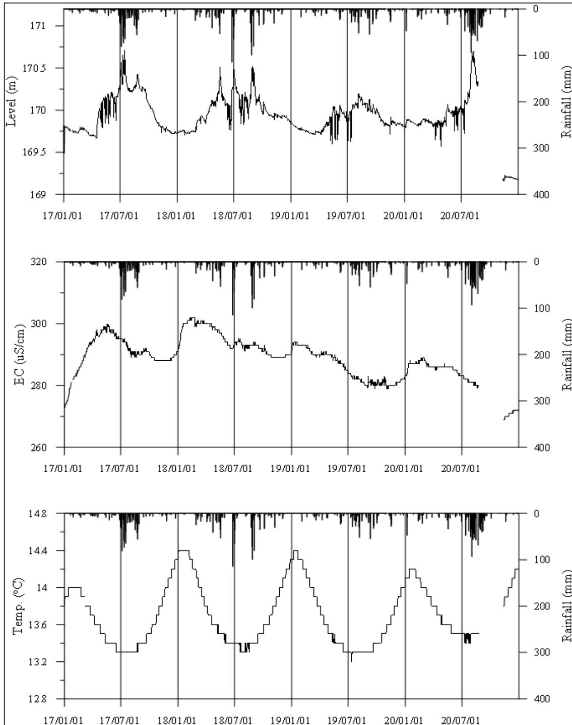
<원주5 관측공의 장기관측자료 (2017.1.1 ~ 2020.12.31)> (a)지하수위, (b)전기전도도, (c)수온
