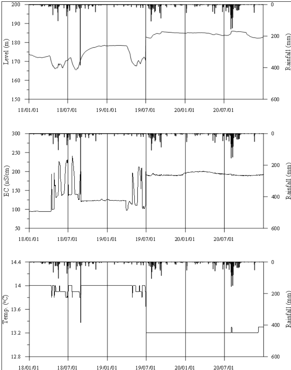
<철원3 관측공의 장기관측자료 (2018.1.1 ~ 2020.12.31)> (a)지하수위, (b)전기전도도, (c)수온
