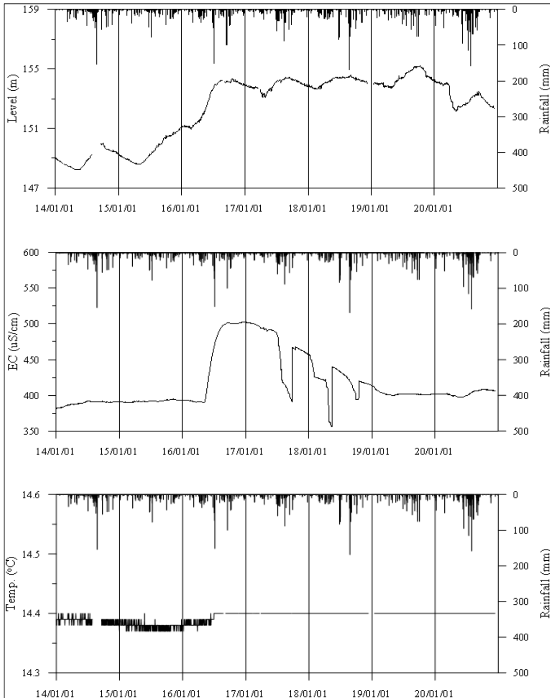
<영동2 관측공의 장기관측자료 (2014.1.1 ~ 2020.12.31)> (a)지하수위, (b)전기전도도, (c)수온
