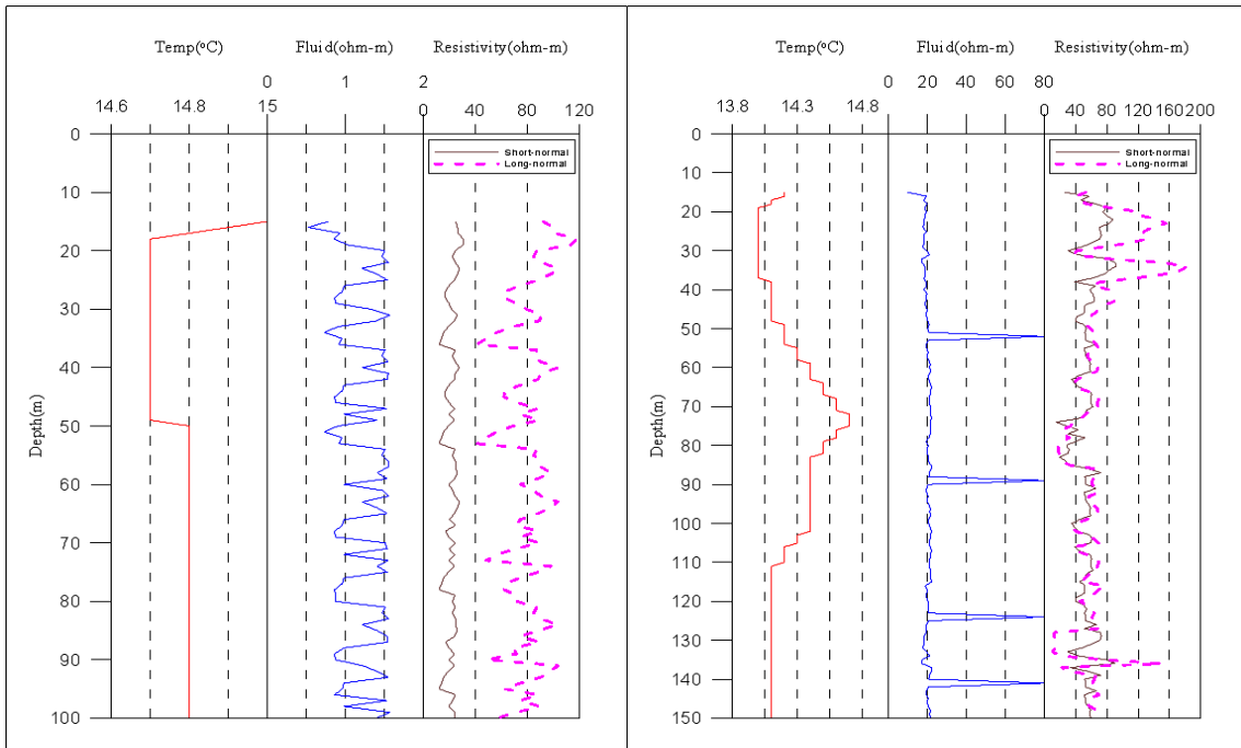
<예천4 관측공 물리검층>
