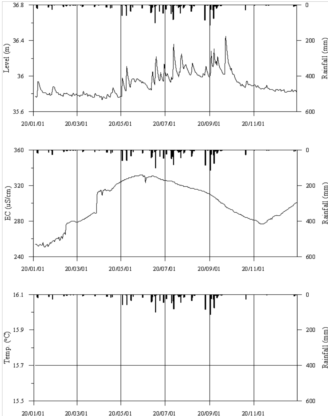
<해남7 관측공의 장기관측자료 (2020.1.1~2020.12.31)> (a)지하수위, (b)전기전도도, (c)수온
