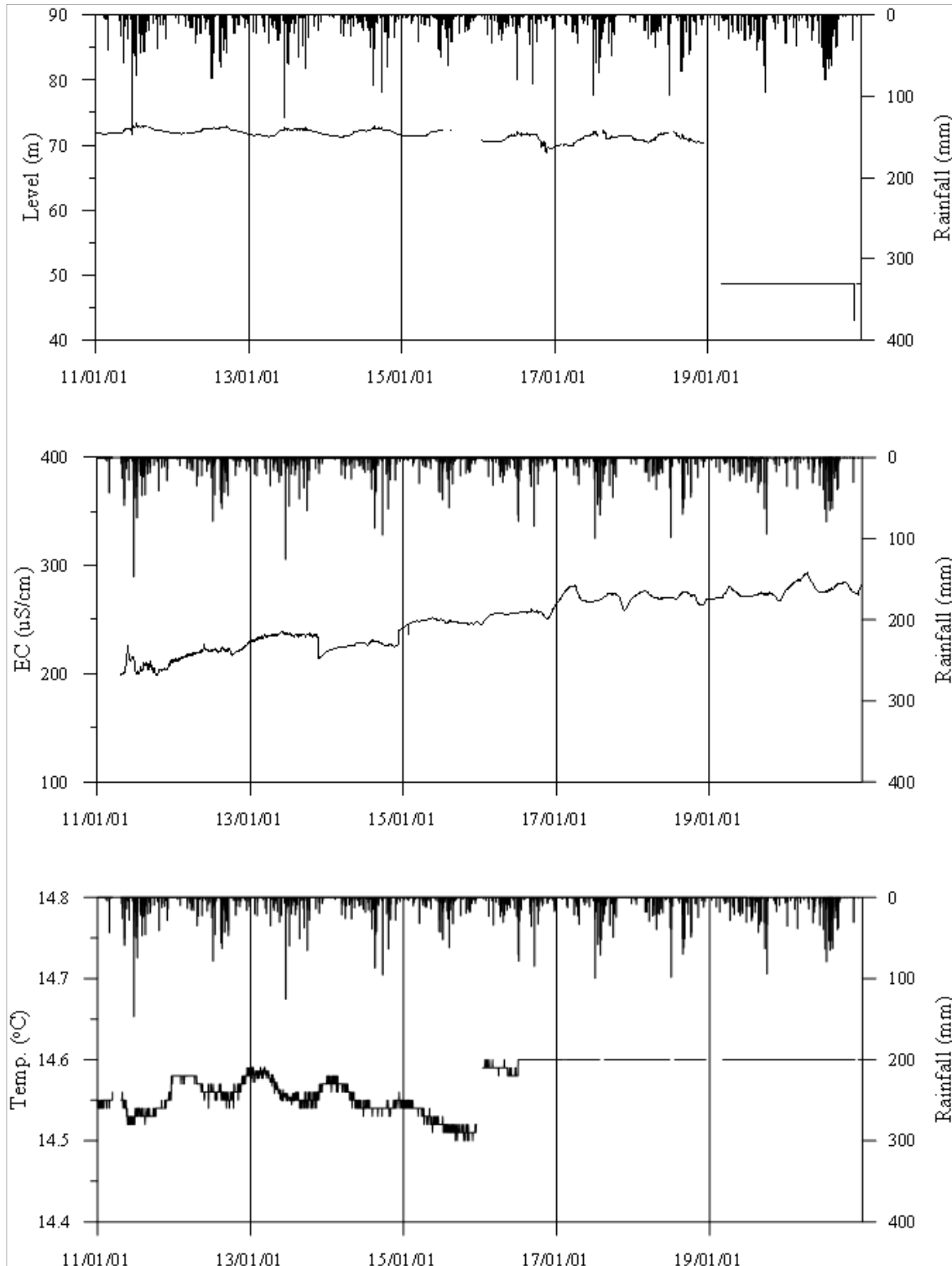
<안동2 관측공의 장기관측자료 (2011.1.1 ~ 2020.12.31)> (a)지하수위, (b)전기전도도, (c)수온
