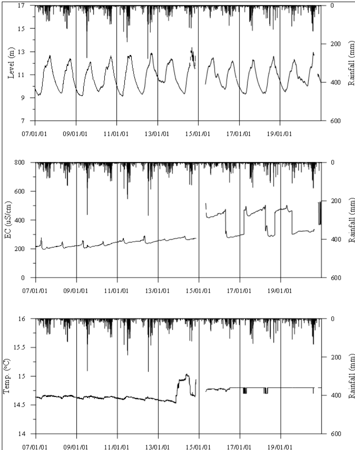
<평택3 관측공의 장기관측자료 (2007.1.1 ~ 2020.12.31)> (a)지하수위, (b)전기전도도, (c)수온
