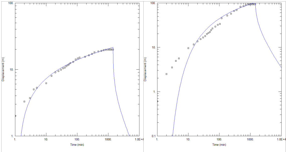
<예천4 관측공 양수시험>
