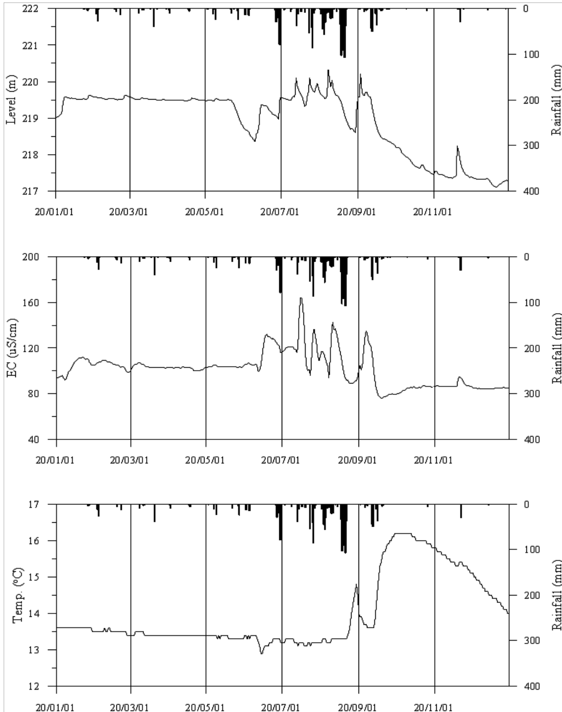
<김천4 관측공의 장기관측자료 (2020.1.1 ~ 2020.12.31.)> (a)지하수위, (b)전기전도도, (c)수온
