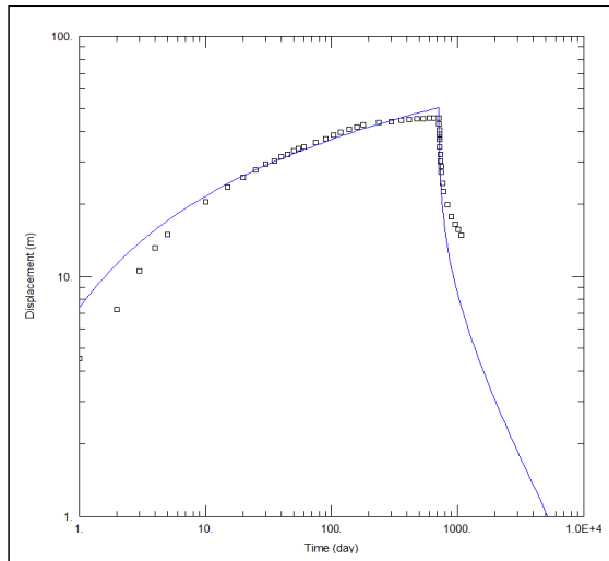
<영월9 관측공 양수시험>
