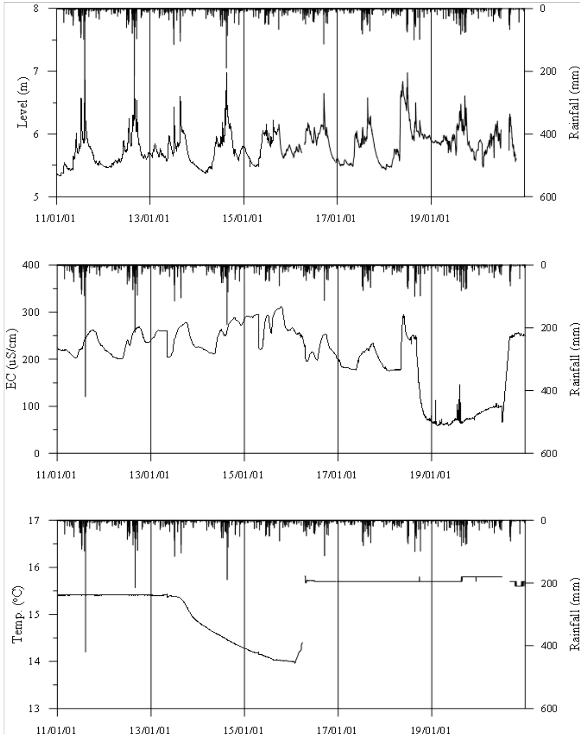
<고창1 관측공의 장기관측자료 (2011.1.1 ~ 2020.12.31)> (a)지하수위, (b)전기전도도, (c)수온
