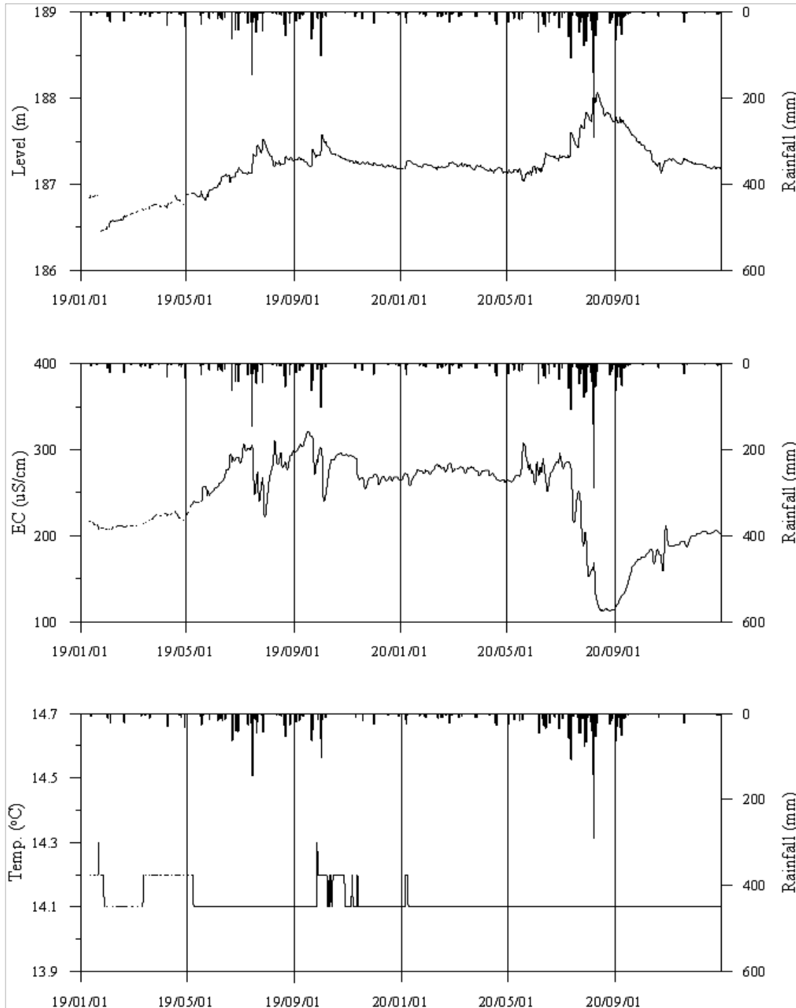
<남원6 관측공의 장기관측자료 (2019.1.1 ~ 2020.12.31)> (a)지하수위, (b)전기전도도, (c)수온
