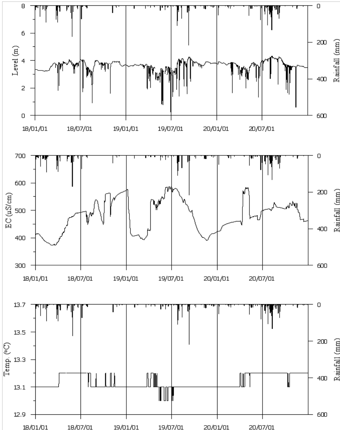
<강화3 관측공의 장기관측자료 (2008.1.1 ~ 2020.12.31)> (a)지하수위, (b)전기전도도, (c)수온
