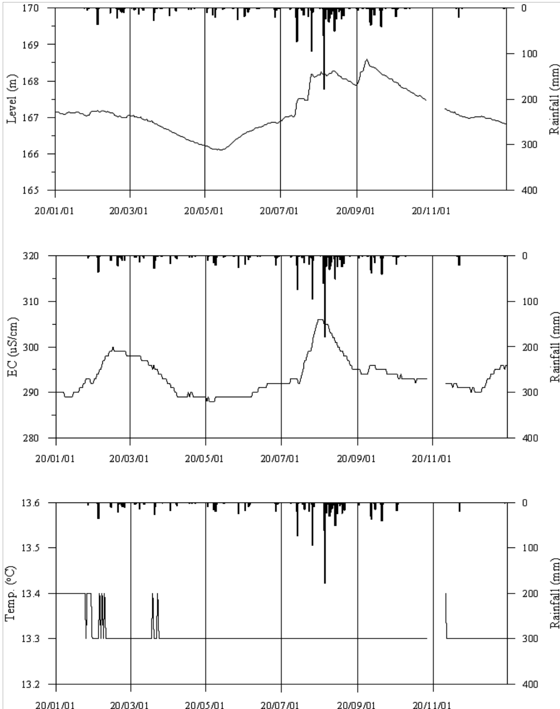
<울진1 관측공의 장기관측자료 (2020.1.1 ~ 2020.12.31.)> (a)지하수위, (b)전기전도도, (c)수온
