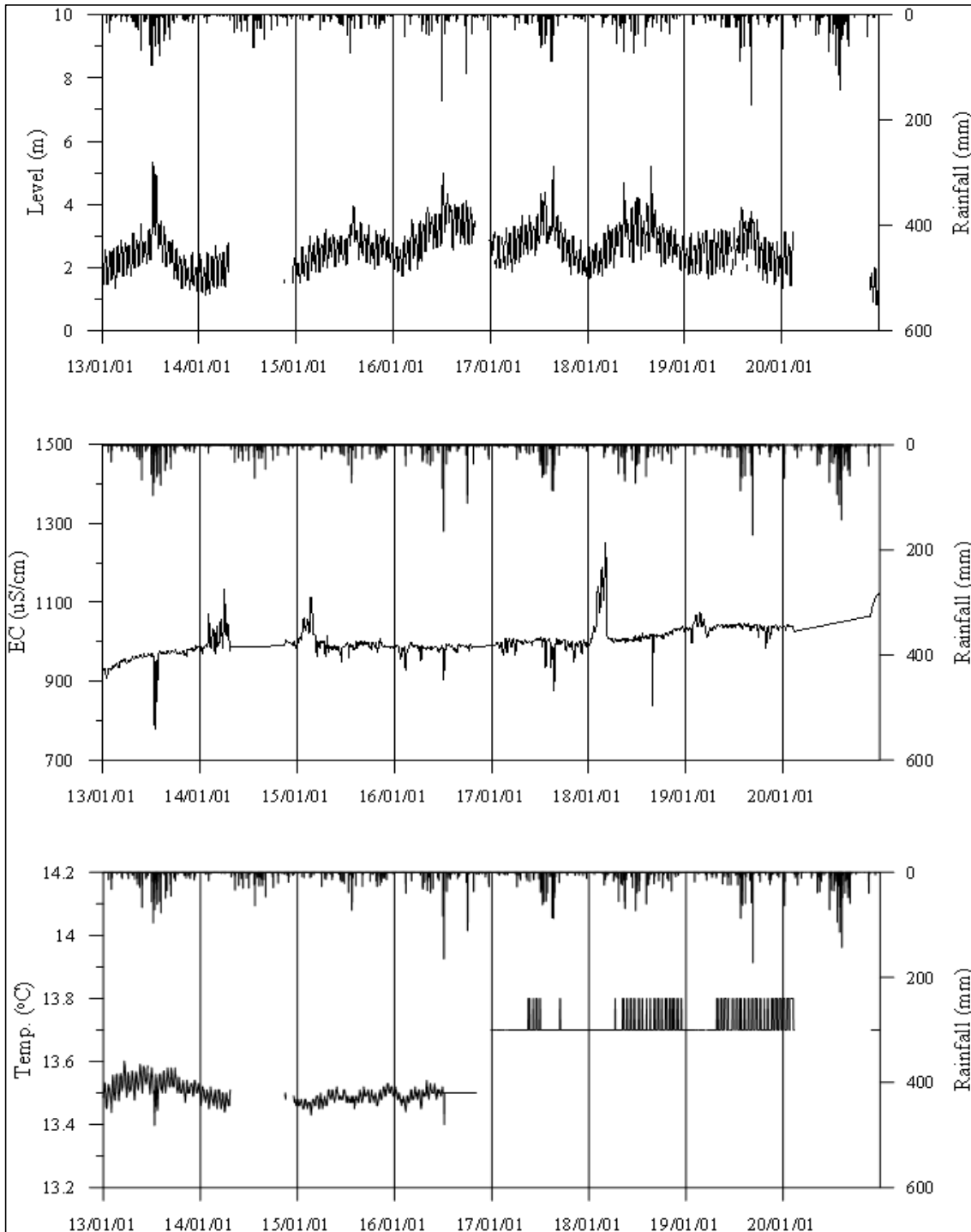
<파주3 관측공의 장기관측자료 (2013.1.1 ~ 2020.12.31)> (a)지하수위, (b)전기전도도, (c)수온
