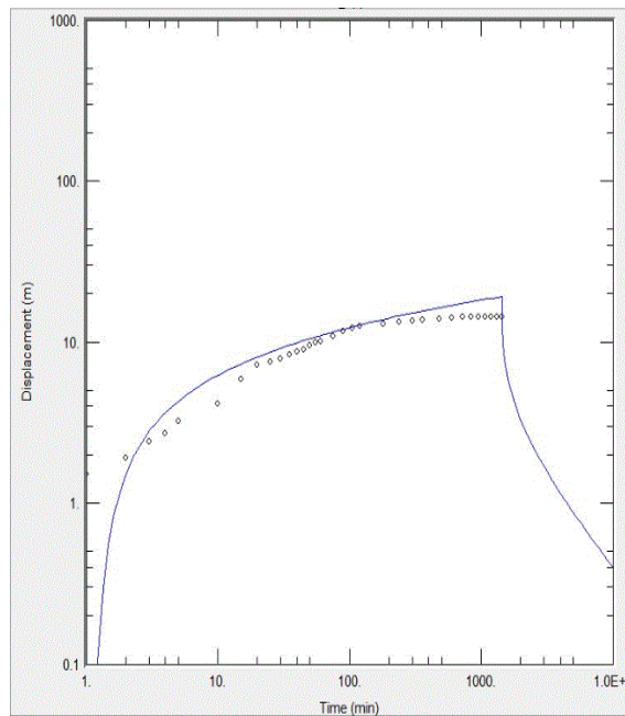
<의성10 관측공 양수시험>
