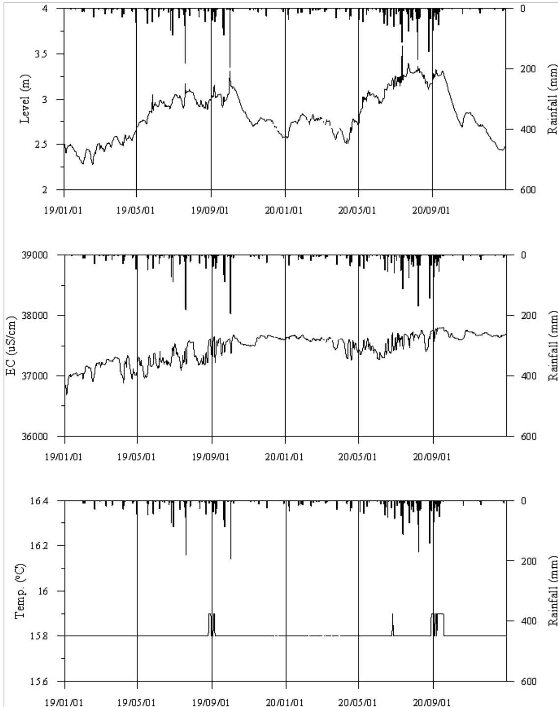
<순천6 관측공의 장기관측자료 (2019.1.1~2020.12.31)> (a)지하수위, (b)전기전도도, (c)수온
