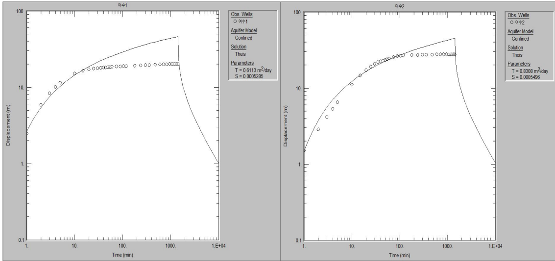
<여수1 관측공 양수시험>
