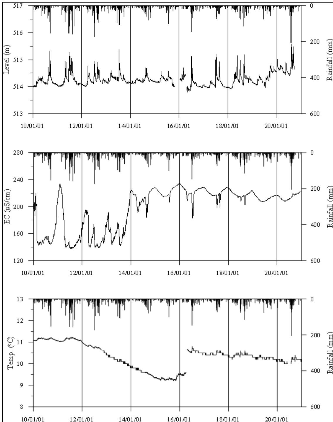
<평창2 관측공의 장기관측자료 (2010.1.1 ~ 2020.12.31)> (a)지하수위, (b)전기전도도, (c)수온
