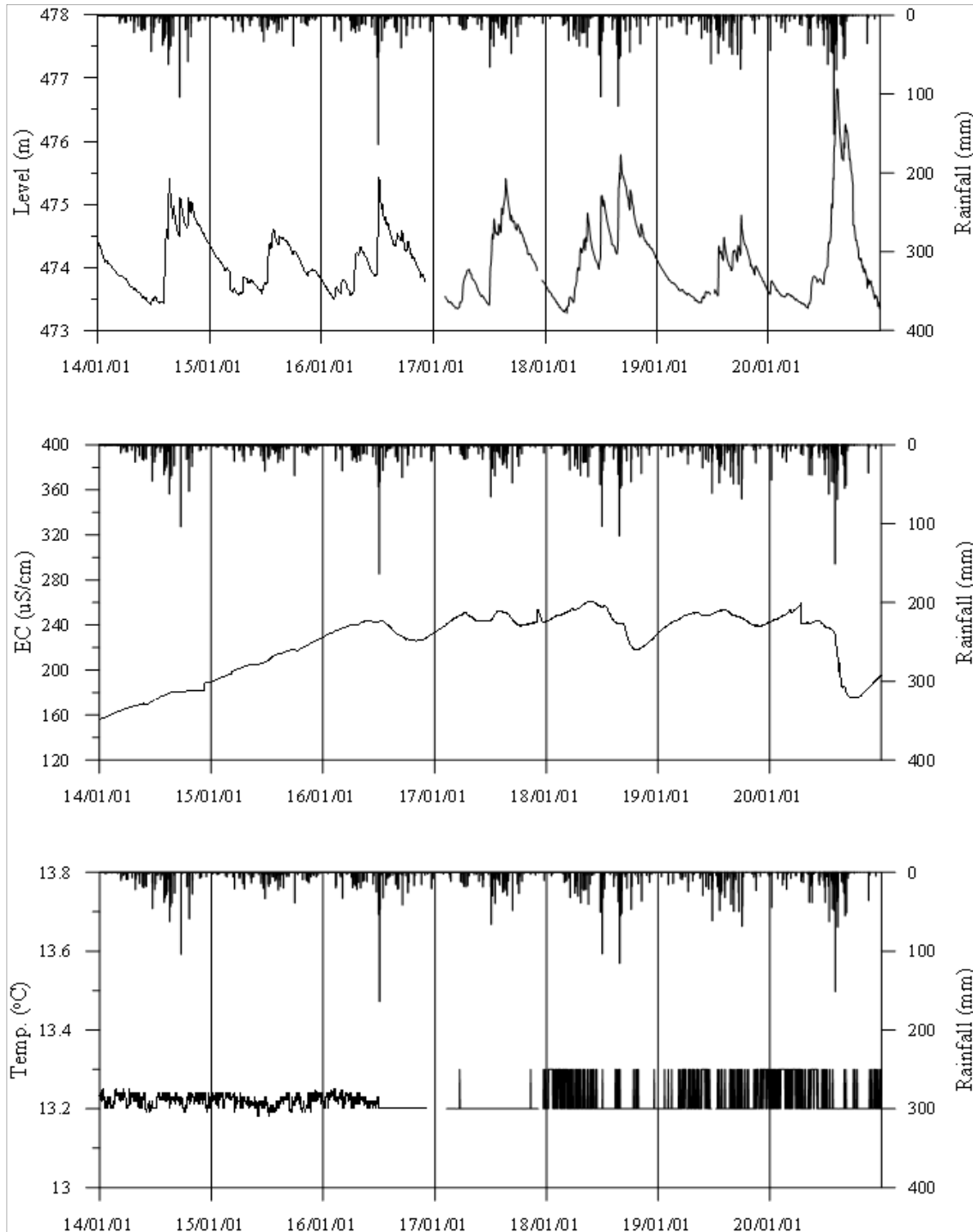
<봉화4 관측공의 장기관측자료 (2014.1.1 ~ 2020.12.31)> (a)지하수위, (b)전기전도도, (c)수온
