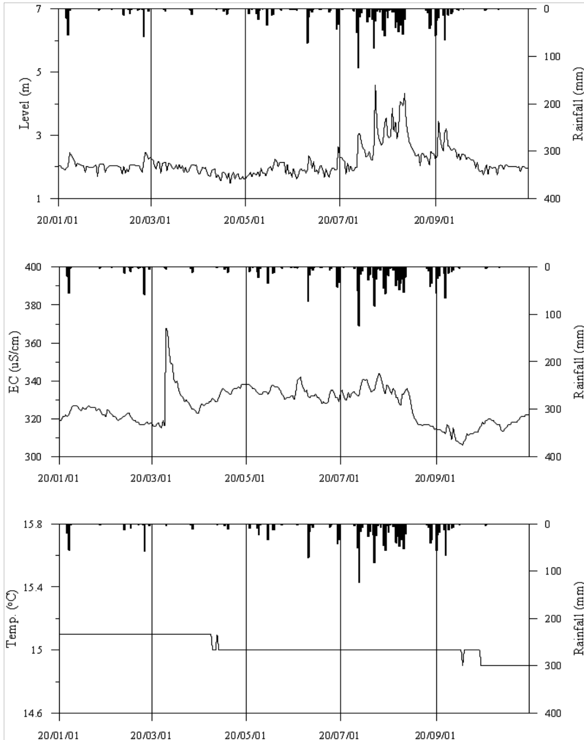
<청양4 관측공의 장기관측자료 (2020.1.1 ~ 2020.12.31)> (a)지하수위, (b)전기전도도, (c)수온
