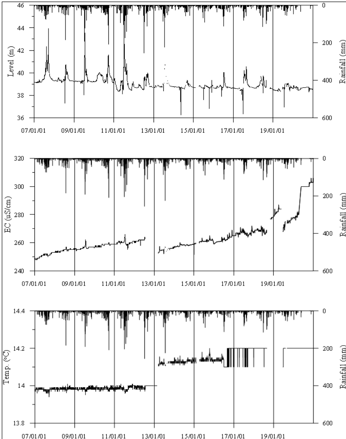
<원주4 관측공의 장기관측자료 (2007.1.1 ~ 2020.12.31)> (a)지하수위, (b)전기전도도, (c)수온
