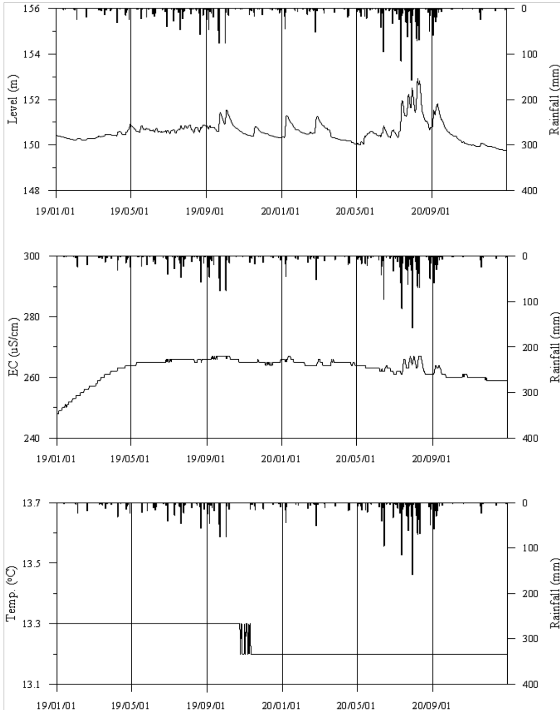
<금산5 관측공의 장기관측자료 (2019.1.1 ~ 2020.12.31)> (a)지하수위, (b)전기전도도, (c)수온
