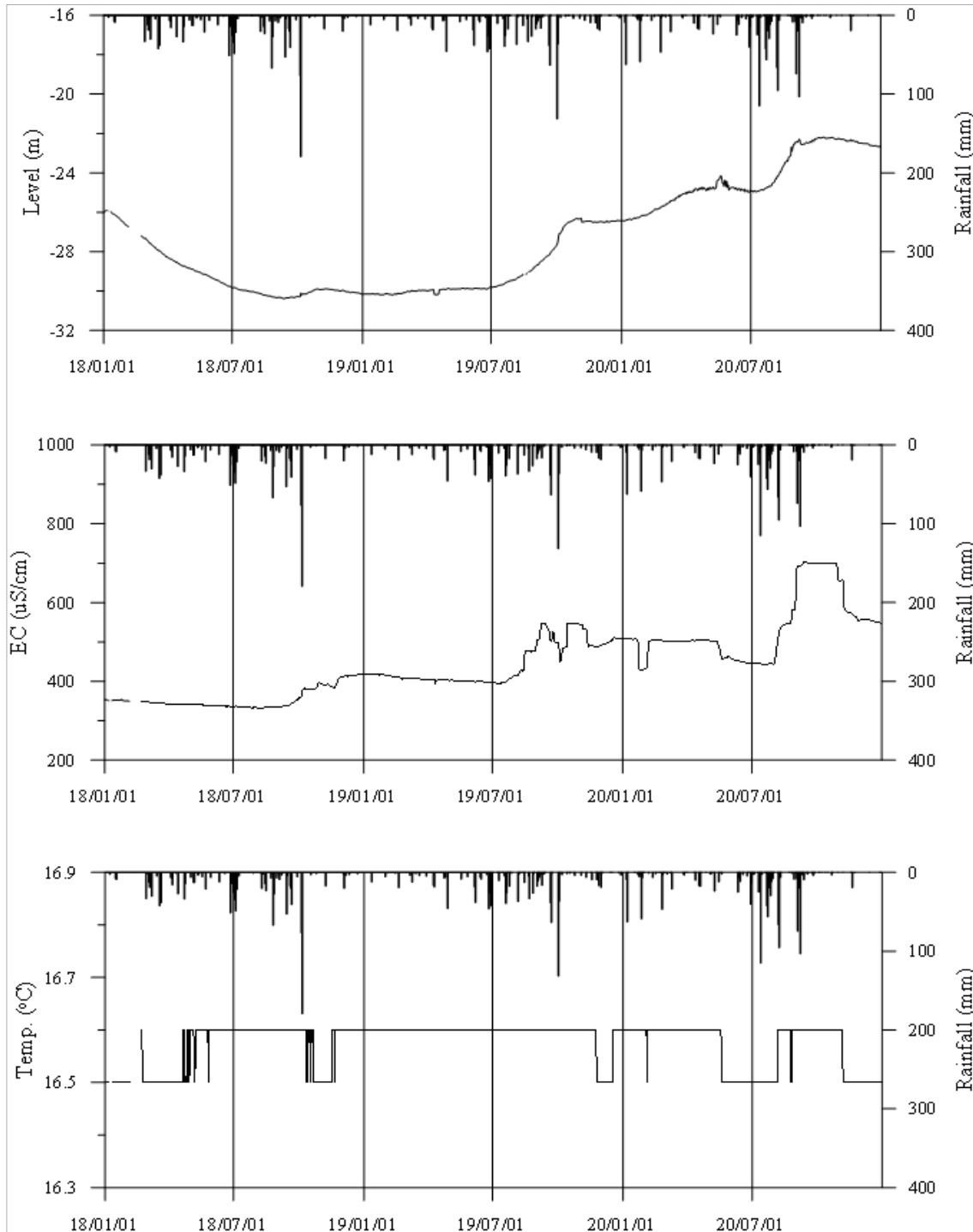
<포항6 관측공의 장기관측자료 (2018.1.1 ~ 2020.12.31)> (a)지하수위, (b)전기전도도, (c)수온
