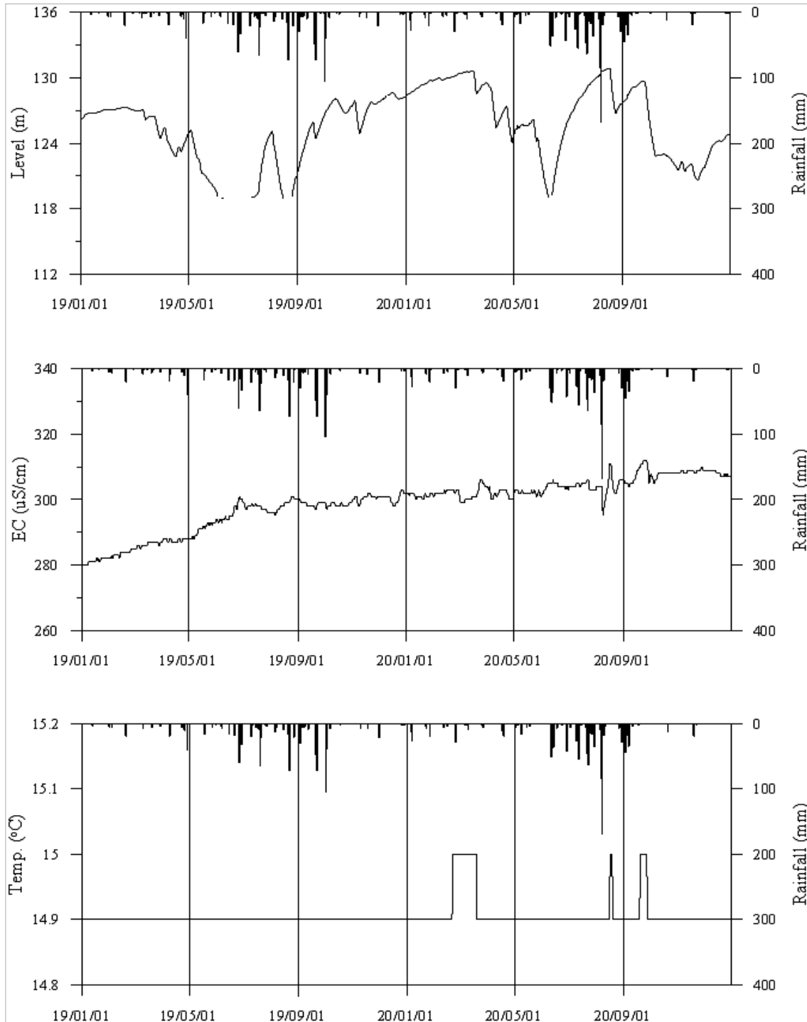
<청도2 관측공의 장기관측자료 (2019.1.1 ~ 2020.12.31.)> (a)지하수위, (b)전기전도도, (c)수온
