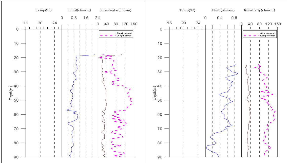
<울진1 관측공 물리검층>
