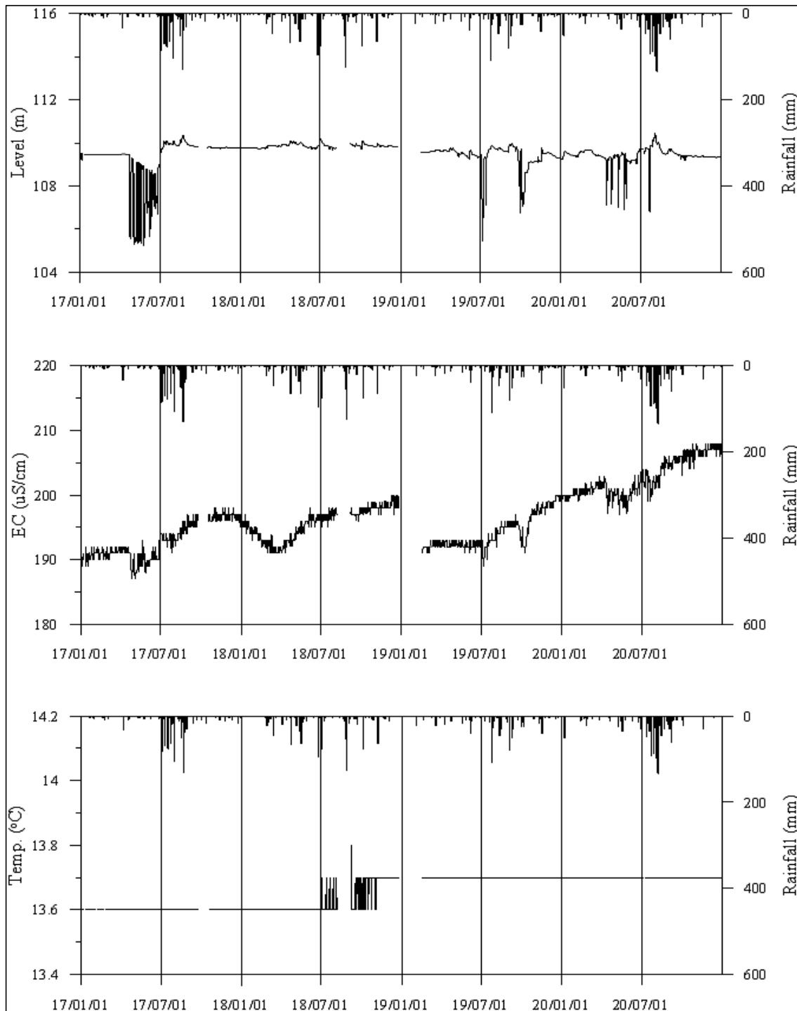
<용인3 관측공의 장기관측자료 (2017.1.1 ~ 2020.12.31)> (a)지하수위, (b)전기전도도, (c)수온
