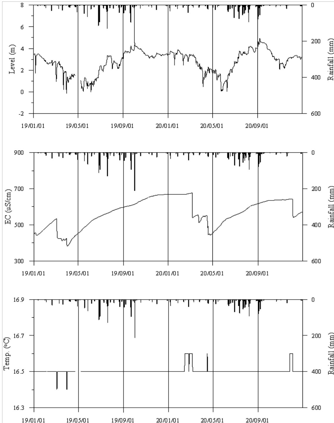
<함안3 관측공의 장기관측자료 (2019.1.1 ~ 2020.12.31)> (a)지하수위, (b)전기전도도, (c)수온
