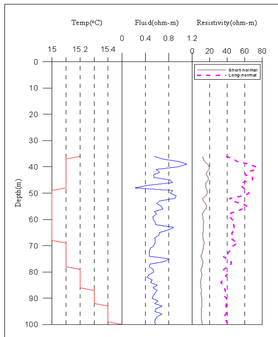
<예천6 관측공 물리검층>
