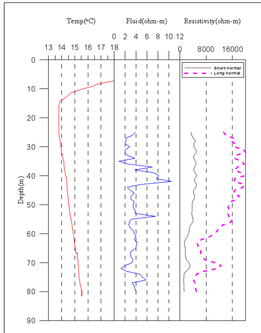
<영월9 관측공 물리검층>
