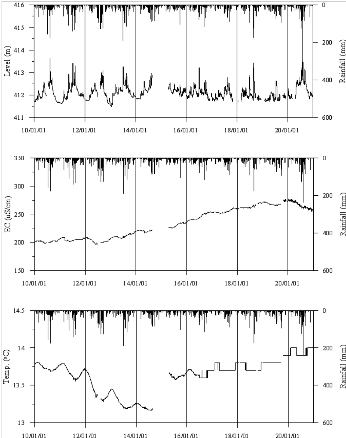
<장수1 관측공의 장기관측자료 (2010.1.1 ~ 2020.12.31)> (a)지하수위, (b)전기전도도, (c)수온
