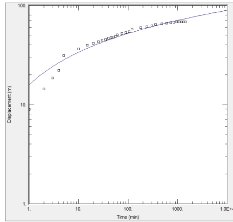
<경남고성3 관측공 양수시험>
