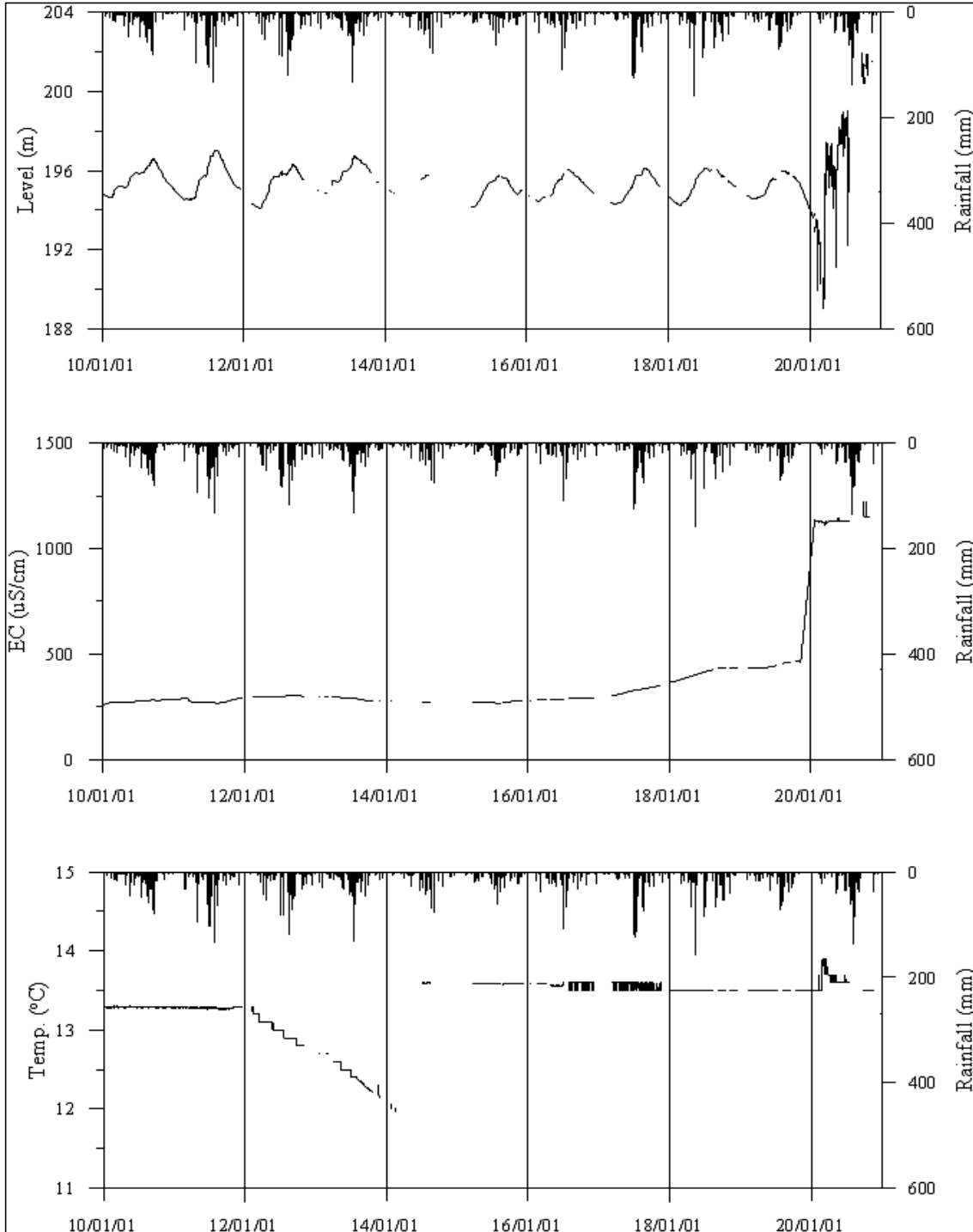
<홍천1 관측공의 장기관측자료 (2010.1.1 ~ 2020.12.31)> (a)지하수위, (b)전기전도도, (c)수온
