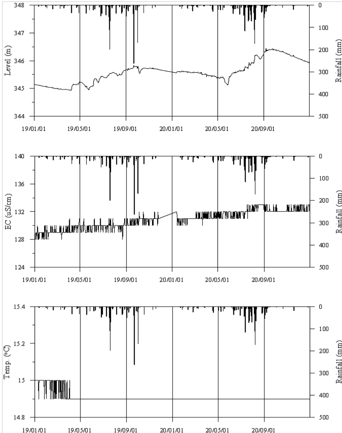
<거창3 관측공의 장기관측자료 (2019.1.1 ~ 2020.12.31)> (a)지하수위, (b)전기전도도, (c)수온
