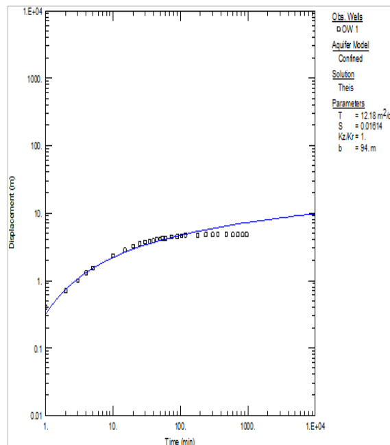
<하동7 관측공 양수시험>
