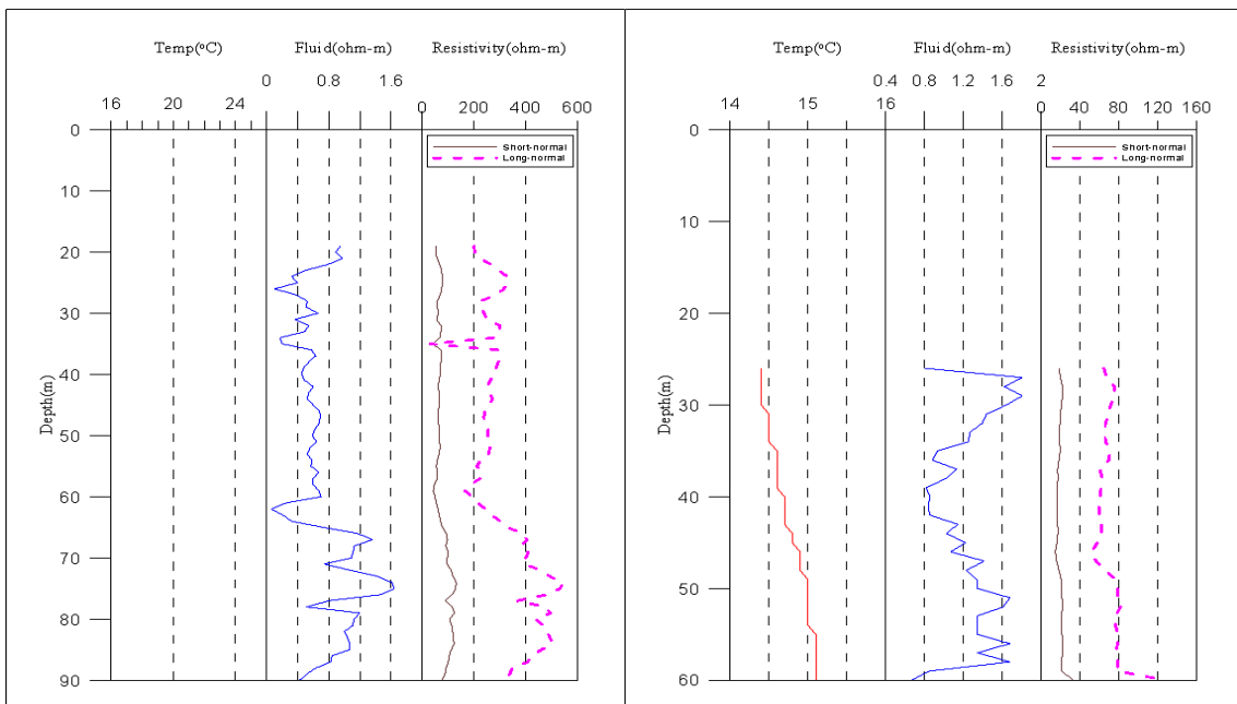
<영주1 관측공 물리검층>
