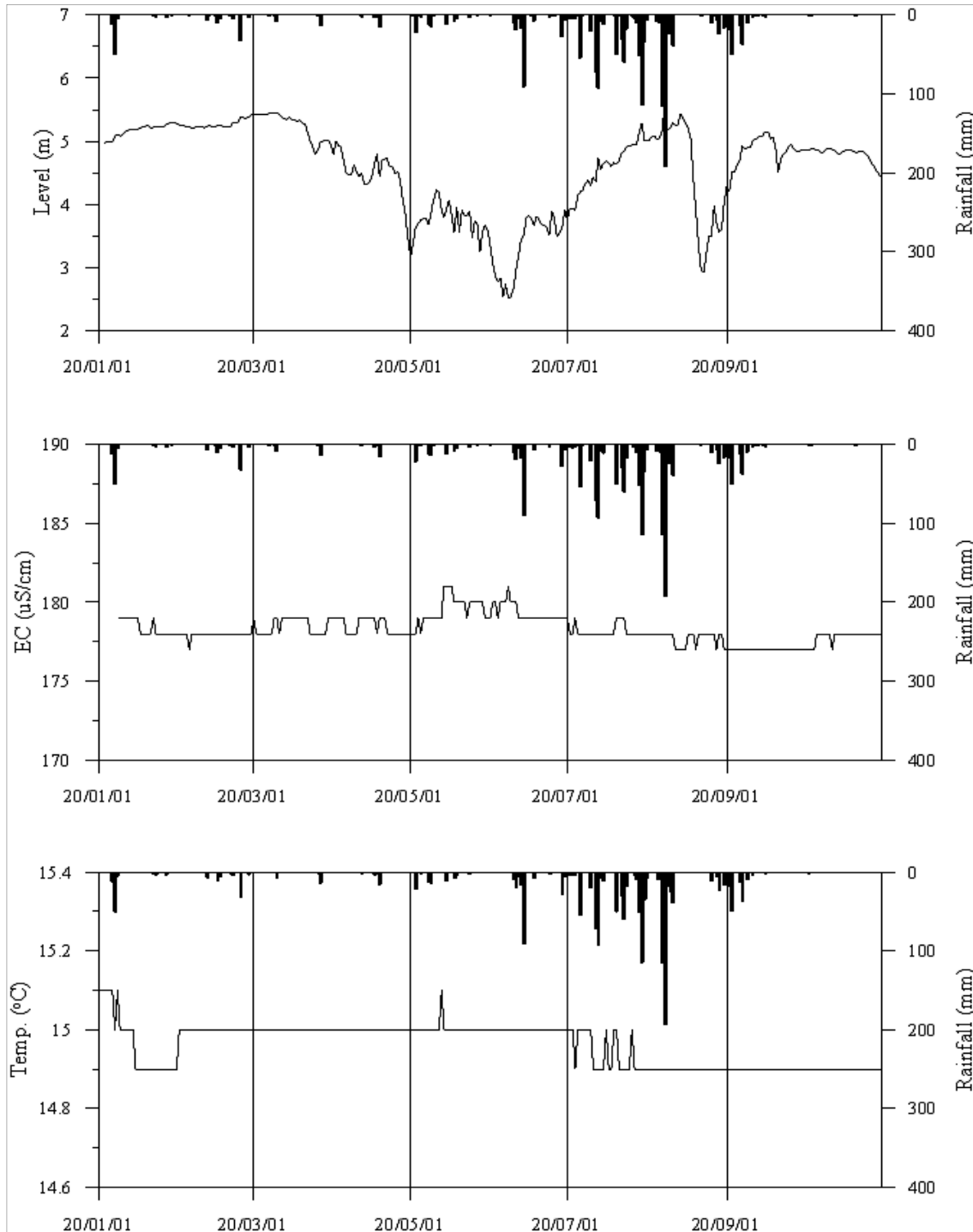
<김제2 관측공의 장기관측자료 (2020.1.1 ~ 2020.12.31)> (a)지하수위, (b)전기전도도, (c)수온
