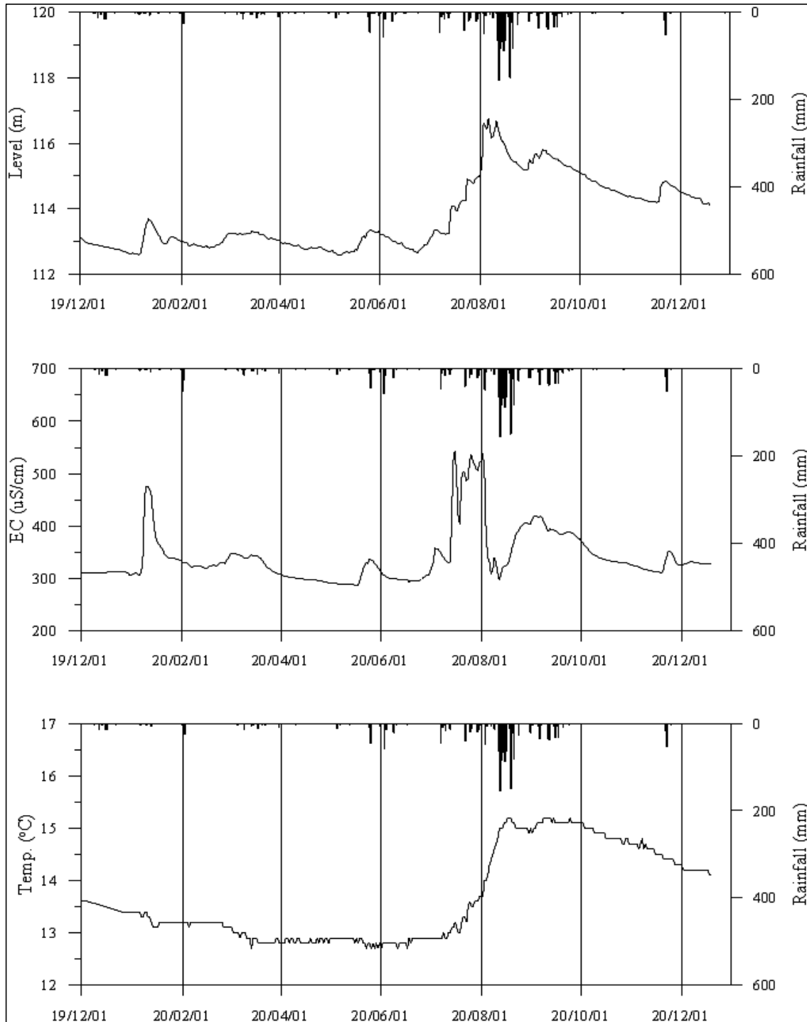
<포천7 관측공의 장기관측자료 (2019.12.1 ~ 2020.12.31)> (a)지하수위, (b)전기전도도, (c)수온
