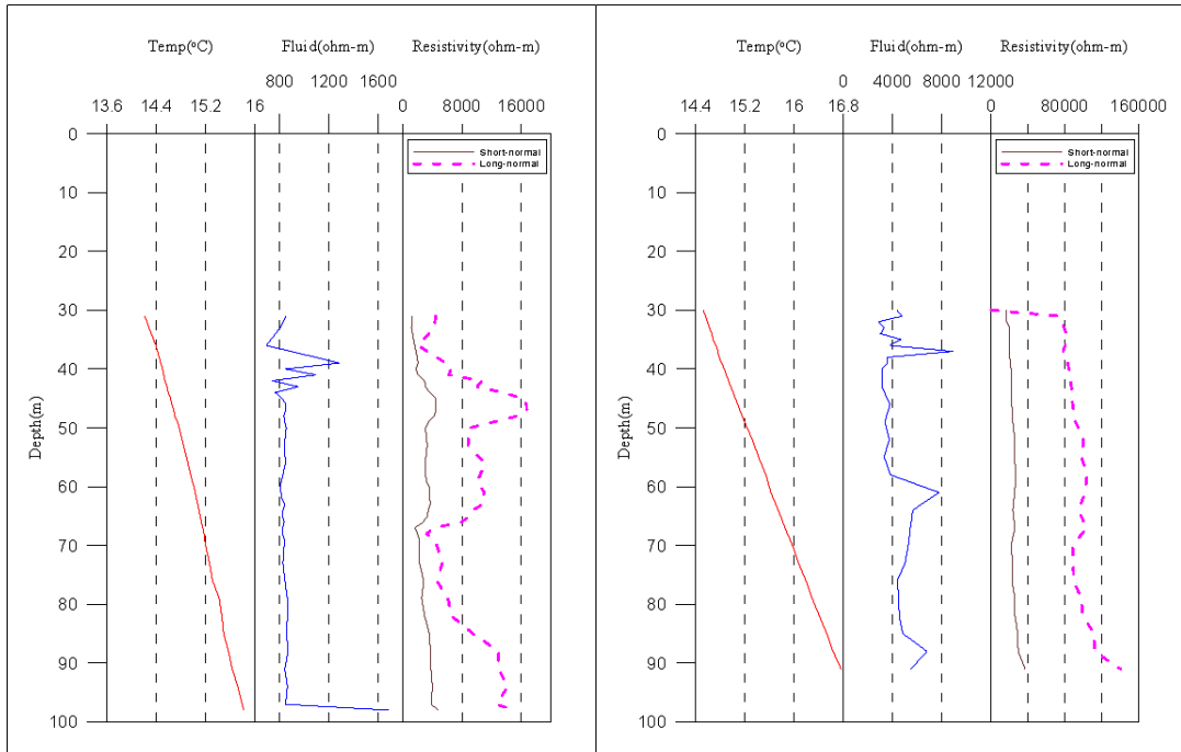
<이천5 관측공 물리검층>
