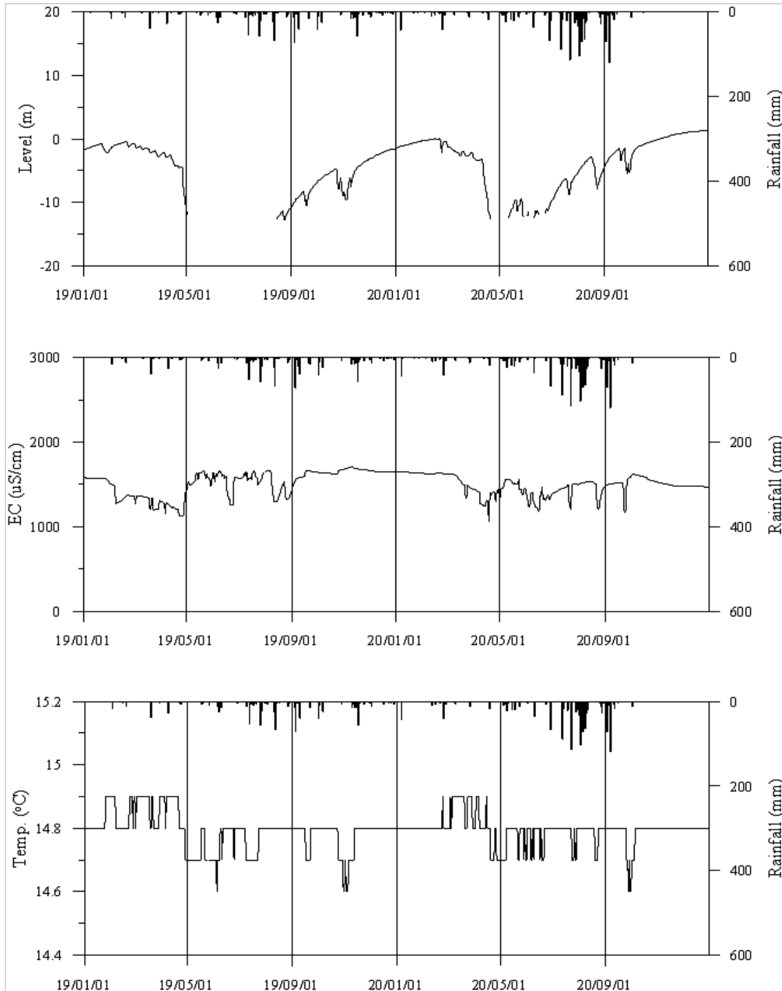
<태안4 관측공의 장기관측자료 (2019.1.1 ~ 2020.12.31)> (a)지하수위, (b)전기전도도, (c)수온
