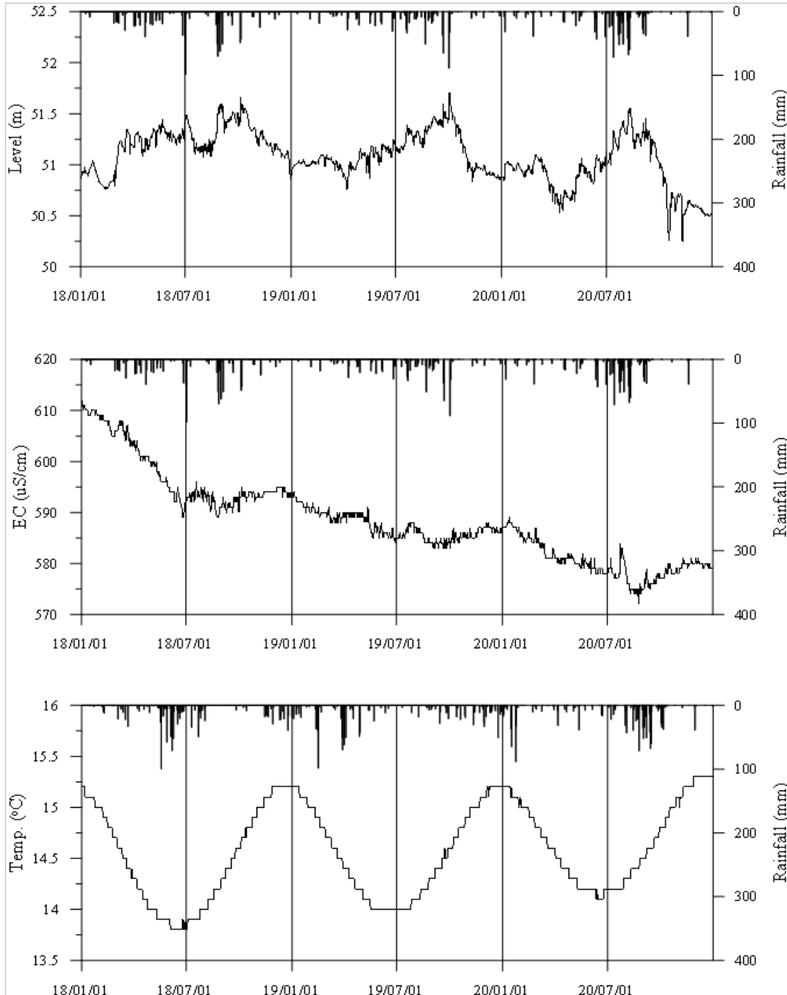
<의성1 관측공의 장기관측자료 (2018.1.1 ~ 2020.12.31.)> (a)지하수위, (b)전기전도도, (c)수온
