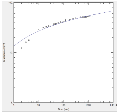
<경남고성1 관측공 양수시험>
