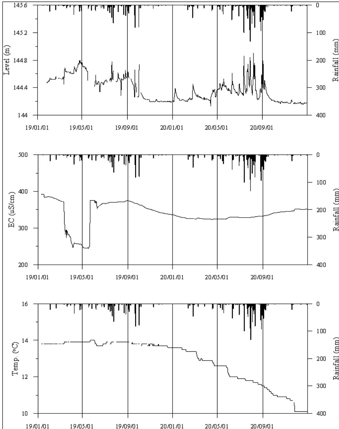
<보은3 관측공의 장기관측자료 (2019.1.1 ~ 2020.12.31)> (a)지하수위, (b)전기전도도, (c)수온
