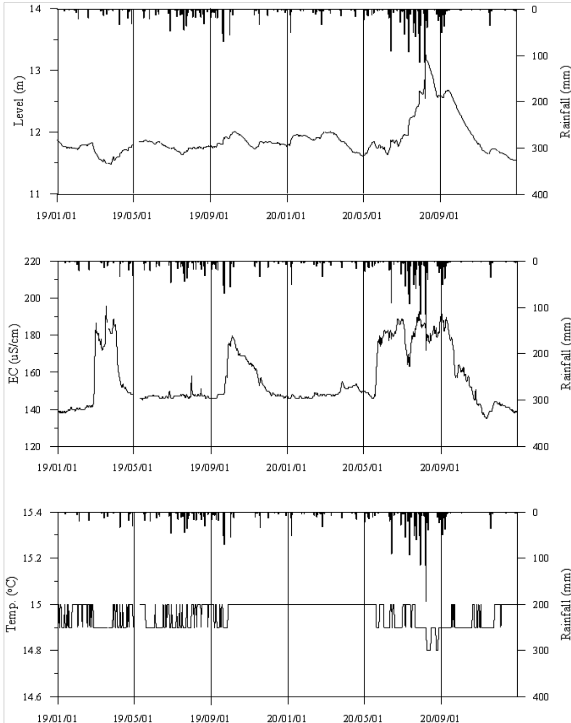
<익산4 관측공의 장기관측자료 (2019.1.1 ~ 2020.12.31)> (a)지하수위, (b)전기전도도, (c)수온
