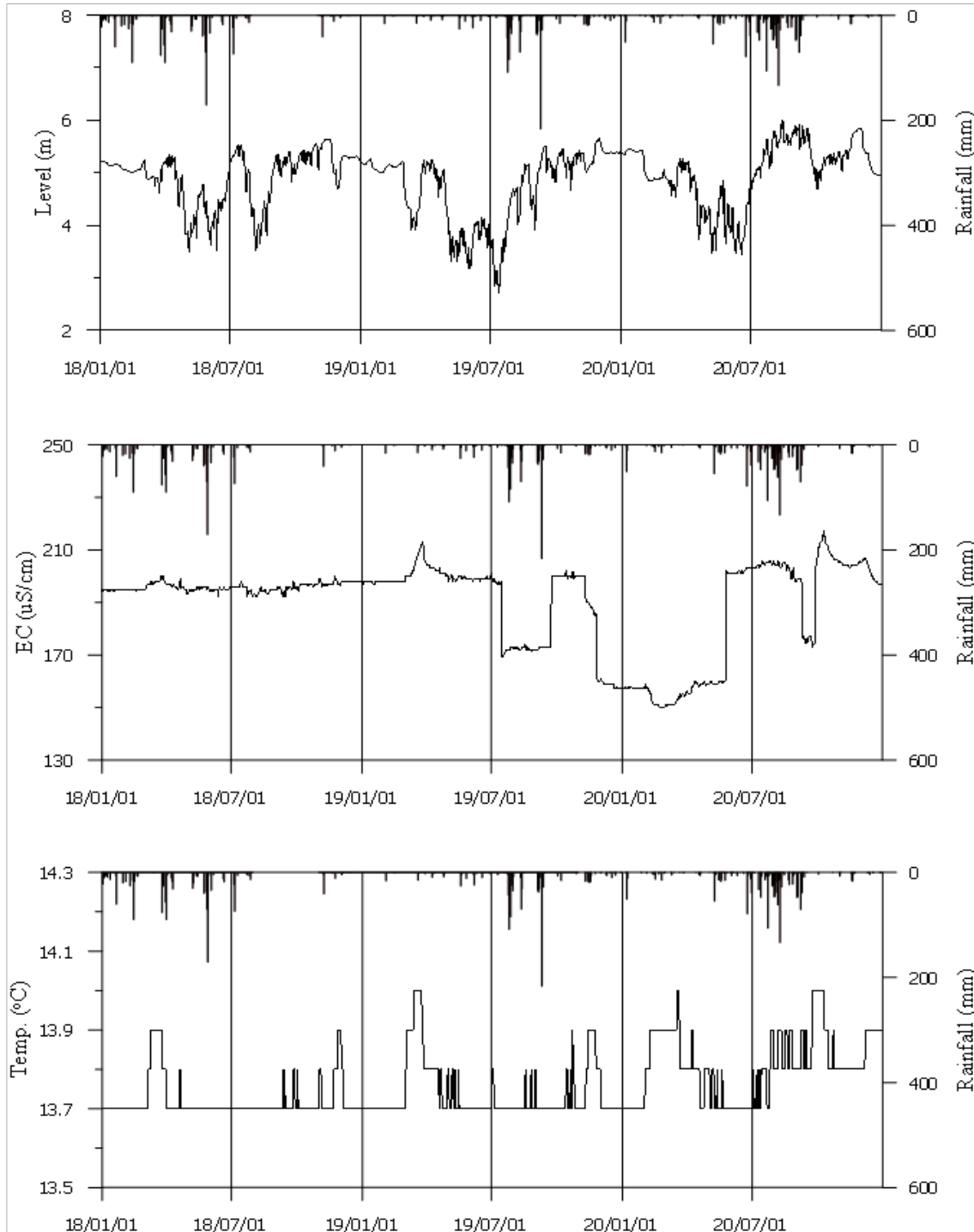
<강화1 관측공의 장기관측자료 (2008.1.1 ~ 2020.12.31)> (a)지하수위, (b)전기전도도, (c)수온
