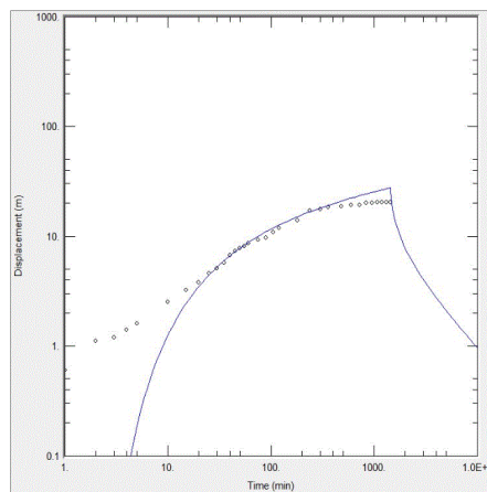
<울진3 관측공 양수시험>
