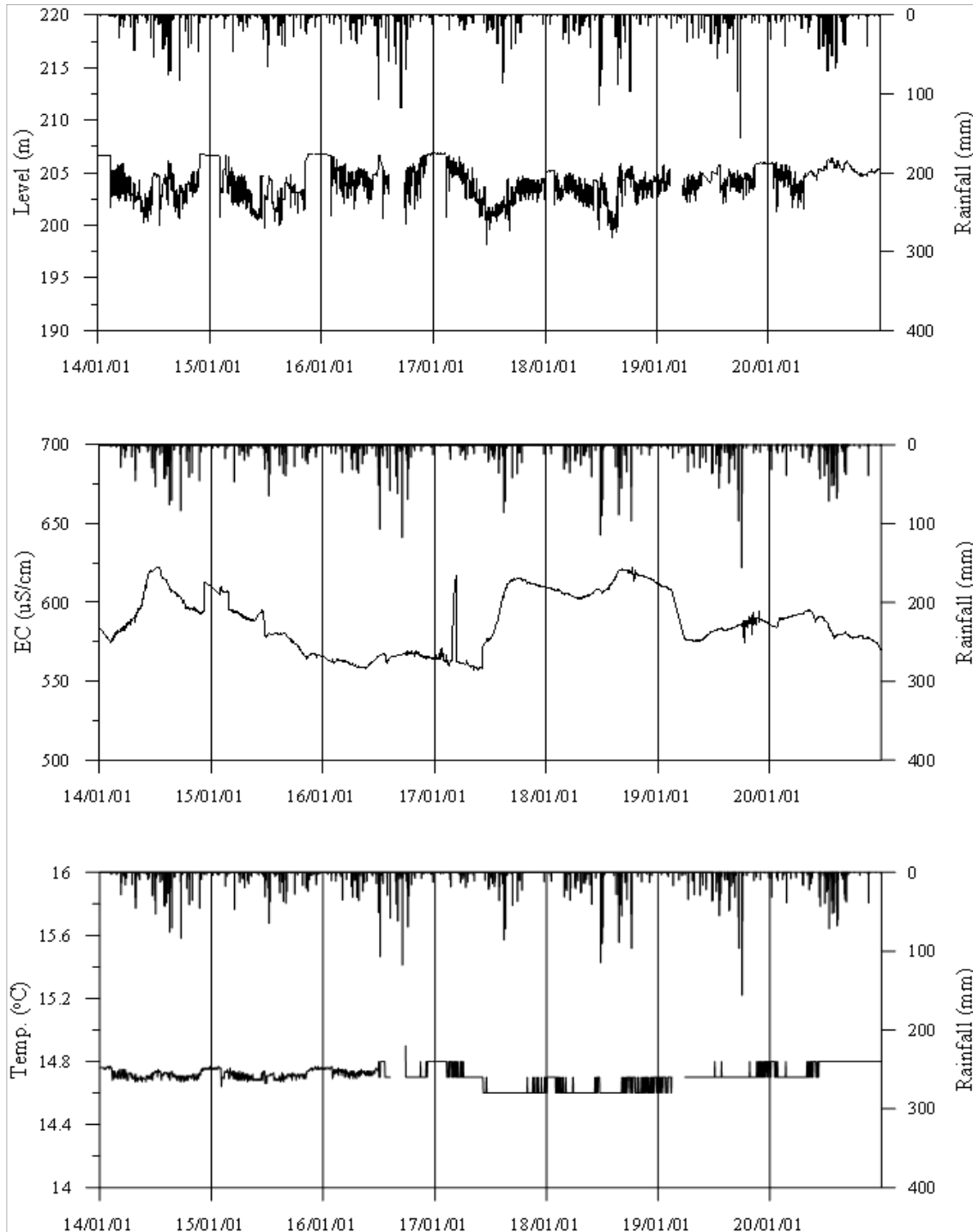
<군위2 관측공의 장기관측자료 (2014.1.1 ~ 2020.12.31)> (a)지하수위, (b)전기전도도, (c)수온
