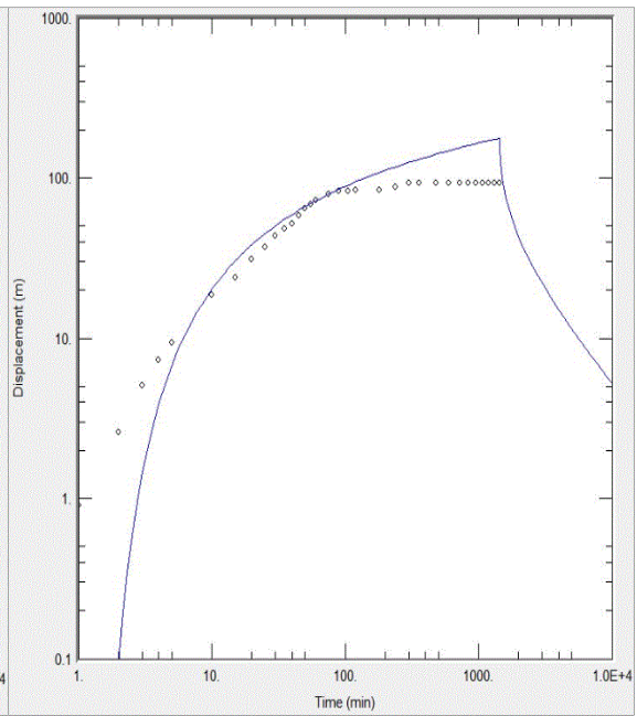
<영양4 관측공 양수시험>
