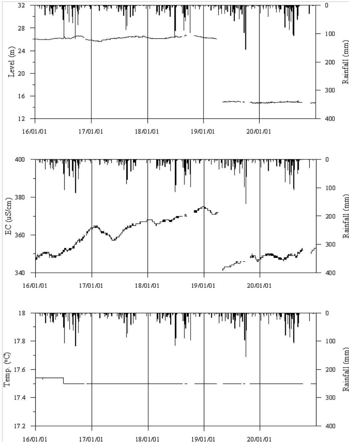
<구미3 관측공의 장기관측자료 (2016.1.1 ~ 2020.12.31)> (a)지하수위, (b)전기전도도, (c)수온
