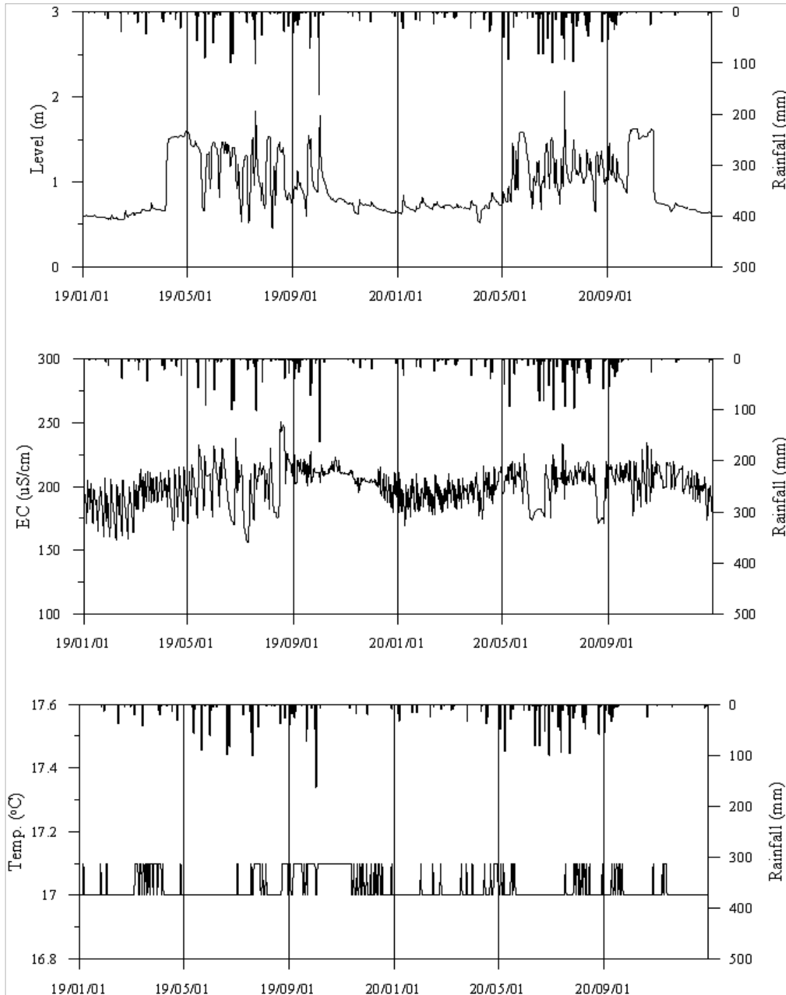
<보성6 관측공의 장기관측자료 (2019.1.1 ~ 2020.12.31)> (a)지하수위, (b)전기전도도, (c)수온
