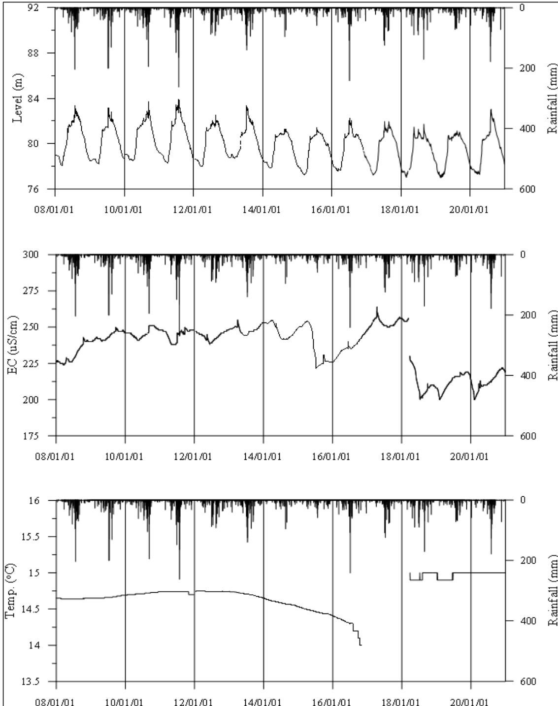
<춘천1 관측공의 장기관측자료 (2008.1.1 ~ 2020.12.31)> (a)지하수위, (b)전기전도도, (c)수온
