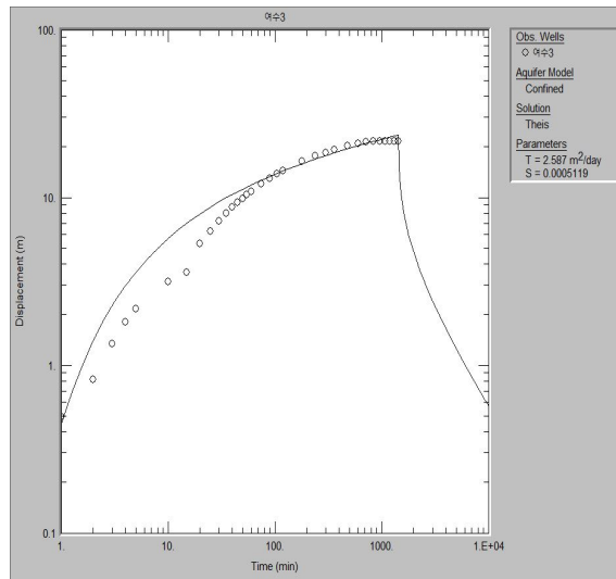
<여수3 관측공 양수시험>
