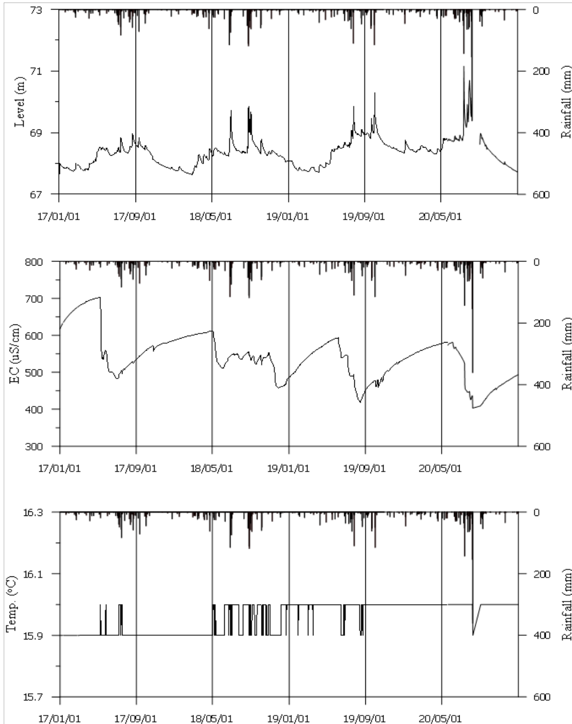
<순창2 관측공의 장기관측자료 (2017.1.1 ~ 2020.12.31)> (a)지하수위, (b)전기전도도, (c)수온
