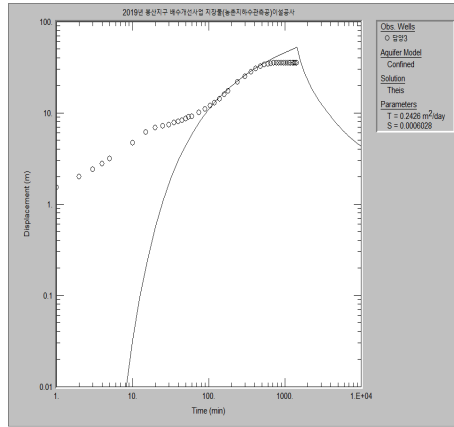
<담양3(신) 관측공 양수시험>
