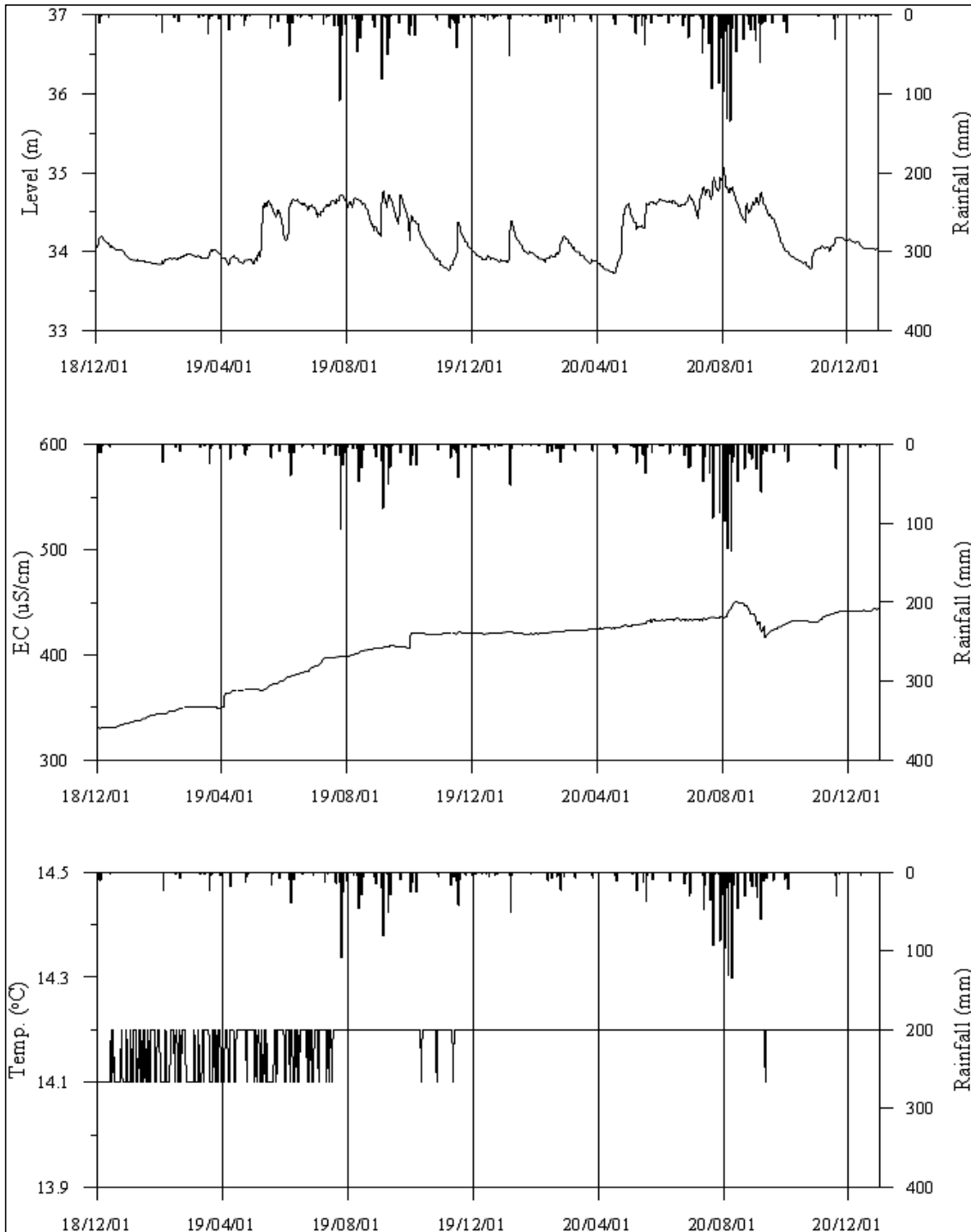
<안성6 관측공의 장기관측자료 (2018.12.1 ~ 2020.12.31)> (a)지하수위, (b)전기전도도, (c)수온
