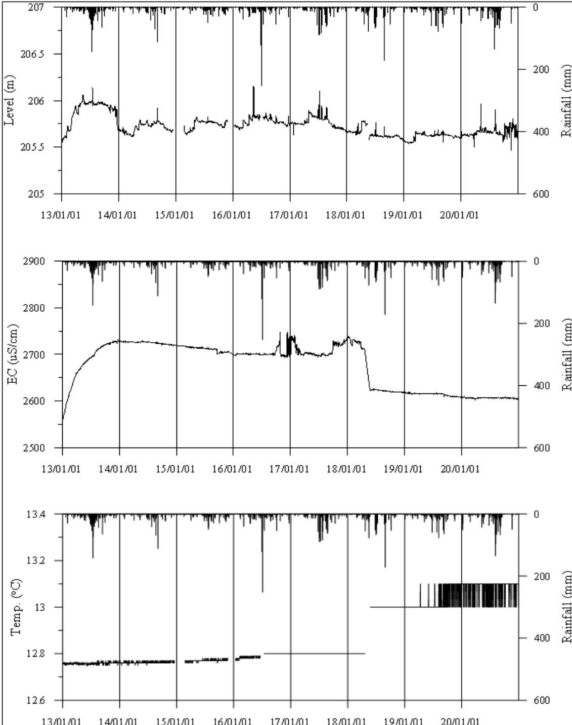
<인제1 관측공의 장기관측자료 (2013.1.1 ~ 2020.12.31)> (a)지하수위, (b)전기전도도, (c)수온
