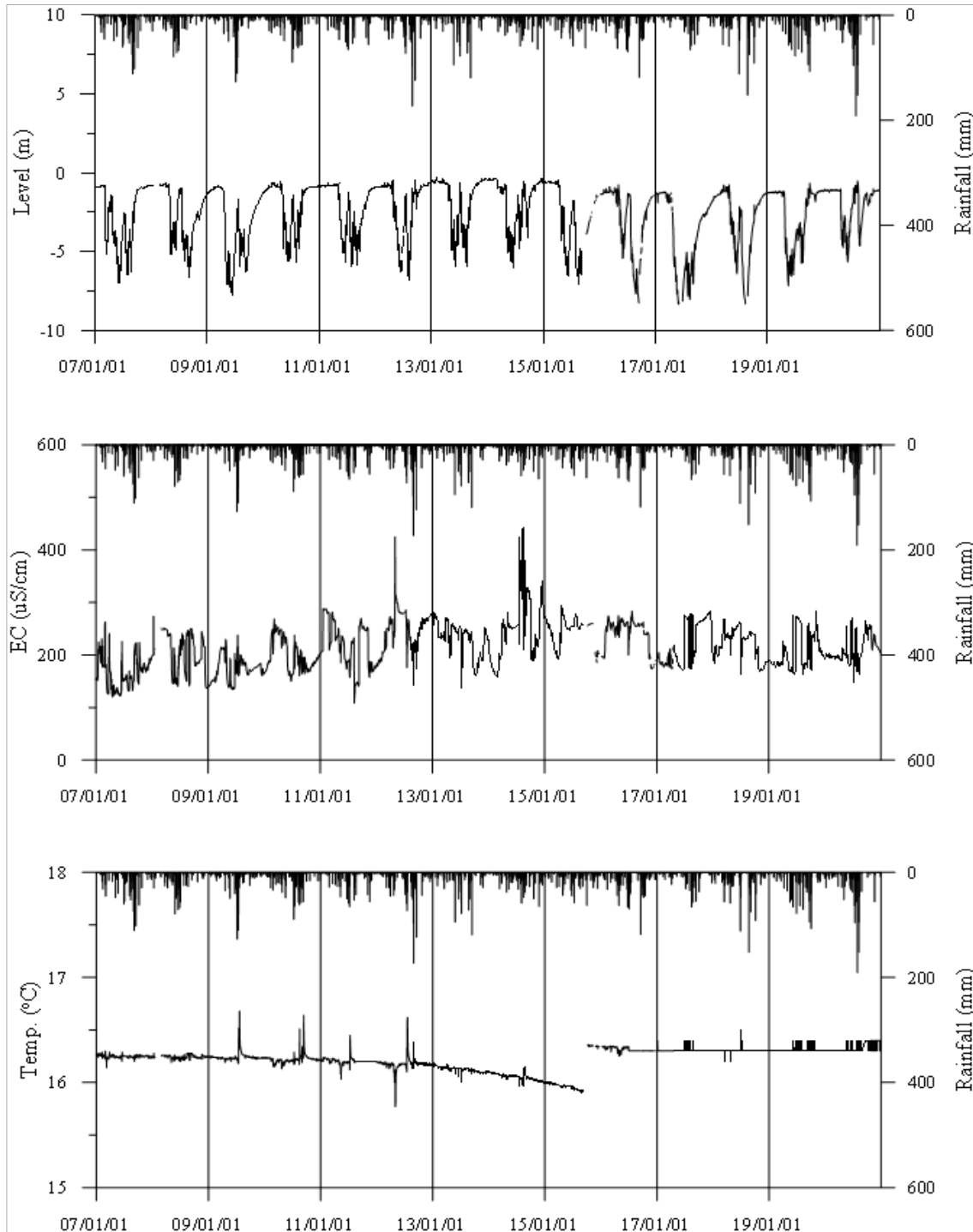
<무안3 관측공의 장기관측자료 (2007.1.1 ~ 2020.12.31)> (a)지하수위, (b)전기전도도, (c)수온
