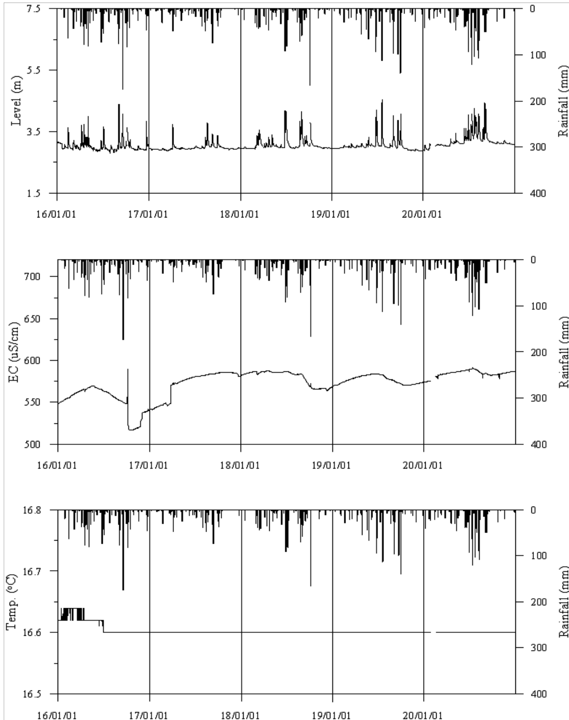
<사천2 관측공의 장기관측자료 (2016.1.1 ~ 2020.12.31)> (a)지하수위, (b)전기전도도, (c)수온
