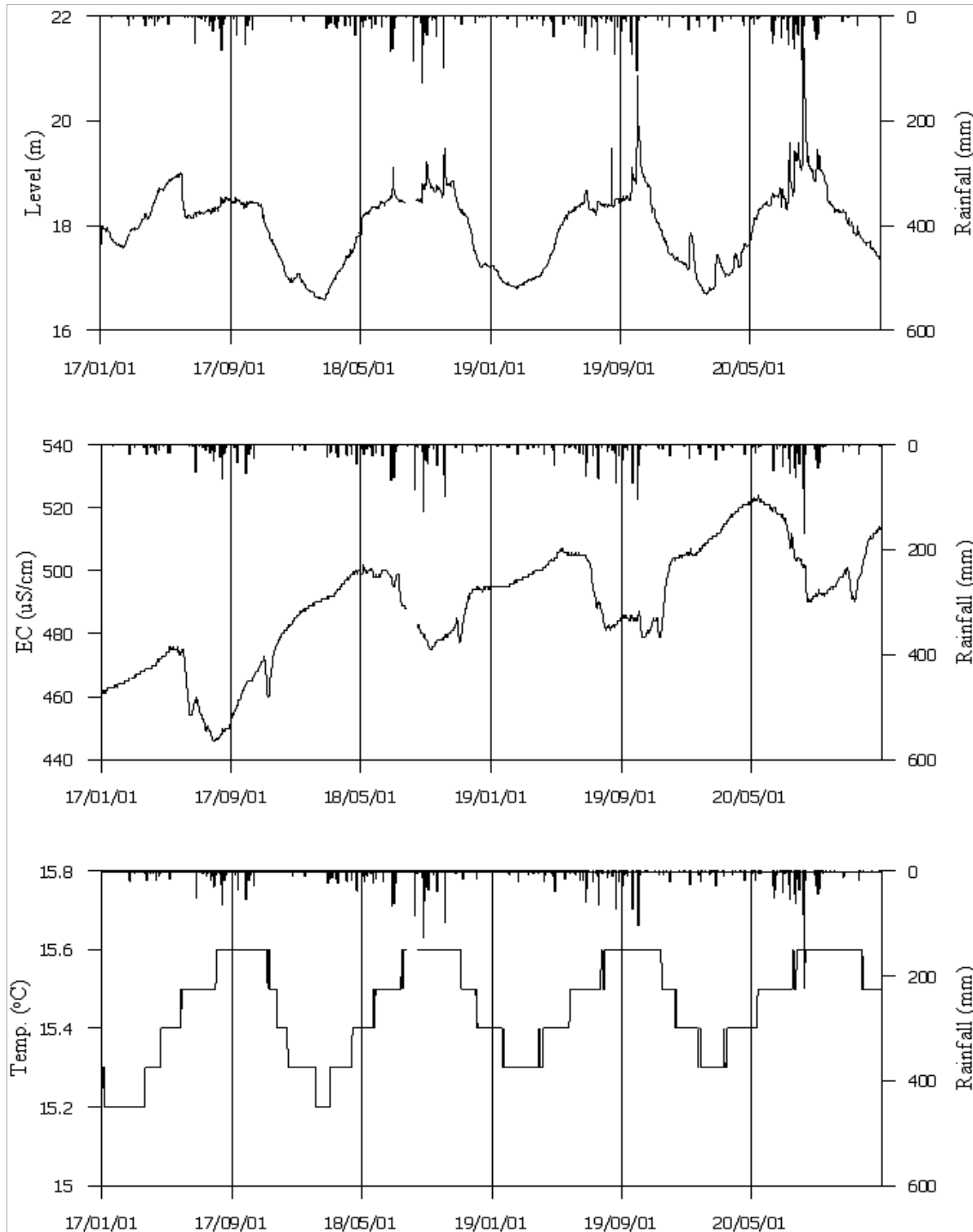
<칠곡2 관측공의 장기관측자료 (2017.1.1 ~ 2020.12.31.)> (a)지하수위, (b)전기전도도, (c)수온
