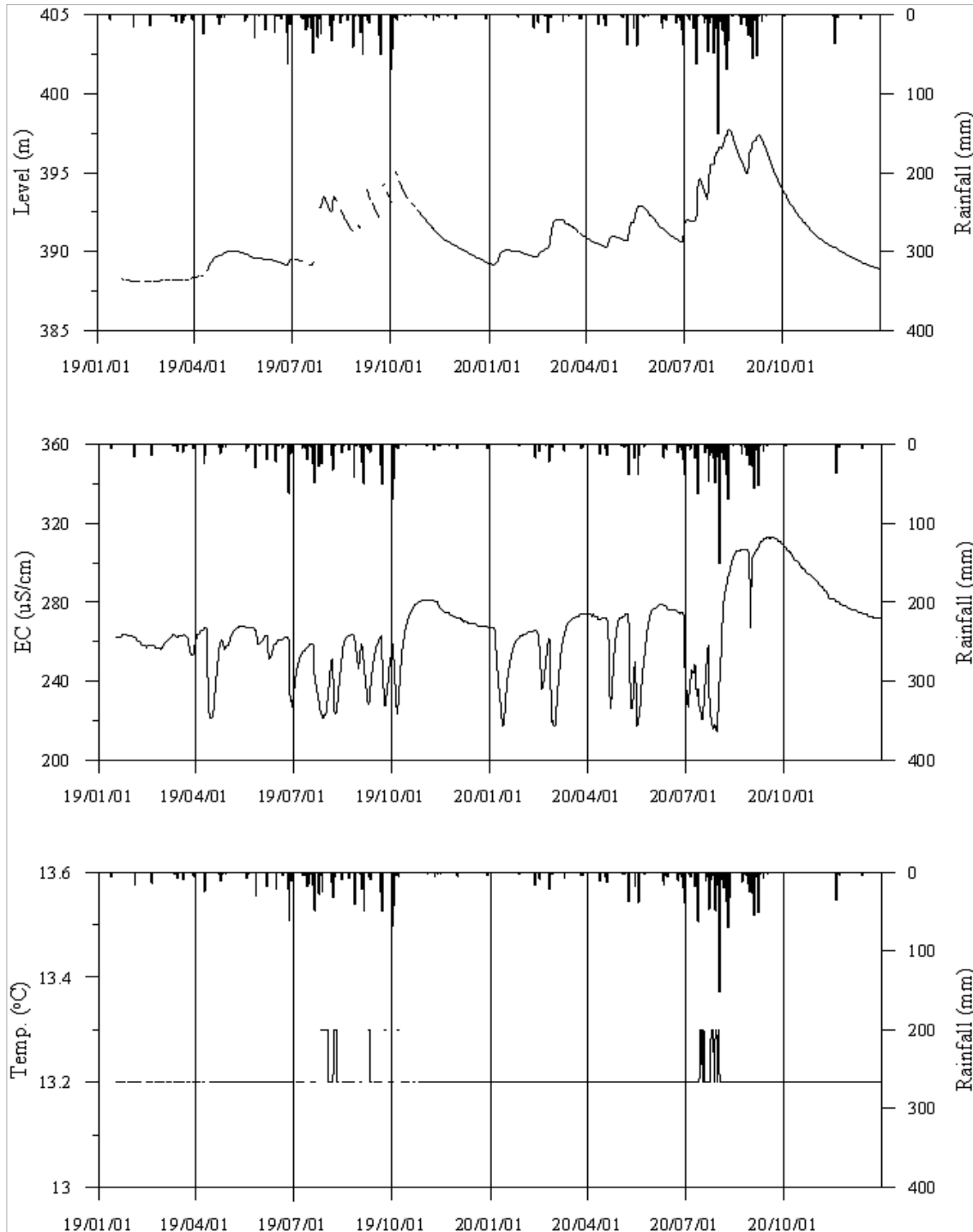
<봉화6 관측공의 장기관측자료 (2019.1.1 ~ 2020.12.31)> (a)지하수위, (b)전기전도도, (c)수온
