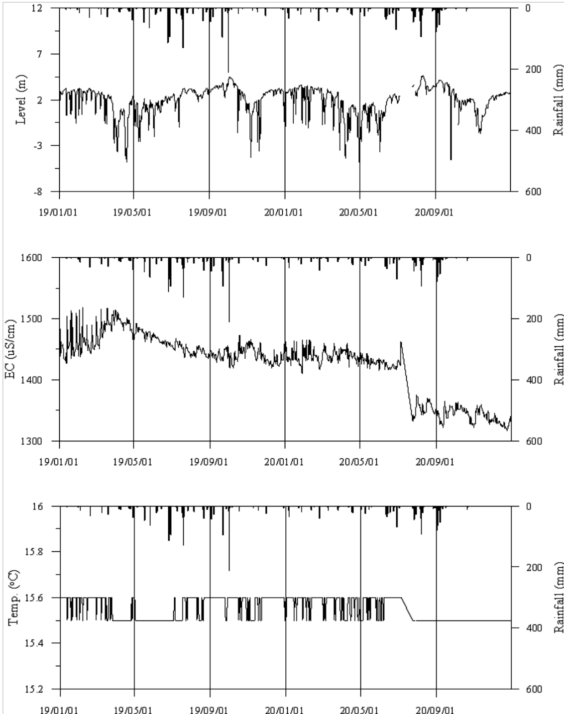
<함안1 관측공의 장기관측자료 (2019.1.1 ~ 2020.12.31)> (a)지하수위, (b)전기전도도, (c)수온
