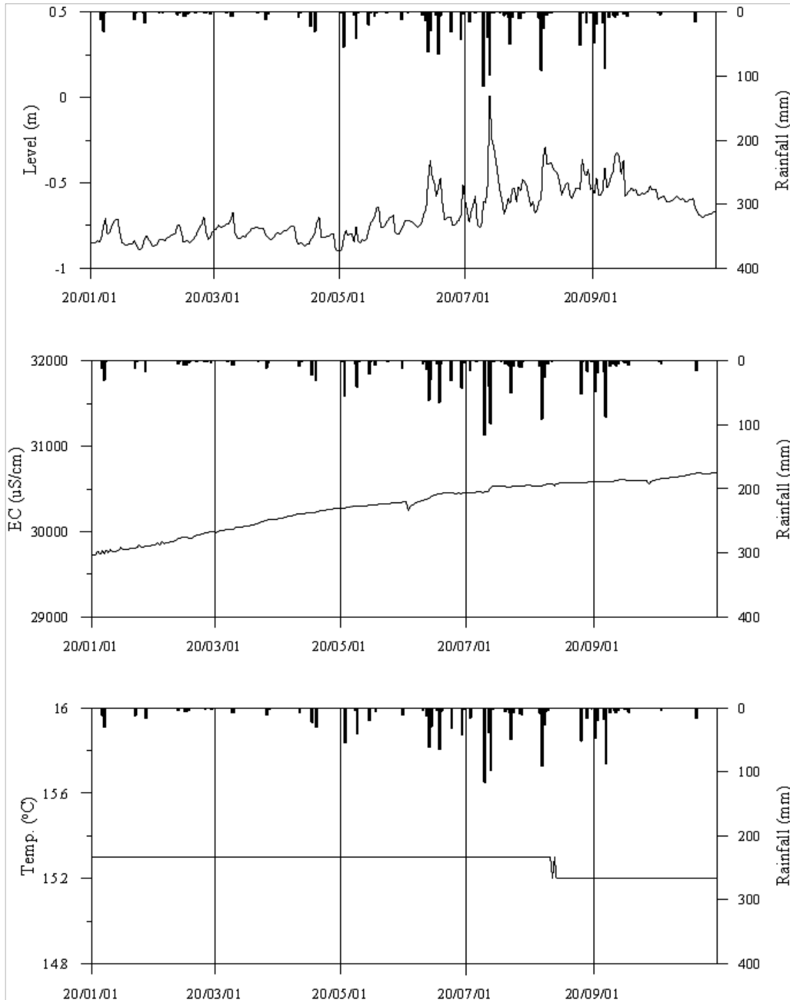
<영암3 관측공의 장기관측자료 (2020.1.1~2020.10.31)> (a)지하수위, (b)전기전도도, (c)수온
