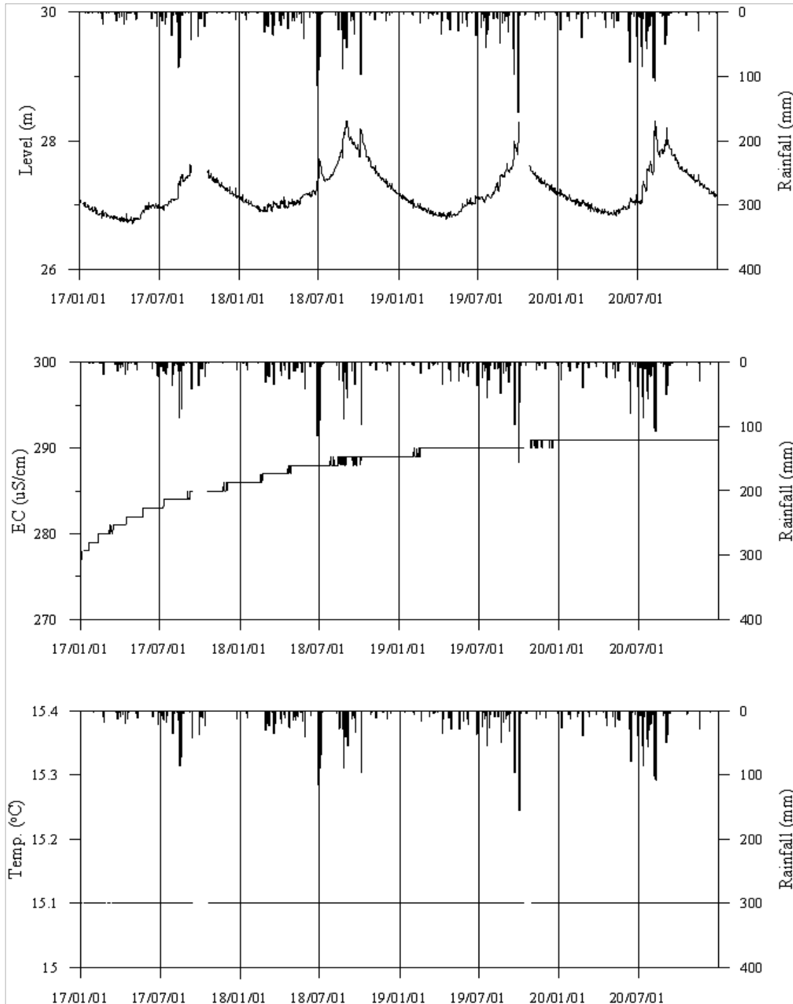
<구미6 관측공의 장기관측자료 (2016.1.1 ~ 2020.12.31)> (a)지하수위, (b)전기전도도, (c)수온
