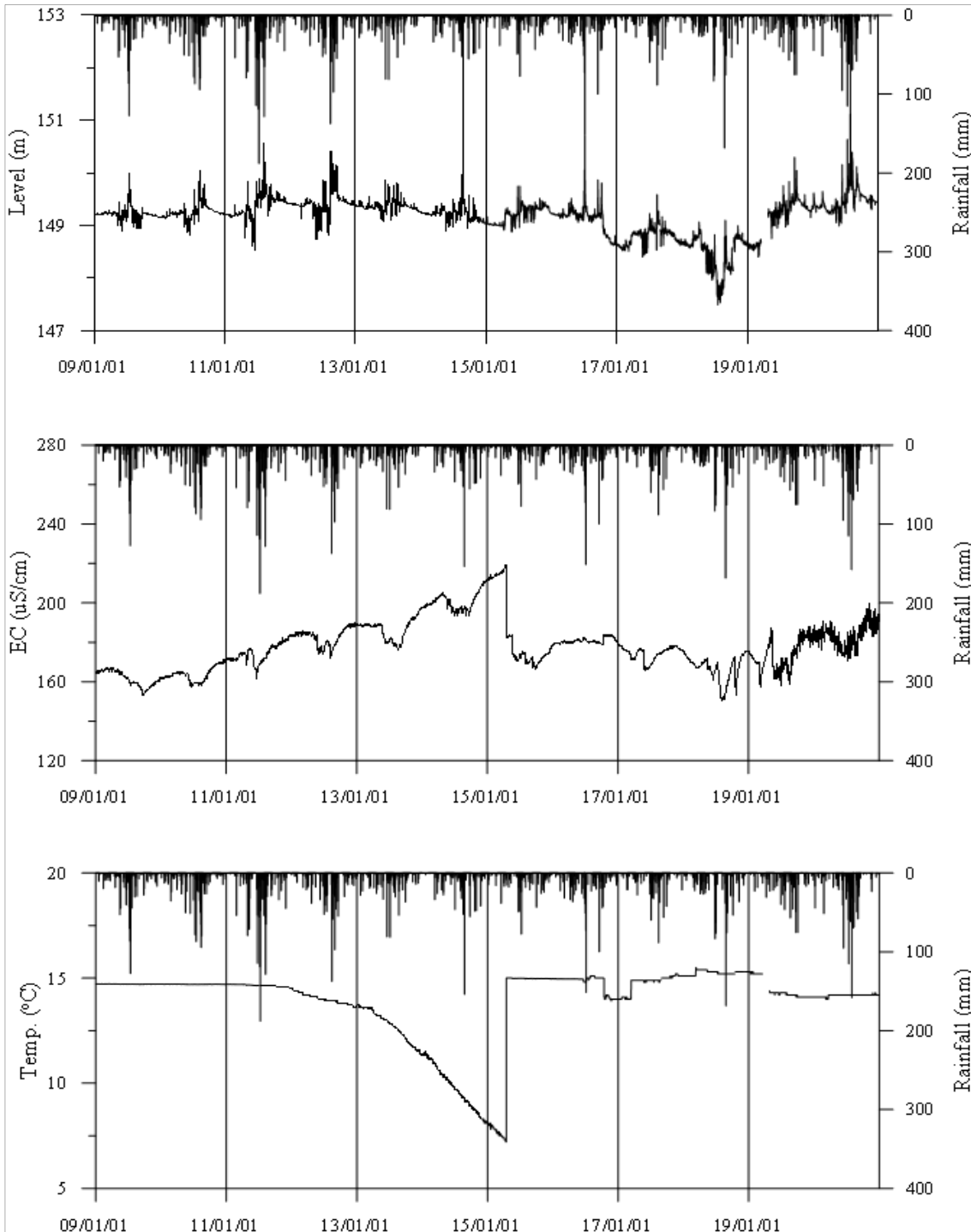
<금산1 관측공의 장기관측자료 (2009.1.1 ~ 2020.12.31)> (a)지하수위, (b)전기전도도, (c)수온
