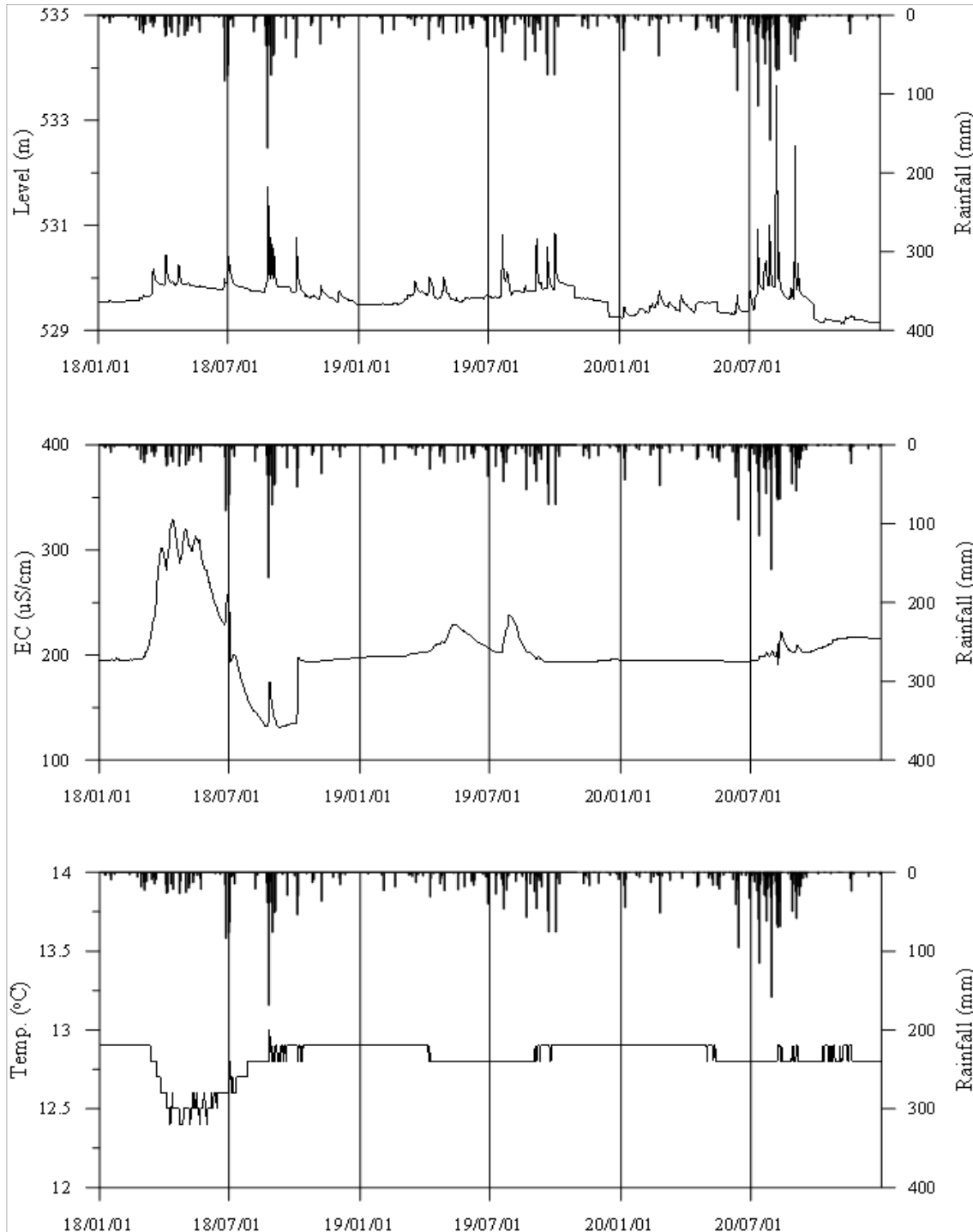
<무주2 관측공의 장기관측자료 (2018.1.1 ~ 2020.12.31)> (a)지하수위, (b)전기전도도, (c)수온
