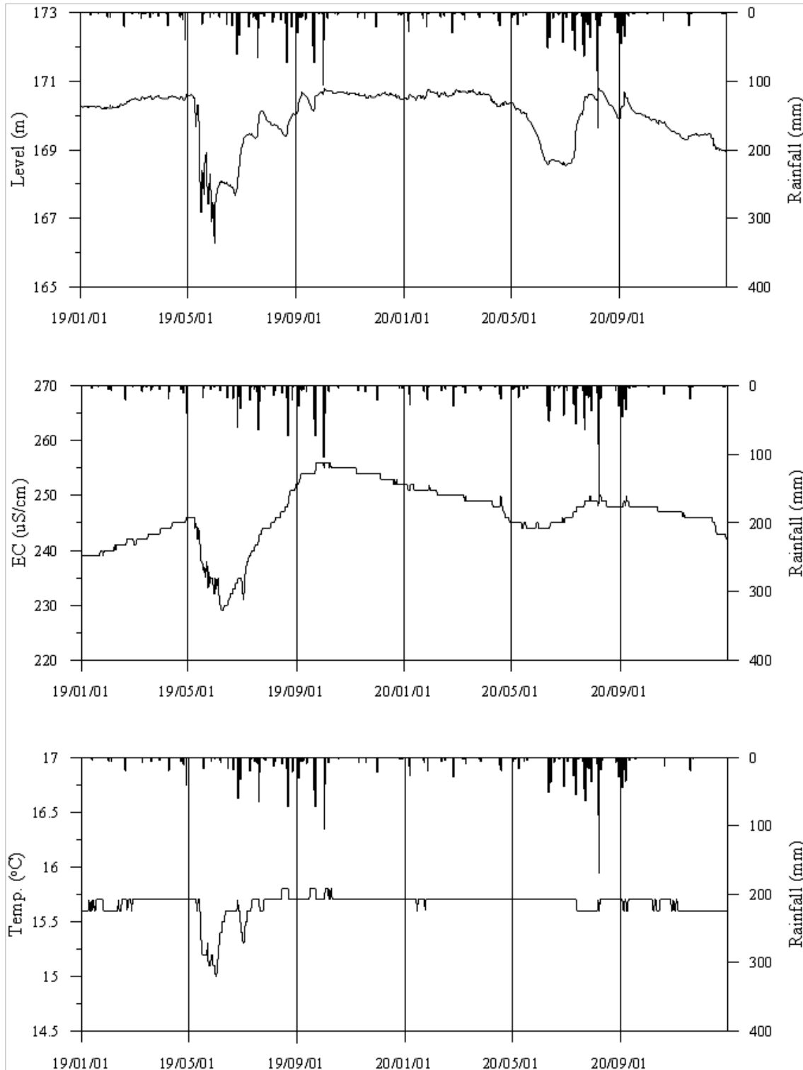
<청도4 관측공의 장기관측자료 (2019.1.1 ~ 2020.12.31)> (a)지하수위, (b)전기전도도, (c)수온
