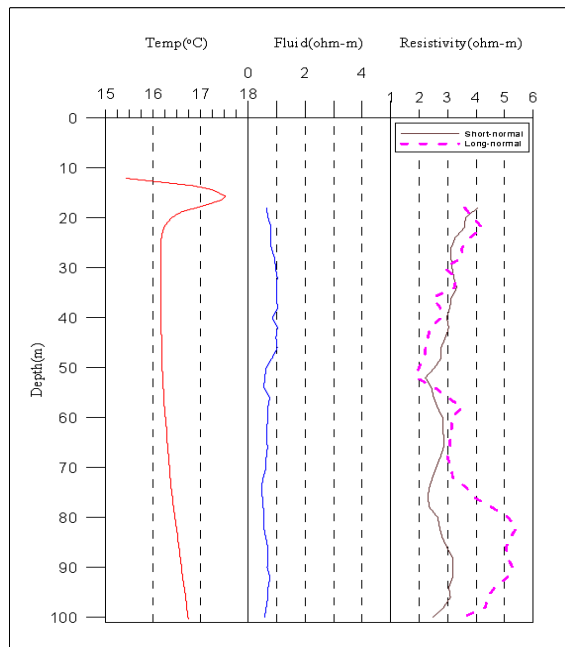
<사천6 관측공 물리검층>
