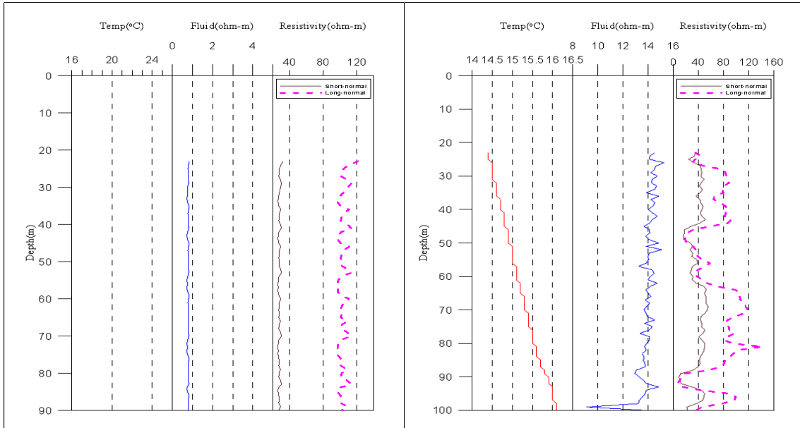
<김천4 관측공 물리검층>
