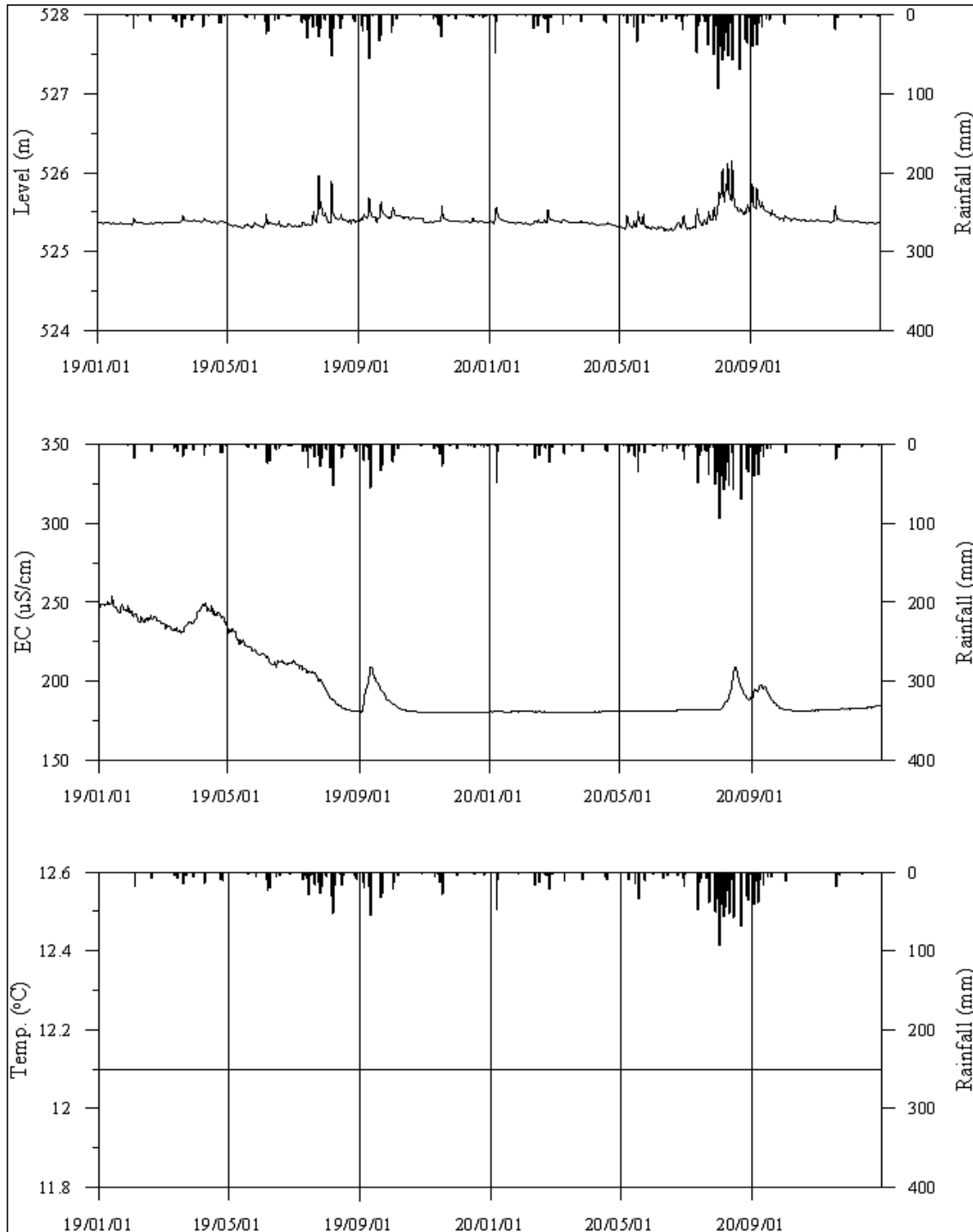
<횡성4 관측공의 장기관측자료 (2019.1.1 ~ 2020.12.31)> (a)지하수위, (b)전기전도도, (c)수온
