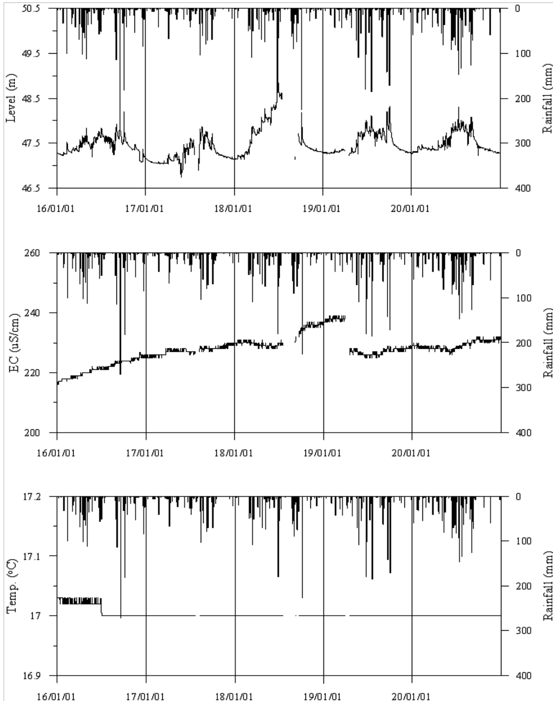
<남해2 관측공의 장기관측자료 (2016.1.1 ~ 2020.12.31)> (a)지하수위, (b)전기전도도, (c)수온
