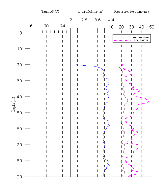
<칠곡4 관측공 물리검층>
