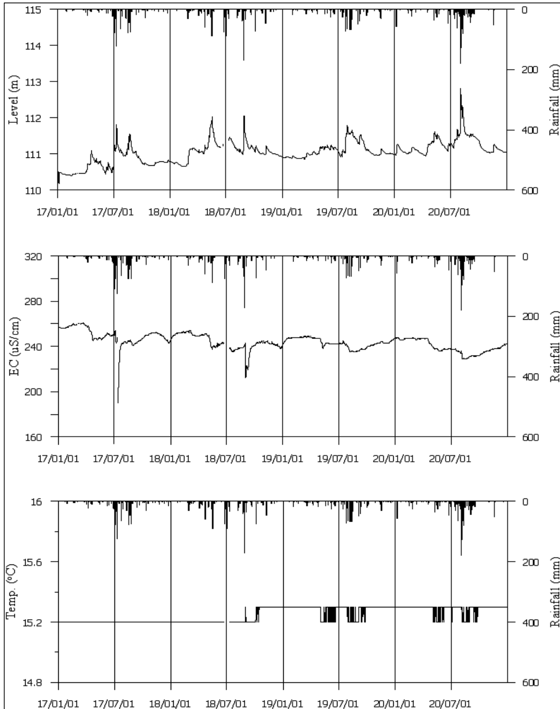
<가평3 관측공의 장기관측자료 (2017.1.1 ~ 2020.12.31)> (a)지하수위, (b)전기전도도, (c)수온
