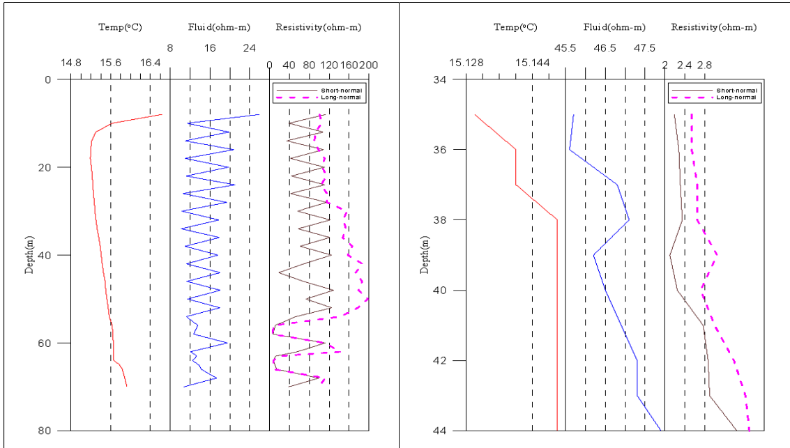
<장흥5 관측공 물리검층>
