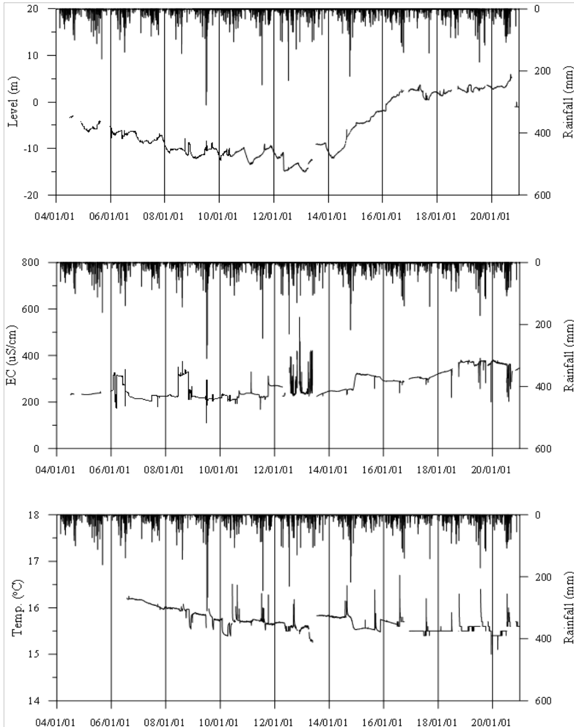
<김해2 관측공의 장기관측자료 (2004.1.1 ~ 2020.12.31)> (a)지하수위, (b)전기전도도, (c)수온
