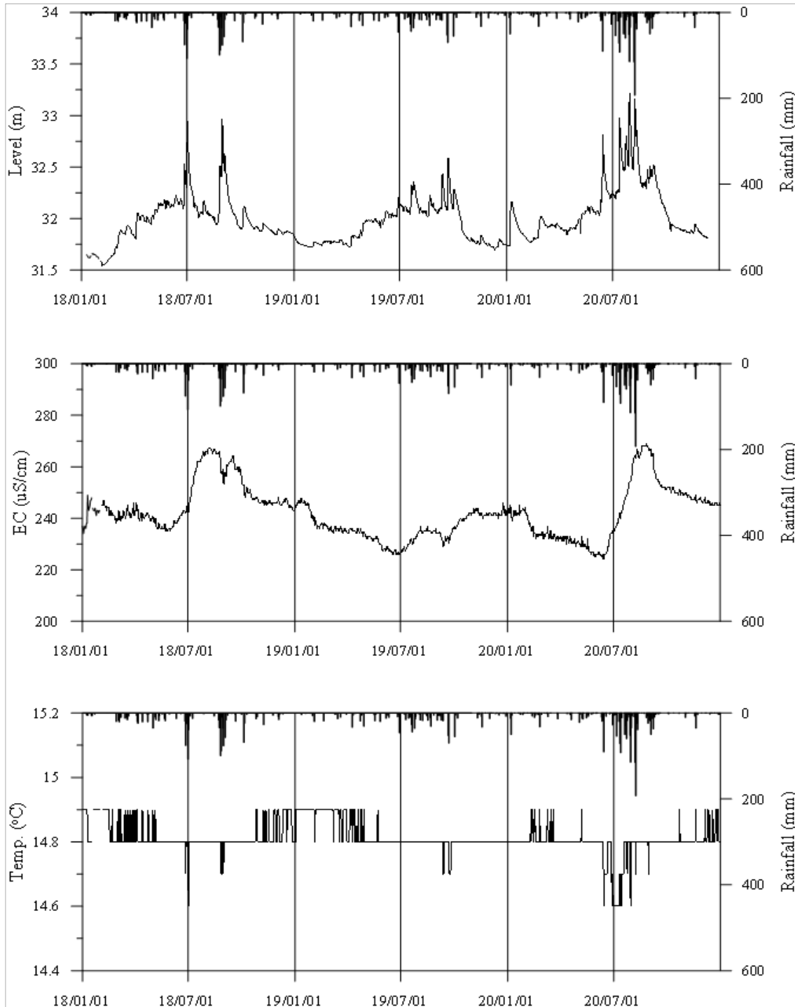
<완주3 관측공의 장기관측자료 (2018.1.1 ~ 2020.12.31)> (a)지하수위, (b)전기전도도, (c)수온
