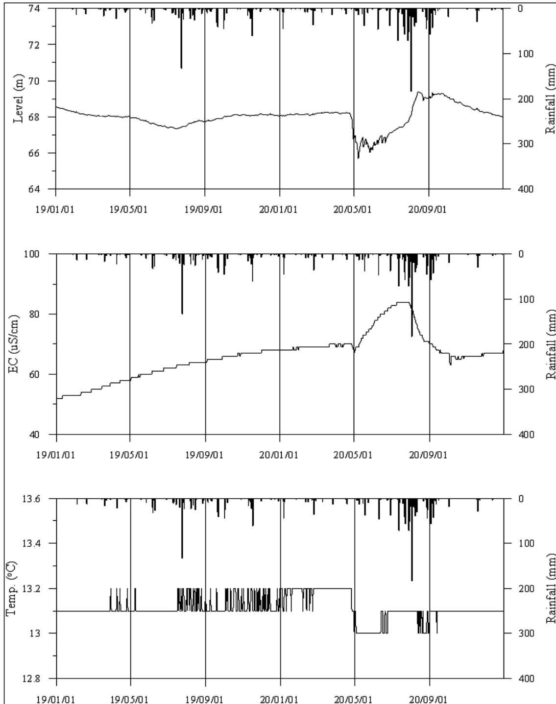
<진천4 관측공의 장기관측자료 (2019.1.1 ~ 2020.12.31)> (a)지하수위, (b)전기전도도, (c)수온
