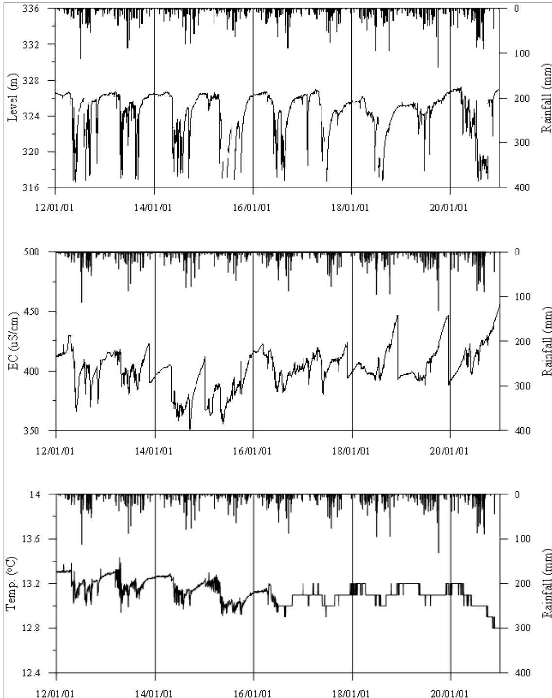
<청송2 관측공의 장기관측자료 (2012.1.1 ~ 2020.12.31)> (a)지하수위, (b)전기전도도, (c)수온
