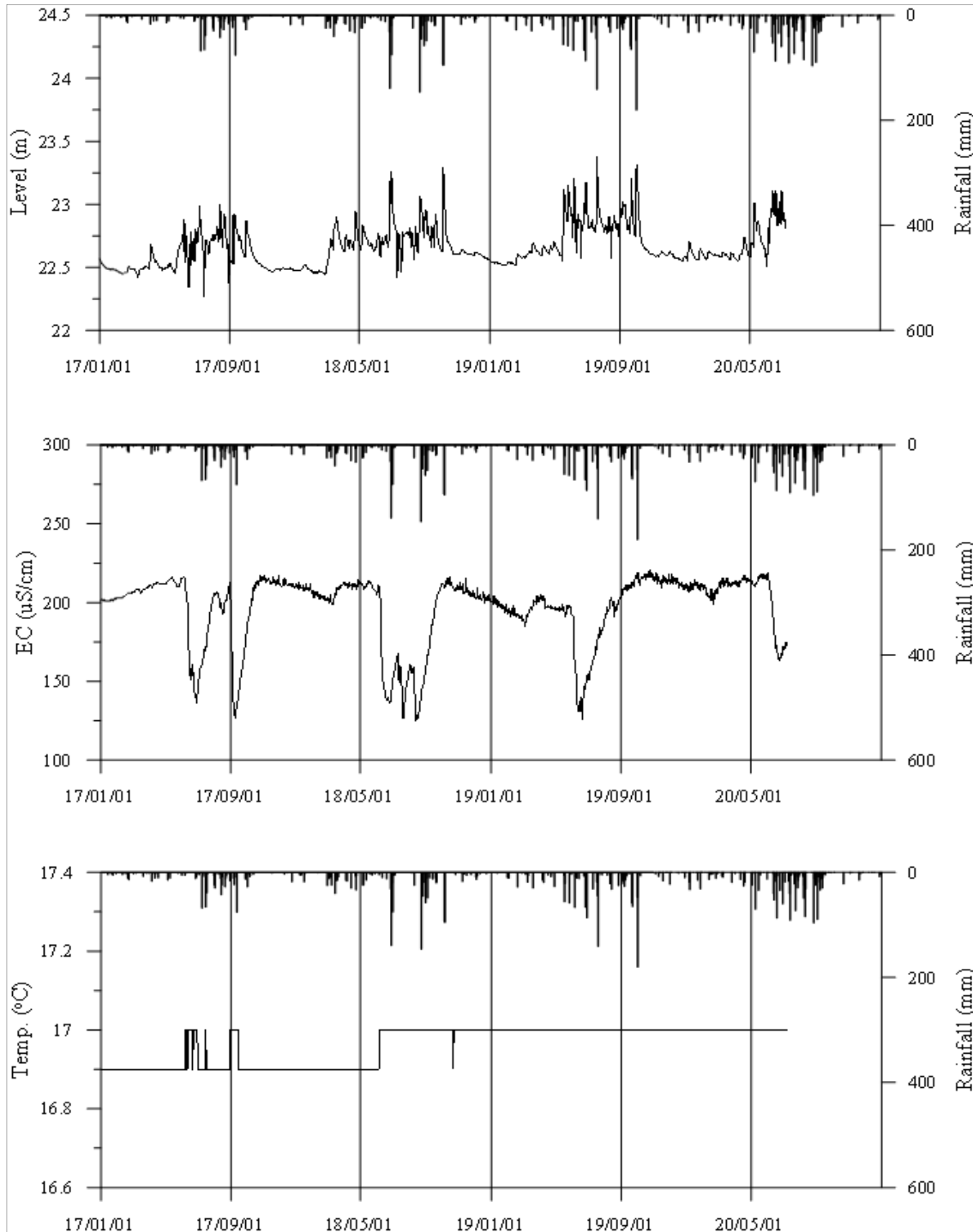
<장흥4 관측공의 장기관측자료 (2017.1.1 ~ 2020.12.31)> (a)지하수위, (b)전기전도도, (c)수온
