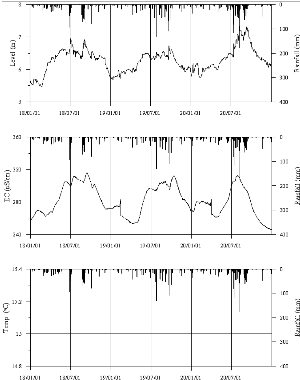
<정읍5 관측공의 장기관측자료 (2018.1.1 ~ 2020.12.31)> (a)지하수위, (b)전기전도도, (c)수온
