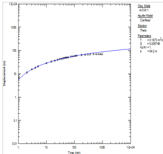
<기장3 관측공 양수시험>
