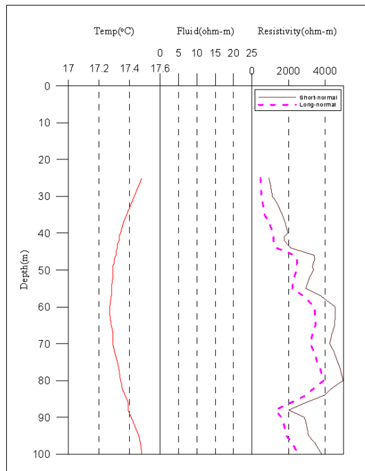
<여수3 관측공 물리검층>
