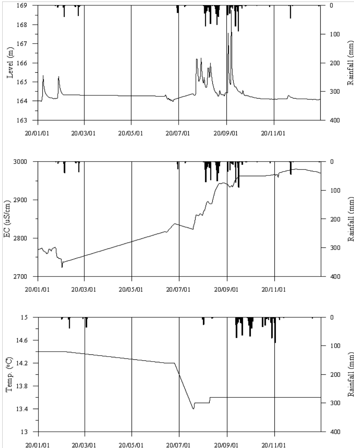
<영양3 관측공의 장기관측자료 (2020.1.1 ~ 2020.12.31.)> (a)지하수위, (b)전기전도도, (c)수온
