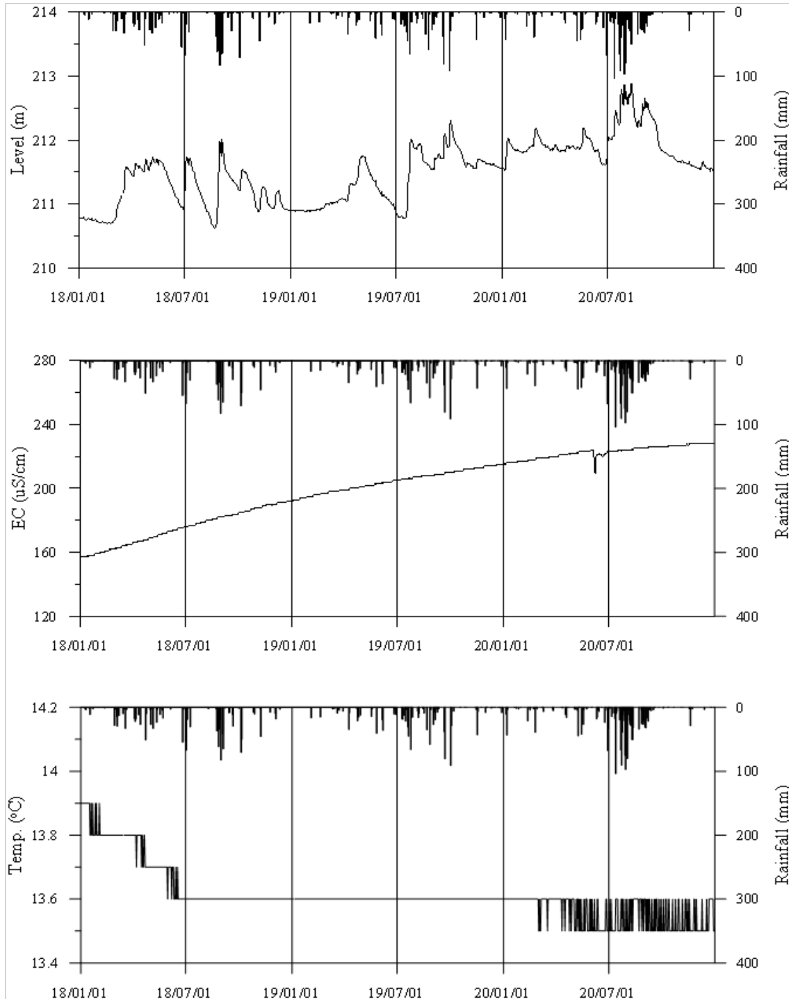
<문경5 관측공의 장기관측자료 (2018.1.1 ~ 2020.12.31.)> (a)지하수위, (b)전기전도도, (c)수온
