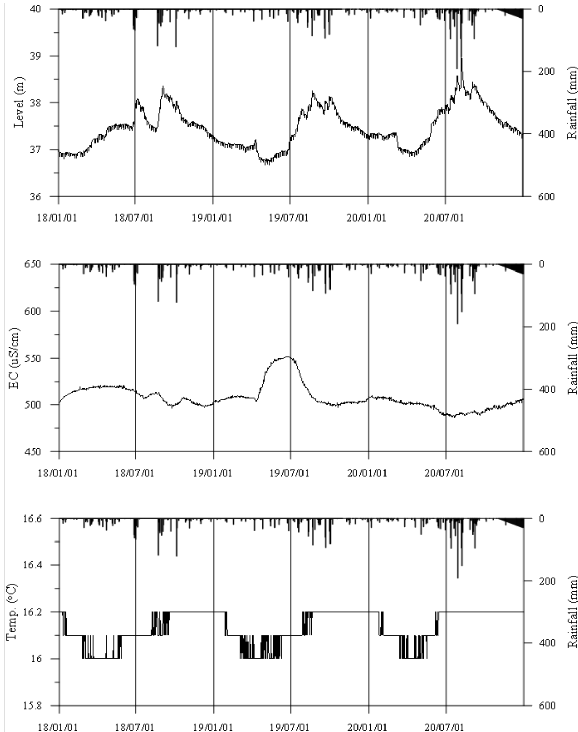
<장성3 관측공의 장기관측자료 (2018.1.1 ~ 2020.12.31)> (a)지하수위, (b)전기전도도, (c)수온
