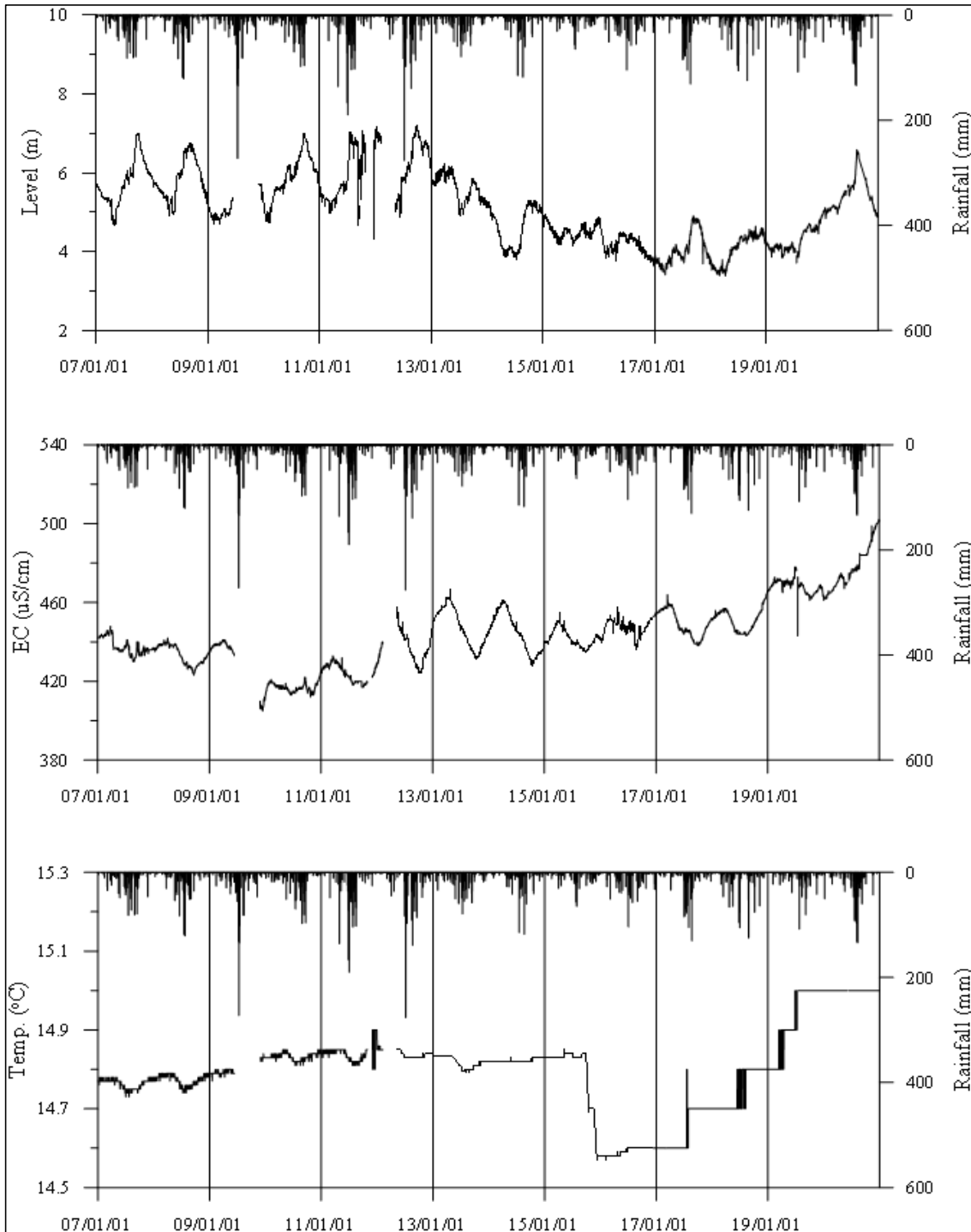
<평택2 관측공의 장기관측자료 (2007.1.1 ~ 2020.12.31)> (a)지하수위, (b)전기전도도, (c)수온
