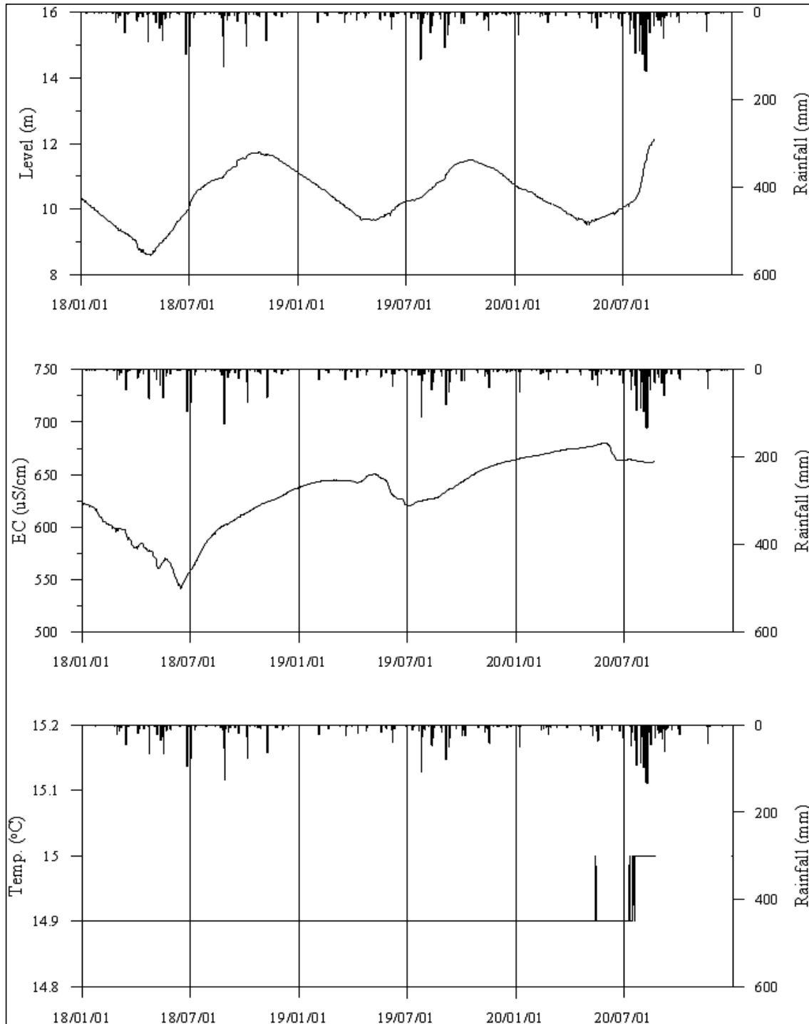
<평택5 관측공의 장기관측자료 (2018.1.1 ~ 2020.12.31)> (a)지하수위, (b)전기전도도, (c)수온
