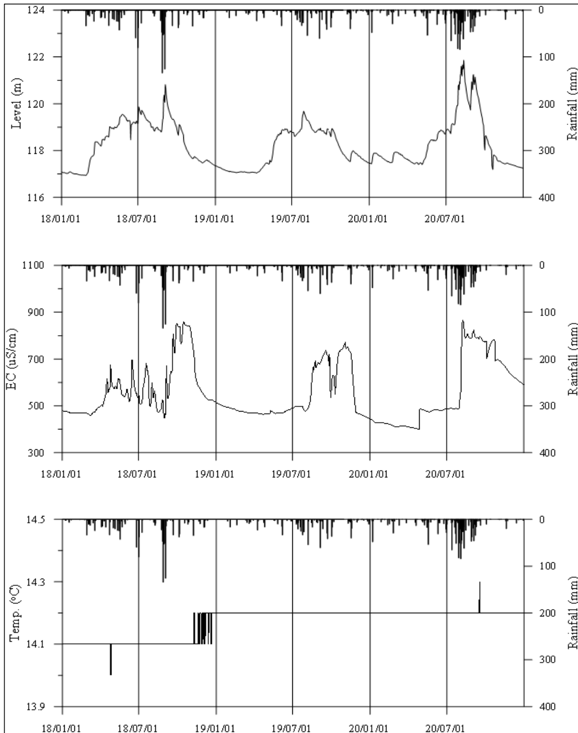
<괴산2 관측공의 장기관측자료 (2018.1.1 ~ 2020.12.31)> (a)지하수위, (b)전기전도도, (c)수온
