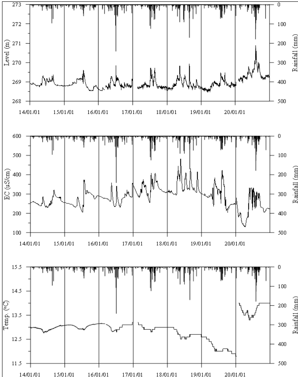
<화전2 관측공의 장기관측자료 (2014.1.1 ~ 2020.12.31)> (a)지하수위, (b)전기전도도, (c)수온
