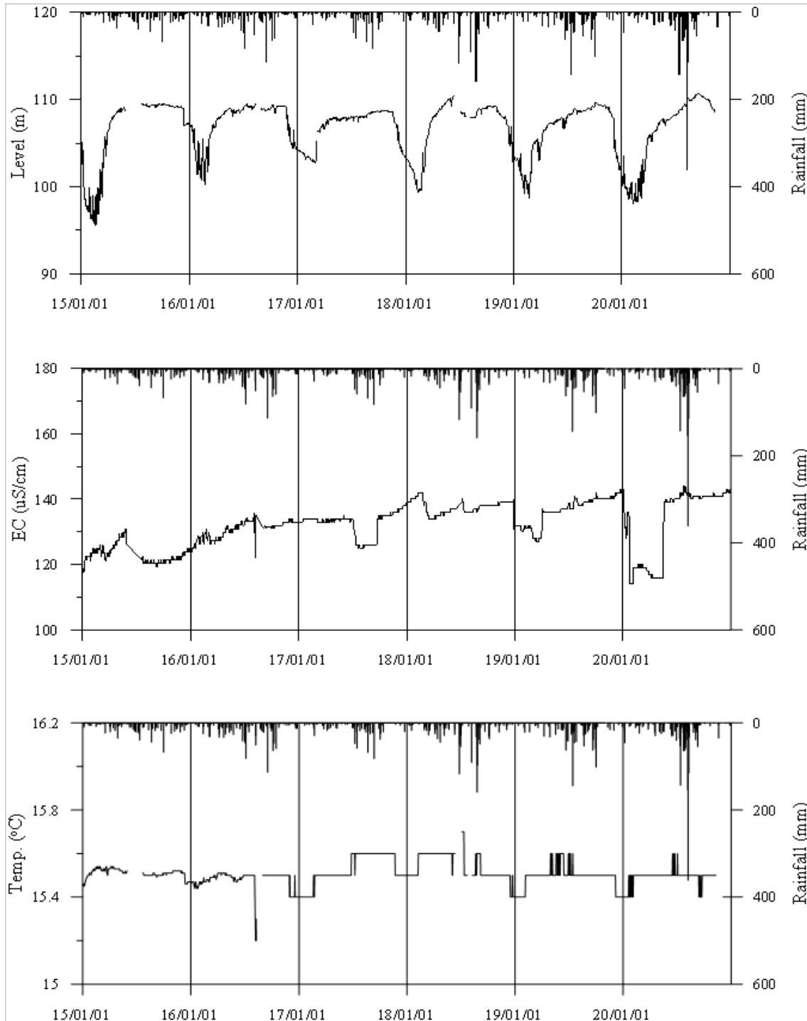
<곡성3 관측공의 장기관측자료 (2015.1.1~2020.12.31)> (a)지하수위, (b)전기전도도, (c)수온
