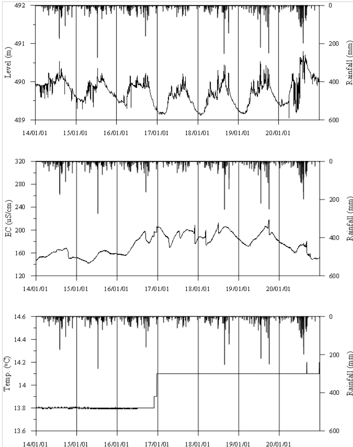
<산청2 관측공의 장기관측자료 (2014.1.1 ~ 2020.12.31)> (a)지하수위, (b)전기전도도, (c)수온
