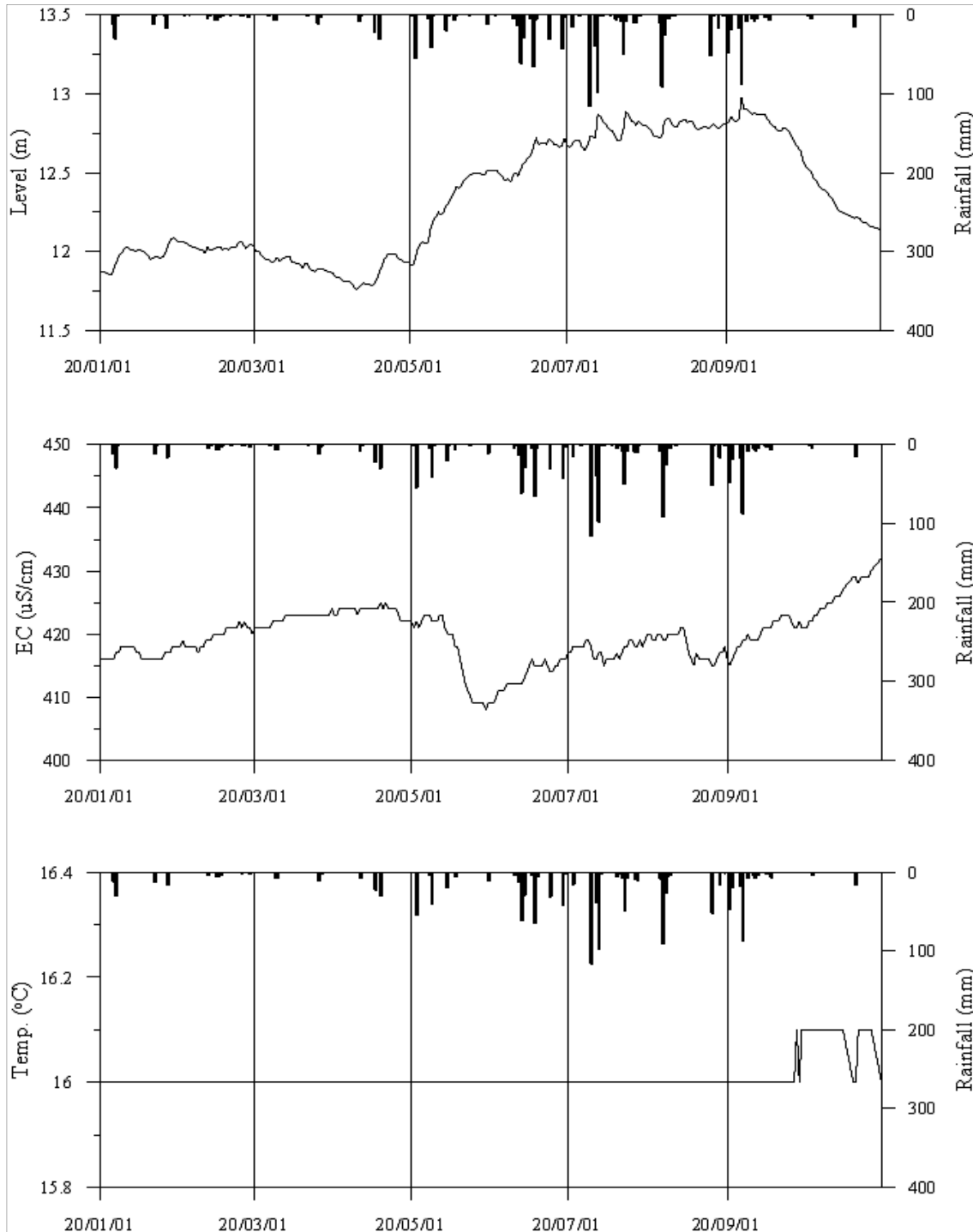
<영암4 관측공의 장기관측자료 (2020.1.1~2020.10.31)> (a)지하수위, (b)전기전도도, (c)수온
