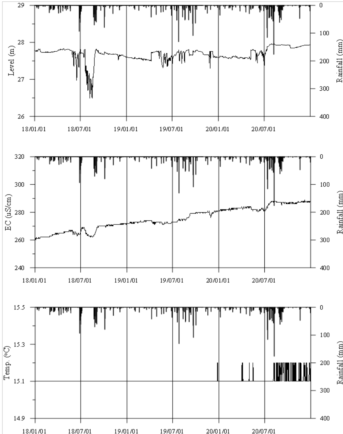
<정읍6 관측공의 장기관측자료 (2018.1.1 ~ 2020.12.31)> (a)지하수위, (b)전기전도도, (c)수온
