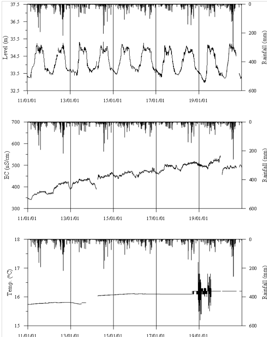
<화순1 관측공의 장기관측자료 (2011.1.1 ~ 2020.12.31)> (a)지하수위, (b)전기전도도, (c)수온
