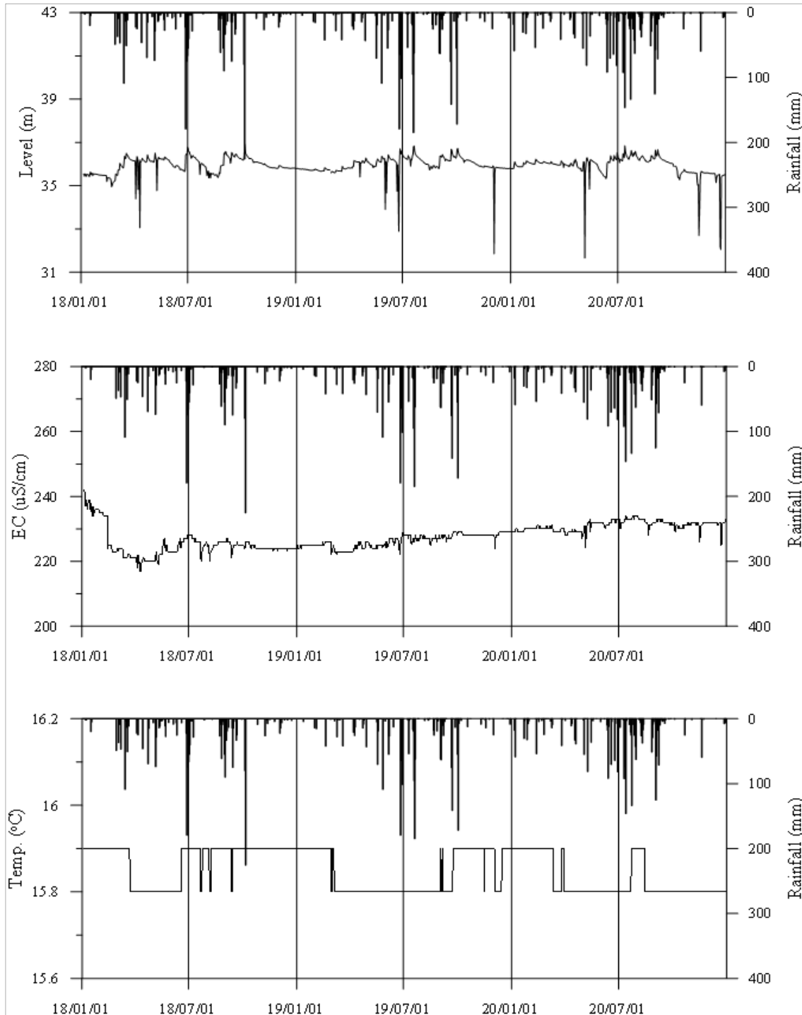
<남해4 관측공의 장기관측자료 (2018.1.1 ~ 2020.12.31)> (a)지하수위, (b)전기전도도, (c)수온
