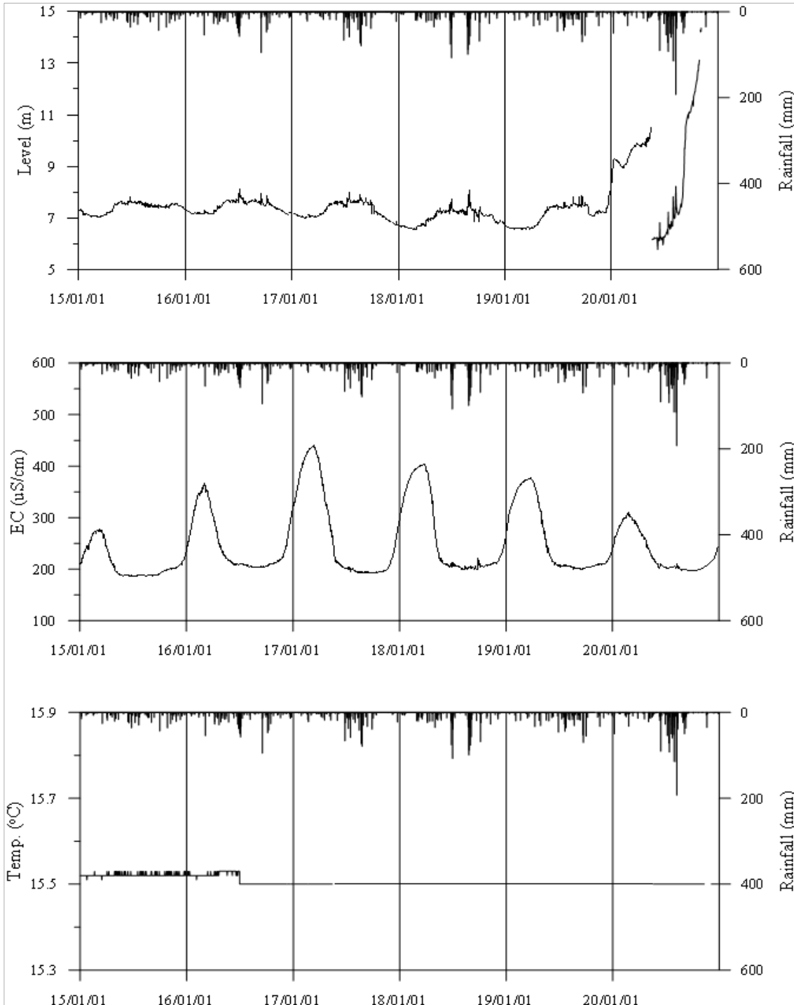
<완주1 관측공의 장기관측자료 (2015.1.1 ~ 2020.12.31)> (a)지하수위, (b)전기전도도, (c)수온
