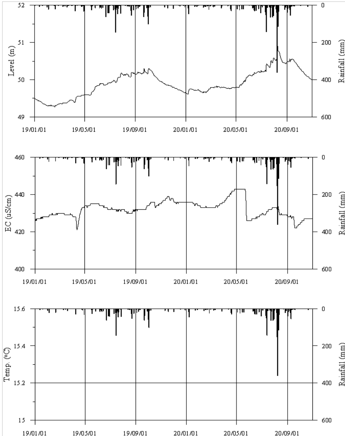
<담양4 관측공의 장기관측자료 (2019.1.1~2020.10.31)> (a)지하수위, (b)전기전도도, (c)수온
