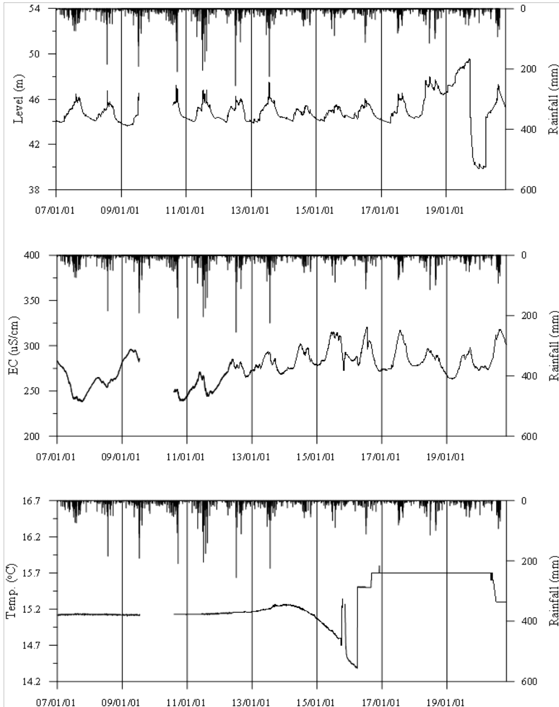
<원주2 관측공의 장기관측자료 (2007.1.1 ~ 2020.12.31)> (a)지하수위, (b)전기전도도, (c)수온
