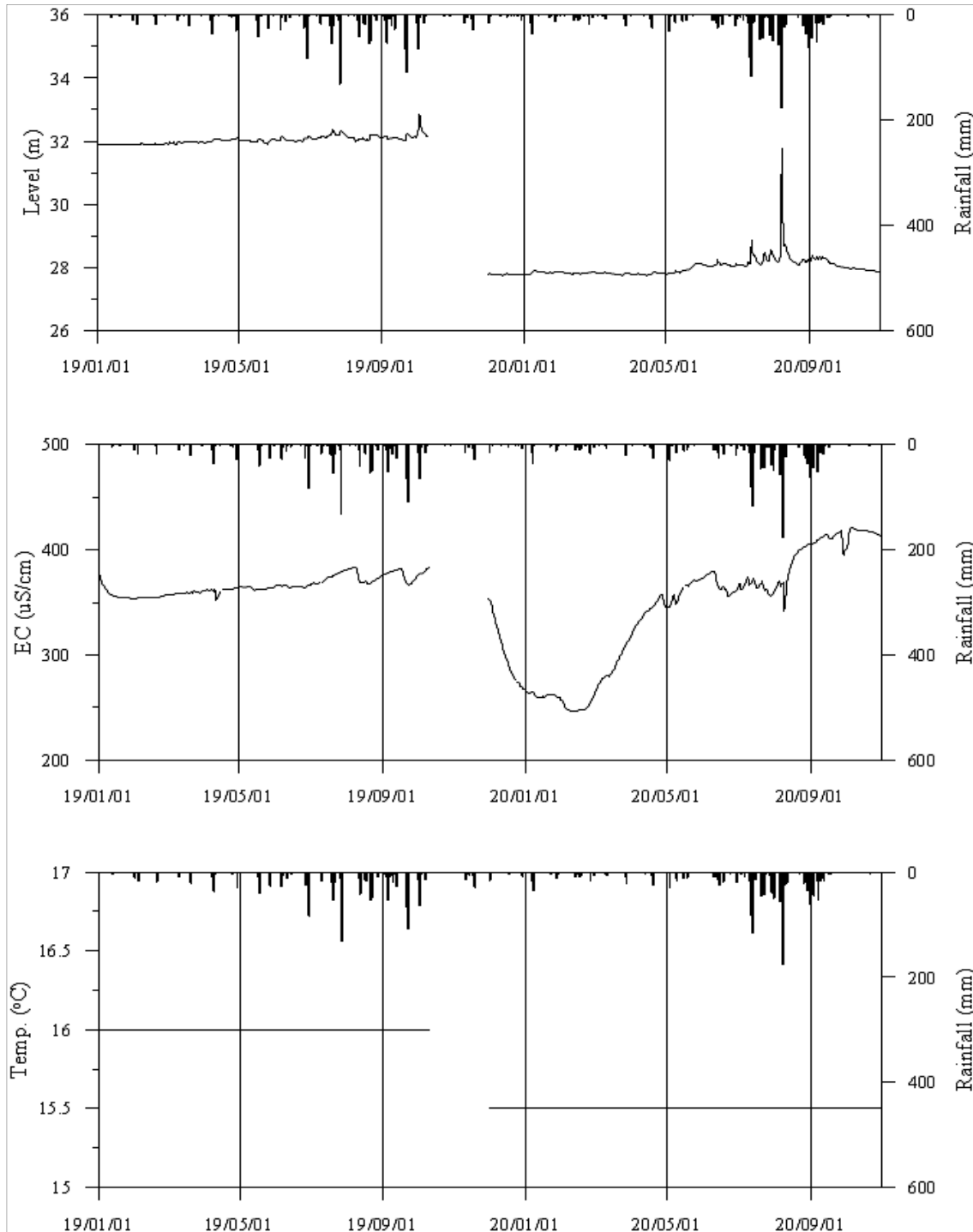
<담양3 관측공의 장기관측자료 (2019.1.1~2020.10.31)> (a)지하수위, (b)전기전도도, (c)수온
