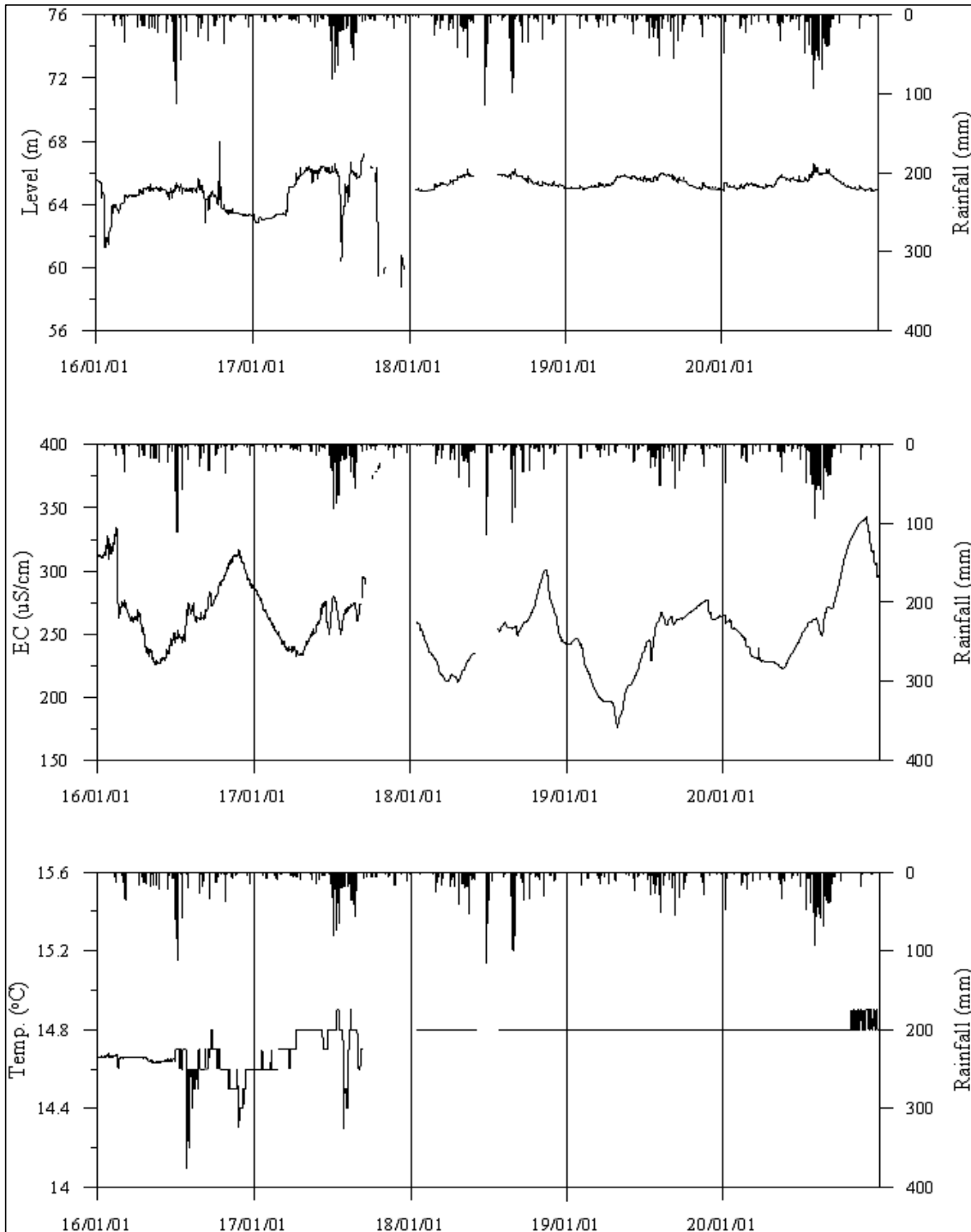
<원주3 관측공의 장기관측자료 (2016.1.1 ~ 2020.12.31)> (a)지하수위, (b)전기전도도, (c)수온
