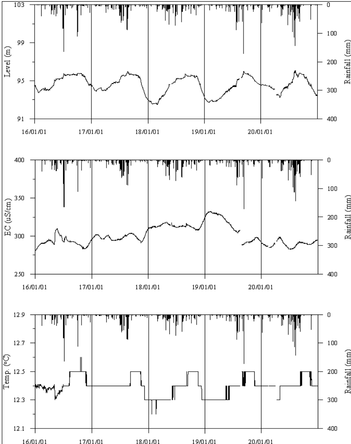
<양주1 관측공의 장기관측자료 (2016.1.1 ~ 2020.12.31)> (a)지하수위, (b)전기전도도, (c)수온
