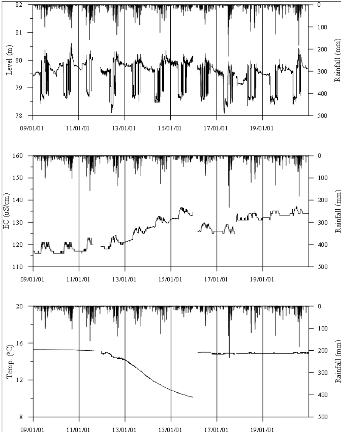
<진천1 관측공의 장기관측자료 (2009.1.1 ~ 2020.12.31)> (a)지하수위, (b)전기전도도, (c)수온
