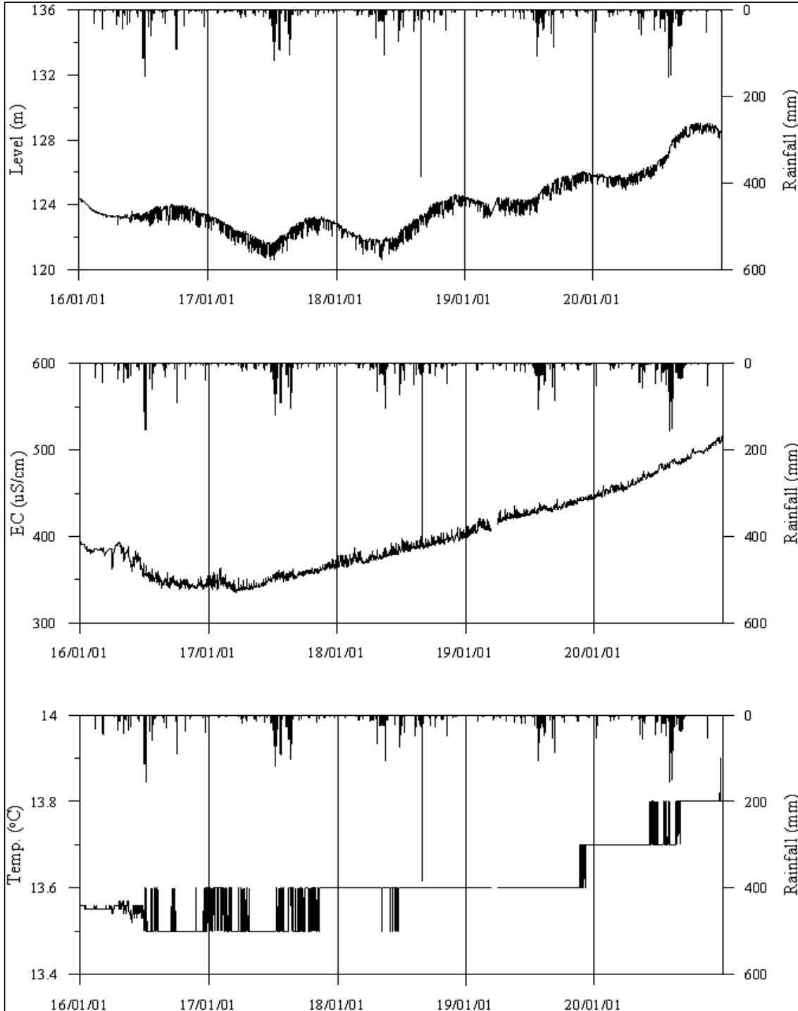
<포천1 관측공의 장기관측자료 (2016.1.1 ~ 2020.12.31)> (a)지하수위, (b)전기전도도, (c)수온
