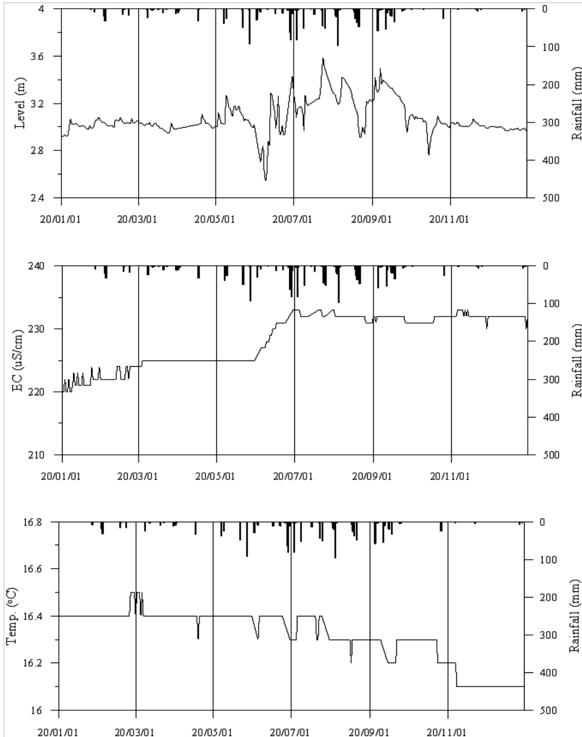
<보성7 관측공의 장기관측자료 (2020.1.1 ~ 2020.12.31)> (a)지하수위, (b)전기전도도, (c)수온
