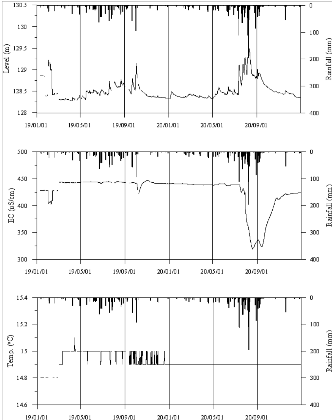
<임실2 관측공의 장기관측자료 (2019.1.1 ~ 2020.12.31)> (a)지하수위, (b)전기전도도, (c)수온
