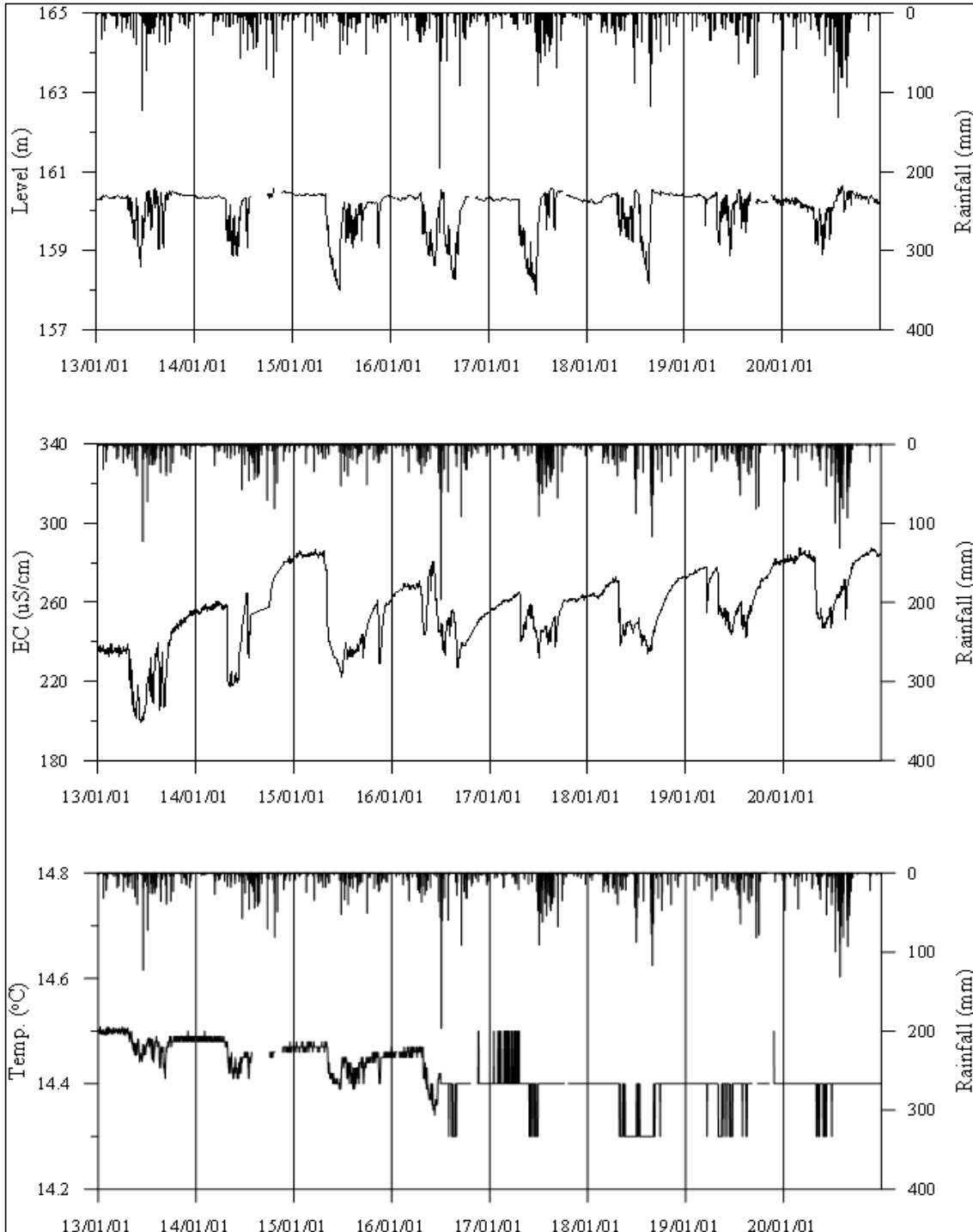
<보은1 관측공의 장기관측자료 (2013.1.1 ~ 2020.12.31)> (a)지하수위, (b)전기전도도, (c)수온
