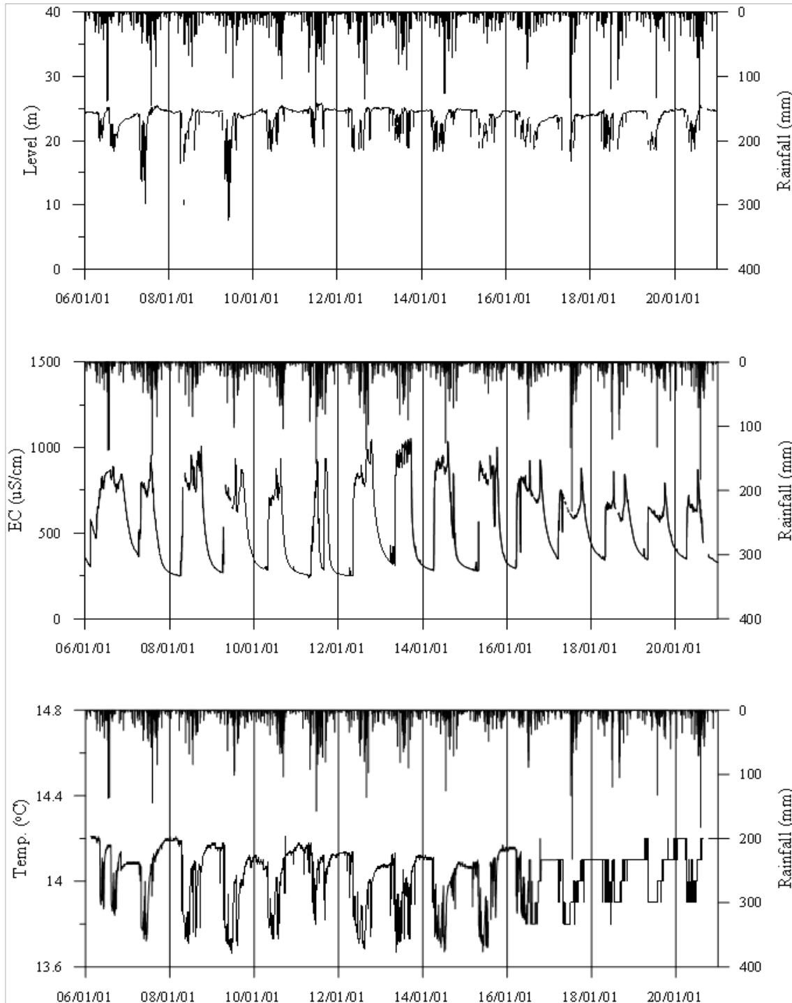
<아산3 관측공의 장기관측자료 (2006.1.1 ~ 2020.12.31)> (a)지하수위, (b)전기전도도, (c)수온
