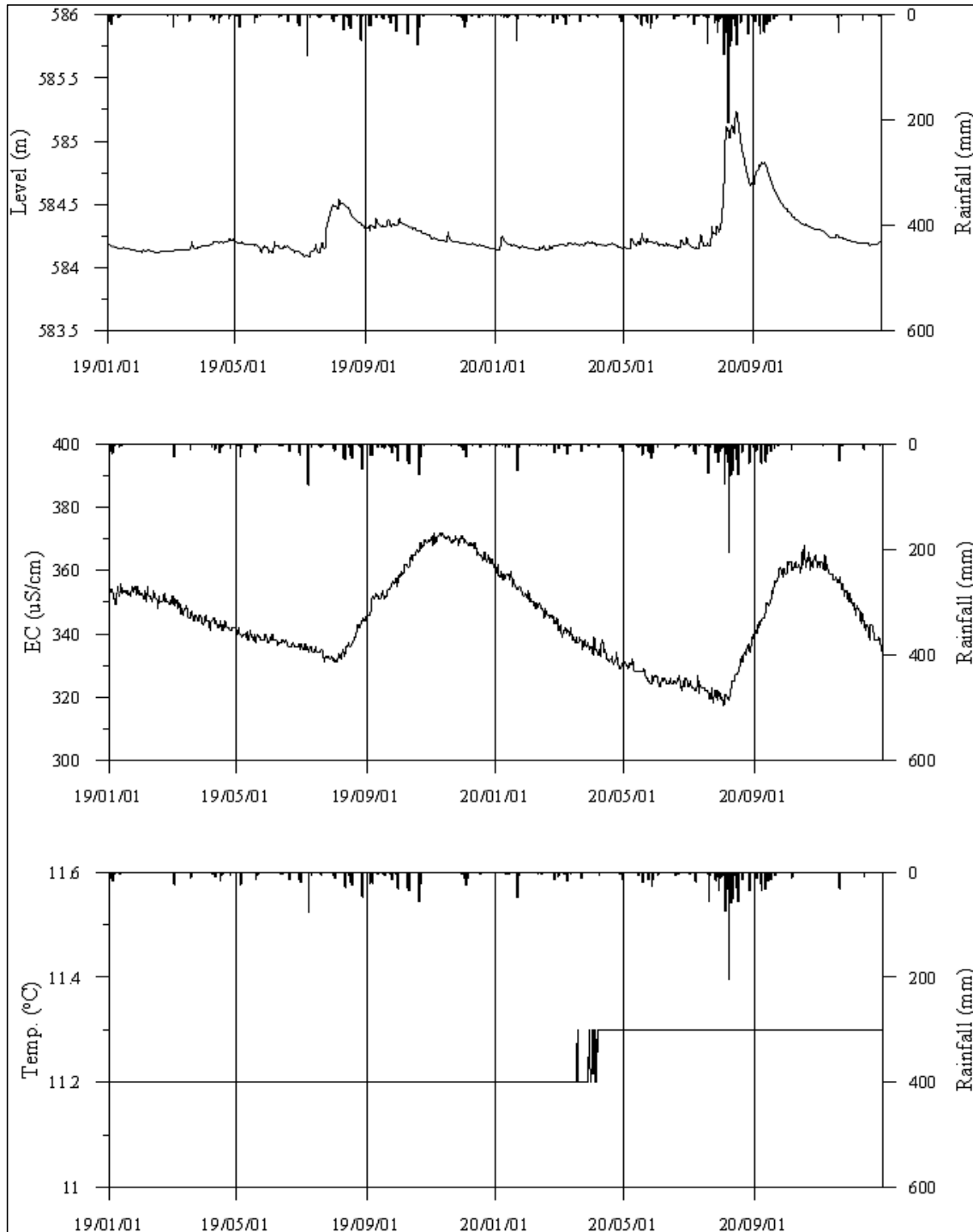
<평창4 관측공의 장기관측자료 (2019.1.1 ~ 2020.12.31)> (a)지하수위, (b)전기전도도, (c)수온
