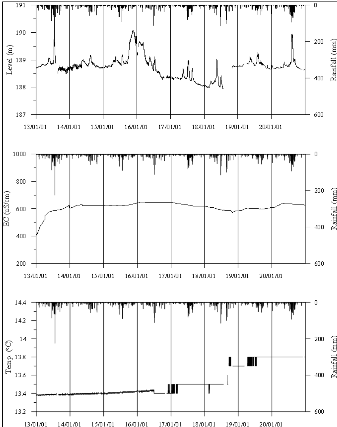
<황성2 관측공의 장기관측자료 (2013.1.1 ~ 2020.12.31)> (a)지하수위, (b)전기전도도, (c)수온
