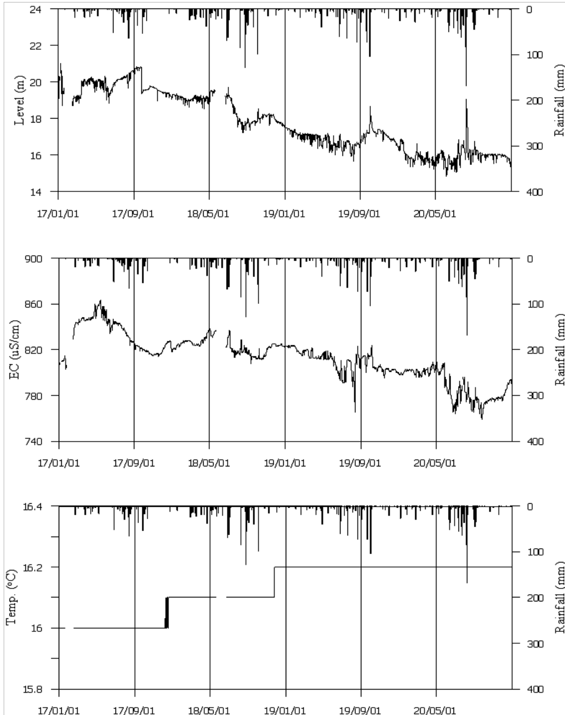
<칠곡1 관측공의 장기관측자료 (2017.1.1 ~ 2020.12.31.)> (a)지하수위, (b)전기전도도, (c)수온
