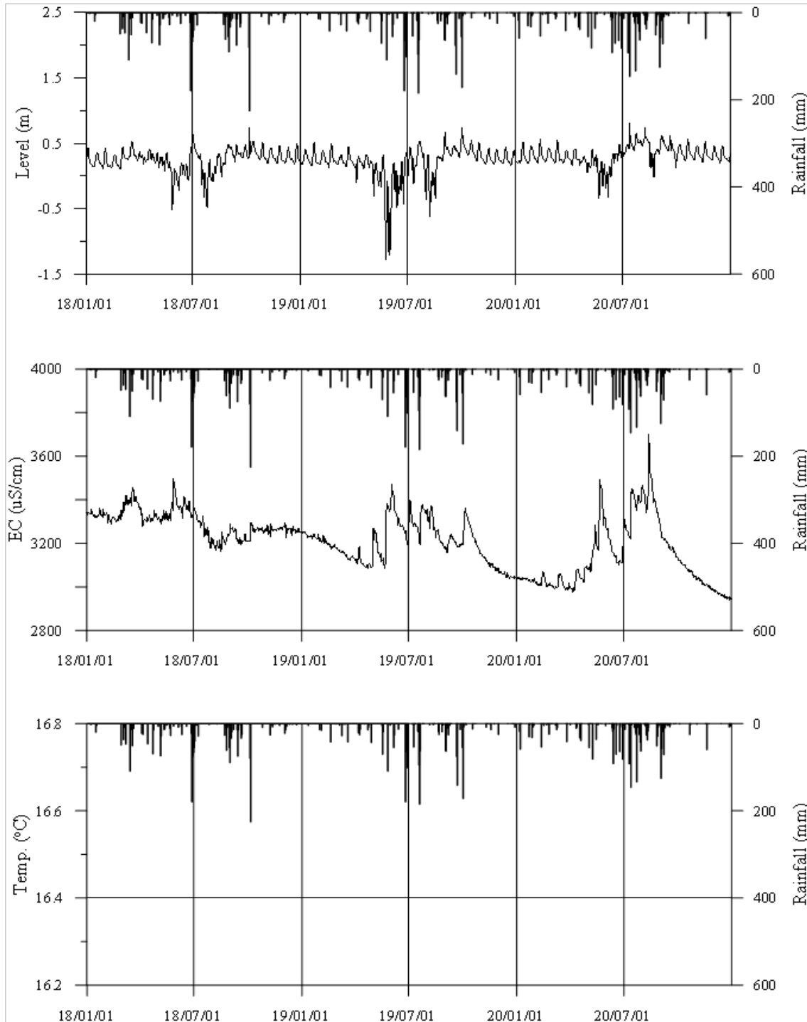
<하동3 관측공의 장기관측자료 (2018.1.1 ~ 2020.12.31)> (a)지하수위, (b)전기전도도, (c)수온
