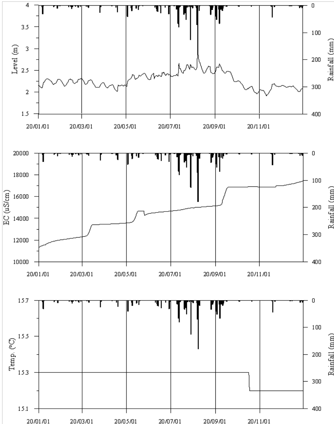
<고창4 관측공의 장기관측자료 (2020.1.1 ~ 2020.12.31)> (a)지하수위, (b)전기전도도, (c)수온
