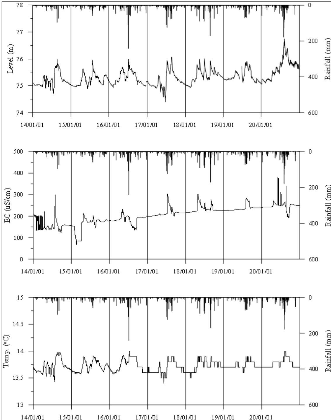
<가평2 관측공의 장기관측자료 (2014.1.1 ~ 2020.12.31)> (a)지하수위, (b)전기전도도, (c)수온
