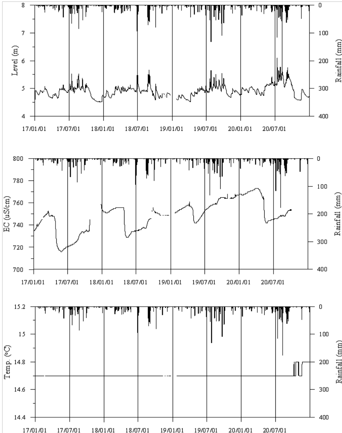
<정읍2 관측공의 장기관측자료 (2017.1.1 ~ 2020.12.31)> (a)지하수위, (b)전기전도도, (c)수온
