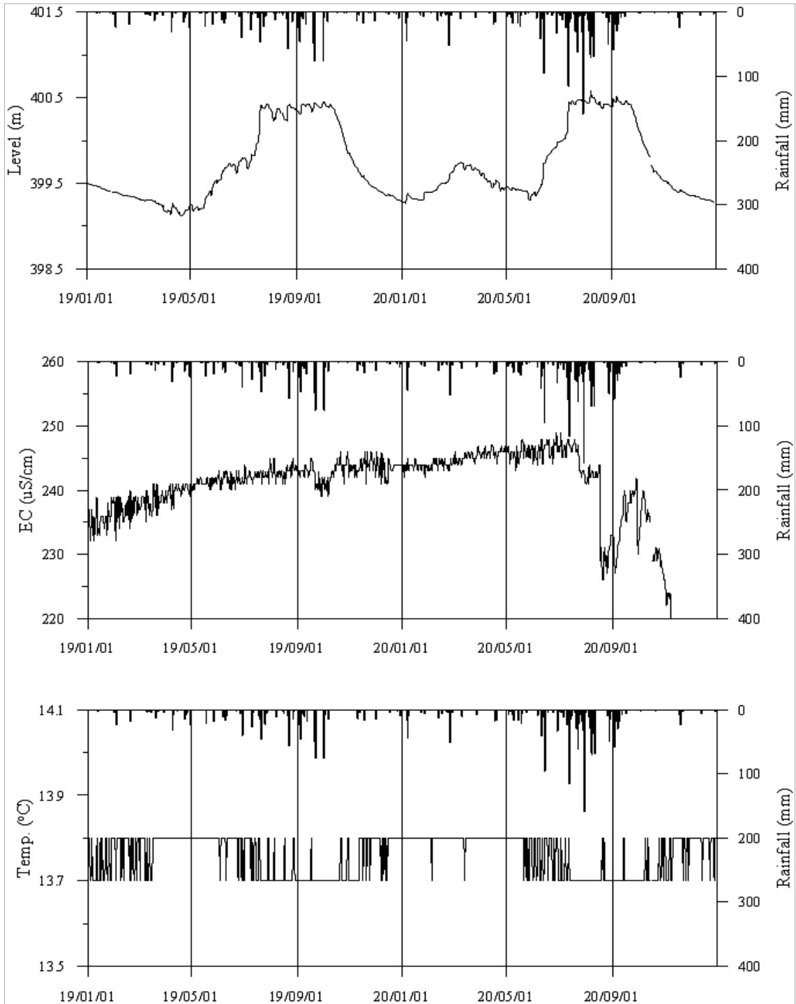
<무주3 관측공의 장기관측자료 (2019.1.1 ~ 2020.12.31)> (a)지하수위, (b)전기전도도, (c)수온
