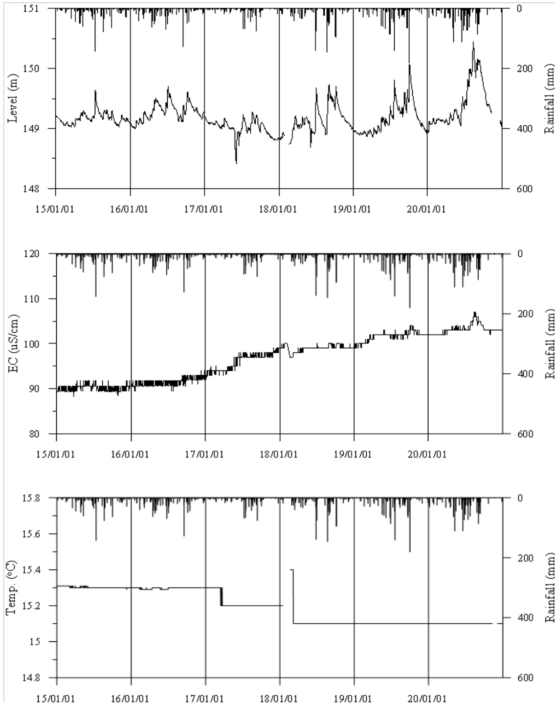
<장흥3 관측공의 장기관측자료 (2015.1.1 ~ 2020.12.31)> (a)지하수위, (b)전기전도도, (c)수온
