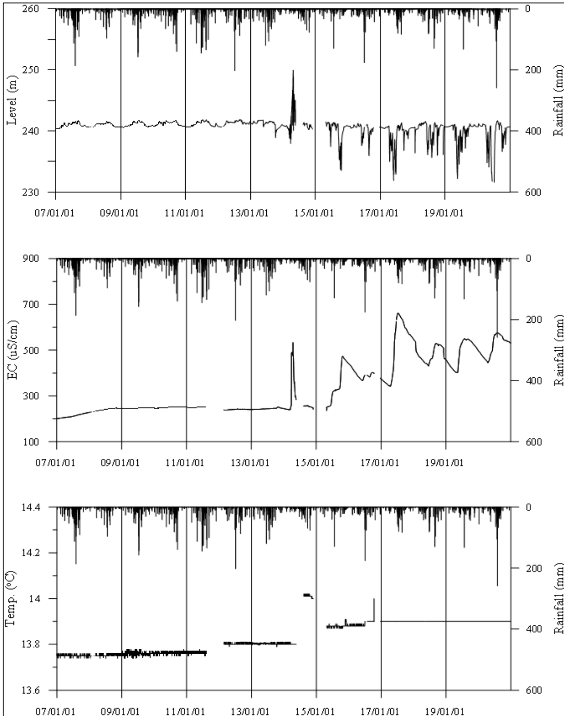
<제천2 관측공의 장기관측자료 (2007.1.1 ~ 2020.12.31)> (a)지하수위, (b)전기전도도, (c)수온
