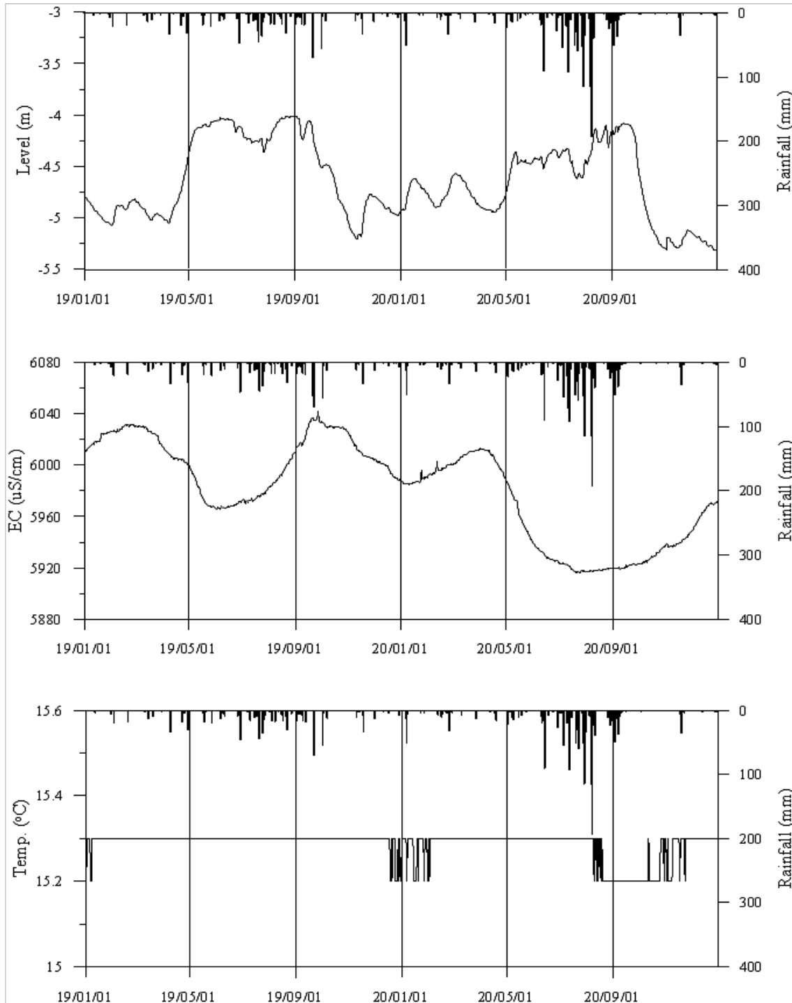
<익산5 관측공의 장기관측자료 (2019.1.1 ~ 2020.12.31)> (a)지하수위, (b)전기전도도, (c)수온
