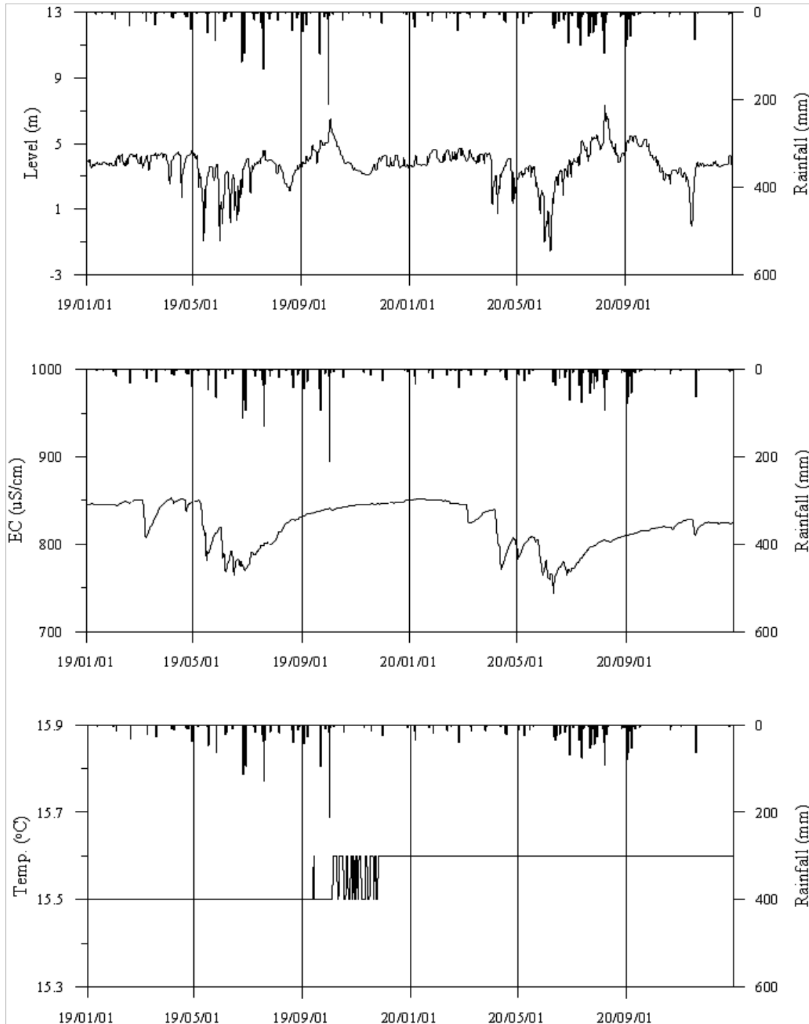
<함안2 관측공의 장기관측자료 (2019.1.1 ~ 2020.12.31)> (a)지하수위, (b)전기전도도, (c)수온
