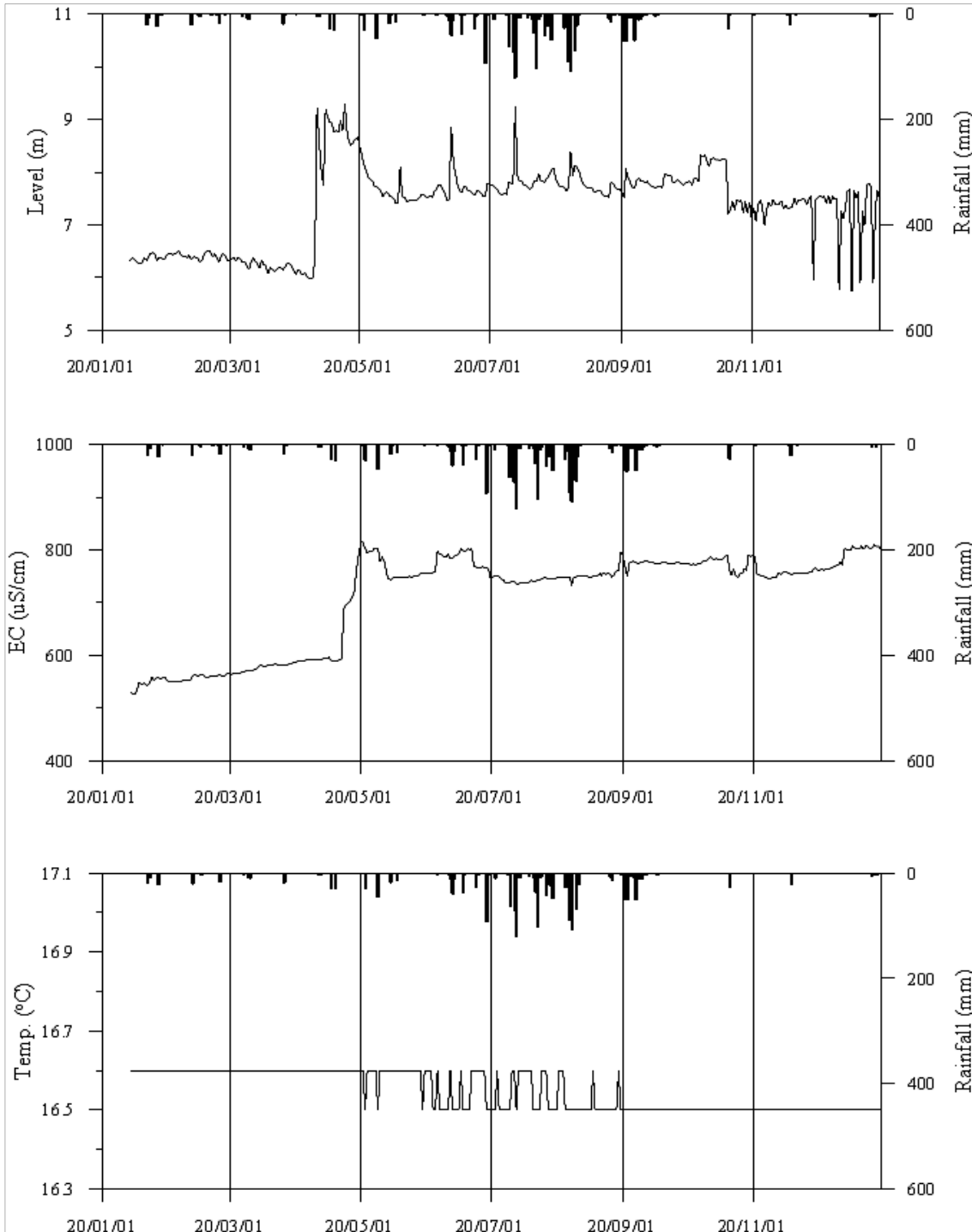
<사천1(신) 관측공의 장기관측자료 (2020.1.1 ~ 2020.12.31)> (a)지하수위, (b)전기전도도, (c)수온
