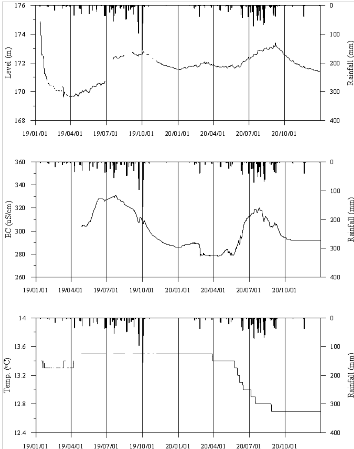
<군위3 관측공의 장기관측자료 (2019.1.1 ~ 2020.12.31)> (a)지하수위, (b)전기전도도, (c)수온
