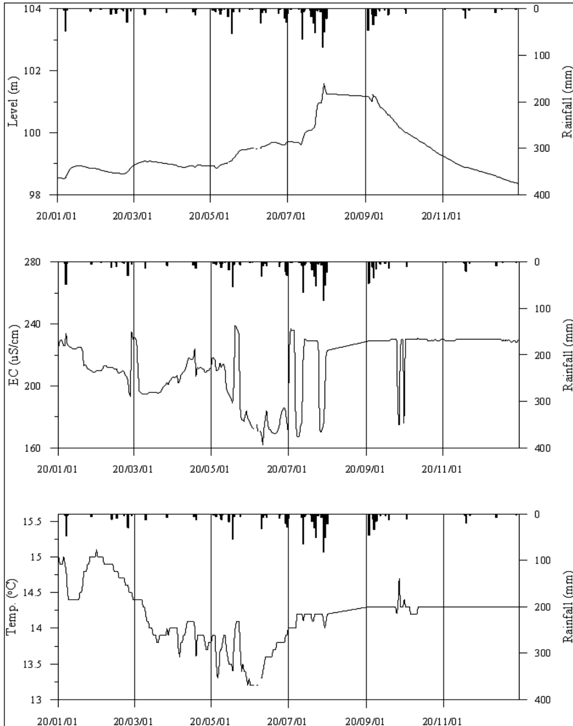
<괴산4 관측공의 장기관측자료 (2020.1.1 ~ 2020.12.31)> (a)지하수위, (b)전기전도도, (c)수온
