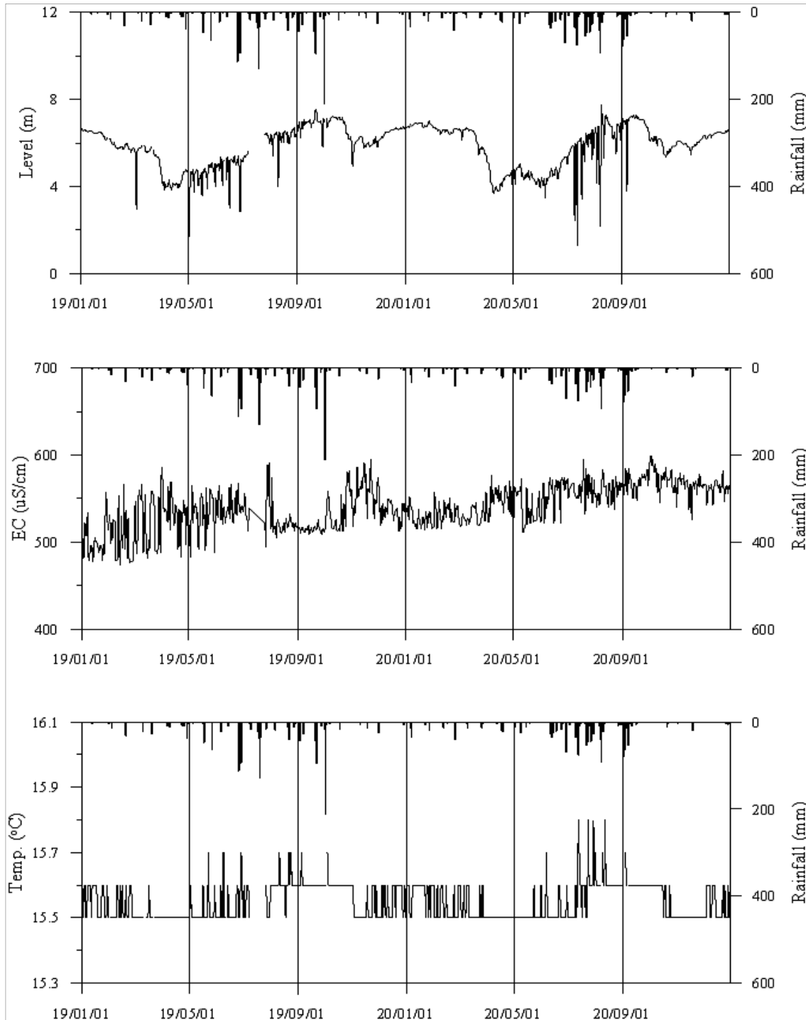
<함안4 관측공의 장기관측자료 (2019.1.1 ~ 2020.12.31)> (a)지하수위, (b)전기전도도, (c)수온
