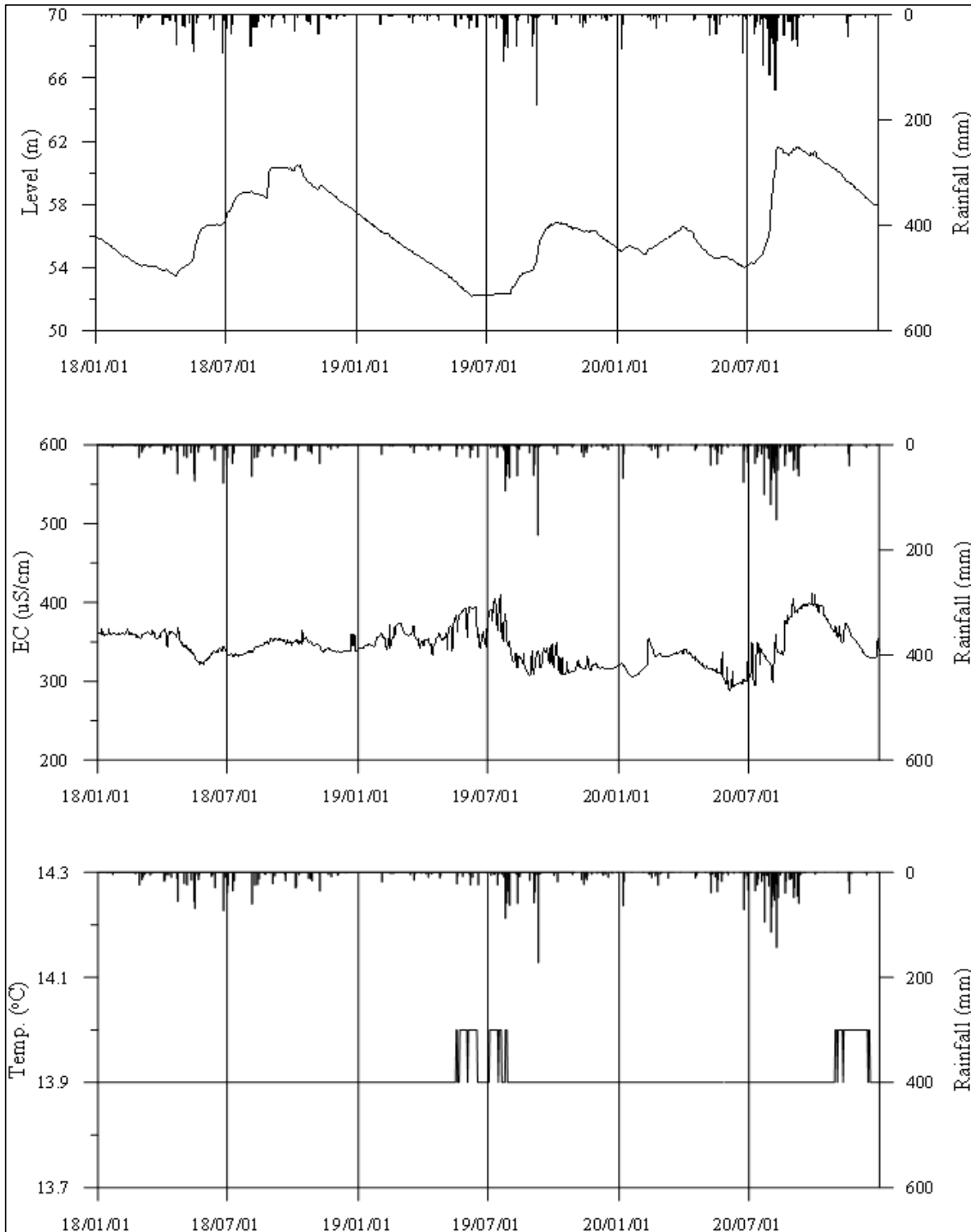
<파주4 관측공의 장기관측자료 (2018.1.1 ~ 2020.12.31)> (a)지하수위, (b)전기전도도, (c)수온
