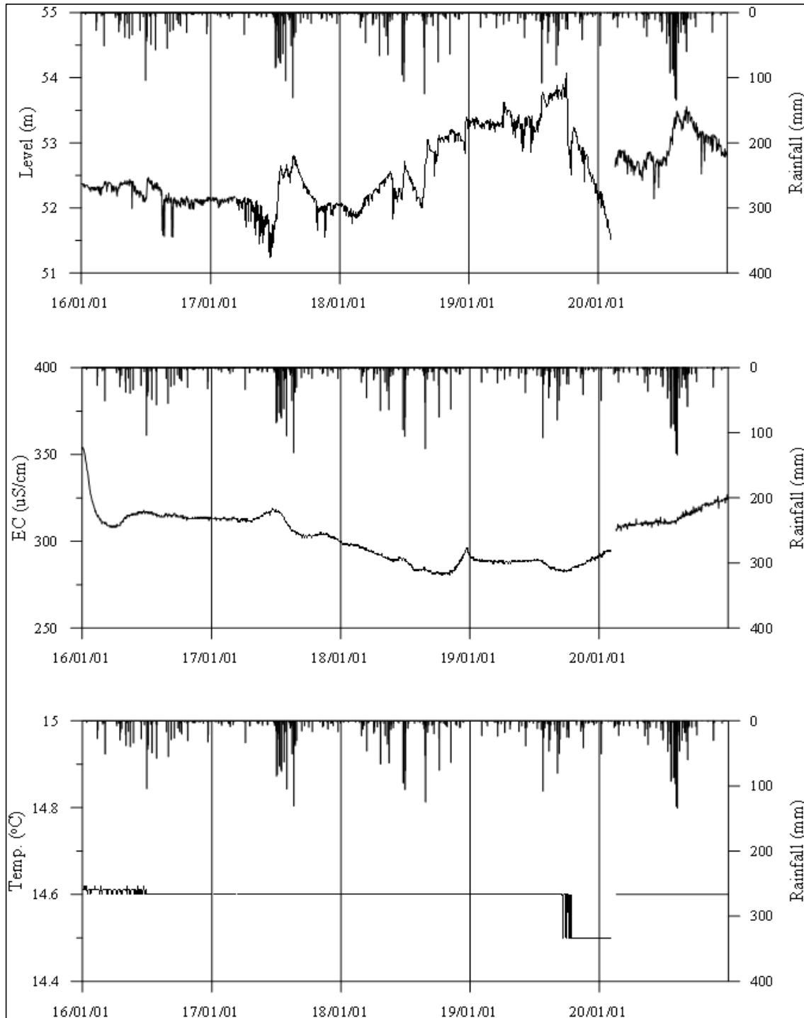
<안성4 관측공의 장기관측자료 (2016.1.1 ~ 2020.12.31)> (a)지하수위, (b)전기전도도, (c)수온
