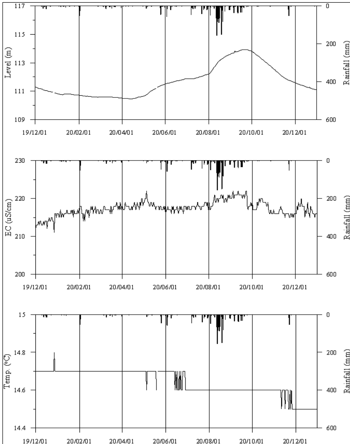
<포천5 관측공의 장기관측자료 (2019.12.1 ~ 2020.12.31)> (a)지하수위, (b)전기전도도, (c)수온
