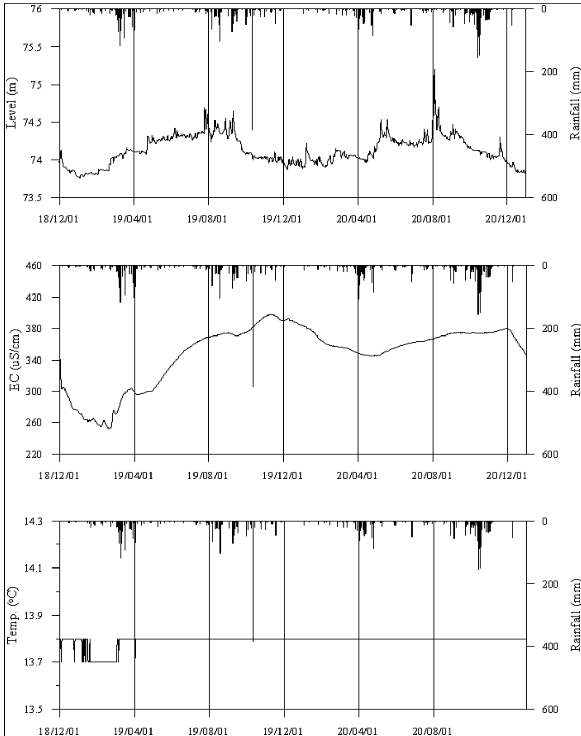
<포천3 관측공의 장기관측자료 (2018.12.1 ~ 2020.12.31)> (a)지하수위, (b)전기전도도, (c)수온
