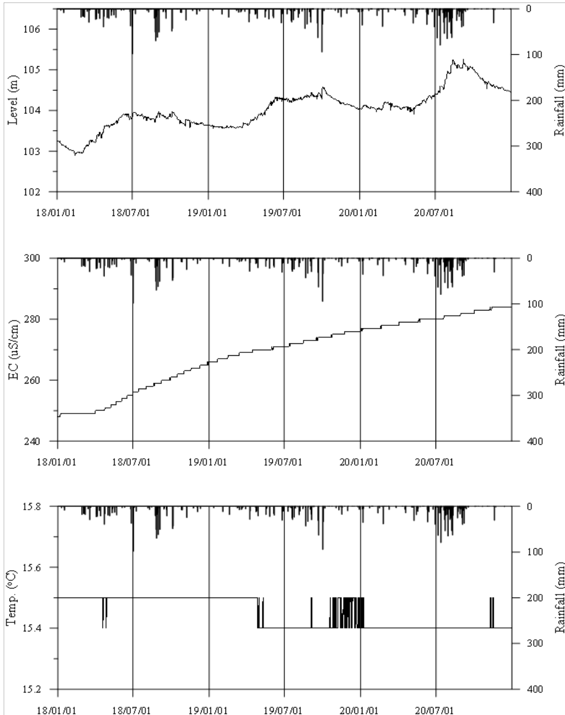
<안동5 관측공의 장기관측자료 (2018.1.1 ~ 2020.12.31)> (a)지하수위, (b)전기전도도, (c)수온
