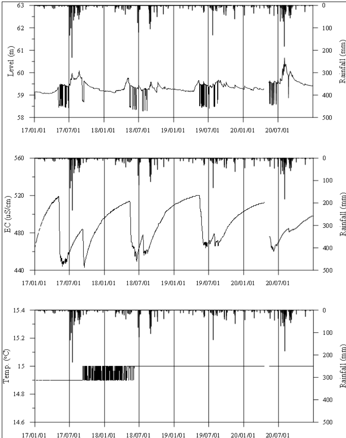
<진천2 관측공의 장기관측자료 (2017.1.1 ~ 2020.12.31)> (a)지하수위, (b)전기전도도, (c)수온
