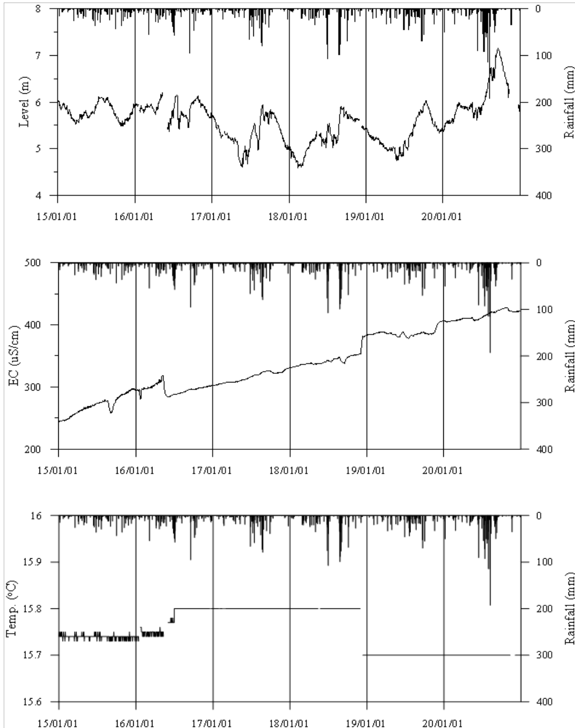
<익산2 관측공의 장기관측자료 (2015.1.1 ~ 2020.12.31)> (a)지하수위, (b)전기전도도, (c)수온
