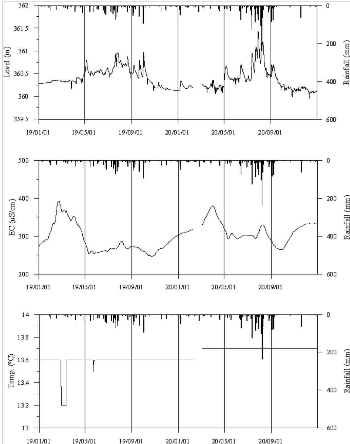
<장수3 관측공의 장기관측자료 (2019.1.1 ~ 2020.12.31)> (a)지하수위, (b)전기전도도, (c)수온
