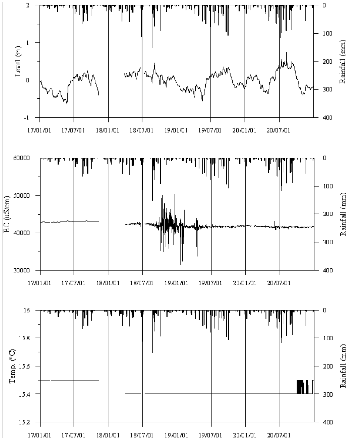
<함평5 관측공의 장기관측자료 (2017.1.1~2020.12.31)> (a)지하수위, (b)전기전도도, (c)수온
