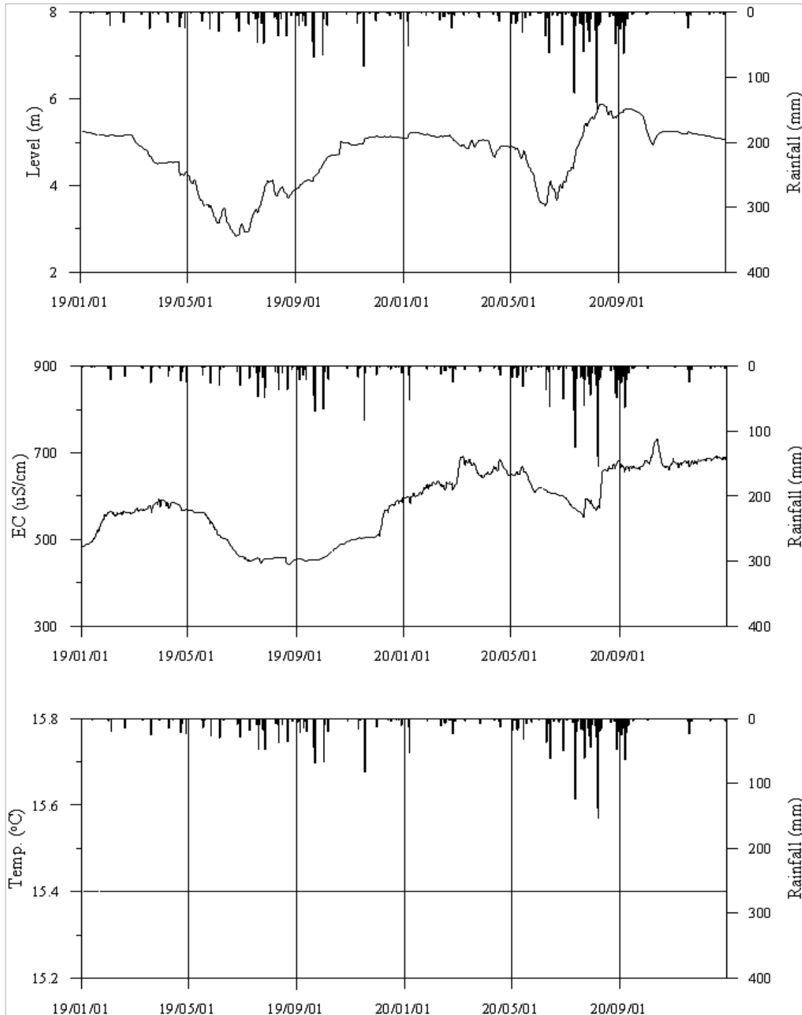
<서천4 관측공의 장기관측자료 (2019.1.1 ~ 2020.12.31)> (a)지하수위, (b)전기전도도, (c)수온
