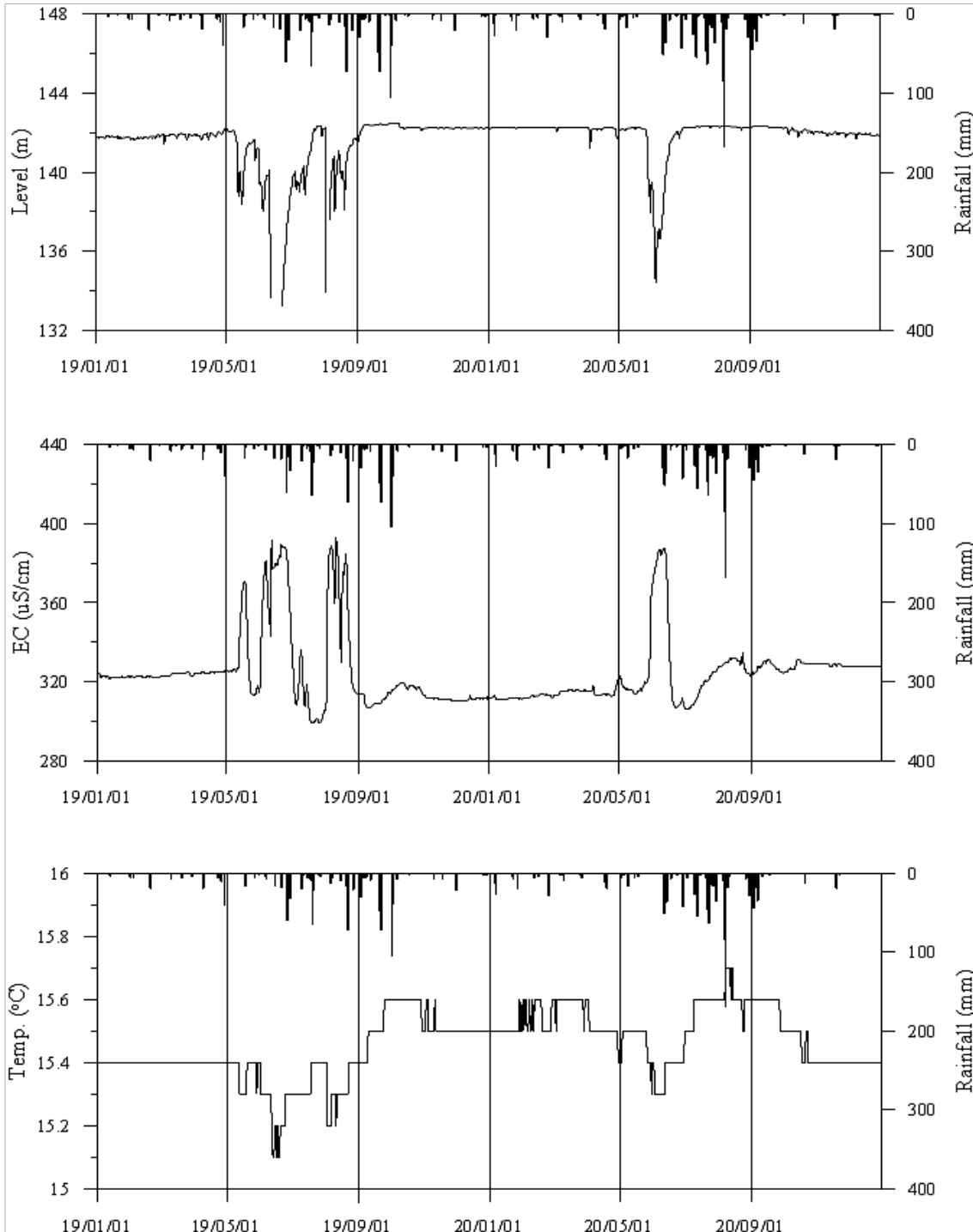
<청도1 관측공의 장기관측자료 (2019.1.1 ~ 2020.12.31.)> (a)지하수위, (b)전기전도도, (c)수온
