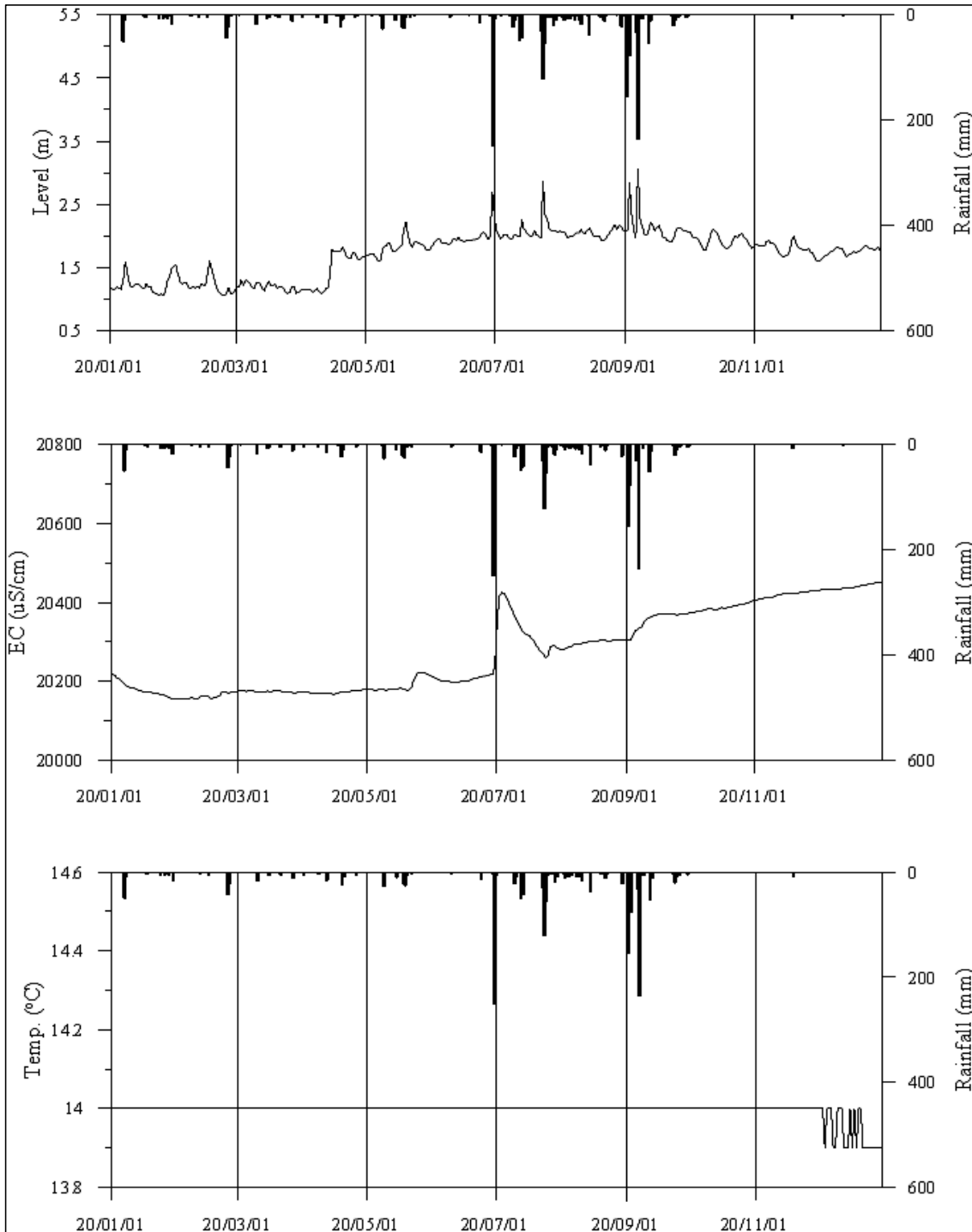
<강릉6 관측공의 장기관측자료 (2020.1.1 ~ 2020.12.31)> (a)지하수위, (b)전기전도도, (c)수온
