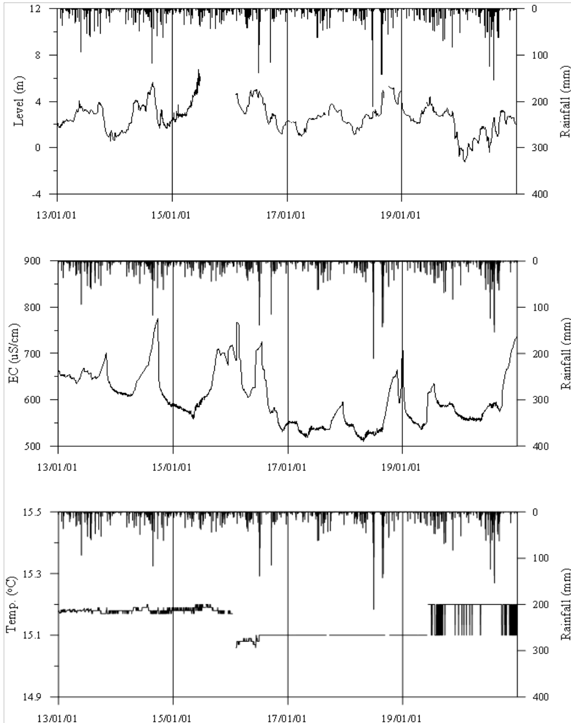
<서천2 관측공의 장기관측자료 (2013.1.1 ~ 2020.12.31)> (a)지하수위, (b)전기전도도, (c)수온
