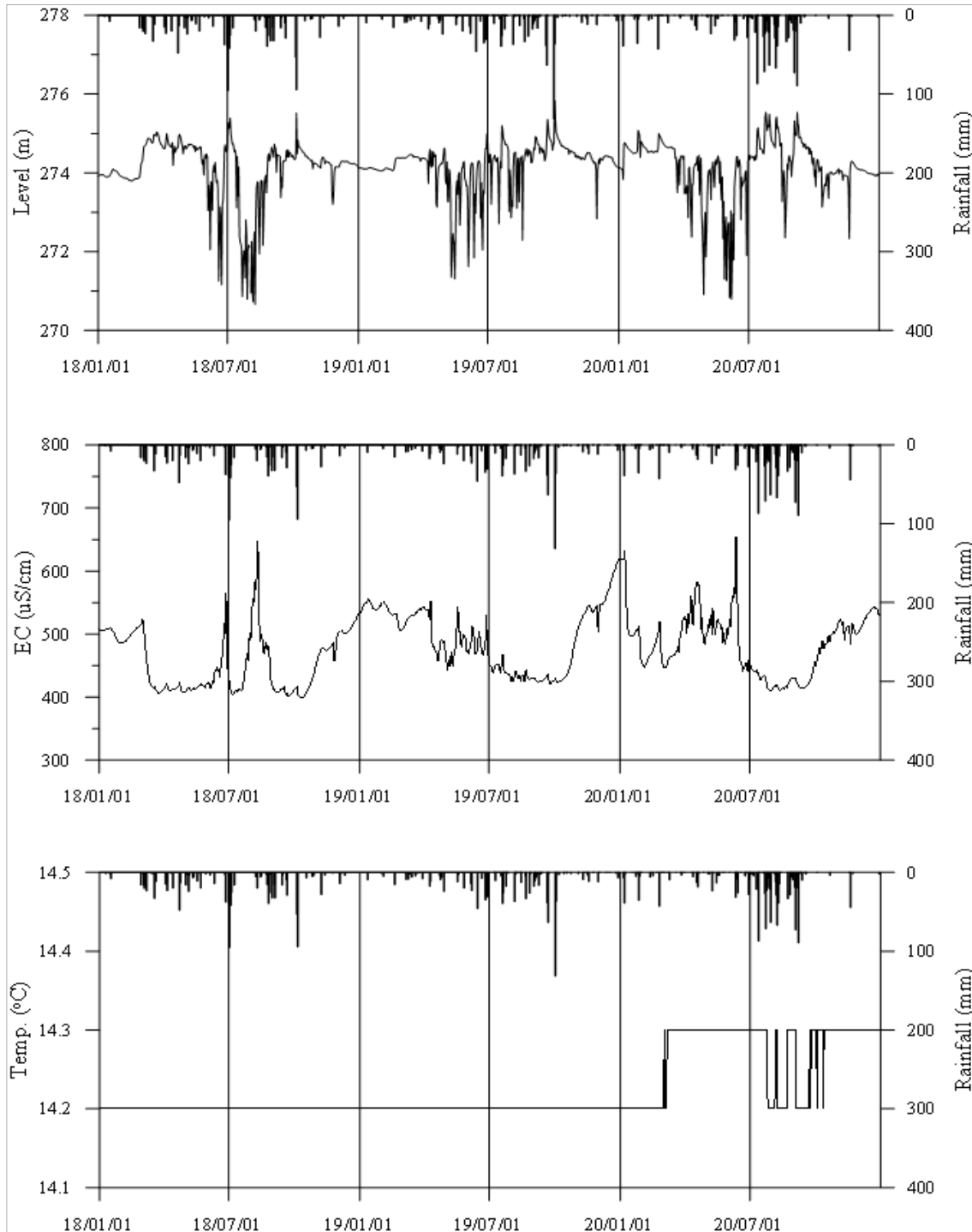
<청송4 관측공의 장기관측자료 (2018.1.1 ~ 2020.12.31)> (a)지하수위, (b)전기전도도, (c)수온
