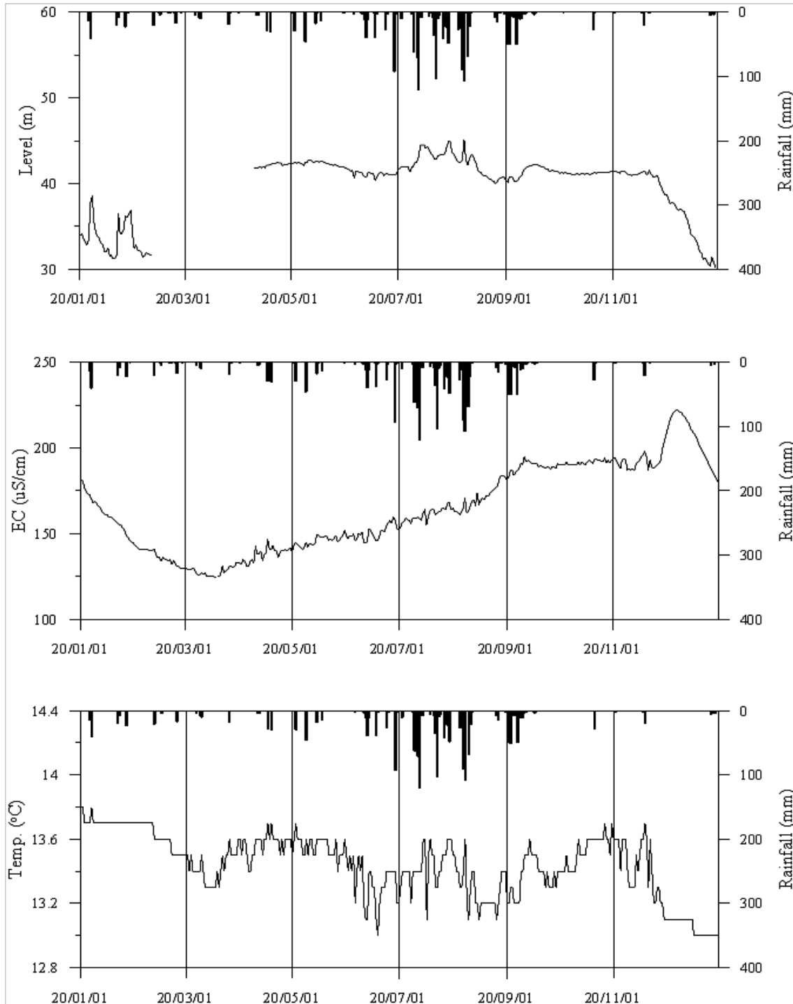
<사천5 관측공의 장기관측자료 (2020.1.1 ~ 2020.12.31)> (a)지하수위, (b)전기전도도, (c)수온
