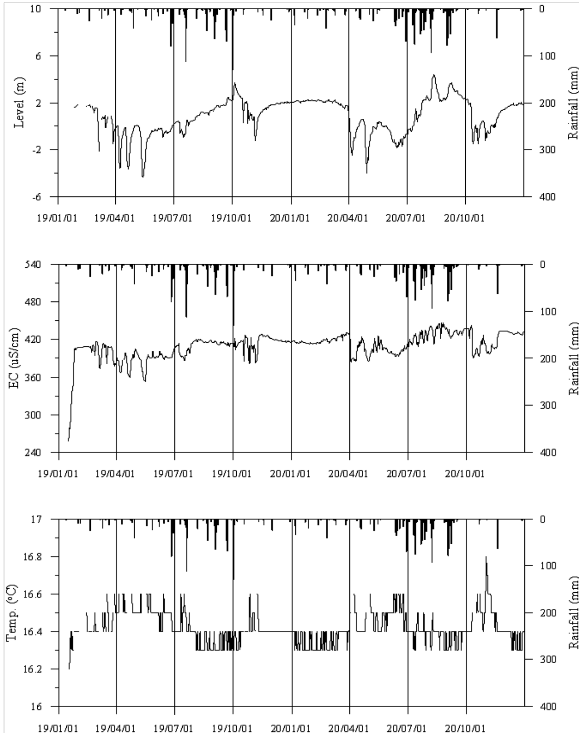
<창녕5 관측공의 장기관측자료 (2019.1.1 ~ 2020.12.31)> (a)지하수위, (b)전기전도도, (c)수온
