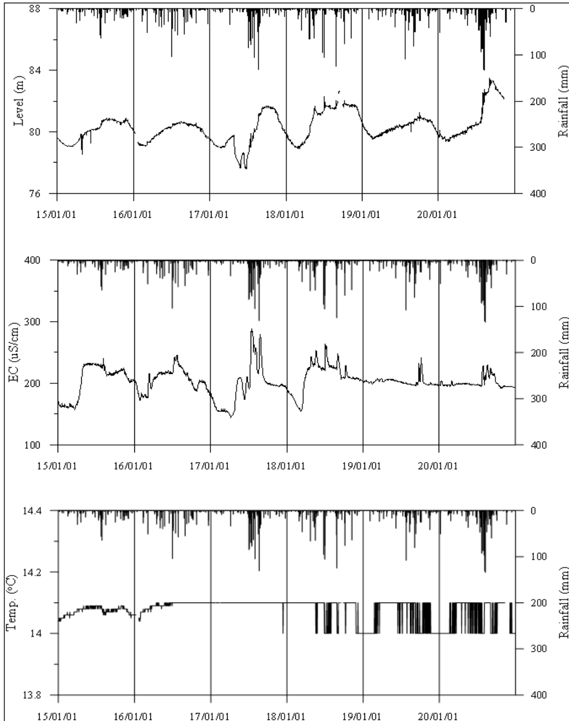
<안성3 관측공의 장기관측자료 (2015.1.1 ~ 2020.12.31)> (a)지하수위, (b)전기전도도, (c)수온
