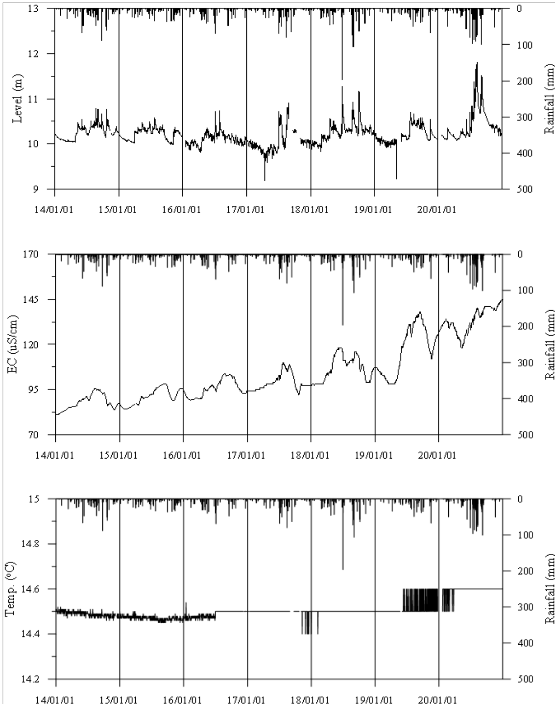
<홍성1 관측공의 장기관측자료 (2014.1.1 ~ 2020.12.31)> (a)지하수위, (b)전기전도도, (c)수온
