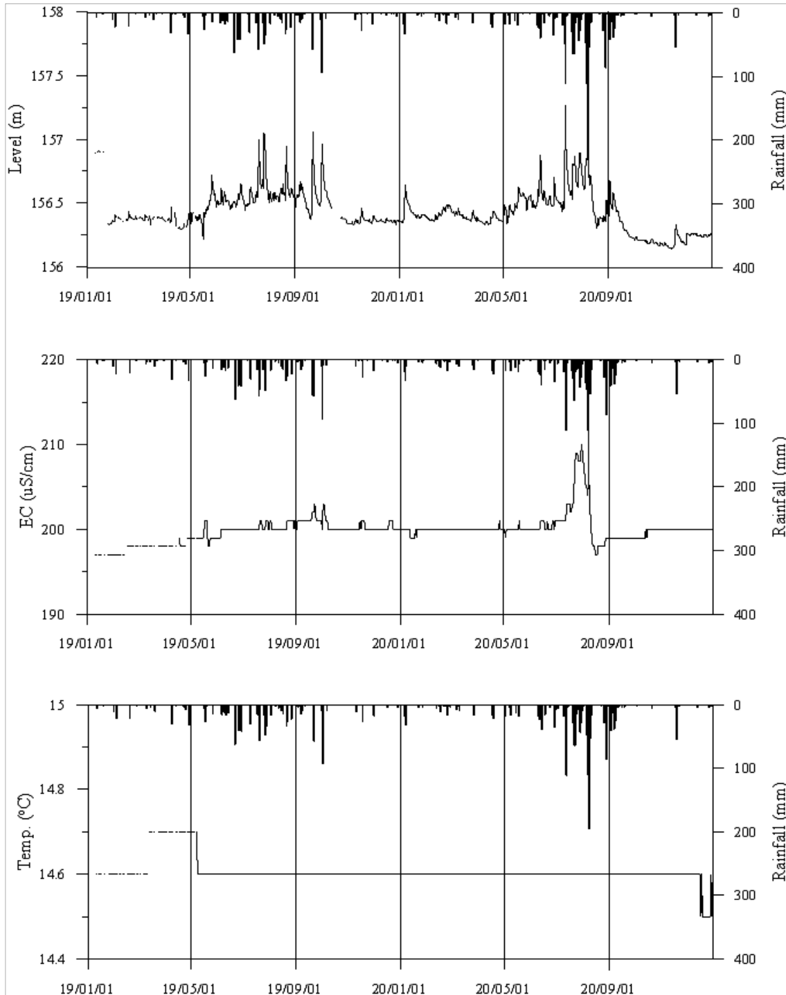
<임실3 관측공의 장기관측자료 (2019.1.1 ~ 2020.12.31)> (a)지하수위, (b)전기전도도, (c)수온
