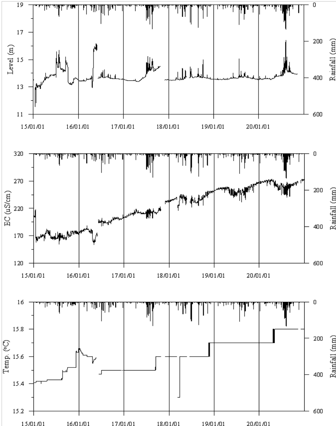
<화성1 관측공의 장기관측자료 (2015.1.1 ~ 2020.12.31)> (a)지하수위, (b)전기전도도, (c)수온
