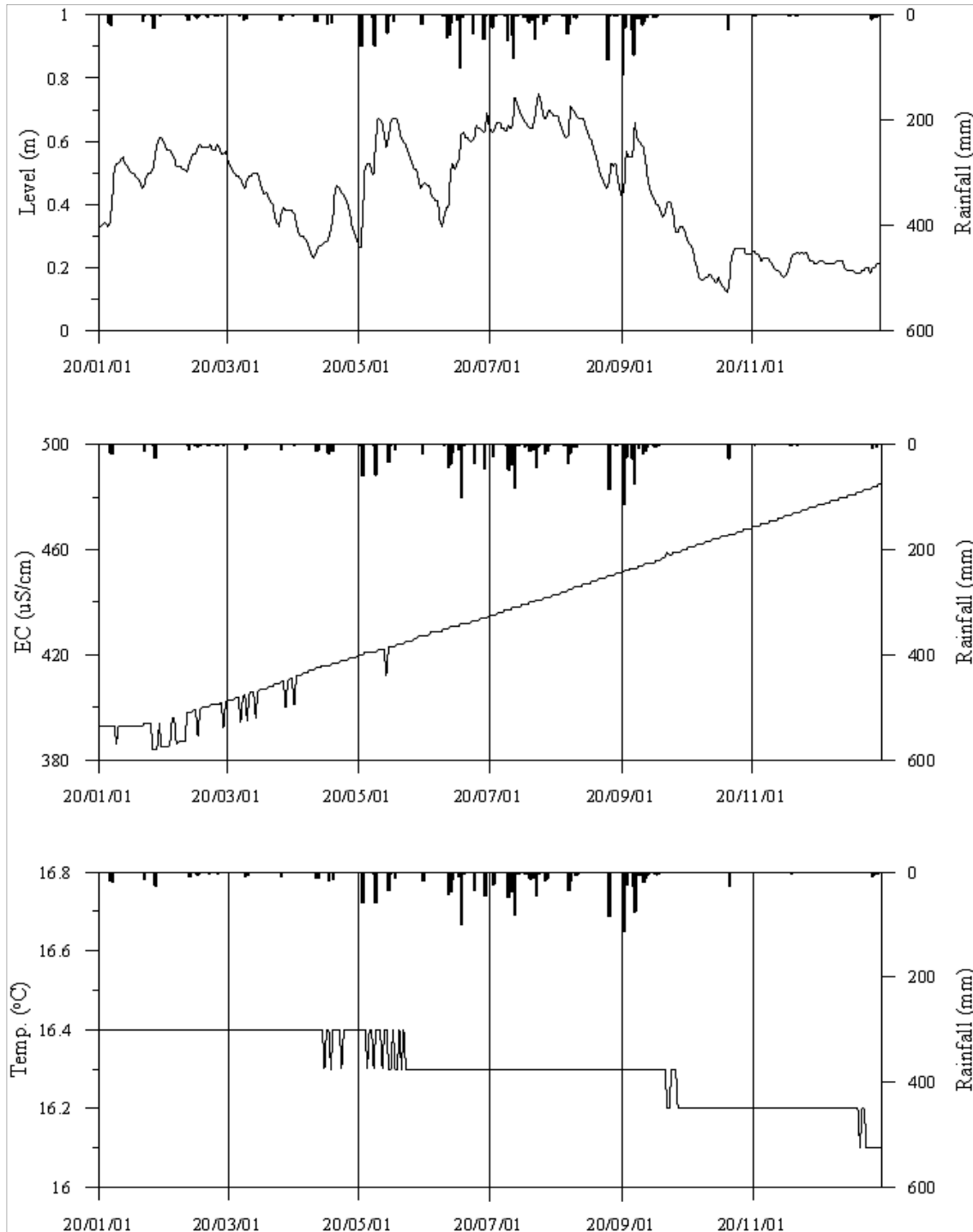
<해남8 관측공의 장기관측자료 (2020.1.1~2020.12.31)> (a)지하수위, (b)전기전도도, (c)수온
