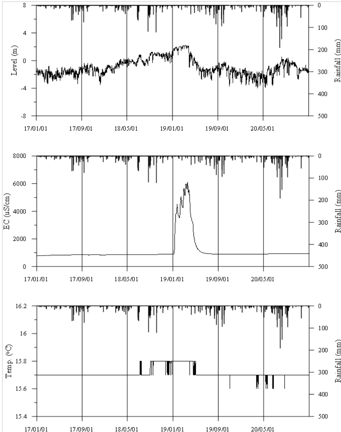
<영광4 관측공의 장기관측자료 (2017.1.1 ~ 2020.12.31)> (a)지하수위, (b)전기전도도, (c)수온
