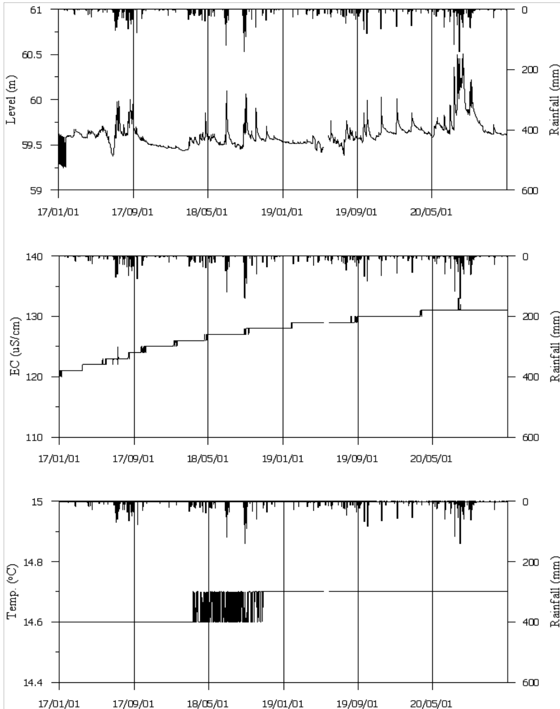
<공주3 관측공의 장기관측자료 (2017.1.1 ~ 2020.12.31)> (a)지하수위, (b)전기전도도, (c)수온
