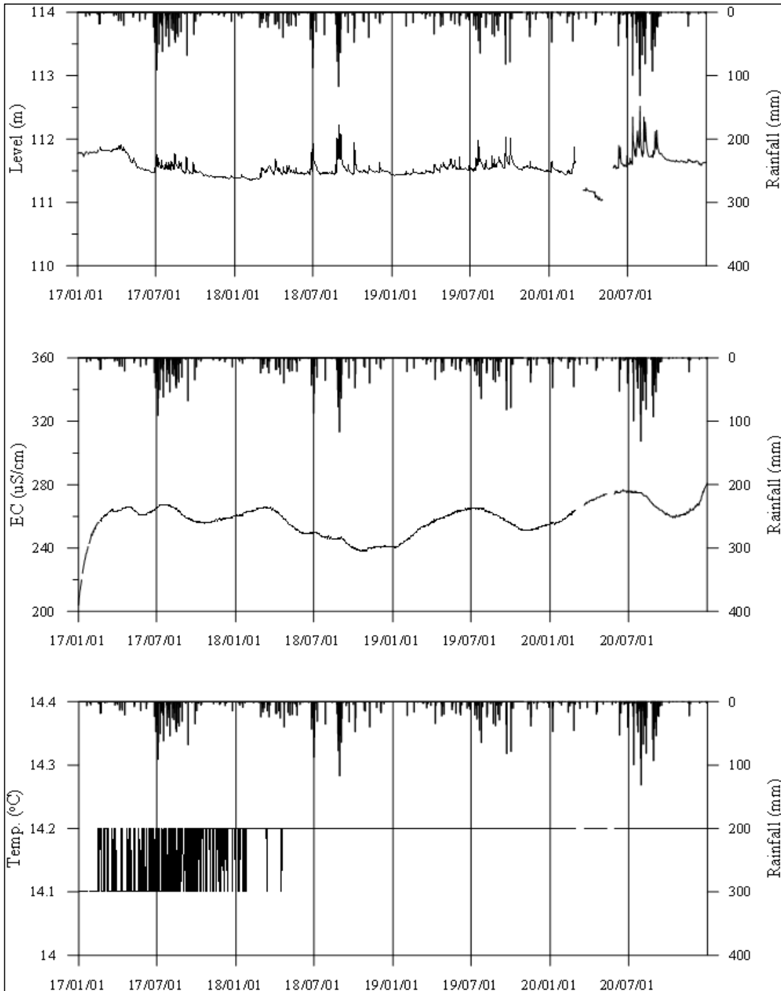
<육천4 관측공의 장기관측자료 (2017.1.1 ~ 2020.12.31)> (a)지하수위, (b)전기전도도, (c)수온
