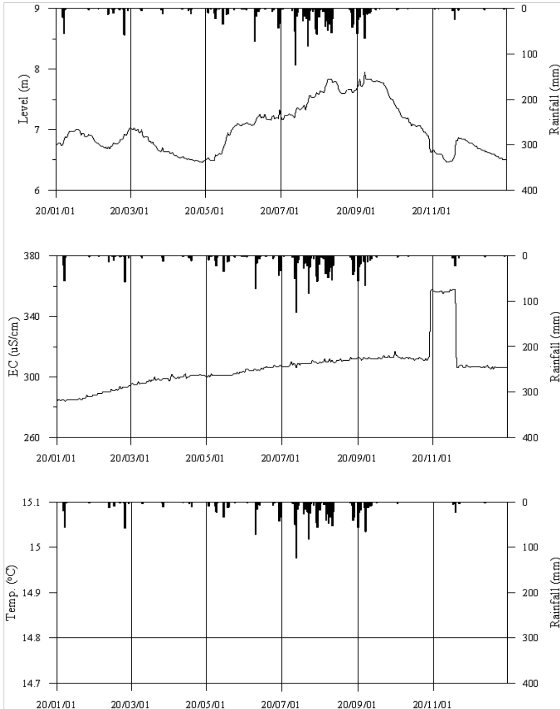
<논산3 관측공의 장기관측자료 (2020.1.1 ~ 2020.12.31)> (a)지하수위, (b)전기전도도, (c)수온
