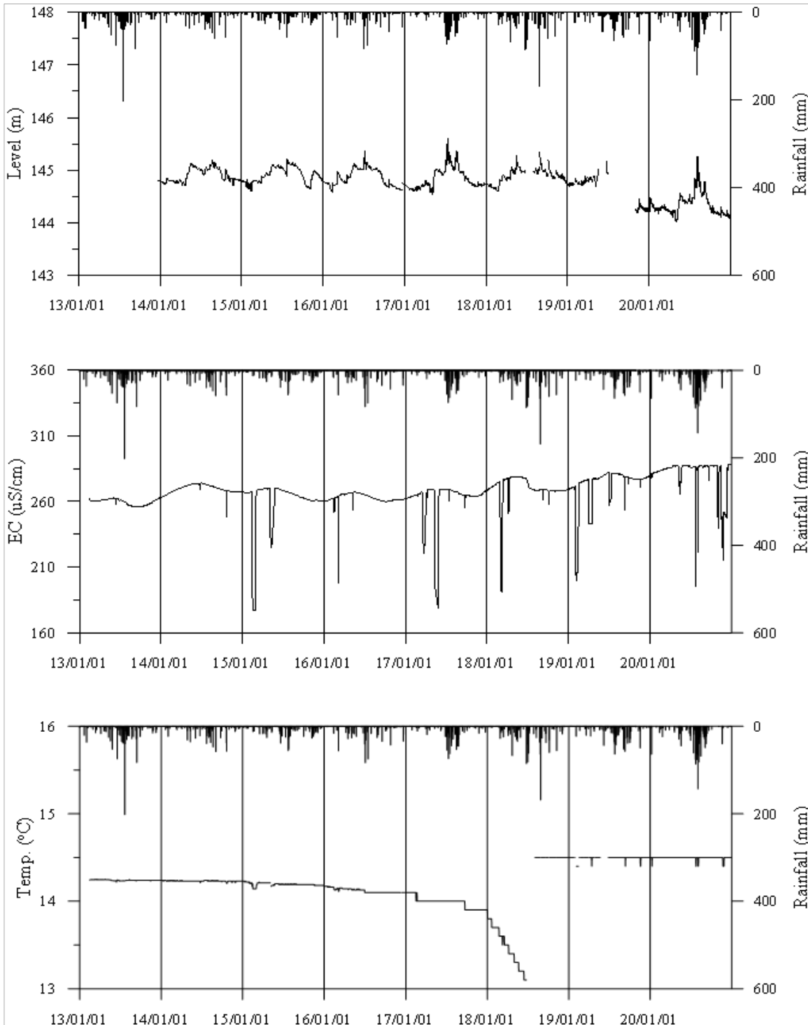
<광주1 관측공의 장기관측자료 (2013.1.1 ~ 2020.12.31)> (a)지하수위, (b)전기전도도, (c)수온
