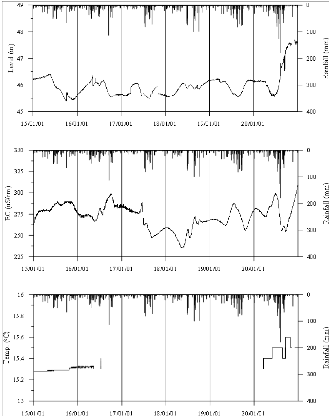
<고창2 관측공의 장기관측자료 (2015.1.1 ~ 2020.12.31)> (a)지하수위, (b)전기전도도, (c)수온
