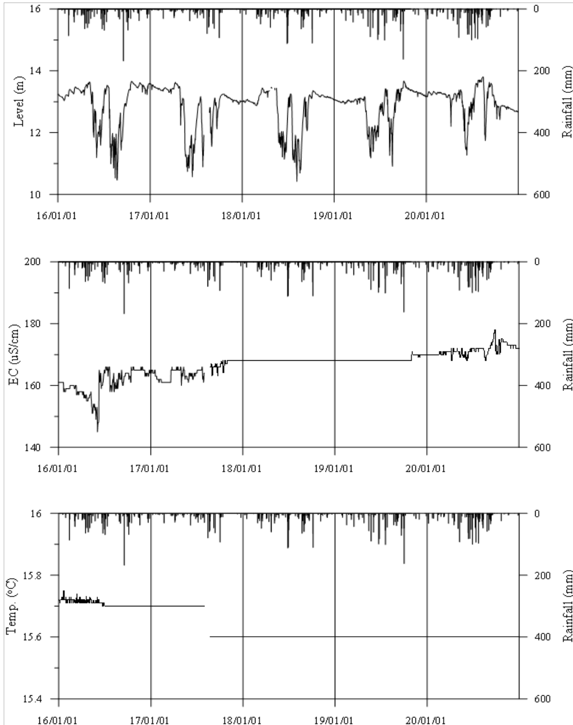
<보성4 관측공의 장기관측자료 (2016.1.1 ~ 2020.12.31)> (a)지하수위, (b)전기전도도, (c)수온
