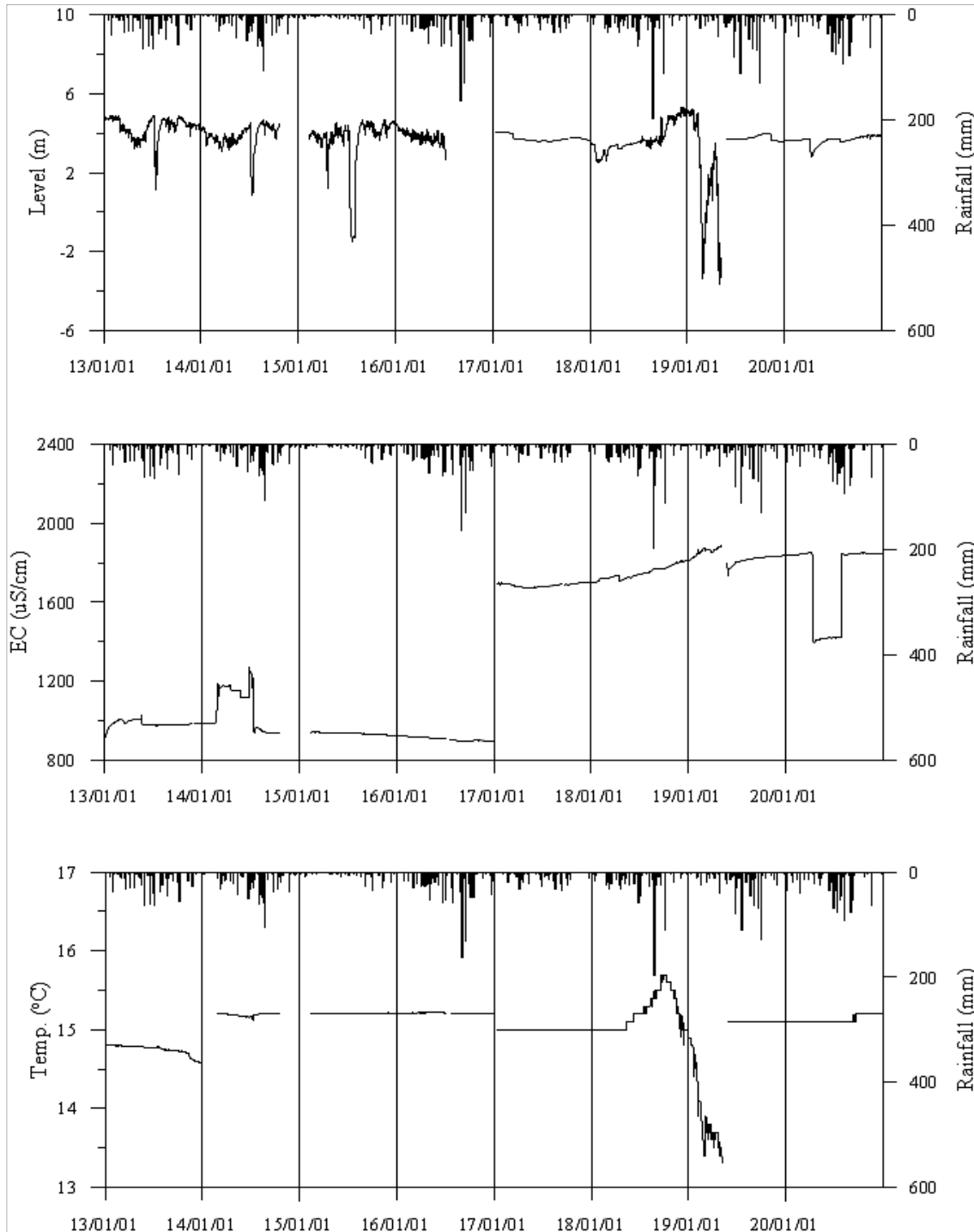
<창녕2 관측공의 장기관측자료 (2013.1.1 ~ 2020.12.31)> (a)지하수위, (b)전기전도도, (c)수온
