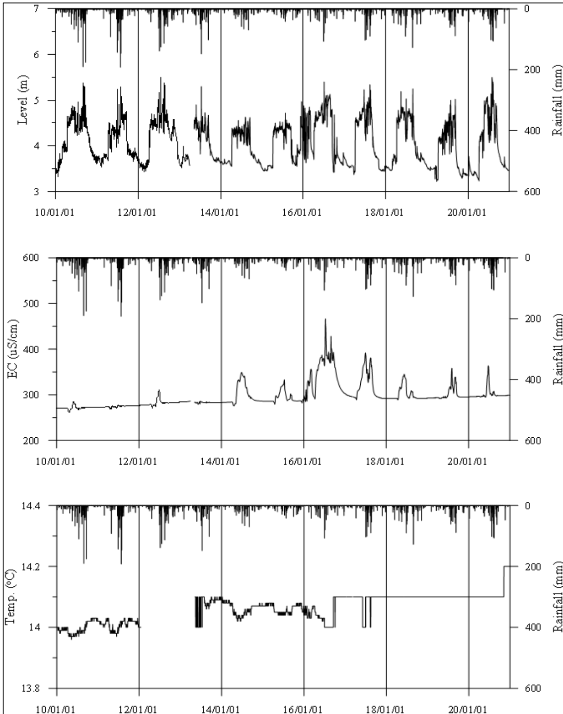
<김포2 관측공의 장기관측자료 (2010.1.1 ~ 2020.12.31)> (a)지하수위, (b)전기전도도, (c)수온
