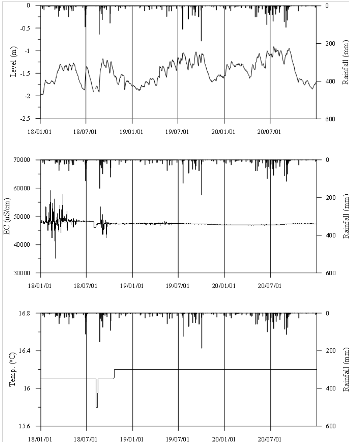
<해남2 관측공의 장기관측자료 (2018.1.1~2020.12.31)> (a)지하수위, (b)전기전도도, (c)수온
