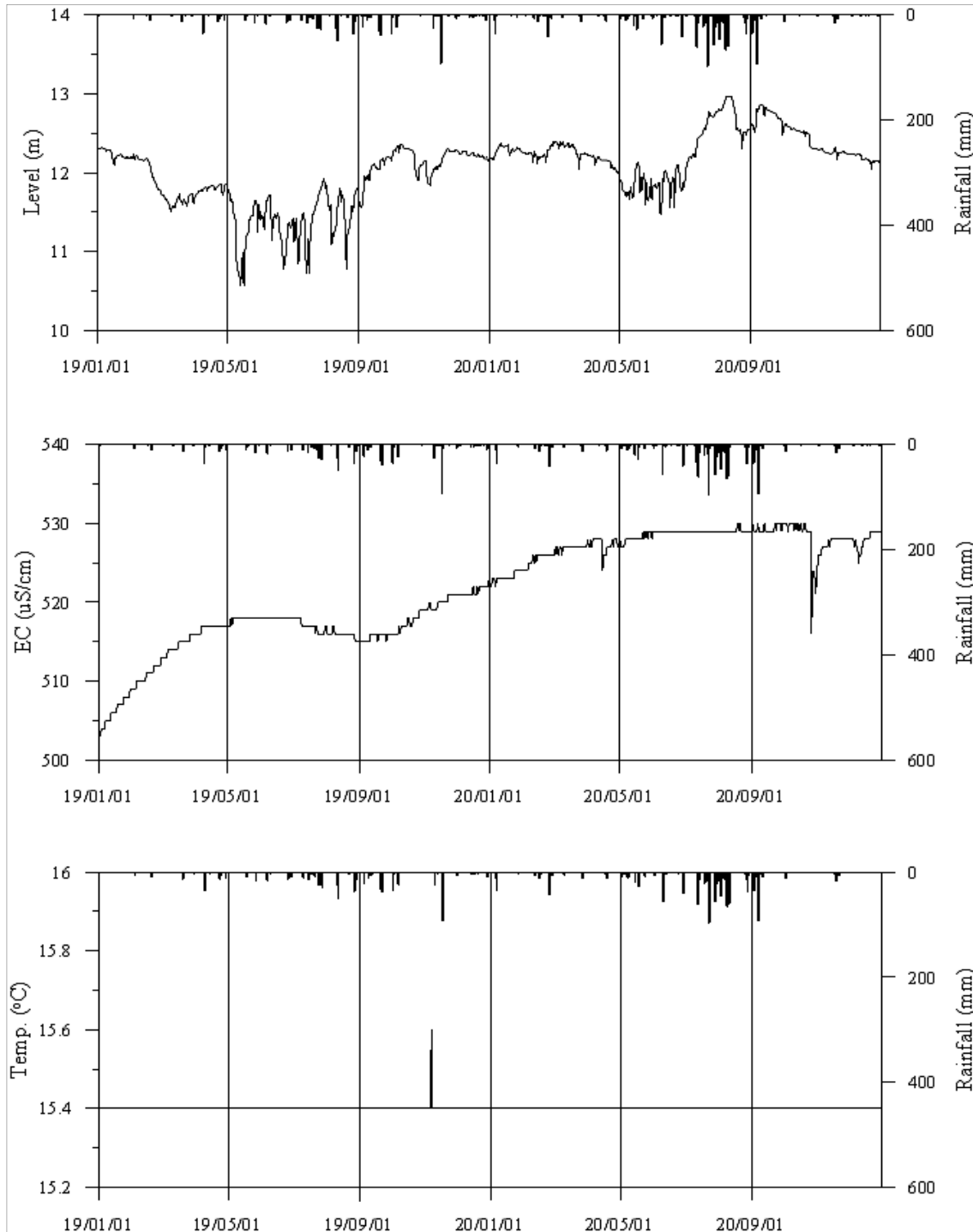
<보령5 관측공의 장기관측자료 (2019.1.1 ~ 2020.12.31)> (a)지하수위, (b)전기전도도, (c)수온
