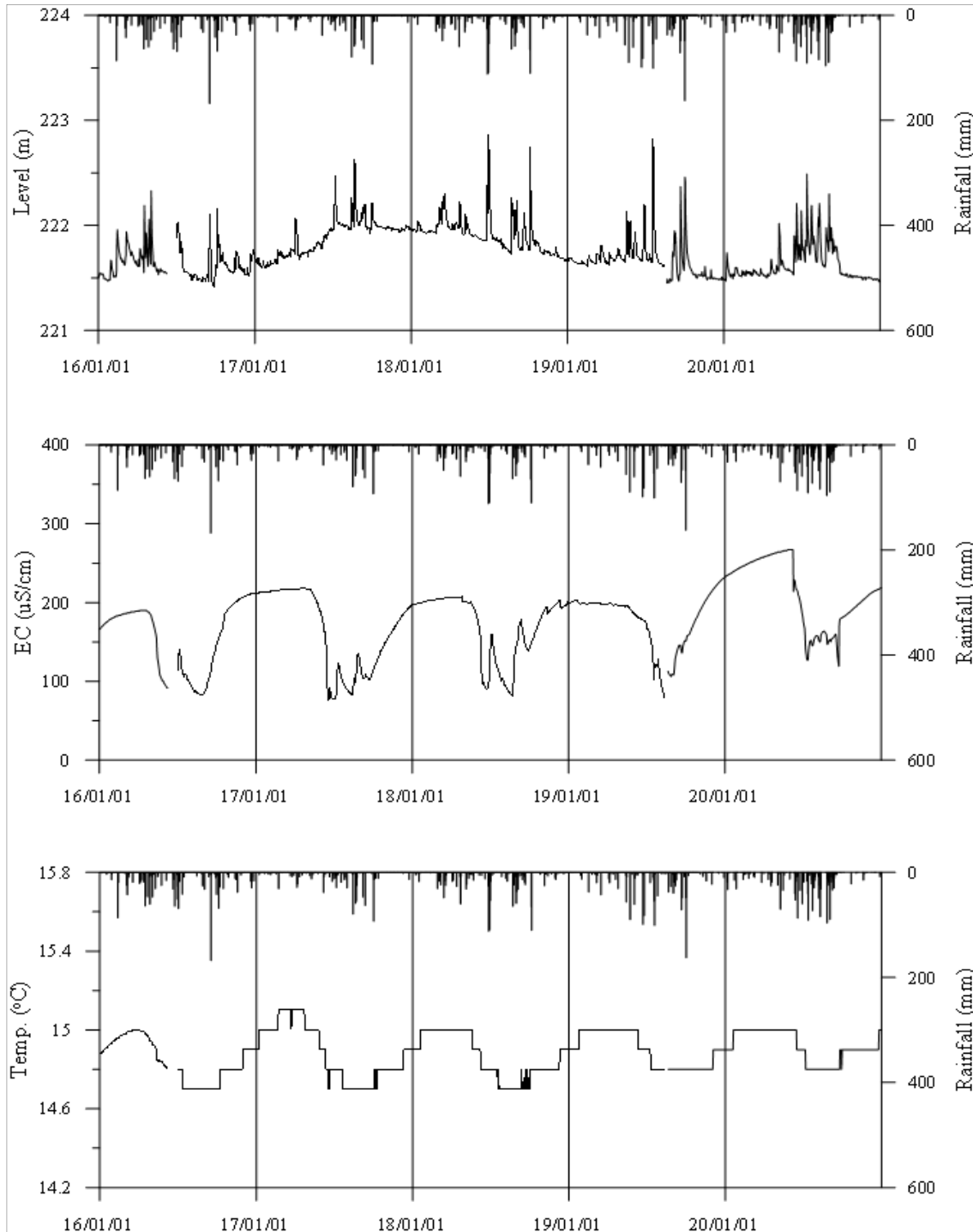
<보성3 관측공의 장기관측자료 (2016.1.1 ~ 2020.12.31)> (a)지하수위, (b)전기전도도, (c)수온
