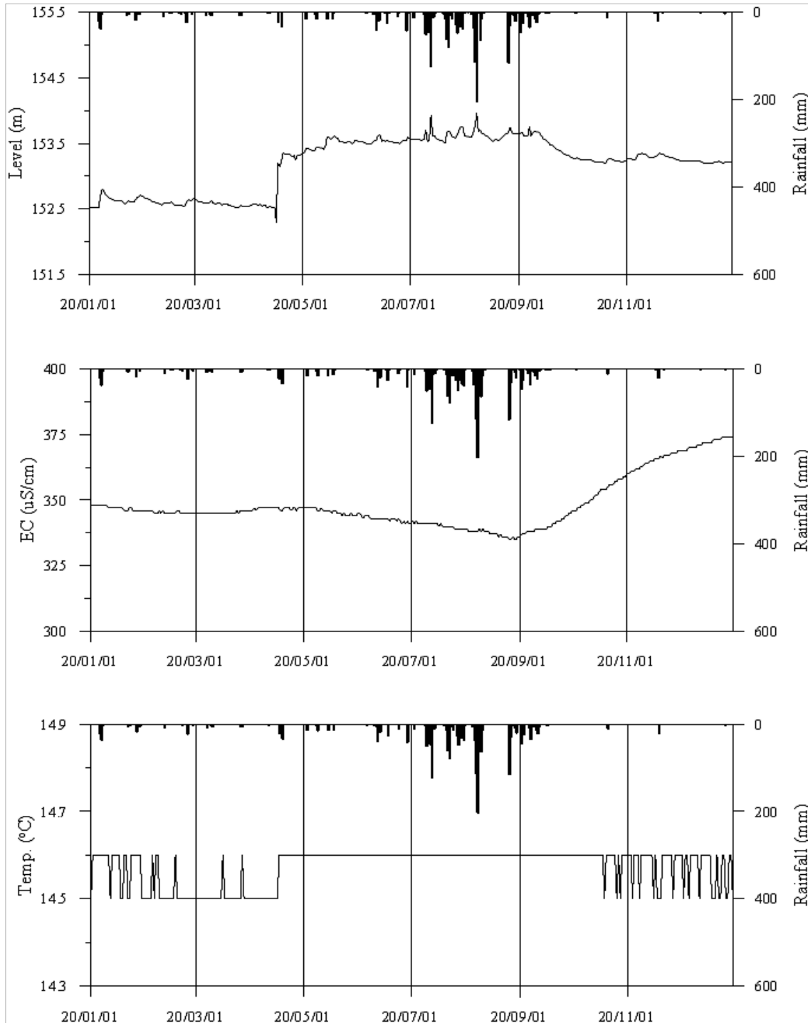
<함양2 관측공의 장기관측자료 (2020.1.1 ~ 2020.12.31)> (a)지하수위, (b)전기전도도, (c)수온
