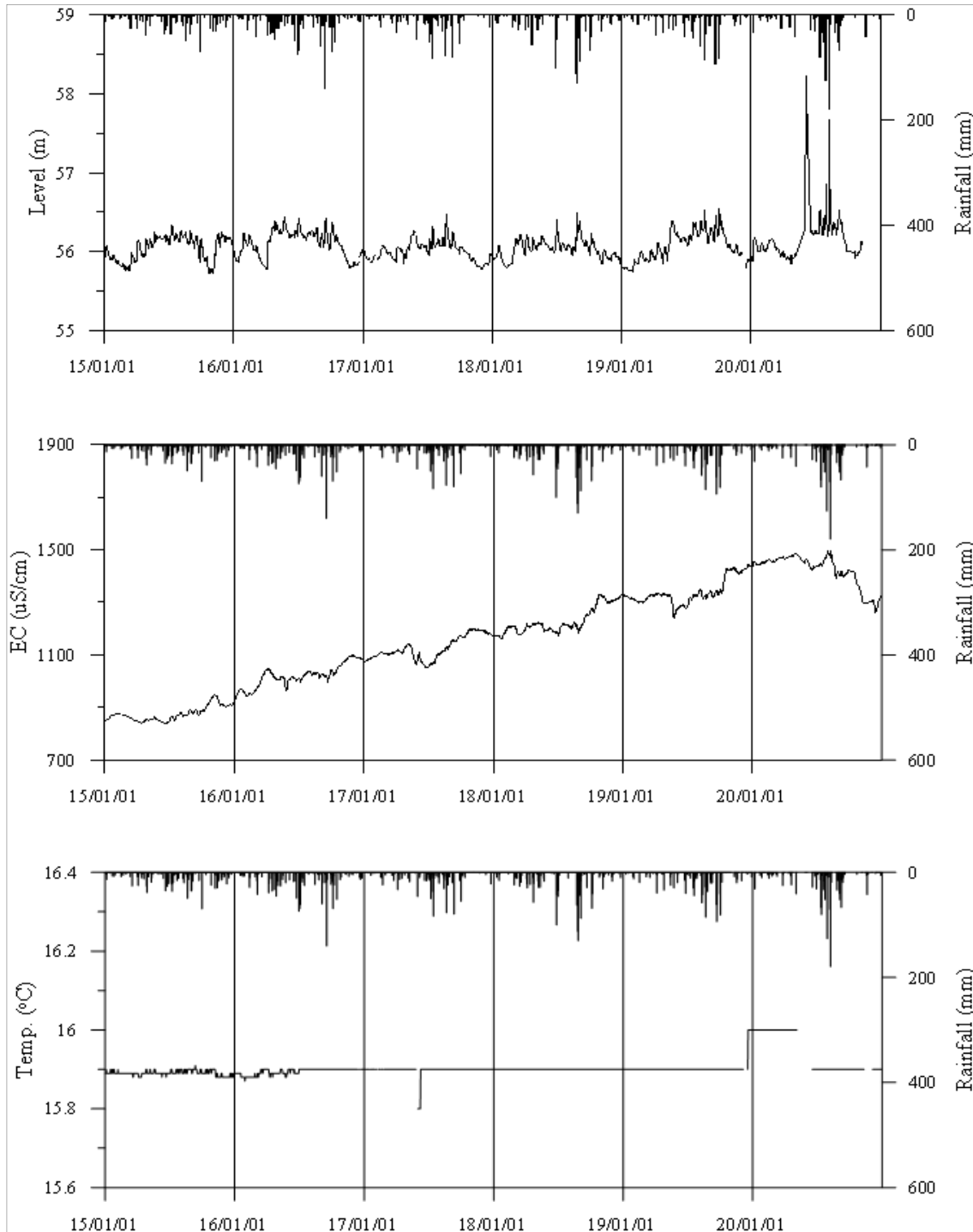
<장성2 관측공의 장기관측자료 (2015.1.1 ~ 2020.12.31)> (a)지하수위, (b)전기전도도, (c)수온
