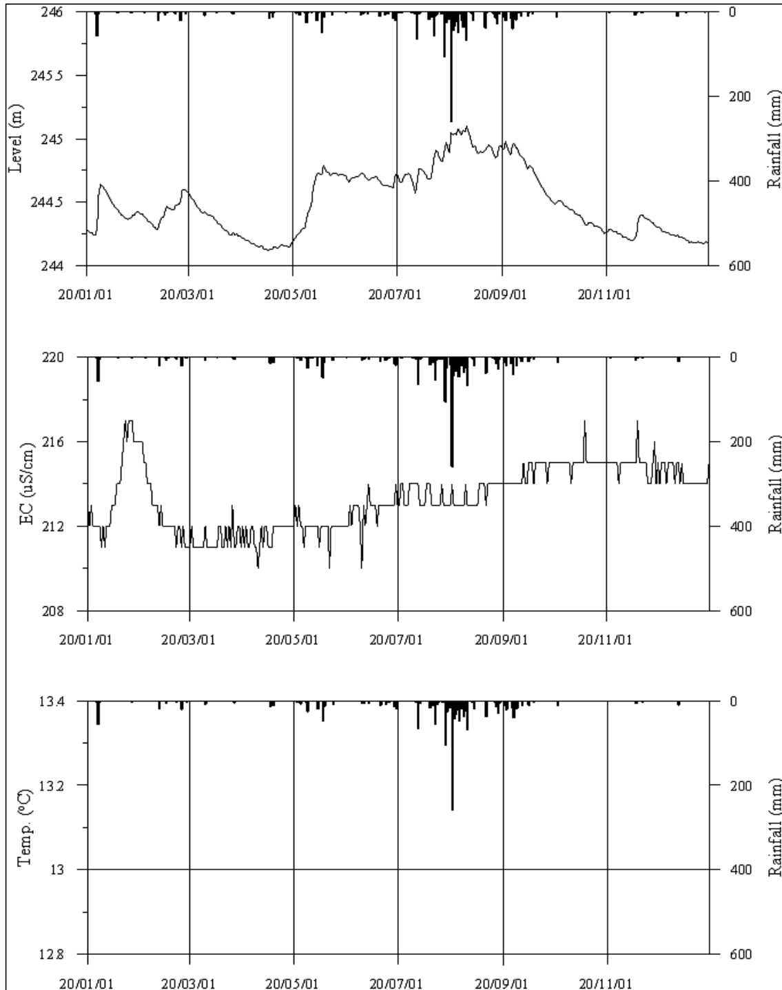
<제천4 관측공의 장기관측자료 (2020.1.1 ~ 2020.12.31)> (a)지하수위, (b)전기전도도, (c)수온
