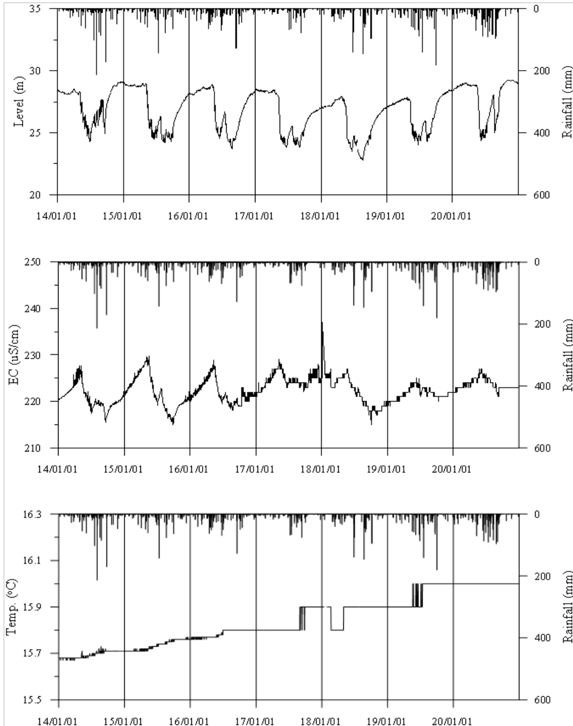
<장흥2 관측공의 장기관측자료 (2014.1.1 ~ 2020.12.31)> (a)지하수위, (b)전기전도도, (c)수온
