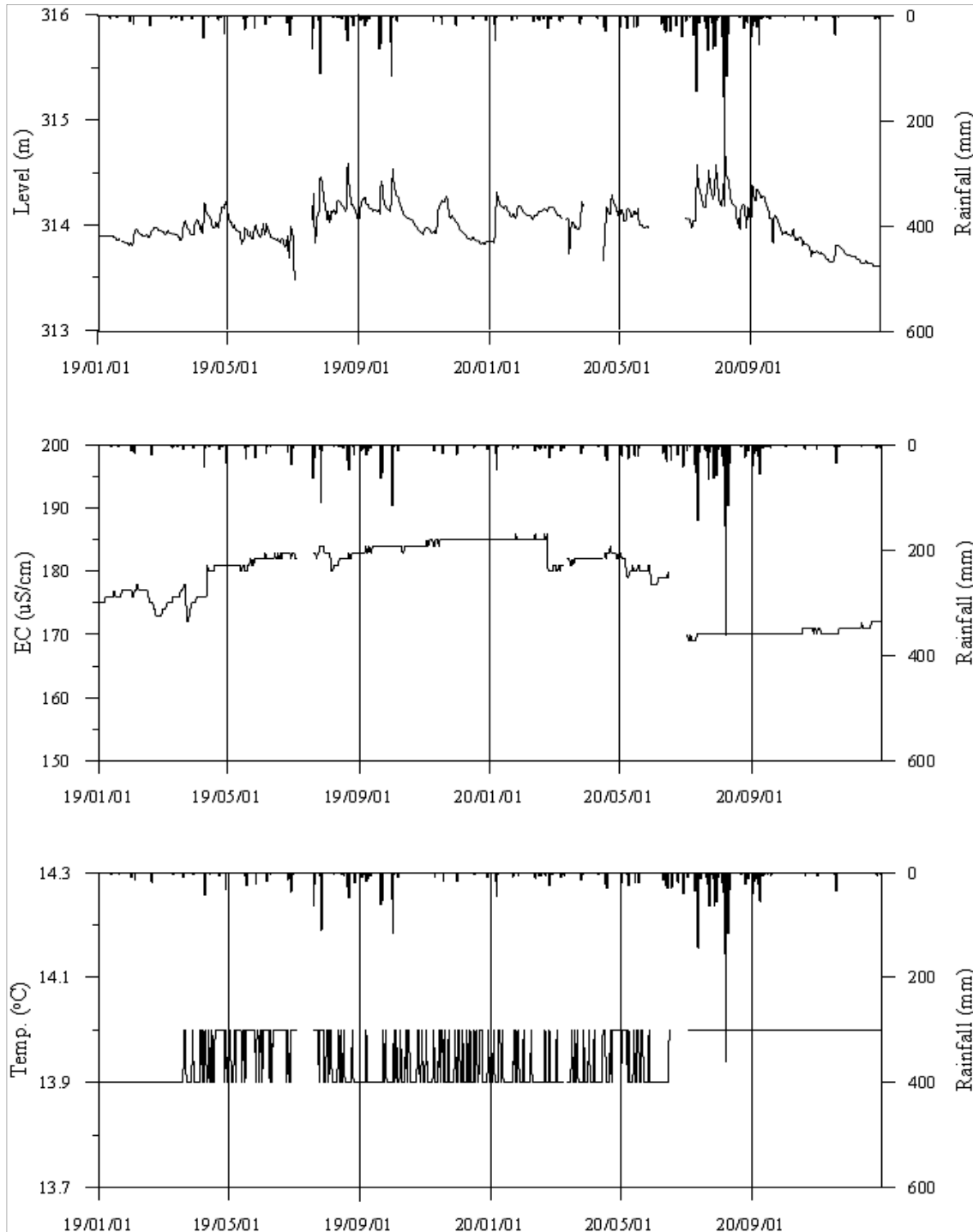
<순창4 관측공의 장기관측자료 (2019.1.1 ~ 2020.12.31)> (a)지하수위, (b)전기전도도, (c)수온
