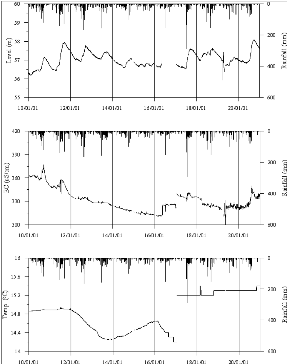
<증평1 관측공의 장기관측자료 (2010.1.1 ~ 2020.12.31)> (a)지하수위, (b)전기전도도, (c)수온
