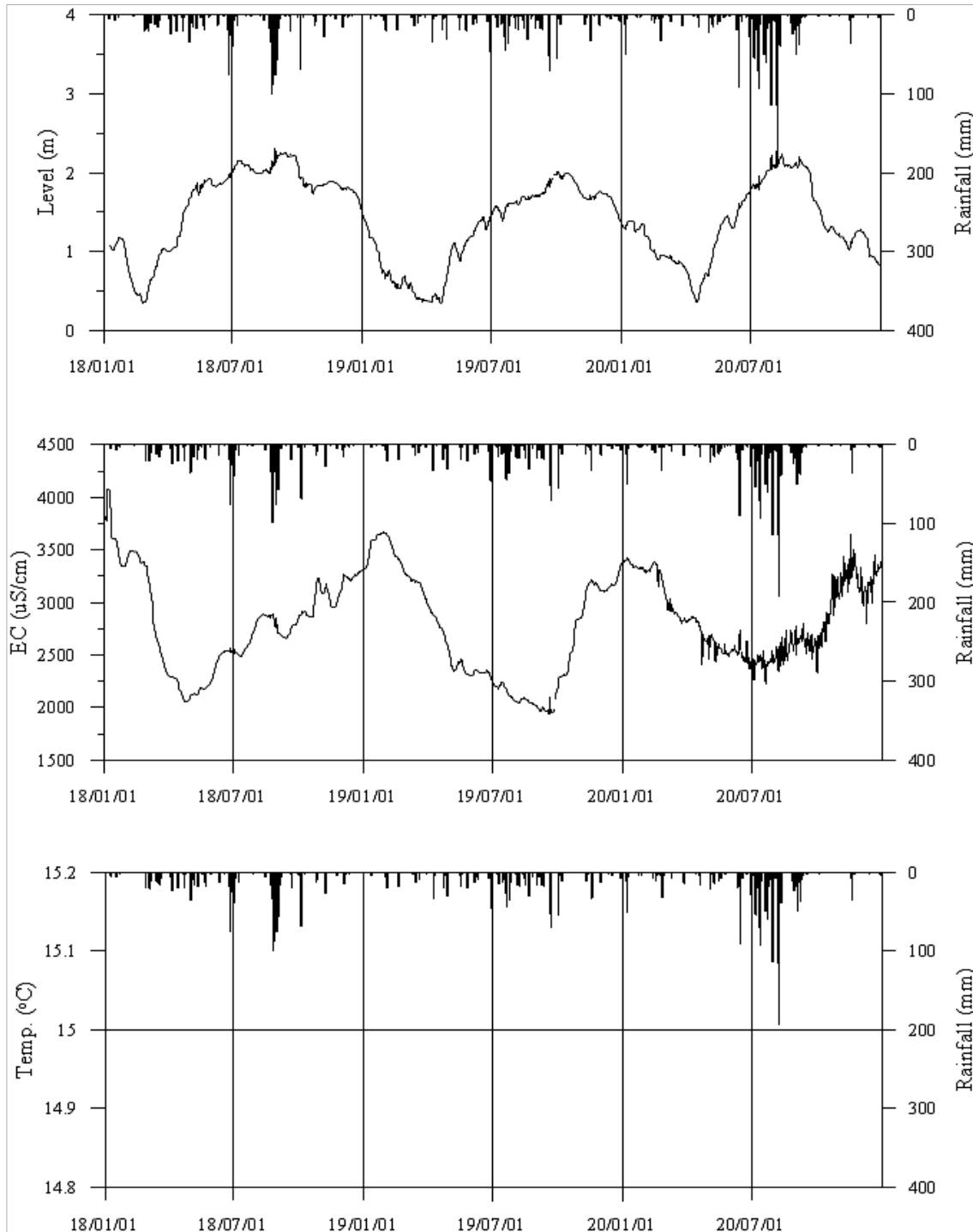
<익산3 관측공의 장기관측자료 (2018.1.1 ~ 2020.12.31)> (a)지하수위, (b)전기전도도, (c)수온
