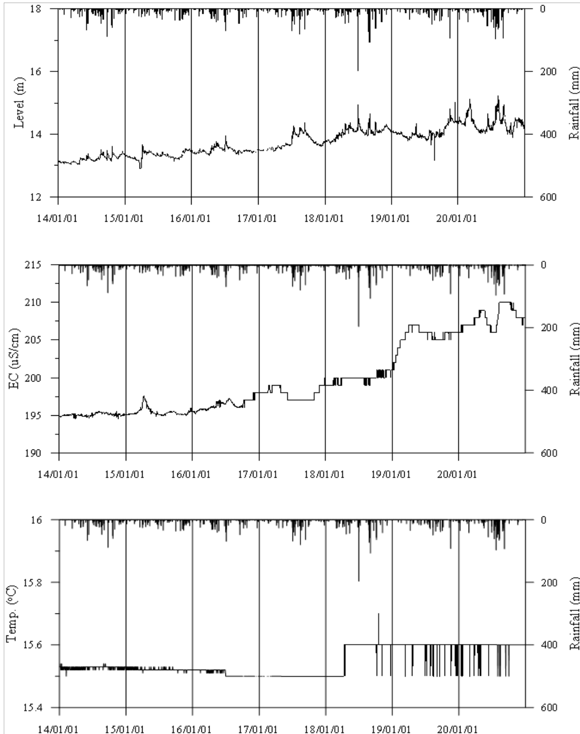
<보령2 관측공의 장기관측자료 (2014.1.1 ~ 2020.12.31)> (a)지하수위, (b)전기전도도, (c)수온
