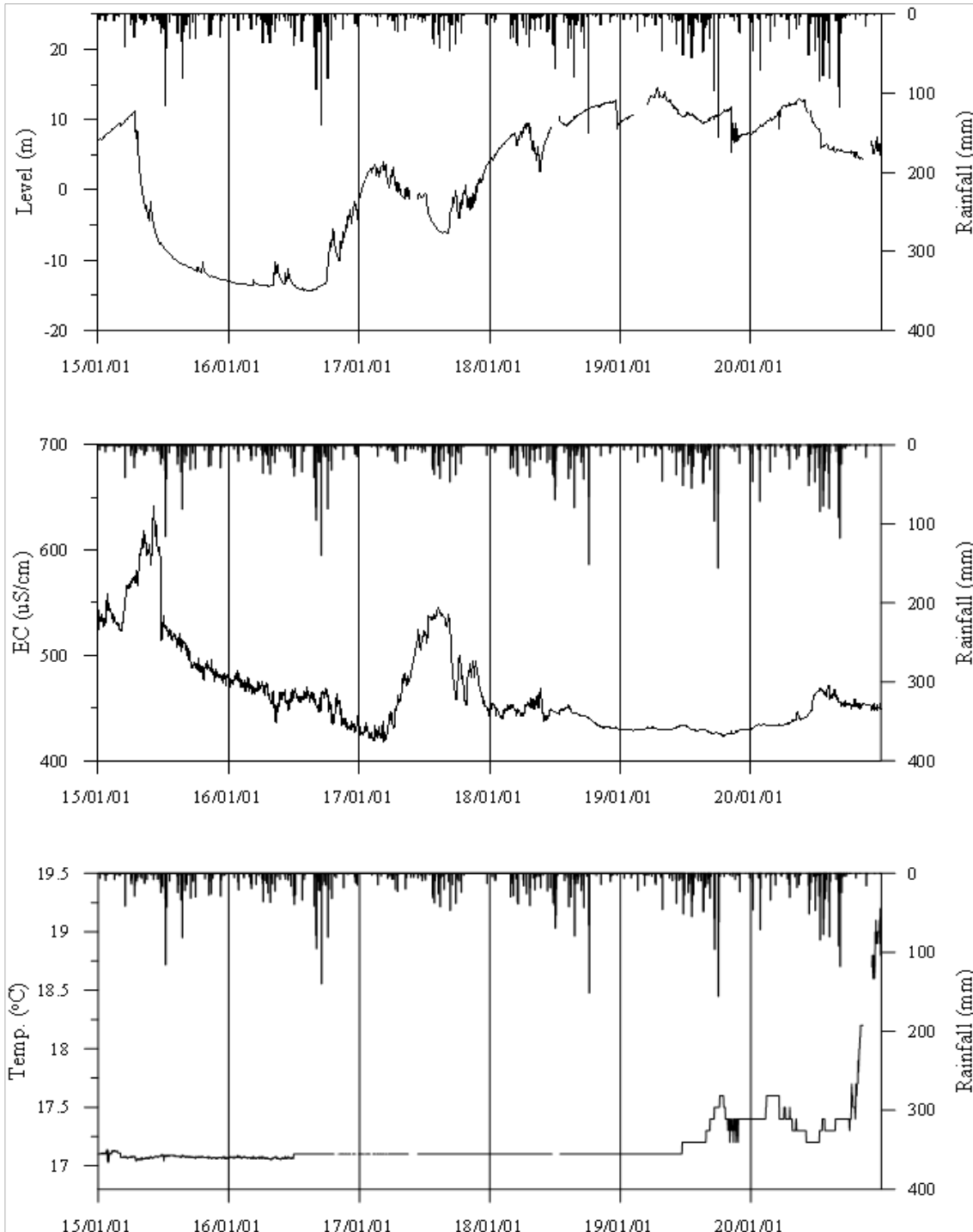
<경주1 관측공의 장기관측자료 (2015.1.1 ~ 2020.12.31)> (a)지하수위, (b)전기전도도, (c)수온
