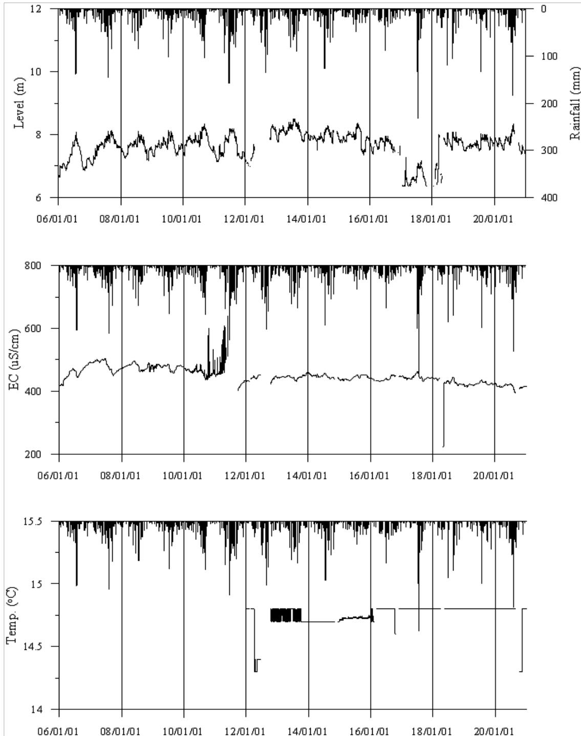
<아산2 관측공의 장기관측자료 (2006.1.1 ~ 2020.12.31)> (a)지하수위, (b)전기전도도, (c)수온
