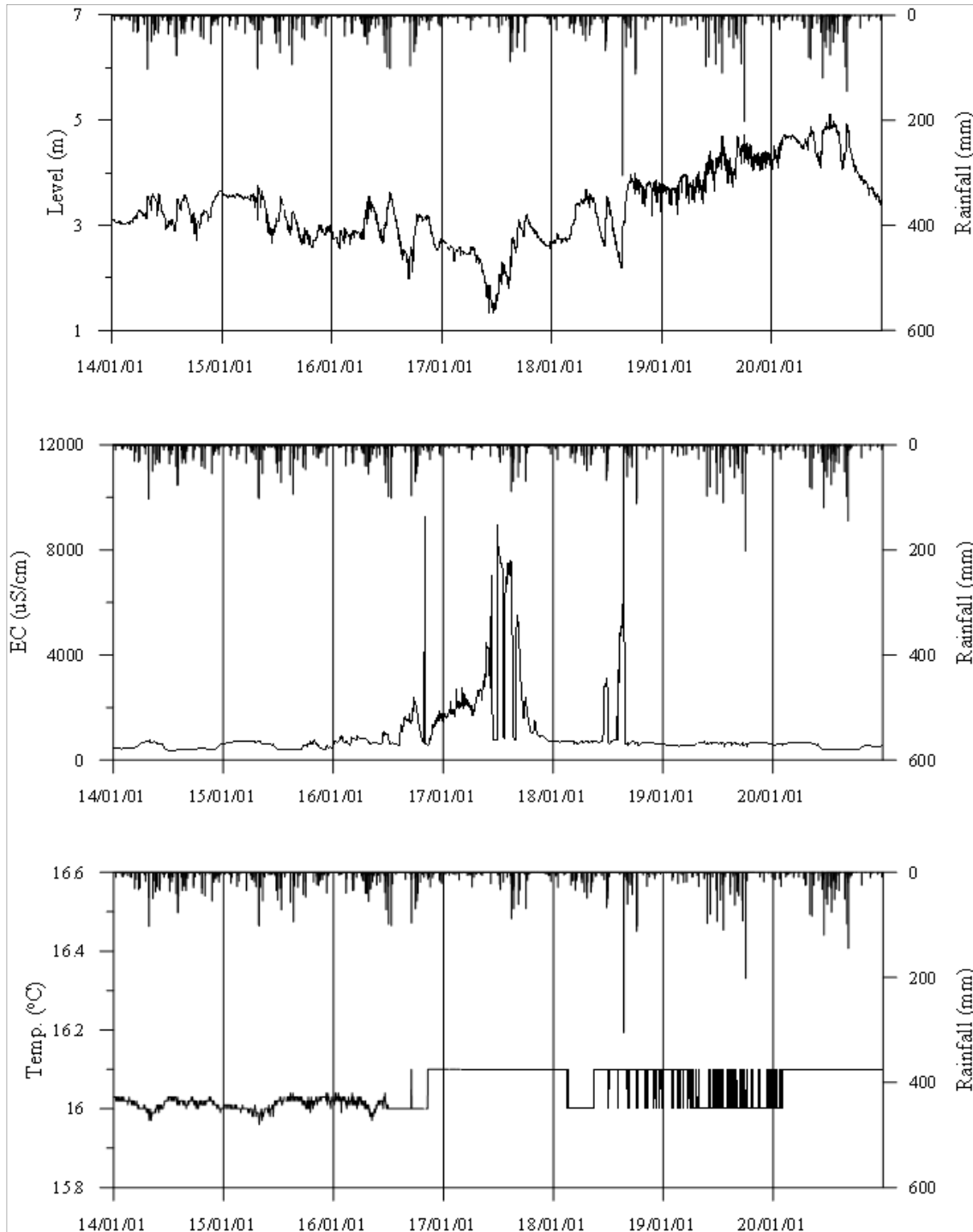
<진도2 관측공의 장기관측자료 (2014.1.1.~2020.12.31)> (a)지하수위, (b)전기전도도, (c)수온
