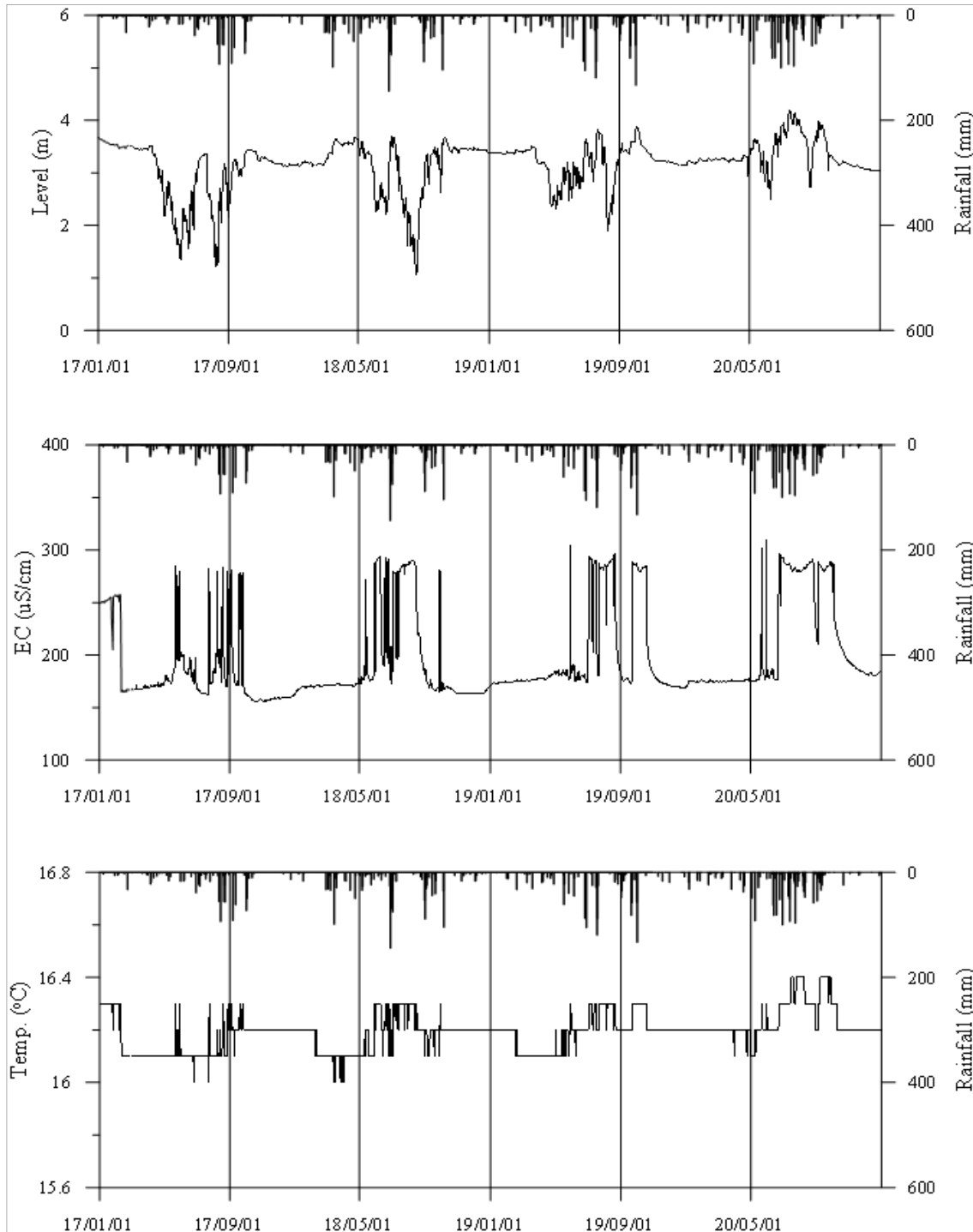
<고흥4 관측공의 장기관측자료 (2017.1.1~2020.12.31)> (a)지하수위, (b)전기전도도, (c)수온
