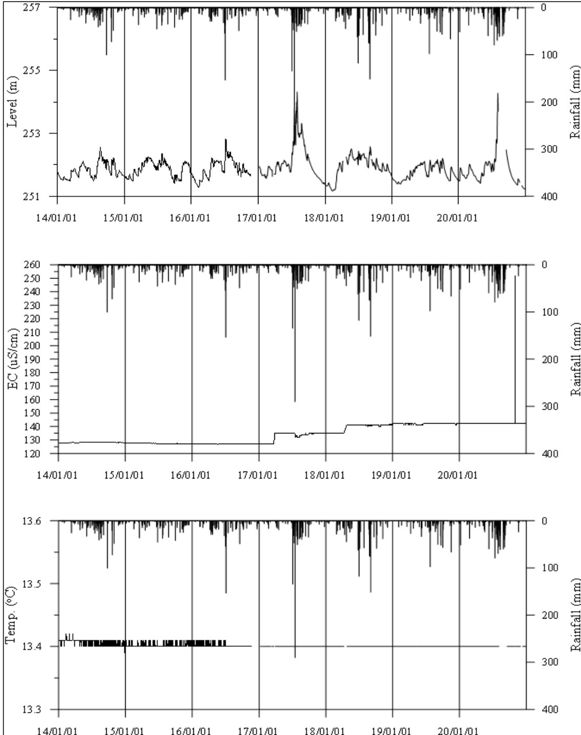
<청원1 관측공의 장기관측자료 (2014.1.1 ~ 2020.12.31)> (a)지하수위, (b)전기전도도, (c)수온
