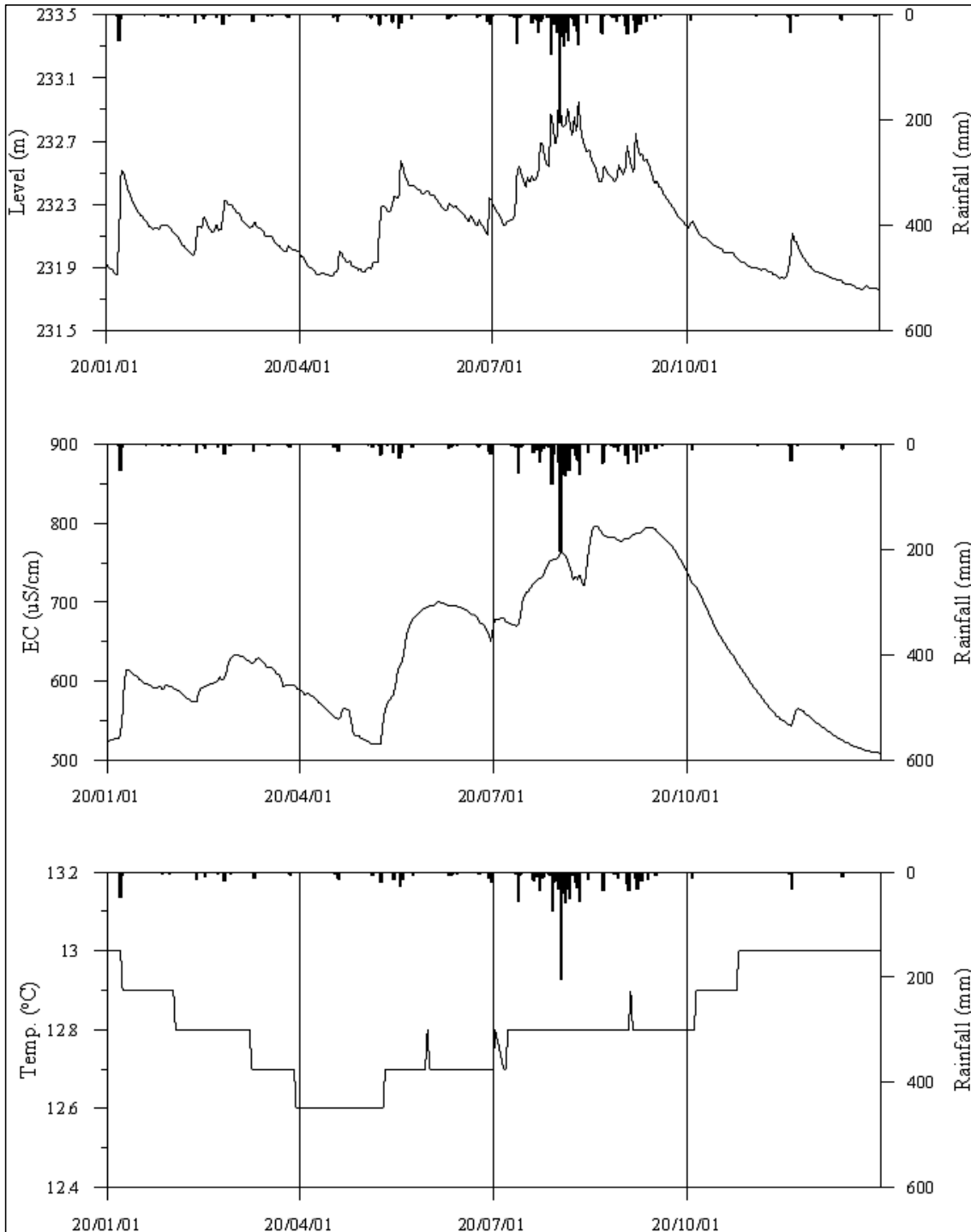
<영월2 관측공의 장기관측자료 (2020.1.1 ~ 2020.12.31)> (a)지하수위, (b)전기전도도, (c)수온
