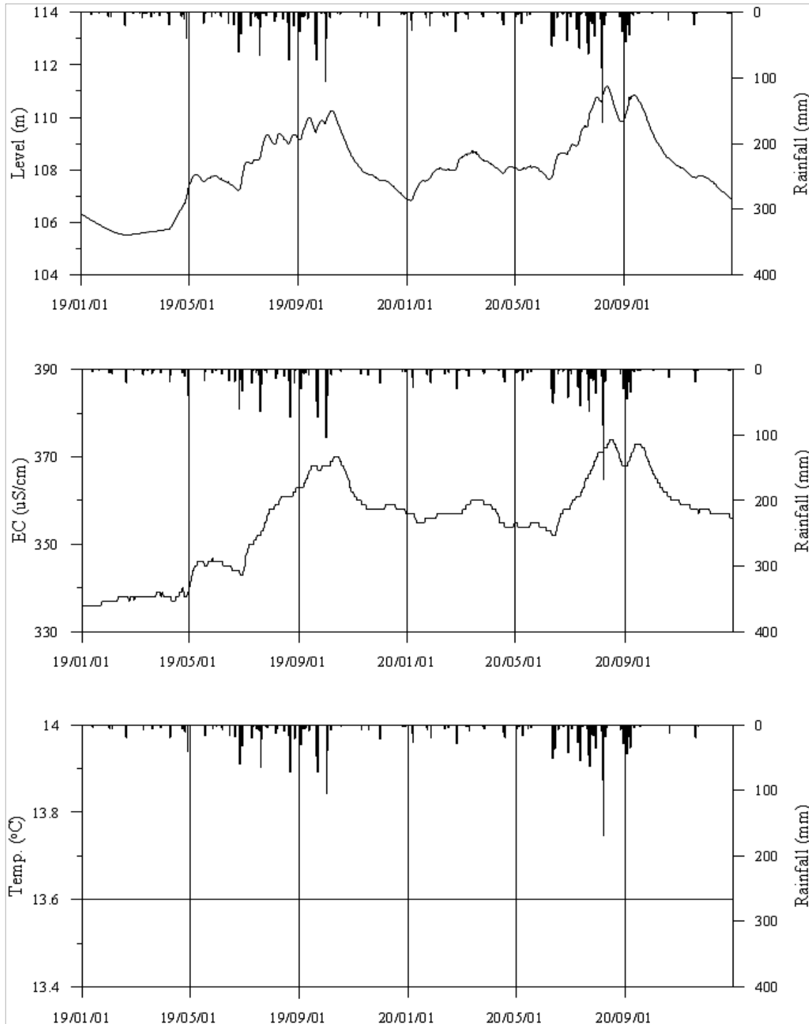
<칠곡3 관측공의 장기관측자료 (2019.1.1 ~ 2020.12.31.)> (a)지하수위, (b)전기전도도, (c)수온
