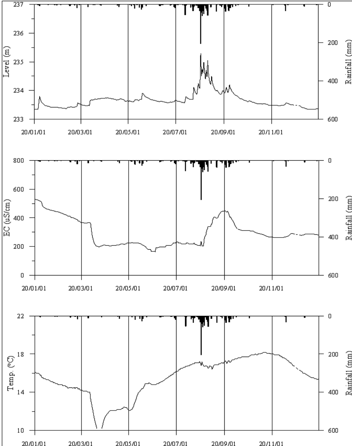
<영월1 관측공의 장기관측자료 (2020.1.1 ~ 2020.12.31)> (a)지하수위, (b)전기전도도, (c)수온
