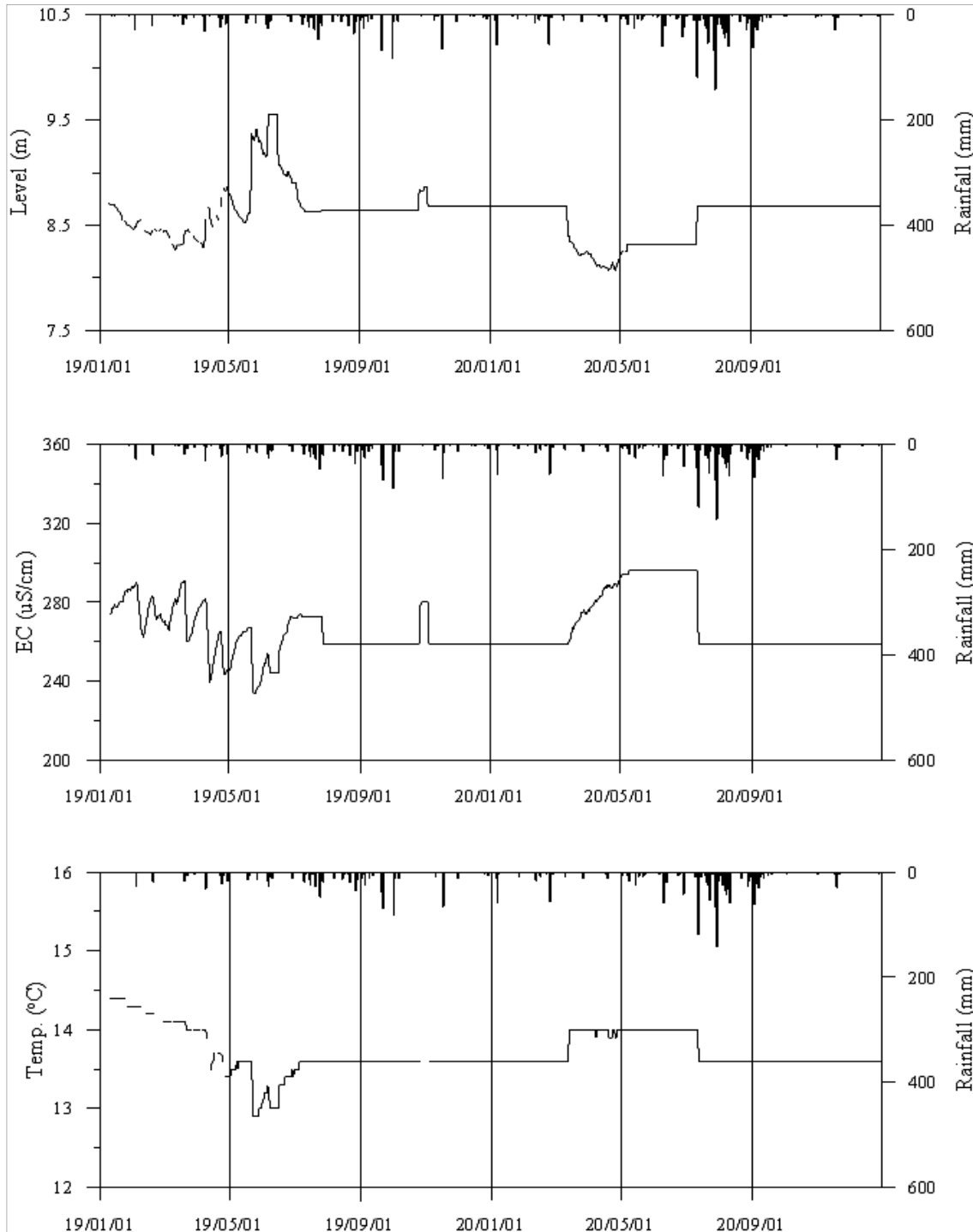
<공주4 관측공의 장기관측자료 (2019.1.1 ~ 2020.12.31)> (a)지하수위, (b)전기전도도, (c)수온
