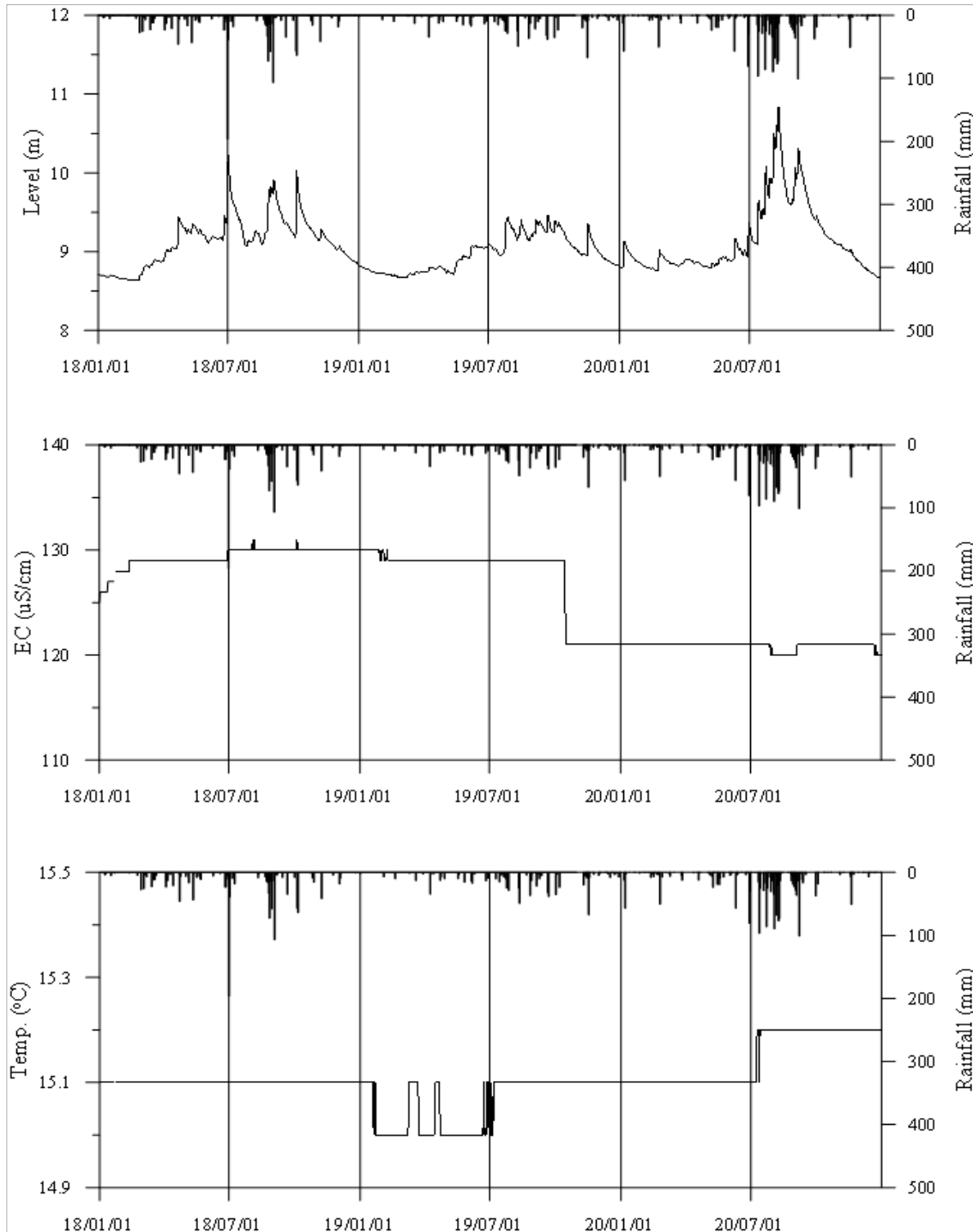
<홍성3 관측공의 장기관측자료 (2018.1.1 ~ 2020.12.31)> (a)지하수위, (b)전기전도도, (c)수온
