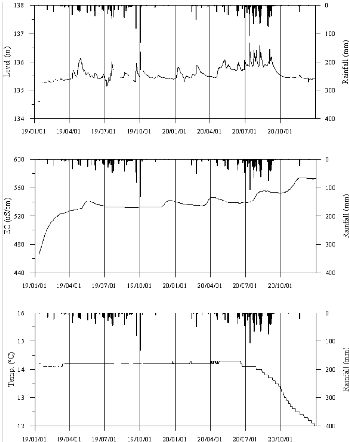
<상주7 관측공의 장기관측자료 (2019.1.1 ~ 2020.12.31)> (a)지하수위, (b)전기전도도, (c)수온
