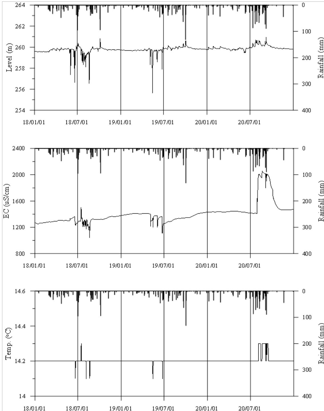
<청송3 관측공의 장기관측자료 (2018.1.1 ~ 2020.12.31)> (a)지하수위, (b)전기전도도, (c)수온
