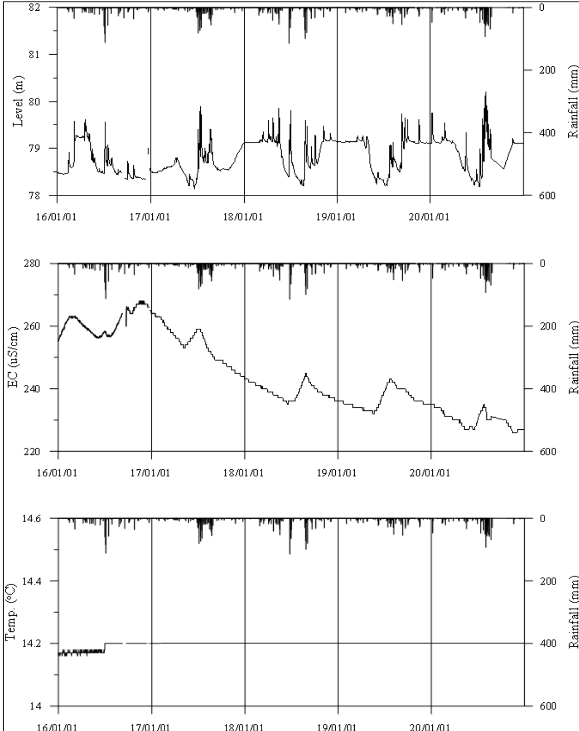
<원주1(신) 관측공의 장기관측자료 (2016.1.1 ~ 2020.12.31)> (a)지하수위, (b)전기전도도, (c)수온
