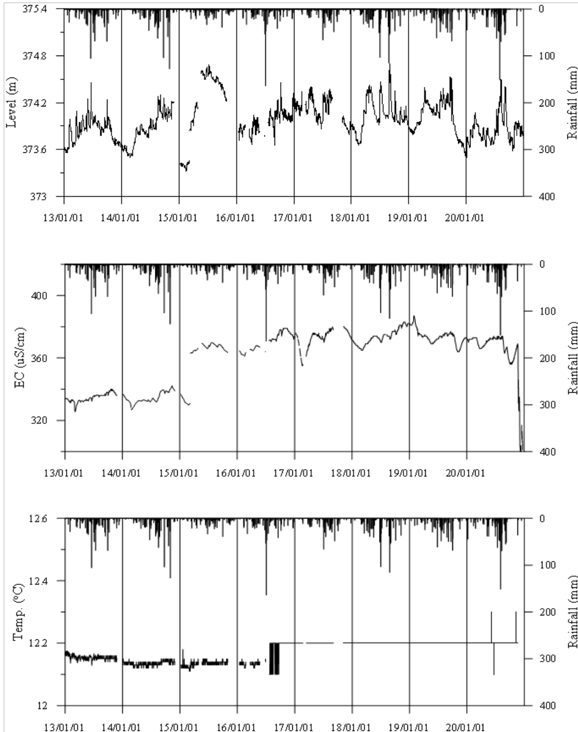
<봉화2 관측공의 장기관측자료 (2013.1.1 ~ 2020.12.31)> (a)지하수위, (b)전기전도도, (c)수온
