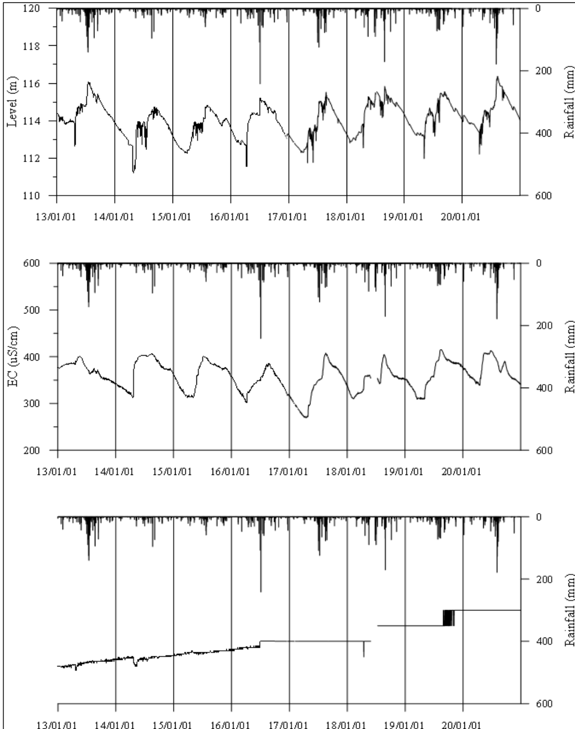
<가평1 관측공의 장기관측자료 (2013.1.1 ~ 2020.12.31)> (a)지하수위, (b)전기전도도, (c)수온
