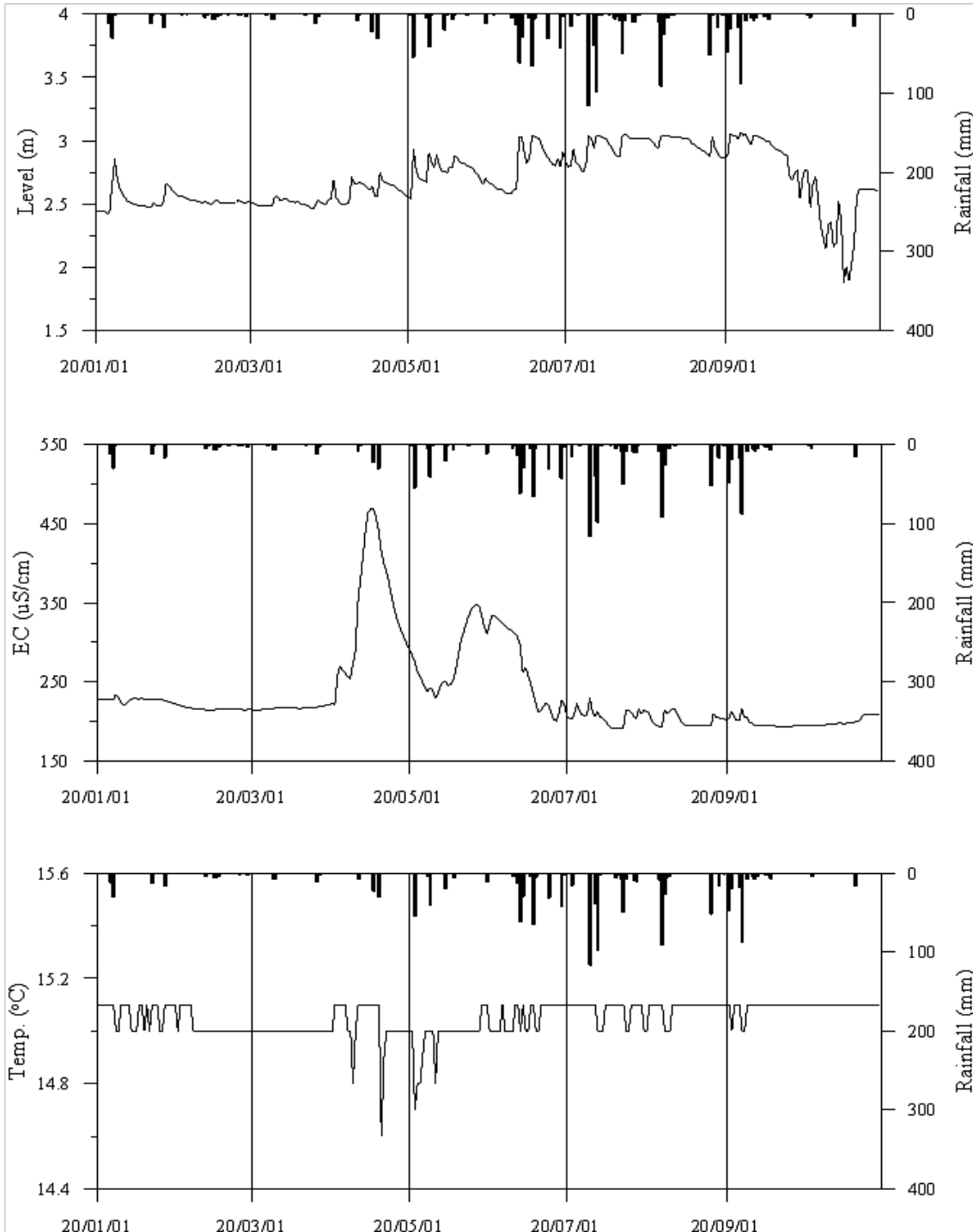
<영암1 관측공의 장기관측자료 (2020.1.1~2020.10.31)> (a)지하수위, (b)전기전도도, (c)수온
