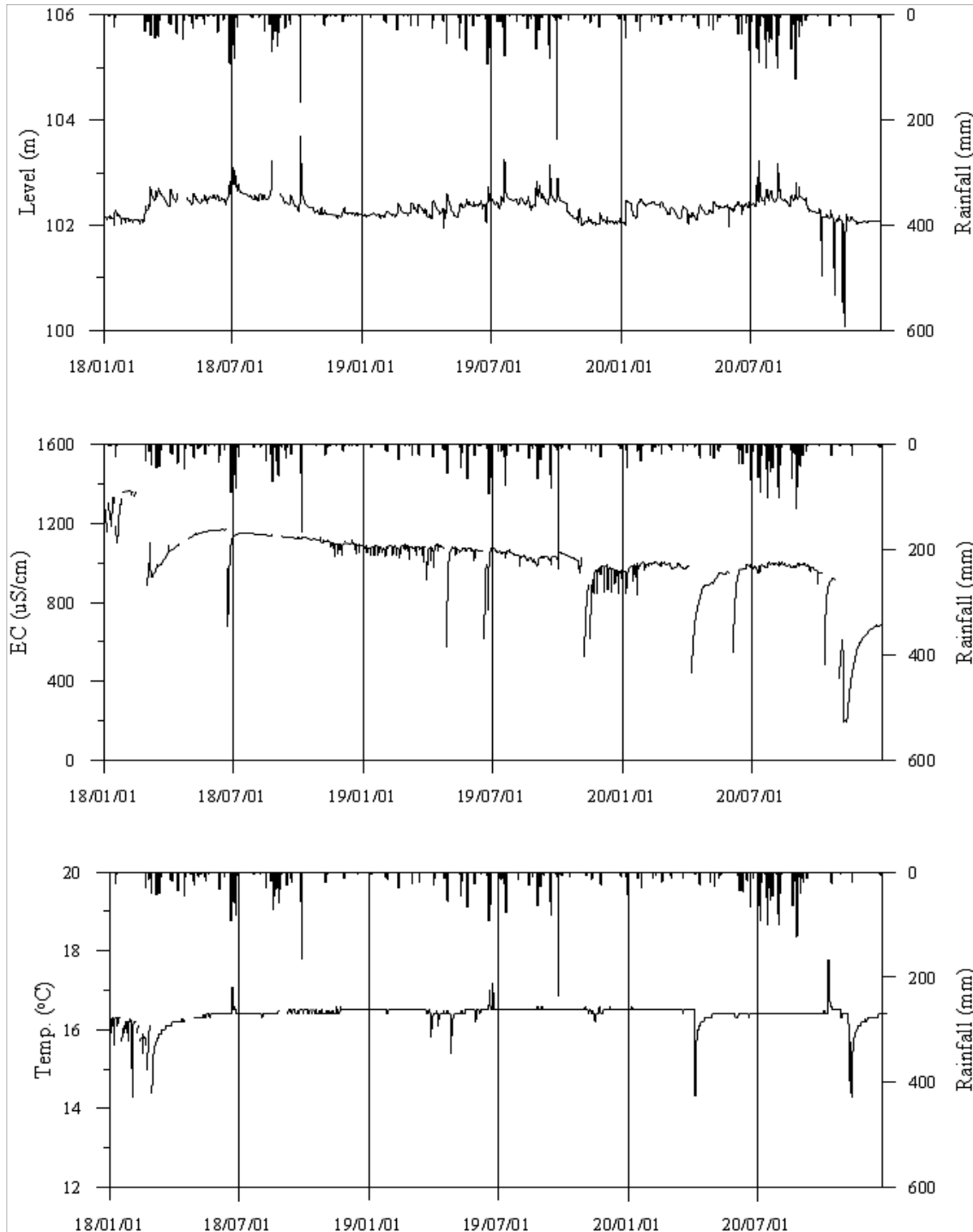
<의령3 관측공의 장기관측자료 (2018.1.1 ~ 2020.12.31)> (a)지하수위, (b)전기전도도, (c)수온
