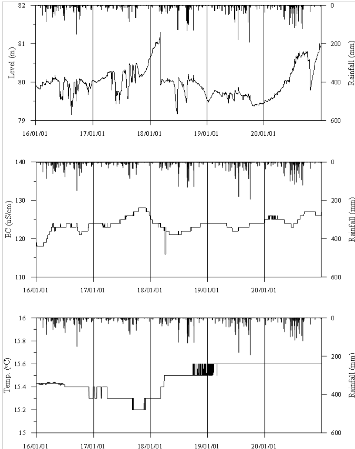
<순천3 관측공의 장기관측자료 (2016.1.1~2020.12.31)> (a)지하수위, (b)전기전도도, (c)수온
