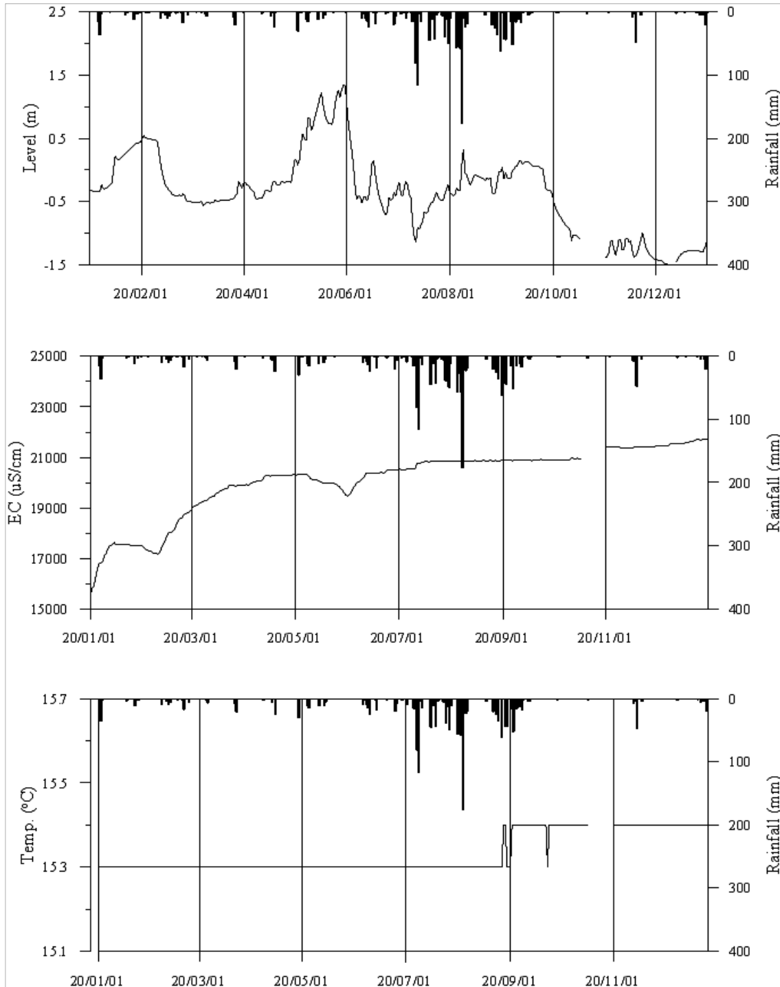
<정읍7 관측공의 장기관측자료 (2020.1.1 ~ 2020.12.31)> (a)지하수위, (b)전기전도도, (c)수온
