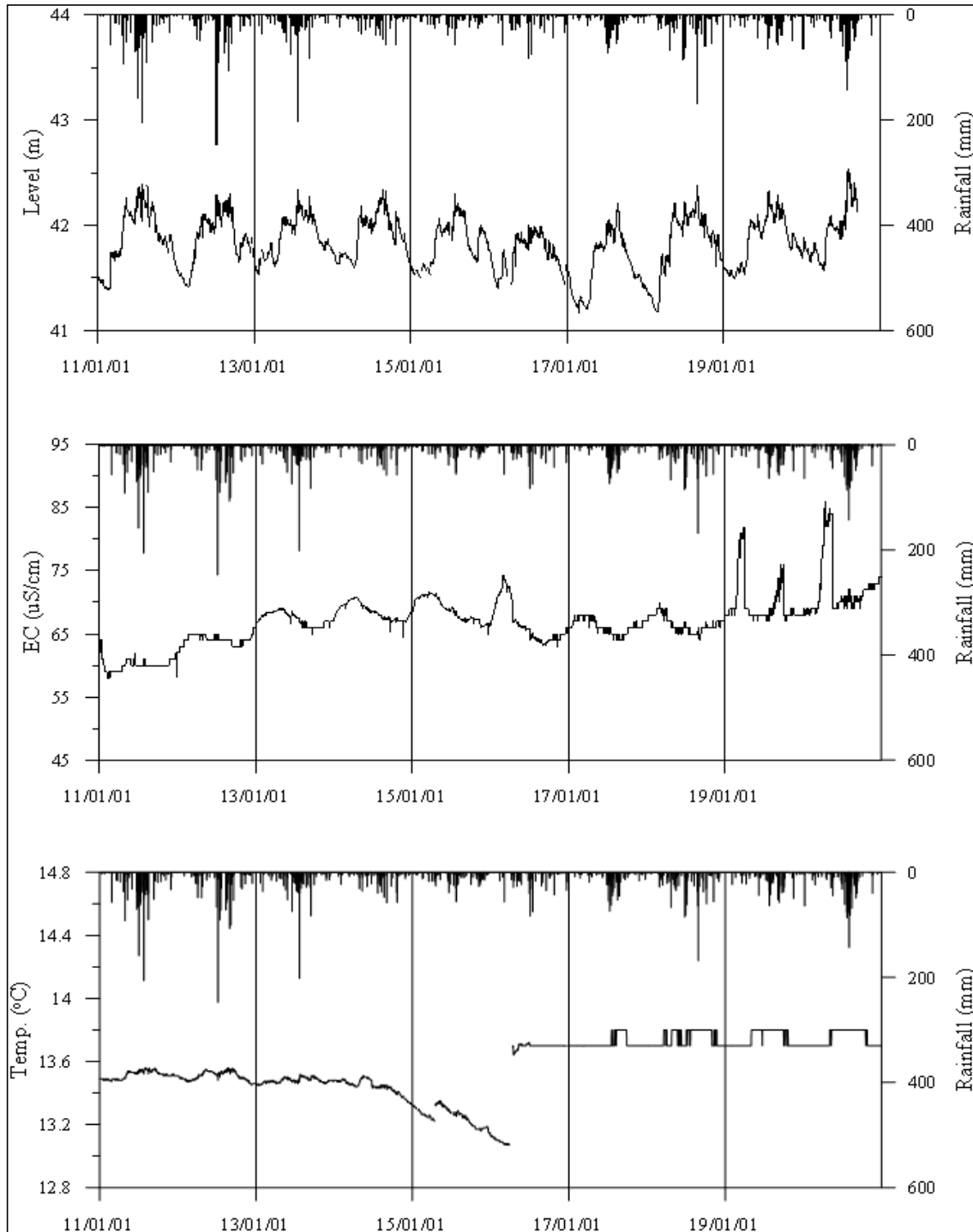
<여주2 관측공의 장기관측자료 (2011.1.1. ~ 2020.12.31)> (a)지하수위, (b)전기전도도, (c)수온
