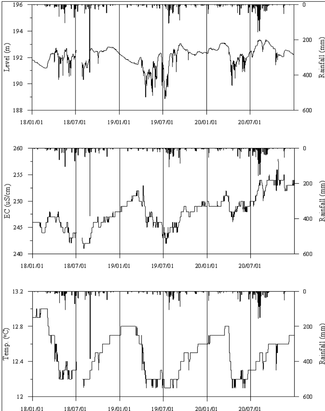
<철원1 관측공의 장기관측자료 (2018.1.1 ~ 2020.12.31)> (a)지하수위, (b)전기전도도, (c)수온
