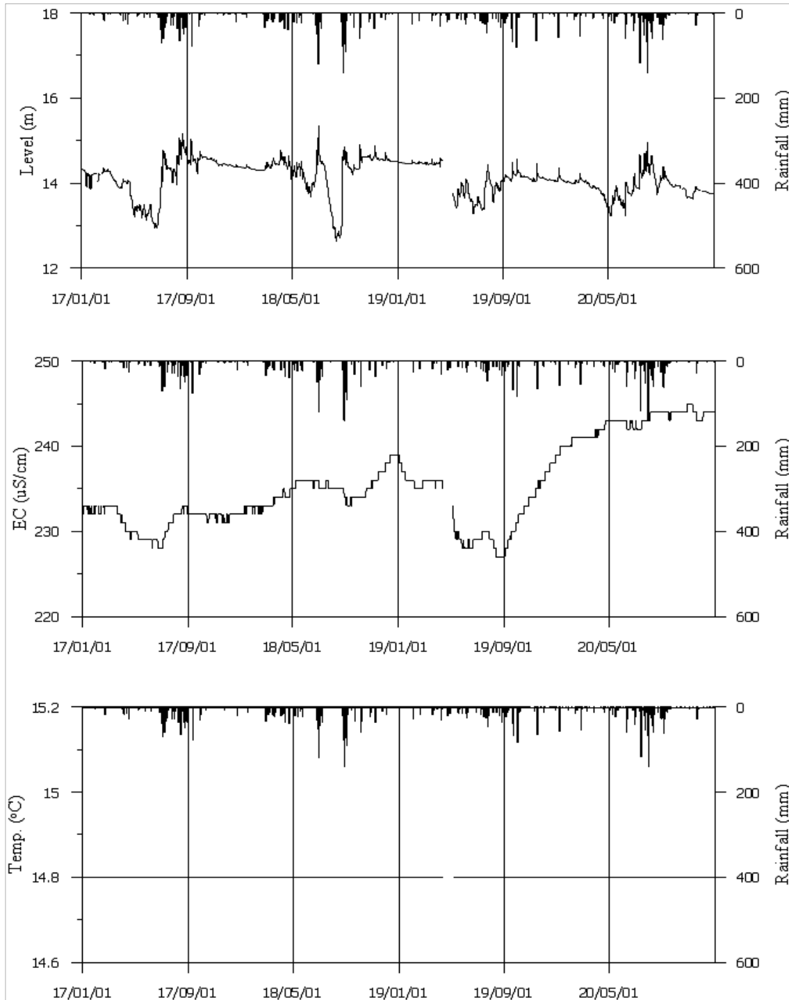
<공주2 관측공의 장기관측자료 (2017.1.1 ~ 2020.12.31)> (a)지하수위, (b)전기전도도, (c)수온
