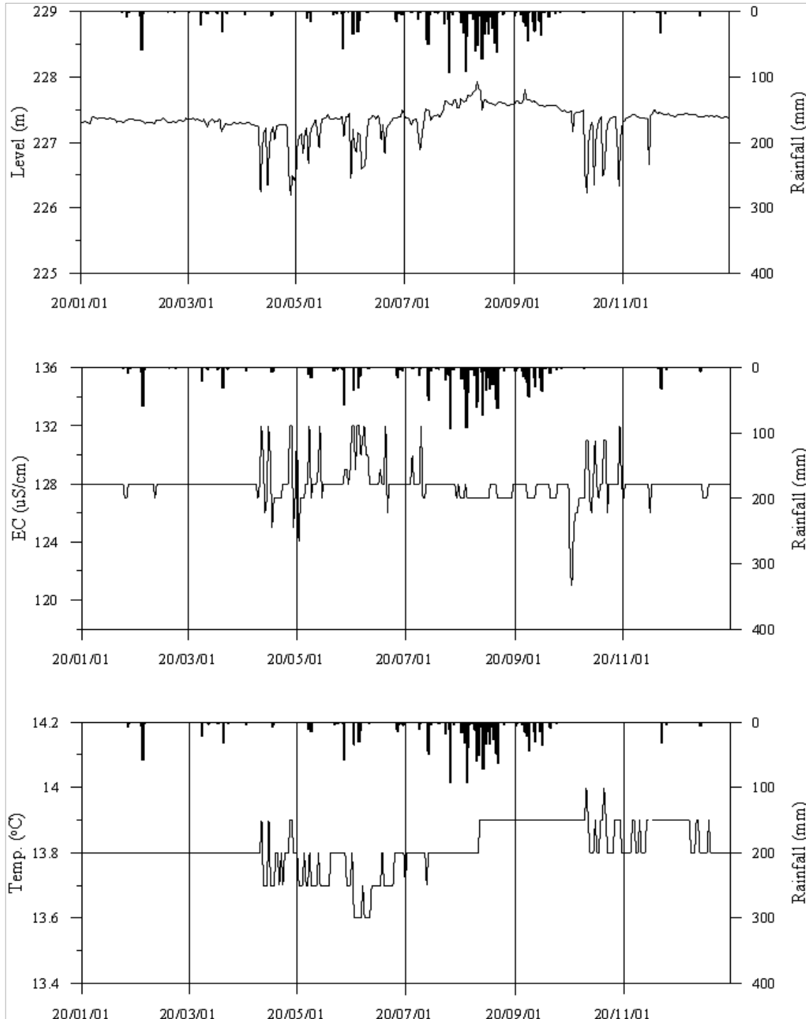
<영주1 관측공의 장기관측자료 (2020.1.1 ~ 2020.12.31.)> (a)지하수위, (b)전기전도도, (c)수온
