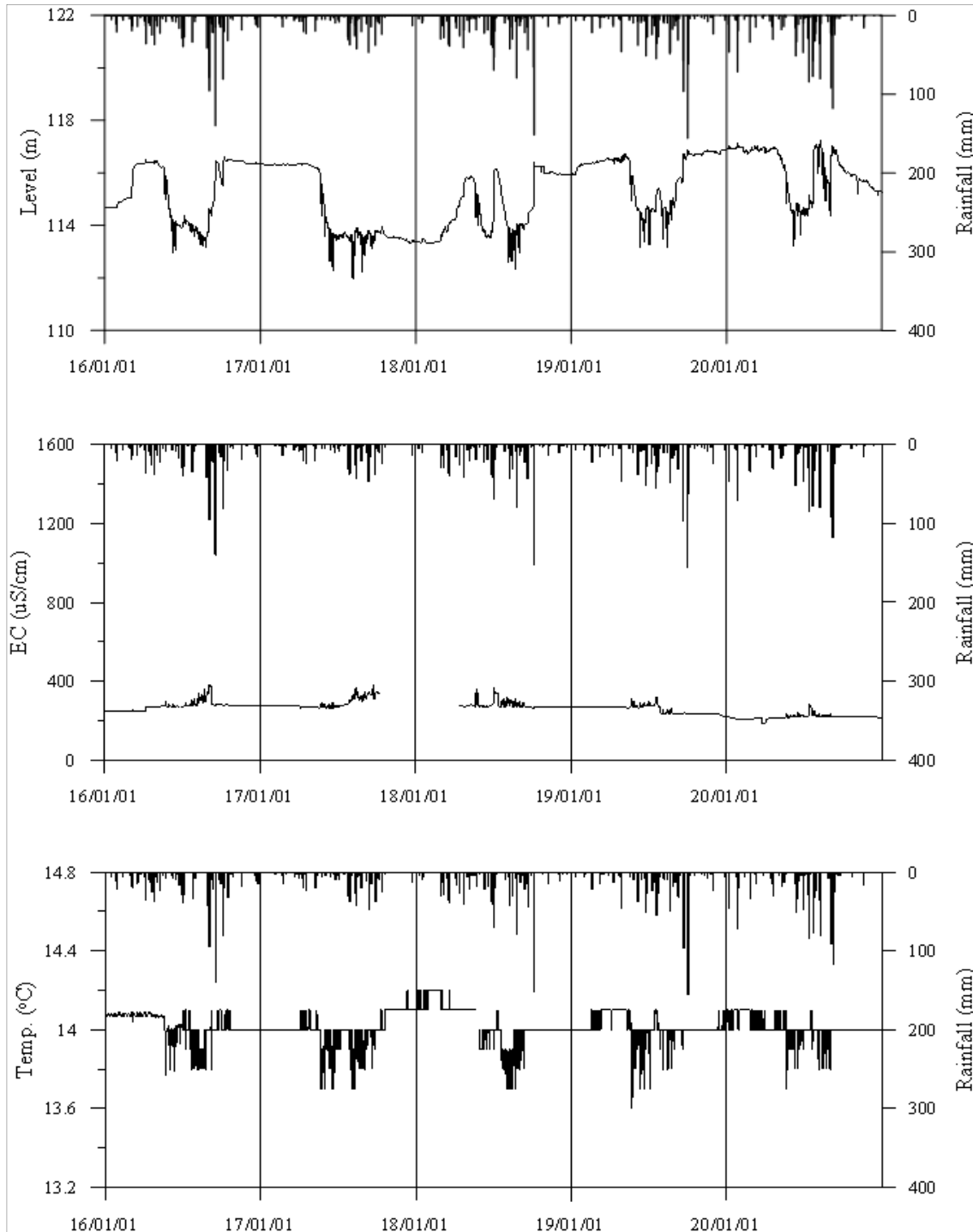
<경주5 관측공의 장기관측자료 (2016.1.1 ~ 2020.12.31)> (a)지하수위, (b)전기전도도, (c)수온
