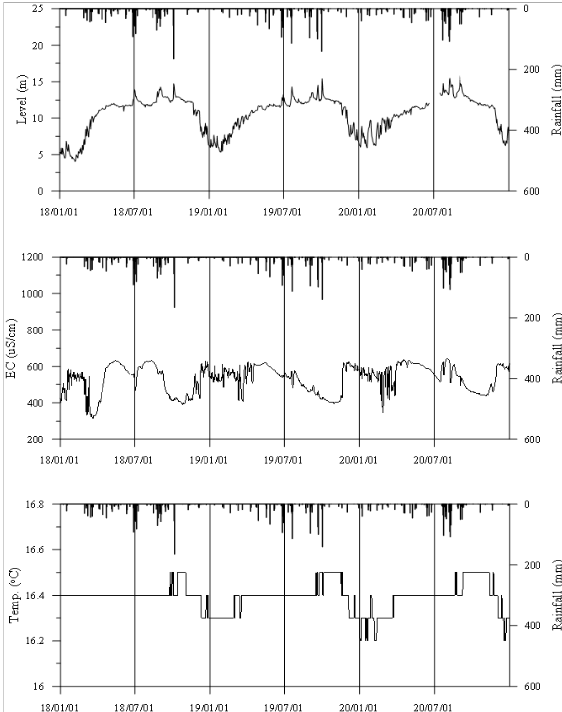
<진주5 관측공의 장기관측자료 (2018.1.1 ~ 2020.12.31)> (a)지하수위, (b)전기전도도, (c)수온
