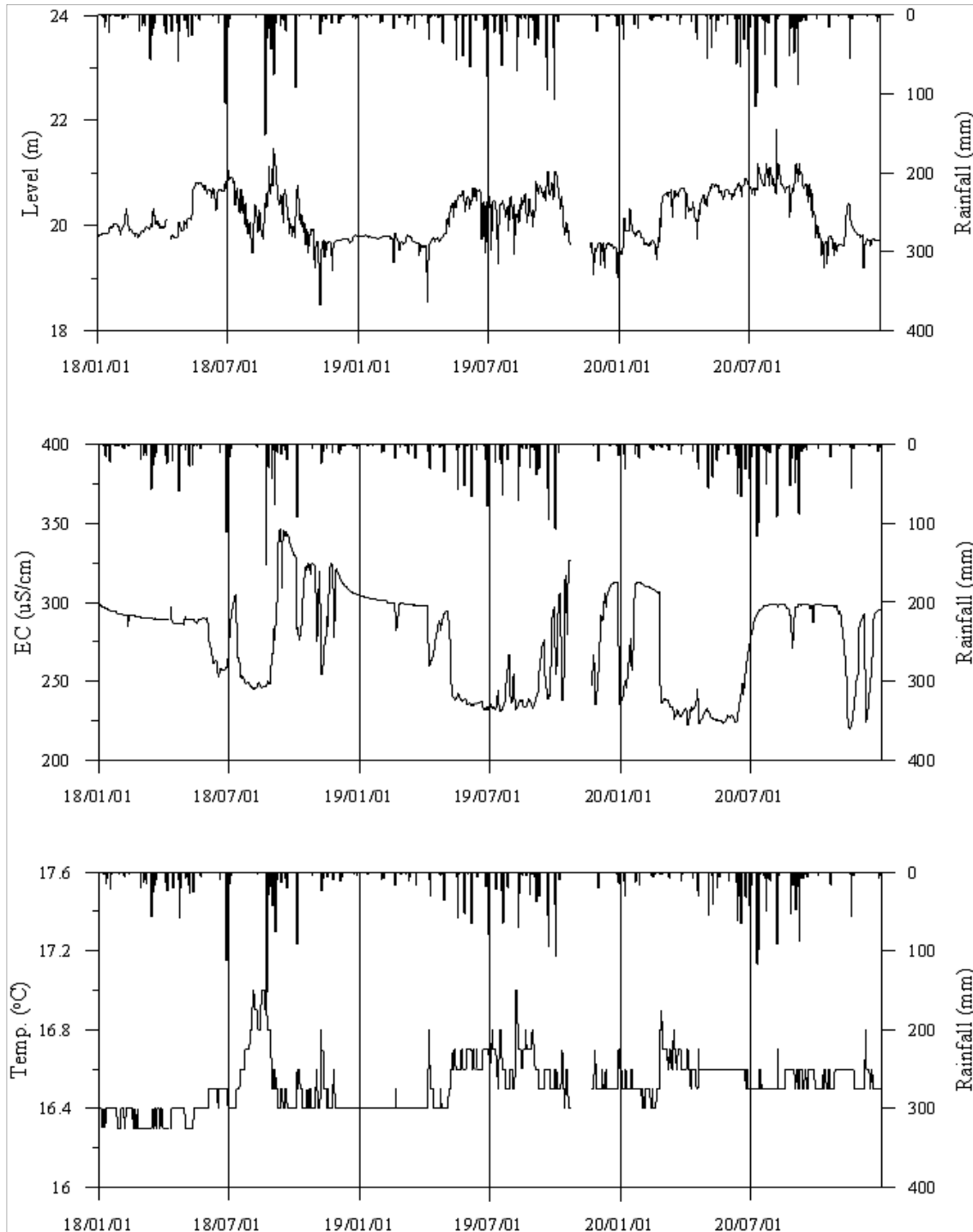
<함평6 관측공의 장기관측자료 (2018.1.1~2020.12.31)> (a)지하수위, (b)전기전도도, (c)수온
