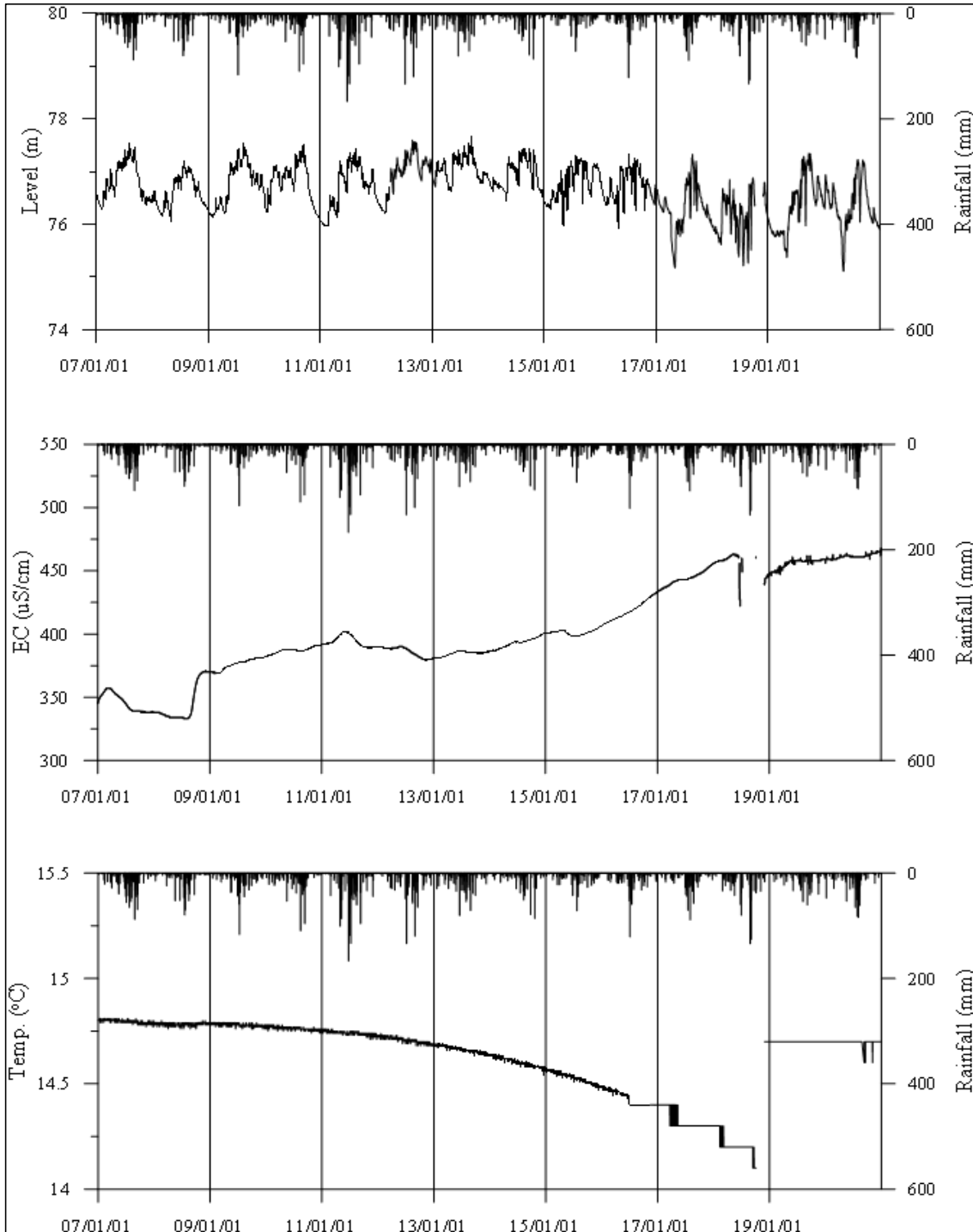
<음성1 관측공의 장기관측자료 (2007.1.1 ~ 2020.12.31)> (a)지하수위, (b)전기전도도, (c)수온
