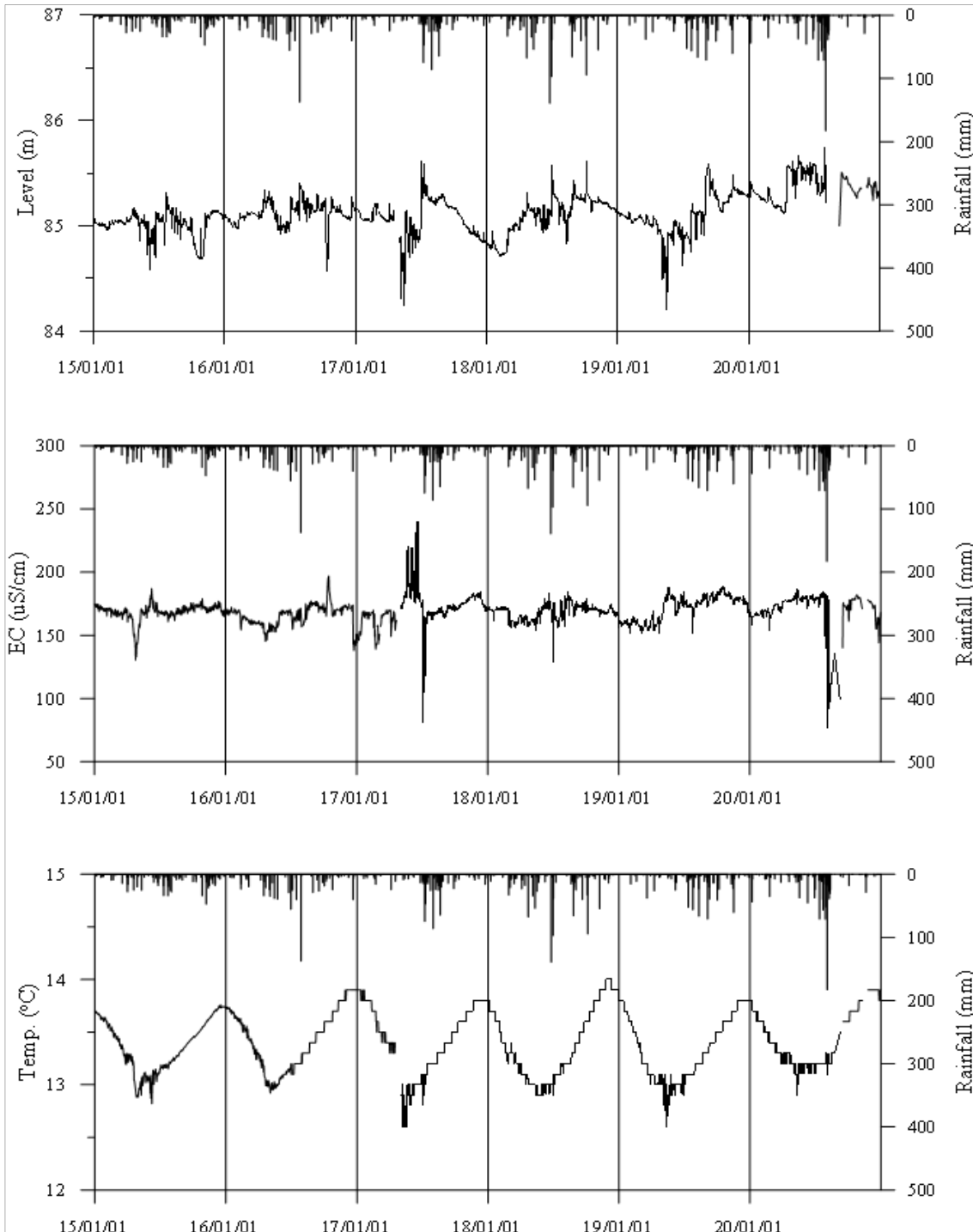
<예산1 관측공의 장기관측자료 (2015.1.1 ~ 2020.12.31)> (a)지하수위, (b)전기전도도, (c)수온
