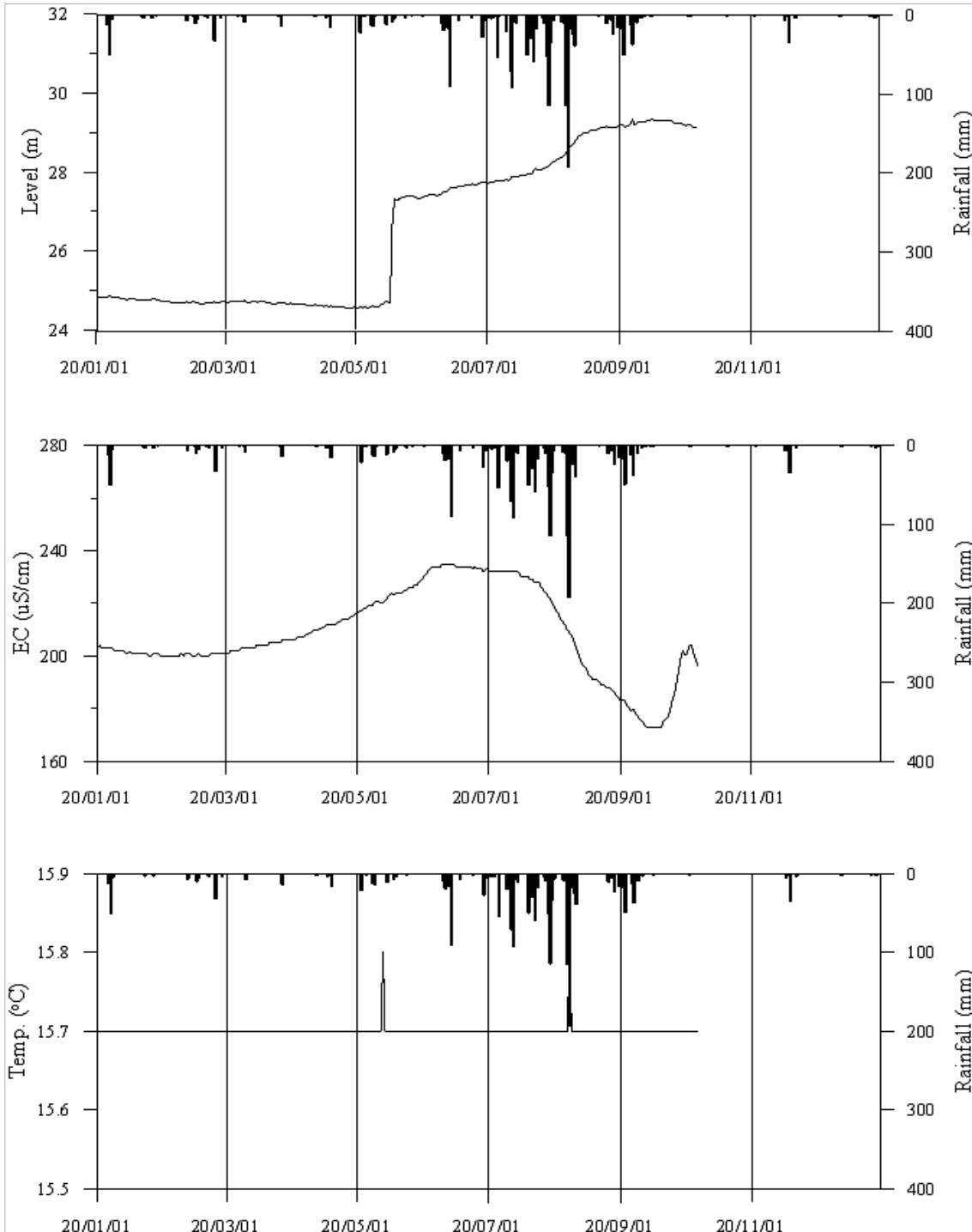
<김제1 관측공의 장기관측자료 (2020.1.1 ~ 2020.12.31)> (a)지하수위, (b)전기전도도, (c)수온
