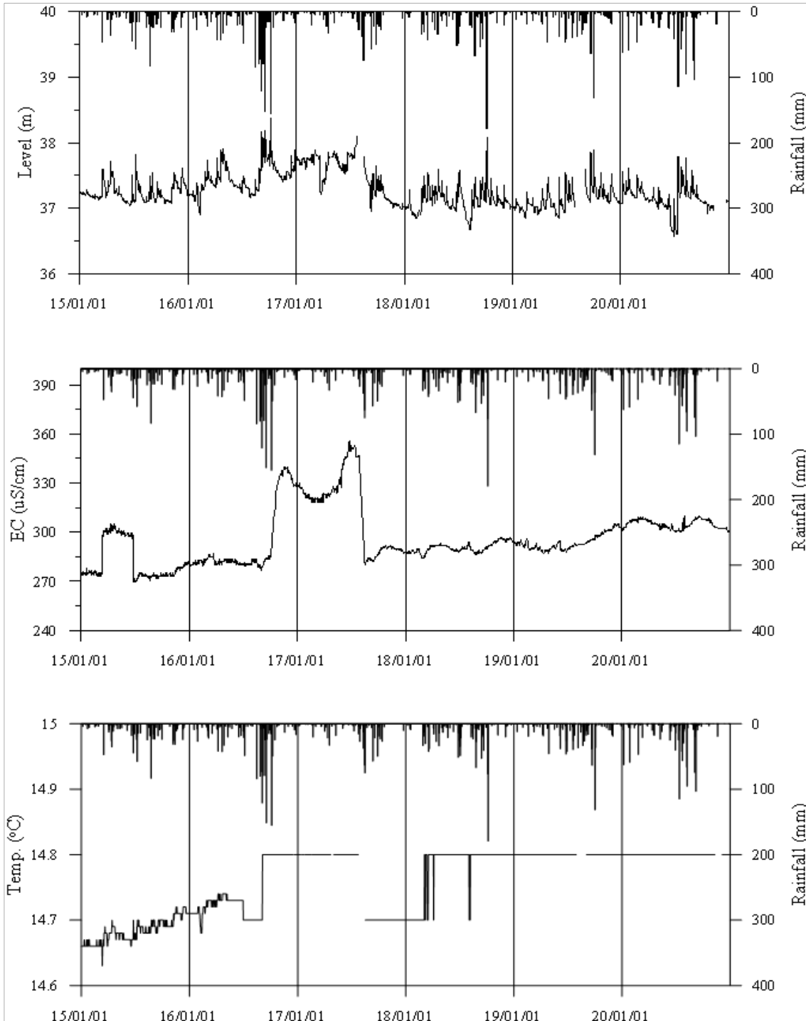
<포항1 관측공의 장기관측자료 (2015.1.1 ~ 2020.12.31)> (a)지하수위, (b)전기전도도, (c)수온
