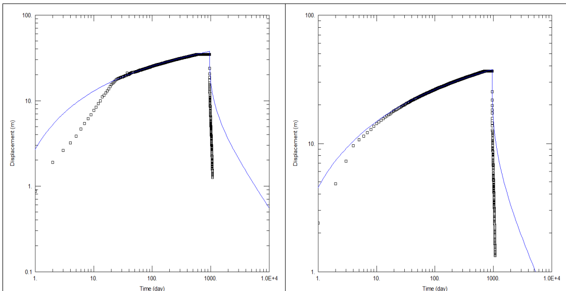
<영월5 관측공 양수시험>
