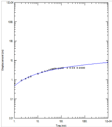
<기장1 관측공 양수시험>
