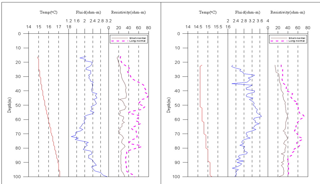
<당진4 관측공 물리검층>
