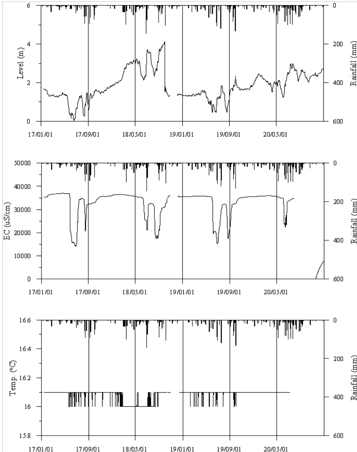
<고흥3 관측공의 장기관측자료 (2017.1.1~2020.12.31)> (a)지하수위, (b)전기전도도, (c)수온
