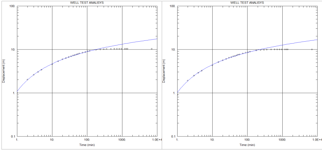
<당진4 관측공 양수시험>
