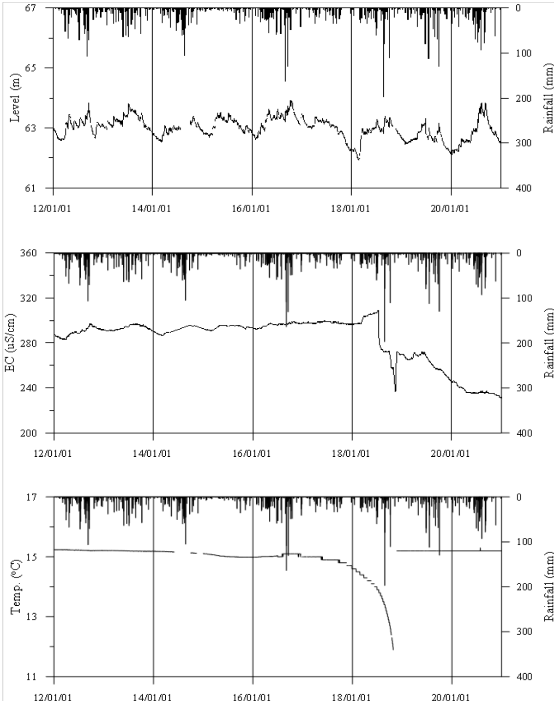
<밀양1 관측공의 장기관측자료 (2012.1.1 ~ 2020.12.31)> (a)지하수위, (b)전기전도도, (c)수온
