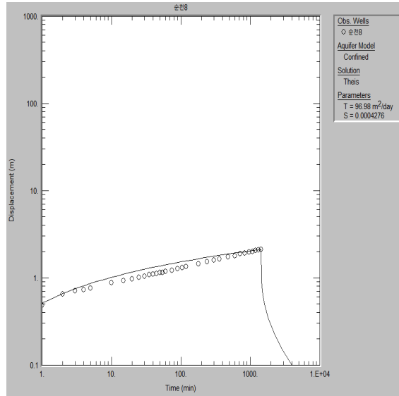
<순천8 관측공 양수시험>
