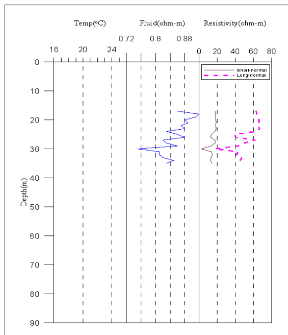
<울진3 관측공 물리검층>
