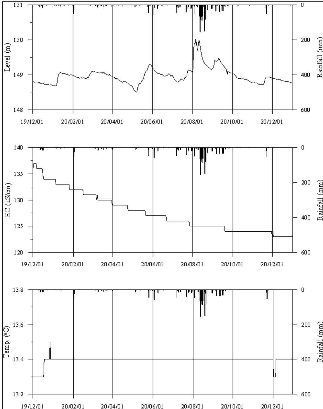
<포천6 관측공의 장기관측자료 (2019.12.1 ~ 2020.12.31)> (a)지하수위, (b)전기전도도, (c)수온
