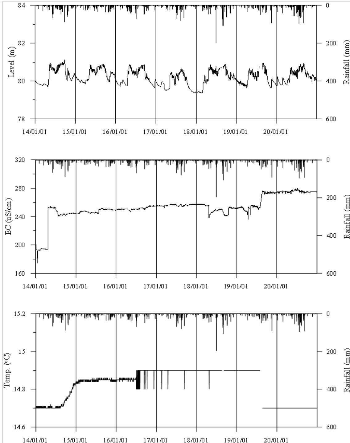
<청양2 관측공의 장기관측자료 (2014.1.1 ~ 2020.12.31)> (a)지하수위, (b)전기전도도, (c)수온
