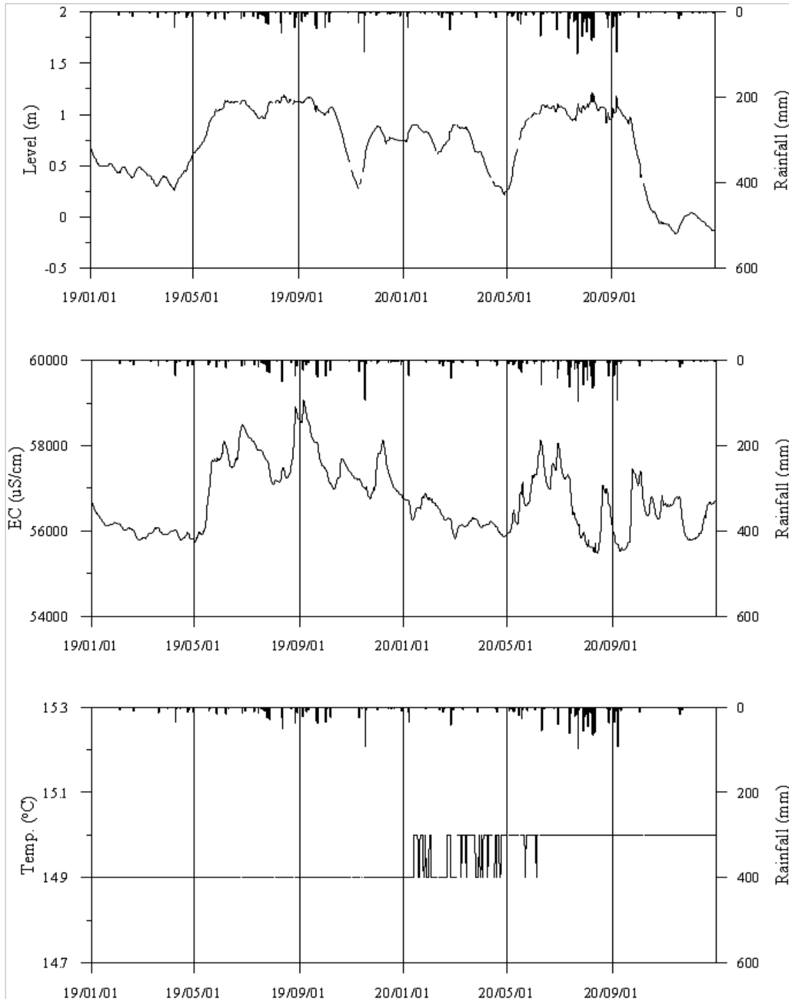
<보령6 관측공의 장기관측자료 (2019.1.1 ~ 2020.12.31)> (a)지하수위, (b)전기전도도, (c)수온
