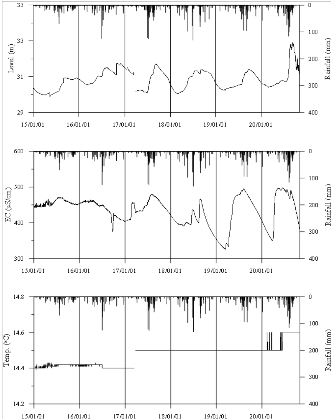
<남양주2 관측공의 장기관측자료 (2015.1.1 ~ 2020.12.31)> (a)지하수위, (b)전기전도도, (c)수온
