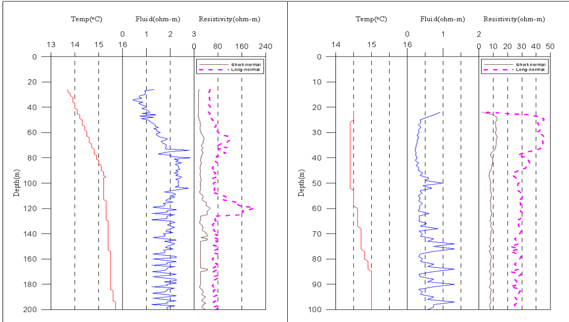
<영주3 관측공 물리검층>
