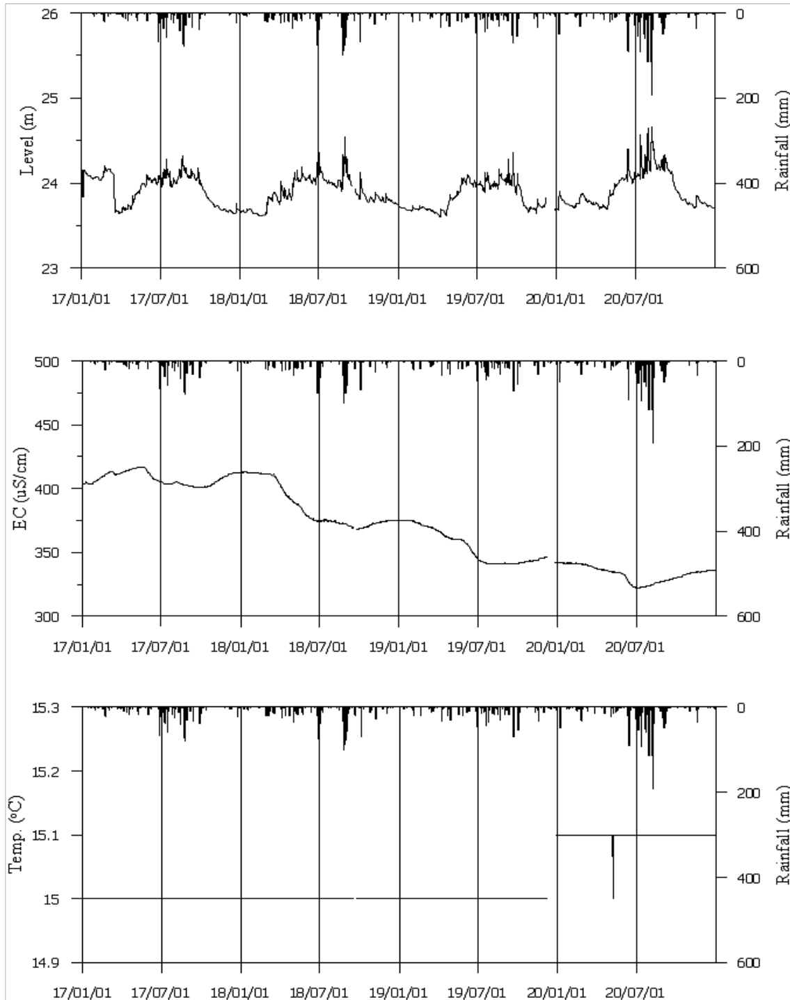
<완주2 관측공의 장기관측자료 (2017.1.1 ~ 2020.12.31)> (a)지하수위, (b)전기전도도, (c)수온
