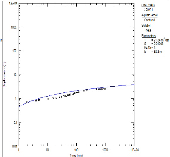
<기장2 관측공 양수시험>
