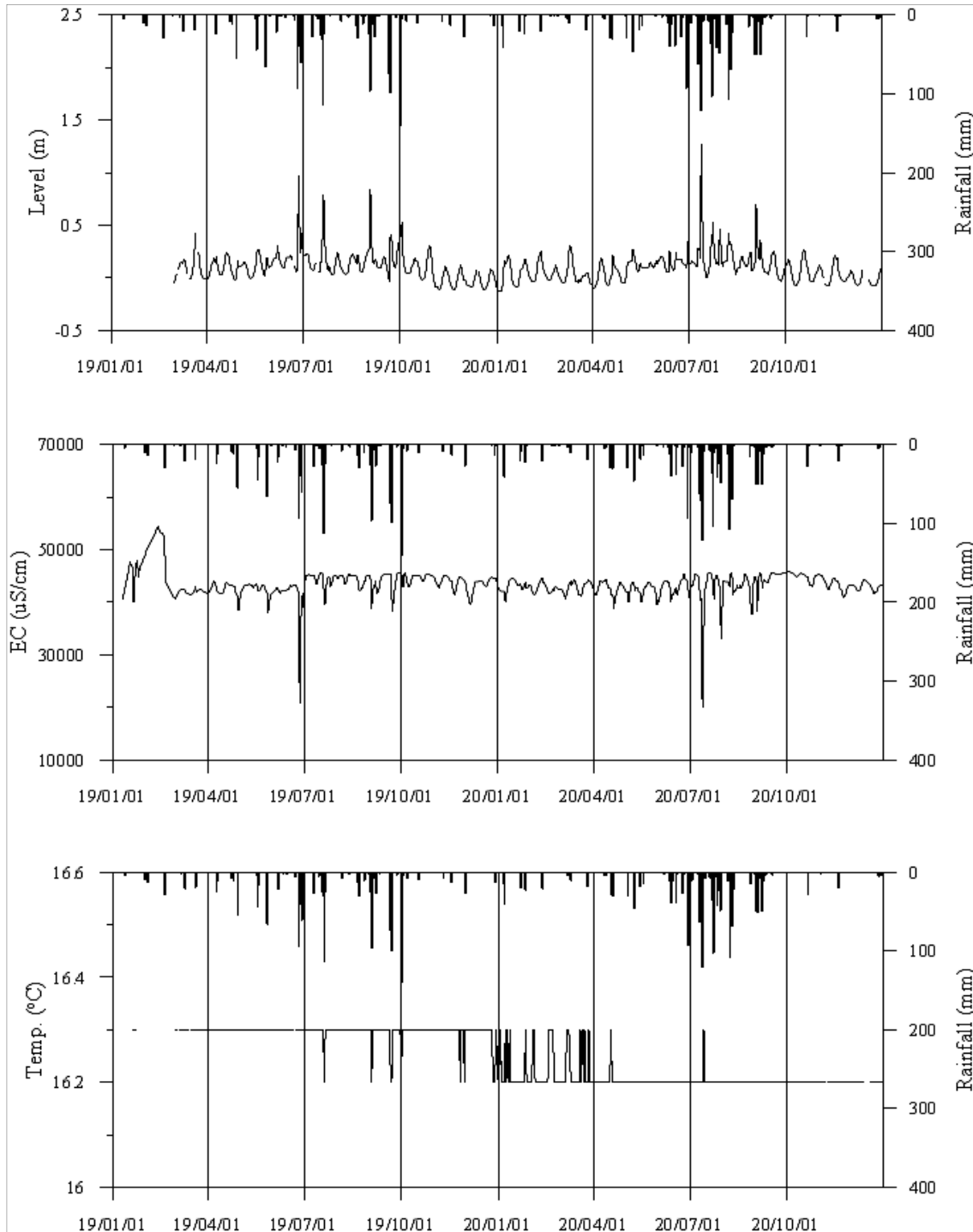
<사천4 관측공의 장기관측자료 (2019.1.1 ~ 2020.12.31)> (a)지하수위, (b)전기전도도, (c)수온
