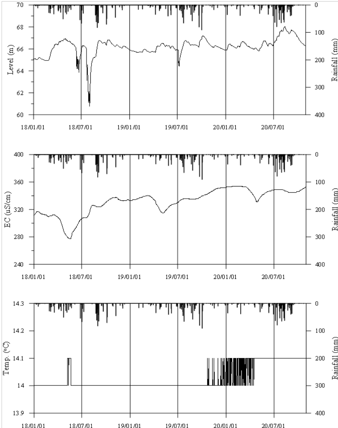
<예천1 관측공의 장기관측자료 (2018.1.1 ~ 2020.12.31)> (a)지하수위, (b)전기전도도, (c)수온
