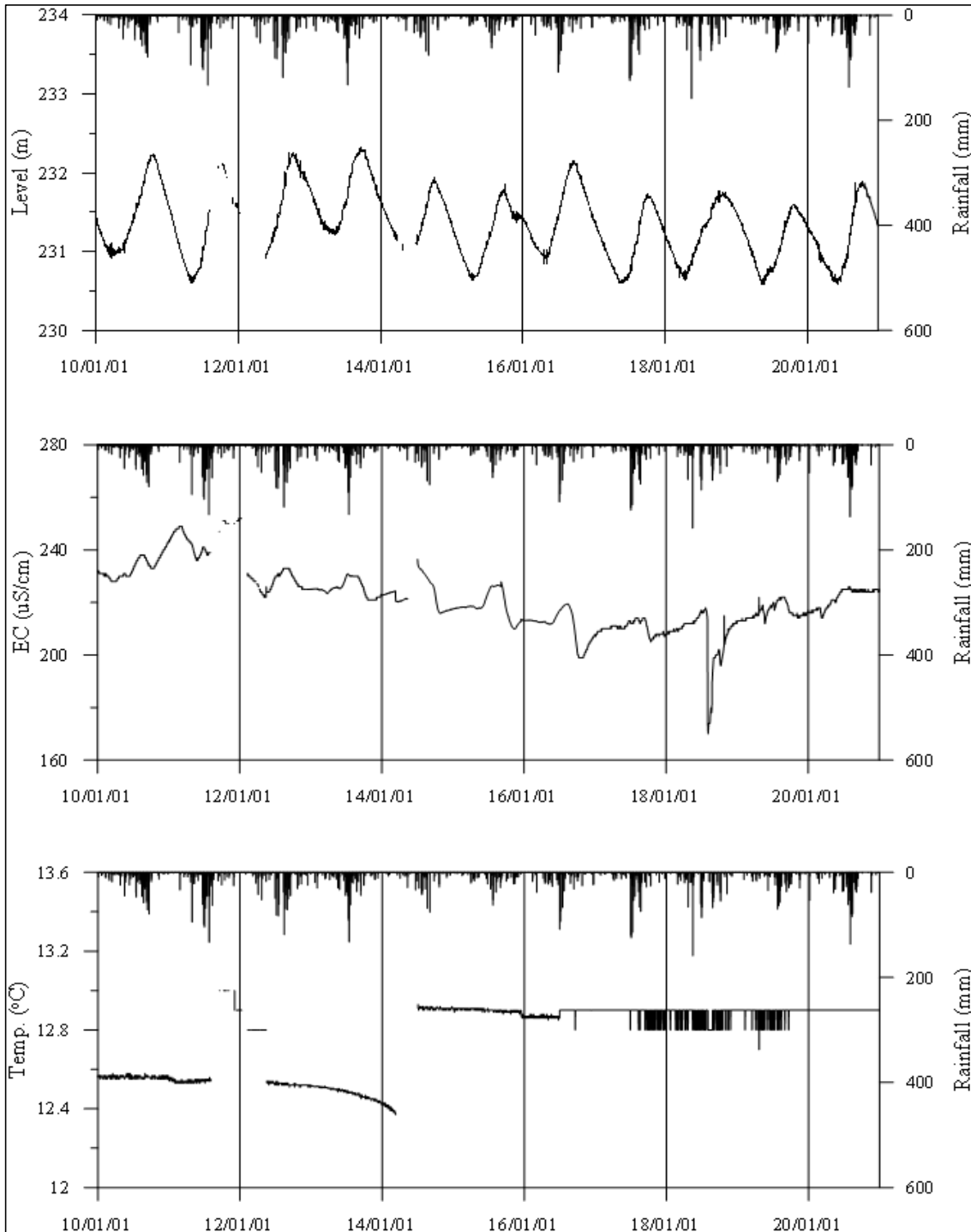
<홍천2 관측공의 장기관측자료 (2010.1.1 ~ 2020.12.31)> (a)지하수위, (b)전기전도도, (c)수온
