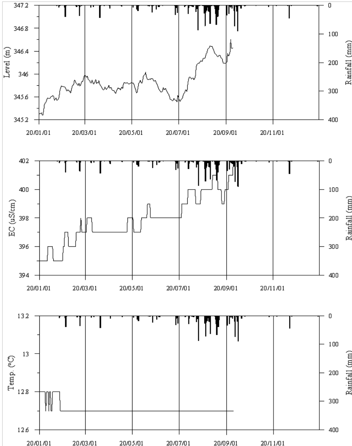
<영양2 관측공의 장기관측자료 (2020.1.1 ~ 2020.12.31.)> (a)지하수위, (b)전기전도도, (c)수온
