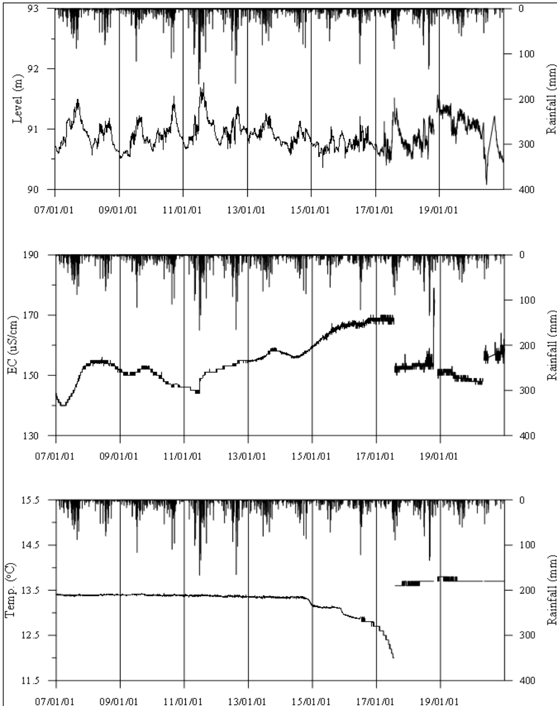
<음성2 관측공의 장기관측자료 (2007.1.1 ~ 2020.12.31)> (a)지하수위, (b)전기전도도, (c)수온
