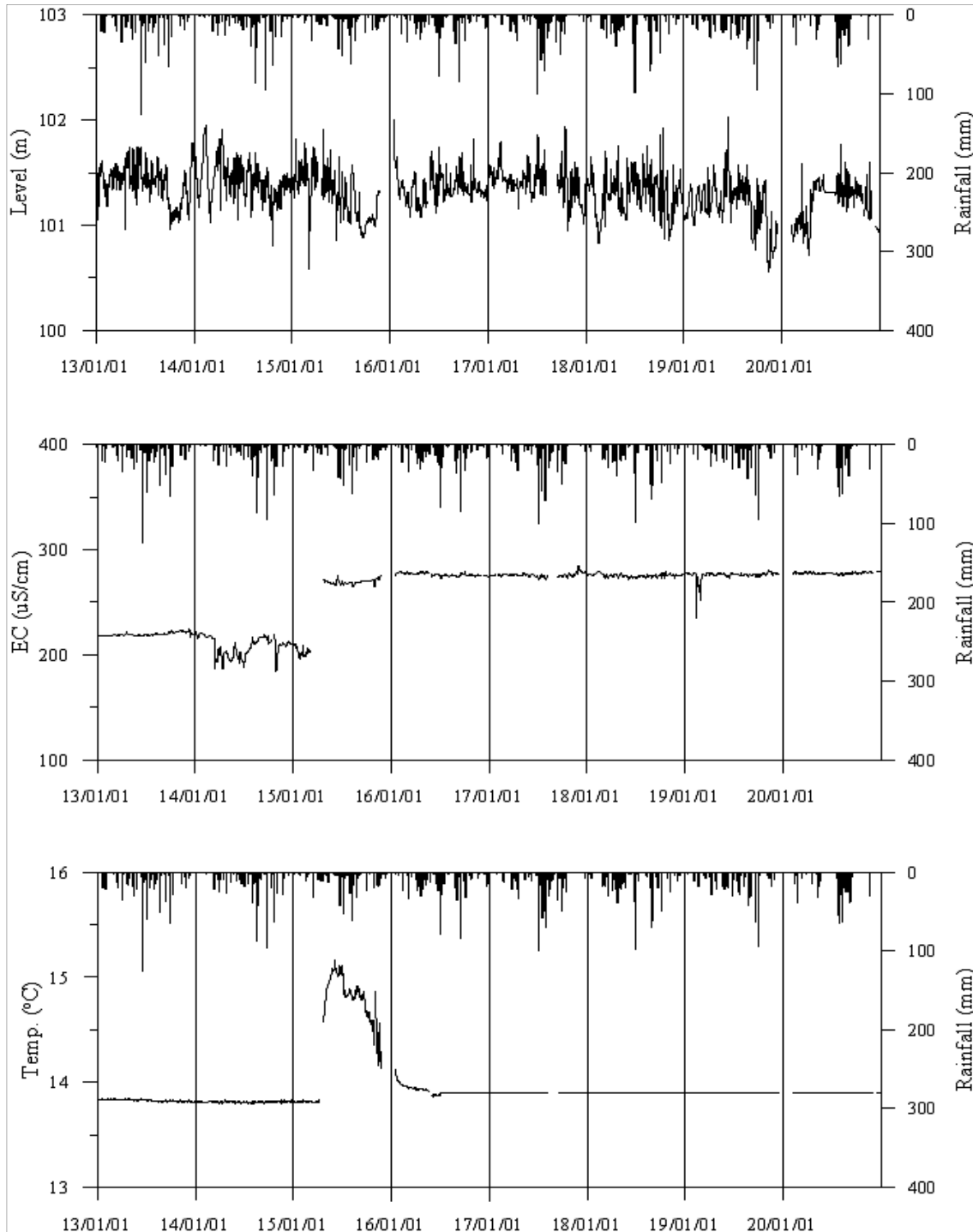
<안동3 관측공의 장기관측자료 (2013.1.1 ~ 2020.12.31)> (a)지하수위, (b)전기전도도, (c)수온
