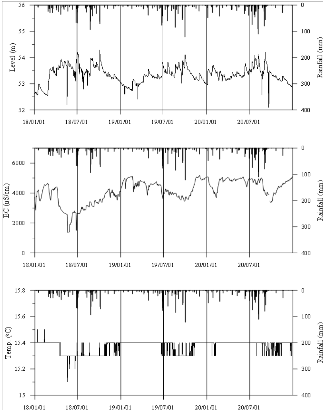
<영천6 관측공의 장기관측자료 (2018.1.1 ~ 2020.12.31)> (a)지하수위, (b)전기전도도, (c)수온
