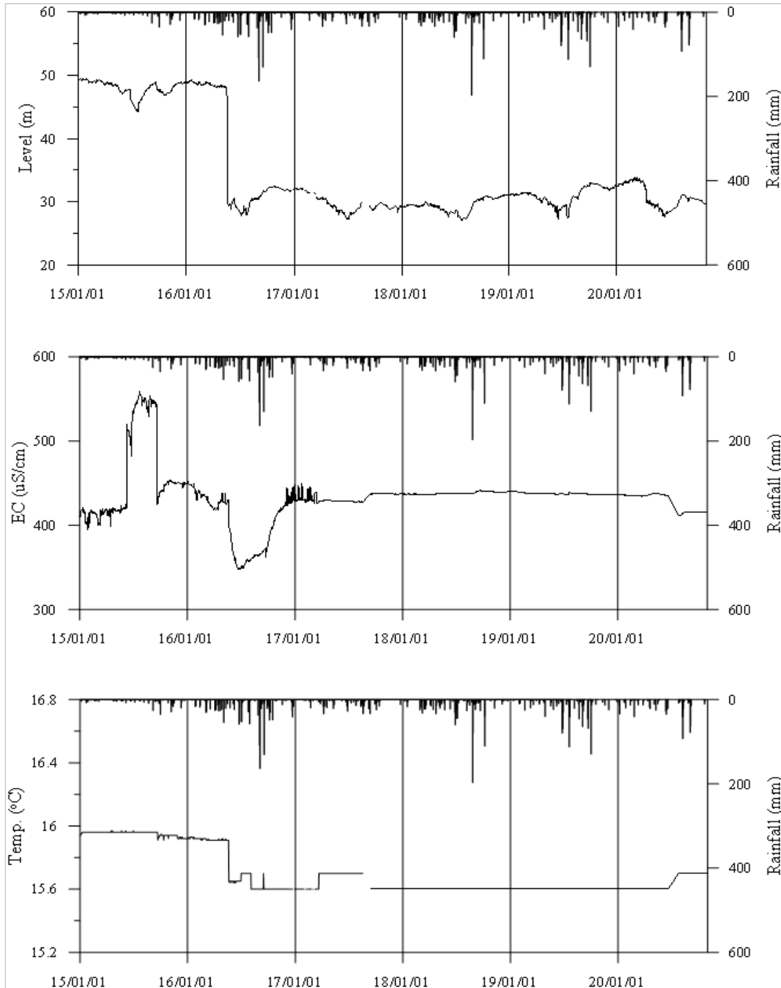
<창녕3 관측공의 장기관측자료 (2015.1.1 ~ 2020.12.31)> (a)지하수위, (b)전기전도도, (c)수온
