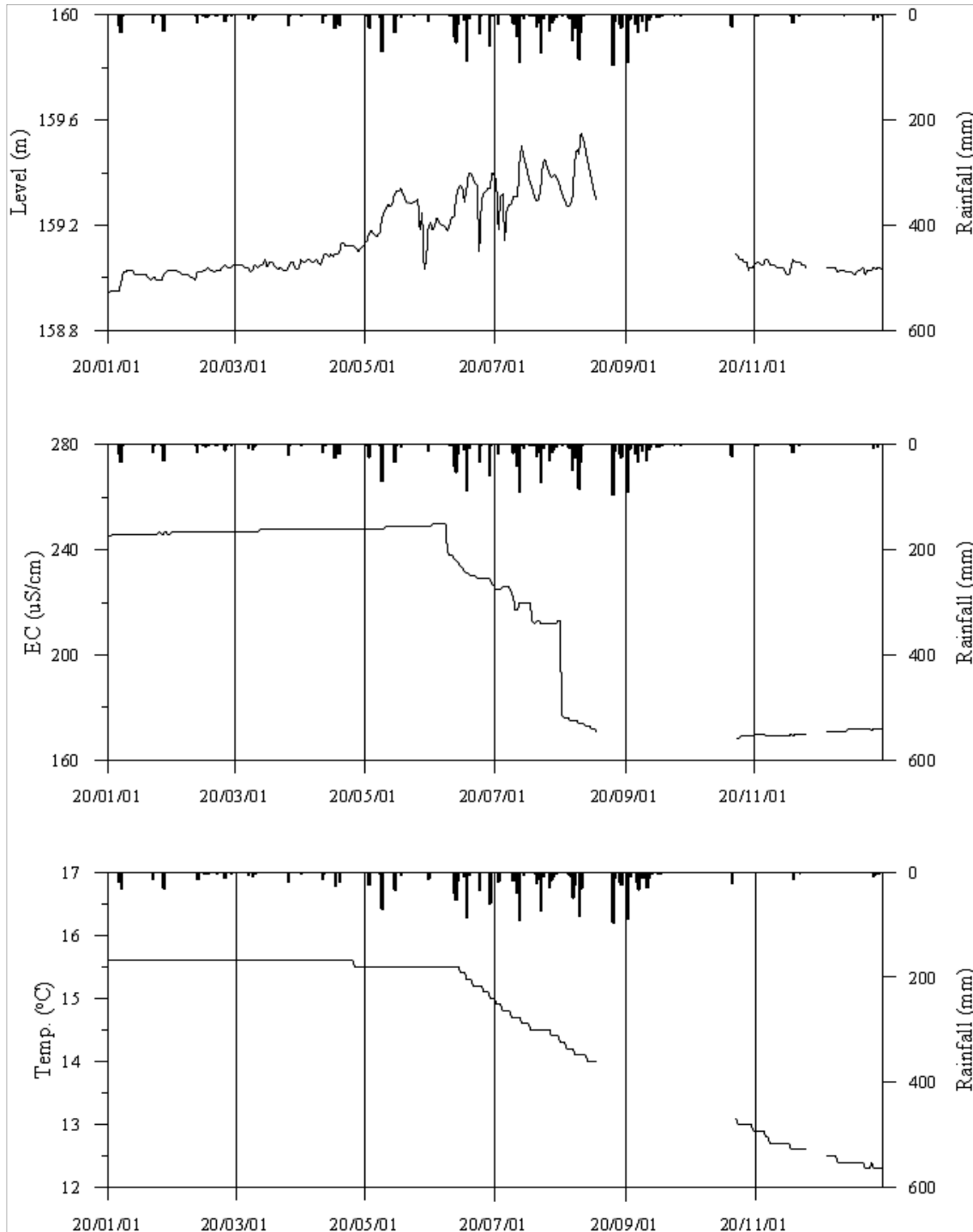
<장흥5 관측공의 장기관측자료 (2020.1.1 ~ 2020.12.31)> (a)지하수위, (b)전기전도도, (c)수온
