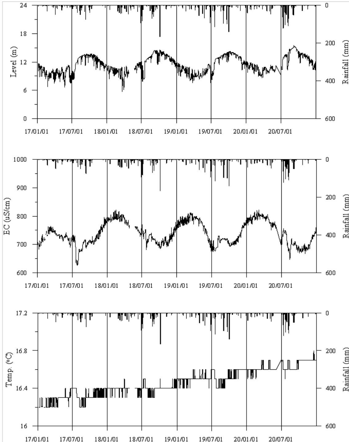
<진주4 관측공의 장기관측자료 (2017.1.1 ~ 2020.12.31)> (a)지하수위, (b)전기전도도, (c)수온
