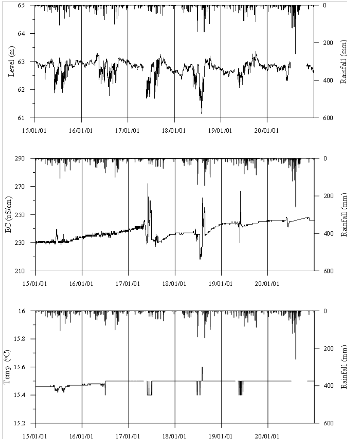
<화순2 관측공의 장기관측자료 (2015.1.1 ~ 2020.12.31)> (a)지하수위, (b)전기전도도, (c)수온
