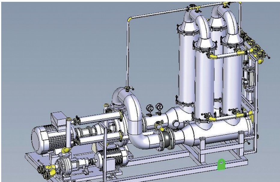
< 정제설비 필터구동부의 3차원 설계도 >
