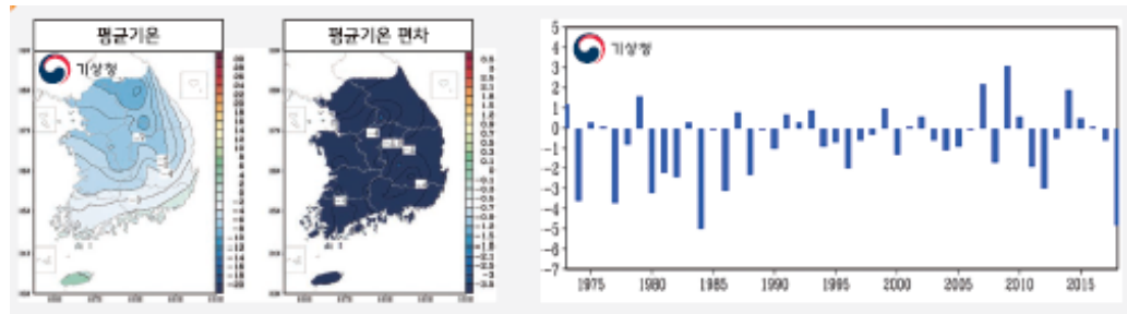
[그림 1-4-5] 전국 45개 지점의 1월 23일~2월 13일 평균기온과 평년편차(°C) 분포도 및 평균기온 시계열(1973~2018년)
