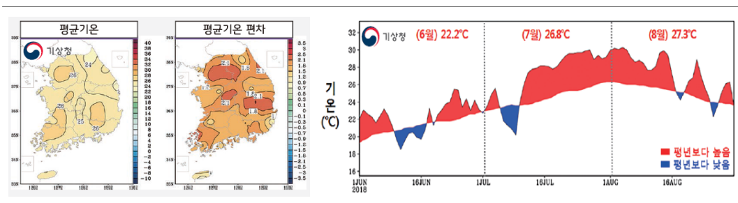
[그림 1-4-12] 전국 45개 지점의 여름철 평균기온과 편차(°C) 분포도 및 일변화 시계열
