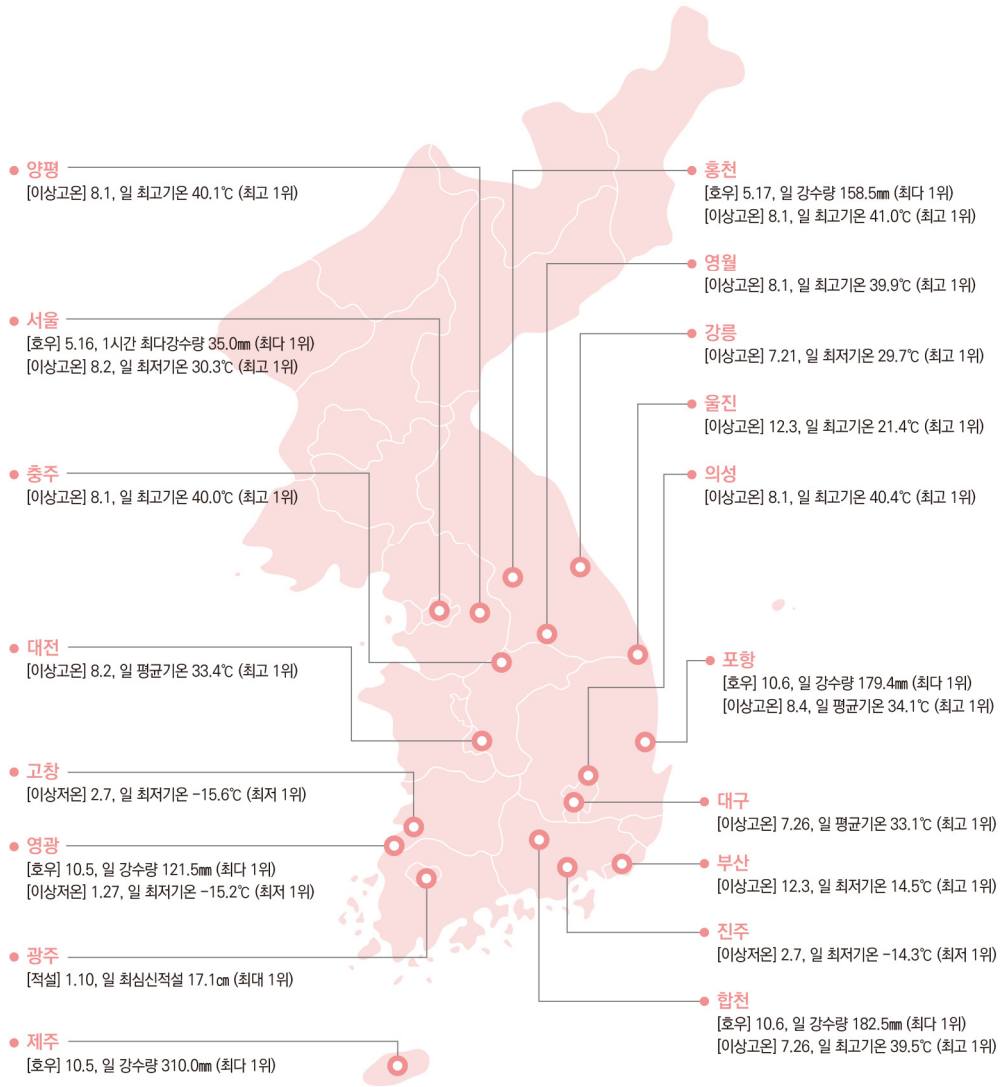
[그림 1-4-4] 우리나라의 이상기후 발생 현황(2018)
