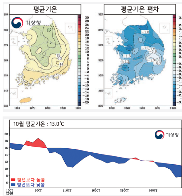
[그림 1-4-15] 전국 45개 지점의 10월 평균기온과 편차( ^{\circ}\text{C} ) 분포도 및 일변화 시계열
