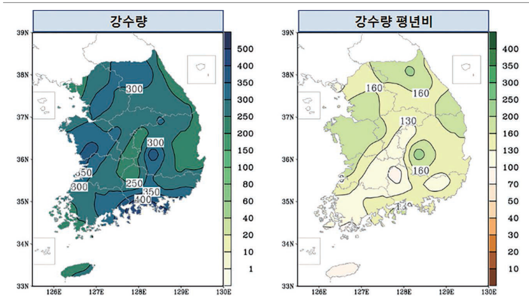
[그림 1-4-9] 장마 기간(6.19 ~ 7.11) 강수량(mm) 및 강수량 평년비(%) 분포도
