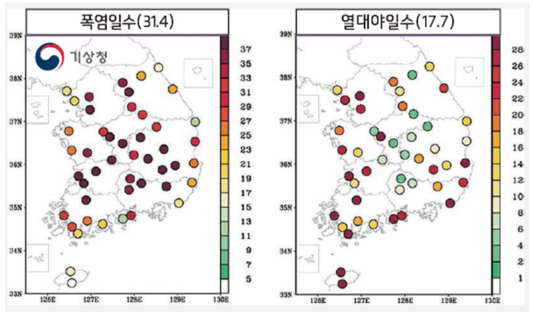
[그림 1-4-13] 여름철 전국 47개 지점의 폭염 일수 및 열대야 일수 분포도
