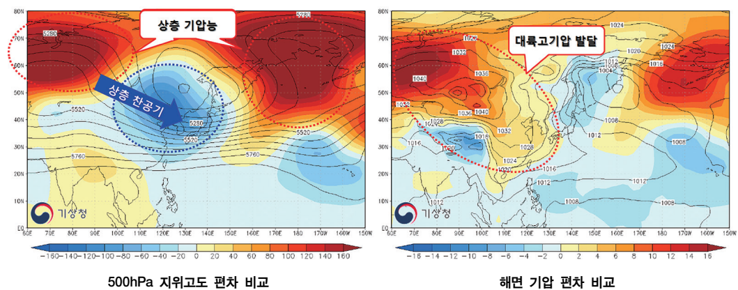
[그림 1-4-6] 2018년 1월 23일 ~ 2월 13일 전 지구 500hPa 지위고도 편차, 해면 기압 편차 분포도
