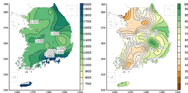
[그림 1-4-2] 2017년 우리나라 연 강수량 및 연 강수량 퍼센타일* 분포도
