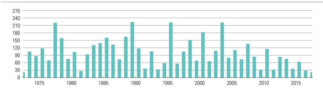
[그림 1-4-11] 장마 시작 전(6.1.~24) 전국 45개 지점의 강수량 시계열(1973~2018년)
