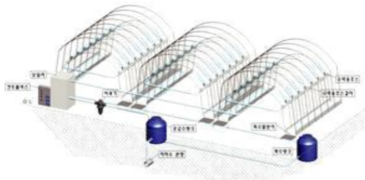
<순환식 수막시스템의 구조>
