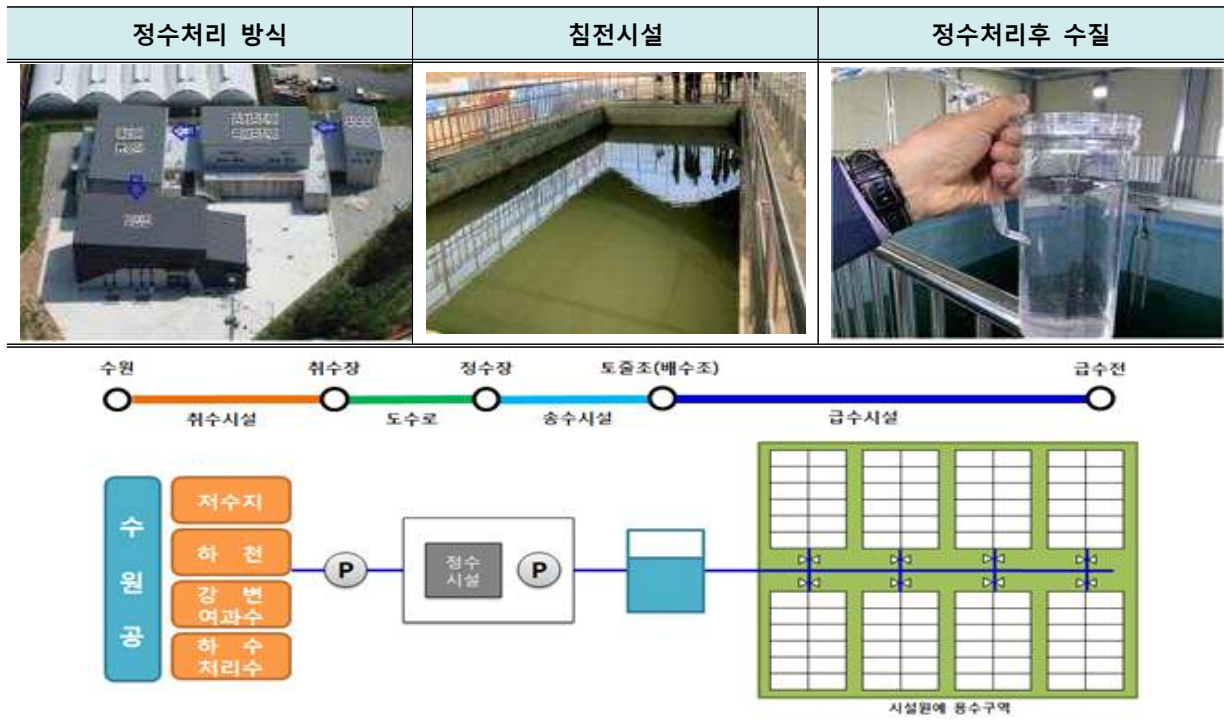
<용수공급체계 개요>
