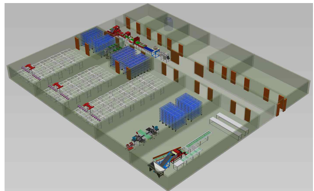
<3D 모델링>
