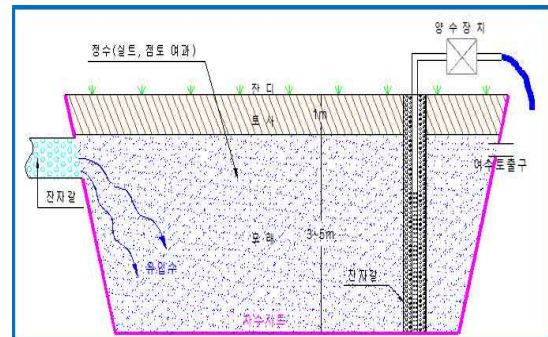
지하돛병 개념 모식도 및 설치단면
