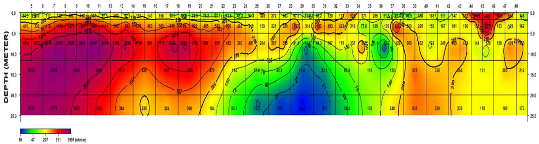
<그림 4-3-4> 10110401_가 유역 수평탐사
