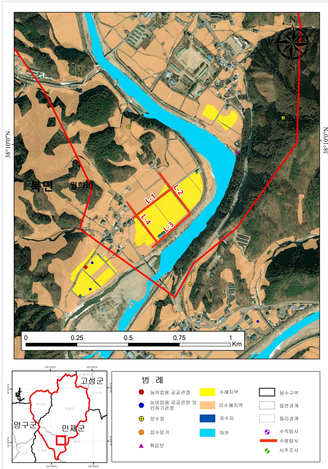
<그림 4-3-5> 10110401_가 유역 전기비저항 탐사 및 시추위치
