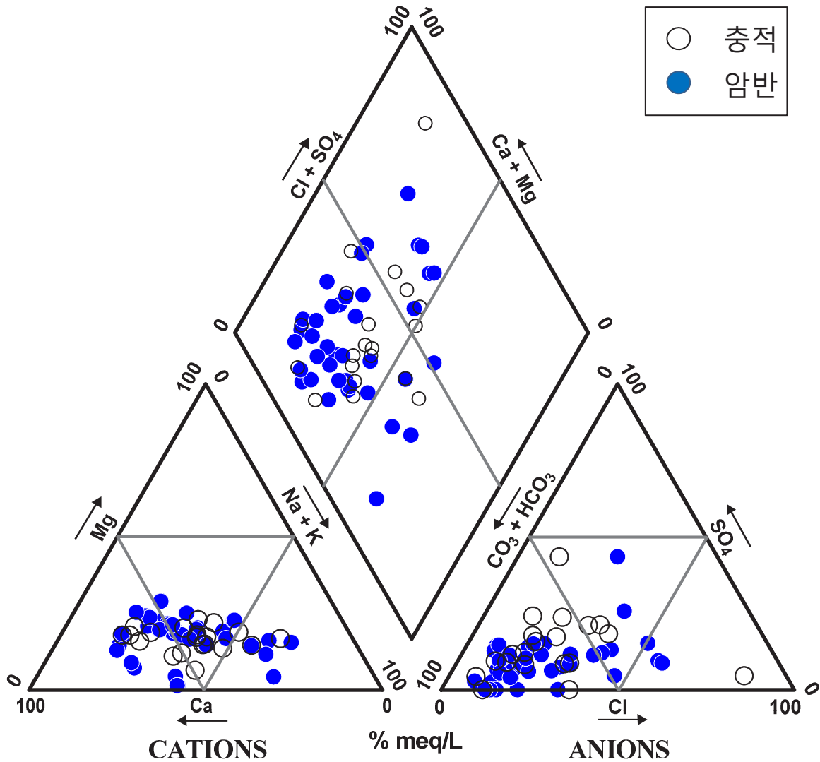
<그림 3-2-10> 남이2지구 지하수의 Piper Diagram
