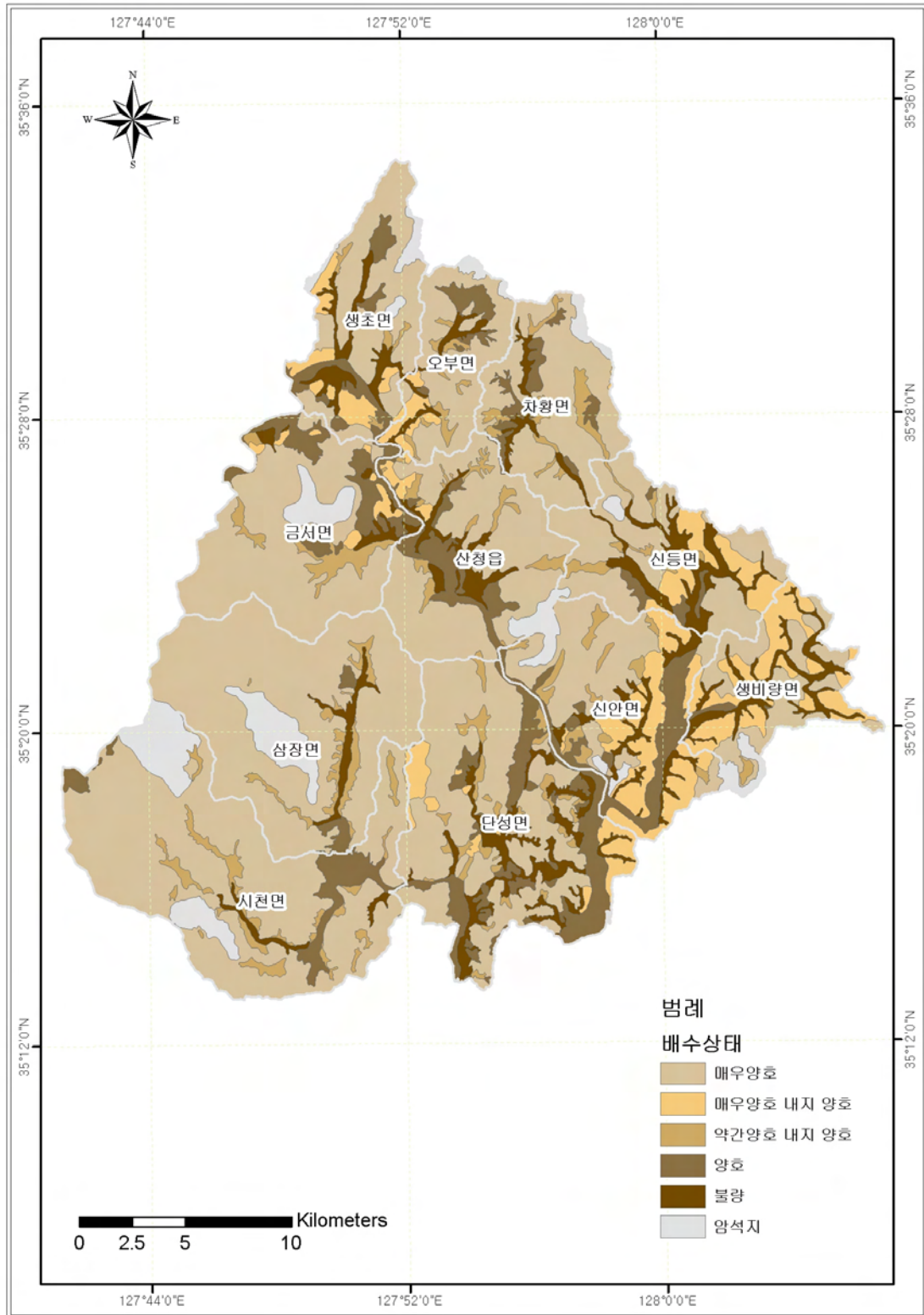
<그림 1-4-8> 토양도
