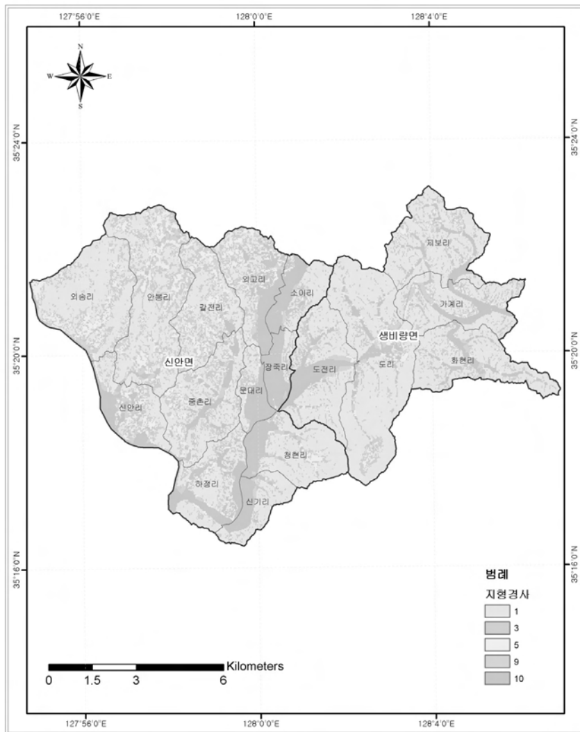
<그림 3-3-6> 지형경사(Topography)
