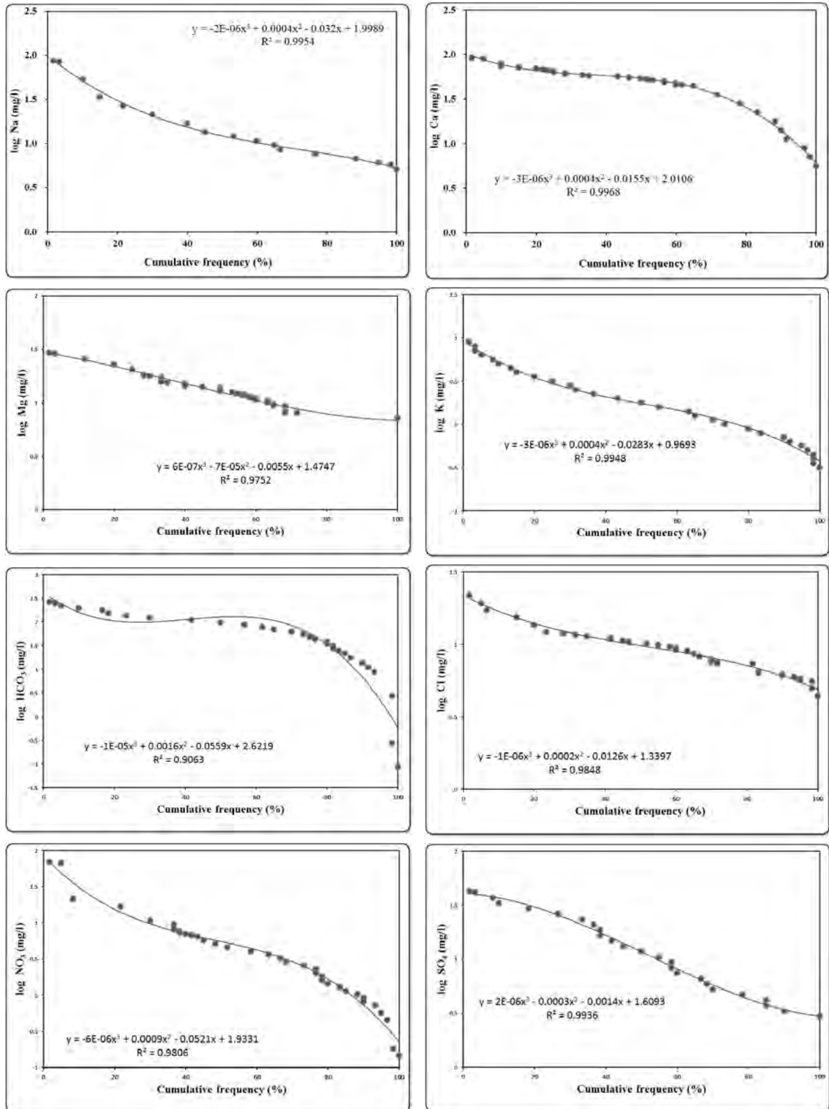
<그림 3-2-17> Sinclair에 의한 배경값(Threshold) 분석
