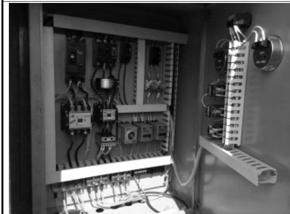
사 진 (배전반)
