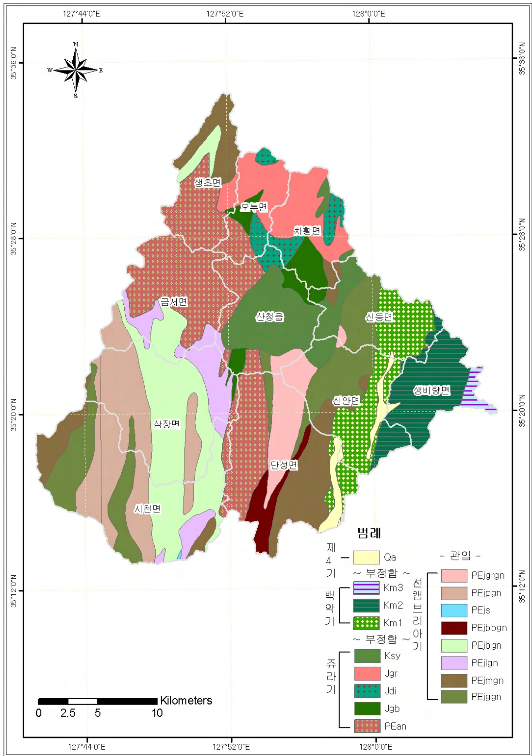
<그림 1-4-5> 지질도
