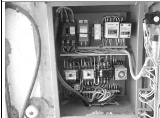
사 진 (배전함)
