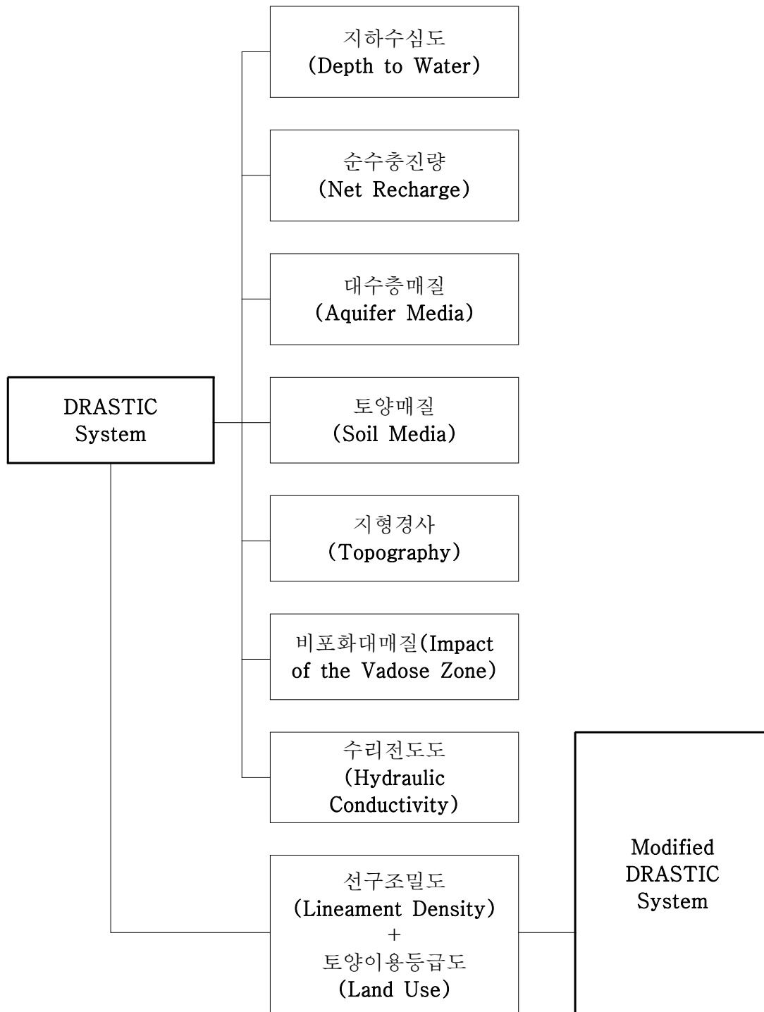
<그림 3-8-1> DRASTIC 시스템
