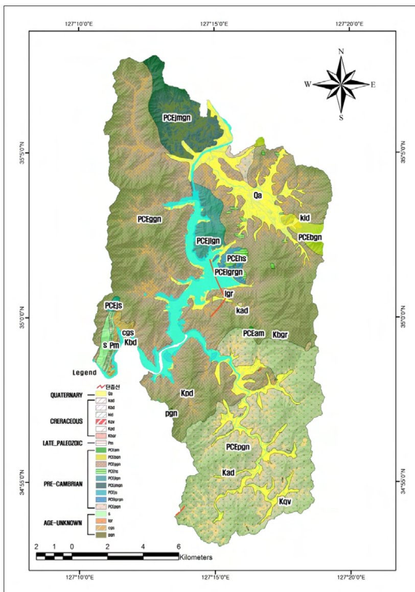
<그림 1-4-4> 승외지구 지질도
