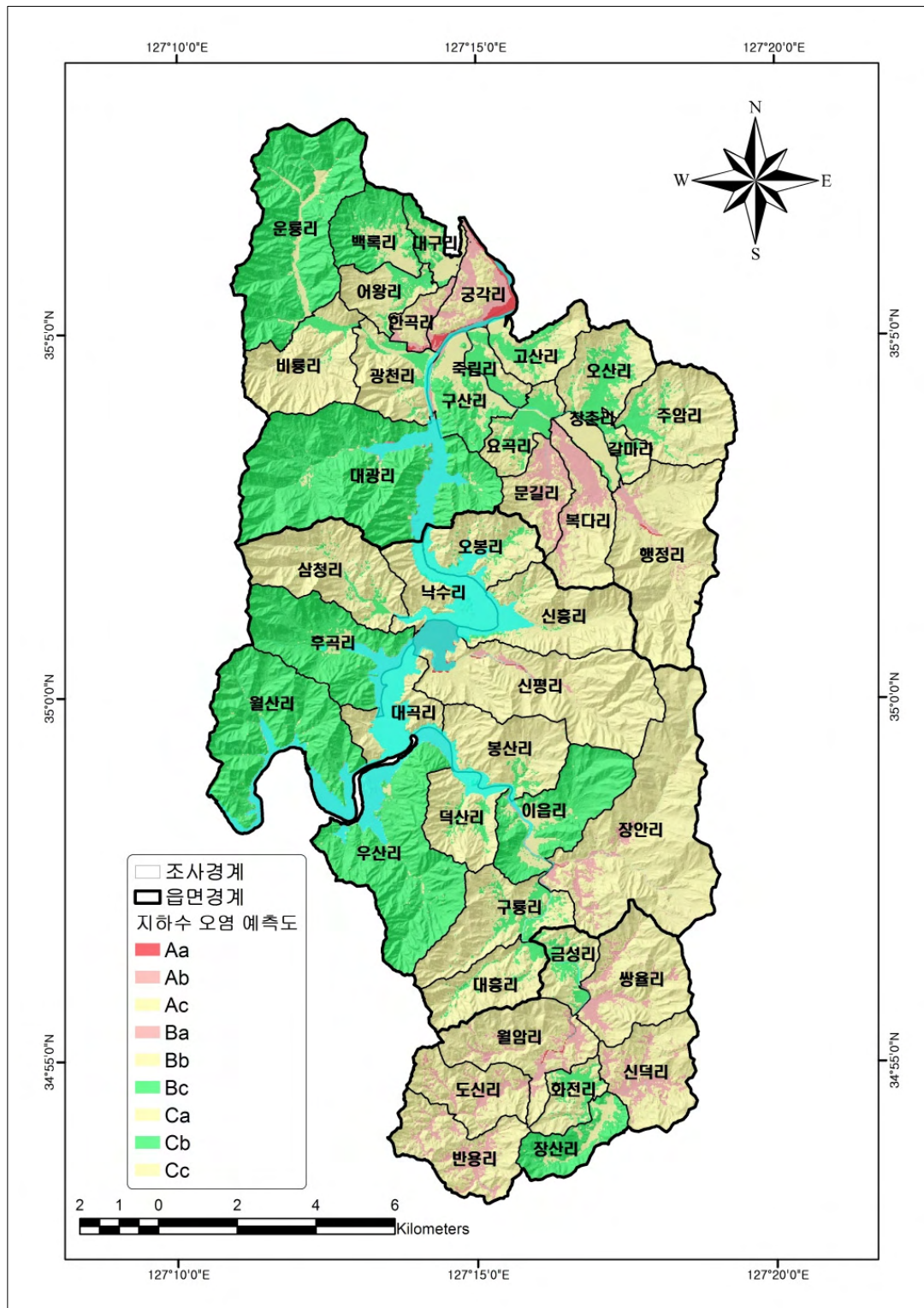
<그림 3-8-6> 승외지구 지하수오염예측도
