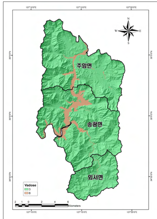
<그림 3-3-7> 비포화대 매질 (Impact of the Vadose Zone)
