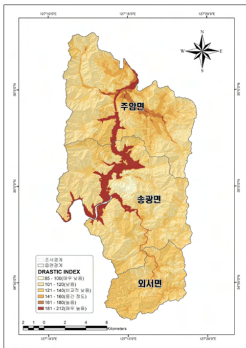
<그림 3-8-1> 승외지구 DRASTIC INDEX Map
