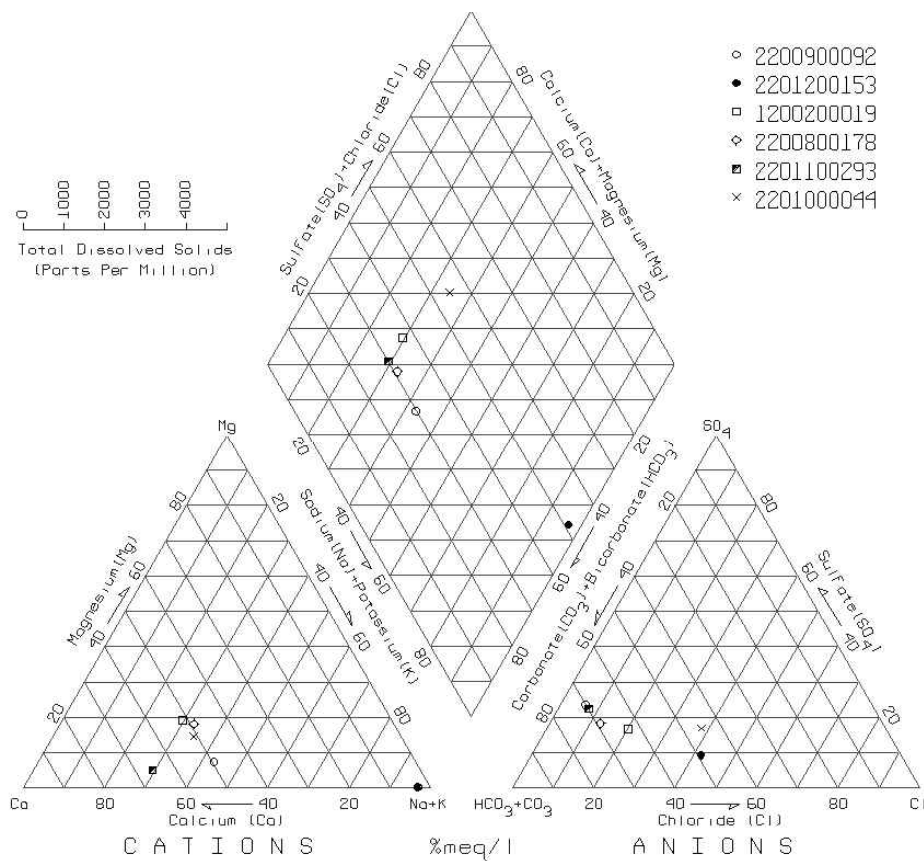
<그림 3-2-19> 승희지구 암반 지하수의 Piper Diagram
