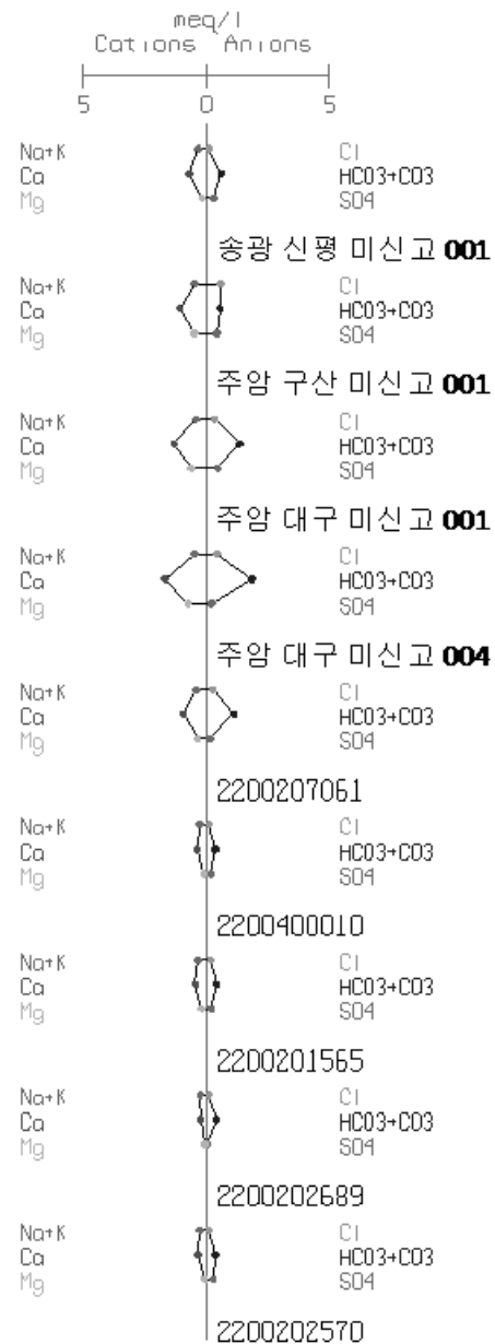
<그림 3-2-22> 승외지구 충적 지하수의 Stiff Diagram
