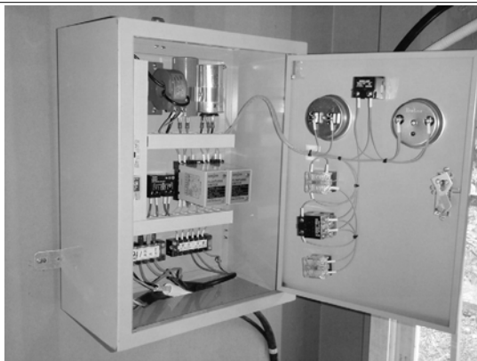
사 진 (배전함)
