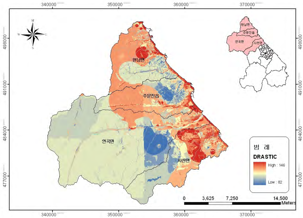
<그림 3-3-10> 일반오염취약성도
