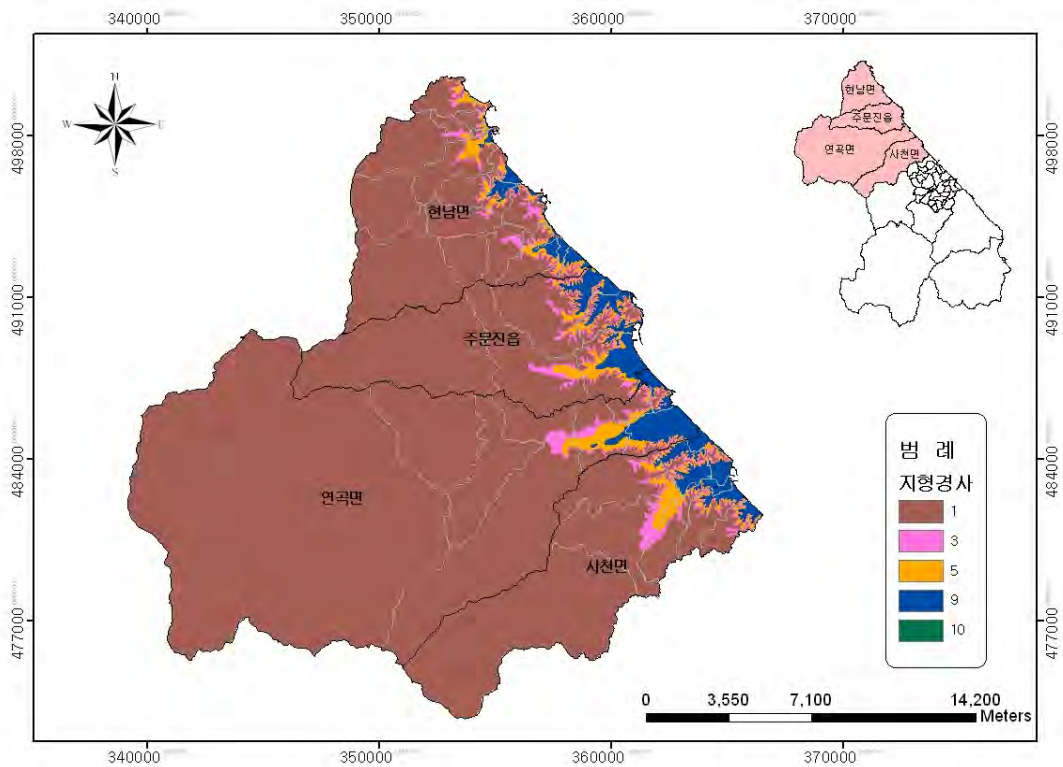
<그림 3-3-6> 지형경사(Topography)
