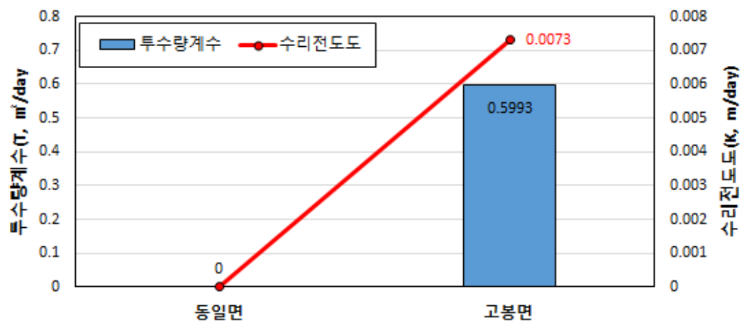
<그림 3-1-6> 읍면별 지하수 투수량계수 및 수리전도도(기하평균)
