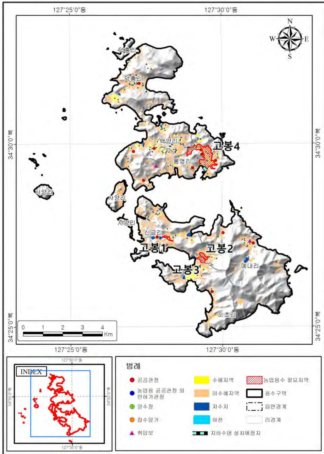
<그림 4-3-1> 고봉지구 지하수개발·이용 방안도
