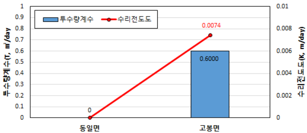
<그림 3-1-5> 읍면별 지하수 투수량계수 및 수리전도도(산술평균)
