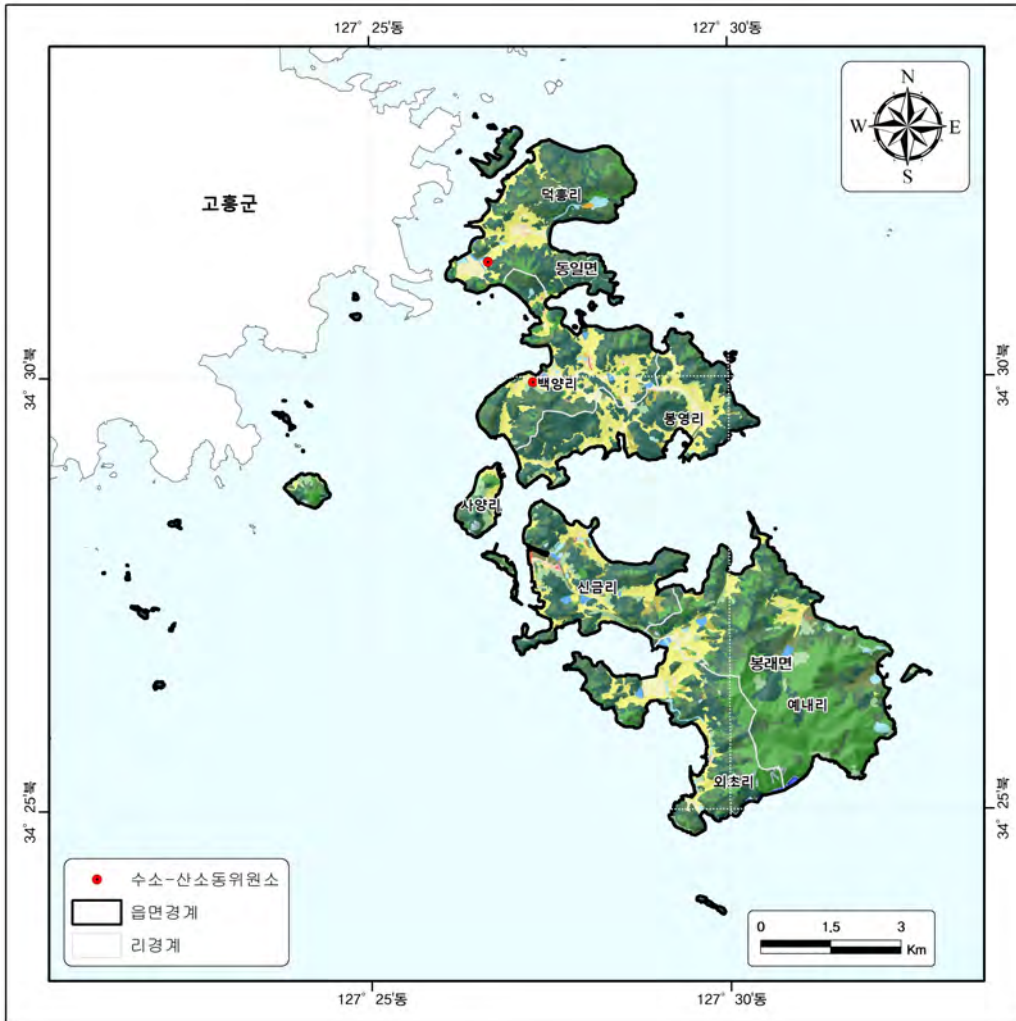
<그림 3-2-25> 고봉지구 지하수의 수소-산소동위원소 위치도
