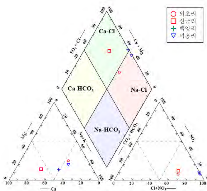
<그림 3-2-23> 고봉지구 지하수의 Piper Diagram
