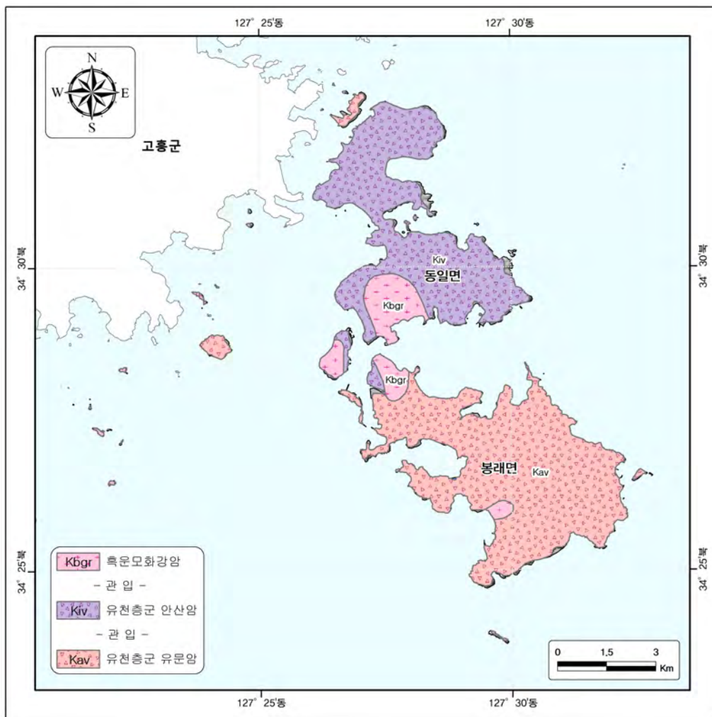
<그림 1-4-5> 고봉지구 지질도
