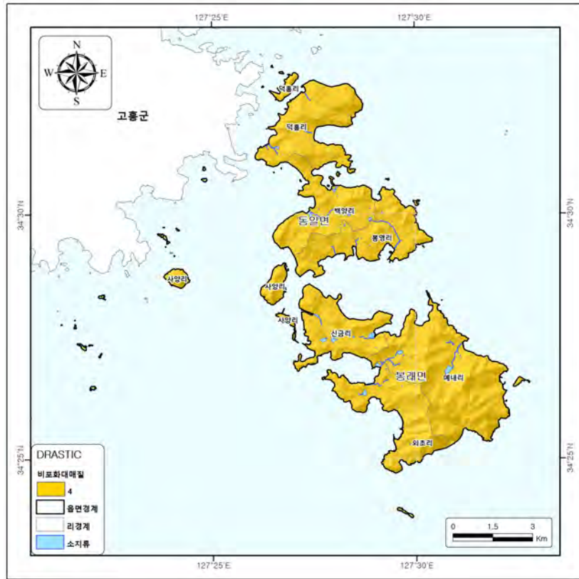
<그림 3-3-7> 비포화대 매질(Impact of Vadose Zone)
