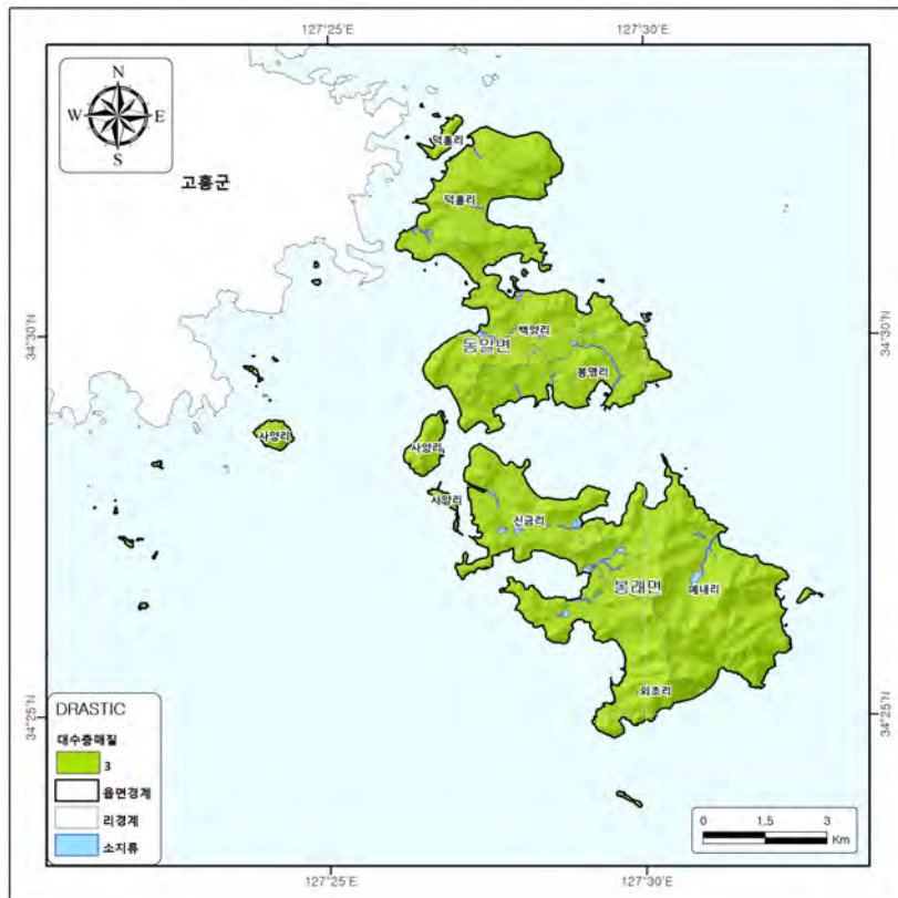
<그림 3-3-4> 대수층 매질(Aquifer Media)
