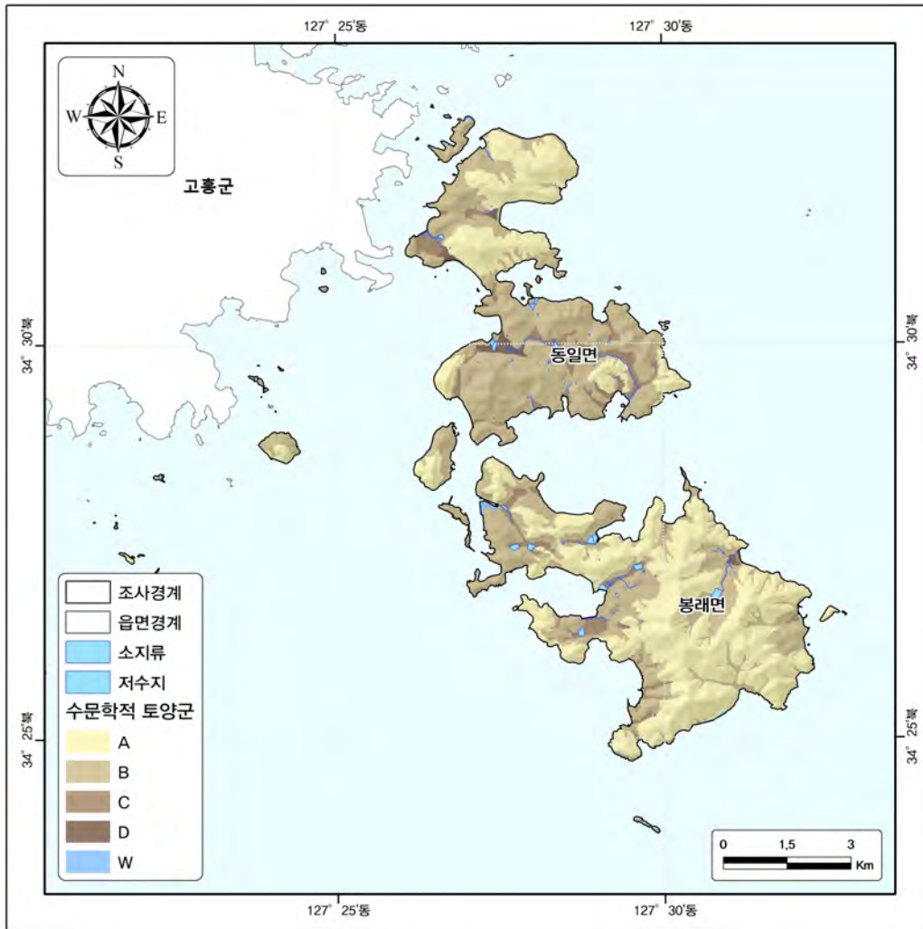
<그림 1-4-8> 고봉지구 NRCS 토양도
