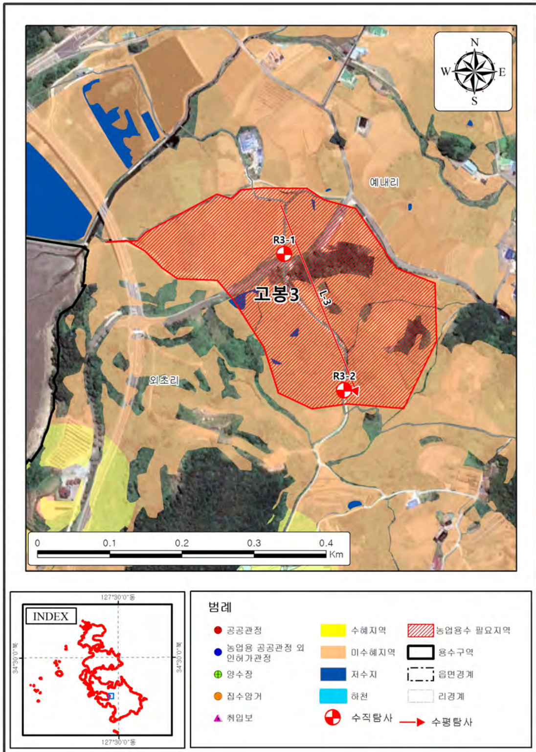
<그림 4-2-7> 물리탐사위치도 (고봉3)
