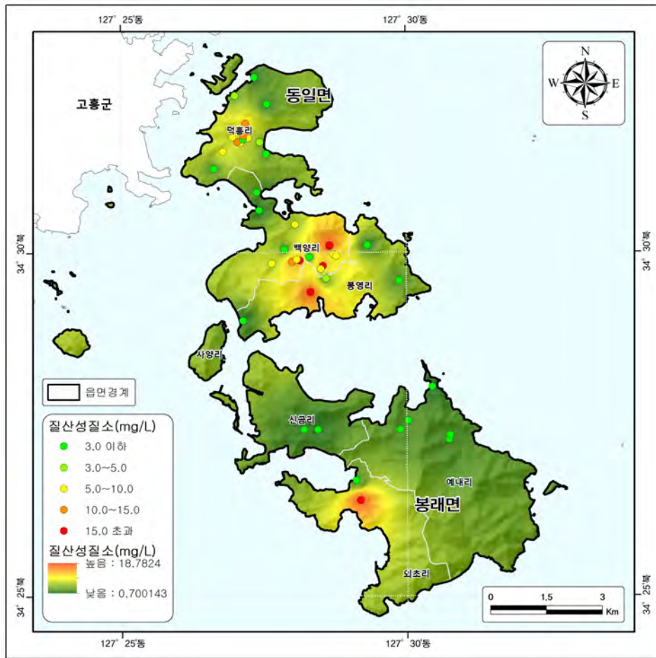
<그림 3-2-18> 고봉지구 지하수의 질산성질소(mg/L) 분포도
