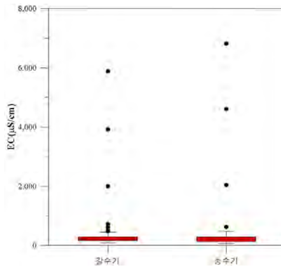
<그림 3-2-13> 고봉지구 지하수의 전기전도도(EC, \mu\text{S/cm} ) Box-whisker
