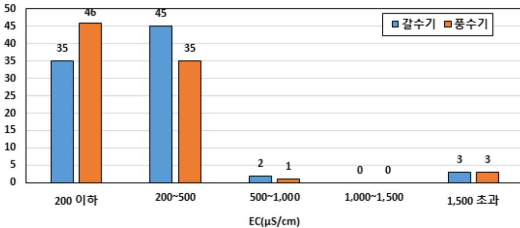
<그림 3-2-12> 고봉지구 지하수의 전기전도도(EC, \mu\text{S/cm} ) 빈도분포도
