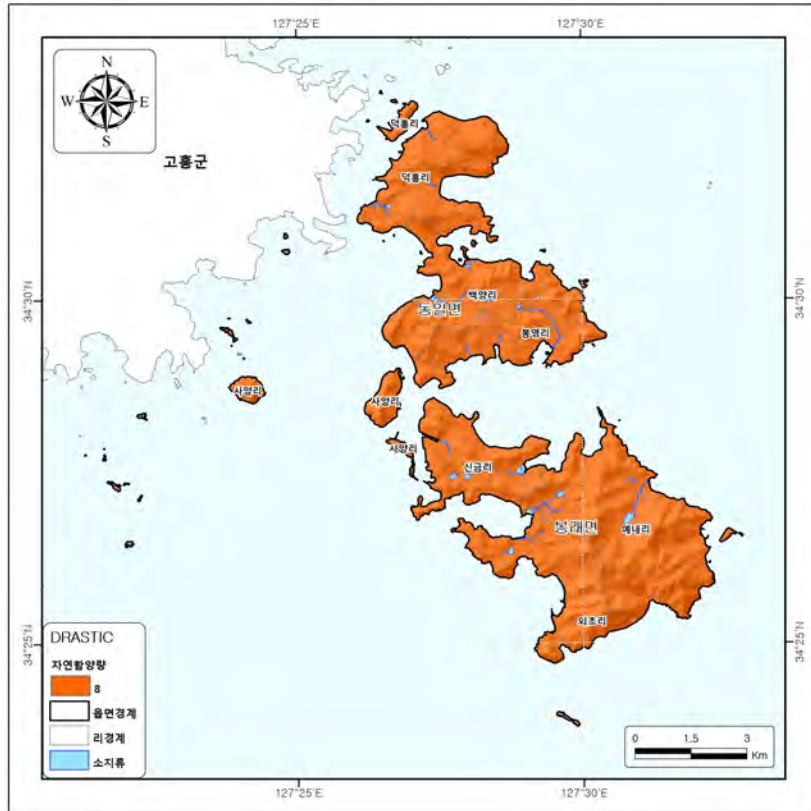
<그림 3-3-3> 자연함양량(Net Recharge)
