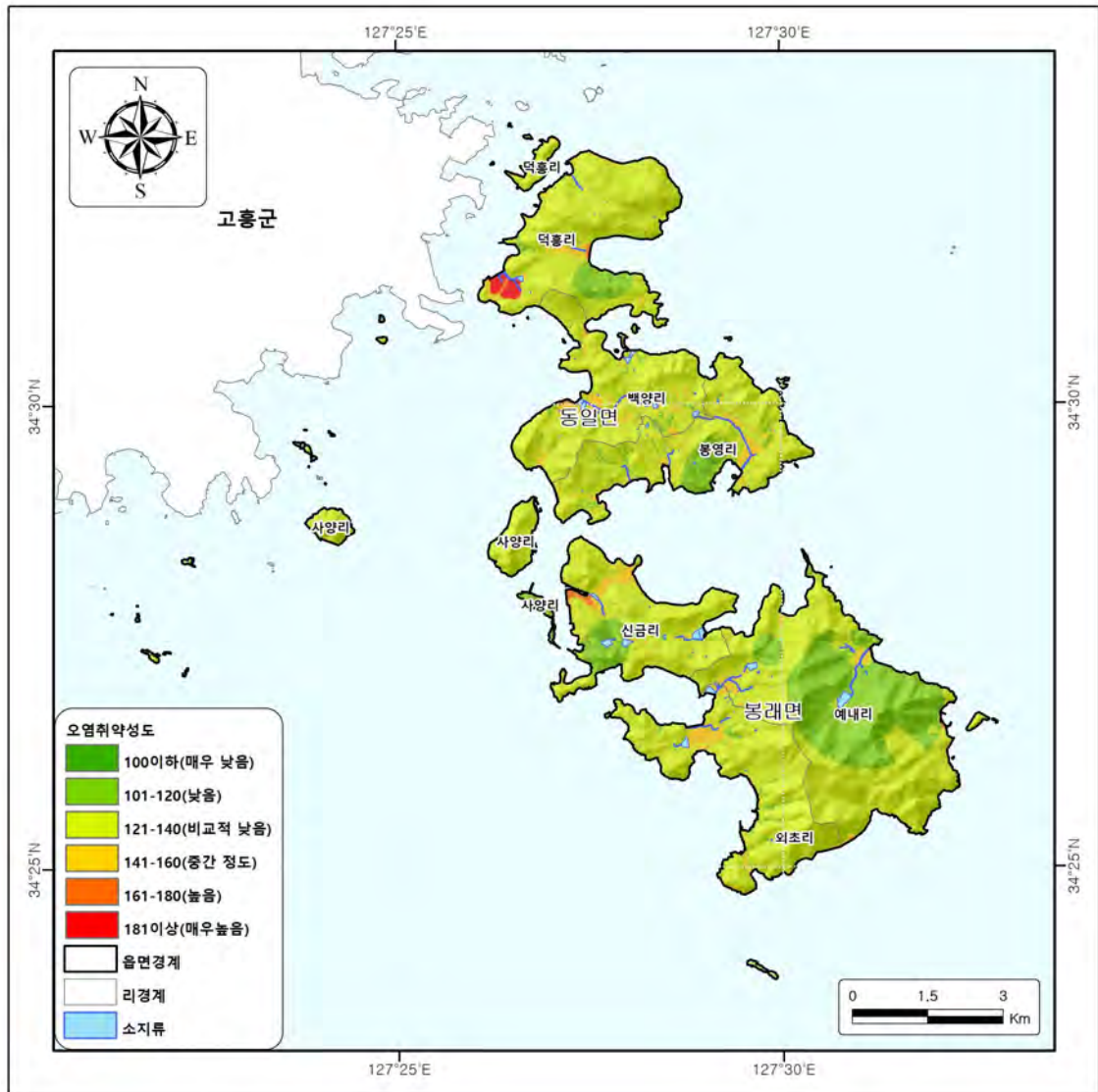
<그림 3-2-2> 고봉지구 DRASTIC INDEX Map
