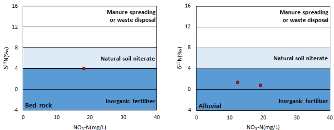
<그림 3-2-19> NO 3 -N과 \delta^{15}\text{N} 의 관계
