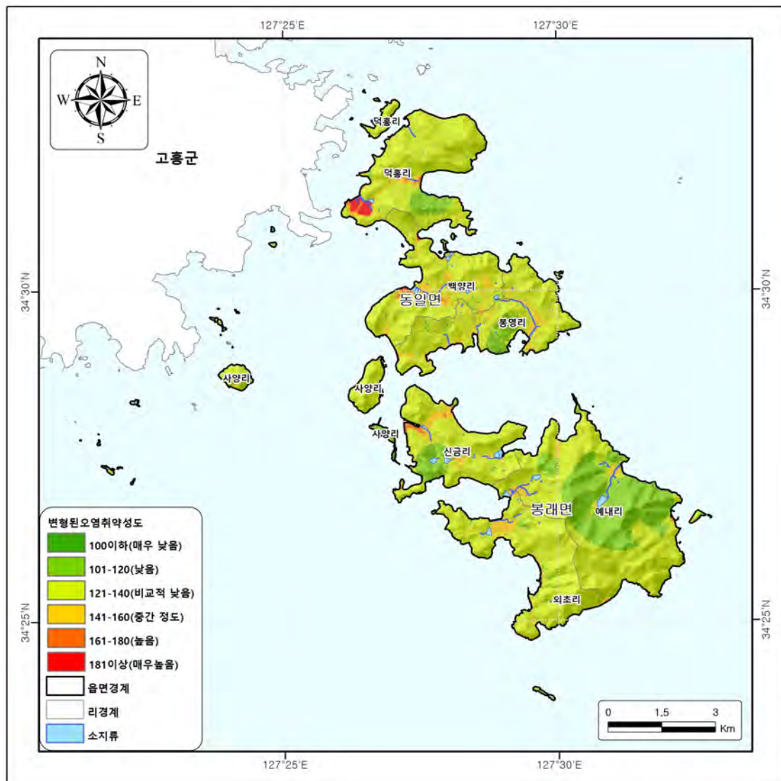
<그림 3-2-3> 고봉지구 Modified DRASTIC INDEX Map
