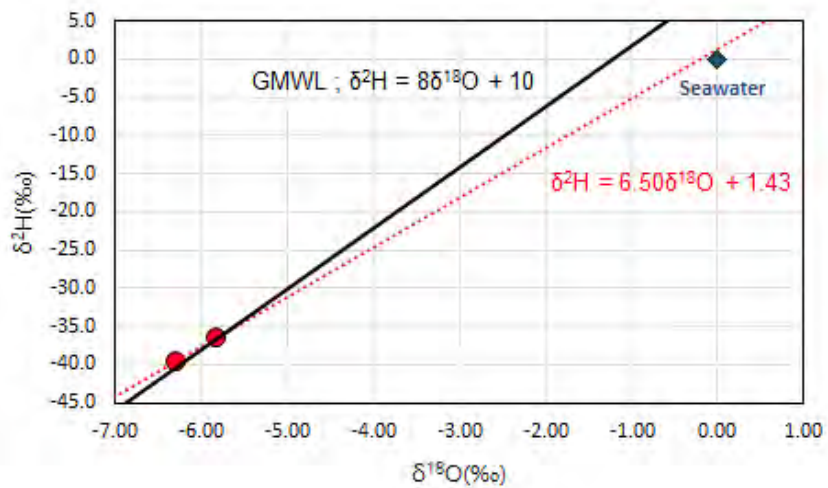
<그림 3-2-26> 수소-산소동위원소 분석결과와 순환수선과의 관계
