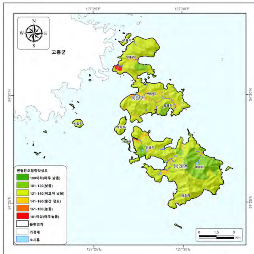
<그림 3-3-11> 고봉지구 변형된 오염취약성도(M-DRASTIC)
