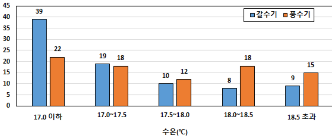
<그림 3-2-6> 고봉지구 지하수의 수온(T) 빈도분포도
