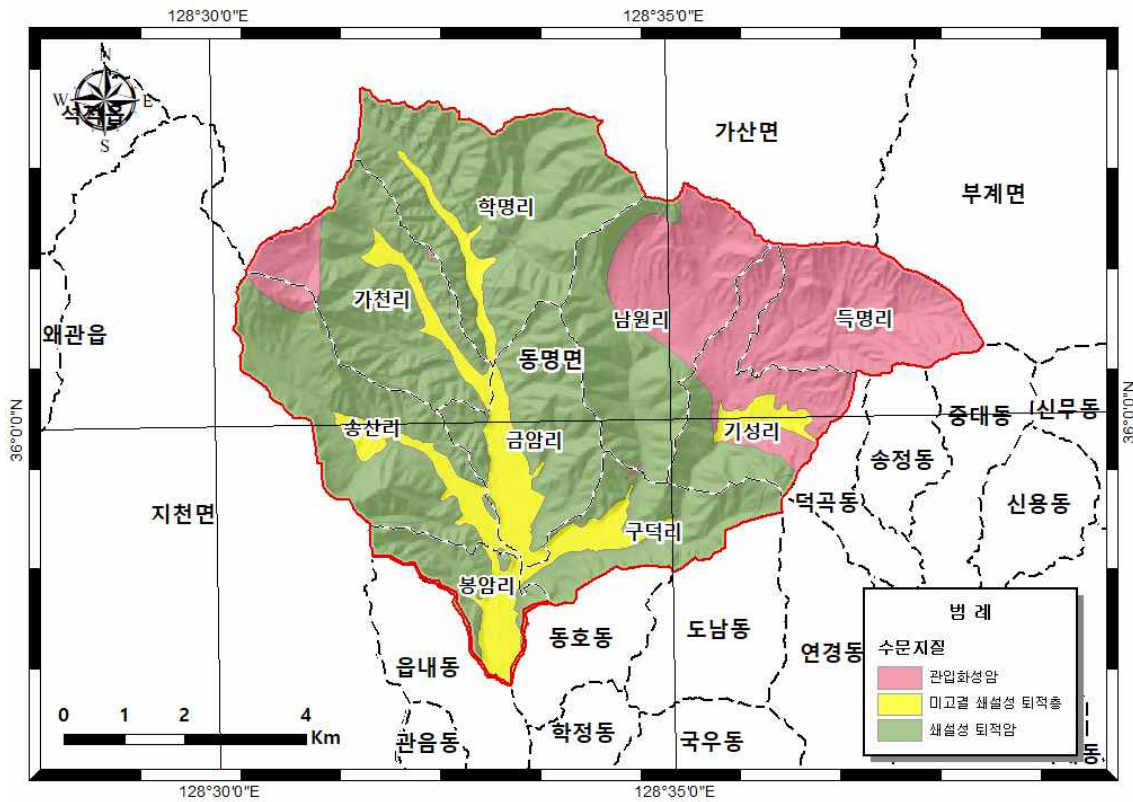
<그림 1-4-8> 칠동지구 수문지질도
