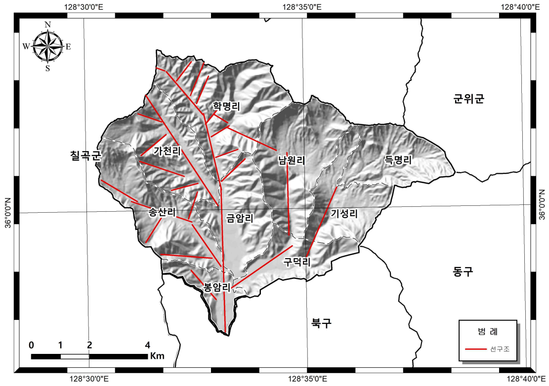
<그림 1-4-6> 선구조도
