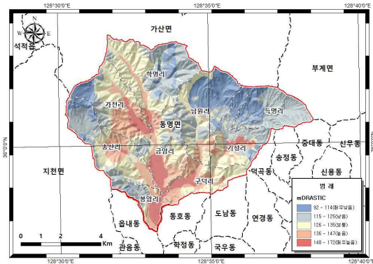
변형된 오염취약성도
