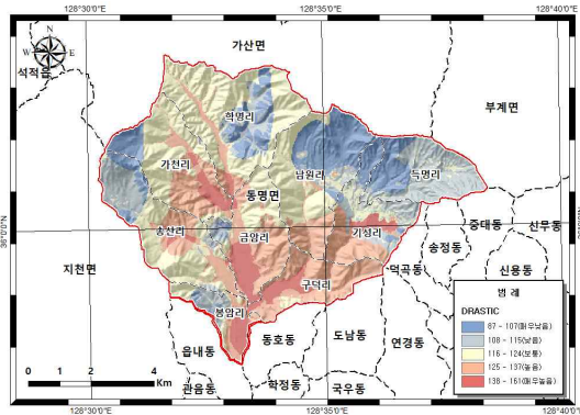
오염취약성도
