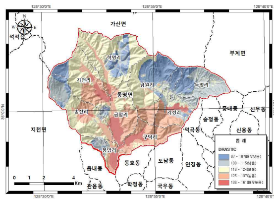
<그림 3-3-1> 칠동지구 Drastic Index Map
