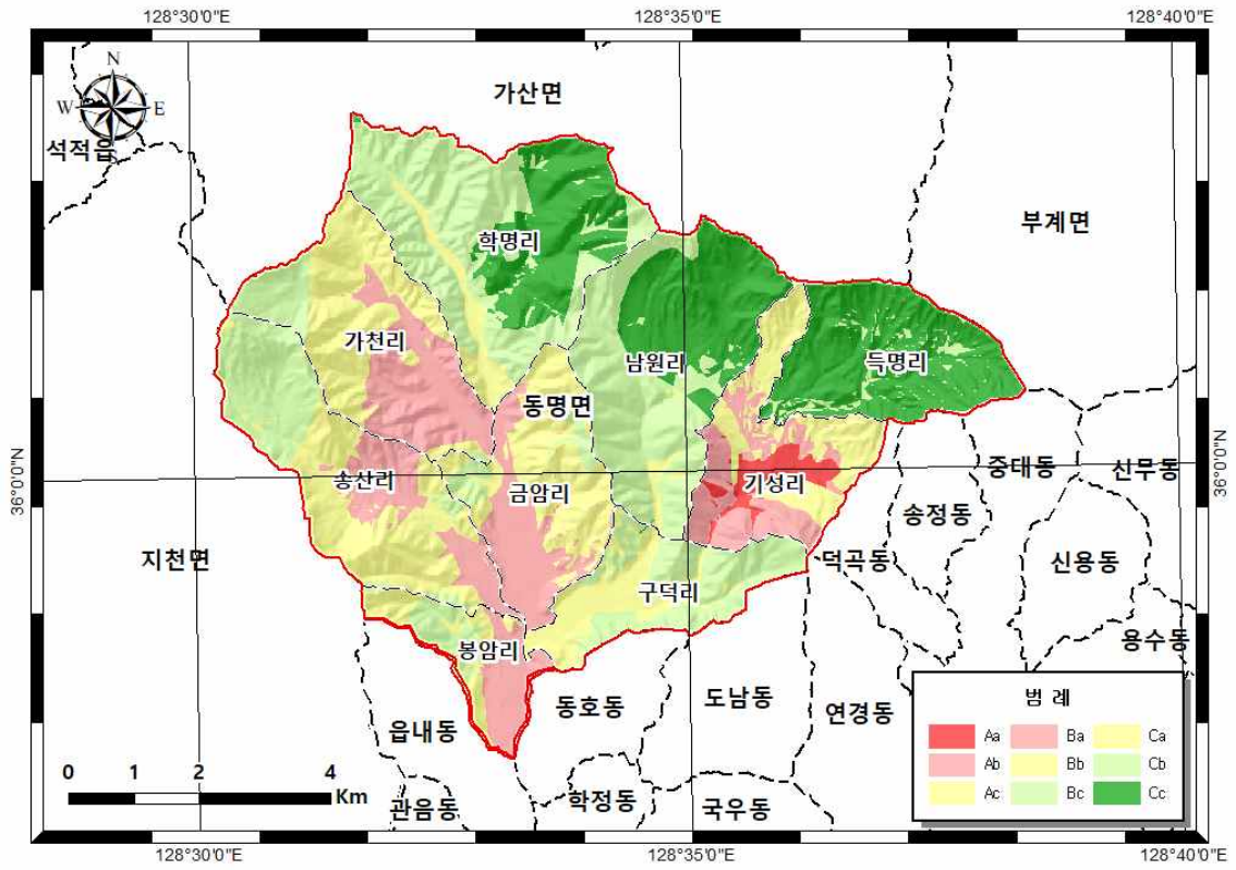
<그림 3-3-5> 지하수오염예측도
