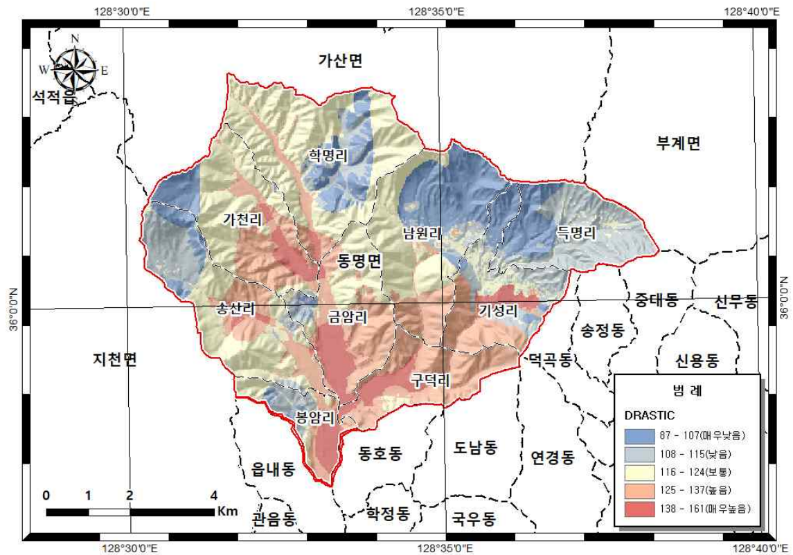
<그림 3-3-2> 오염취약성도
