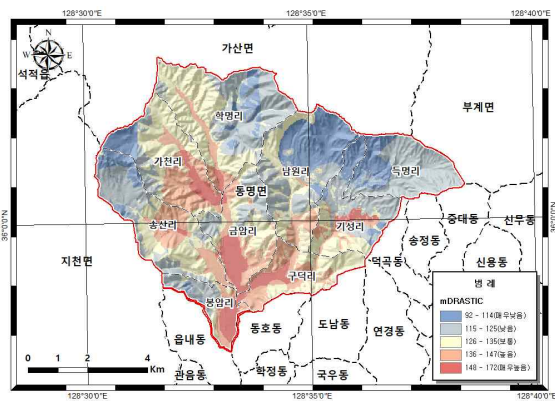
<그림 3-3-2> 칠동지구 Modified Drastic Index Map
